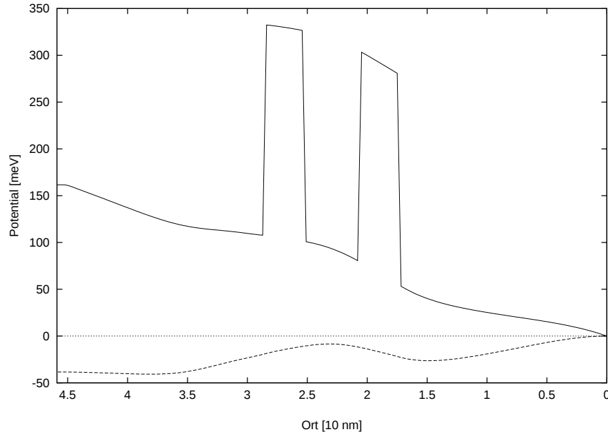
Abbildung 5.15: Selbstkonsistentes Potential bei einer externen Spannung von 220 mV entlang der Tunnel-diode. Die gestrichelte Linie ist der Beitrag des induzierten Potentials.
