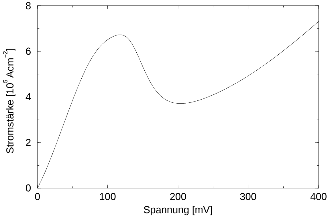
Abbildung 5.4: Berechnete Kennlinie einer resonanten Tunneldiode. Die Parameter der Barrierenstruktur entsprechen den in Abbildung 5.3 beschriebenen.
