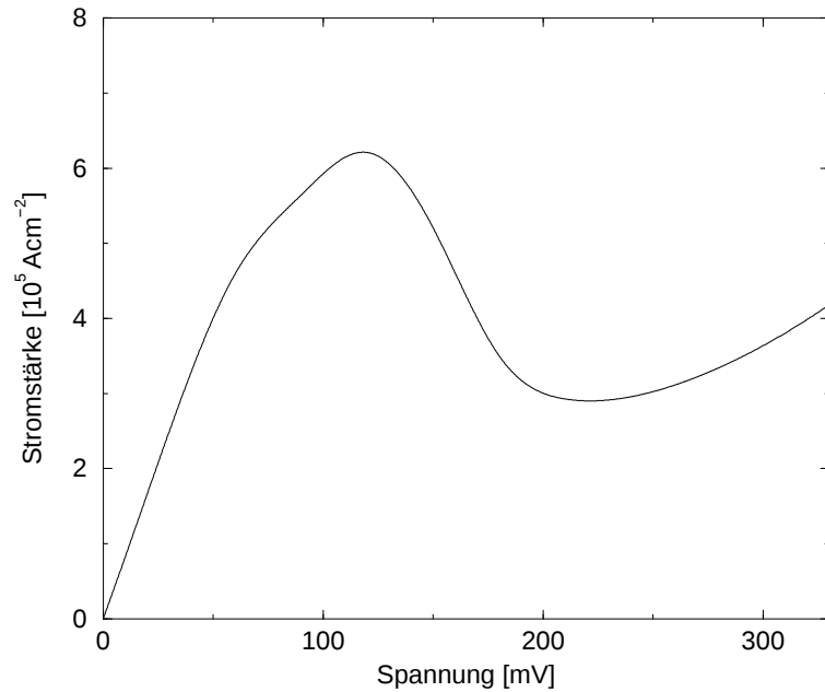
Abbildung 5.17: Kennlinie ohne Berücksichtigung von Selbstkonsistenzbedingungen. Die Parameter der Tunneldiode sind die gleichen wie für Abbildung 5.16.
