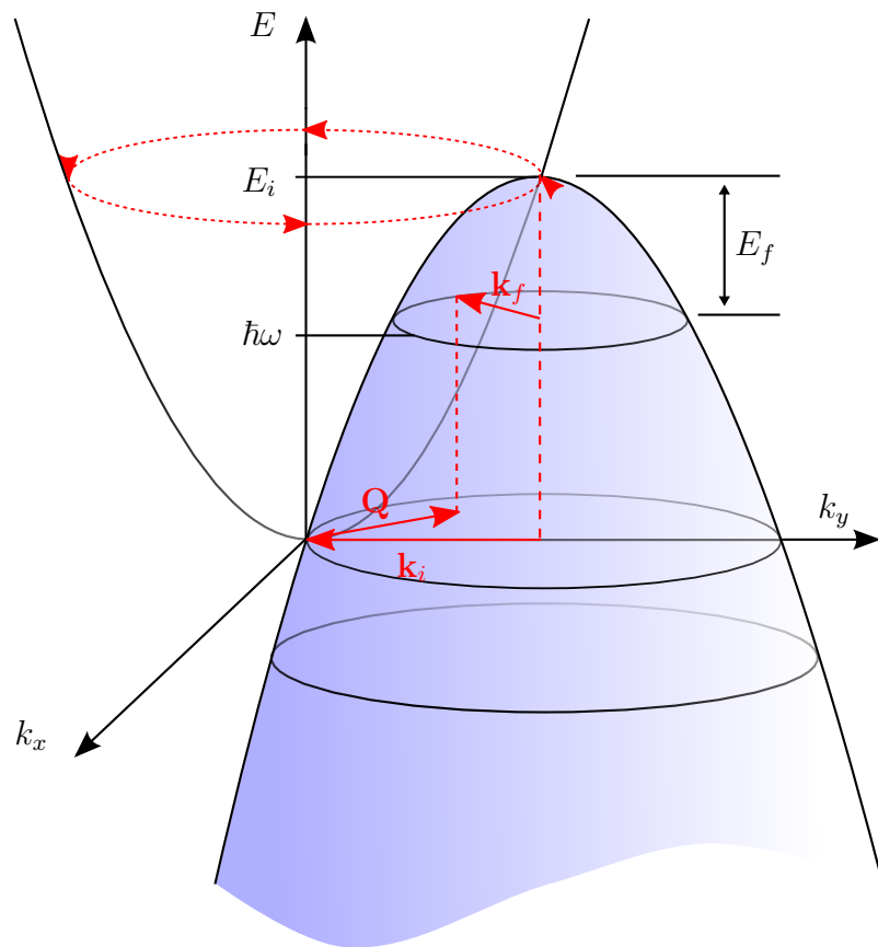
Abbildung 3.7: Schema zum Zusammenhang von Eingangs- ( E_i ), Ausgangsenergie E_f und \mathbf{k} . Die angedeutete Drehung des Paraboloiden entspricht dem Messvorgang am Flugzeitspektrometer ARCS.
