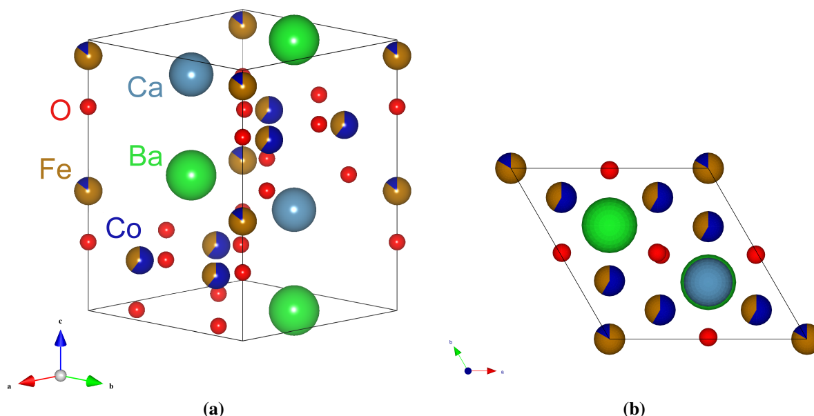
Abbildung E.1: Aus der Heidimessung ermittelte Elementarzelle von \text{CaBaCo}_2\text{Fe}_2\text{O}_7 . Die Tortendigramme geben die Besetzungswahrscheinlichkeiten an.
