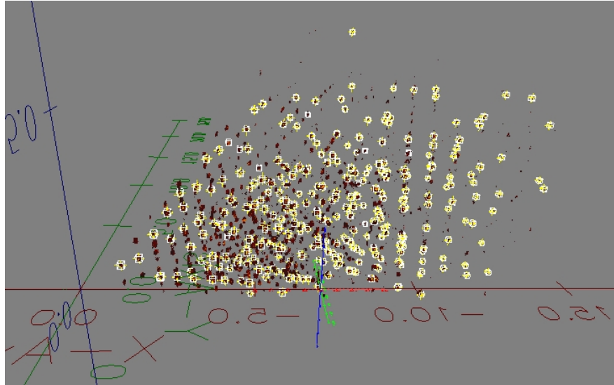
Abbildung 3.9: Darstellung der mit Isaw ausgewerteten Lauedaten. Rot sind die renormierten Messpunkte. Weiß markiert sind die gefundenen Peaks und gelb die mit der gefundenen Elementarzelle indizierten Peaks.
