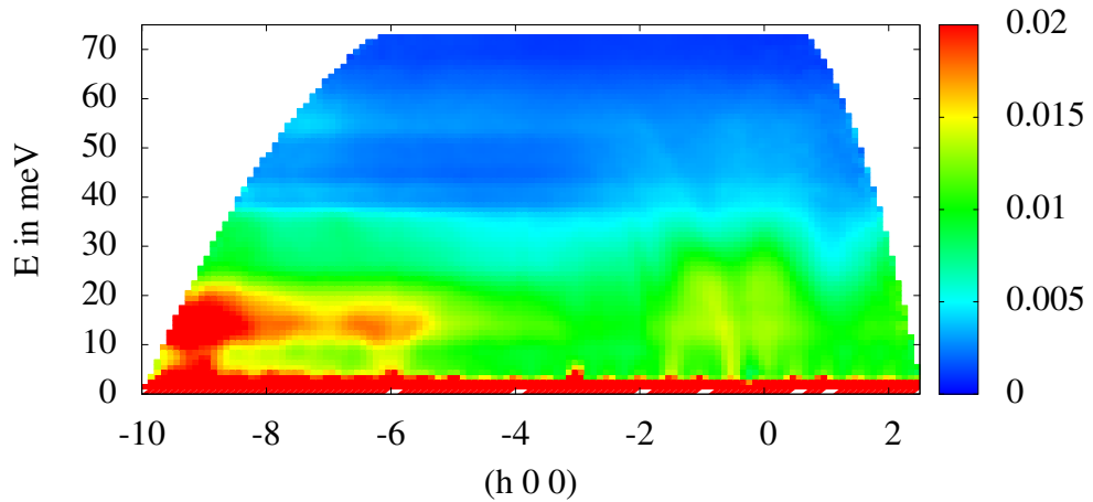
Abbildung 5.9: Anregungsspektrum in [1\ 0\ 0] -Richtung, bei vollständiger Integration in den dazu senkrechten Richtungen. Betrachtung möglicher Anregungswege und Intensität aus Phononenstreuung bei h < -6 . Aus der Messung des hk0 -Kristalls bei 5 K und 80 meV Eingangsenergie.
