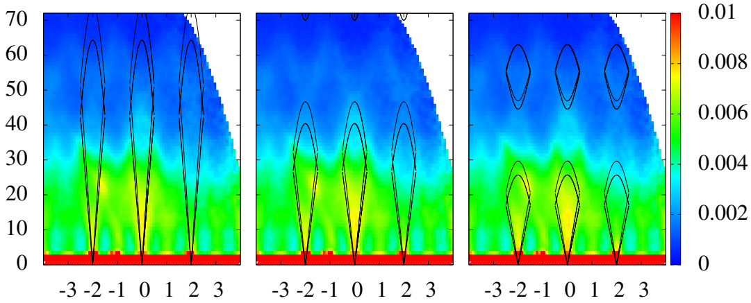
Abbildung 6.7: Anpassung der Moden in [001] -Richtung jeweils an das Anregungsspektrum aus Messung von ARCS am hhl-Kristall bei 5 K und einer Eingangsenergie von 80 meV. Mit den Skalierungsfaktoren J_1 = 35 meV (aus Panda), J_1 = 22 meV (Anpassung an die niederenergetischen Moden) und J_1 = 14 meV (Anpassung an die höherenergetischen Moden) (v.l.n.r.).
