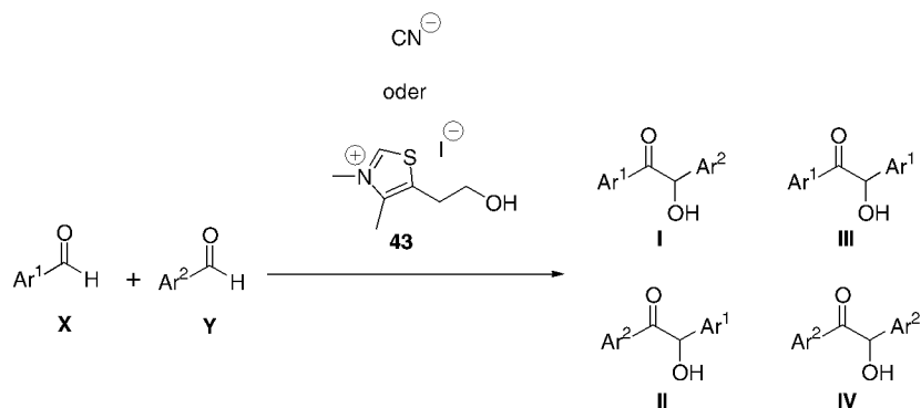
Abb. 3-35: Chemisch katalysierte Kreuzkupplung von Benzaldehyd-Derivaten.
