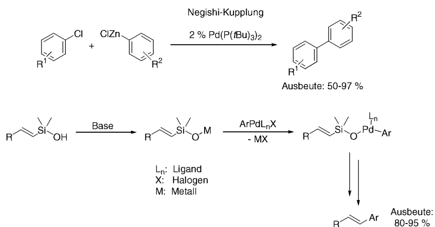
Abb. 1-2: Unter der Bezeichnung "Kreuzkupplung" publizierte Synthesen von Biarylen [4a] und Alkenen. [4b]
