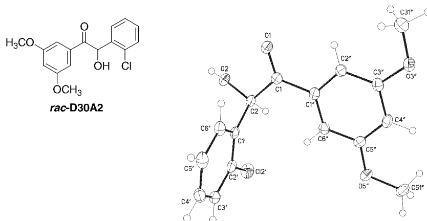
Abb. 3-38: Durch Röntgen-Kristallstrukturanalyse bestimmte Struktur des rac-D30A2 .
