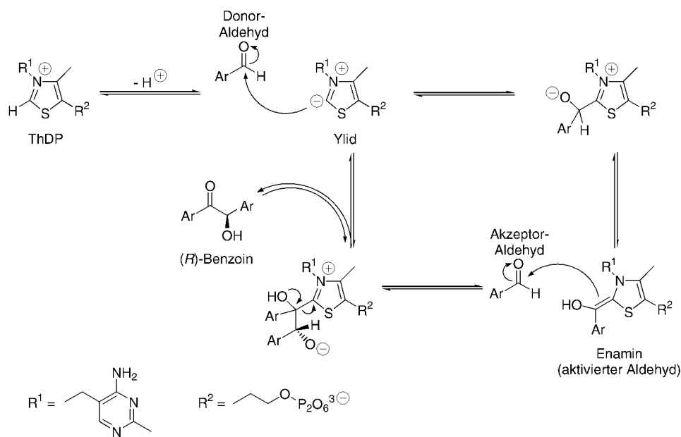
Abb. 2-16: Mechanismus der enzymatischen ThDP-katalysierten Benzoin-Kondensation. [52]
