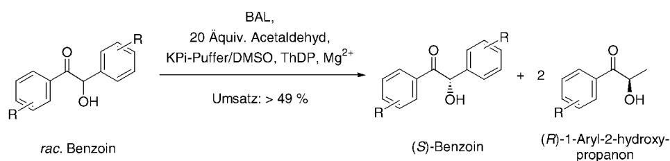
Abb. 2-18: Kinetische Racematspaltung durch C-C-Bindungsspaltung mittels BAL. [50]
