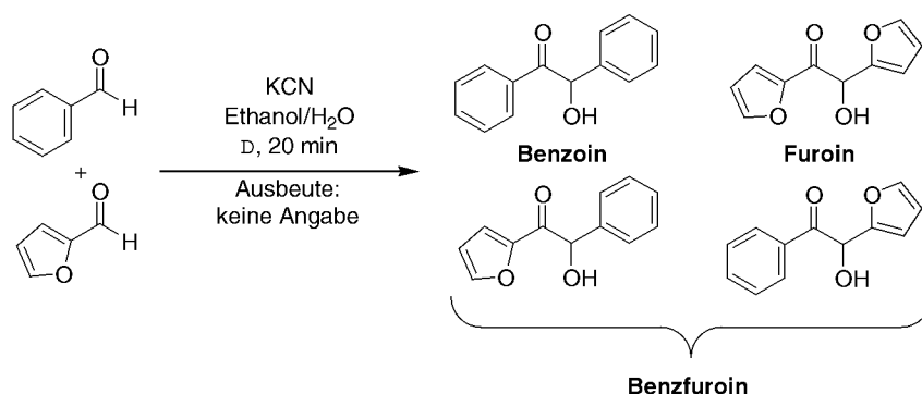
Abb. 2-1: Erste publizierte Kreuz-Benzoin-Kondensation nach E. Fischer . [7]
