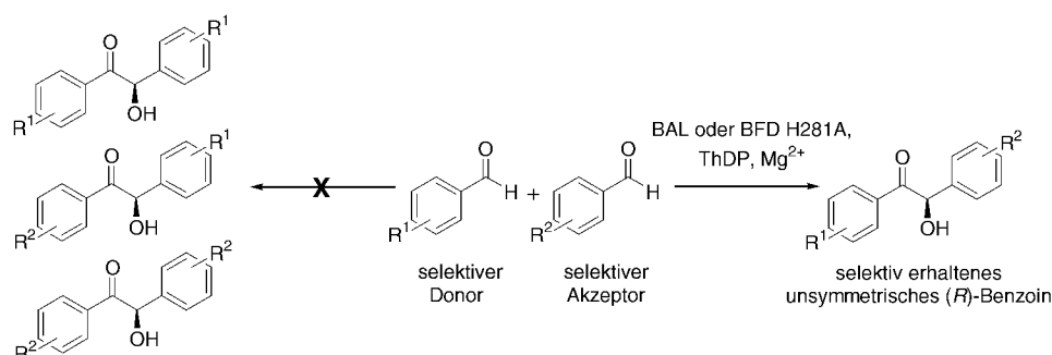
Abb. 4-1: Schematische Darstellung des Donor/Akzeptor-Konzeptes.
