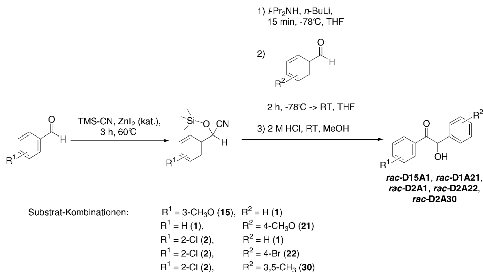
Abb. 3-37: Synthese-Schema für die Generierung der racemischen, gemischten Benzoine rac-D15A1 , rac-D1A21 , rac-D2A1 , rac-D2A22 und rac-D2A30 . [14a,b]
