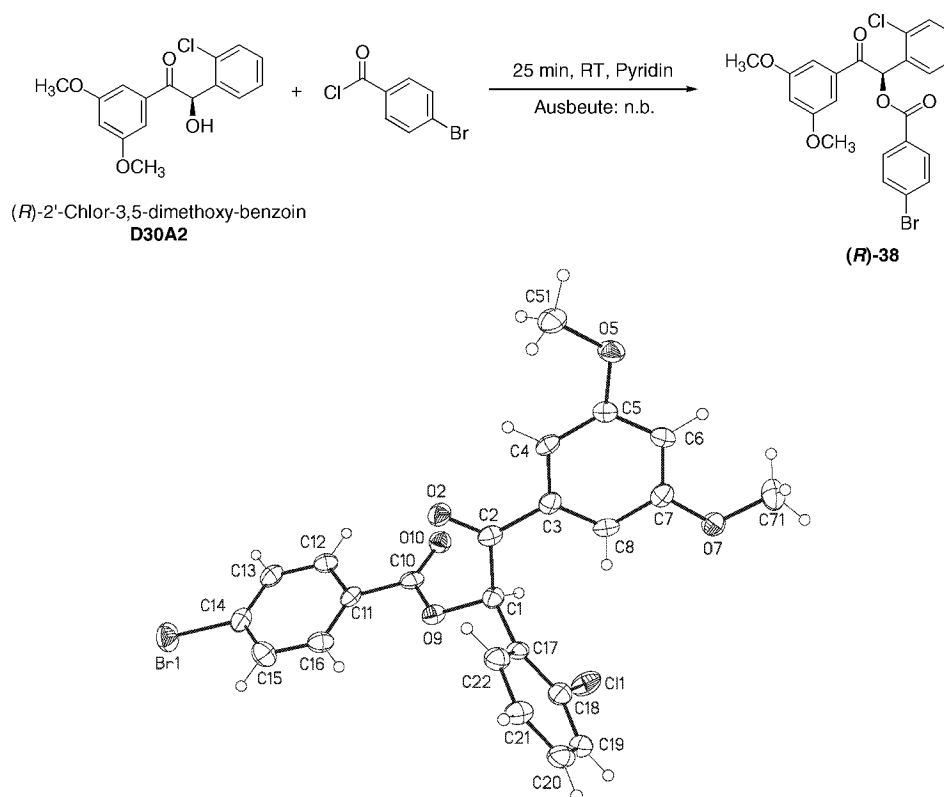
Abb. 3-19: Syntheschema und Struktur des Benzoin-Derivates ( R )- 38 .
