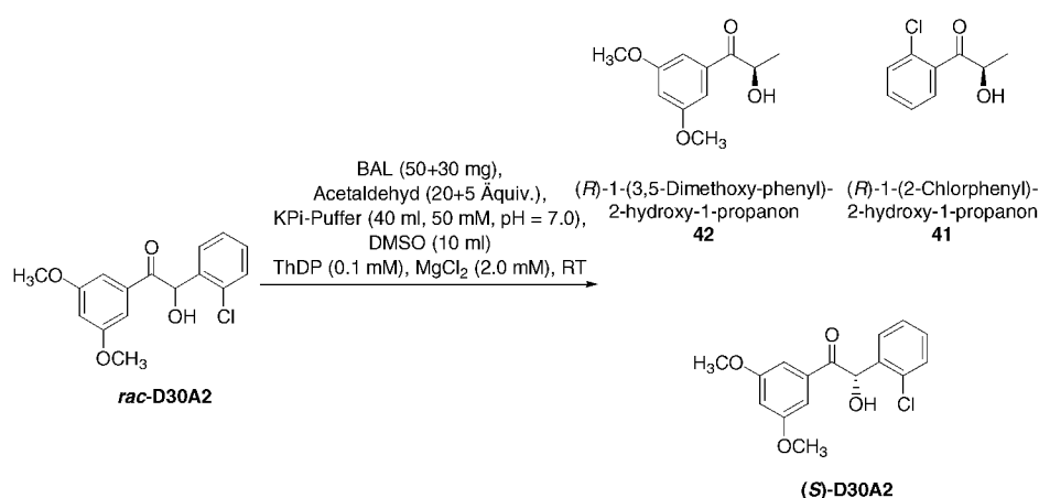
Abb. 3-28: Synthese von ( S )-2'-Chlor-3,5-dimethoxy-benzoin (( S )- D30A2 ) durch Racematspaltung.
