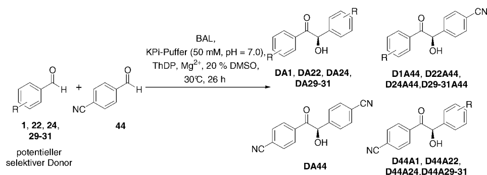
Abb. 3-40: Schematische Darstellung der Umsetzung von 4-Cyanbenzaldehyd ( 44 ) mit potentiell selektiven Donor-Aldehyden katalysiert durch BAL.
