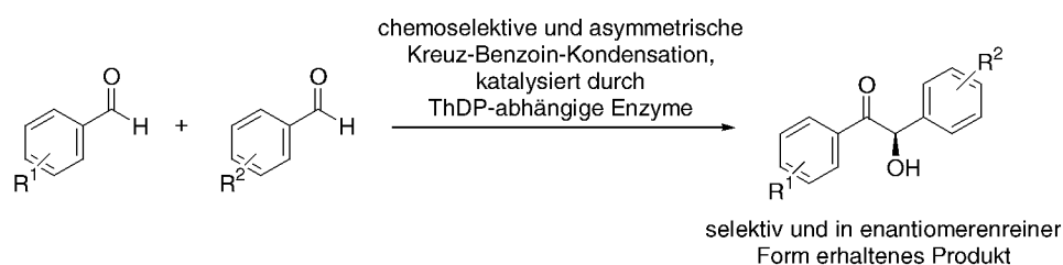
Abb. 1-3: Schematische Darstellung der Zielsetzung des Promotionsvorhabens.
