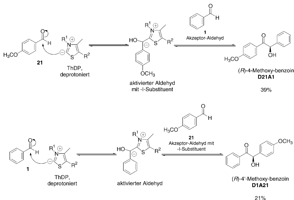
Abb. 3-33: Bildung der beiden unsymmetrischen (R)-Benzoine D21A1 und D1A21 .
