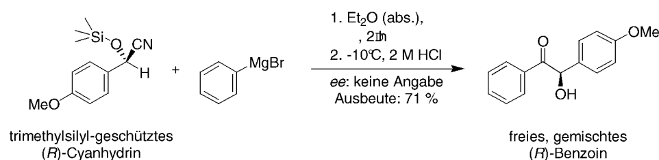
Abb. 2-7: Asymmetrische, chemische Synthese eines gemischten Benzoins. [17a]
