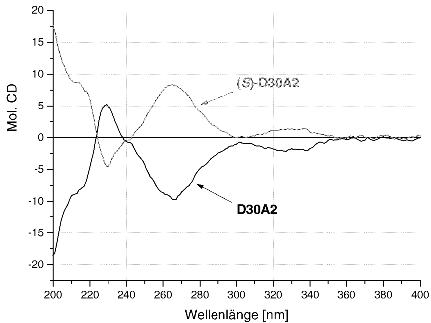
Abb. 3-30: CD-Kurven der beiden Enantiomere von 2'-Chlor-3,5-dimethoxy-benzoin (D30A2 und (S)-D30A2) gemessen in Acetonitril.
