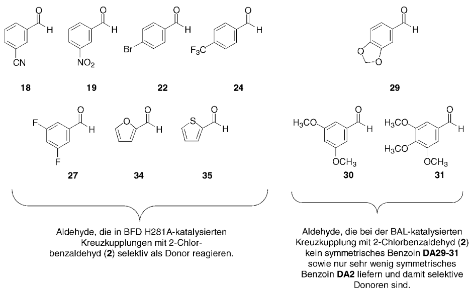
Abb. 3-8: Graphische Zusammenfassung des Donor-Screenings
