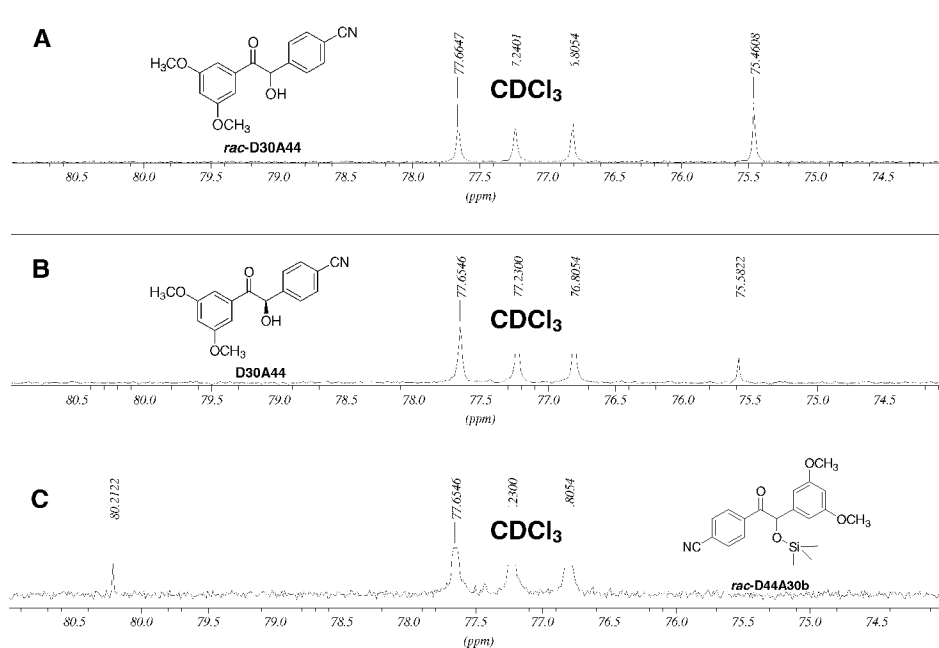
Abb. 3-42: Ausschnitte aus den 13 C-NMR-Spektren der Verbindungen rac -D30A44 (A), D30A44 (B) und rac -D44A30b (C). Gezeigt sind die chemischen Verschiebungen der Carbinol-Kohlenstoff-Atome.
