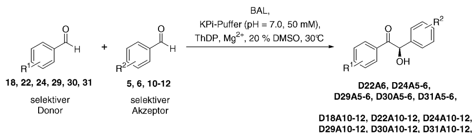
Abb. 3-9a: Schematische Darstellung des permutativen Screenings.
