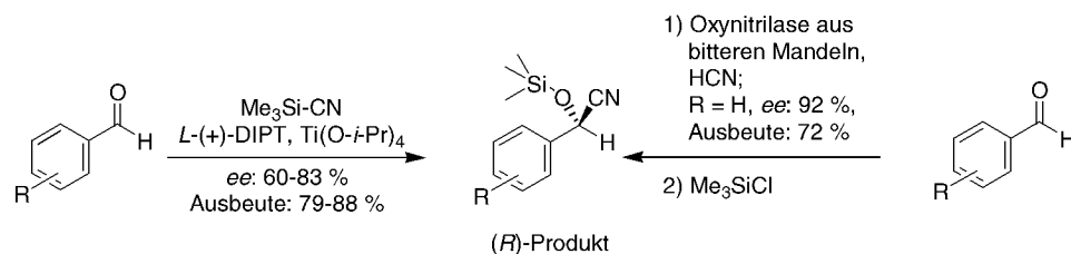
Abb. 2-8: Asymmetrische Synthese von trimethylsilyl-geschützten Cyanhydrinen. [35,36]
