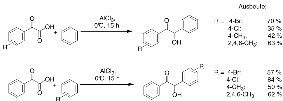
Abb. 2-10: Synthese beider Isomere von gemischten Benzoinen durch Umsetzung von Phenylglyoxalen mit Benzen-Derivaten. [38b]
