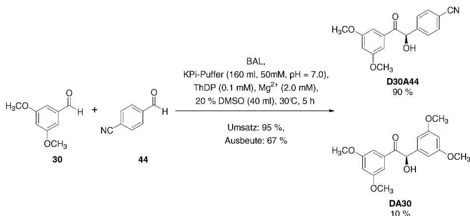
Abb. 3-41: Synthese von ( R )-4'-Cyan-3,5-dimethoxy-benzoin ( D30A44 ) im präparativen Maßstab.
