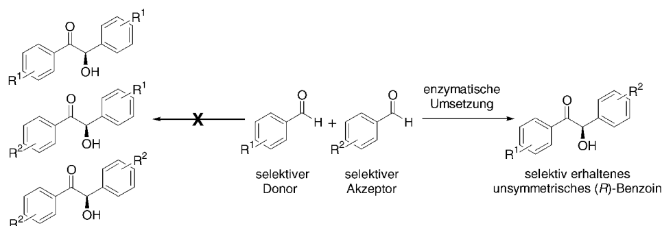
Abb. 3-1: Schematische Darstellung des enzymatischen Donor/Akzeptor-Konzeptes.
