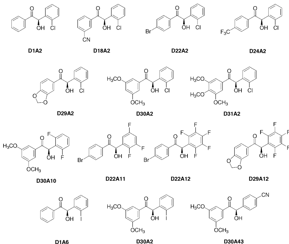
Abb. 4-2: Durch enzymatische Kreuz-Benzoin-Kondensation im präparativen Maßstab erhaltene unsymmetrische ( R )-Benzoinen.
