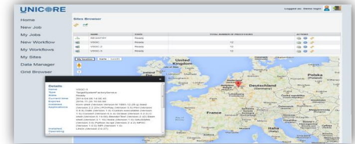
Web portal
