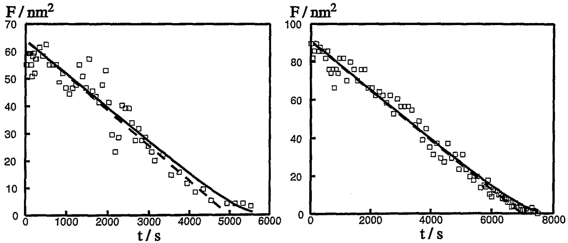
Abbildung 4.12: Leerstelleninselzerfall: Radius als Funktion der Zeit.
