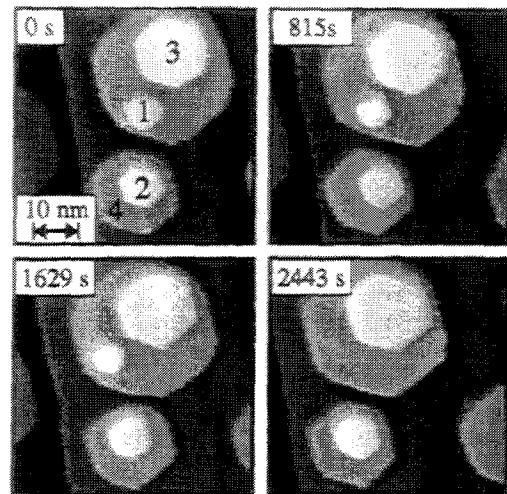
Abbildung 4.10: Stufenbarriere: Die Insel '1' mit aufsteigender Stufenkante '3' als Adatomsenke; Insel '2' mit absteigender Stufenkante '4' als Adatomsenke; U_t = -0,79 V, I_t = 0,29 nA, T = 277 K bis 279 K.
