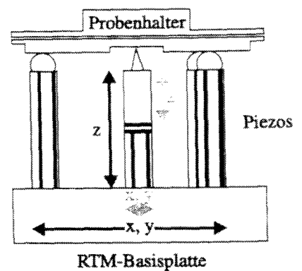
Abbildung 2.1: Beetle-RTM: Prinzipieller Aufbau; schwarz: Auslenkungen im klassischen Betrieb; grau: im modifizierten Betrieb.
