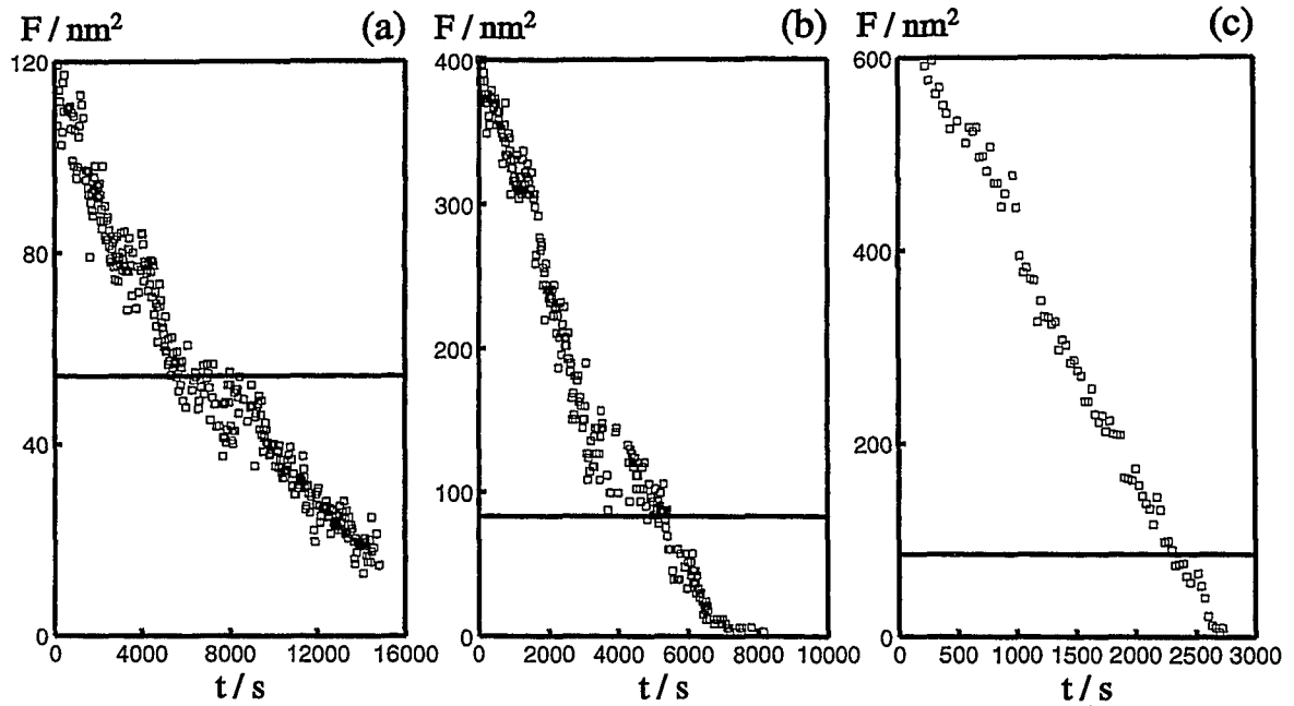
Abbildung 4.13: Leerstelleninselzerfall: Fläche als Funktion der Zeit: (a) 320 K bis 308 K (b) 339 K bis 329 K (c) 358 K bis 351 K; Querlinie markiert die Grenze der Gültigkeit der Näherungen der LSW-Theorie.
