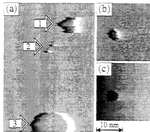
Abbildung 2.3: Aufnahmemoden: (a) klassischer Modus, Aufnahmezeit t_i = 2,4 min; U_t = -0,5 V, I_t = 10 nA, RT; (b) klassischer Modus, t_i = 160 s, U_t = -0,5 V, I_t = 5 nA, RT; (c) modifizierter Modus, t_i = 16 s, U_t = -0,5 V, I_t = 5 nA, RT.
