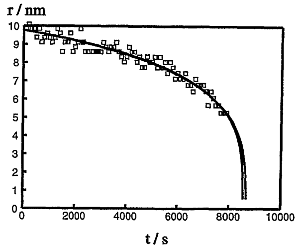
Abbildung 4.7: Ostwald-Reifung: Radius als Funktion der Zeit von Insel '6' und integrierte Kurven.
