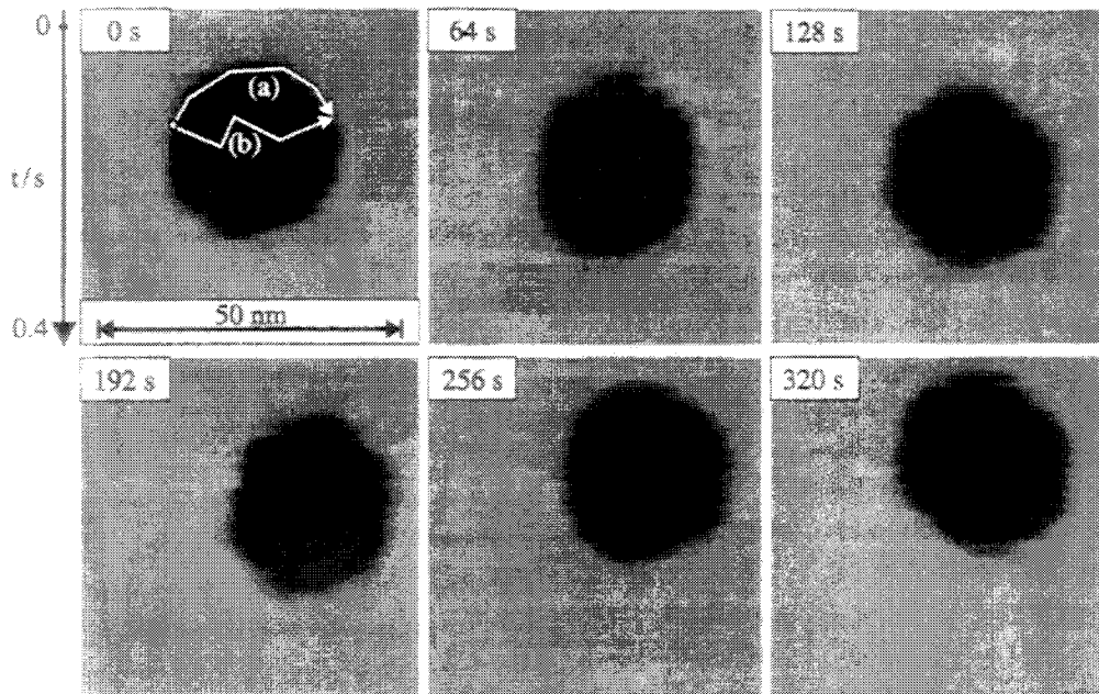
Abbildung 3.5: Randfluktuation einer Leerstelleninsel: denkbare atomare Mechanismen des Massentransportes sind eingezeichnet; I_t = 10 \text{ nA} , U_t = -0.5 \text{ V} , RT.
