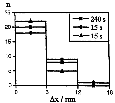
Abbildung 3.8: Einfluß des Meßprozesses: Positive Hälfte der Verschiebungsverteilung zweier Leerstelleninseln mit d = 11 nm, \Delta t = 240 s; Aufnahmezeit: 12 s/Bild.
