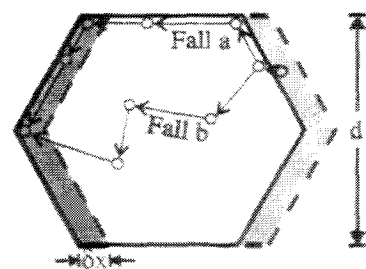
Abbildung 3.1: Inselbewegung: Skizze einer Leerstelleninsel der linearen Ausdehnung d , die sich in \delta t um \delta x nach rechts bewegt, und möglicherweise zugrundeliegende Adatombewegungen.
