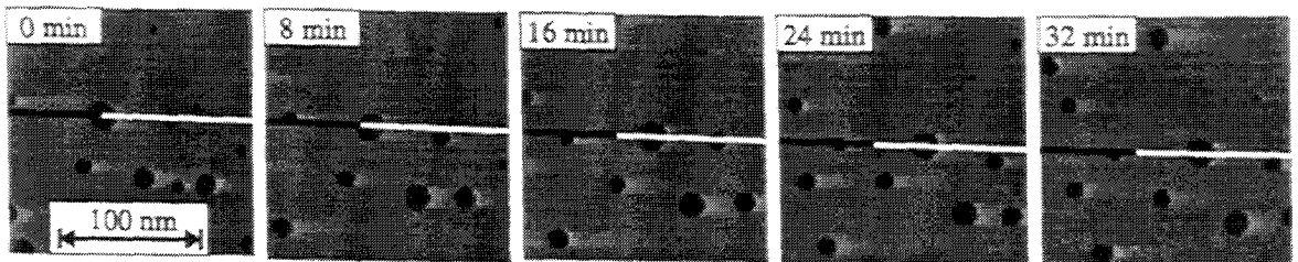
Abbildung 2.5: Thermische Verschiebung: Die Linie markiert den Massenschwerpunkt der größten Leerstelleninsel; der schwarze Teil hat dieselbe Länge auf allen Bildern; U_t = -0,5 \text{ V} , I_t = 5 \text{ nA} , RT.
