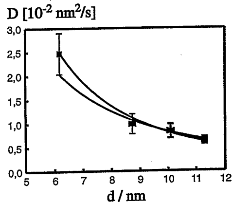
Abbildung 3.14: Adatominselbewegung: Diffusionskonstante als Funktion des Inseldurchmessers für den Temperaturbereich 279 K bis 286 K.
