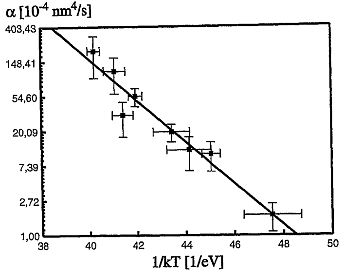
Abbildung 3.15: Adatominselbewegung: Arrhenius-Auftragung des Vorfaktor \alpha_\beta(T) über der Temperatur und berechnete Gerade.
