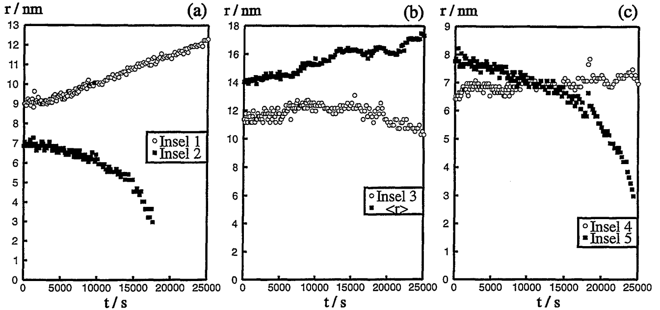
Abbildung 4.6: Ostwald-Reifung: Inselradien und mittlerer Radius als Funktion der Zeit.
