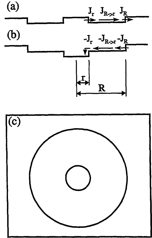
Abbildung 4.1: Schematische Darstellung mehrlagiger Systeme (a) Adatominsel in Leerstelleninsel (b) Leerstelleninsel in Leerstelleninsel (c) Aufsicht (identisch für (a) und (b)); und Flüsse, die den Zerfall der inneren Insel in einer Kontinuumsstheorie beschreiben.
