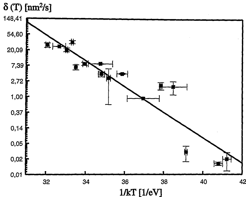
Abbildung 4.14: Leerstelleninselzerfall: Arrhenius-Darstellung von \delta(T) .
