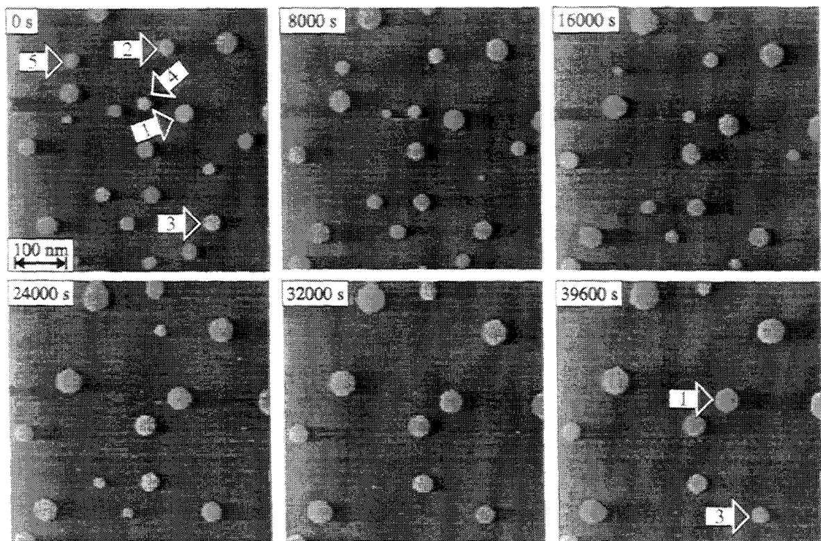
Abbildung 4.8: Ostwald-Reifung: \phi = 0,08 ; I_t = 3 \text{ nA} , U_t = -0,5 \text{ V} .
