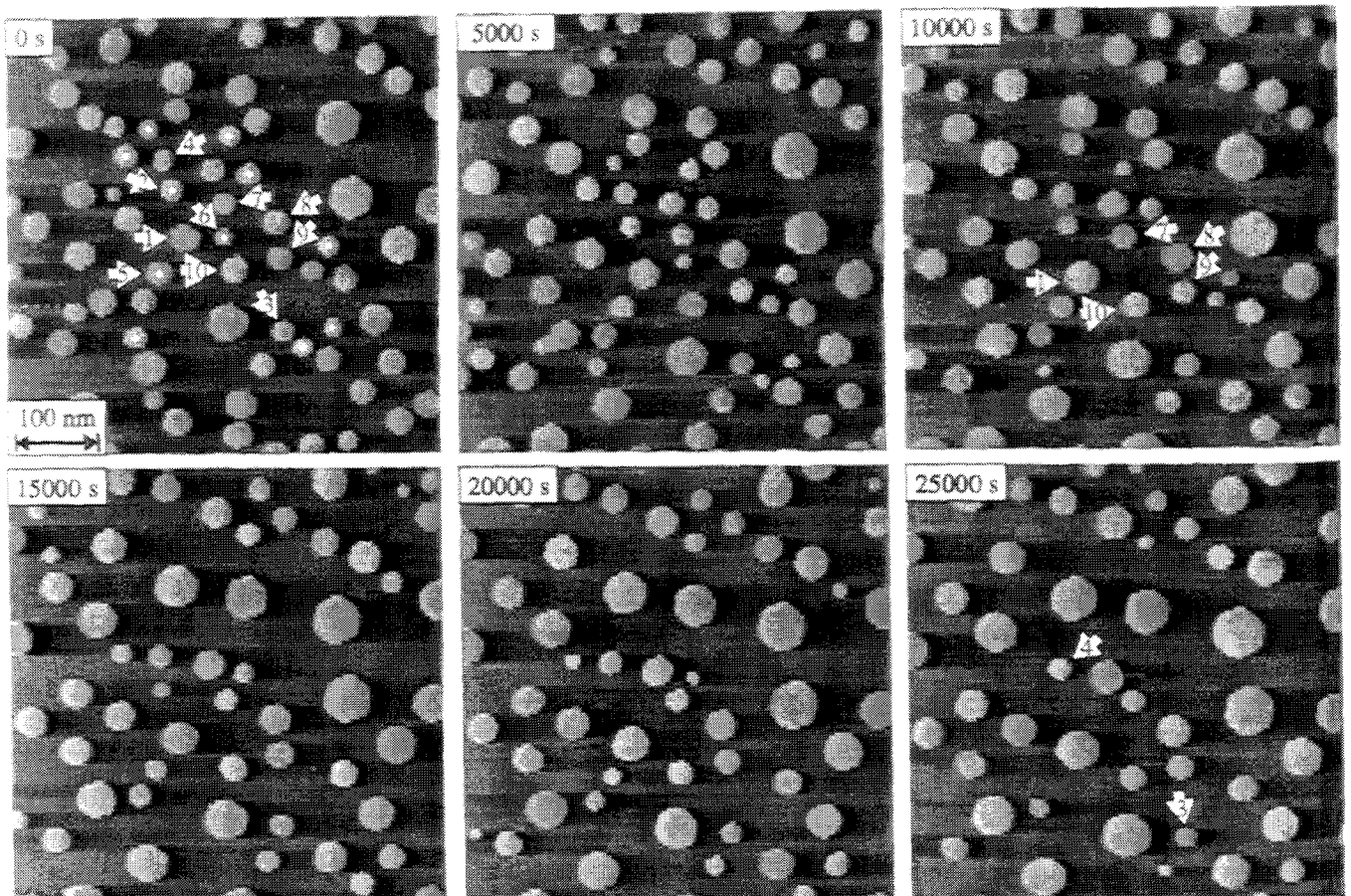
Abbildung 4.5: Ostwald-Reifung: \phi = 0,21 , I_t = 3 \text{ nA} , U_t = -0,5 \text{ V} , RT.
