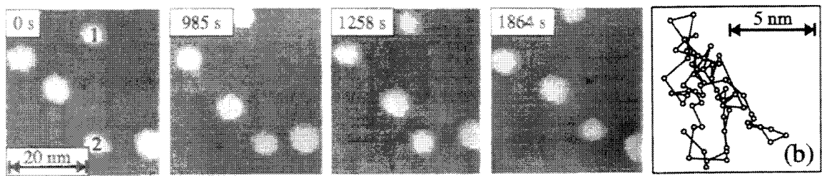
Abbildung 3.10: Bewegung von Adatominseln: U_t = -2,09 \text{ V} , I_t = 0,09 \text{ nA} , 263 K bis 266 K; (b) relative Bewegung der Inseln '1' und '2'.
