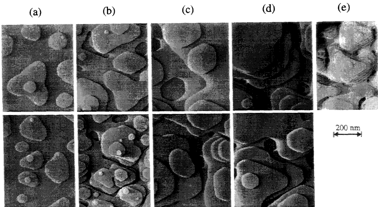
Abbildung A.1: Dreidimensionales Wachstum: Je zwei Beispiele für verschiedene Bedeckungen; Depositionsrate; Bedeckung; I_t ; U_t : (a) 0,32 ML/min; 0,42 ML; 3 nA, -0,6 V; 7,2 nA, -0,6 V (b) 0,80 ML/min; 1,5 ML; 2 nA, -1 V; 5 nA, -1 V (c) 0,53 ML/min; 2,1 ML; 3 nA, -1 V; 2 nA, -1V (d) 0,40 ML/min; 3,8 ML; 2 nA, -0,6 V; 3 nA, -0,6 V (e) 0,35 ML/min; 6,6 ML. 0,3 nA; -1 V.
