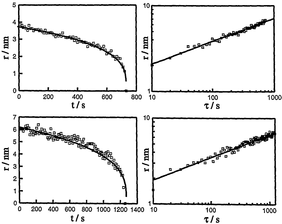
Abbildung 4.3: Adatominselzerfall: Radius als Funktion der Zeit und doppeltlogarithmische Darstellung; offene Quadrate: experimentelle Daten; Linien: berechnete Kurven.
