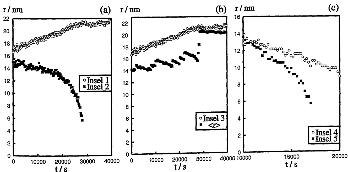
Abbildung 4.9: Ostwald-Reifung: Inselradien und mittlerer Radius als Funktion der Zeit.
