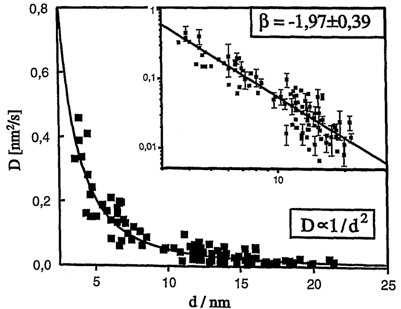
Abbildung 3.7: Leerstelleninseldiffusionskonstante als Funktion der Leerstelleninselgröße; Einschub: doppeltlogarithmische Darstellung; d^{-2} -Kurven sind eingezeichnet.
