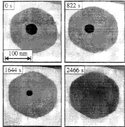
Abbildung 4.11: Zweilagige Leerstelleninsel: erzeugt durch zweimaligen \text{Ne}^+ -Ionenbeschuß, 30 s bei 370 K und 5 s bei 300 K, und Zerfall der inneren Leerstelleninsel bei 350 K, I_t = 1 \text{ nA} , U_t = 2 \text{ V} .
