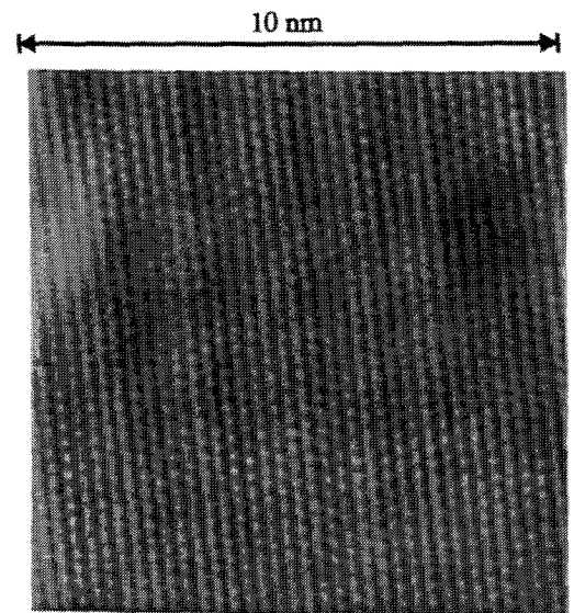
Abbildung 2.2: Ag(111)-Fläche in atomarer Auflösung; I_t = 5 \text{ nA} , U_t = -0,5 \text{ V} , RT.
