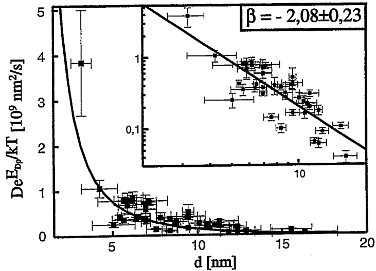
Abbildung 3.13: Adatominselbewegung: Diffusionskonstante als Funktion des Inseldurchmessers und doppeltlogarithmische Darstellung mit berechneter Geraden.
