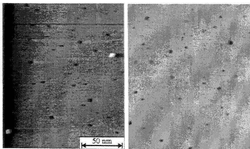
Abbildung A.3: Oberfläche nach Ionenbeschußpuls (600 eV, \text{Ar}^+ ), der ca. 0,05 ML aus der obersten Substratschicht entfernt hat; Aufnahmestart: (a) 4 min (b) 8 min nach Ionenbeschußpuls; (a) I_t = 3 nA; U_t = -0,5 V, RT; (b) I_t = 4 nA; U_t = -0,5 V, RT.
