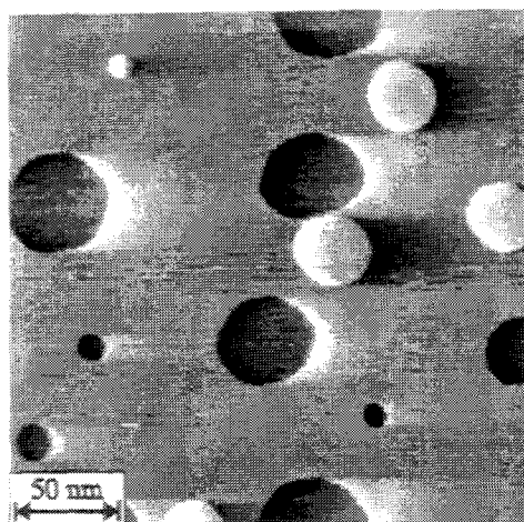
Abbildung A.5: Ionenpulsinduziertes Lagenwachstum: Deposition von 0,92 ML Ag; Depositionsrate: 1,2 \cdot 10^{-2} ML/s; Depositionsstart: 1 min nach Ionenbeschußpuls (600 eV, \text{Ar}^+ ); I_t = 5,2 nA, U_t = -0,5 V, RT.
