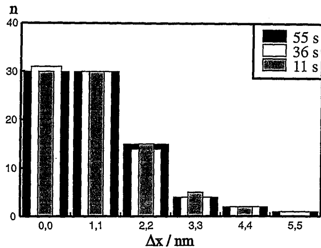
Abbildung 3.9: Einfluß des Meßprozesses: Positive Hälfte der Verschiebungsverteilung zweier Leerstelleninseln mit d = 14 nm bei verschiedenen Bildaufnahmezeiten, \Delta t = 60 s.
