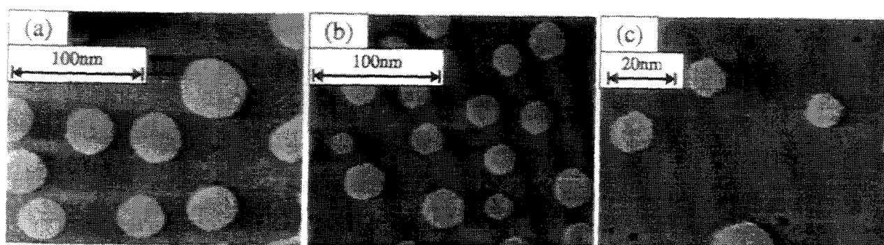
Abbildung A.4: Inseldichtenerhöhung: Deposition mit 0,01 ML/s; Depositionsstart: t_D nach einem 600eV- \text{Ar}^+ -Ionenbeschusspuls; (a) 0,26 ML, t_D = 30 s, I_t = 3,5 nA, U_t = -0,5 V, RT; (b) 0,21 ML, t_D = 0 s, I_t = 3 nA, U_t = -0,5 V, RT; (c) 0,08 ML, t_D = 0 s, I_t = 3 nA, U_t = -0,5 V, RT.
