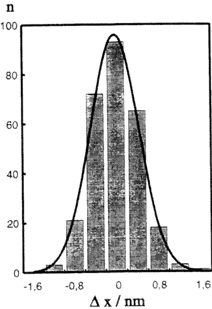
Abbildung 3.11: Histogramm der relativen Verschiebung zweier Adatominseln mit d_1 = 10,0 \text{ nm} und d_2 = 10,6 \text{ nm} , \Delta t = 60 \text{ s} ; Gefüllte Balken: experimentelle Werte; Kurve: erwartete Gaußverteilung.
