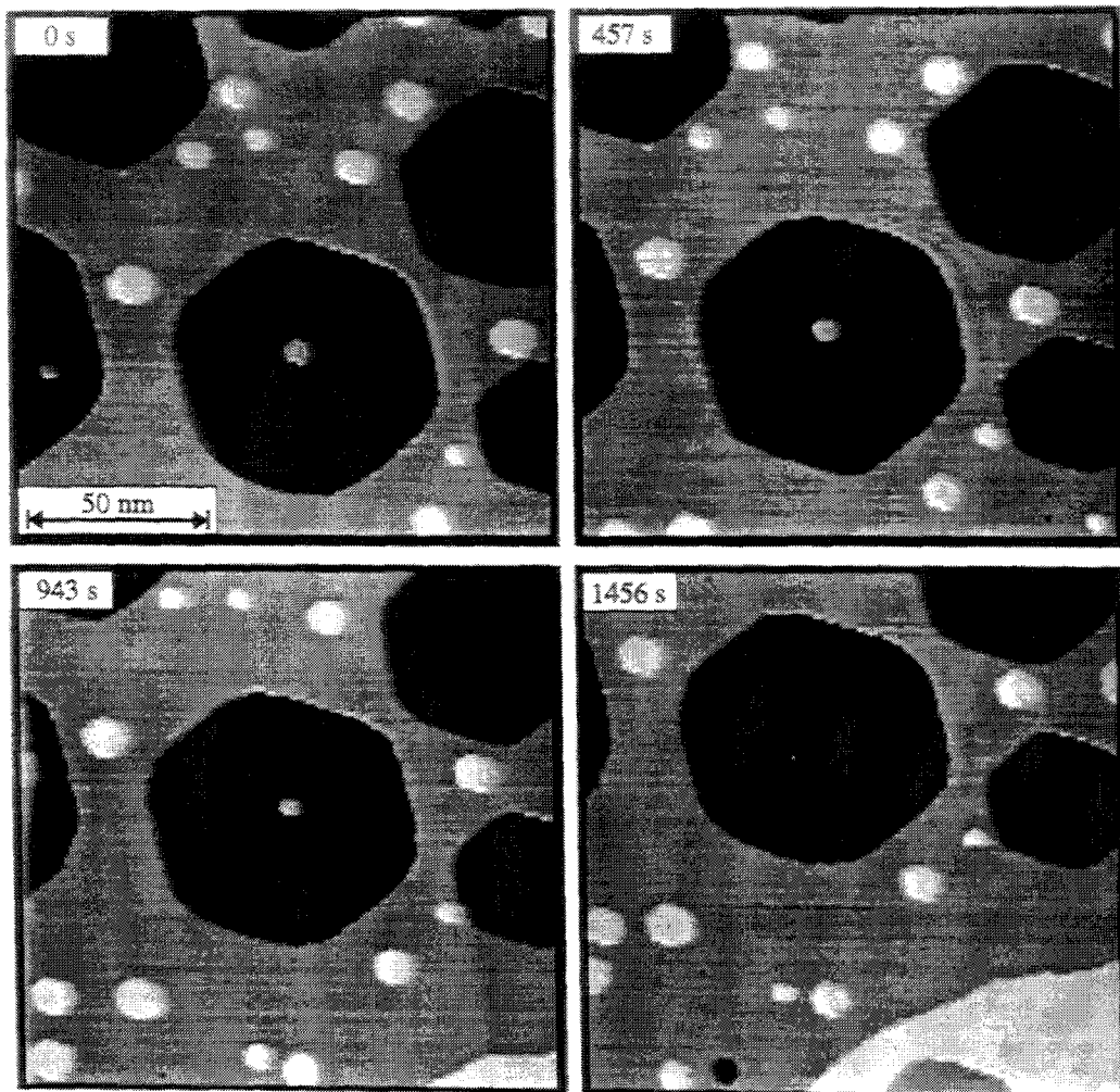
Abbildung 4.4: Adatominselzerfall in Leerstelleninsel: I_t = 0,03 nA U_t = -2 V; T = 275 K bis T = 278 K.
