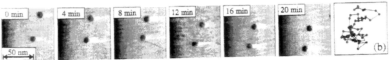
Abbildung 3.3: Leerstelleninselbewegung: Relative Bewegung zweier Leerstelleninseln gleicher Größe: U_t = -0.49 V, I_t = 9.5 nA, RT; (b) relative Verschiebung für alle 56 Bilder des Films, vergrößert um einen Faktor 3, \Delta t = 30 s.
