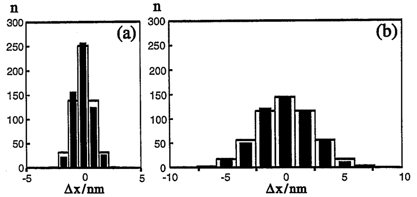
Abbildung 3.4: Gaußverteilung: Relative Verschiebung zweier Leerstelleninseln der Durchmesser d_1 und d_2 im Zeitintervall \Delta t ; Gefüllte Balken: experimentelle Werte; offene Balken: erwartete Gaußverteilung (a) d_1 = 21 Atome, d_2 = 24 Atome, \Delta t = 1 s (b) d_1 = d_2 = 21 Atome, \Delta t = 10 s.
