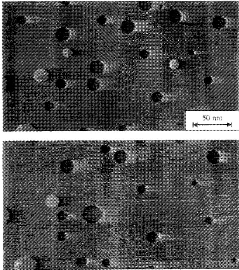
Abbildung 1.1: Oberflächenveränderung: RTM-Bilder einer Ag(111)-Oberfläche aufgenommen im Abstand von 45 min; I_t = 5 \text{ nA} , U_t = -0,8 \text{ V} , RT.
