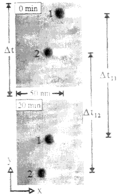
Abbildung 2.4: Unterschied zwischen dem Zeitintervall \Delta t zwischen den Bildaufnahmestarts und \Delta t_I zwischen den Inselabbildungen; I_t = 9,5 \text{ nA} , U_t = -0,49 \text{ V} , RT.
