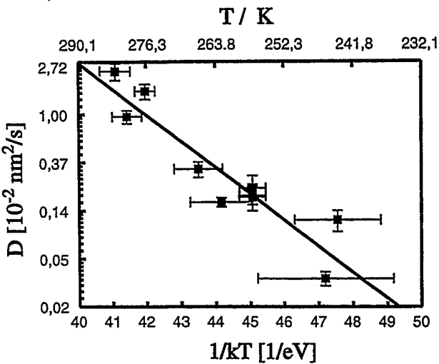
Abbildung 3.12: Adatominselbewegung: Arrhenius-Darstellung der Adatominseldiffusionskonstante über der Temperatur für Inseln mit Durchmessern zwischen 6,2 nm und 7,0 nm.
