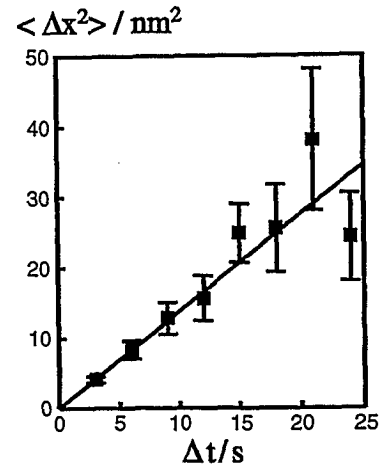
Abbildung 3.6: Diffusionskonstantenbestimmung: Mittlere quadratische Abweichung des Leerstelleninselabstands als Funktion der Zeit mit berechneter Geraden; d_1 = 13 Atome, d_2 = 18 Atome.
