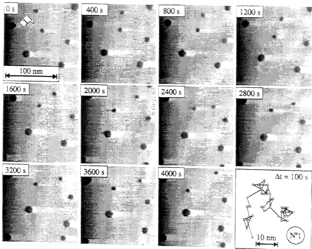
Abbildung 3.2: Leerstelleninselbewegung; Folge von RTM-Bildern; I_t = 4,9 nA, U_t = -2,9 V, RT; und Positionen, die die Leerstelleninsel Nr. (1) auf allen 48 Bildern hatte, vergrößert um einen Faktor 3, \Delta t = 10 s.
