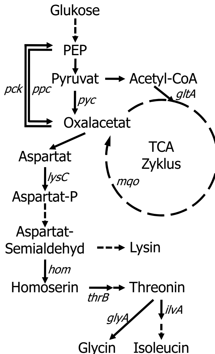
Abbildung 9: Schematische Übersicht des Stoffwechselwegs ausgehend von dem Substrat Glukose zu dem Produkt L-Threonin und dessen Abbauprodukte Glycin und L-Isoleucin. Zusätzlich sind Stoffwechsel-relevante Gene gezeigt, die für folgende Enzyme kodieren: gltA – Citrat-Synthase, glyA – Serinhydroxymethyltransferase, hom – Homoserin-Dehydrogenase, ilvA – Threonin-Dehydratase, lysC – Aspartat-Kinase, mgo – Malatquinon-Oxidoreduktase, pck – Phosphoenolpyruvat-Carboxykinase, ppc – Phosphoenolpyruvat-Carboxylase, pyc – Pyruvat- Carboxylase, thrB – Homoserin-Kinase
