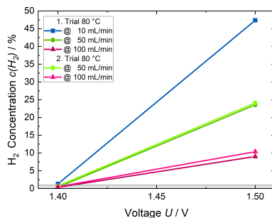
(d) H_2 evolution at 80 °C.
