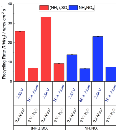
(d) Recycling Rate @ 5 mL/min, 80 °C
