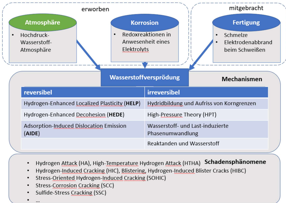
Abbildung 2.2.4.1: Eigene Darstellung: Übersicht zur Wasserstoffversprödung, von der Herkunft (oben) über die unterliegenden Mechanismen (Mitte) zu den zutage tretenden Schadensphänomenen (unten).
