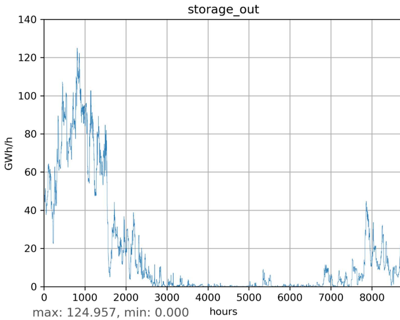
Abbildung 5.2.3.4: Sektorzeitreihe: Ausspeicherung aus Gasspeichern
