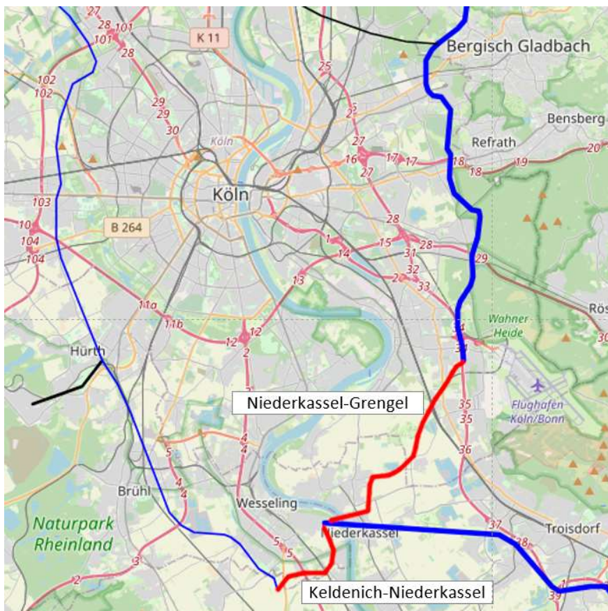
Abbildung 5.2.3.1: Bild: Bottlenecks auf den Pipelineabschnitten Niederkassel-Grengel und Keldenich-Niederkassel.
