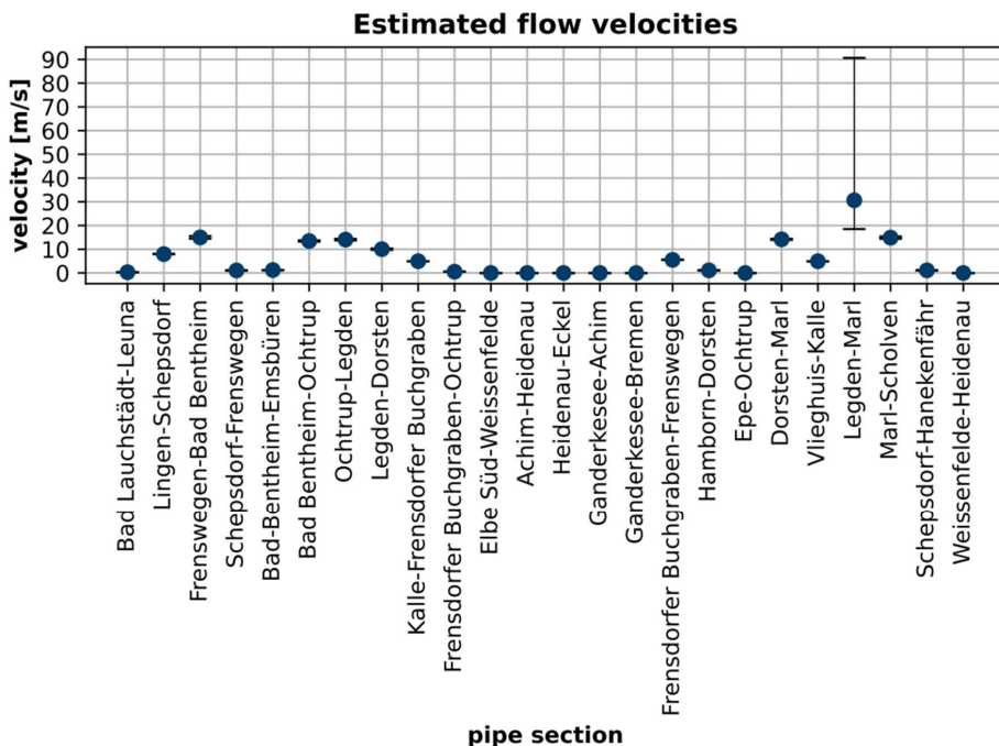
Abbildung 4.1.10.3: Geschätzte Fließgeschwindigkeiten im 2025 Basisszenario (durchschnittlich) bei 30 bar Maximaldruck. Die „Fehlerschranken“ geben die Fließgeschwindigkeit am Pipelineeintritt bzw. am -austritt an.
