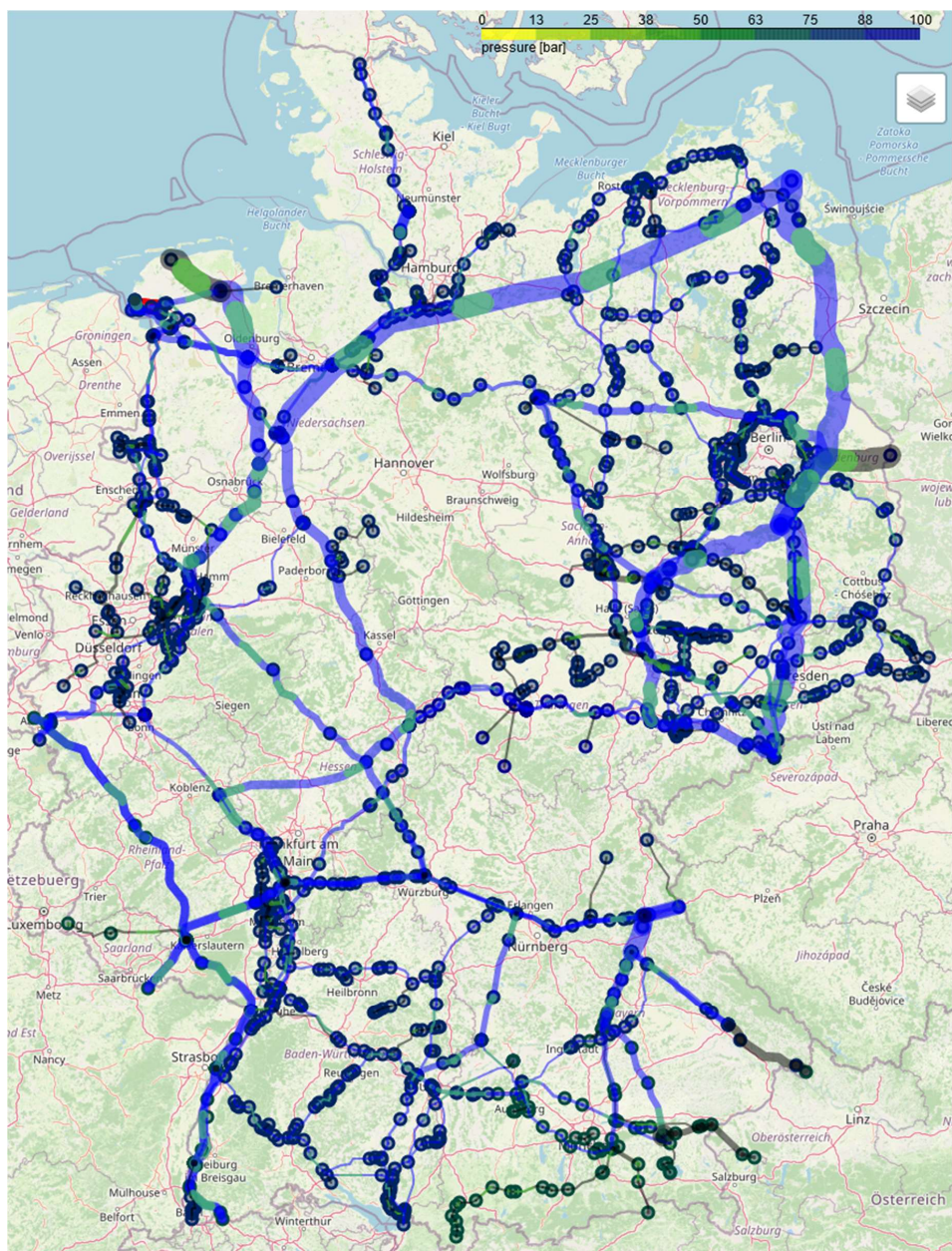
Abbildung 5.2.3.18: Flüsse und Drücke in der Erdgas-Nominierung des 04.07.2015 um 00:00 Uhr. Bei Maximierung (10%-Optimality-Gap) der Drücke an den Netzknoten. Die Drücke an den Knoten sind entsprechend des dargestellten Farbcodes (oben rechts) eingefärbt. Die Dicke der Kanten ist proportional zum Fluss darüber.
