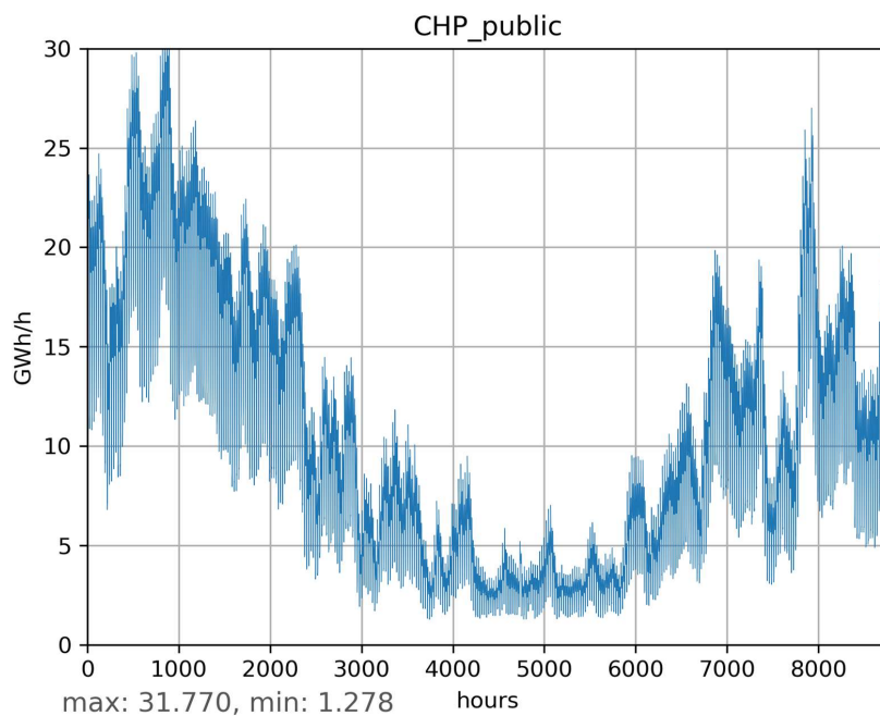
Abbildung 5.2.3.7: Sektorzeitreihe: Öffentliche Kraft-Wärme-Kopplung
