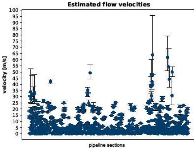
Abbildung 5.2.3.13: Durchschnittlich geschätzte Fließgeschwindigkeiten von Wasserstoff entlang der Pipelineabschnitte (x-Achse) am 11.08.2015 um 15:00 Uhr. Die Fehlerschranken kennzeichnen die Fließgeschwindigkeit am Ein- bzw. Austritt der Pipeline. Mit wenigen Ausnahmen liegen die Geschwindigkeiten unter 25 m/s bzw. unter 15 m/s.
