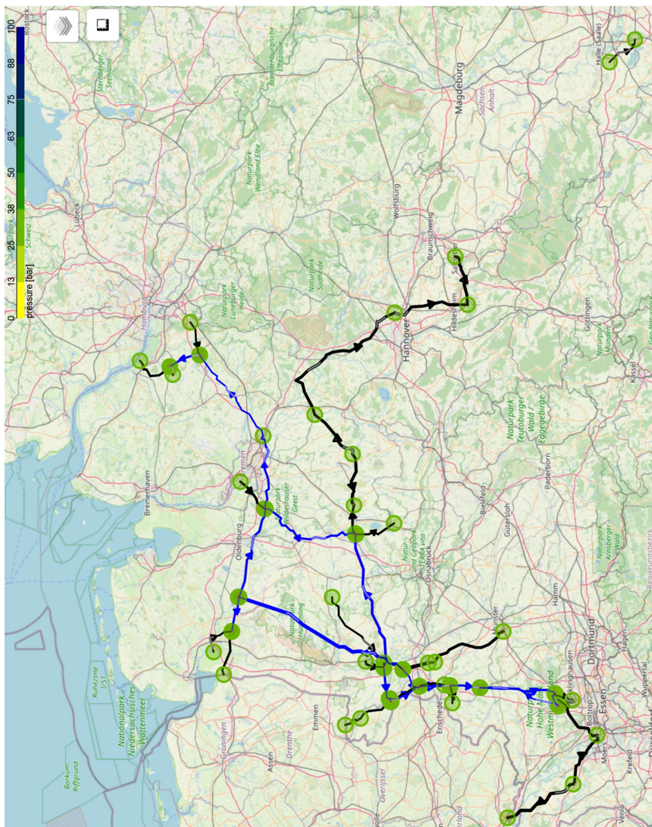
Abbildung I.8.11.3: Drücke im Variation 1 Szenario 2030 bei 30 bar Maximaldruck und angenommener Rohrrauigkeit von 0,1 mm. Legende, siehe Tabelle I.8.1.1.
