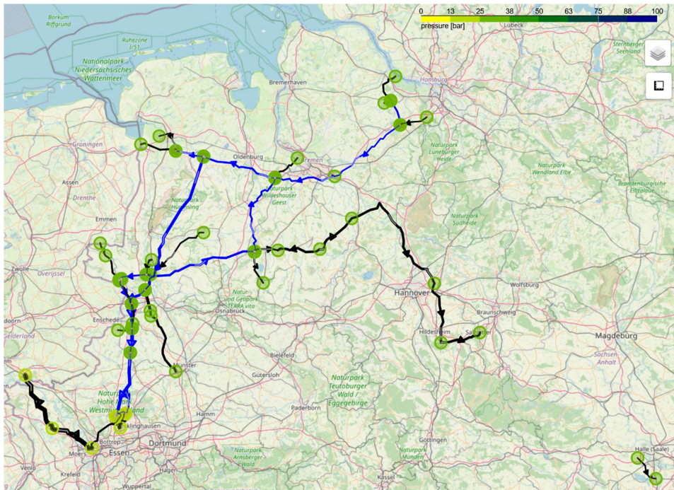
Abbildung 5.2.1.2: Drücke im Basisszenario 2030 bei 30 bar Maximaldruck und angenommener Rohrrauigkeit von 0.1 mm. Die Drücke an den Netzknoten sind farblich entsprechend der Farbskala kodiert. Die Dicke einer Kante des Graphen ist proportional zum Fluss über die Kante. Einige Knoten erscheinen ausgefüllt, dies ist jedoch nur auf die Überlagerung von nahe beieinander liegenden Knoten zurückzuführen.
