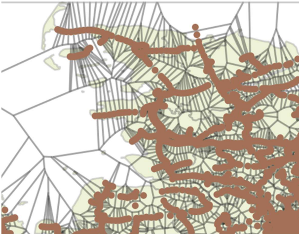
Abbildung 3.2.3.3: Verbesserte Einlastung flächenspezifischer Lasten unter Zuhilfenahme eines höher aufgelösten Datensatzes in Verbindung mit einer Breitensuche (BFS). Veranschaulichung der Knotenzuordnung auf Basis eines Zoom-Ausschnitts von Norddeutschland: 1. Schritt: Erzeugung von Voronoi-Polygonen um die Netzknoten des feinaufgelösten Datensatzes.
