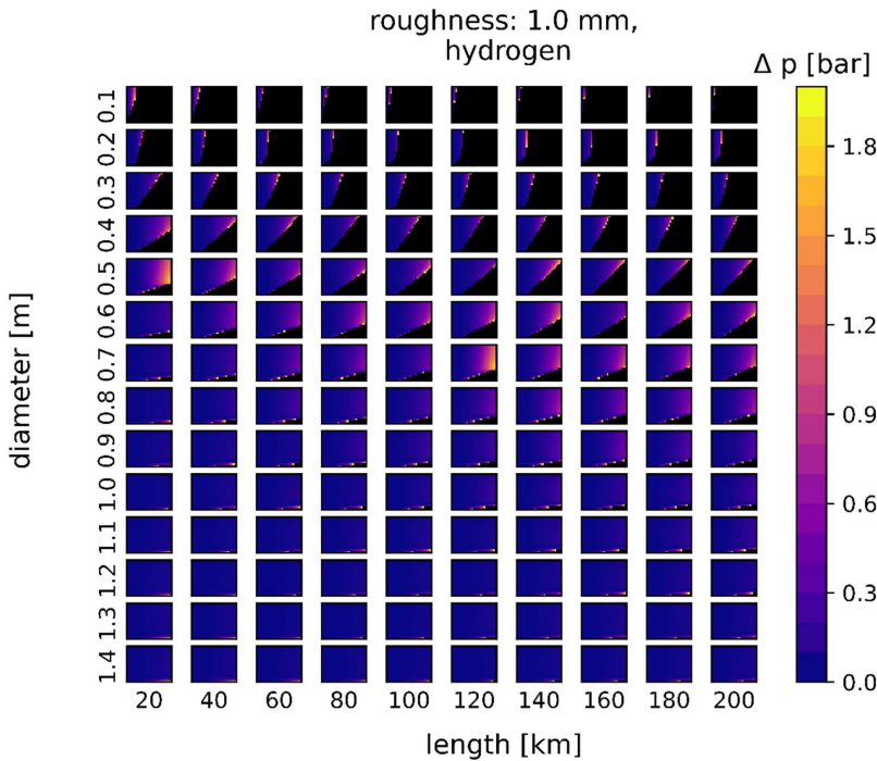
Abbildung 4.1.10.4: Screening: Differenz des Ausgangsdrucks nach Gleichung Gl. 4.3 gegenüber pandapipes: Für jede Kachel: Flüsse (x-Achse): [0,1 kg/s - 0,5 kg/s, 1 - 20 kg/s], Eingangsdrücke (y-Achse): 5-100 bar, Wasserstoff, Rohrrauigkeit 1 mm.
