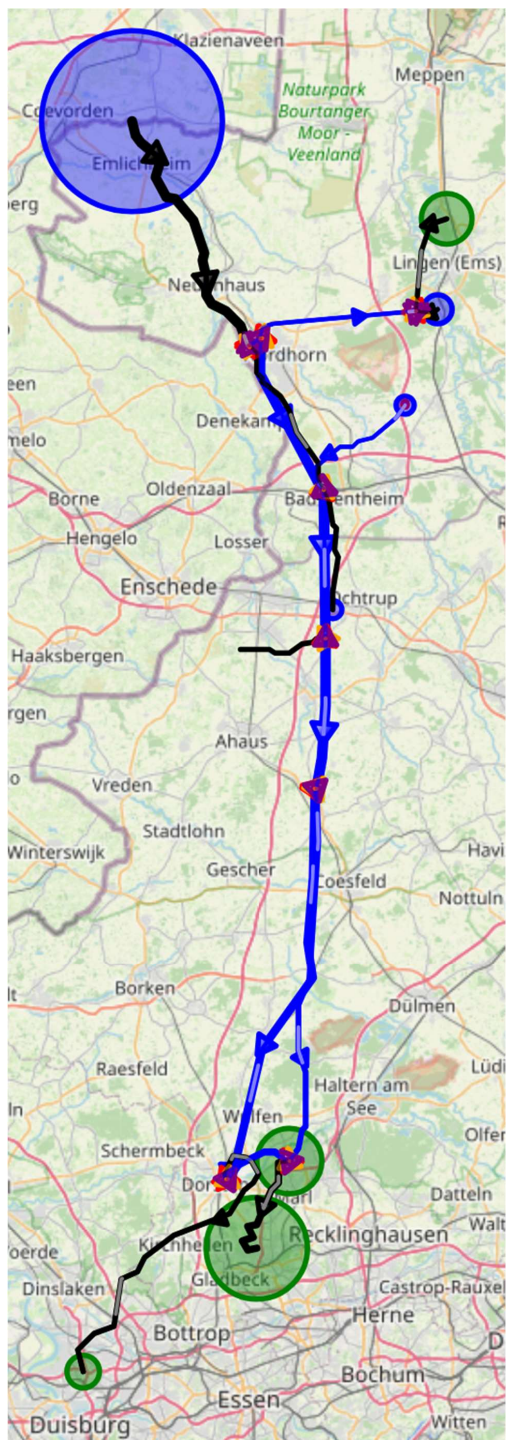
Abbildung I.8.3.2: Flüsse im 2025 Basisszenario bei 30 bar Maximaldruck und angenommener Rohrrauigkeit von 0,1 mm. Legende, siehe Tabelle I.8.1.1.
