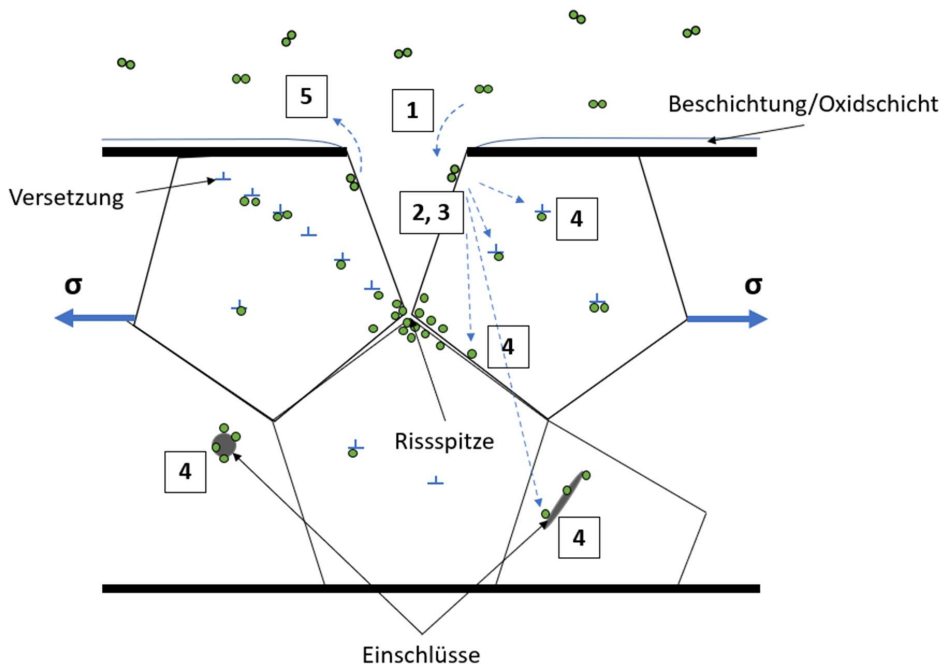
Abbildung 2.2.4.2: Eigene Darstellung in Anlehnung an [28]: Interaktion zwischen Wasserstoff und metallischer Oberfläche. (1): Physisorption aus der Gasphase an die oxid-freie, metallische Oberfläche. (2): Chemisorption einer Monolage. (3): Dissoziation zu atomarem Wasserstoff. (4): Diffusion des atomaren H^+ durch das Metallgitter und Trapping an energetisch günstigen Stellen (Versetzungen, Einschlüsse, Korngrenzen). (5): Rekombination von atomarem H^+ zu H_2 und Desorption.
