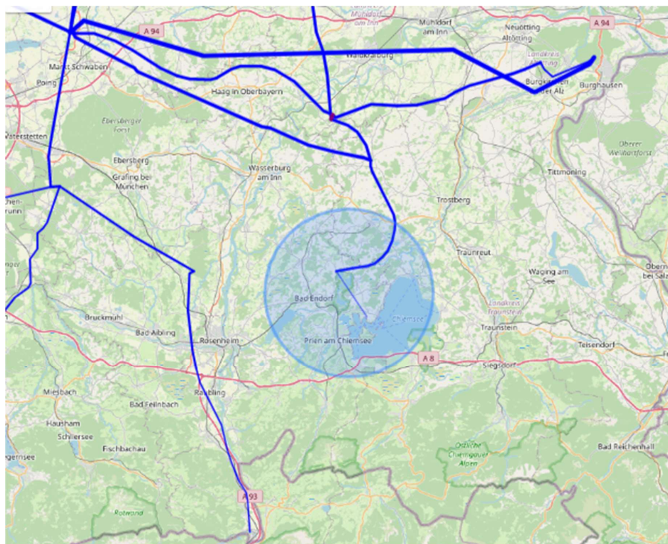
Abbildung 5.2.3.2: Bottleneck: Die Nominierung für den 06.02.2015 um 06:00 Uhr zeigt einen Bottleneck am Chiemsee auf.
