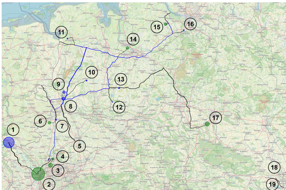
Abbildung 3.1.7.1: Überblick über die Quellen- und Senkenverteilung im Basisszenario 2030. Die Kreisgrößen stellen die relative lokale Ein-/Auspeisung im Verhältnis zur maximalen Ein-/Auspeisung innerhalb des Szenarios dar, wobei die Skalierung über den Radius (nicht die Fläche) erfolgt. Zur Wahrung der Lesbarkeit sind Mindest- und Maximalradien definiert. Ein Vergleich der Kreisgrößen zwischen verschiedenen Szenarien ist daher nicht zulässig.
