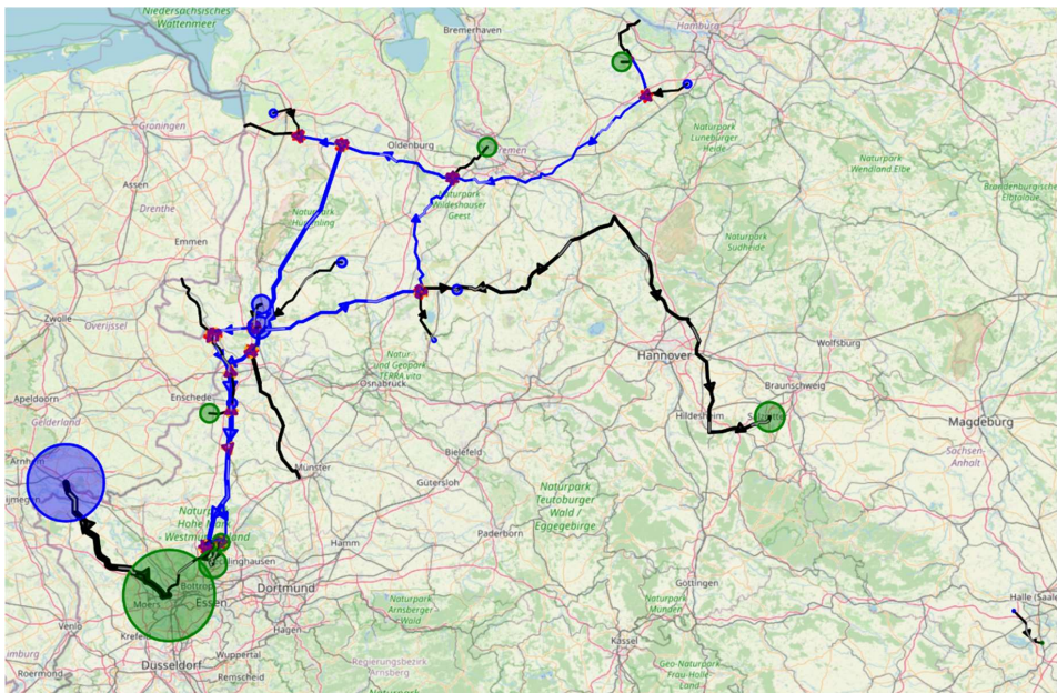
Abbildung 5.2.1.1: Flüsse im 2030 Basisszenario bei 30 bar Maximaldruck und angenommener Rohrrauigkeit von 0,1 mm. Die Ein-/Auspeisemengen sind als Kreise dargestellt und relativ zueinander skaliert. Quellen sind blau gefärbt und Senken grün. Die jeweilige Ein-/Auspeisemenge ist proportional zum Kreisdurchmesser. Die Dicke einer Kante des Graphen ist proportional zum Fluss über die Kante. Die größte Auspeisung hier liegt bei 6,65 kg/s in Hamborn (ThyssenKrupp). Zum Vergleich siehe auch Tabelle 5.2.1.2.
