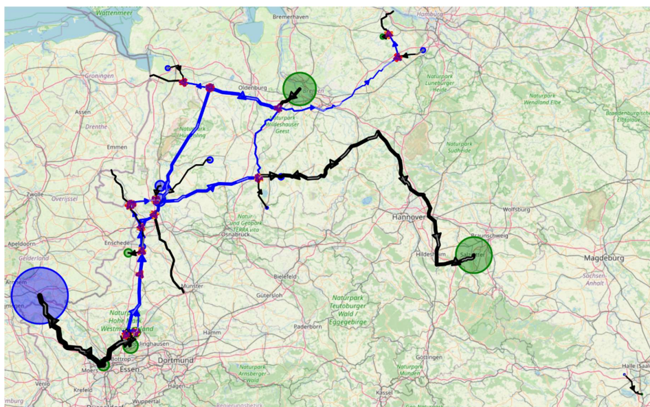
Abbildung 5.2.3.1: Flüsse im Variation 2 Szenario 2030 bei 30 bar Maximaldruck und angenommener Rohrrauigkeit von 0,1 mm. Die Ein-/Auspeisemengen sind als Kreise dargestellt und relativ zueinander skaliert. Die jeweilige Ein-/Auspeisemenge ist proportional zum Kreisdurchmesser. Quellen sind blau gefärbt und Senken grün. Die Dicke einer Kante des Graphen ist proportional zum Fluss über die Kante. Die größte Einspeisung liegt hier bei 7,51 kg/s in Elten. Zum Vergleich siehe auch Tabelle 5.2.3.1.
