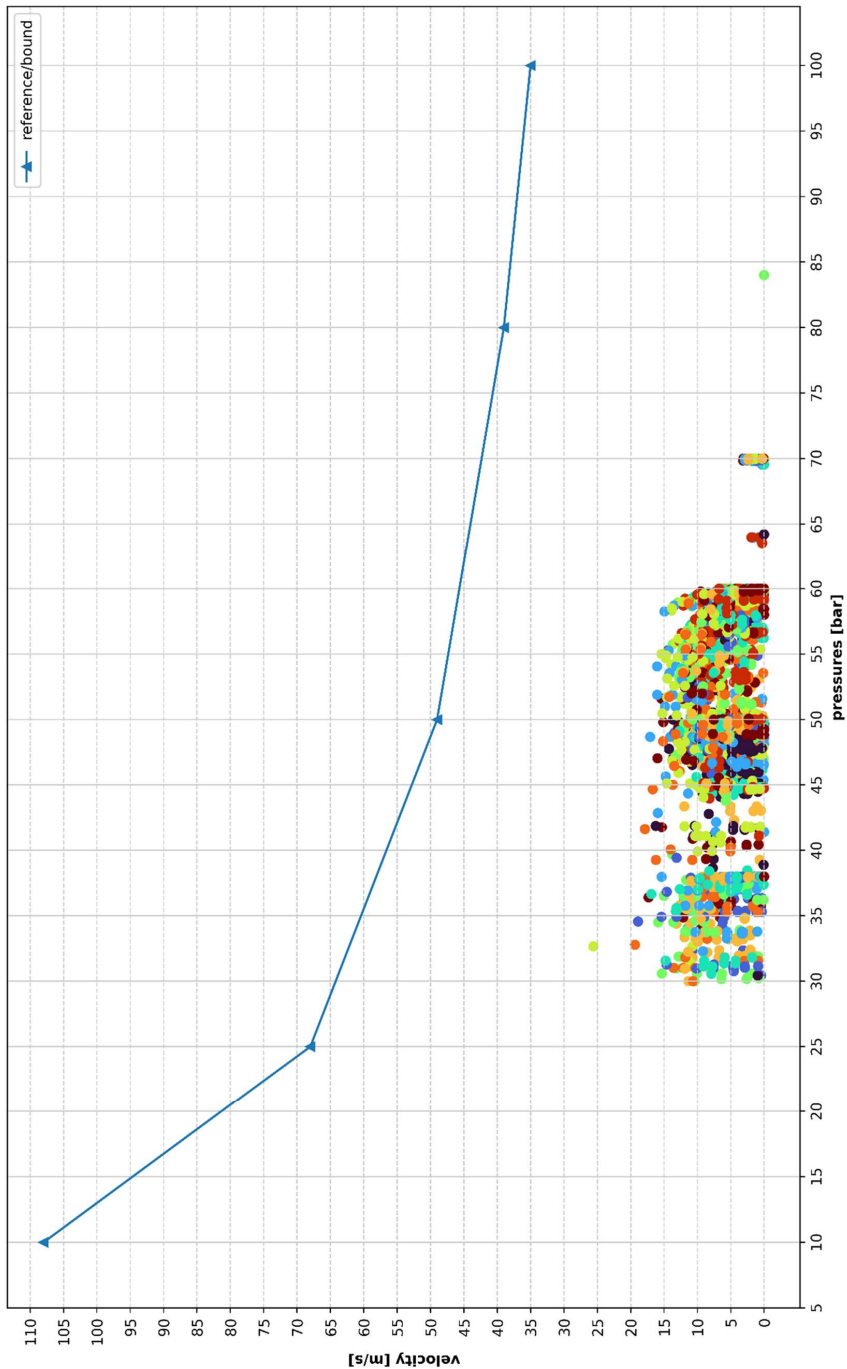
Abbildung 5.2.3.5: 200 Zufällige Lastfälle: Druck-Geschwindigkeits-Paare im Verhältnis zur Grenzwertkurve gemäß Tabelle 2.2.4.2 bei einer globalen Druck-Unterschranke von 30 bar ohne Druckregelventile an den Kreuzungspunkten. Unterschiedliche Farben stehen für unterschiedliche Lastfälle.
