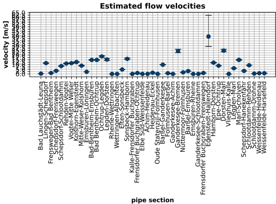
Abbildung I.8.15.1: Geschätzte Fließgeschwindigkeiten im Variation 2 Szenario 2030 (durchschnittlich) bei 30 bar Maximaldruck und angenommener Rohrrauigkeit von 0,1 mm. Die Fehlerschranken geben die Fließgeschwindigkeit am Pipelineintritt bzw. am -austritt an.
