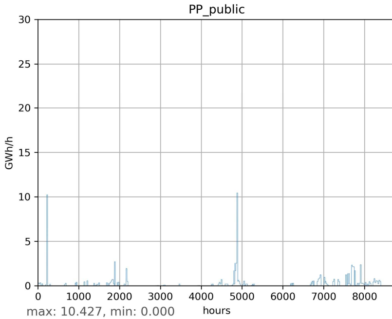
Abbildung 5.2.3.12: Sektorzeitreihe: Kraftwerke (öffentlich)
