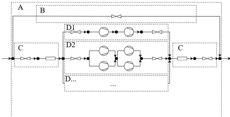
Abbildung 4.1.9.1: Abbildung einer generischen Verdichterstation; A: Station; B: internes Bypass-Ventil; C: Einlass-/Auslassventil mit künstlichem Widerstand zur Abbildung interner Verrohrungsverluste; D1-D...: Verdichterkonfigurationen, flach ausgelegt, schaltbar über Ein-/Ausgangsventile; D1: Reihenschaltung von zwei Verdichtern; D2: Parallelschaltung zweier Verdichter mit zwei Stufen in Reihe; D...: weitere Konfigurationen analog zu D1 und D2.
