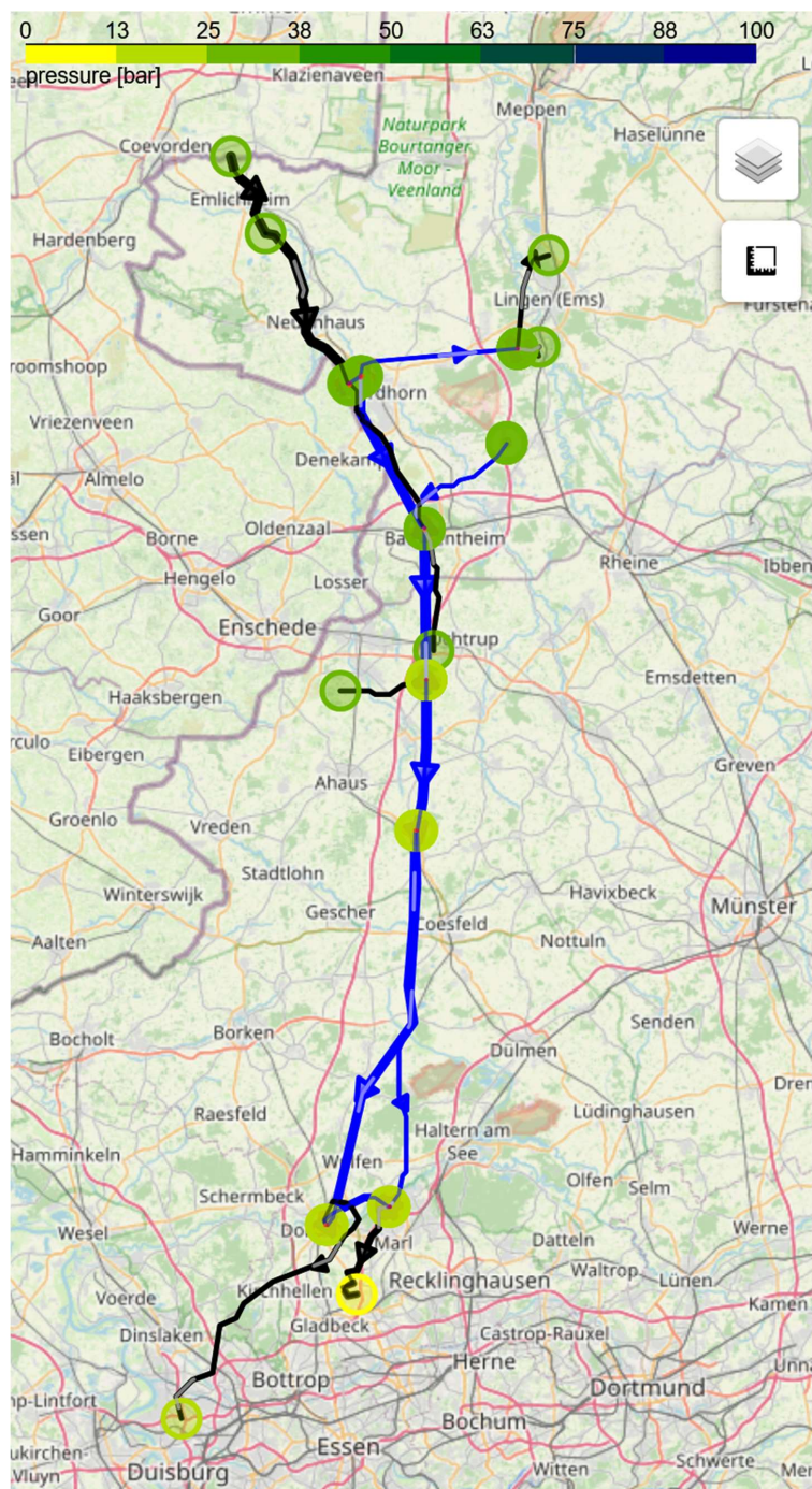
Abbildung I.8.2.2: Drücke im 2025 Basisszenario bei 30 bar Maximaldruck und angenommener Rohrrauigkeit von 1 mm. Legende, siehe Tabelle I.8.1.1.
