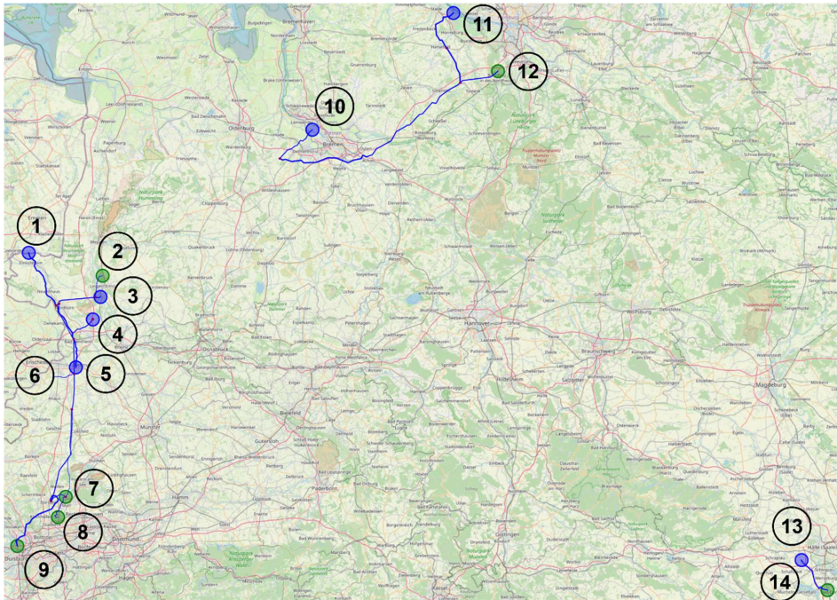
Abbildung 3.1.4.1: Überblick: Modellierter Wasserstoffnetzwerktopologie 2025. Blaue Kreise stehen für Quellen, und Grüne Kreise für Senken (siehe Tabelle 3.1.4.1). In dieser Darstellung dienen die Kreise lediglich der Verortung der Quellen und Senken und geben keinerlei Auskunft über Ein- oder Auspeisemengen.
