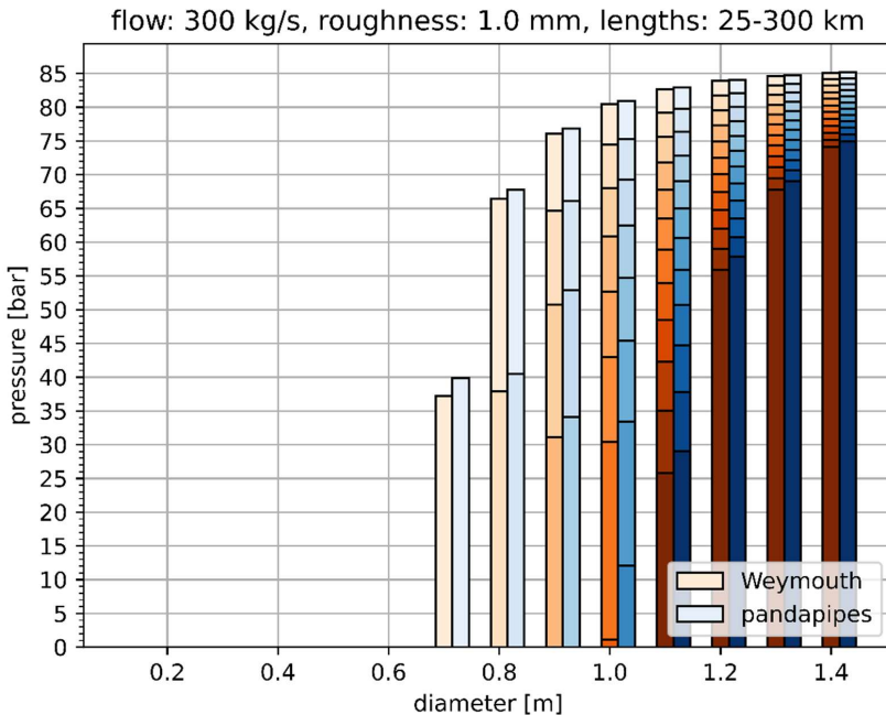
Abbildung 4.1.10.2: Vergleich Druckabfall Gleichung Gl. 4.3 gegenüber pandapipes: Fluss 300 kg/s Erdgas, Rohrrauigkeit 1 mm, Eingangsdruck 86 bar. Variiert über den Rohrdurchmesser (x-Achse, 100 mm Schritte) und über die Rohrlänge (Bildtiefe, 25 km Schritte).
