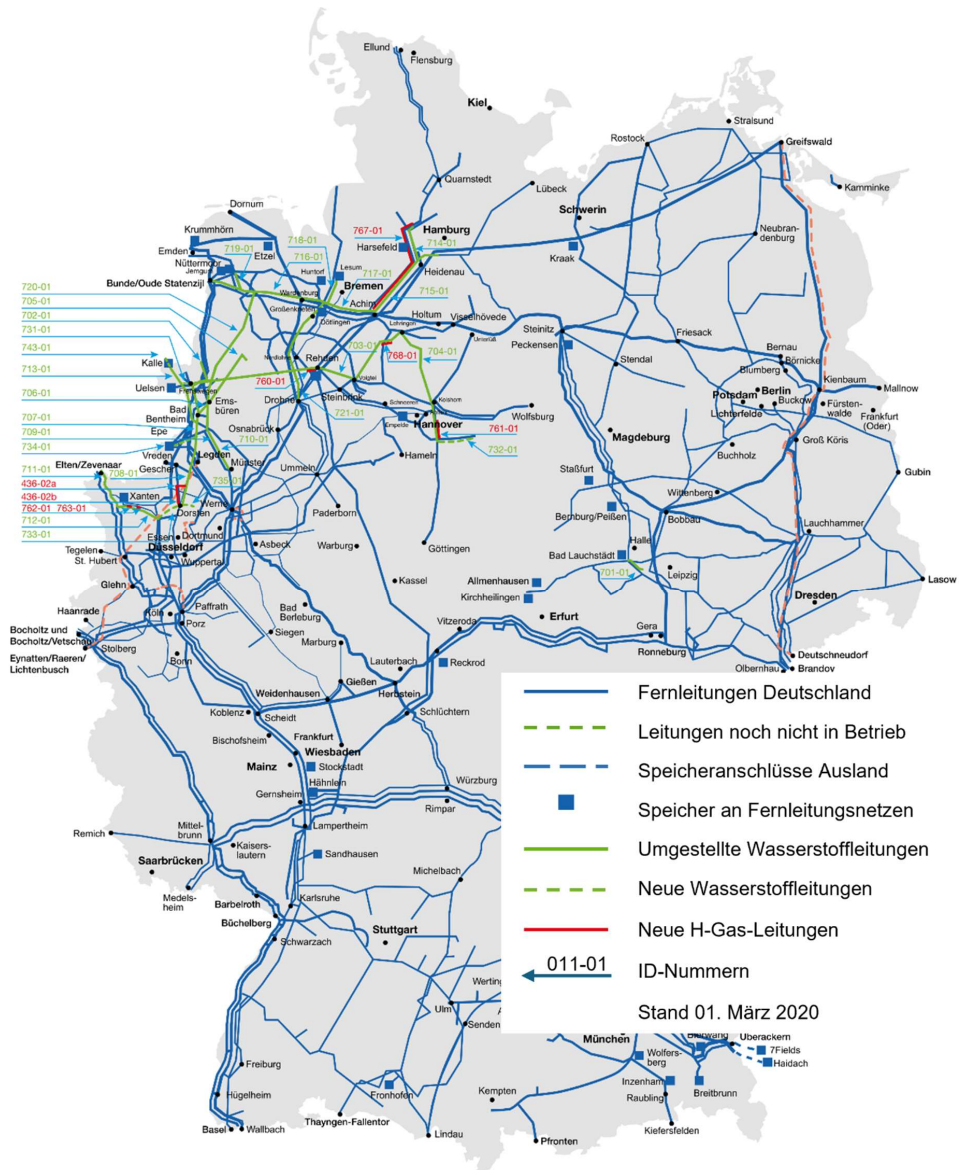
Abbildung 3.1.6.2: Überblick: Wasserstoffnetzwerktopologie 2030 (in Grün) gemäß Netzentwicklungsplan Gas 2020 [7]. Quelle: FNB Gas e.V.
