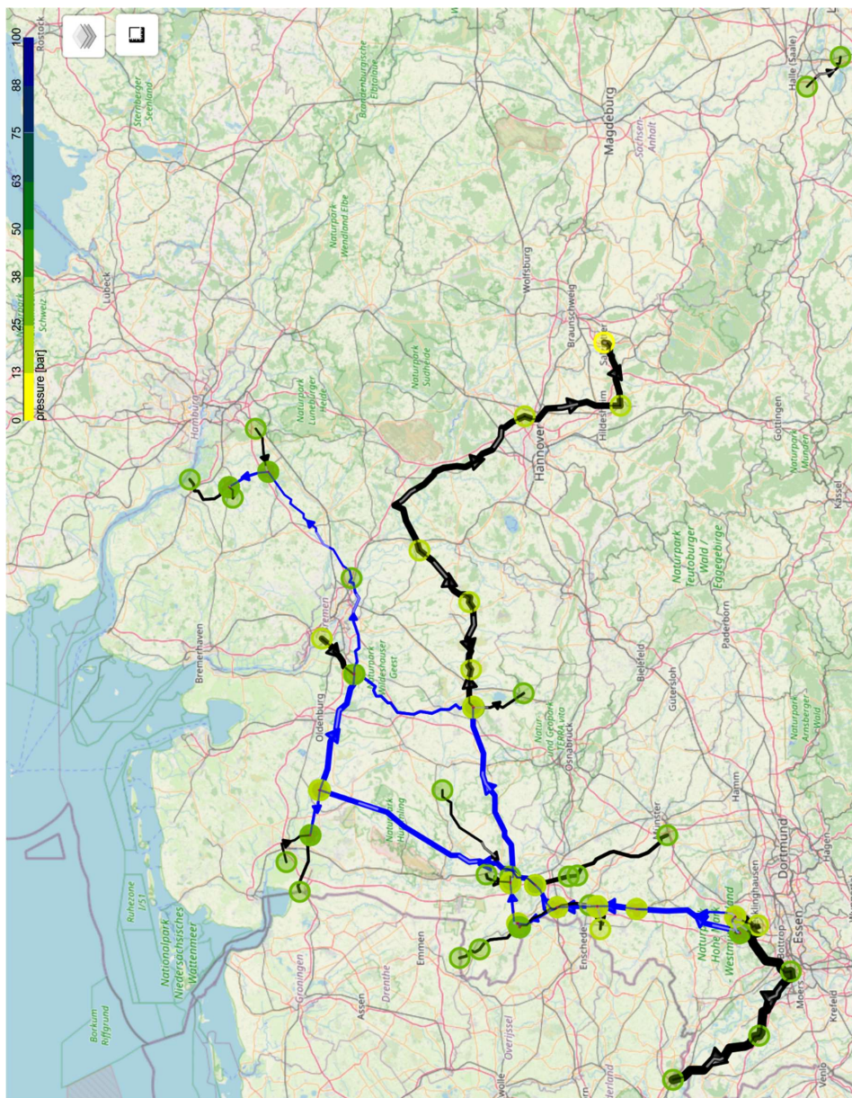
Abbildung I.8.15.3: Drücke im Variation 2 Szenario 2030 bei 30 bar Maximaldruck und angenommener Rohrrauigkeit von 0,1 mm. Legende, siehe Tabelle I.8.1.1.
