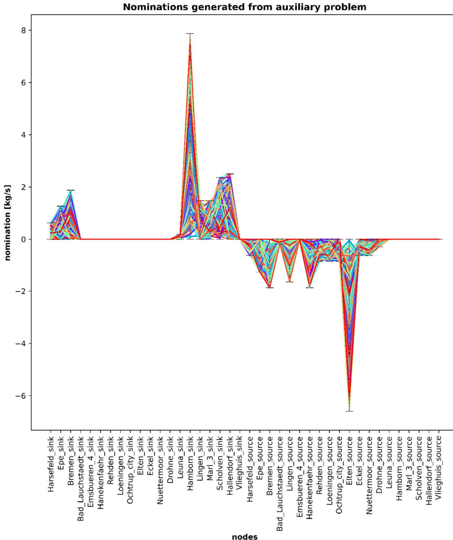
Abbildung 5.2.3.1: 200 Zufällige Lastfälle mit angesetzten Ein-/Ausspeiseintervallen. Die Linienverbindung dient lediglich der Orientierung, da mehrere Lastfälle gleichzeitig abgebildet sind. Jeder Quellen-/Senkenknoten ist, analog zur Problemformulierung in Gl. 7.1 - Gl. 7.12, einmal als Senke (linke Hälfte) und einmal als Quelle (rechte Hälfte) aufgeführt.
