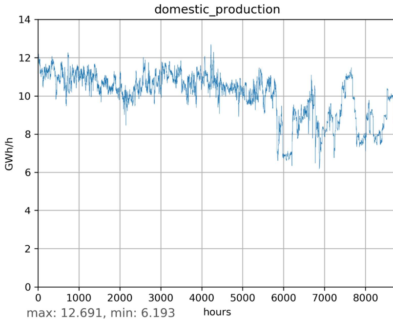
Abbildung 5.2.3.16: Sektorzeitreihe: Inländische Produktion/Förderung
