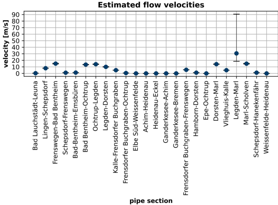
Abbildung 1.8.3.1: Geschätzte Fließgeschwindigkeiten im 2025 Basisszenario (durchschnittlich) bei 30 bar Maximaldruck und angenommener Rohrrauigkeit von 0,1 mm. Die Fehlerschranken geben die Fließgeschwindigkeit am Pipelineeintritt bzw. am -austritt an.
