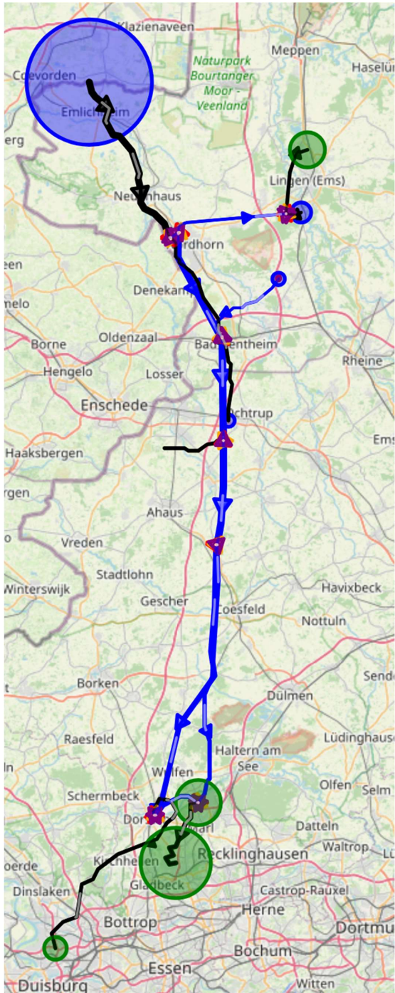
Abbildung I.8.5.2: Flüsse im 2025 Basisszenario bei 60 bar Maximaldruck und angenommener Rohrrauigkeit von 0,1 mm. Legende, siehe Tabelle I.8.1.1.
