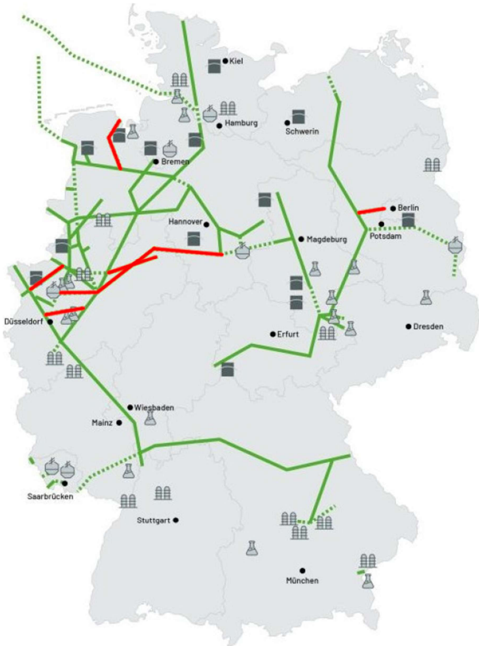
Abbildung 3.1.9.2: Skizze des geplanten Netzes 2030 gemäß Entwurf Szenariorahmen NEP-Gas 2022
