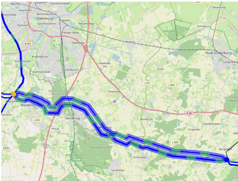
Abbildung 5.2.3.17: Loopeitung mit hoher Fließgeschwindigkeit bei Oldenburg in der Node-Slack-Lösung.
