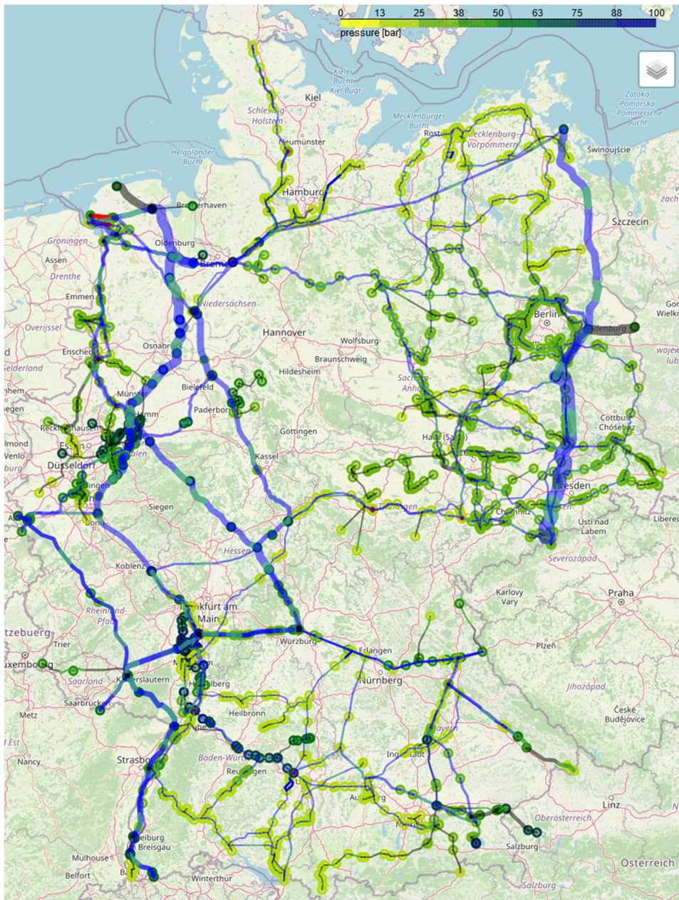
Abbildung I.8.18.3: Flüsse und Drücke in der Wasserstoff-Nominierung des 06.02.2015 um 06:00 Uhr (unlösbar, d.h. verbleibendes Node-Slack). Die Drücke an den Knoten sind entsprechend des dargestellten Farbcodes (oben rechts) eingefärbt. Die Dicke der Kanten ist proportional zum Fluss darüber. Legende, siehe Tabelle I.8.1.1.
