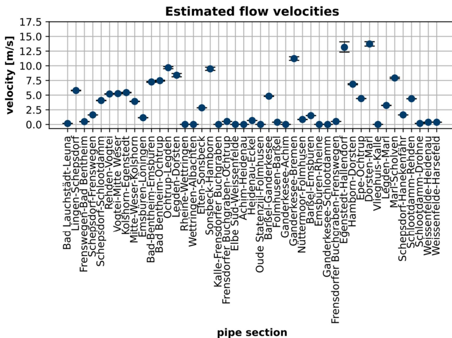
Abbildung I.8.16.1: Geschätzte Fließgeschwindigkeiten im Variation 2 Szenario 2030 (durchschnittlich) bei 60 bar Maximaldruck und angenommener Rohrrauigkeit von 1 mm. Die Fehlerschranken geben die Fließgeschwindigkeit am Pipelineeintritt bzw. am -austritt an.
