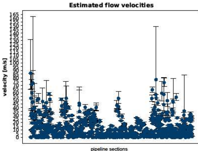
Abbildung 5.2.3.16: Durchschnittlich geschätzte Fließgeschwindigkeiten von Wasserstoff entlang der Pipelineabschnitte (x-Achse) am 02.12.2015 um 05:00 Uhr. Die Fehlerschranken kennzeichnen die Fließgeschwindigkeit am Ein- bzw. Austritt der Pipeline. Mit wenigen Ausnahmen liegen die Geschwindigkeiten unter 35 m/s bzw. unter 25 m/s. Die maximal erreichte Fließgeschwindigkeit liegt hier bei 163 m/s.
