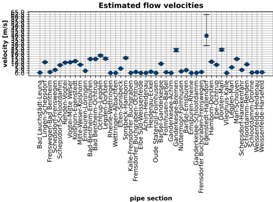
Abbildung 5.2.3.2: Geschätzte Fließgeschwindigkeiten im Variation 2 Szenario 2030 (durchschnittlich) bei 30 bar Maximaldruck und angenommener Rohrrauigkeit von 0,1 mm. Die Fehlerschranken geben die Fließgeschwindigkeit am Pipelineeintritt bzw. am -austritt an.
