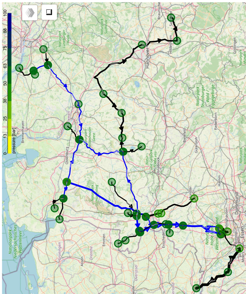
Abbildung I.8.8.3: Drücke im 2030 Basisszenario bei 60 bar Maximaldruck und angenommener Rohrrauigkeit von 1 mm. Legende, siehe Tabelle I.8.1.1.
