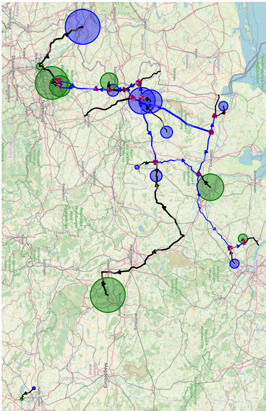
Abbildung I.8.11.2: Flüsse im Variation 1 Szenario 2030 bei 30 bar Maximaldruck und angenommener Rohrrauigkeit von 0,1 mm. Legende, siehe Tabelle I.8.1.1.
