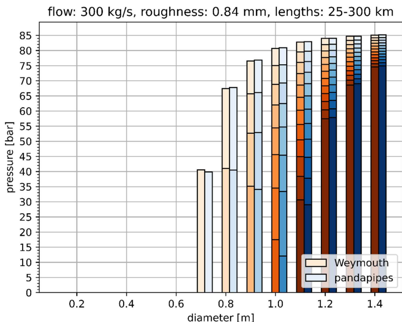
Abbildung 4.1.10.5: Vergleich Druckabfall Gleichung Gl. 4.3 gegenüber pandapipes: Fluss 300 kg/s Erdgas, Rohrrauigkeit 0.84 mm, Eingangsdruck 86 bar. Variiert über den Rohrdurchmesser (x-Achse, 100 mm Schritte) und über die Rohrlänge (Bildtiefe, 25 km Schritte).
