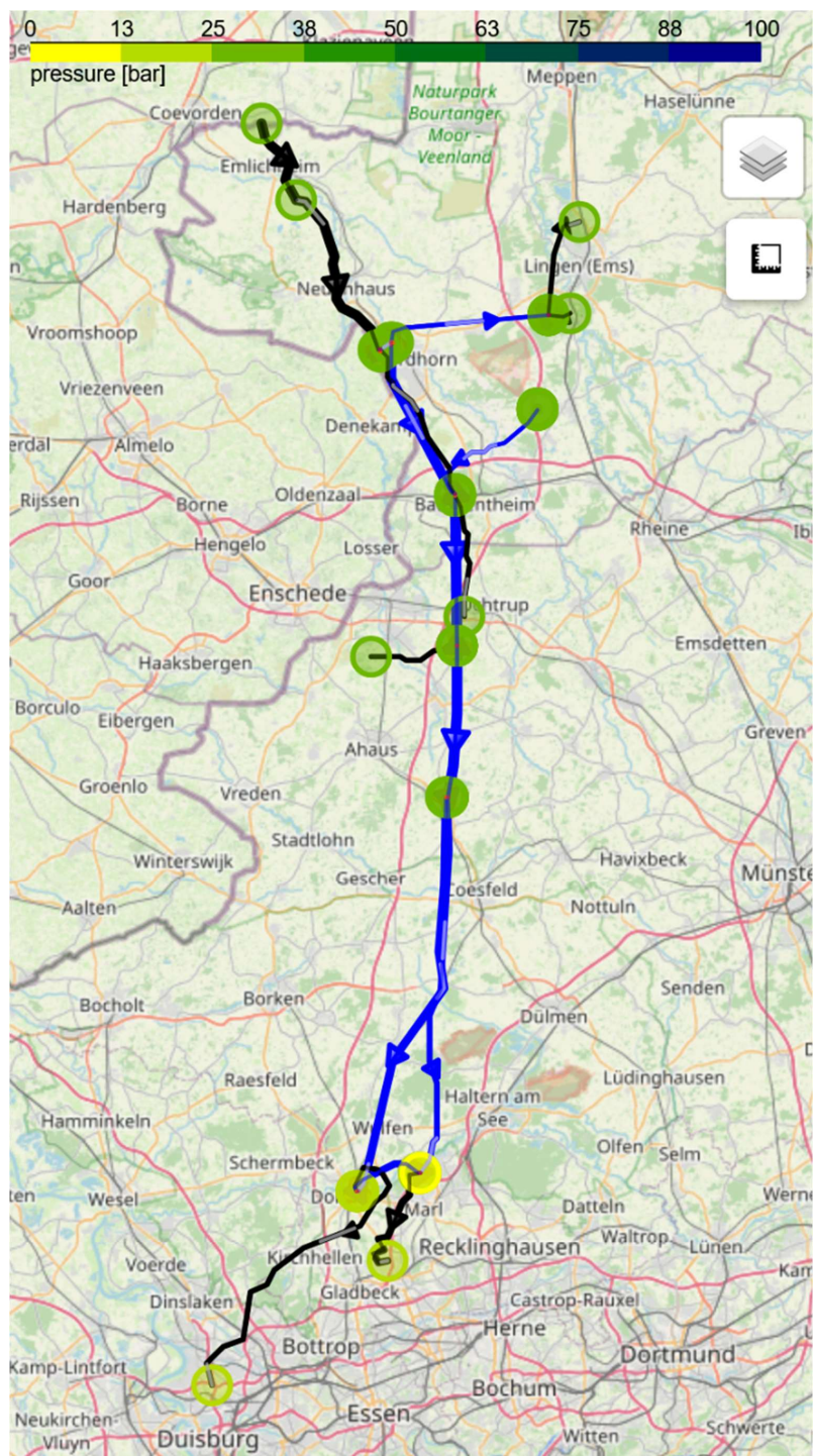
Abbildung I.8.3.3: Drücke im 2025 Basisszenario bei 30 bar Maximaldruck und angenommener Rohrrauigkeit von 0,1 mm. Legende, siehe Tabelle I.8.1.1.
