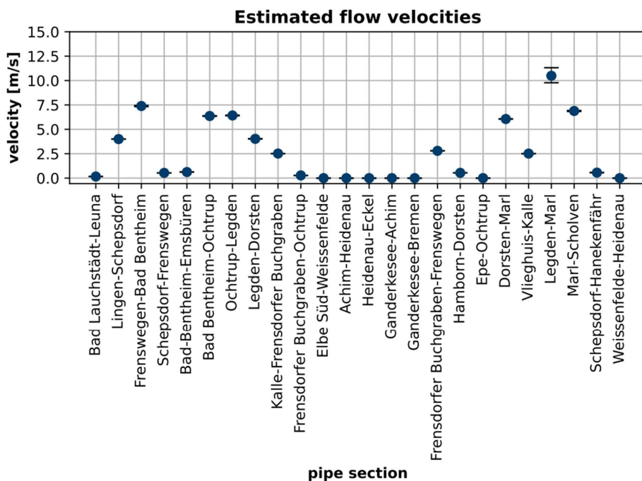
Abbildung 1.8.5.1: Geschätzte Fließgeschwindigkeiten im 2025 Basisszenario (durchschnittlich) bei 60 bar Maximaldruck und angenommener Rohrrauigkeit von 0,1 mm. Die Fehlerschranken geben die Fließgeschwindigkeit am Pipelineeintritt bzw. am -austritt an.
