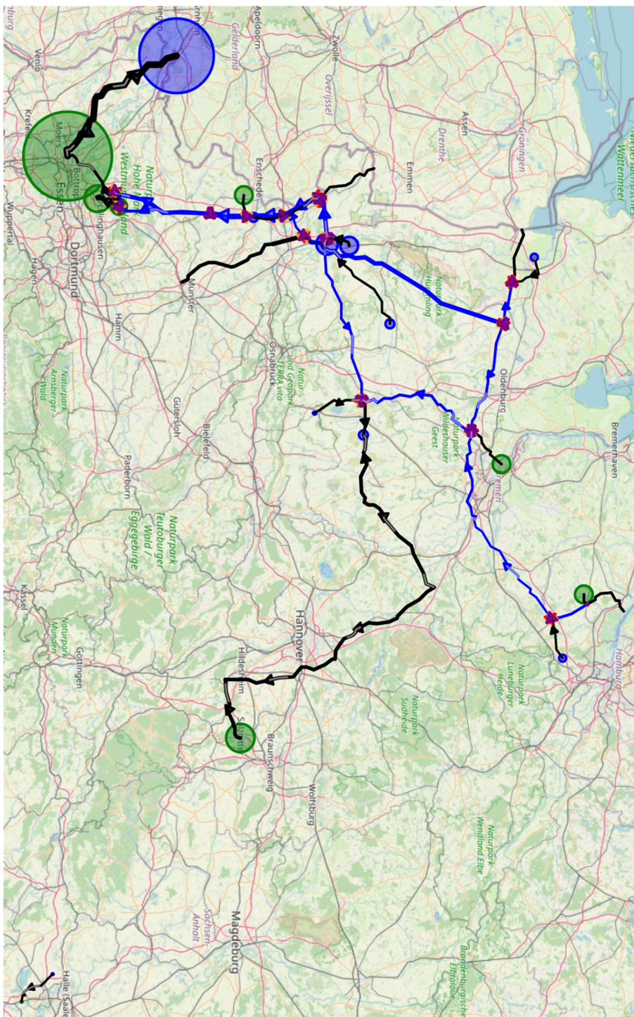
Abbildung I.8.9.2: Flüsse im 2030 Basisszenario bei 60 bar Maximaldruck und angenommener Rohrrauigkeit von 0,1 mm. Legende, siehe Tabelle I.8.1.1.
