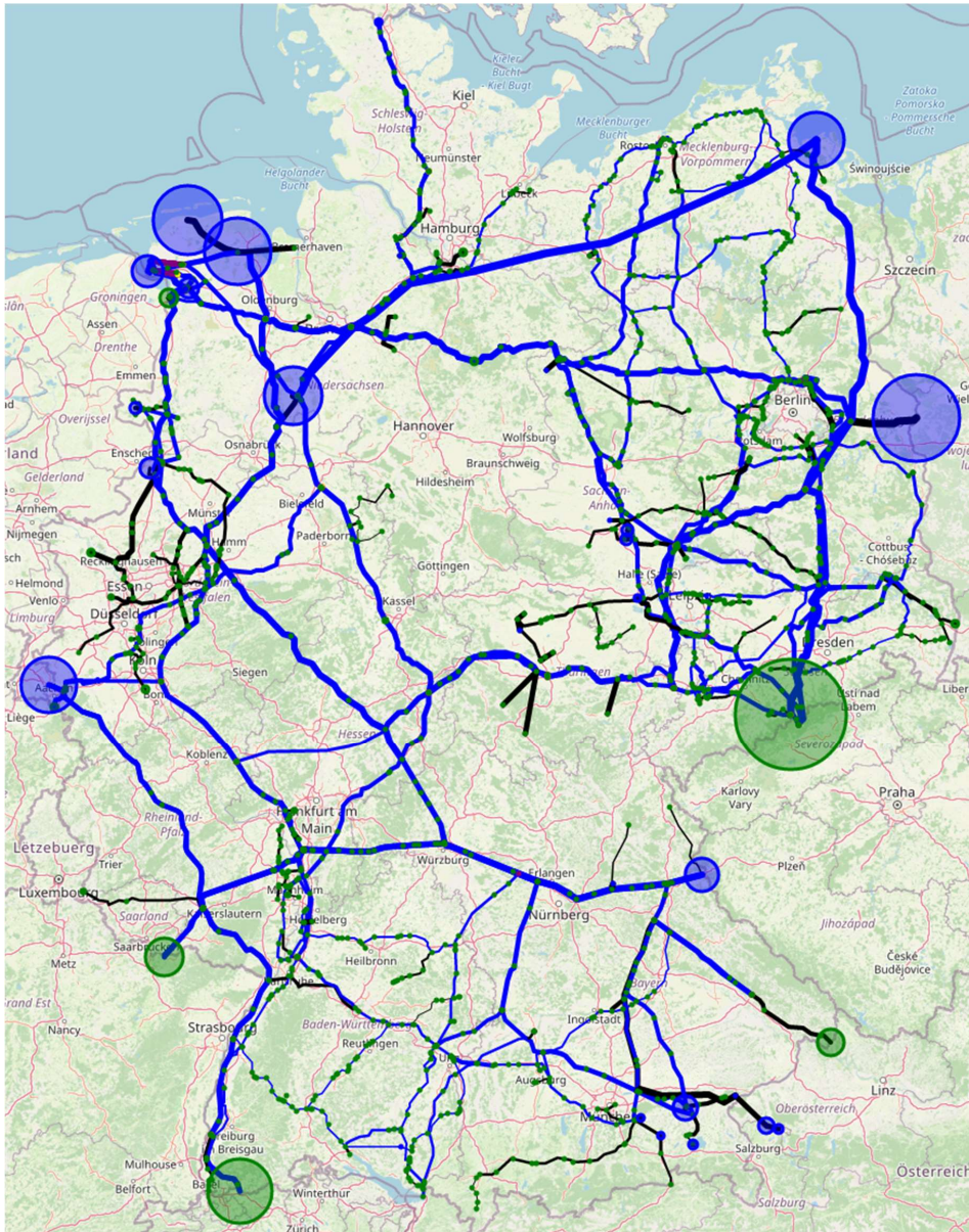
Abbildung 5.2.3.1: Ein-/Auspeisesituation der Erdgas-Nominierung des 06.02.2015 um 06:00 Uhr. Blaue Kreise repräsentieren Einspeisungen und grüne Kreise Auspeisungen. Ihre Größe ist proportional zur Größe der Ein-/Auspeisung. Die Dicke der Kanten ist proportional zum Durchmesser der jeweiligen Pipeline. Auf schwarz gefärbten Kanten (Pipelines) wurde der Fluss durch das Preprocessing auf einen festen Wert fixiert. Es ist darauf hinzuweisen, dass parallele Pipelinestränge aufgrund des Zoomlevels nicht erkennbar sind, aber abgebildet sind.
