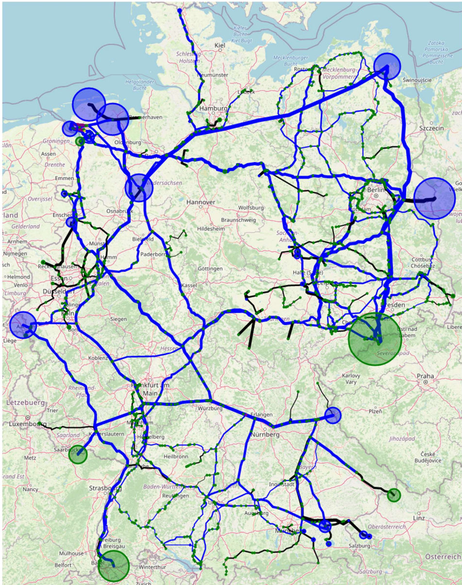
Abbildung I.8.18.1: Ein-/Auspeisesituation der Erdgas-Nominierung des 06.02.2015 um 06:00 Uhr. Blaue Kreise repräsentieren Einspeisungen und grüne Kreise Ausspeisungen. Ihre Größe ist proportional zur Größe der Ein-/Ausspeisung. Die Dicke der Kanten ist proportional zum Durchmesser der jeweiligen Pipeline. Auf schwarz gefärbten Kanten (Pipelines) wurde
