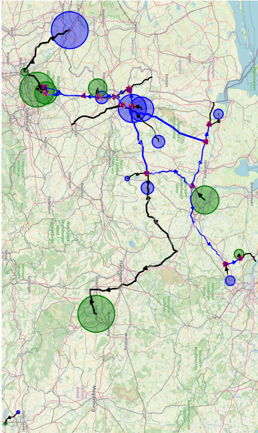
Abbildung I.8.12.2: Flüsse im Variation 1 Szenario 2030 bei 60 bar Maximaldruck und angenommener Rohrrauigkeit von 1 mm. Legende, siehe Tabelle I.8.1.1.
