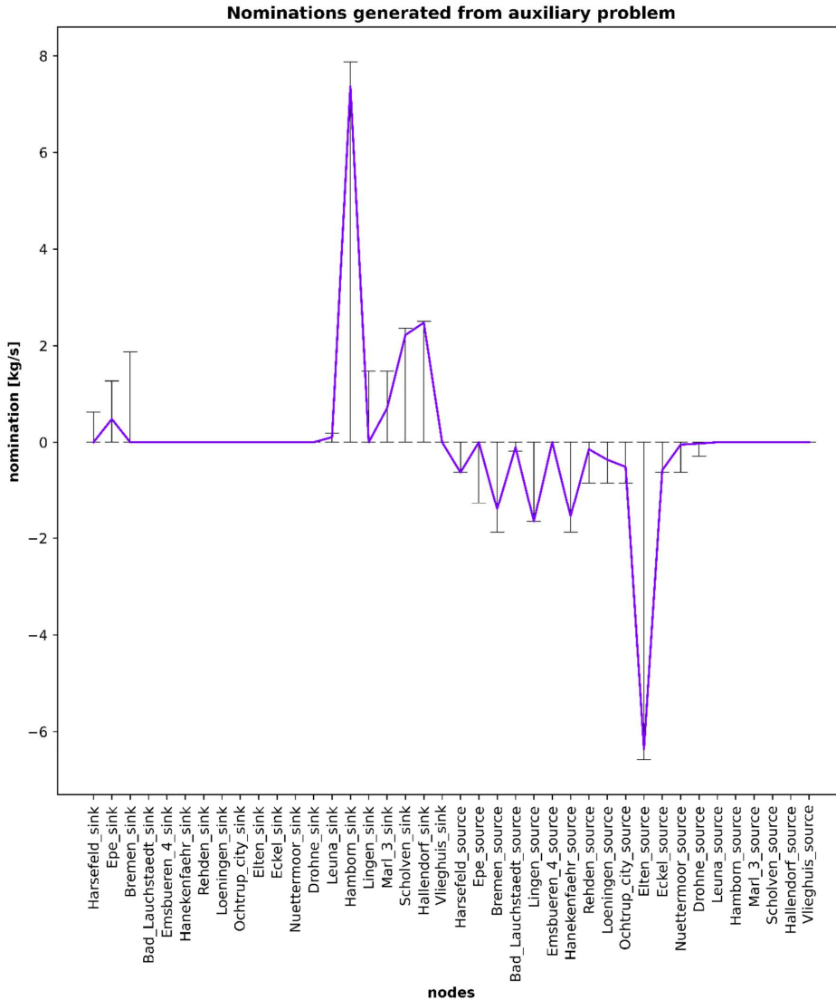
Abbildung 3.1.8.1: Beispielhafter Lastfall: Ein-/Ausspeiseintervalle mit darauf verorteten Lastflüssen. In diesem Beispiel wird eine Mindestnachfrage für jene Standorte angenommen, deren untere Intervallgrenze nicht auf der Nulllinie liegt. Hinweis zur Darstellung: Die Linienverbindung dient lediglich der verbesserten Sichtbarkeit, falls mehrere Lastfälle gleichzeitig abgebildet sind. Jeder Quellen-/Senkenknoten ist, analog zur Problemformulierung in Gl. 7.1 - Gl. 7.12, einmal als Senke (linke Hälfte) und einmal als Quelle (rechte Hälfte) aufgeführt.
