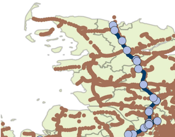
Abbildung 3.2.3.4: Verbesserte Einlastung flächenspezifischer Lasten unter Zuhilfenahme eines höher aufgelösten Datensatzes in Verbindung mit einer Breitensuche (BFS). Veranschaulichung der Knotenzuordnung auf Basis eines Zoom-Ausschnitts von Norddeutschland: 2. Schritt: Zuordnung der Knoten des reduzierten Netzwerkdatensatzes zu den nächsten Nachbarknoten des feinaufgelösten Netzwerks (Voronoi-Knoten).
