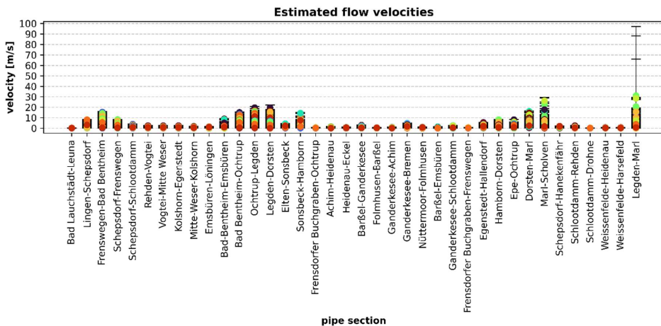
Abbildung 5.2.3.2: 200 Zufällige Lastfälle: Resultierende Fließgeschwindigkeiten bei Druckmaximierung im Netz mit 10% Optimality-Gap. Unterschiedliche Farben stehen für unterschiedliche Lastfälle. Kernpunkt ist jedoch, dass man erkennt, dass nur auf wenigen Pipelines die Geschwindigkeit stärker schwankt.
