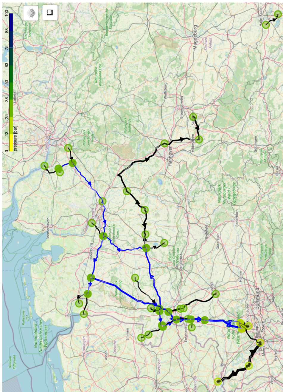
Abbildung I.8.7.3: Drücke im 2030 Basisszenario bei 30 bar Maximaldruck und angenommener Rohrrauigkeit von 0,1 mm. Legende, siehe Tabelle I.8.1.1.
