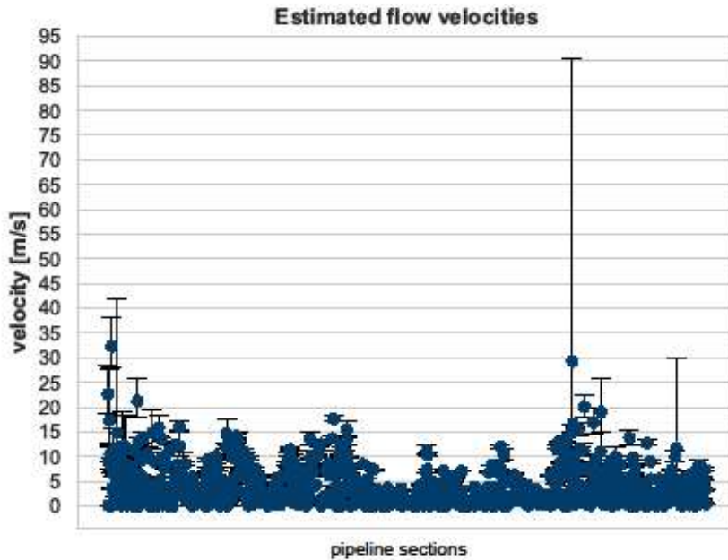
Abbildung 5.2.3.11: Durchschnittlich geschätzte Fließgeschwindigkeiten von Erdgas entlang der Pipelineabschnitte (x-Achse) am 02.12.2015 um 05:00 Uhr. Die Fehlerschranken kennzeichnen die Fließgeschwindigkeit am Ein- bzw. Austritt der Pipeline. Mit wenigen Ausnahmen liegen die Geschwindigkeiten unter 10 m/s. Bemerkenswert ist hier ein großer Ausreißer mit bis zu 90 m/s.
