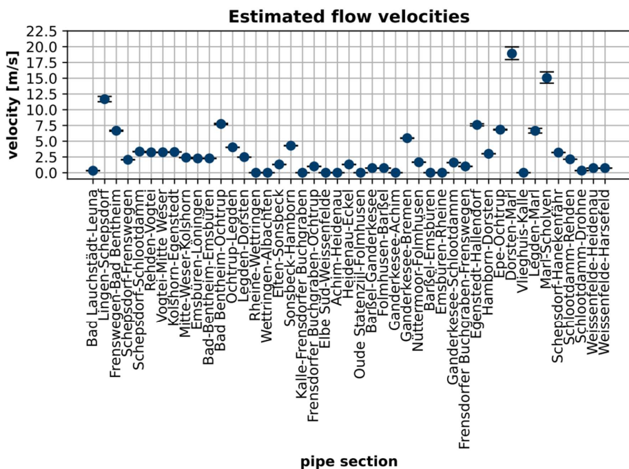
Abbildung I.8.10.1: Geschätzte Fließgeschwindigkeiten im Variation 1 Szenario 2030 (durchschnittlich) bei 30 bar Maximaldruck und angenommener Rohrrauigkeit von 1 mm. Die Fehlerschranken geben die Fließgeschwindigkeit am Pipelineeintritt bzw. am -austritt an.
