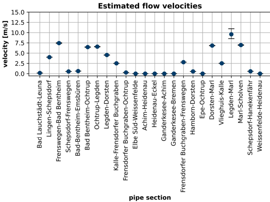
Abbildung 1.8.4.1: Geschätzte Fließgeschwindigkeiten im 2025 Basisszenario (durchschnittlich) bei 60 bar Maximaldruck und angenommener Rohrrauigkeit von 1 mm. Die Fehlerschranken geben die Fließgeschwindigkeit am Pipelineeintritt bzw. am -austritt an.
