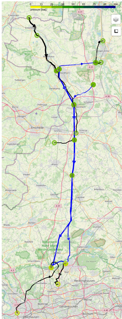
Abbildung 4.1.10.2: Flüsse und Drücke im Cluster West des Basisszenarios für das Jahr 2025. Die Drücke an den Netzknoten sind farblich entsprechend der Farbskala kodiert. Die Dicke einer Kante des Graphen ist proportional zum Fluss über die Kante. Einige Knoten erscheinen ausgefüllt, dies ist jedoch nur auf die Überlagerung von nahe beieinander liegenden Knoten zurückzuführen.
