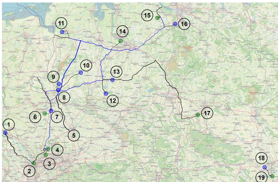
Abbildung 3.1.6.1: Überblick: Modellierter Wasserstoffnetzwerktopologie 2030. Blaue Kreise stehen für Quellen, und Grüne Kreise für Senken (siehe Tabelle 3.1.6.1). In dieser Darstellung dienen die Kreise lediglich der Verortung der Quellen und Senken und geben keinerlei Auskunft über Ein- oder Auspeisemengen.
