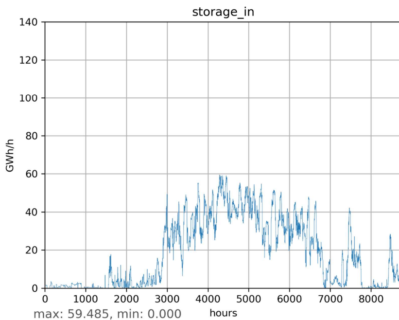
Abbildung 5.2.3.3: Sektorzeitreihe: Einspeicherung in Gasspeicher
