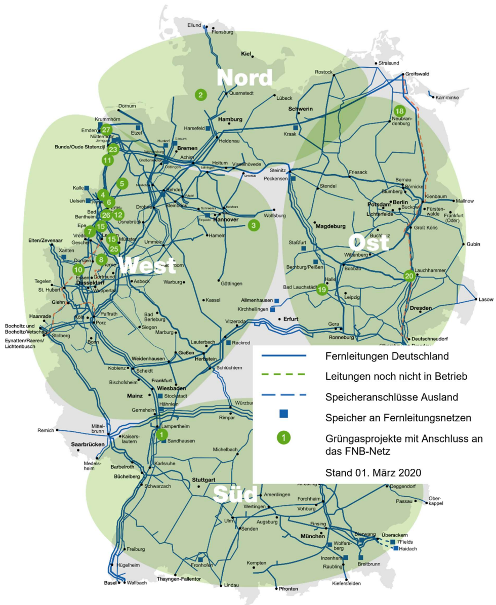
Abbildung 2.4.3.1: Bild: Cluster der Grüngasvariante im NEP-Gas 2020 [7]. Quelle: FNB Gas e.V.
