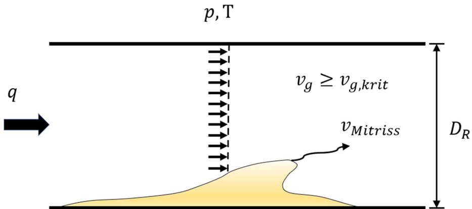
Abbildung 2.2.4.3: Eigene Darstellung nach [52]: Mitriss von Staubpartikeln und Flüssigkeitstropfen. q : Fluss, p : Druck, T : Temperatur, v_g : Gasgeschwindigkeit, v_{g,krit} : kritische Gasgeschwindigkeit für den Mitriss, v_{Mitriss} : Partikel-/Tropfengeschwindigkeit
