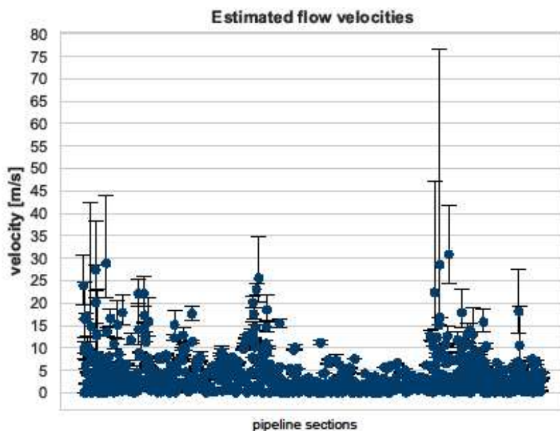
Abbildung 5.2.3.6: Durchschnittlich geschätzte Fließgeschwindigkeiten von Erdgas entlang der Pipelineabschnitte (x-Achse) am 06.02.2015 um 06:00 Uhr. Die Fehlerschranken kennzeichnen die Fließgeschwindigkeit am Ein- bzw. Austritt der Pipeline. Mit wenigen Ausnahmen liegen die Geschwindigkeiten unter 15 m/s bzw. unter 10 m/s.
