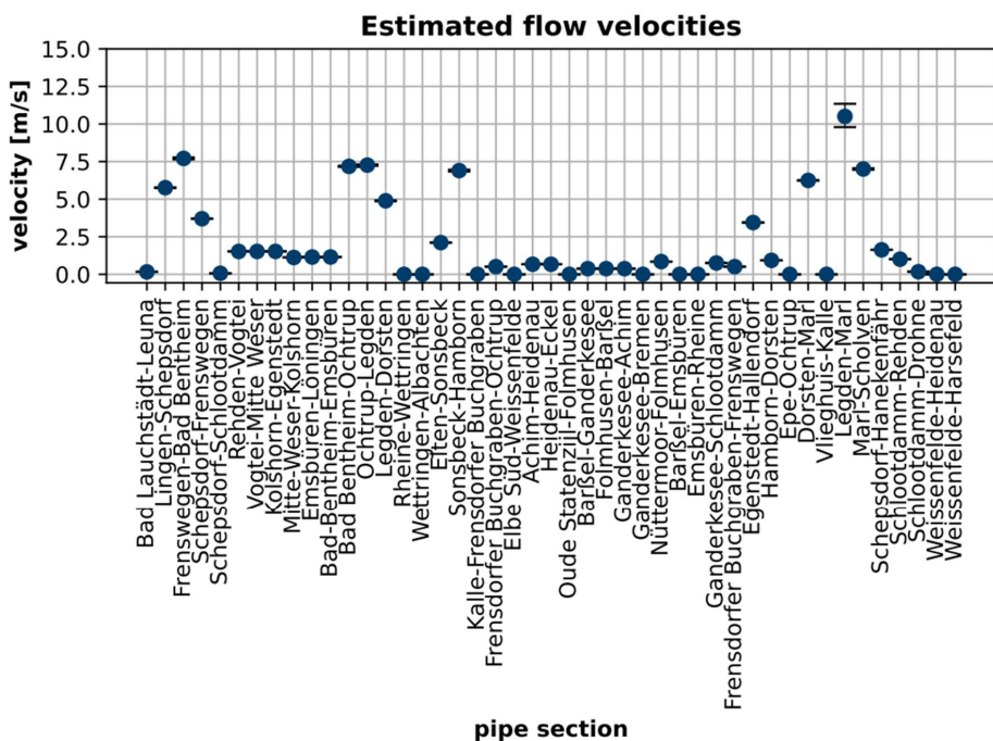
Abbildung 1.8.9.1: Geschätzte Fließgeschwindigkeiten im 2030 Basisszenario (durchschnittlich) bei 60 bar Maximaldruck und angenommener Rohrrauigkeit von 0,1 mm. Die Fehlerschranken geben die Fließgeschwindigkeit am Pipelineeintritt bzw. am -austritt an.
