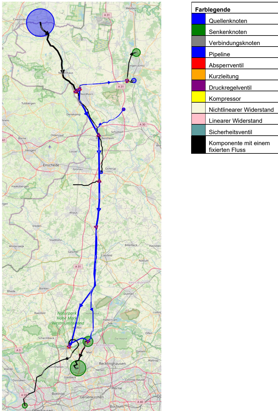
Abbildung 4.1.10.1: Flüsse im Cluster West des Basisszenarios für das Jahr 2025. Die Ein-/Auspeisemengen sind als Kreise dargestellt und relativ zueinander skaliert. Quellen sind blau gefärbt und Senken grün. Die jeweilige Ein-/Auspeisemenge ist proportional zum Kreisdurchmesser. Die Dicke einer Kante des Graphen ist proportional zum Fluss über die Kante. Die größte Einspeisung hier liegt bei 3,52 kg/s in Vlieghuis.
