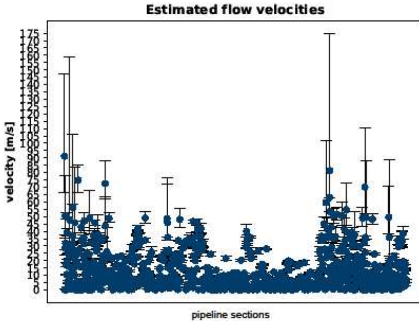
Abbildung 5.2.3.15: Durchschnittlich geschätzte Fließgeschwindigkeiten von Wasserstoff entlang der Pipelineabschnitte (x-Achse) am 27.11.2015 um 17:00 Uhr. Die Fehlerschranken kennzeichnen die Fließgeschwindigkeit am Ein- bzw. Austritt der Pipeline. Mit wenigen Ausnahmen liegen die Geschwindigkeiten unter 45 m/s bzw. unter 25 m/s. Die maximal erreichte Fließgeschwindigkeit liegt hier bei 175 m/s.
