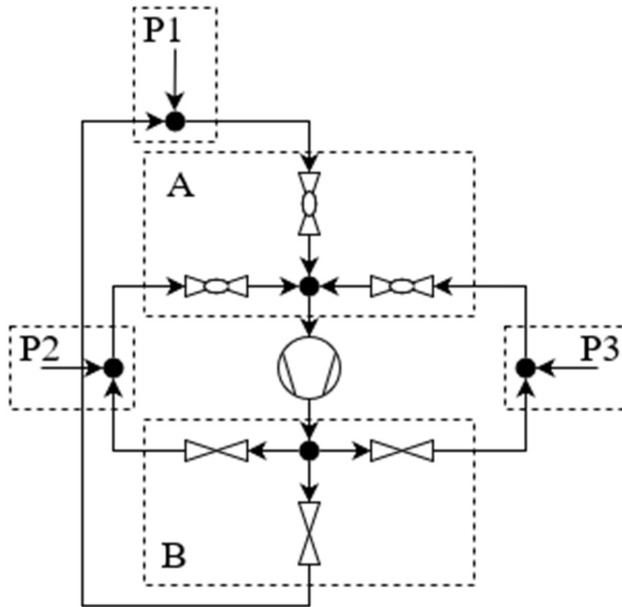
Abbildung 4.1.9.2: Vereinfachte Darstellung von Verdichterstationen mit Peripherie als Verknüpfung zweier Sternschaltungen aus Druckregelventilen auf der Eingangsseite und Absperrventilen auf der Ausgangsseite. Hier beispielhaft für 3 angeschlossene Pipelines P1-P3; A: Eingangssternschaltung aus Druckregelventilen; B: Ausgangssternschaltung aus Absperrventilen.
