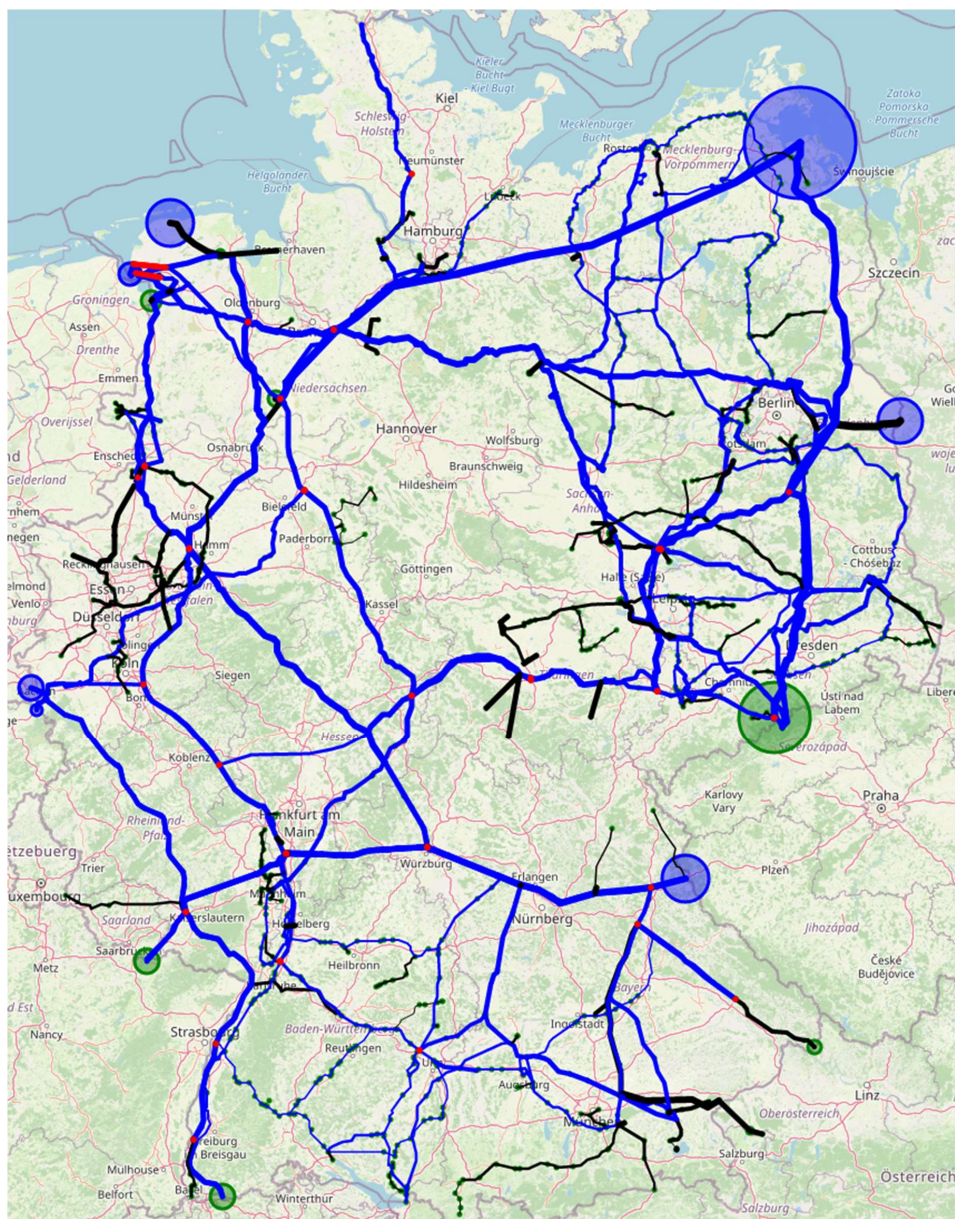
Abbildung I.8.18.4: Ein-/Auspeisesituation der Erdgas-Nominierung des 04.07.2015 um 00:00 Uhr. Blaue Kreise repräsentieren Einspeisungen und grüne Kreise Auspeisungen. Ihre Größe ist proportional zur Größe der Ein-/Auspeisung. Die Dicke der Kanten ist proportional zum Durchmesser der jeweiligen Pipeline. Auf schwarz gefärbten Kanten (Pipelines) wurde der Fluss durch das Preprocessing auf einen festen Wert fixiert. Es ist darauf hinzuweisen, dass parallele Pipelinestränge aufgrund des Zoomlevels nicht erkennbar sind, aber abgebildet sind. Legende, siehe Tabelle I.8.1.1.
