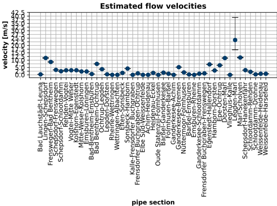
Abbildung 5.2.2.2: Geschätzte Fließgeschwindigkeiten im Variation 1 Szenario 2030 (durchschnittlich) bei 30 bar Maximaldruck und angenommener Rohrrauigkeit von 0.1 mm. Die Fehlerschranken geben die Fließgeschwindigkeit am Pipelineintritt bzw. am -austritt an.
