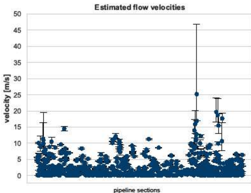
Abbildung 5.2.3.8: Durchschnittlich geschätzte Fließgeschwindigkeiten von Erdgas entlang der Pipelineabschnitte (x-Achse) am 11.08.2015 um 15:00 Uhr. Die Fehlerschranken kennzeichnen die Fließgeschwindigkeit am Ein- bzw. Austritt der Pipeline. Mit wenigen Ausnahmen liegen die Geschwindigkeiten unter 10 m/s bzw. unter 5 m/s.
