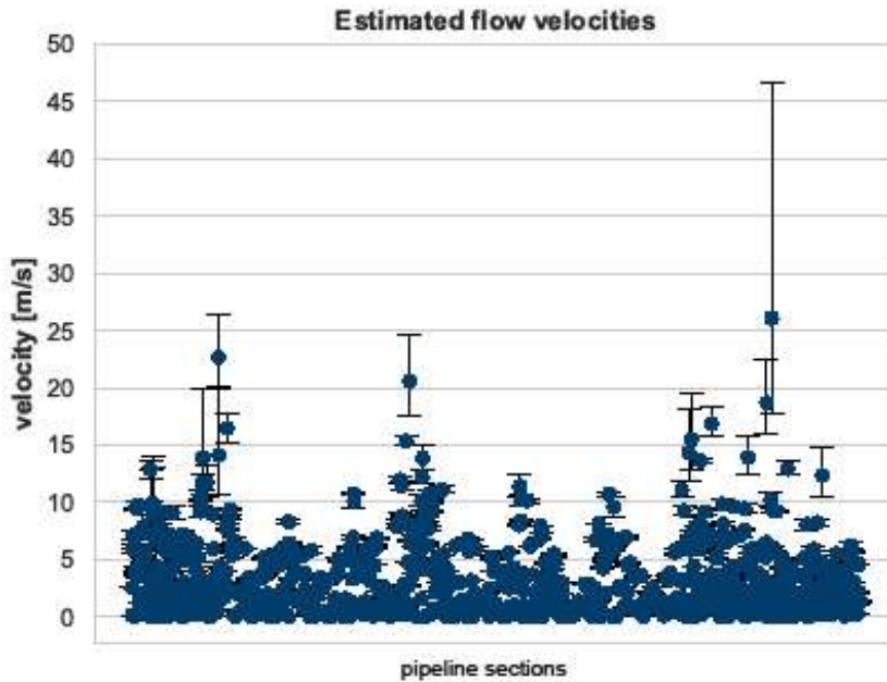
Abbildung 5.2.3.9: Durchschnittlich geschätzte Fließgeschwindigkeiten von Erdgas entlang der Pipelineabschnitte (x-Achse) am 17.08.2015 um 09:00 Uhr. Die Fehlerschranken kennzeichnen die Fließgeschwindigkeit am Ein- bzw. Austritt der Pipeline. Mit wenigen Ausnahmen liegen die Geschwindigkeiten unter 10 m/s.
