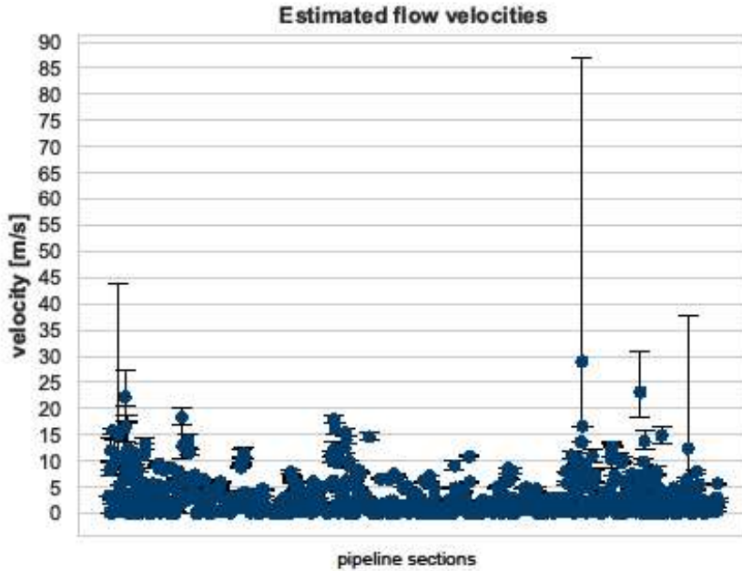
Abbildung 5.2.3.7: Durchschnittlich geschätzte Fließgeschwindigkeiten von Erdgas entlang der Pipelineabschnitte (x-Achse) am 04.07.2015 um 00:00 Uhr. Die Fehlerschranken kennzeichnen die Fließgeschwindigkeit am Ein- bzw. Austritt der Pipeline. Mit wenigen Ausnahmen liegen die Geschwindigkeiten unter 10 m/s bzw. unter 5 m/s. Bemerkenswert ist hier ein großer Ausreißer mit bis zu 87 m/s.
