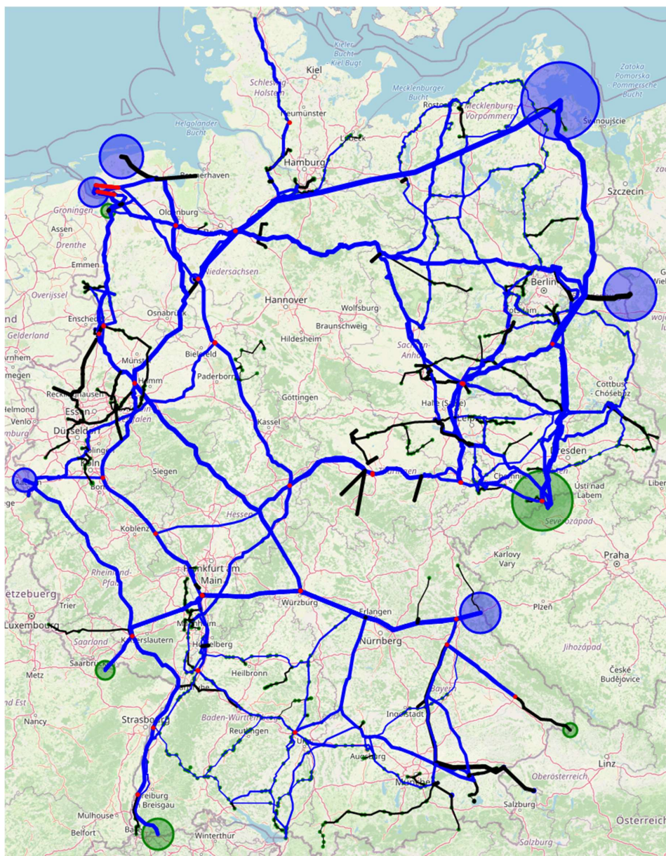
Abbildung I.8.18.13: Ein-/Auspeisesituation der Erdgas-Nominierung des 27.11.2015 um 17:00 Uhr. Blaue Kreise repräsentieren Einspeisungen und grüne Kreise Auspeisungen. Ihre Größe ist proportional zur Größe der Ein-/Auspeisung. Die Dicke der Kanten ist proportional zum Durchmesser der jeweiligen Pipeline. Auf schwarz gefärbten Kanten (Pipelines) wurde der Fluss durch das Preprocessing auf einen festen Wert fixiert. Es ist darauf hinzuweisen, dass parallele Pipelinestränge aufgrund des Zoomlevels nicht erkennbar sind, aber abgebildet sind. Legende, siehe Tabelle I.8.1.1.
