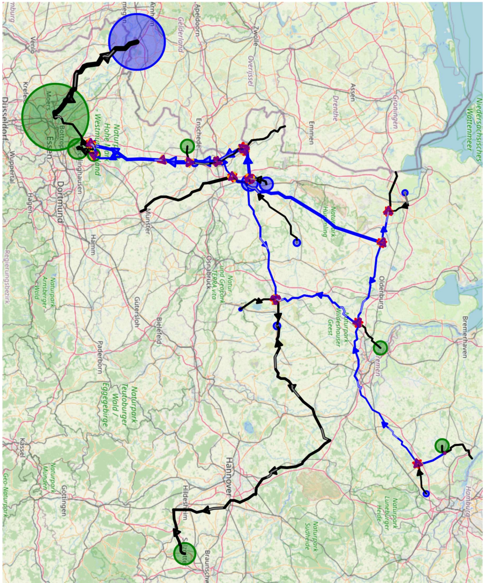
Abbildung I.8.8.2: Flüsse im 2030 Basisszenario bei 60 bar Maximaldruck und angenommener Rohrrauigkeit von 1 mm. Legende, siehe Tabelle I.8.1.1.
