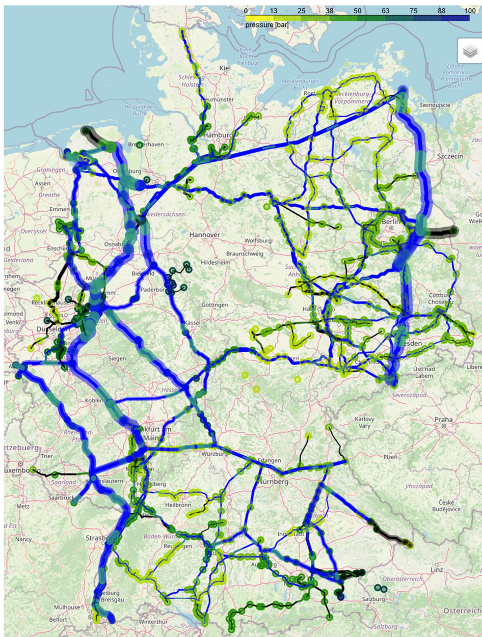
Abbildung I.8.18.2: Flüsse und Drücke in der Erdgas-Nominierung des 06.02.2015 um 06:00 Uhr. Die Drücke an den Knoten sind entsprechend des dargestellten Farbcodes (oben rechts) eingefärbt. Die Dicke der Kanten ist proportional zum Fluss darüber. Legende, siehe Tabelle I.8.1.1.
