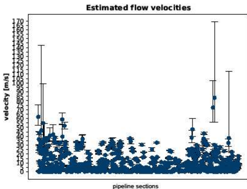
Abbildung 5.2.3.12: Durchschnittlich geschätzte Fließgeschwindigkeiten von Wasserstoff entlang der Pipelineabschnitte (x-Achse) am 04.07.2015 um 00:00 Uhr. Die Fehlerschranken kennzeichnen die Fließgeschwindigkeit am Ein- bzw. Austritt der Pipeline. Mit wenigen Ausnahmen liegen die Geschwindigkeiten unter 35 m/s. Die maximal erreichte Fließgeschwindigkeit liegt hier bei 168 m/s.
