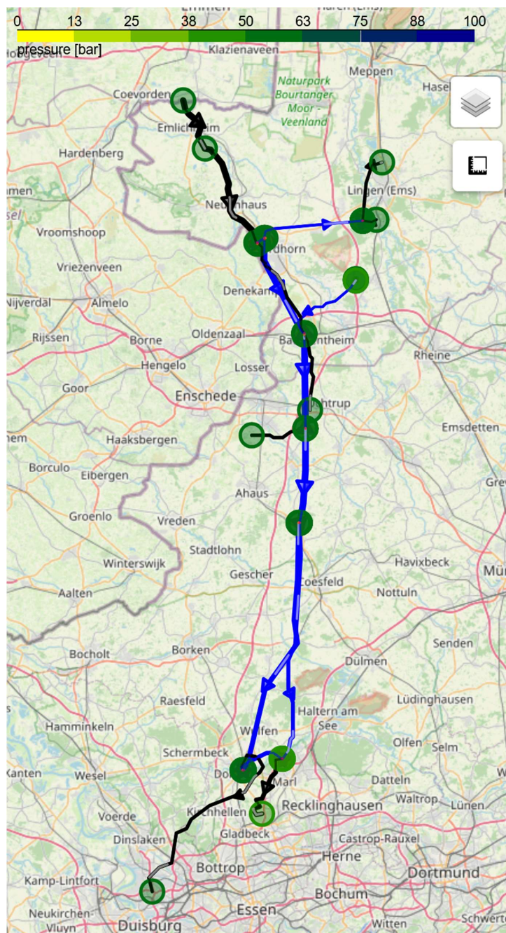
Abbildung I.8.5.3: Drücke im 2025 Basisszenario bei 60 bar Maximaldruck und angenommener Rohrrauigkeit von 0,1 mm. Legende, siehe Tabelle I.8.1.1.
