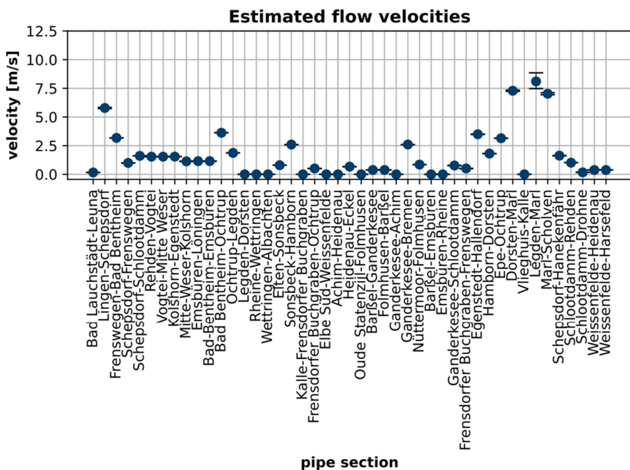
Abbildung I.8.12.1: Geschätzte Fließgeschwindigkeiten im Variation 1 Szenario 2030 (durchschnittlich) bei 60 bar Maximaldruck und angenommener Rohrrauigkeit von 1 mm. Die Fehlerschranken geben die Fließgeschwindigkeit am Pipelineeintritt bzw. am -austritt an.
