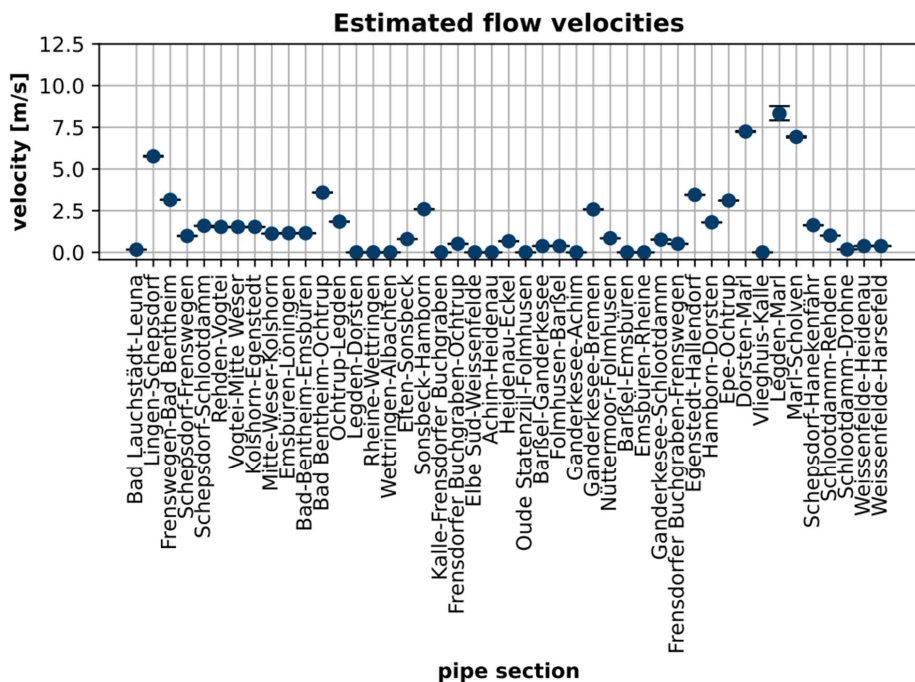
Abbildung I.8.13.1: Geschätzte Fließgeschwindigkeiten im Variation 1 Szenario 2030 (durchschnittlich) bei 60 bar Maximaldruck und angenommener Rohrrauigkeit von 0,1 mm. Die Fehlerschranken geben die Fließgeschwindigkeit am Pipelineintritt bzw. am - austritt an.
