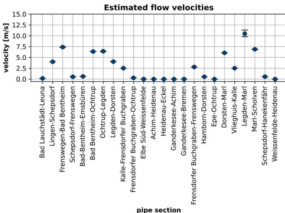
Abbildung 4.1.10.4: Geschätzte Fließgeschwindigkeiten im 2025 Basisszenario (durchschnittlich) bei 60 bar Maximaldruck und angenommener Rohrrauigkeit von 0,1 mm. Die Fehlerschranken geben die Fließgeschwindigkeit am Pipelineeintritt bzw. am -austritt an.
