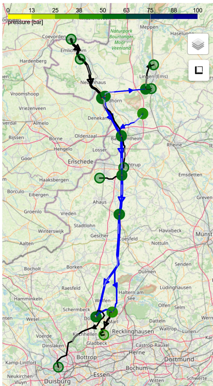
Abbildung I.8.4.3: Drücke im 2025 Basisszenario bei 60 bar Maximaldruck und angenommener Rohrrauigkeit von 1 mm. Legende, siehe Tabelle I.8.1.1.
