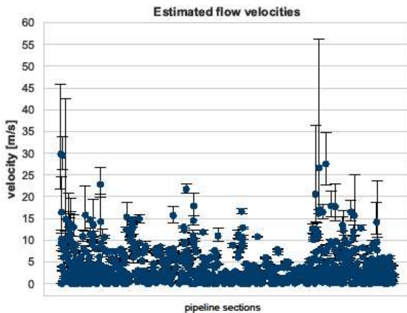
Abbildung 5.2.3.10: Durchschnittlich geschätzte Fließgeschwindigkeiten von Erdgas entlang der Pipelineabschnitte (x-Achse) am 27.11.2015 um 17:00 Uhr. Die Fehlerschranken kennzeichnen die Fließgeschwindigkeit am Ein- bzw. Austritt der Pipeline. Mit wenigen Ausnahmen liegen die Geschwindigkeiten unter 10 m/s.
