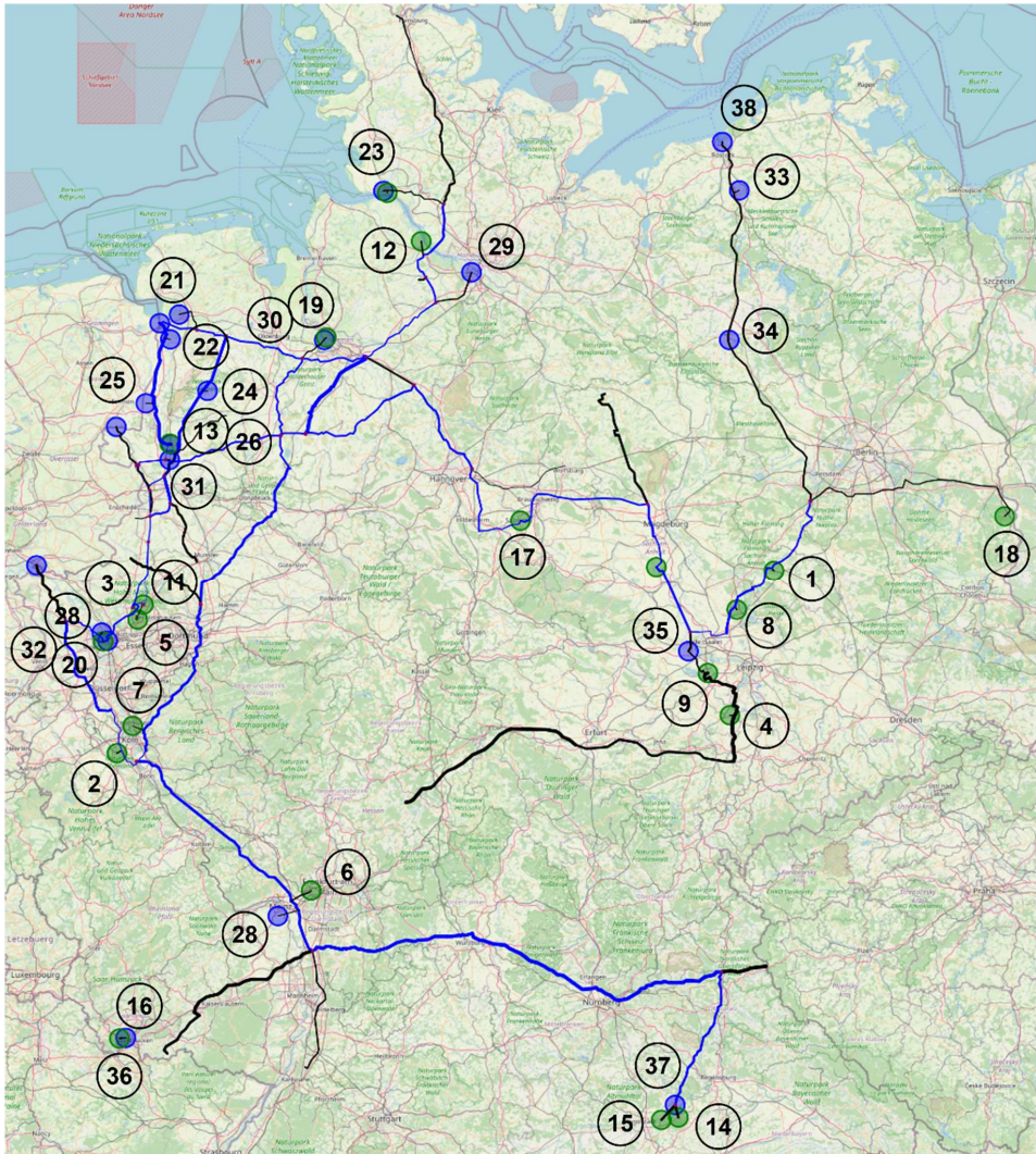
Abbildung 3.1.9.1: Überblick: Modellierter Wasserstoffnetzwerktopologie 2030 ([114]) gemäß Entwurf Szenariorahmen NEP-Gas 2022 (Stand Juni 2022). Blaue Kreise stehen für Quellen, und grüne Kreise für Senken, wobei in dieser Darstellung die Kreise lediglich der Verortung der Quellen und Senken dienen und keinerlei Auskunft über Ein- oder Ausspeisemengen geben. Die Nummerierung der Quellen und Senken entspricht der „Id“-Spalte aus Tabelle 3.1.9.1, Tabelle 3.1.9.2 und Tabelle 3.1.9.3.
