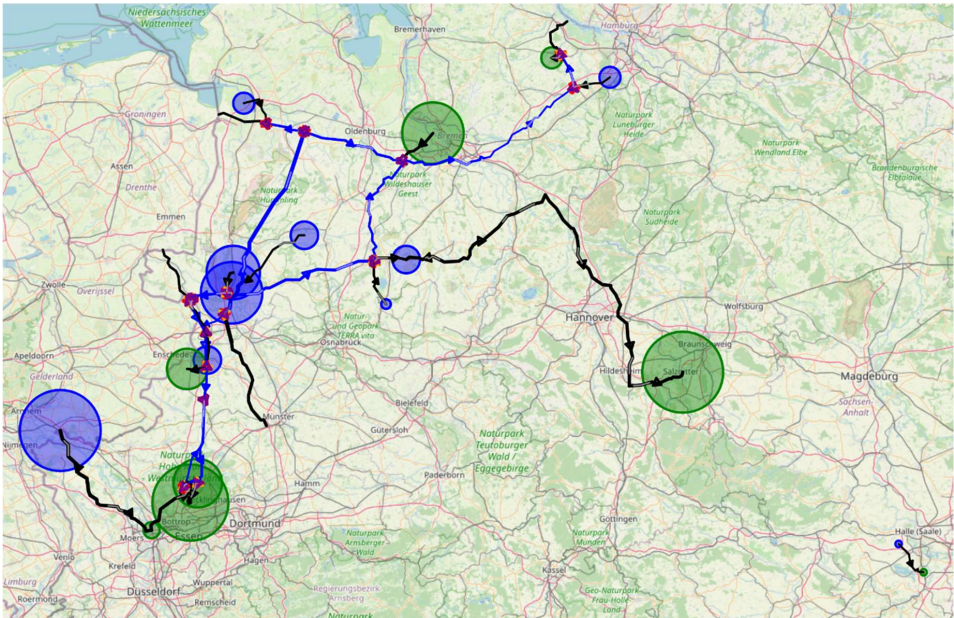
Abbildung 5.2.2.1: Flüsse im Variation 1 Szenario 2030 bei 30 bar Maximaldruck und angenommener Rohrrauigkeit von 0,1 mm. Die Ein-/Auspeisemengen sind als Kreise dargestellt und relativ zueinander skaliert. Die jeweilige Ein-/Auspeisemenge ist proportional zum Kreisdurchmesser. Quellen sind blau gefärbt und Senken grün. Die Dicke einer Kante des Graphen ist proportional zum Fluss über die Kante. Die größte Auspeisung hier liegt bei 2,11 kg/s in Hallendorf (Salzgitter Flachstahl). Zum Vergleich siehe auch Tabelle 5.2.2.2.
