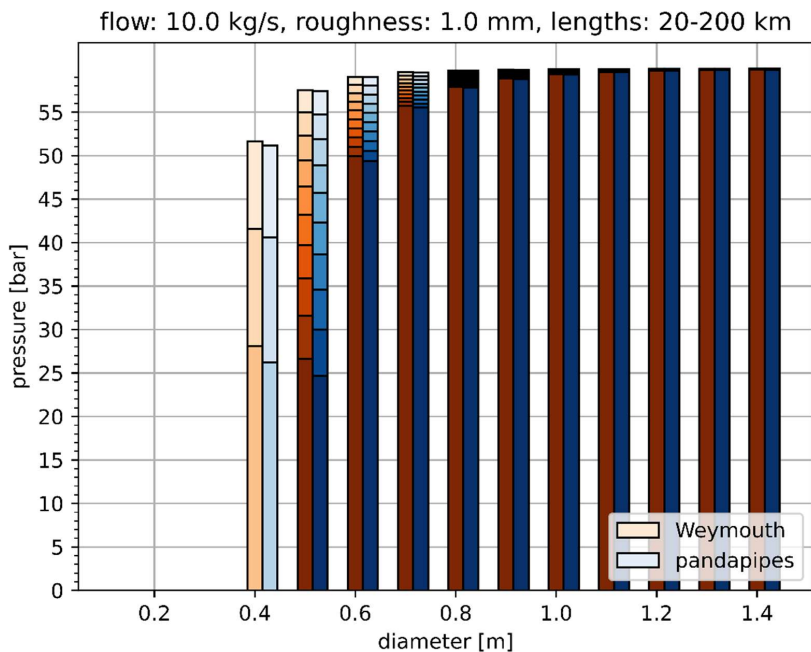
Abbildung 4.1.10.3: Vergleich Druckabfall Gleichung Gl. 4.3 gegenüber pandapipes: Fluss 10 kg/s Wasserstoff, Rohrrauigkeit 1 mm, Eingangsdruck 60 bar. Variiert über den Rohrdurchmesser (x-Achse, 100 mm Schritte) und über die Rohrlänge (Bildtiefe, 20 km Schritte).
