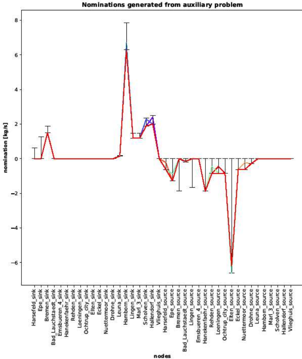
Abbildung 5.2.3.7: 200 Zufällige Lastfälle mit angesetzten Ein-/Ausspeiseintervallen und einer zu deckenden Mindestnachfrage von 80% der jeweiligen maximalen Ausspeisung bei der Industrie.
