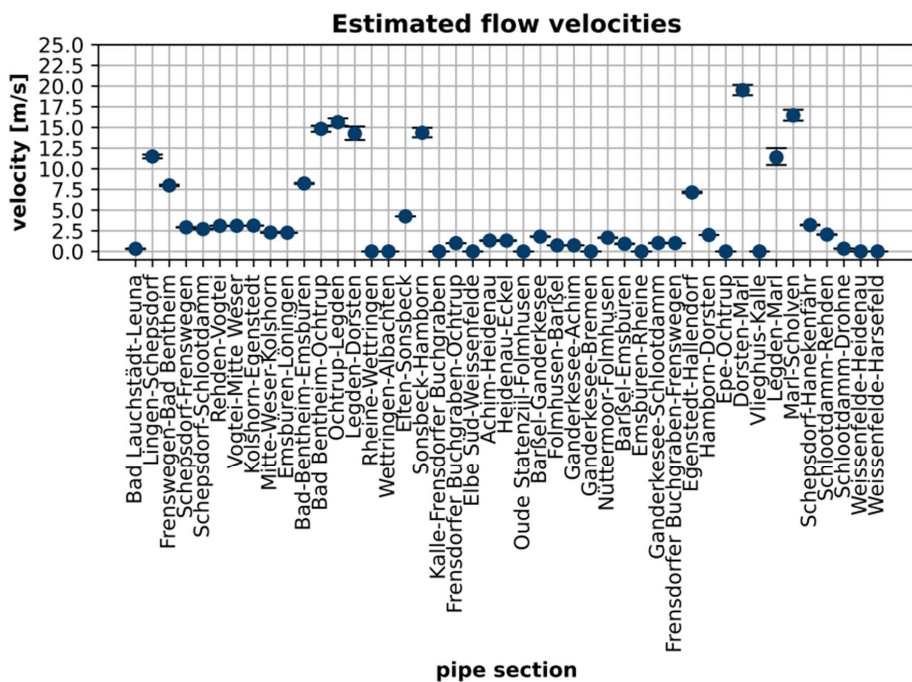
Abbildung I.8.7.1: Geschätzte Fließgeschwindigkeiten im 2030 Basisszenario (durchschnittlich) bei 30 bar Maximaldruck und angenommener Rohrrauigkeit von 0,1 mm. Die Fehlerschranken geben die Fließgeschwindigkeit am Pipelineintritt bzw. am -austritt an.
