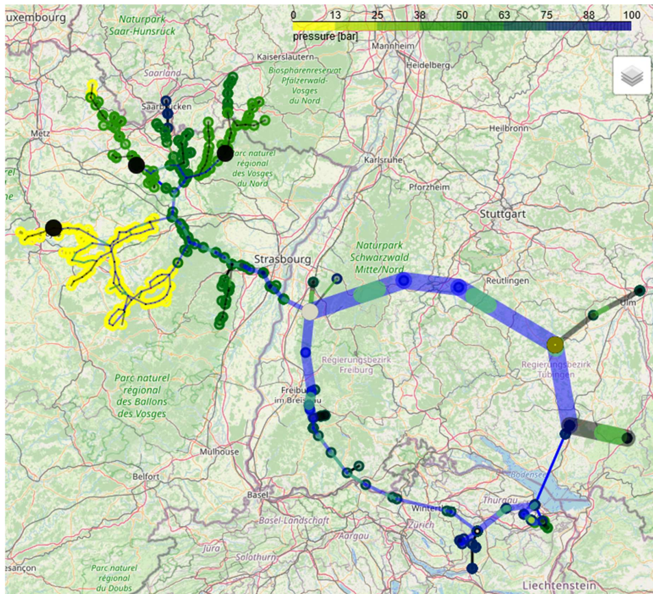
Abbildung 4.1.10.1: Beispiel-Plot für das Ergebnis einer Nominierung im GasLib-582-v2 Benchmark-Netzwerk. Die Druckverteilung über die Knoten, gemäß der Farbkennung, ist klar erkennbar. Die Dicke der dargestellten Kanten ist proportional zum Fluss über die jeweilige Kante.
