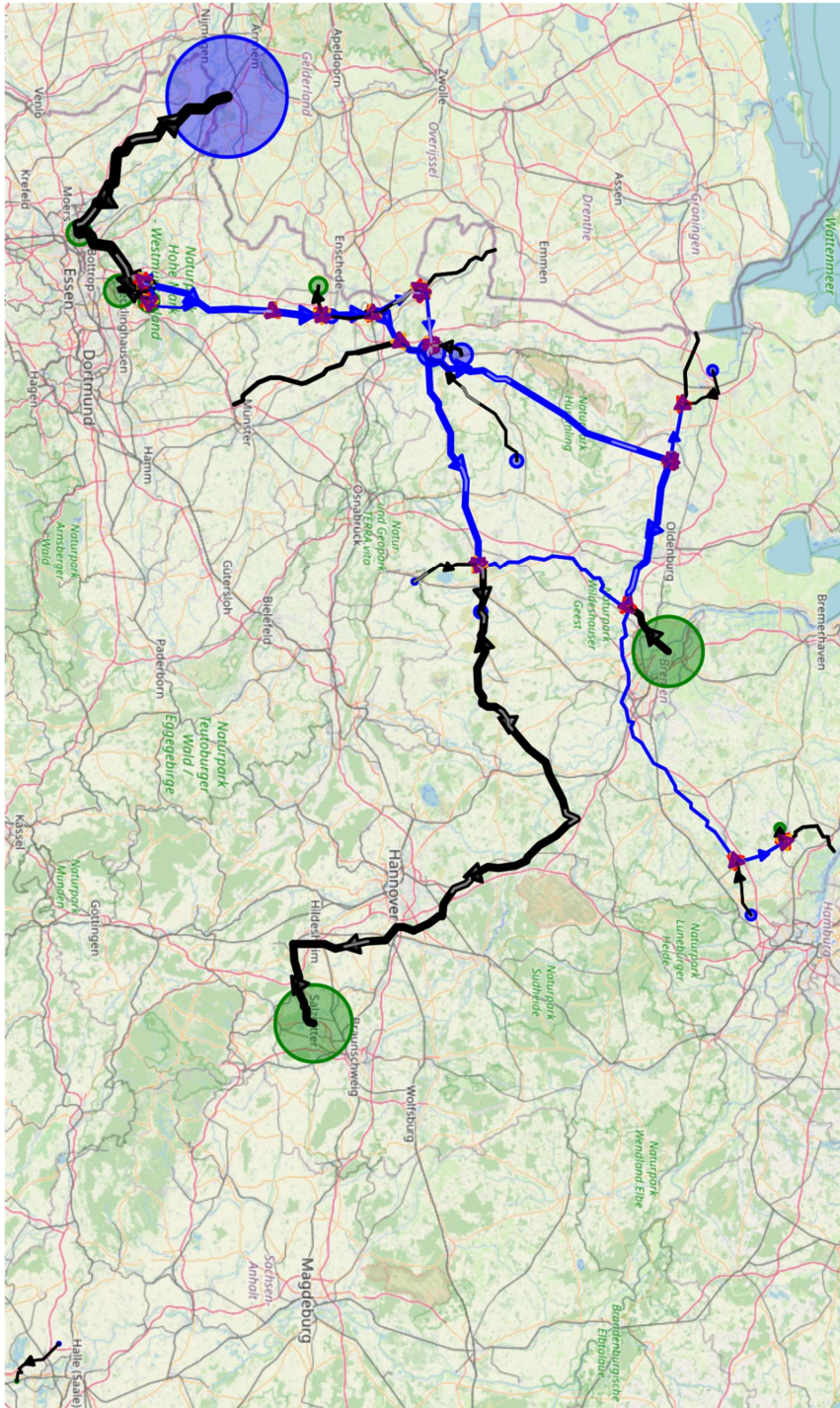
Abbildung I.8.17.2: Flüsse im Variation 2 Szenario 2030 bei 60 bar Maximaldruck und angenommener Rohrrauigkeit von 0,1 mm. Legende, siehe Tabelle I.8.1.1.
