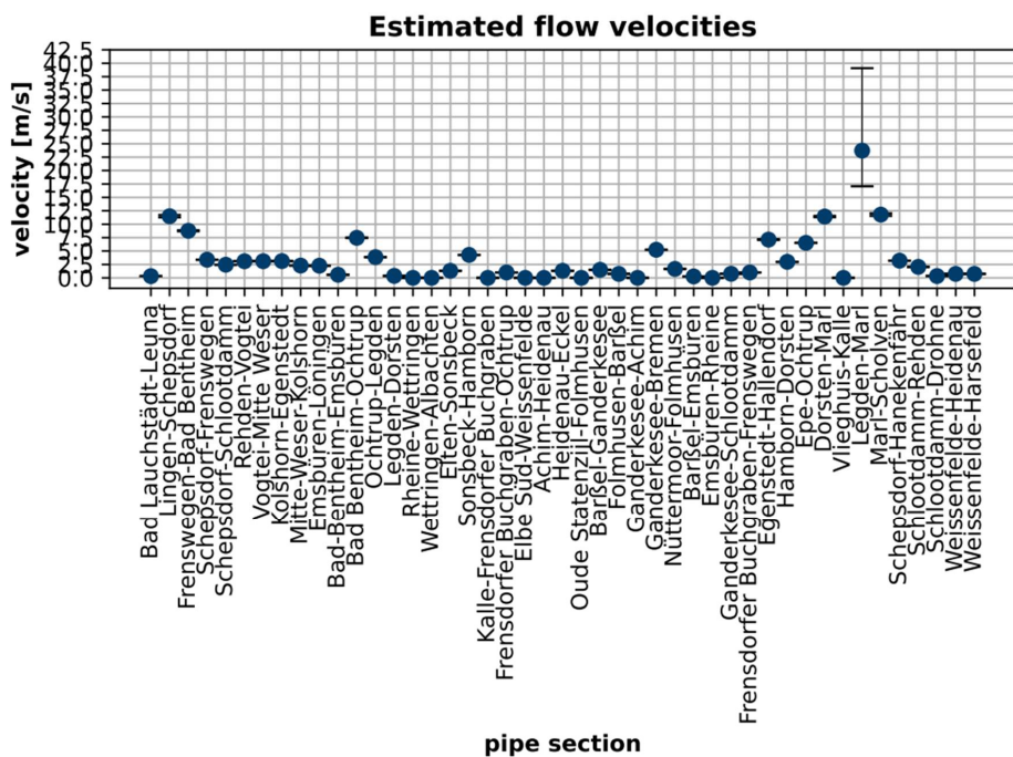
Abbildung I.8.11.1: Geschätzte Fließgeschwindigkeiten im Variation 1 Szenario 2030 (durchschnittlich) bei 30 bar Maximaldruck und angenommener Rohrrauigkeit von 0,1 mm. Die Fehlerschranken geben die Fließgeschwindigkeit am Pipelineintritt bzw. am -austritt an.
