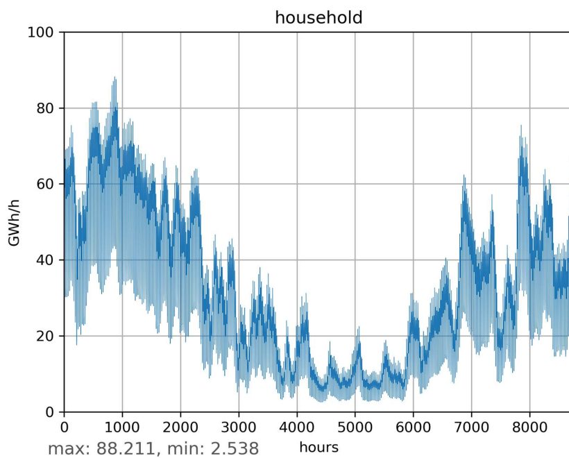
Abbildung 5.2.3.1: Sektorzeitreihe: Energienachfrage Haushalt
