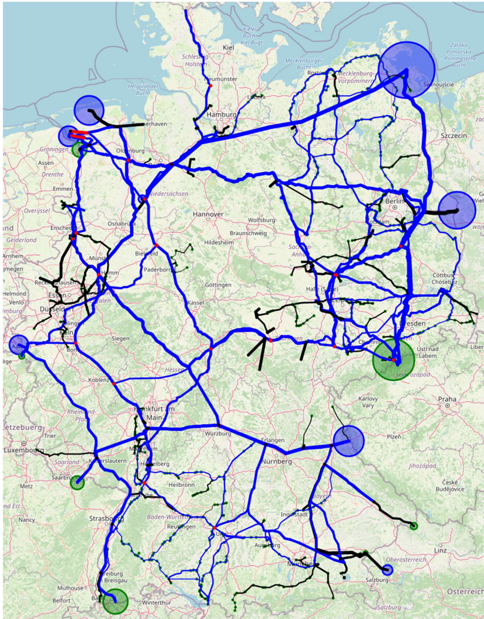
Abbildung 5.2.3.3: Ein-/Auspeisesituation der Erdgas-Nominierung des 02.12.2015 um 05:00 Uhr. Blaue Kreise repräsentieren Einspeisungen und grüne Kreise Ausspeisungen. Ihr Durchmesser ist proportional zur Größe der Ein-/Ausspeisung. Die Dicke der Kanten ist proportional zum Durchmesser der jeweiligen Pipeline. Auf schwarz gefärbten Kanten (Pipelines) wurde der Fluss durch das Preprocessing auf einen festen Wert fixiert. Es ist darauf hinzuweisen, dass parallele Pipelinestränge aufgrund des Zoomlevels nicht erkennbar sind, aber abgebildet sind.
