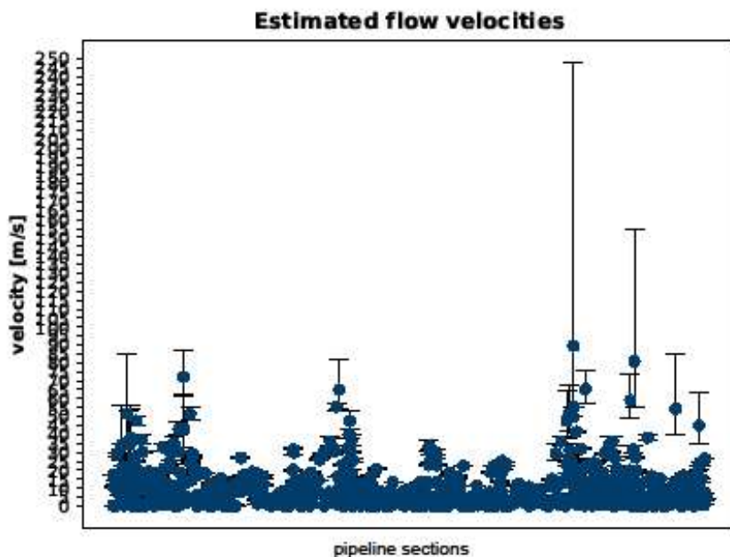
Abbildung 5.2.3.14: Durchschnittlich geschätzte Fließgeschwindigkeiten von Wasserstoff entlang der Pipelineabschnitte (x-Achse) am 17.08.2015 um 09:00 Uhr. Die Fehlerschranken kennzeichnen die Fließgeschwindigkeit am Ein- bzw. Austritt der Pipeline. Mit wenigen Ausnahmen liegen die Geschwindigkeiten unter 25 m/s. Die maximal erreichte Fließgeschwindigkeit liegt hier bei 248 m/s.
