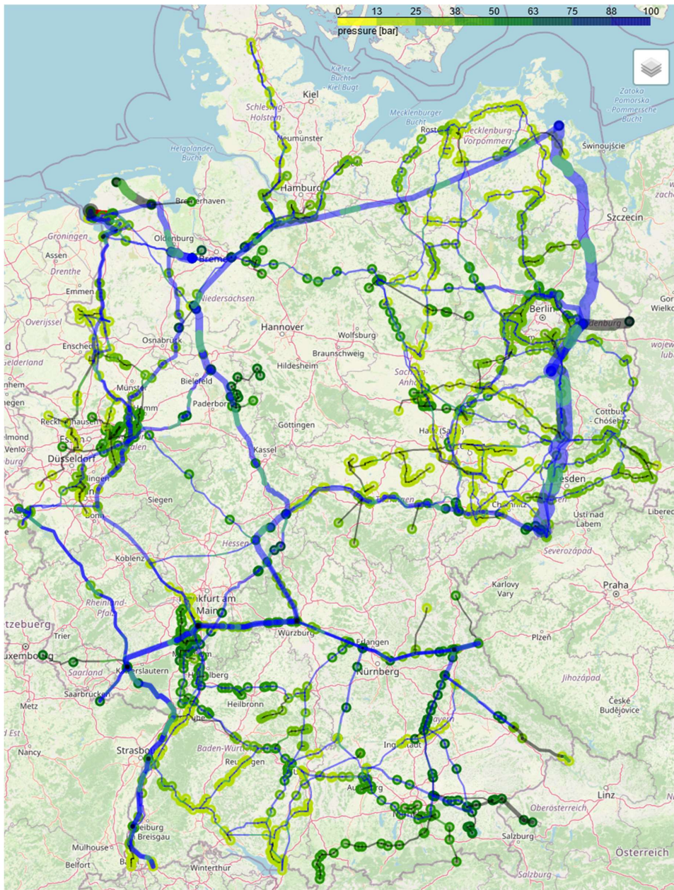
Abbildung 5.2.3.5: Flüsse und Drücke in der Wasserstoff-Nominierung des 02.12.2015 um 05:00 Uhr. Die Drücke an den Knoten sind entsprechend des dargestellten Farbcodes (oben rechts) eingefärbt. Die Dicke der Kanten ist proportional zum Fluss darüber.
