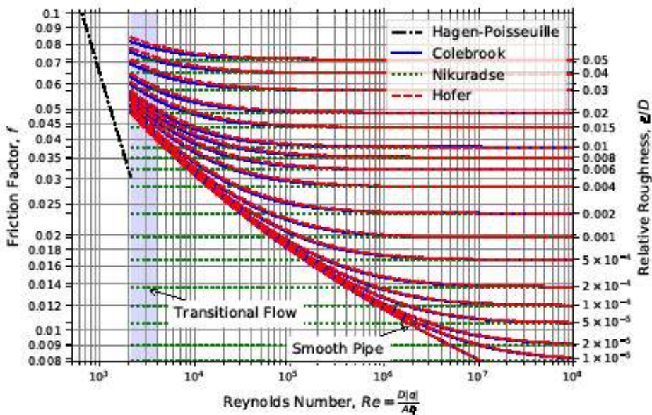
Abbildung 4.1.10.1: Eigene Darstellung: Moody-Diagramm: Darstellung des Druckverlustkoeffizienten (y-Achse links) in Abhängigkeit der Reynoldszahl (x-Achse) und der relativen Rauigkeit (y-Achse rechts) für verschiedene Modelle (Hagen-Poiseuille (laminar), Nikuradse ( Re \rightarrow \infty ), Hofer (explizit), Colebrook-White (implizit)).
