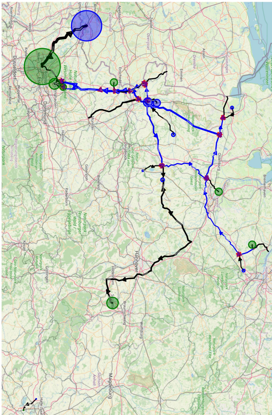
Abbildung I.8.7.2: Flüsse im 2030 Basisszenario bei 30 bar Maximaldruck und angenommener Rohrrauigkeit von 0,1 mm. Legende, siehe Tabelle I.8.1.1.
