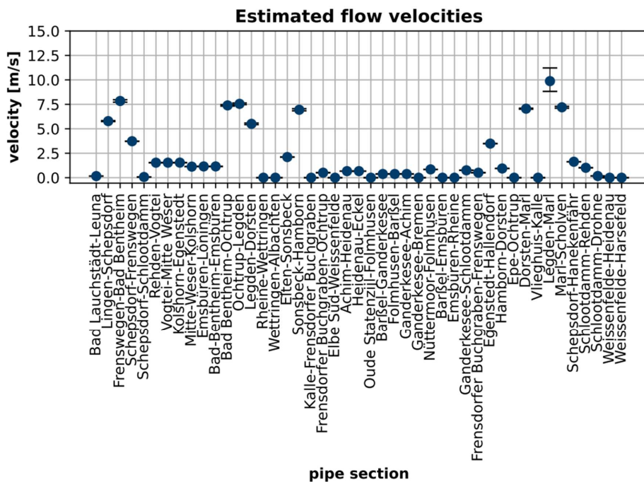
Abbildung I.8.8.1: Geschätzte Fließgeschwindigkeiten im 2030 Basisszenario (durchschnittlich) bei 60 bar Maximaldruck und angenommener Rohrrauigkeit von 1 mm. Die Fehlerschranken geben die Fließgeschwindigkeit am Pipelineeintritt bzw. am -austritt an.
