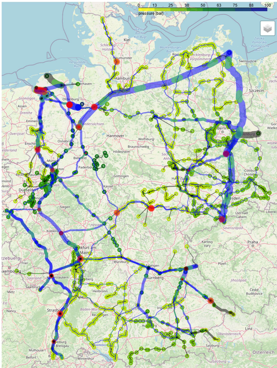
Abbildung I.8.18.5: Flüsse und Drücke in der Erdgas-Nominierung des 04.07.2015 um 00:00 Uhr. Die Drücke an den Knoten sind entsprechend des dargestellten Farbcodes (oben rechts) eingefärbt. Die Dicke der Kanten ist proportional zum Fluss darüber. Legende, siehe Tabelle I.8.1.1.
