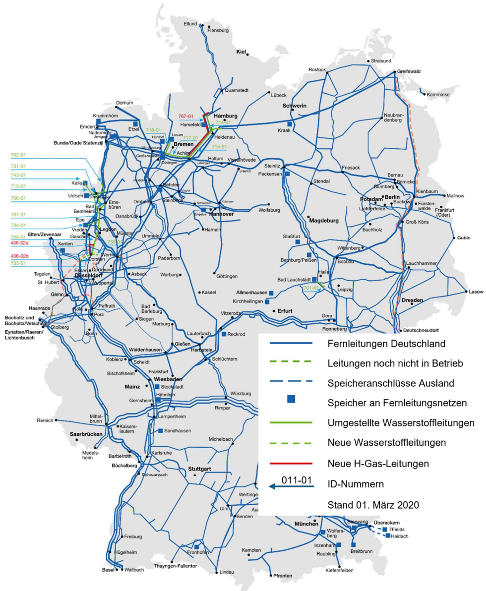
Abbildung 3.1.4.2: Überblick: Wasserstoffnetzwerktopologie 2025 (in Grün) gemäß Netzentwicklungsplan Gas 2020 [7].
