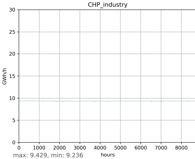
Abbildung 5.2.3.6: Sektorzeitreihe: Industrielle Kraft-Wärme-Kopplung (quasi-konstant)
