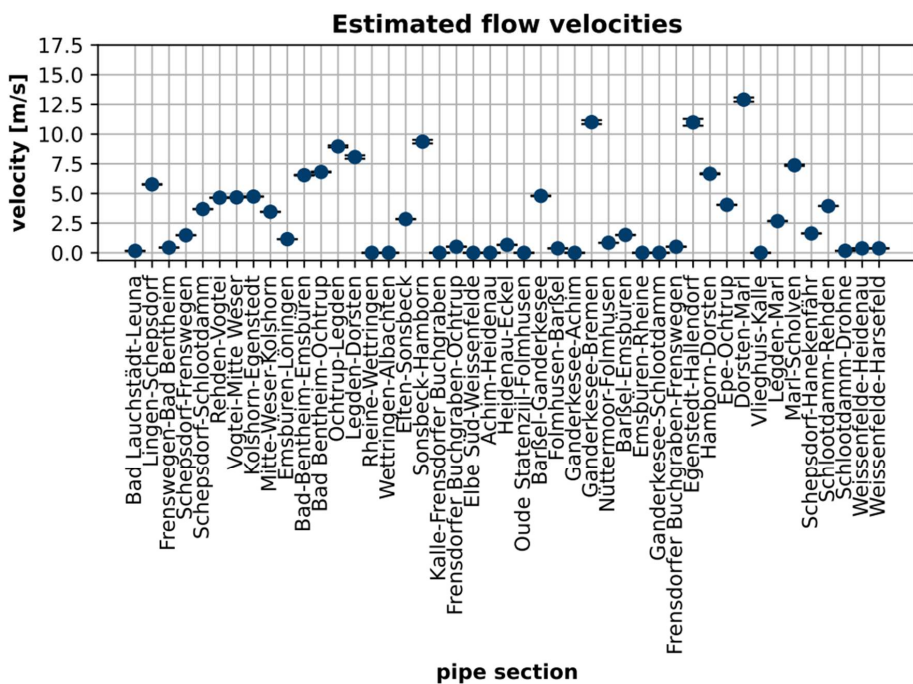
Abbildung I.8.17.1: Geschätzte Fließgeschwindigkeiten im Variation 2 Szenario 2030 (durchschnittlich) bei 60 bar Maximaldruck und angenommener Rohrrauigkeit von 0,1 mm. Die Fehlerschranken geben die Fließgeschwindigkeit am Pipelineintritt bzw. am -austritt an.
