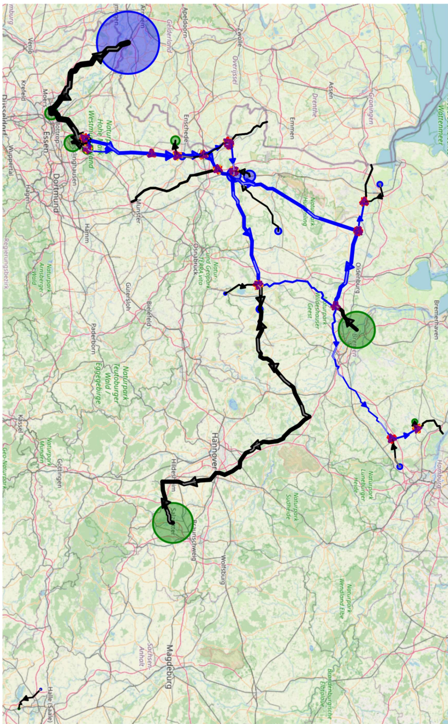
Abbildung I.8.15.2: Flüsse im Variation 2 Szenario 2030 bei 30 bar Maximaldruck und angenommener Rohrrauigkeit von 0,1 mm. Legende, siehe Tabelle I.8.1.1.
