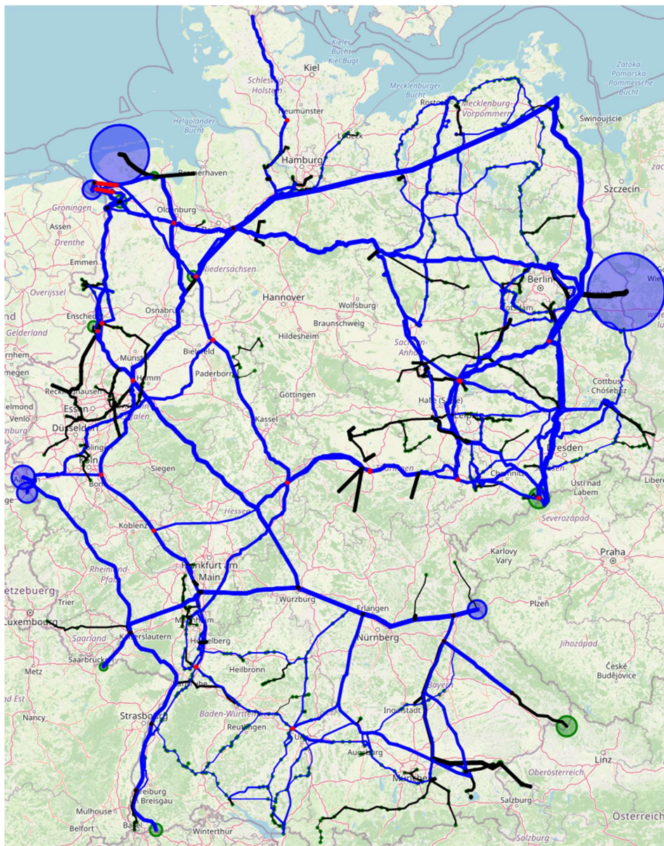
Abbildung I.8.18.10: Ein-/Auspeisesituation der Erdgas-Nominierung des 17.08.2015 um 09:00 Uhr. Blaue Kreise repräsentieren Einspeisungen und grüne Kreise Auspeisungen. Ihre Größe ist proportional zur Größe der Ein-/Auspeisung. Die Dicke der Kanten ist proportional zum Durchmesser der jeweiligen Pipeline. Auf schwarz gefärbten Kanten (Pipelines) wurde der Fluss durch das Preprocessing auf einen festen Wert fixiert. Es ist darauf hinzuweisen, dass parallele Pipelinestränge aufgrund des Zoomlevels nicht erkennbar sind, aber abgebildet sind. Legende, siehe Tabelle I.8.1.1.
