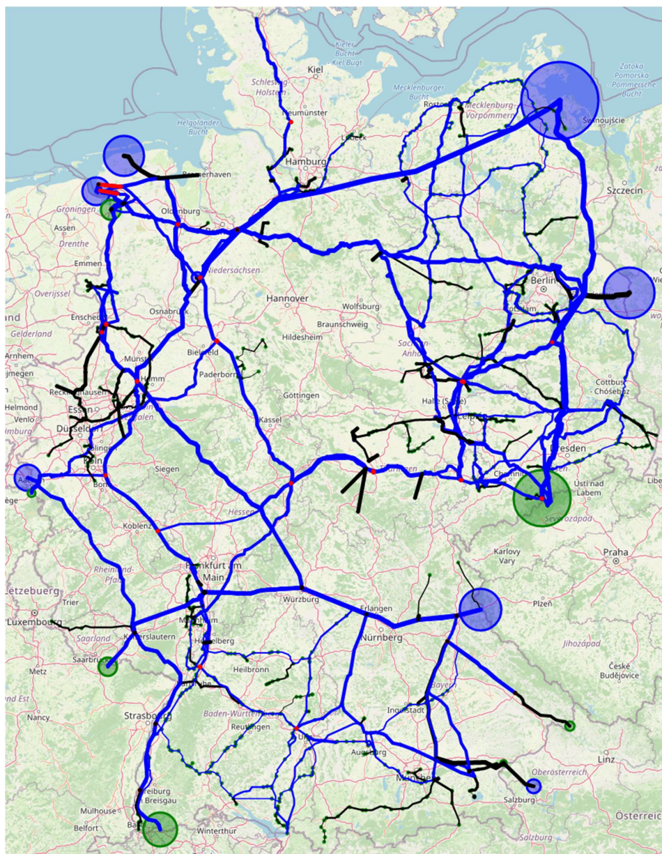
Abbildung I.8.18.16: Ein-/Auspeisesituation der Erdgas-Nominierung des 02.12.2015 um 05:00 Uhr. Blaue Kreise repräsentieren Einspeisungen und grüne Kreise Auspeisungen. Ihre Größe ist proportional zur Größe der Ein-/Auspeisung. Die Dicke der Kanten ist proportional zum Durchmesser der jeweiligen Pipeline. Auf schwarz gefärbten Kanten (Pipelines) wurde der Fluss durch das Preprocessing auf einen festen Wert fixiert. Es ist darauf hinzuweisen, dass parallele Pipelinestränge aufgrund des Zoomlevels nicht erkennbar sind, aber abgebildet sind. Legende, siehe Tabelle I.8.1.1.
