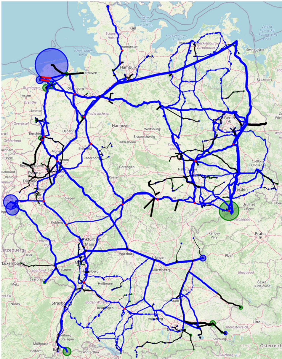
Abbildung I.8.18.7: Ein-/Ausspeisesituation der Erdgas-Nominierung des 11.08.2015 um 15:00 Uhr. Blaue Kreise repräsentieren Einspeisungen und grüne Kreise Ausspeisungen. Ihre Größe ist proportional zur Größe der Ein-/Ausspeisung. Die Dicke der Kanten ist proportional zum Durchmesser der jeweiligen Pipeline. Auf schwarz gefärbten Kanten (Pipelines) wurde der Fluss durch das Preprocessing auf einen festen Wert fixiert. Es ist darauf hinzuweisen, dass parallele Pipelinestränge aufgrund des Zoomlevels nicht erkennbar sind, aber abgebildet sind. Legende, siehe Tabelle I.8.1.1.
