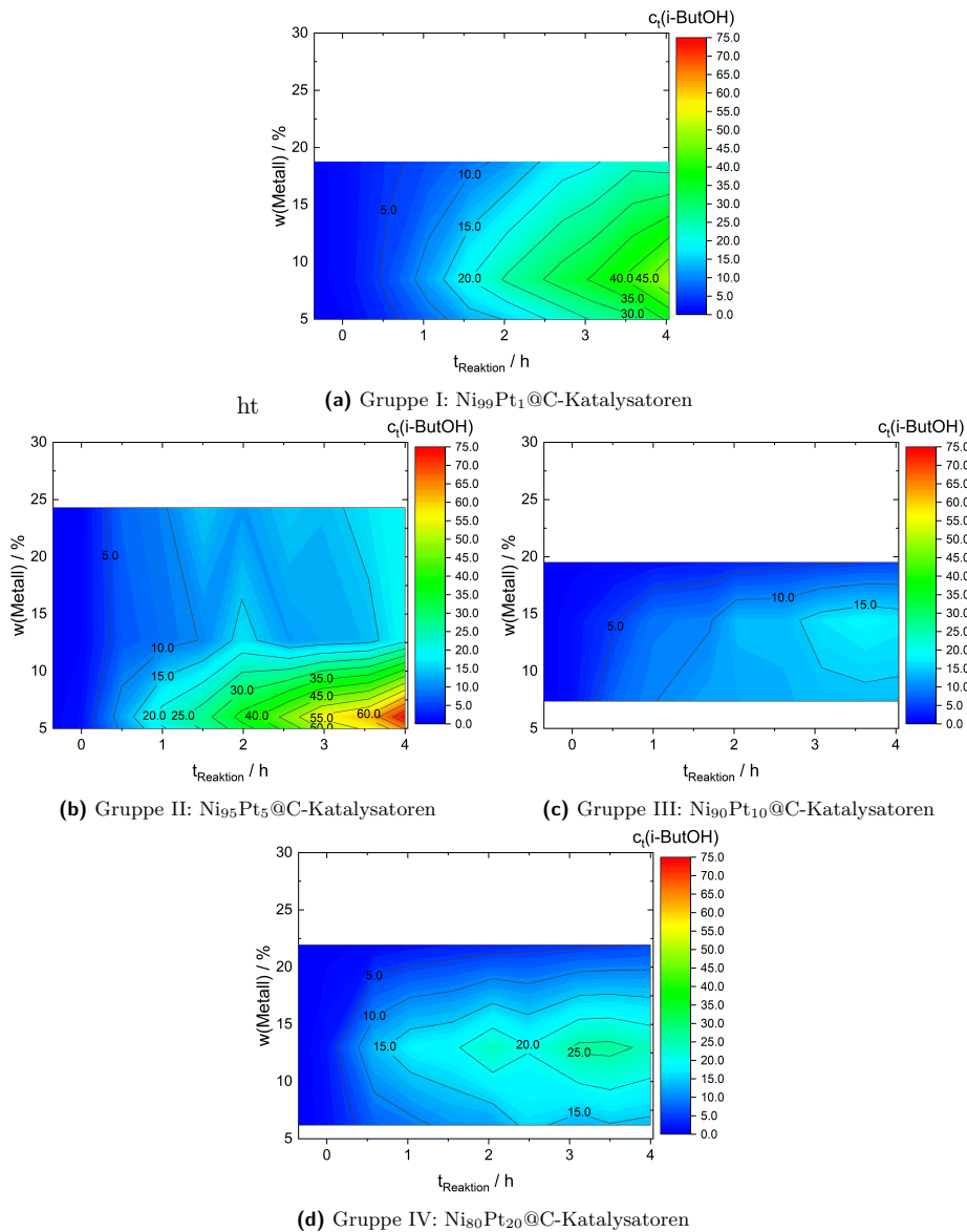
Abbildung 11.25. Darstellung der i -Butanolkonzentration über die Reaktionsdauer für verschiedene \text{Ni}_x\text{Pt}_{1-x}\text{@C} -Katalysatoren. Der angestrebte Bereich für die Metallbeladung ist 5 bis 30 wt %. Die real erreichten Beladungen werden im Höhenliniendiagramm dargestellt. Zwischen den Datenpunkten wird linear interpoliert. Messbedingungen: m_{\text{Kat}} = 250 \text{ mg} , T = 165^\circ\text{C} , c(\text{EtOH}) = 600 \text{ mmol/L} , c(\text{NaOH}) = 450 \text{ mmol/L} , t_R = 4 \text{ h} , V_R = 70 \text{ mL} , N_{\text{Rührer}} = 1000 \text{ rpm} . Reproduziert aus [180] mit Genehmigung der Royal Society of Chemistry.
