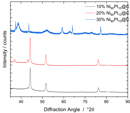
Abbildung 11.22. Darstellung der Diffraktogramme für den \text{Ni}_{90}\text{Pt}_{10}@C -Katalysator mit unterschiedlichen Beladungen. Messbedingungen: K_\alpha(Cu) , \lambda = 1.5419 \text{ \AA} , Schrittweite = 0.02 \text{ deg/s} . Reproduziert aus [180] mit Genehmigung der Royal Society of Chemistry.
