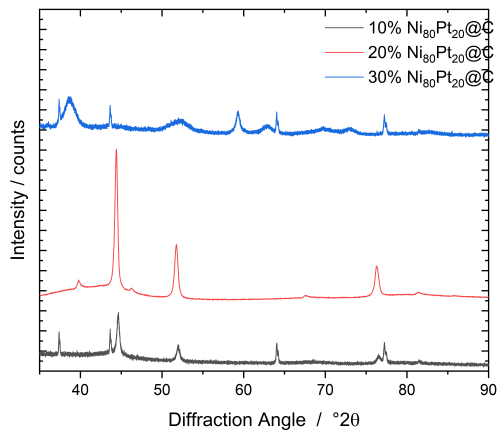
Abbildung 11.23. Darstellung der Diffraktogramme für den \text{Ni}_{80}\text{Pt}_{20}@C -Katalysator mit unterschiedlichen Beladungen. Messbedingungen: K_\alpha(Cu) , \lambda = 1.5419 \text{ \AA} , Schrittweite = 0.02 \text{ deg/s} . Reproduziert aus [180] mit Genehmigung der Royal Society of Chemistry.
