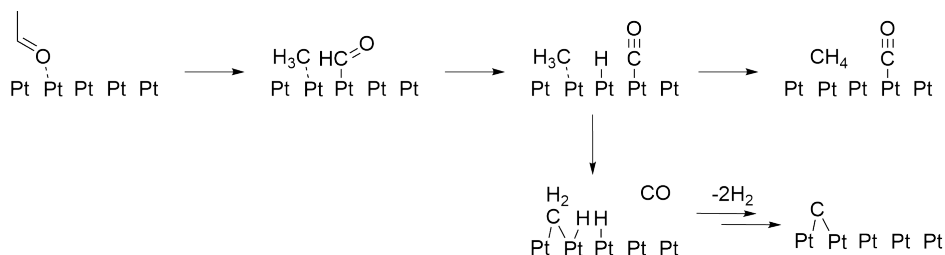
Schema 12.2 Deaktivierung der Katalysatoroberfläche durch Kohlenstoffablagerungen aus der Zersetzung von Acetaldehyd. In Anlehnung an [109].
