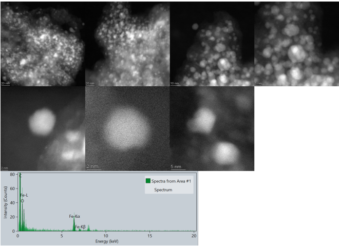
Abbildung D.13. Gesamtheit der TEM-Aufnahmen des Fe 99 Pt 1 /C Katalysators bei verschiedenen Vergrößerungen im Dunkelfeld mit Spektrum der EDX-Messungen der Einzelpartikel.
