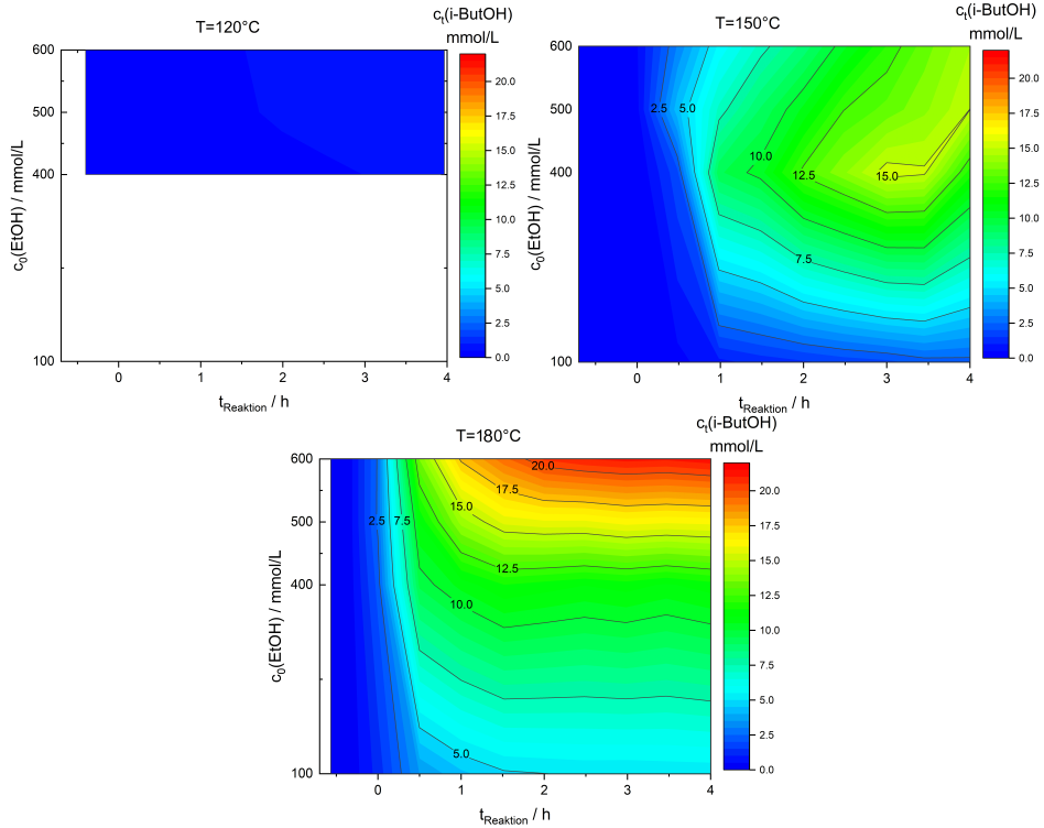
Abbildung 10.12. Zeitabhängige Konzentrationsverläufe von i-Butanol über die Reaktionszeit in Abhängigkeit der Reaktionstemperaturen 120 °C, 150 °C und 180 °C und Ethanolkonzentration 100 mmol/L, 400 mmol/L, 500 mmol/L und 600 mmol/L. Eingesetzt wurde der Pt/C-Katalysator. Reaktionsbedingungen: m_{\text{Kat,trocken}} = 250 mg, w_{\text{Metall}} = 5\% , \varnothing_{\text{Pulver}} < 75 \mu\text{m} , t_R = 4 h, c_{\text{NaOH}} = 450 mmol/L, c_{n\text{-Decan}} = 15 mmol/L, V_R = 70 ml. Zur Besseren Vergleichbarkeit wurde bei allen Diagrammen der gleiche Skalierungsbereich verwendet. In weiß gehaltenen Bereichen wurden keine Experimente durchgeführt. Datentabelle im Anhang Tabelle B.2
