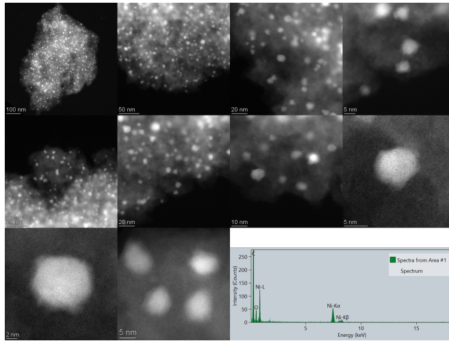
Abbildung D.15. Gesamtheit der TEM-Aufnahmen des \text{Ni}_{99}\text{Pt}_1/\text{C} Katalysators bei verschiedenen Vergrößerungen im Dunkelfeld mit Spektrum der EDX-Messungen der Einzelpartikel.
