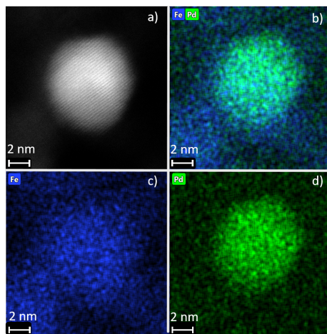
Abbildung 11.9. TEM-EDX-Aufnahmen des \text{Fe}_{99}\text{Pd}_1/\text{C} Katalysators. Dargestellt ist die STEM-Aufnahme im Dunkelfeld (a), die Überlagerung der EDX-Mappings von Fe und Pd (b), sowie die Elementmappings für die Signale von Fe (c) und Pd (d). Entommen aus [151] CC 4.0, © 2024 Häusler et al.
