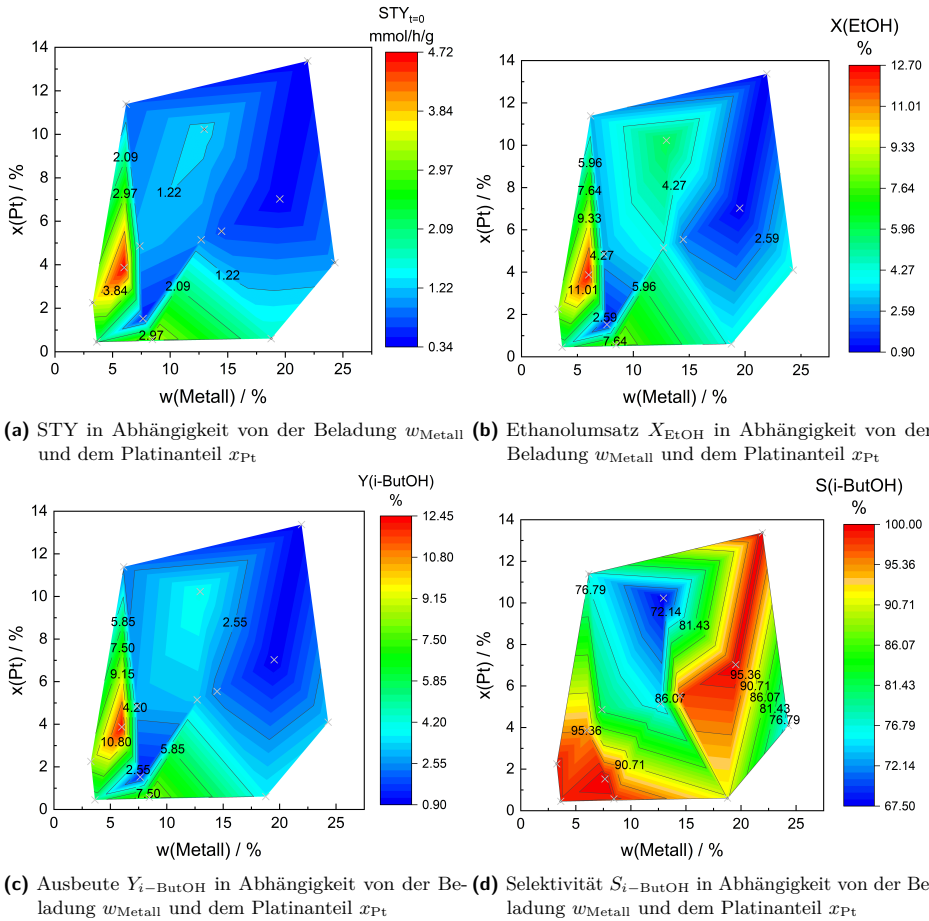
Abbildung 11.28. Darstellung des Ethanolumsatzes, sowie der Selektivität, Ausbeute, und Raumzeitausbeute von i -Butanol als Funktion der Katalysatorbeladung und dem Stoffmengenanteil Platin für die \text{Ni}_x\text{Pt}_{1-x}\text{@C} -Katalysatoren mit 80 > x > 1 . Messbedingungen: m_{\text{Kat}} = 250 \text{ mg} , T = 165^\circ\text{C} , c(\text{EtOH}) = 600 \text{ mmol/L} , c(\text{NaOH}) = 450 \text{ mmol/L} , t_R = 4 \text{ h} , V_R = 70 \text{ mL} , N_{\text{Rührer}} = 1000 \text{ rpm} . Reproduziert aus [180] mit Genehmigung der Royal Society of Chemistry.
