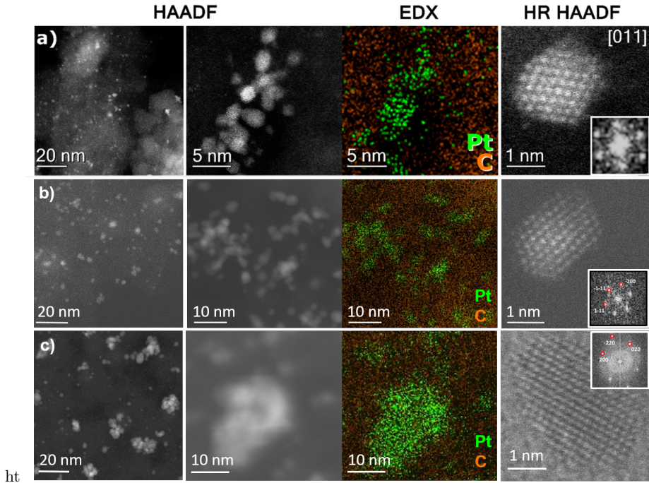
Abbildung 10.17. HAADF-STEM und EDX-Messungen von: (a) frischem Pt/C-Katalysator (oberer Teil) Entnommen mit Genehmigung aus [109], CC 4.0, ©2020 Pasel et al. ; (b) Pt/C-Katalysator nach 4 h Reaktionsdauer bei 120 °C (mittlerer Teil); und (c) Pt/C-Katalysator nach 4 h Reaktionsdauer bei 180 °C (unterer Teil). Platin ist in den EDX-Karten in Grün und der C-Träger in Orange dargestellt. HR-HAADF-STEM-Bilder zeigen eine Nahaufnahme von Nanopartikeln mit Fast-Fourier-Transform (FFT)-Mustern.
