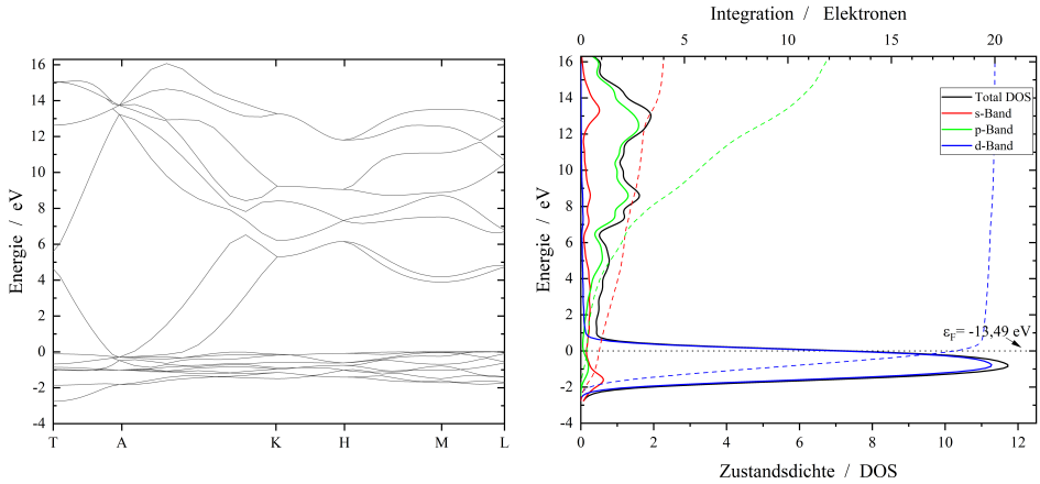
(a) Bandstruktur von Nickel. Die Fermi -Kante wurde als Nullpunkt gesetzt. (b) PDOS Diagramm für Nickel. Schwarze Linie: PDOS; rote, grüne und blaue Linien: Beiträge der s, p und d-Orbitale. Die gleichfarbigen gestrichelten Linien stellen die Integration über die im entsprechenden Orbital befindlichen Elektronen dar.
