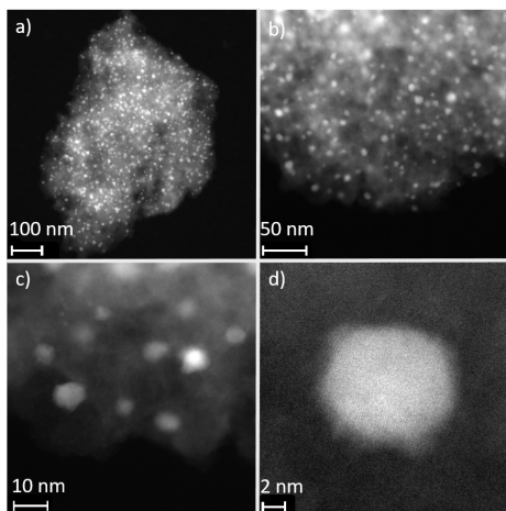
Abbildung 11.5. TEM-Aufnahmen des \text{Ni}_{99}\text{Pt}_1/\text{C} Katalysators bei verschiedenen Vergrößerungen im Dunkelfeld. Entommen aus [151] CC 4.0, © 2024 Häusler et al.
