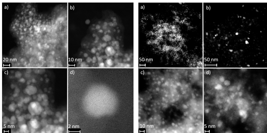
(a) TEM-Aufnahmen des Fe 99 Pt 1 /C Katalysators bei verschiedenen Vergrößerungen im Dunkelfeld. (b) TEM-Aufnahmen des Fe 99 Pd 1 /C Katalysators bei verschiedenen Vergrößerungen im Dunkelfeld.
