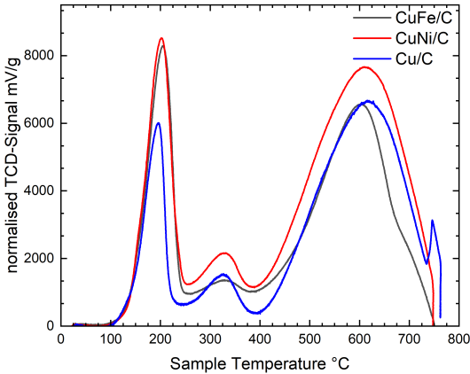
Abbildung 11.2. TPR Messungen der durch Imprägnierung hergestellten Kupferkatalysatoren Cu/C, CuFe/C und CuNi/C. Dargestellt ist das massennormierte Signal des WLD. Messbedingungen: 2 %H 2 in Argon, \dot{V} =30 mL/min; \beta =10 K/min. Entommen aus [151] CC 4.0, ©2024 Häusler et al.
