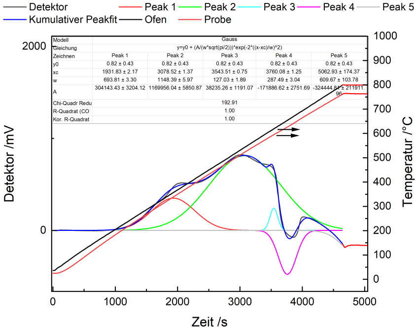
Abbildung D.7. TPR Profil des Fe/C Katalysators mit Peakzerlegung mittels Gauss-Funktionen. Messbedingungen: m_{Kat}=89.4 mg, 2 %H 2 in Argon, \dot{V}=30 mL/min; \beta=10 K/min. Der Kalibrierfaktor f_{WLD}=9.19209 \cdot 10^{-8} mmols/mV wurde mit CuO 99.9995 % Reinheit ermittelt. Die Peakzerlegung wurde mit dem Peakanpassungstool der Software OriginPro , Version 2021. OriginLab Corporation, Northampton, MA, USA, durchgeführt. Die Basislinie wurde auf 0.00 mV festgelegt. Messdaten ab Temperaturen über 798 °C wurden maskiert, um Einflüsse der verlangsamten Heizrate zu reduzieren.
