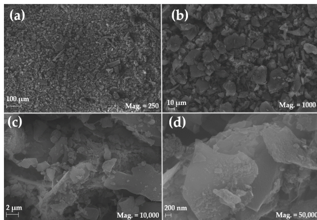
Abbildung 10.5. REM-Bilder von 3% Cu/C in Vergrößerungen von 250 bis 50.000. Alle Bilder wurden mit den folgenden Parametern aufgenommen: EHT=20.0 kV, WD=8.5 mm, SingalA=InLens. Entommen aus [153] CC 4.0, ©2021 Häusler et al.
