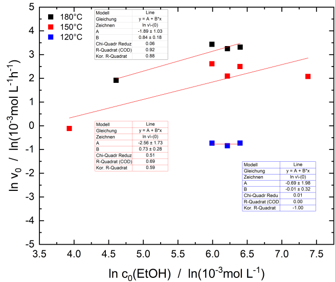
Abbildung 10.14. Anfangsgeschwindigkeiten v_0 der Bildung von i-Butanol in Abhängigkeit der Startkonzentration von Ethanol für die Temperaturen 120 °C, 150 °C und 180 °C. Methanol stellt Reaktant und Lösungsmittel dar, weshalb dessen Konzentration als konstant betrachtet wird. Die Geraden wurden mittels linearer Regression ermittelt.
