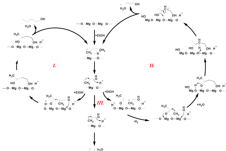
Schema 3.7 Katalysezyklus entsprechend des Mechanismusvorschlags nach Chierigato et al. [90]
