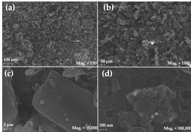
Abbildung 10.6. REM-Bilder von 1% Ir/C in Vergrößerungen von 250 bis 100.000. Alle Bilder wurden mit den folgenden Parametern aufgenommen: EHT=20.0 kV, WD=8.5 mm, SingalA=InLens. Entommen aus [153] CC 4.0, ©2021 Häusler et al.
