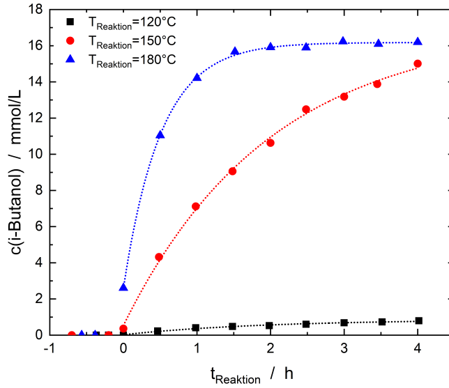
Abbildung 10.15. Auftragung der gemessenen Konzentrationen von i-Butanol bei verschiedenen Reaktionstemperaturen. Die Beschreibung des Konzentrationsverlaufs unter Berücksichtigung mit der exponentiellen Funktion y = y_0 + A * \exp(R_0 * x) ist als gepunktete Linie dargestellt. Die Fitparameter sind in Tabelle B.3 aufgelistet. m_{\text{Pt/C}} = 250 \text{ mg} , w_{\text{Metall}} = 5 \% , \varnothing_{\text{Pulver}} < 75 \mu\text{m} , c_0(\text{EtOH}) = 500 \text{ mmol/L} , c_{\text{NaOH}} = 450 \text{ mmol/L} , c_{n\text{-Decan}} = 15 \text{ mmol/L} , V_R = 70 \text{ ml} , t_R = 4 \text{ h}
