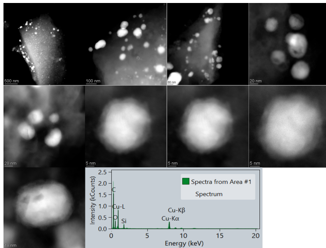
Abbildung D.12. Gesamtheit der TEM-Aufnahmen des \text{Cu}_{99}\text{Ni}_1/\text{C} Katalysators bei verschiedenen Vergrößerungen im Dunkelfeld mit Spektrum der EDX-Messungen der Einzelpartikel.
