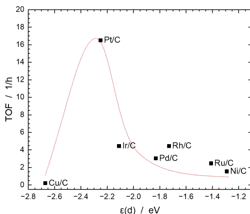
Abbildung 10.11. Resultierendes Vulkandiagramm für die TOF der Übergangsmetallkatalysatoren bei der \beta -Methylierung von 2-Phenylethanol. T=120^\circ\text{C} , 1,5 Äquivalente NaOH und t(\text{Reaktion}) = 24\text{ h} . Die rote Kurve wurde aus Gründen der Übersichtlichkeit gezeichnet. Entommen aus [153] CC 4.0, ©2021 Häusler et al.
