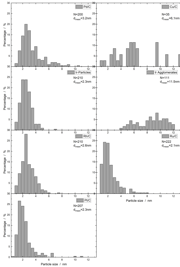
Abbildung D.10. Histogramme der Partikelgrößenverteilung für die monometallischen Katalysatoren aus den TEM Messungen. Entnommen aus [153], CC 4.0 ©Häusler et al.
