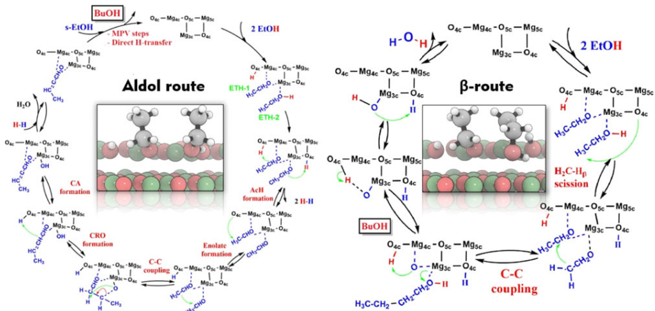
Abbildung 3.7. Postulierter Mechanismus von Souza et al. auf MgO als Katalysator. Die \beta -Route findet bei Temperaturen unterhalb von 300 °C statt, während bei Temperaturen oberhalb 400 °C, die Aldolroute den Hauptreaktionspfad für die Bildung von 1-Butanol stattfindet. Entnommen aus [89] Copyright ©2020 American Chemical Society.
