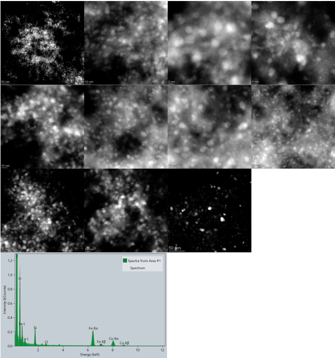
Abbildung D.14. Gesamtheit der TEM-Aufnahmen des Fe 99 Pd 1 /C Katalysators bei verschiedenen Vergrößerungen im Dunkelfeld mit Spektrum der EDX-Messungen der Einzelpartikel.
