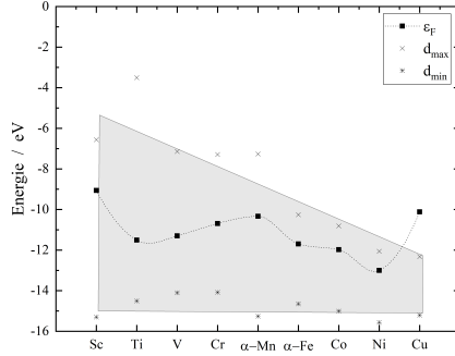
Abbildung 2.2. Die Fermi-Kante \epsilon_F wurde für die Übergangsmetalle der ersten Periode des d-Blocks berechnet. Das Polygon deutet die Dispersion des d-Bandes an, während die berechneten Werte als Kreuze dargestellt werden. In Anlehnung an R. Hoffmann [34]
