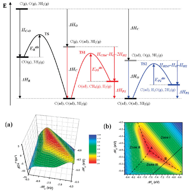
Abbildung 2.5. Das obere Diagramm stellt das Energiediagramm für die CO-Hydrierung mit den drei Schlüsselschritten dar. Die hypothetischen Elementarschritte der CO-Dissoziation, Hydrierung von adsorbiertem Kohlenstoff und der Hydrierung von adsorbiertem Sauerstoff sind in Schwarz, Rot und Blau dargestellt. Im unteren Teil sind der resultierende 3-D-Vulkan-Plot (a) für die dissoziative Chemisorptionsenergie von Sauerstoff und Kohlenstoff gegen die berechnete TOF sowie der Konturplot (b) abgebildet. Adaptiert mit Genehmigung von [50] Copyright 2008, American Chemical Society
