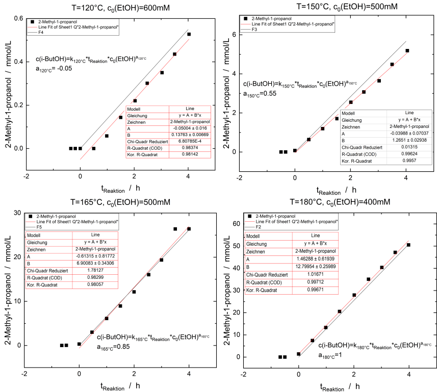
Abbildung D.17. Auftragung der Berechneten und gemessenen Konzentrationen von i-Butanol bei verschiedenen Reaktionstemperaturen und Starkkonzentrationen an Ethanol m_{\text{Ni}_{99}\text{Pt}_{1/C}} = 250 \text{ mg} , w_{\text{Metall}} = 5 \% , \varnothing_{\text{Pulver}} < 75 \mu\text{m} , t_R = 4 \text{ h} , c_{\text{NaOH}} = 450 \text{ mmol/L} , c_{n\text{-Decan}} = 15 \text{ mmol/L} , V_R = 70 \text{ ml}
