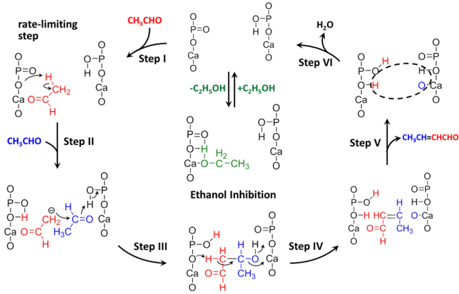
Abbildung 3.5. Reaktionsmechanismus für die Aldolroute auf dem HAP-Katalysator. Entnommen mit Genehmigung aus [86] Copyright ©2015 American Chemical Society
