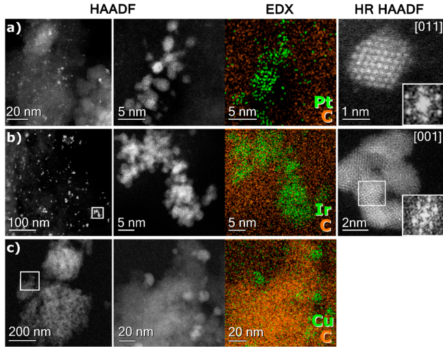
Abbildung 10.7. HAADF-STEM-Übersichtsbilder neben Übersichtsbildern der entsprechenden EDX-Elementkarten von: (a) frischem Pt/C-Katalysator (oberer Teil); (b) frischem Ir/C-Katalysator (mittlerer Teil); und (c) frischem Cu/C-Katalysator (unterer Teil). Die Metalle sind in den EDX-Karten in Grün und der C-Träger in Orange dargestellt. HR-HAADF-STEM-Bilder für Pt/C und Ir/C zeigen eine Nahaufnahme von Nanopartikeln mit Fast-Fourier-Transform (FFT)-Mustern in den Einschüben. Entnommen mit Genehmigung aus [109], CC 4.0, ©2020 Pasel et al.
