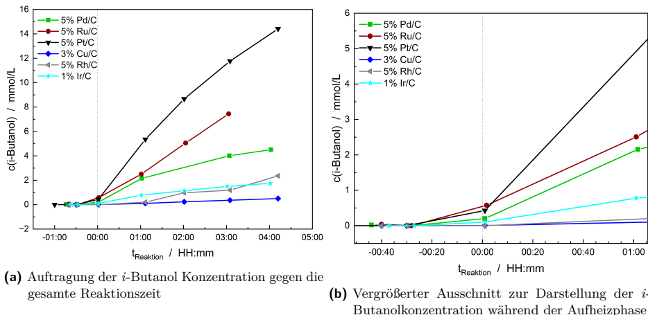
Abbildung 10.9. Auftragung der i -Butanol Konzentration gegen die Reaktionszeit für alle monometallischen Katalysatoren. t(\text{Reaktion}) = 4 \text{ h} , T = 150 \text{ }^{\circ}\text{C} , N = 1000 \text{ RPM} , V = 70 \text{ mL} und m(\text{Katalysator}) = 0.1 \text{ g} . Die gestrichelte Linie markiert den Punkt, an dem 150 \text{ }^{\circ}\text{C} erreicht wurden. Entommen aus [153] CC 4.0, ©2021 Häusler et al.
