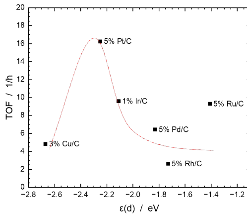
Abbildung 10.10. Resultierende Vulkankurve für die Umschlagshäufigkeit (TOF) der monometallischen Übergangsmetallkatalysatoren in der i -Butanol-Synthese. Die rote Kurve wurde aus Gründen der Übersichtlichkeit eingezeichnet. Entommen aus [153] CC 4.0, ©2021 Häusler et al.
