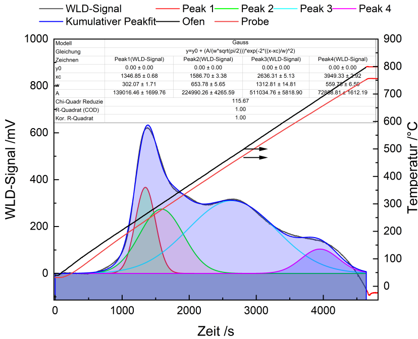
Abbildung D.4. TPR Profil des Ni/C Katalysators mit Peakzerlegung mittels Gauss -Funktionen. Messbedingungen: m_{Kat}=80.7 mg, 2 %H 2 in Argon, \dot{V}=30 mL/min; \beta=10 K/min. Der Kalibrierfaktor f_{WLD}=9.19209 \cdot 10^{-8} mmols/mV wurde mit CuO 99.9995 % Reinheit ermittelt. Die Peakzerlegung wurde mit dem Peakanpassungstool der Software OriginPro , Version 2021. OriginLab Corporation, Northampton, MA, USA, durchgeführt. Die Basislinie wurde auf 0.00 mV festgelegt. Messdaten ab Temperaturen über 798 °C wurden maskiert, um Einflüsse der verlangsamten Heizrate zu reduzieren.
