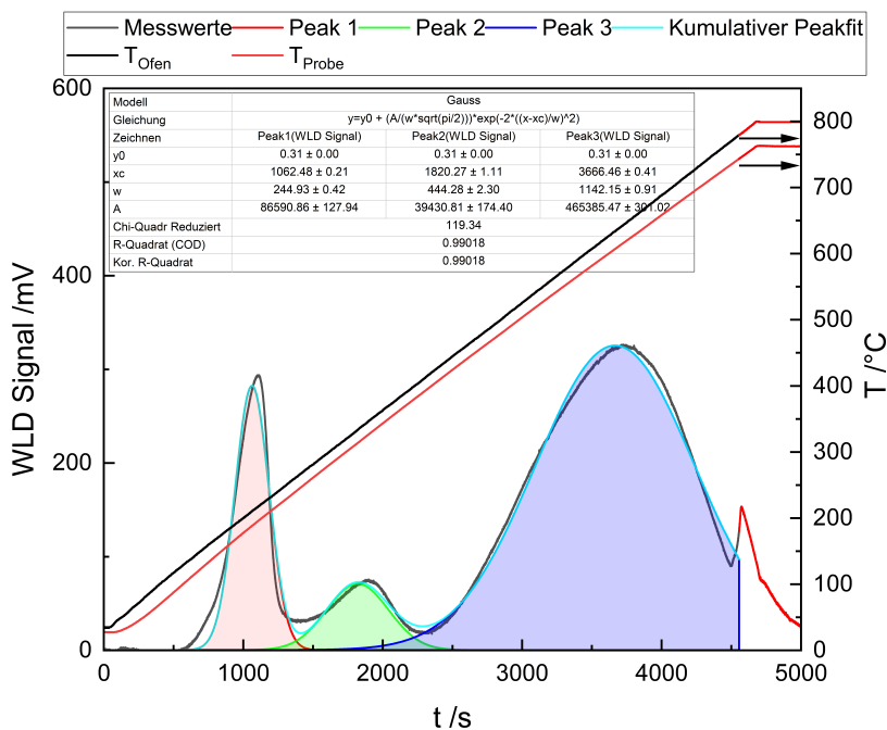
Abbildung D.1. TPR Profil des CuFe/C Katalysators mit Peakzerlegung mittels Gauss -Funktionen. Messbedingungen: m_{Kat} =48.9 mg, 2 %H 2 in Argon, \dot{V} =30 mL/min; \beta =10 K/min. Der Kalibrierfaktor f_{WLD} = 9.19209 \cdot 10^{-8} mmols/mV wurde mit CuO 99.9995 % Reinheit ermittelt. Die Peakzerlegung wurde mit dem Peakanpassungstool der Software OriginPro, Version 2021. OriginLab Corporation, Northampton, MA, USA, durchgeführt. Die Basislinie wurde auf 0.31 mV festgelegt. Messdaten ab Temperaturen über 779 °C wurden maskiert, um Einflüsse der verlangsamten Heizrate zu reduzieren.
