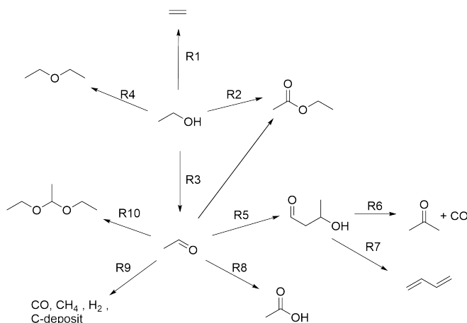
Abbildung 3.8. Produkte der Nebenreaktionen in der Guerbet -Reaktion, ausgehend von Ethanol. Adaptiert aus [93]
