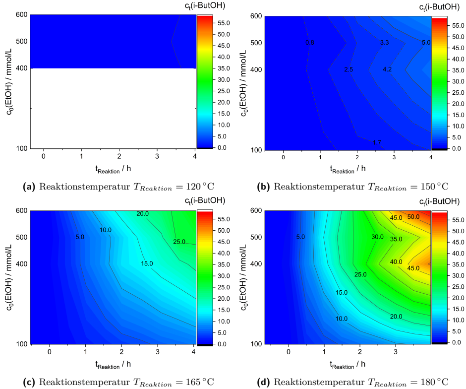
Abbildung 11.14. Zeitabhängige Konzentrationsverläufe von i -Butanol über die Reaktionszeit in Abhängigkeit der Reaktionstemperaturen und Ethanolkonzentrationen 100 mmol/L, 400 mmol/L, 500 mmol/L und 600 mmol/L zu Reaktionsstart. Eingesetzt wurde der \text{Ni}_{99}\text{Pt/C} -Katalysator, der mittels Imprägnierung hergestellt wurde. Reaktionsbedingungen: m_{\text{Kat,trocken}} = 250\text{ mg} , w_{\text{Metall}} = 5\% , \varnothing_{\text{Pulver}} < 75\text{ }\mu\text{m} , t_R = 4\text{ h} , c_{\text{NaOH}} = 450\text{ mmol/L} , c_{n\text{-Decan}} = 15\text{ mmol/L} , V_R = 70\text{ ml} . Versuchsdaten in Tabelle B.5. Reproduziert aus [152] mit Genehmigung der Royal Society of Chemistry.
