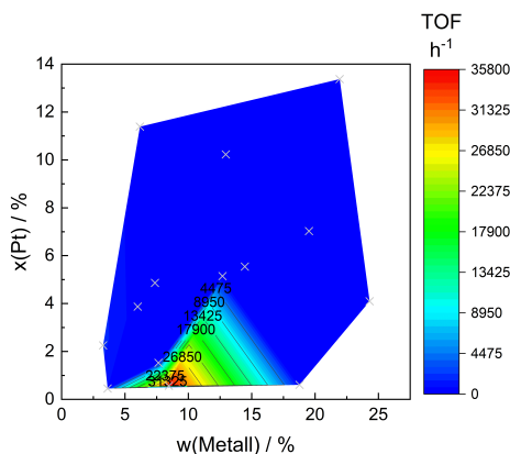
Abbildung 12.1. Darstellung der TOF von i -Butanol in Abhängigkeit von der Katalysatorbeladung und dem Stoffmengenanteil Platin für die Ni_xPt_{1-x} @C-Katalysatoren mit 80 > x < 1 . Messbedingungen: m_{Kat} = 0.25 g, T = 165^\circ\text{C} , t_R = 4 h, V_R = 70 mL, 1000 Umdrehungen pro Minute.
