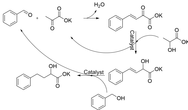
Abbildung 3.2. Reaktionszyklus für die Aldolkondensation und Transferhydrierung nach Veibel et al. [73].
