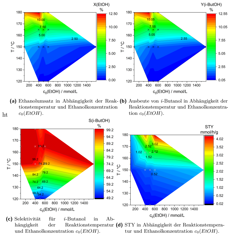
Abbildung 11.15. Ethanolumsatz, Ausbeute und Selektivität für i -Butanol, sowie STY für i -Butanol als Funktion der Reaktionstemperatur und der Startkonzentration Ethanol. Die Kennzahlen wurden zum Ende der Reaktionsdauer ermittelt. Messpunkte wurden als Kreuze dargestellt. Zwischen den Messpunkten wurde linear interpoliert. Eingesetzt wurde der \text{Ni}_{99}\text{Pt/C} -Katalysator, der mittels Imprägnierung hergestellt wurde. Reaktionsbedingungen: m_{\text{Kat,trocken}} = 250 \text{ mg} , w_{\text{Metall}} = 5 \% , \varnothing_{\text{Pulver}} < 75 \mu\text{m} , t_R = 4 \text{ h} , c_{\text{NaOH}} = 450 \text{ mmol/L} , c_{\text{n-Decan}} = 15 \text{ mmol/L} , V_R = 70 \text{ ml} . Reproduziert aus [152] mit Genehmigung der Royal Society of Chemistry.
