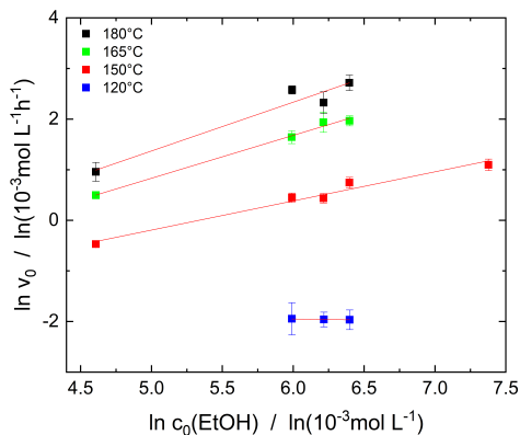
Abbildung 11.16. Anfangsgeschwindigkeiten v_0 der Bildung von i -Butanol in Abhängigkeit der Startkonzentration von Ethanol für die Temperaturen 120 °C, 150 °C, 165 °C und 180 °C. Methanol stellt Reaktand und Lösungsmittel dar, weshalb dessen Konzentration als konstant betrachtet wird. Die Fehlerbalken stellen \pm\sigma(v_0) dar. Die Geraden wurden mittels linearer Regression ermittelt. Die Messpunkte wurden anhand \sigma(v_0) gewichtet. Die Fitparameter sind in Tabelle B.7, die Messwerte in Tabelle B.6 aufgelistet. Reproduziert aus [152] mit Genehmigung der Royal Society of Chemistry.
