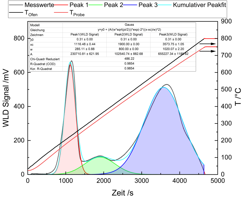
Abbildung D.3. TPR Profil des CuFe/C Katalysators mit Peakzerlegung mittels Gauss -Funktionen. Messbedingungen: m_{Kat}=80.7 mg, 2 %H 2 in Argon, \dot{V}=30 mL/min; \beta=10 K/min. Der Kalibrierfaktor f_{WLD}=9.19209 \cdot 10^{-8} mmols/mV wurde mit CuO 99.9995 % Reinheit ermittelt. Die Peakzerlegung wurde mit dem Peakanpassungstool der Software OriginPro , Version 2021. OriginLab Corporation, Northampton, MA, USA, durchgeführt. Die Basislinie wurde auf 0.31 mV festgelegt. Messdaten ab Temperaturen über 779 °C wurden maskiert, um Einflüsse der verlangsamten Heizrate zu reduzieren. Um eine stabile Lösung zu erhalten, wurde der Wert xc und w für Peak 2 fixiert.
