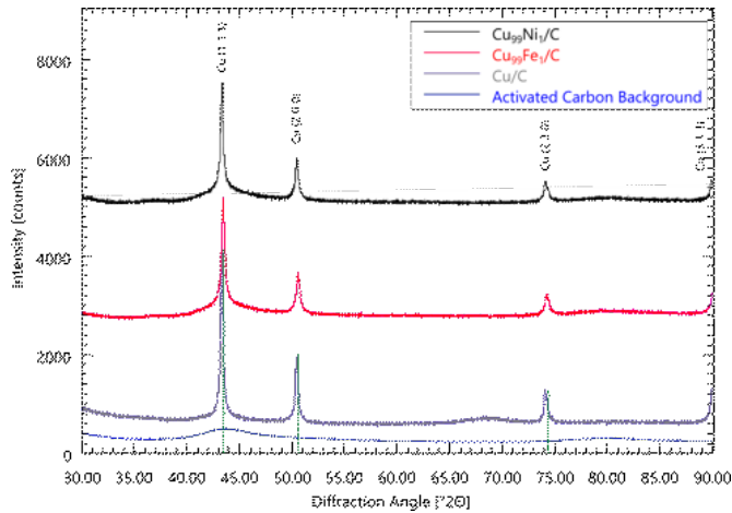
Abbildung 11.1. Diffraktogramm der Kupfer basierten Katalysatormaterialien, die durch Imprägnierung nach Calcinierung bei 500^\circ\text{C} erhalten werden. Gemessen wurde im Bereich von 10 bis 90^\circ 2\theta mit \text{Cu}_\alpha -Strahlung. Von oben nach unten dargestellt sind; \text{Cu}_{99}\text{Ni}_1/\text{C} schwarz, \text{Cu}_{99}\text{Fe}_1/\text{C} rot, \text{Cu}/\text{C} grau und Aktivkohle (blau) als Untergrund. Indizes stellen die angestrebte chemische Zusammensetzung in Atomprozent dar. Der Untergrund ist in den Graphen nicht subtrahiert. In grün dargestellt sind die Cu-Reflexe mit Indexierung. Entommen aus [151] CC 4.0, ©2024 Häusler et al.
