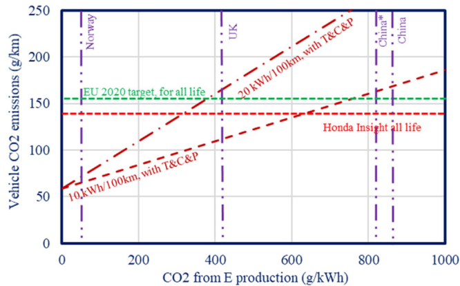
Abbildung 1.1. CO 2 Emissionen pro kilometer über den Fahrzeuglebenszyklus in Abhängigkeit des CO 2 Fußabdrucks der Energieerzeugung. Grün dargestellt die EU Ziele 2020. Violett stellt die CO 2 Emissionen pro erzeugter kWh für die Länder Norwegen, Vereinigtes Königreich und China dar. In dunkelrot dargestellt sind die Fahrzeugemissionen der BEV mit den Durchschnittsverbräuchen von 10 kWh/100km und 20 kWh/100km. Entnommen aus [15] ©2021 Elsevier Ltd.
