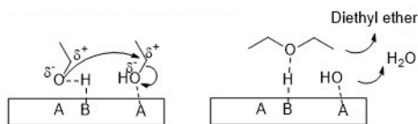
Schema 3.5 Mechanismus für die Dehydratisierung von Ethanol zu Diethylether auf Mg/Al-Oxiden. A und B stellen Lewis-Säure bzw. Brønsted-Basen Zentren dar. Entnommen aus [76] ©1998 Academic Press.
