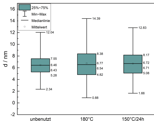
Abbildung 11.19. Boxplot der Partikelverteilung aus den TEM-Aufnahmen für den Pt/C Katalysator vor und nach der Reaktion. In der Box ist das zweite und dritte Quartil und der Median angegeben. Der Mittelwert wird durch ein Kästchen dargestellt. Die Wisker stellen die Extrema der Partikelgrößen dar. Reaktionsbedingungen: m_{\text{Katalysator}}=250 mg, V_R=70 mL, c_{\text{EtOH}}=600 mol/dm 3 . Stichprobengröße N_{\text{frisch}}=375 , N_{180^\circ\text{C}}=844 , N_{180^\circ\text{C}/24\text{h}}=677 . Reproduziert aus [152] mit Genehmigung der Royal Society of Chemistry.
