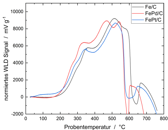
Abbildung 11.10. Massennormiertes Reduktionsprofil der TPR-Messungen für die durch Imprägnierung hergestellten Eisenkatalysatoren Fe/C, Fe 99 Pd 1 /C und Fe 99 Pt 1 /C. Dargestellt ist das massennormierte Signal des WLD. Messbedingungen: 2 % H 2 in Argon, \dot{V} = 30 mL/min, \beta = 10 K/min. Entommen aus [151] CC 4.0, © 2024 Häusler et al.
