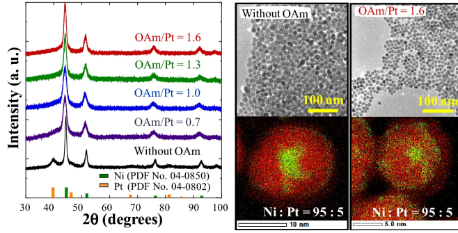
Abbildung A.3. XRD-Diffraktogramme der \text{Ni}_{95}\text{Pt}_5 -Nanopartikel für das Oleylamin (OAm)/Platin Verhältnis von 0 bis 1.6. Die TEM Bilder zeigen die Partikel im Kontrastbild, sowie die Elementverteilung für ausgewählte repräsentative Partikel, die bei der Synthese ohne Oleylamin und mit einem OAm/Pt-Verhältnis von 1.6 erhalten wurden. In grün dargestellt sind die Platinatome, in rot dargestellt die Nickelatome. Adaptiert mit Genehmigung aus [198] ©Springer Nature Switzerland AG 2018
