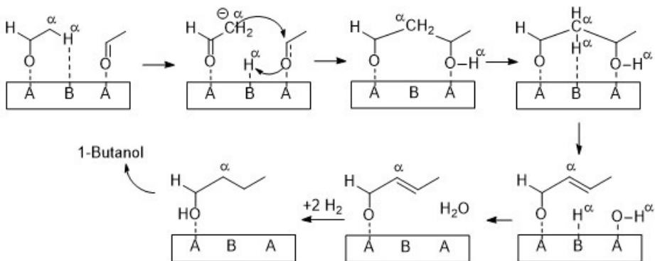
Schema 3.2 Mechanismus für die Aldolkondensation von Acetaldehyd auf Mg/Al-Oxiden. A und B stellen Lewis-Säure bzw. Brønsted-Basen Zentren dar. Entnommen aus [76] ©1998 Academic Press.
