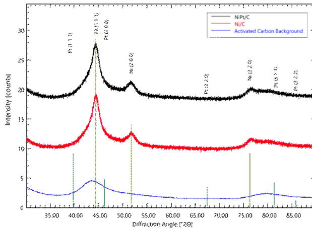
Abbildung 11.4. Diffraktogramm der nickelhaltigen Katalysatormaterialien nach Calcinierung bei 500 °C für vier Stunden im Stickstoffstrom. Messbereich: von 10° bis 90° 2θ mit Cu-K α Strahlung \lambda=0.15406 nm. Von oben nach unten: Ni 99 Pt 1 /C in schwarz, Ni/C in rot und Aktivkohle als Untergrund in blau. Die Nickel und Platinreflexe sind in grün dargestellt. Entommen aus [151] CC 4.0, ©2024 Häusler et al.
