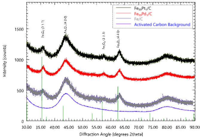
Abbildung 11.7. Diffraktogramm der eisenhaltigen Katalysatormaterialien nach Calcinierung bei 500 °C für vier Stunden im Stickstoffstrom. Messbereich: von 10° bis 90° 2 \theta mit Cu-K \alpha Strahlung \lambda=0.154\,06 nm. Von oben nach unten: Fe 99 Pt 1 /C in schwarz, Fe 99 Pd 1 /C in rot, Fe/C in grau und Aktivkohle als Untergrund in blau. Die Reflexe für Fe 3 O 4 sind in grün dargestellt. Entommen aus [151] CC 4.0, © 2024 Häusler et al.
