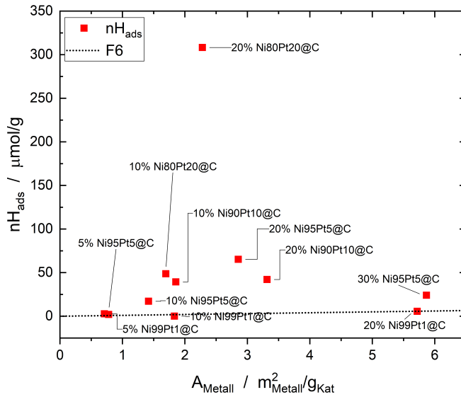
Abbildung D.19. Auftragung der adsorbierten Menge Wasserstoff gegen die Metallfläche auf dem NiPt-Katalysatoren. Die schwarze Linie verdeutlicht den Fall dass ein linearer Zusammenhang zwischen der adsorbierten Menge Wasserstoff und der Metalloberfläche auftreten würde.
