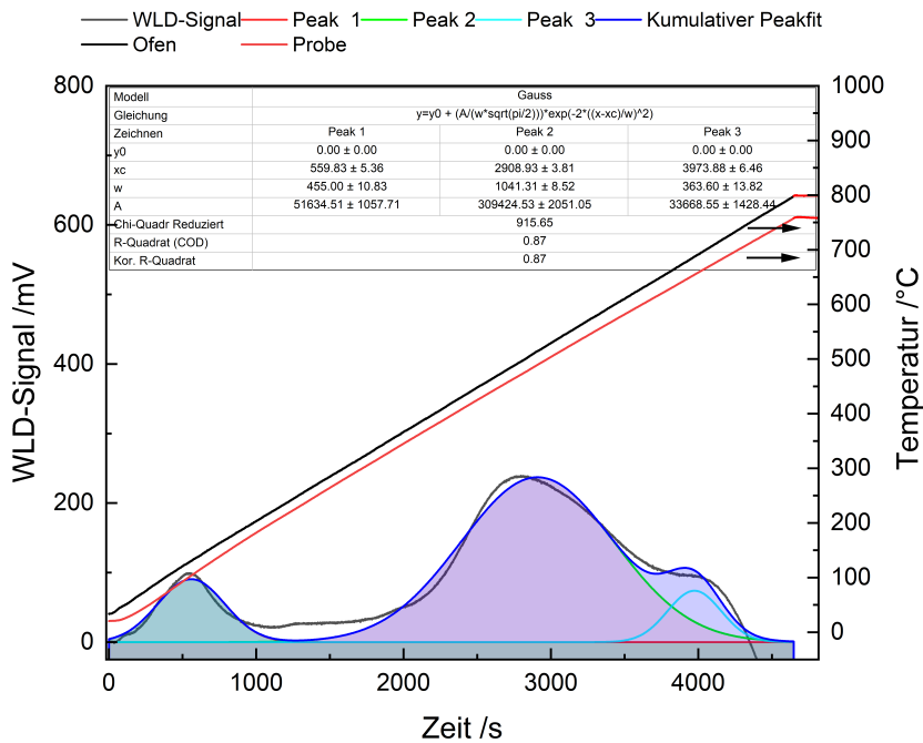
Abbildung D.6. TPR Profil des NiPt@C Katalysators mit Peakzerlegung mittels Gauss -Funktionen. Messbedingungen: m_{Kat}=80.7 mg, 2 %H 2 in Argon, \dot{V}=30 mL/min; \beta=10 K/min. Der Kalibrierfaktor f_{WLD}=9.19209 \cdot 10^{-8} mmols/mV wurde mit CuO 99.9995 % Reinheit ermittelt. Die Peakzerlegung wurde mit dem Peakanpassungstool der Software OriginPro , Version 2021. OriginLab Corporation, Northampton, MA, USA, durchgeführt. Die Basislinie wurde auf 0.00 mV festgelegt. Messdaten ab Temperaturen über 798 °C wurden maskiert, um Einflüsse der verlangsamten Heizrate zu reduzieren.
