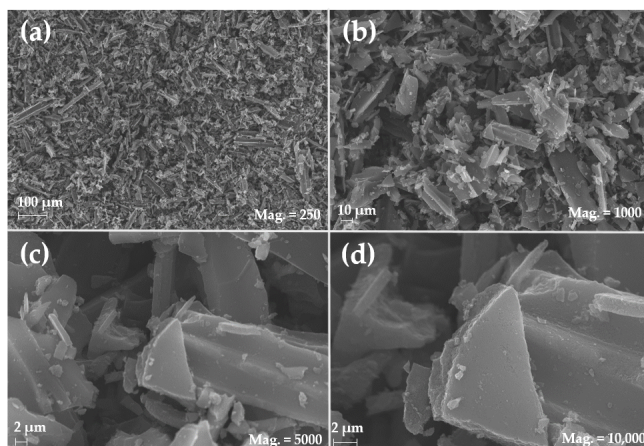
Abbildung 10.2. REM-Bilder von 5% Pt/C in Vergrößerungen von 250 bis 10.000. Alle Bilder wurden mit den folgenden Parametern aufgenommen: EHT=20.0 kV, WD=8.5 mm, SingalA=InLens. Entommen aus [153] CC 4.0, ©2021 Häusler et al.
