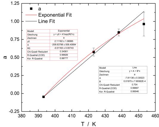
Abbildung 11.17. Darstellung der Pseudo-Reaktionsordnung a in Abhängigkeit der Reaktionstemperatur. Die Regression von a wurde mit einer Exponentialfunktion, sowie einer linearen Funktion mit Gewichtung durch die Fehler der Messpunkte durchgeführt. Reaktionsbedingungen: m_{\text{Ni}_{99}\text{Pt}_1/\text{C}} = 250 \text{ mg} , w_{\text{Metall}} = 5 \% , \varnothing_{\text{Pulver}} < 75 \mu\text{m} , t_R = 4 \text{ h} , c_{\text{NaOH}} = 450 \text{ mmol/L} , c_{n\text{-Decan}} = 15 \text{ mmol/L} , V_R = 70 \text{ ml} . Tabellierte Rohdaten in Tabelle B.8. Reproduziert aus [152] mit Genehmigung der Royal Society of Chemistry.
