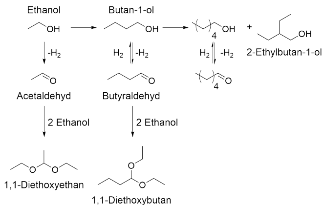
Abbildung 3.3. Reaktionsschema für die Dimerisierung von Ethanol zu 1-Butanol am basischen Zeolithkatalysator. Hierbei unterläuft Ethanol einer direkten Dimerisierung unter Wasserfreisetzung. Die Aldehyde stellen lediglich Nebenprodukte der Dehydrierung dar. Adaptiert aus [75] Copyright ©1993 Academic Press. All rights reserved.
