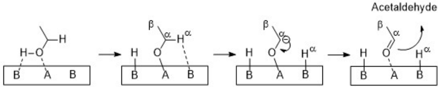
Schema 3.1 Mechanismus für die Dehydrierung von Ethanol auf Mg/Al-Oxiden. A und B stellen Lewis-Säure bzw. Brønsted-Basen Zentren dar. Entnommen aus [76] ©1998 Academic Press.
