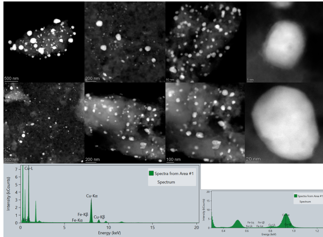
Abbildung D.11. Gesamtheit der TEM-Aufnahmen des \text{Cu}_{99}\text{Fe}_1/\text{C} Katalysators bei verschiedenen Vergrößerungen im Dunkelfeld mit Spektrum der EDX-Messungen der Einzelpartikel.
