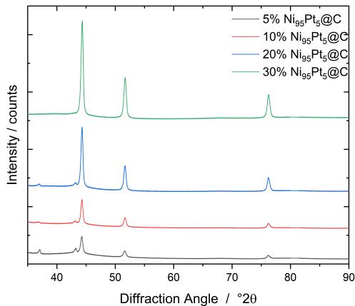
Abbildung 11.21. Darstellung der Diffraktogramme für den Ni 95 Pt 5 @C-Katalysator mit unterschiedlichen Beladungen. Messbedingungen: K_{\alpha}(Cu) , \lambda = 1.5419 \text{ \AA} , Schrittweite=0.02 deg/s. Reproduziert aus [180] mit Genehmigung der Royal Society of Chemistry.
