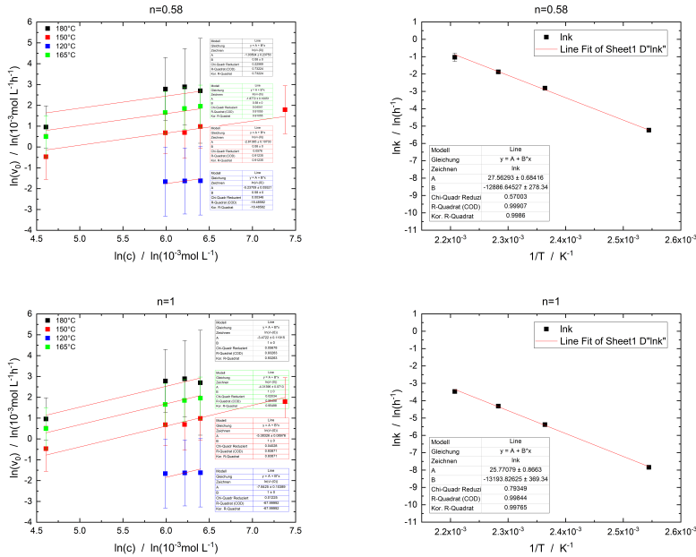
Abbildung D.18. Auftragung der ermittelten kinetischen Parameter bei fester Pseudo-Reaktionsordnung n (links) gegen die Reaktionstemperatur. Die Regression wurde mit einer linearen Funktion mit Gewichtung durch die Fehler der Messpunkte durchgeführt. (Rechts) Arrheniusplot der temperaturabhängigen Reaktionskonstante k . Die Regression wurde mit der logarithmierten Arrheniusfunktion durchgeführt. Reaktionsbedingungen: m_{\text{Ni}_{99}\text{Pt}_{1/\text{C}}} = 250 \text{ mg} , w_{\text{Metall}} = 5 \% , \varnothing_{\text{Pulver}} < 75 \mu\text{m} , t_R = 4 \text{ h} , c_{\text{NaOH}} = 450 \text{ mmol/L} , c_{n-\text{Decan}} = 15 \text{ mmol/L} , V_R = 70 \text{ ml}
