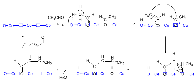
Schema 4.1 Der von Liang et al. vorgeschlagene Mechanismus postuliert, dass die Sauerstoff-Fehlstellen als aktive Zentren in der Aldolkondensation einen wesentlichen Beitrag zur Katalysatoraktivität beitragen [128]. In blau dargestellt die Ceroxid Oberfläche. Die Kästchen symbolisieren Sauerstoff-Fehlstellen.
