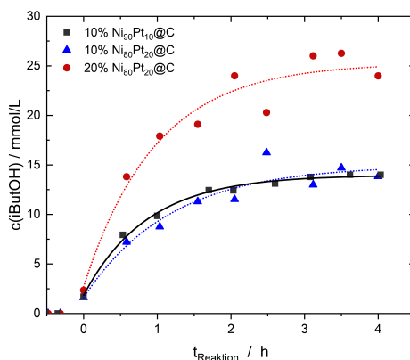
Abbildung 11.26. Darstellung der i -Butanolkonzentration als Funktion der Reaktionszeit, für die Ni x Pt 1-x @C-Katalysatoren der Gruppe III und IV. Reaktionsbedingungen: m_{Kat} = 250 mg, T = 165 °C, c_0(EtOH) = 600 mmol/L, c(NaOH) = 450 mmol/L, t_R = 4 h, V_R = 70 mL, N_{Rührer} = 1000 rpm. Die Werte der Anpassungsfunktionen sind in Tabelle B.9 tabelliert. Reproduziert aus [180] mit Genehmigung der Royal Society of Chemistry.
