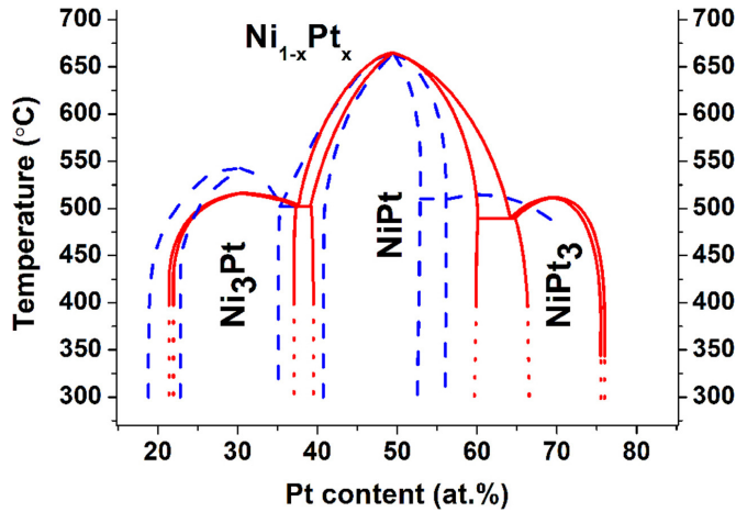
Abbildung A.2. Phasendiagramm des Ni-Pt Systems über den gesamten Mischungsbereich \text{Ni}_{1-x}\text{Pt}_x mit 0 < x < 1 . In rot ist das von Popov et al. ermittelte Phasendiagramm dargestellt. Die gestrichelten Linien deuten Extrapolationen in den tieferen Temperaturbereich an. In blau ist das bisher von Cadeville et al. publizierte Phasendiagramm dargestellt. Entnommen mit Genehmigung aus [197], ©2021, Elsevier B.V.
