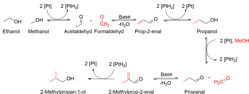
Schema 12.1 Reaktionsmechanismus für die C-Methylierung von Ethanol zu 2-Methylpropanol. In rot dargestellt sind die neu hinzukommenden, aus dem Methanol stammenden C-C-Bindungen. In Anlehnung an [109] CC 4.0, © 2020 Pasel et al.
