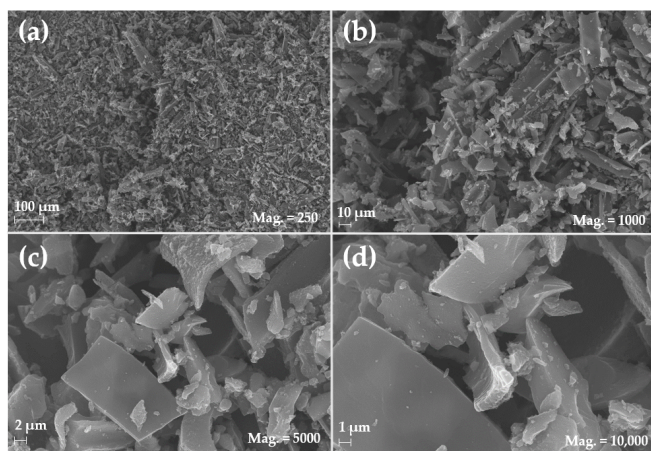
Abbildung 10.1. REM-Bilder von 5% Pd/C in Vergrößerungen von 250 bis 10.000. Alle Bilder wurden mit den folgenden Parametern aufgenommen: EHT=20.0 kV, WD=8.5 mm, SingalA=InLens. Entommen aus [153] CC 4.0, ©2021 Häusler et al.
