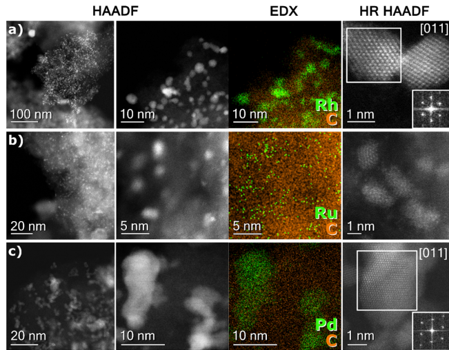
Abbildung 10.8. HAADF-STEM-Aufnahmen der monometallischen Katalysatoren Rh/C, Ru/C und Pd/C zeigen die Verteilung des Katalysators auf dem C-Träger. Daneben zeigen die Übersichtsbilder und entsprechenden EDX-Elementkarten den orangefarbenen C-Träger mit den grün gefärbten Metallen des Rh/C-Katalysators in Reihe a), des Ru/C-Katalysators in Reihe b) und des Pd/C-Katalysators in Reihe c). Die HR-HAADF-STEM-Bilder von Einzelkatalysator-Nanopartikeln sind auf der rechten Seite dargestellt, mit Fast-Fourier-Transform-Mustereinblendungen für Rh und Pd. Entommen aus [153] CC 4.0, ©2021 Häusler et al.
