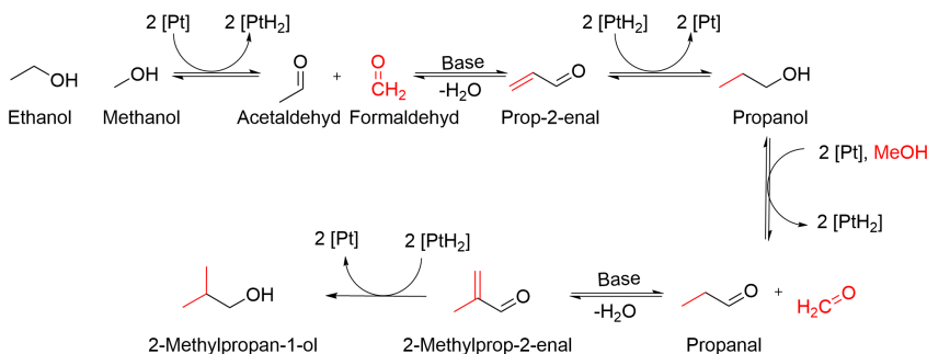
Schema 9.1 Reaktionsmechanismus für die C-Methylierung von Ethanol zu 2-Methylpropanol. In rot dargestellt sind die neu hinzukommenden, aus dem Methanol stammenden C-C-Bindungen. In Anlehnung an [109] CC 4.0, © 2020 Pasel et al.
