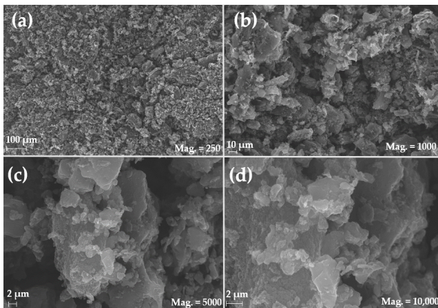
Abbildung 10.4. REM-Bilder von 5% Ru/C in Vergrößerungen von 250 bis 10.000. Alle Bilder wurden mit den folgenden Parametern aufgenommen: EHT=20.0 kV, WD=8.5 mm, SingalA= InLens. Entommen aus [153] CC 4.0, ©2021 Häusler et al.
