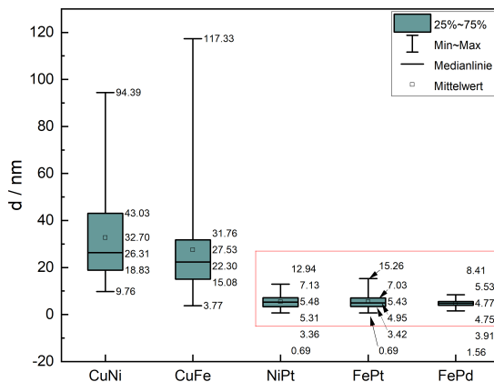
Abbildung 11.11. Boxplot der Partikelverteilung aus den TEM-Aufnahmen für die Katalysatoren \text{Ni}_{99}\text{Pt}_1/\text{C} , \text{Cu}_{99}\text{Ni}_1/\text{C} , \text{Cu}_{99}\text{Fe}_1/\text{C} , \text{Fe}_{99}\text{Pt}_1/\text{C} und \text{Fe}_{99}\text{Pd}_1/\text{C} . In der Box ist das zweite und dritte Quartil und der Median angegeben. Der Mittelwert wird durch ein Kästchen dargestellt. Die Wisker stellen die Extrema der Partikelgrößen dar. Der rote Kasten ist vergrößert in Abb. D.16 dargestellt. Entommen aus [151] CC 4.0, © 2024 Häusler et al.
