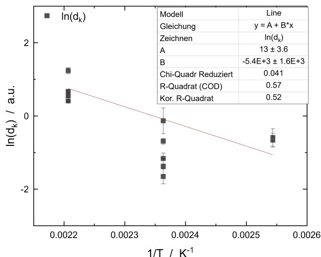
Abbildung 10.16. Arrheniusdiagramm für die Deaktivierungsrate d_k des Pt/C-Katalysators aus den Daten von Tabelle B.1
