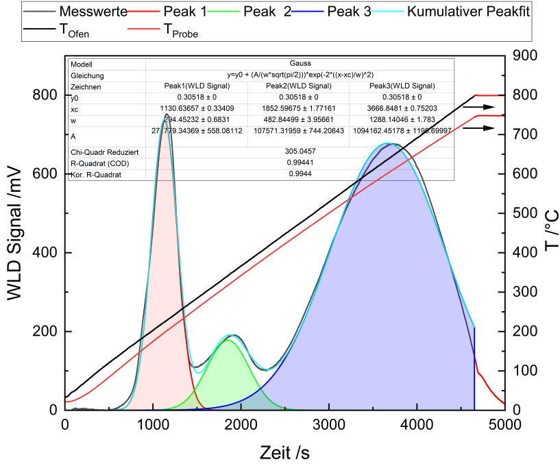
Abbildung D.2. TPR Profil des CuNi/C Katalysators mit Peakzerlegung mittels Gauss -Funktionen. Messbedingungen: m_{Kat}=88.3 mg, 2 %H 2 in Argon, \dot{V}=30 mL/min; \beta=10 K/min. Der Kalibrierfaktor f_{WLD}=9.19209 \cdot 10^{-8} mmols/mV wurde mit CuO 99.9995 % Reinheit ermittelt. Die Peakzerlegung wurde mit dem Peakanpassungstool der Software OriginPro , Version 2021. OriginLab Corporation, Northampton, MA, USA, durchgeführt. Die Basislinie wurde auf 0.31 mV festgelegt. Messdaten ab Temperaturen über 779 °C wurden maskiert, um Einflüsse der verlangsamten Heizrate zu reduzieren.
