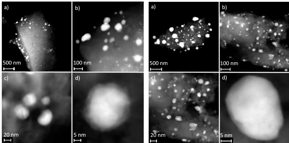
(a) TEM-Aufnahmen des \text{Cu}_{99}\text{Ni}_1/\text{C} Katalysators bei verschiedenen Vergrößerungen im Dunkelfeld. (b) TEM-Aufnahmen des \text{Cu}_{99}\text{Fe}_1/\text{C} Katalysators bei verschiedenen Vergrößerungen im Dunkelfeld.
