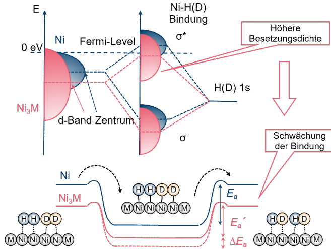
Abbildung 2.4. Darstellung des Energiediagramms für die DOS von Nickel und den intermetallischen Verbindungen nach Wechselwirkung mit dem Wasserstoff(Deuterium)-Atom und der daraus resultierenden Reduktion der Aktivierungsenergie für die dissoziative Isomerisierung von Wasserstoff. Reproduziert aus [44] mit Genehmigung der Royal Society of Chemistry.
