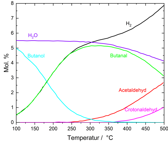
Abbildung 3.4. Thermodynamisches Gleichgewicht für die Guerbet Reaktion in Abhängigkeit der Temperatur. Adaptiert aus [81] Copyright ©2014 Elsevier B.V. All rights reserved
