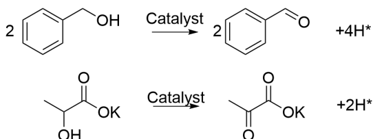
Abbildung 3.1. Initiation des Reaktionsmechanismus durch Dehydrierung der Alkoholfunktionalitäten von Benzylalkohol und Kaliumlactat am Katalysator [73]
