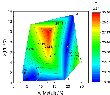
Abbildung 11.27. Darstellung des sich einstellenden Reaktordrucks als Funktion der Katalysatorbeladung und dem Stoffmengenanteil Platin für die \text{Ni}_x\text{Pt}_{1-x} @C-Katalysatoren mit 80 > x > 1 . Bezeichnung d: Katalysator deaktiviert. s: Konzentrationsmessung streut und ist nicht streng linear. nd: Katalysator deaktiviert nicht, linearer Produktanstieg in Abhängigkeit von t_R . Messbedingungen: m_{Kat} = 250 mg, T = 165 °C, c(\text{EtOH}) = 600 mmol/L, c(\text{NaOH}) = 450 mmol/L, t_R = 4 h, V_R = 70 mL, N_{Rührer} = 1000 rpm.
