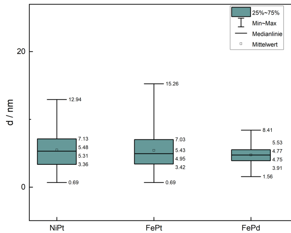
Abbildung D.16. Vergrößerter Boxplot der Partikelverteilung aus den TEM-Aufnahmen für die Katalysatoren \text{Ni}_{99}\text{Pt}_1/\text{C} , \text{Fe}_{99}\text{Pt}_1/\text{C} und \text{Fe}_{99}\text{Pd}_1/\text{C} . In der Box ist das zweite und dritte Quartil und der Median angegeben. Der Mittelwert wird durch ein Kästchen dargestellt. Die Wisker stellen die Extrema der Partikelgrößen dar.
