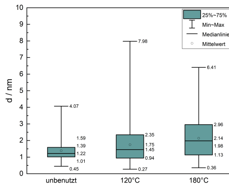
Abbildung 10.18. Boxplot der Partikelverteilung aus den TEM-Aufnahmen für den Pt/C Katalysator vor und nach der Reaktion. In der Box ist das zweite und dritte Quartil und der Median angegeben. Der Mittelwert wird durch ein Kästchen dargestellt. Die Wisker stellen die Extrema der Partikelgrößen dar. Reaktionsbedingungen: t_R = 4 h, m_{Katalysator} = 250 mg, V_R = 70 mL, c_{EtOH} = 600 mol/dm 3 . Stichprobengröße N_{frisch} = 107 , N_{120^\circ C} = 410 , N_{180^\circ C} = 635 .
