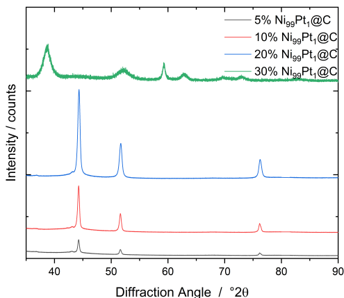
Abbildung 11.20. Darstellung der Diffraktogramme für den \text{Ni}_{99}\text{Pt}_1\text{@C} -Katalysator mit unterschiedlichen Beladungen. Messbedingungen: K_{\alpha}(\text{Cu}) , \lambda = 1.5419 \text{ \AA} , Schrittweite = 0.02 \text{ deg/s} . Reproduziert aus [180] mit Genehmigung der Royal Society of Chemistry.
