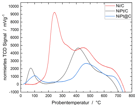
Abbildung 11.6. TPR Messungen der durch Imprägnierung hergestellten Nickelkatalysatoren Ni/C, NiPt/C und NiPt@C. Dargestellt ist das Massennormierte Signal des WLD. Messbedingungen: 2 %H 2 in Argon, \dot{V} = 30 mL/min; \beta = 10 K/min. Entnommen aus [151] CC 4.0, © 2024 Häusler et al.
