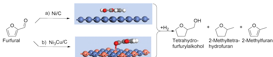
Abbildung 2.3. Energetisch günstigste Bindungsgeometrien von Furfural: a) parallele Adsorptionsgeometrie auf der Nickeloberfläche b) leicht gekippte Adsorptionsgeometrie auf der \text{Ni}_3\text{Cu} -Oberfläche. Adaptiert aus [43] mit Genehmigung von Elsevier.
