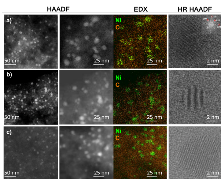
Abbildung 11.18. HAADF-STEM und EDX-Messungen von: (a) frischem \text{Ni}_{99}\text{Pt}_1/\text{C} -Katalysator (oberer Teil) ; (b) \text{Ni}_{99}\text{Pt}_1/\text{C} -Katalysator nach 4 h Reaktionsdauer bei 180 °C (mittlerer Teil); und (c) \text{Ni}_{99}\text{Pt}_1/\text{C} -Katalysator nach 24 h Reaktionsdauer bei 150 °C (unterer Teil). Nickel ist in den EDX-Karten in Grün und der C-Träger in Orange dargestellt. Platin konnte nicht detektiert werden und wurde daher nicht im EDX dargestellt. HR-HAADF-STEM-Bilder zeigen eine Nahaufnahme von Nanopartikeln mit Fast-Fourier-Transform (FFT)-Mustern wo möglich. Reproduziert aus [152] mit Genehmigung der Royal Society of Chemistry.
