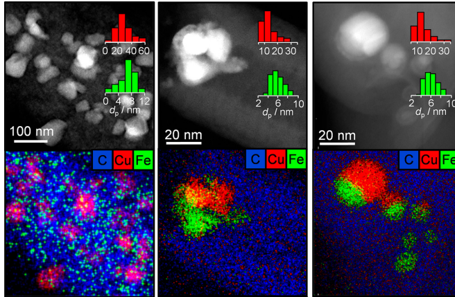
Abbildung A.1. TEM und EDX-Messungen für den Cu 2 Fe-Katalysator auf unterschiedlichen Kohlenstoffträgern. Links: Reduzierter Katalysator auf Aktivkohle. Mitte: Reduzierter Katalysator auf konischen Kohlenstoff-Nanofasern mit Kaliumzusatz vor der Reaktion. Rechts: Reduzierter Katalysator auf konischen Kohlenstoff-Nanofasern mit Kaliumzusatz nach der Reaktion. Adaptiert mit Genehmigung aus [190]. ©2018 American Chemical Society.
