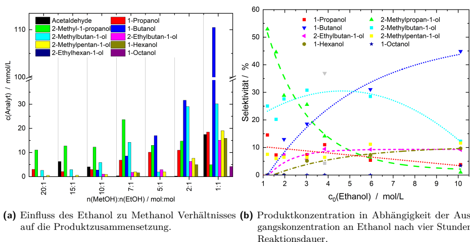
Abbildung 9.2. Reaktionsbedingungen: Katalysator Pt/C, m_{\text{Kat,trocken}} = 250\text{ mg} , w_{\text{Pt}} = 5\% , \varnothing_{\text{Pulver}} < 75\text{ }\mu\text{m} , t_R = 4\text{ h} , T_R = 150\text{ }^\circ\text{C} , c_{\text{EtOH}} = 5900\text{ mmol/L} , \text{MeOH:EtOH}=2:1 , c_{\text{NaOH}} = 450\text{ mmol/L} , c_{\text{n-Decan}} = 15\text{ mmol/L} , V_R = 70\text{ ml} .
