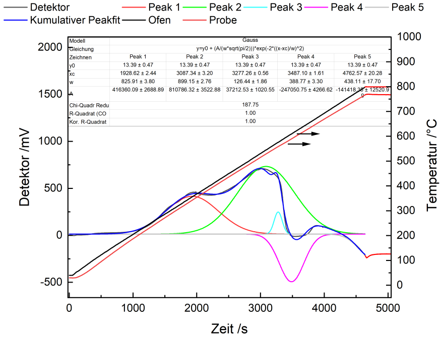
Abbildung D.9. TPR Profil des FePt/C Katalysators mit Peakzerlegung mittels Gauss -Funktionen. Messbedingungen: m_{Kat}=81.8 mg, 2 %H 2 in Argon, \dot{V}=30 mL/min; \beta=10 K/min. Der Kalibrierfaktor f_{WLD}=9.19209 \cdot 10^{-8} mmols/mV wurde mit CuO 99.9995 % Reinheit ermittelt. Die Peakzerlegung wurde mit dem Peakanpassungstool der Software OriginPro , Version 2021. OriginLab Corporation, Northampton, MA, USA, durchgeführt. Die Basislinie wurde auf 0.00 mV festgelegt. Messdaten ab Temperaturen über 798 °C wurden maskiert, um Einflüsse der verlangsamten Heizrate zu reduzieren.
