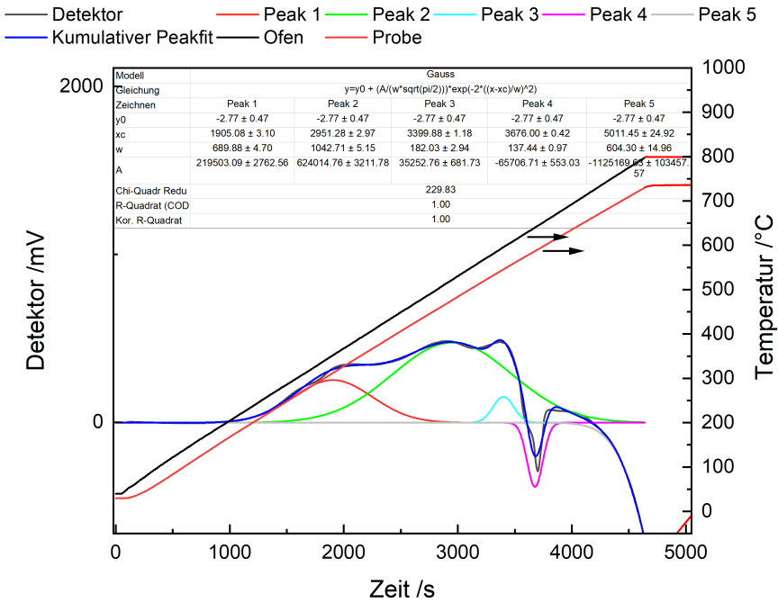
Abbildung D.8. TPR Profil des FePd/C Katalysators mit Peakzerlegung mittels Gauss -Funktionen. Messbedingungen: m_{Kat}=54.1 mg, 2 %H 2 in Argon, \dot{V}=30 mL/min; \beta=10 K/min. Der Kalibrierfaktor f_{WLD}=9.19209 \cdot 10^{-8} mmols/mV wurde mit CuO 99.9995 % Reinheit ermittelt. Die Peakzerlegung wurde mit dem Peakanpassungstool der Software OriginPro , Version 2021. OriginLab Corporation, Northampton, MA, USA, durchgeführt. Die Basislinie wurde auf 0.00 mV festgelegt. Messdaten ab Temperaturen über 798 °C wurden maskiert, um Einflüsse der verlangsamten Heizrate zu reduzieren.
