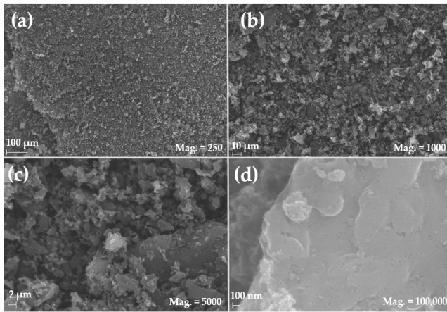
Abbildung 10.3. REM-Bilder von 5% Rh/C in Vergrößerungen von 250 bis 100.000. Alle Bilder wurden mit den folgenden Parametern aufgenommen: EHT=20.0 kV, WD=8.5 mm, SingalA= InLens. Entommen aus [153] CC 4.0, ©2021 Häusler et al.
