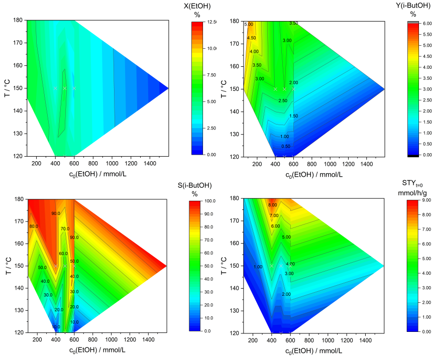
Abbildung 10.13. Ethanolumsatz, Ausbeute und Selektivität als Funktion der Reaktionstemperatur und der Startkonzentration Ethanol. Die STY ist im gleichen Parameterfeld dargestellt. Die Kennzahlen wurden zum Ende der Reaktionsdauer ermittelt. Messpunkte wurden als graue Kreuze dargestellt. Zwischen den Messpunkten wurde linear interpoliert. Eingesetzt wurde der kommerzielle Pt/C-Katalysator. Reaktionsbedingungen: m_{Kat,trocken} = 250 \text{ mg} , w_{Metall} = 5 \% , \varnothing_{Pulver} < 75 \mu\text{m} , t_R = 4 \text{ h} , c_{NaOH} = 450 \text{ mmol/L} , c_{n-Decan} = 15 \text{ mmol/L} , V_R = 70 \text{ ml}
