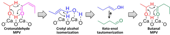
Abbildung 3.6. Reaktionsmechanismus für die Transferhydrierung mittels Meerwein-Verley-Ponendorf Mechanismus auf dem HAP-Katalysator. Entnommen mit Genehmigung aus [86] Copyright ©2015 American Chemical Society
