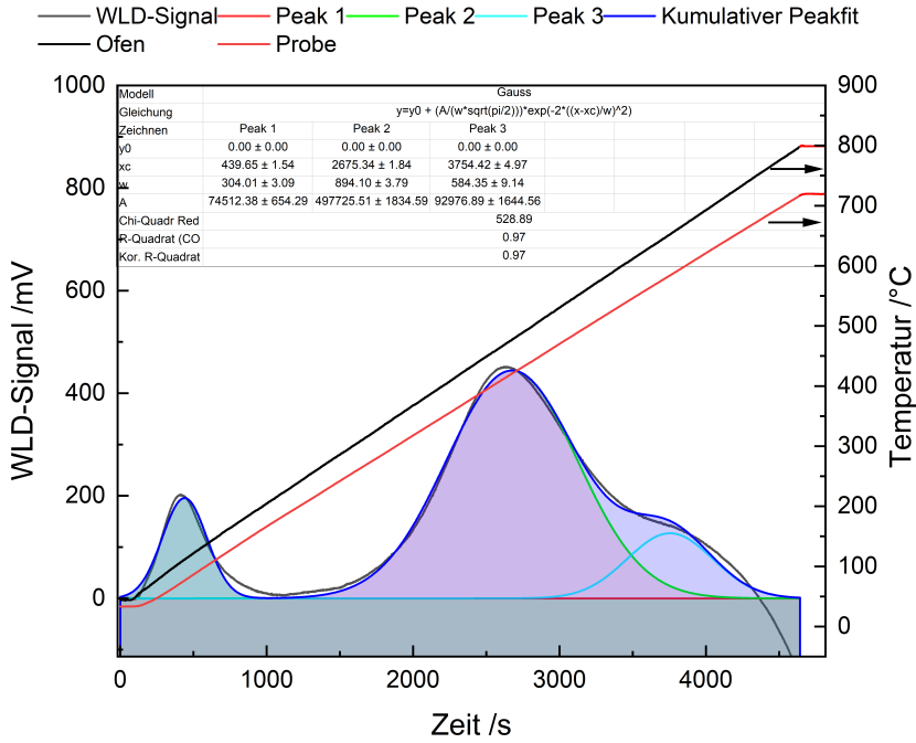
Abbildung D.5. TPR Profil des NiPt/C Katalysators mit Peakzerlegung mittels Gauss -Funktionen. Messbedingungen: m_{Kat}=80.7 mg, 2 %H 2 in Argon, \dot{V}=30 mL/min; \beta=10 K/min. Der Kalibrierfaktor f_{WLD}=9.19209 \cdot 10^{-8} mmols/mV wurde mit CuO 99.9995 % Reinheit ermittelt. Die Peakzerlegung wurde mit dem Peakanpassungstool der Software OriginPro , Version 2021. OriginLab Corporation, Northampton, MA, USA, durchgeführt. Die Basislinie wurde auf 0.00 mV festgelegt. Messdaten ab Temperaturen über 798 °C wurden maskiert, um Einflüsse der verlangsamten Heizrate zu reduzieren.
