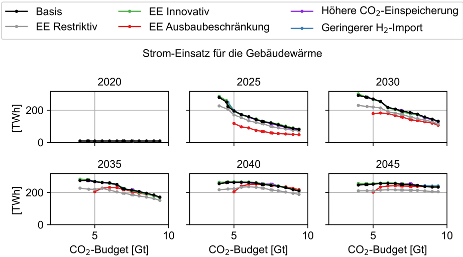
Abbildung C.162: Einsatz von Strom für die Gebäudewärme der Szenarien in Abhängigkeit des CO 2 -Budgets
