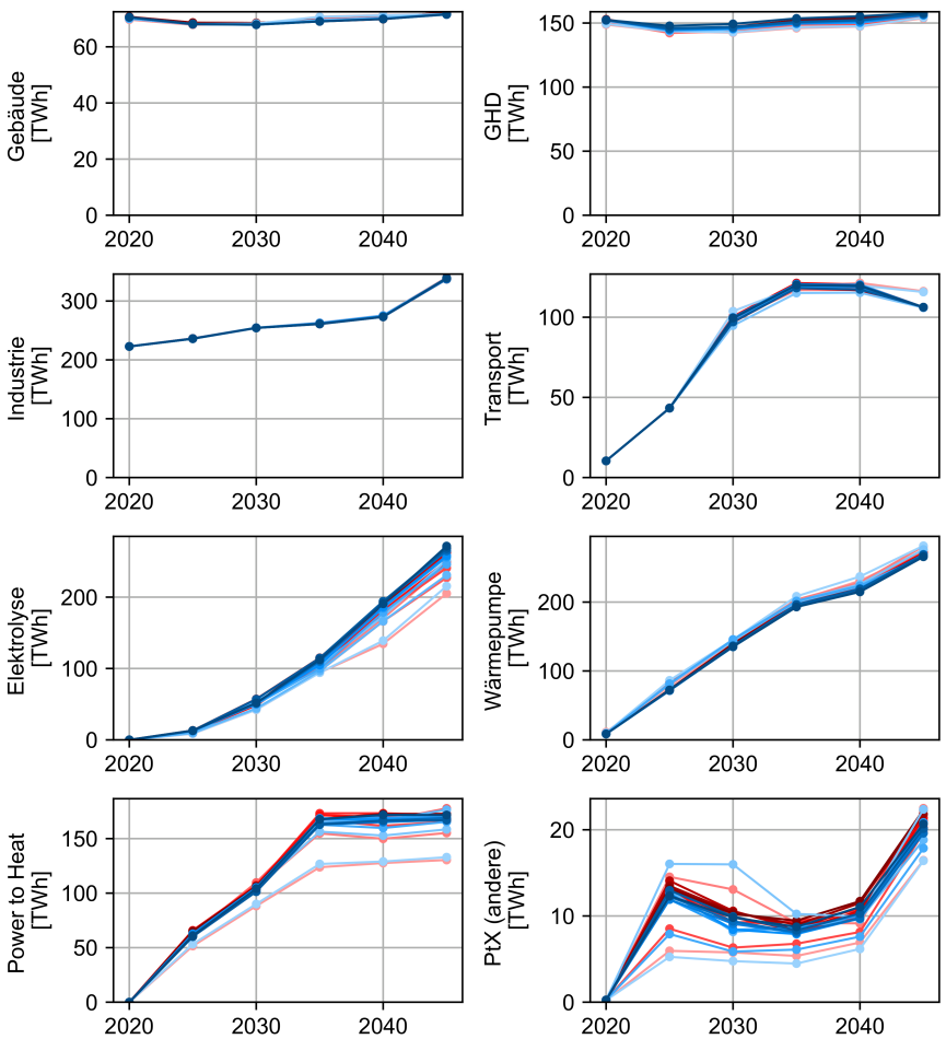
Abbildung C.14: Einfluss der Zeitreihenaggregation auf die Stromnachfrage für die Szenarien mit perfekter Voraussicht
