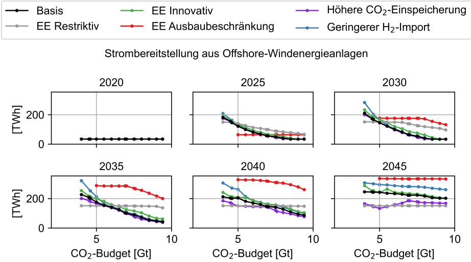
Abbildung C.89: Strombereitstellung durch Offshore-Windenergieanlagen der Szenarien in Abhängigkeit des CO 2 -Budgets
