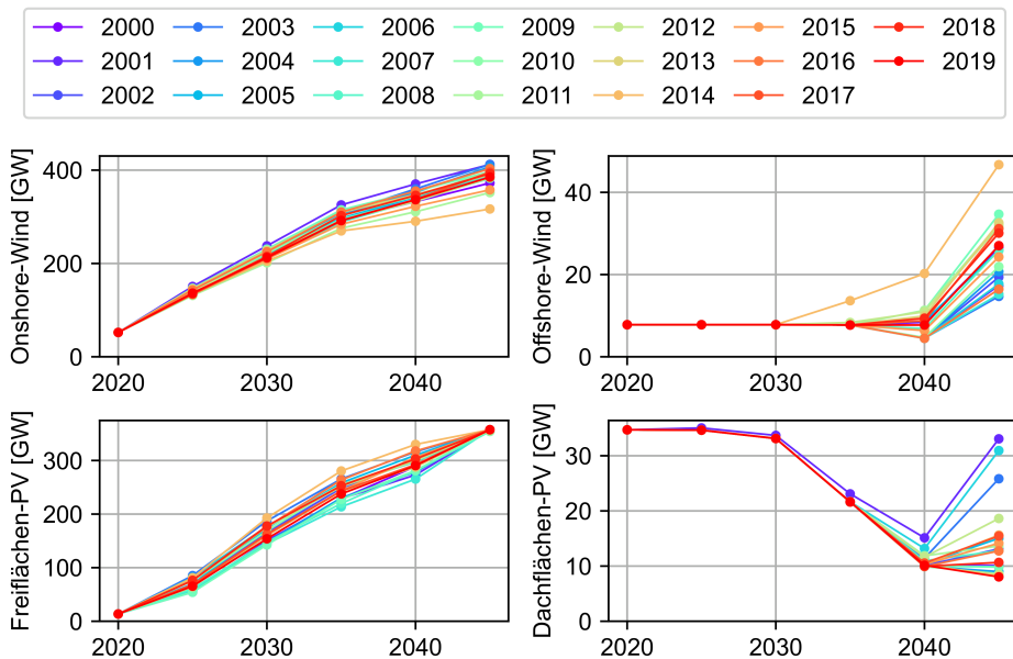
Abbildung 5.11: Einfluss des historischen Wetterjahres zur Simulation der potenziellen Einspeisung der PV- und Windenergieanlagen auf den Ausbau dieser
