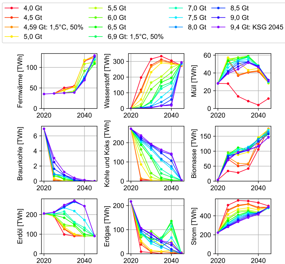
Abbildung 5.40: Einfluss des CO 2 -Budgets auf die Energienachfrage des Industriesektors
