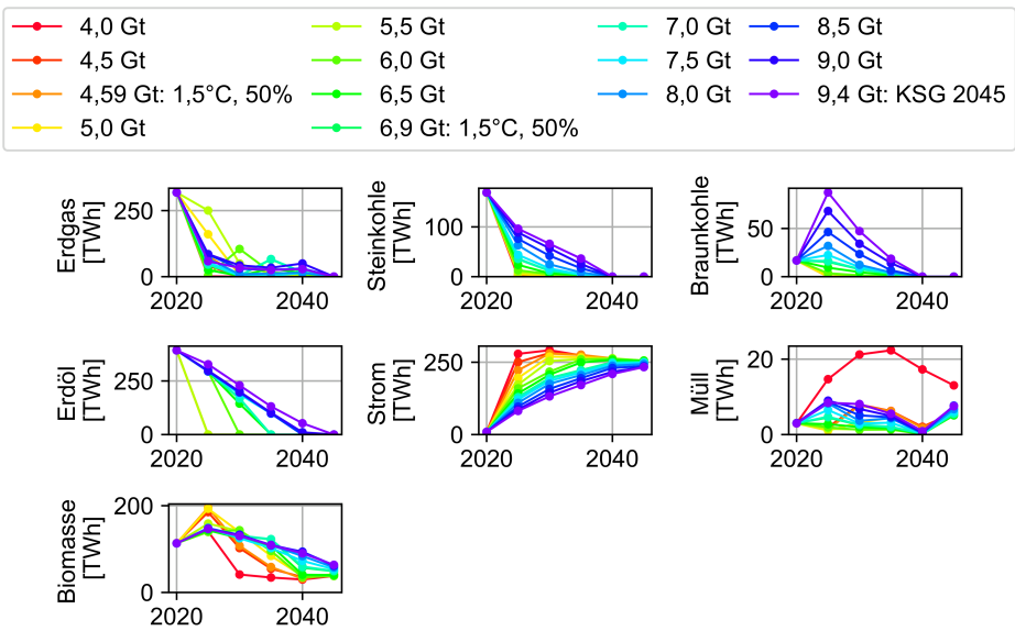
Abbildung C.59: Einfluss des CO 2 -Budgets auf die Wärmeerzeugung der Gebäude des Basis-Szenarios
