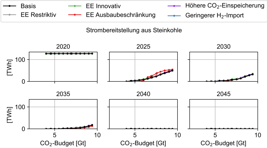
Abbildung C.81: Strombereitstellung durch Steinkohle der Szenarien in Abhängigkeit des CO 2 -Budgets
