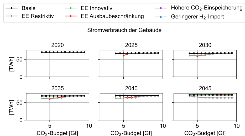
Abbildung C.95: Stromverbrauch der Gebäude der Szenarien in Abhängigkeit des CO 2 -Budgets
