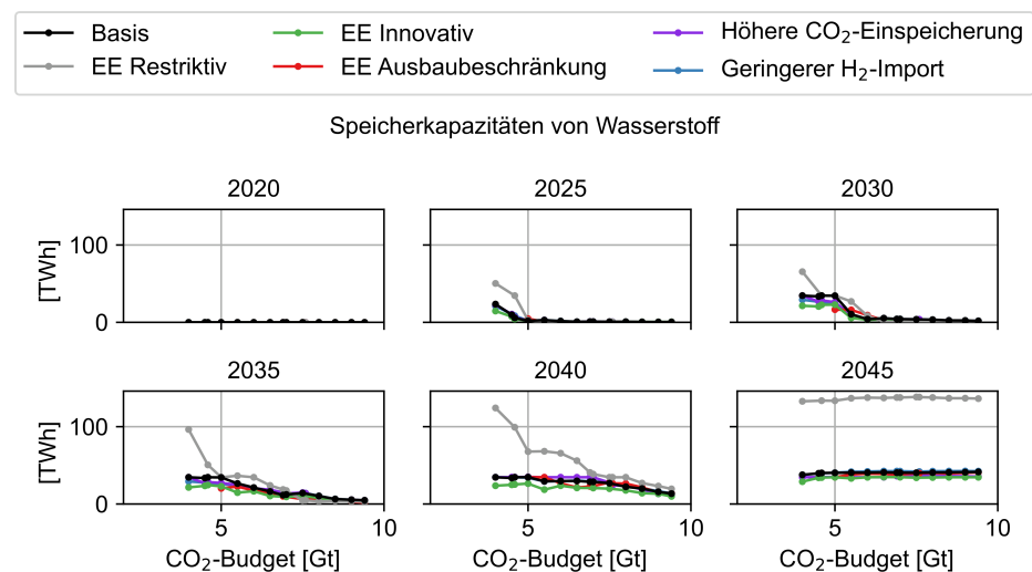
Abbildung C.167: Kapazitäten der Wasserstoffspeicher der Szenarien in Abhängigkeit des CO 2 -Budgets
