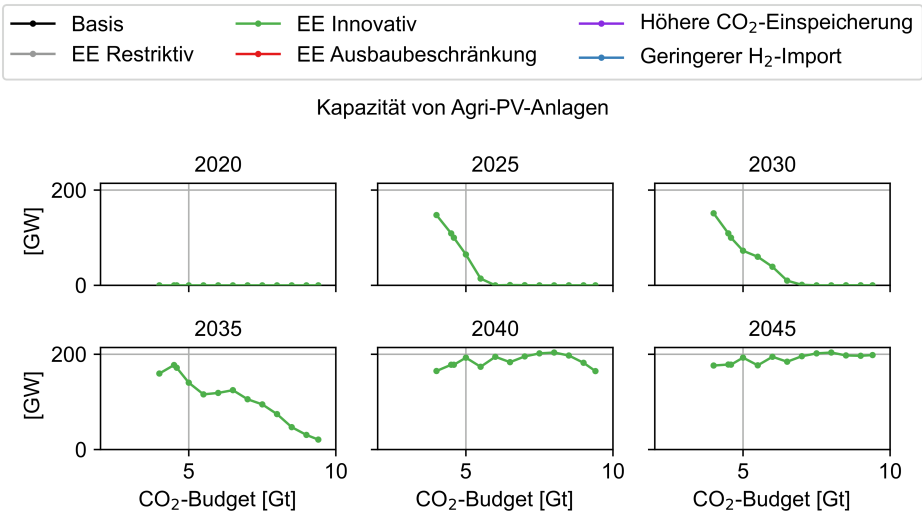
Abbildung C.106: Installierte Leistung der Agri-PV-Anlagen der Szenarien in Abhängigkeit des CO 2 -Budgets
