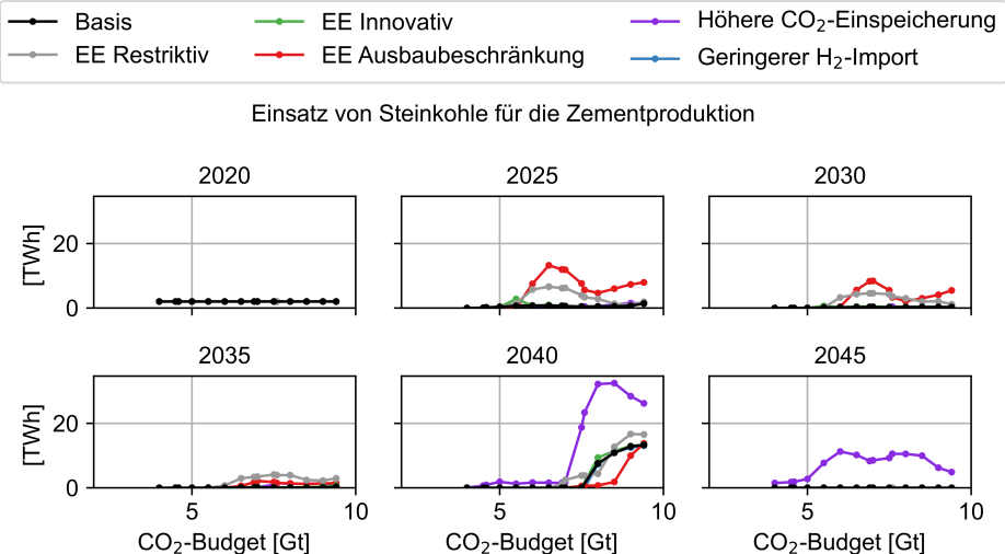
Abbildung C.135: Einsatz von Steinkohle in der Zementproduktion der Szenarien in Abhängigkeit des CO 2 -Budgets
