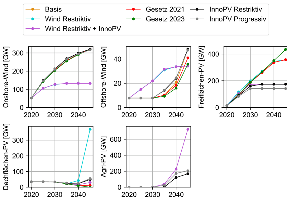
Abbildung 5.3: Einfluss der Potenziale auf den Ausbau der PV- und Windenergieanlagen
