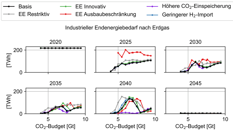
Abbildung C.155: Erdgas-Endenergiebedarf der Industrie der Szenarien in Abhängigkeit des CO 2 -Budgets
