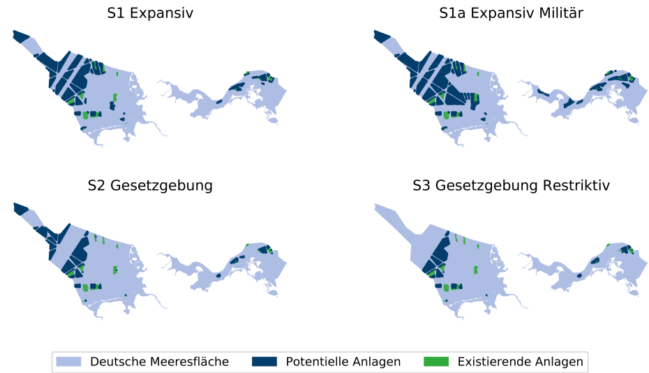
Abbildung 4.4: Potenzielle und existierende Offshore-Windenergieanlagen im deutschen Meeresgebiet pro Szenario
