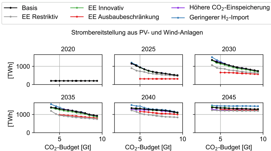
Abbildung 5.52: Strombereitstellung aus PV- und Windenergieanlagen der Szenarien in Abhängigkeit des CO 2 -Budgets
