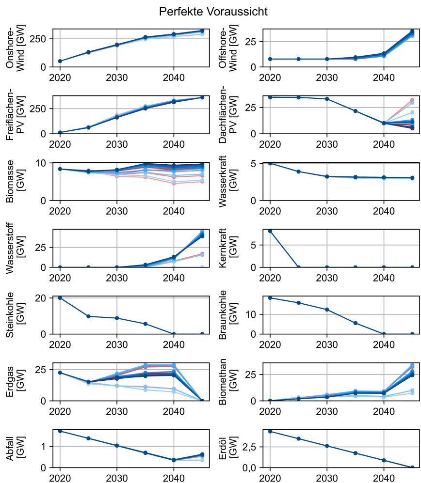
Abbildung C.16: Einfluss der Zeitreihenaggregation auf die Kapazitäten des Stromsystems für die Szenarien mit perfekter Voraussicht
