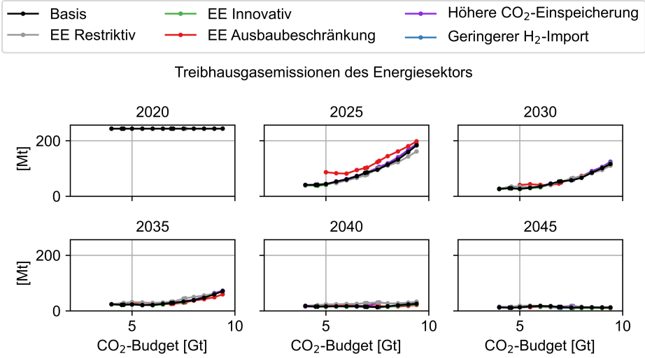
Abbildung C.74: Emissionen des Energiesektors der Szenarien in Abhängigkeit des CO 2 -Budgets
