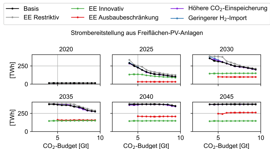
Abbildung C.87: Strombereitstellung durch Freiflächen-PV-Anlagen der Szenarien in Abhängigkeit des CO 2 -Budgets
