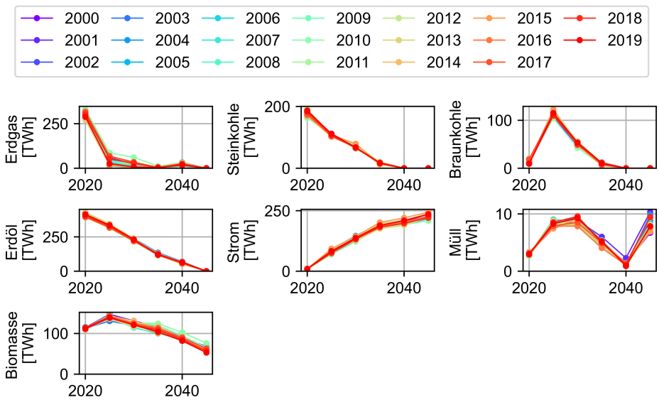
Abbildung C.22: Einfluss des historischen Wetterjahres zur Simulation der potenziellen Einspeisung der PV- und Windenergie-Technologien auf die Wärmebereitstellung im Gebäudesektor
