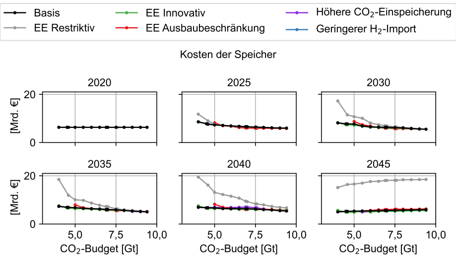
Abbildung C.71: Einfluss des CO 2 -Budgets auf die Kosten der Speicher der Szenarien
