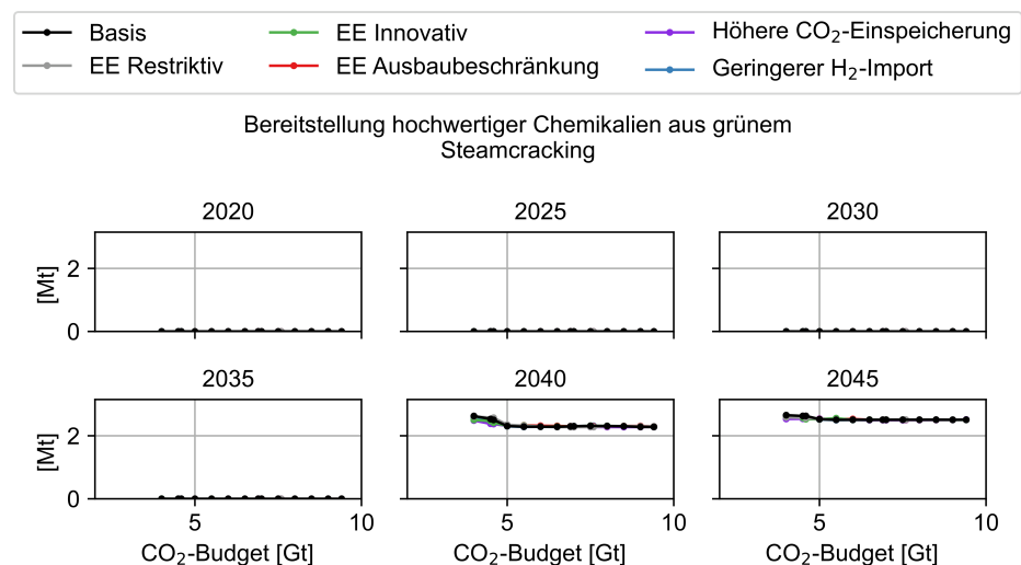
Abbildung C.144: Herstellung hochwertiger Chemikalien aus regenerativ-basiertem Steamcracking der Szenarien in Abhängigkeit des CO 2 -Budgets
