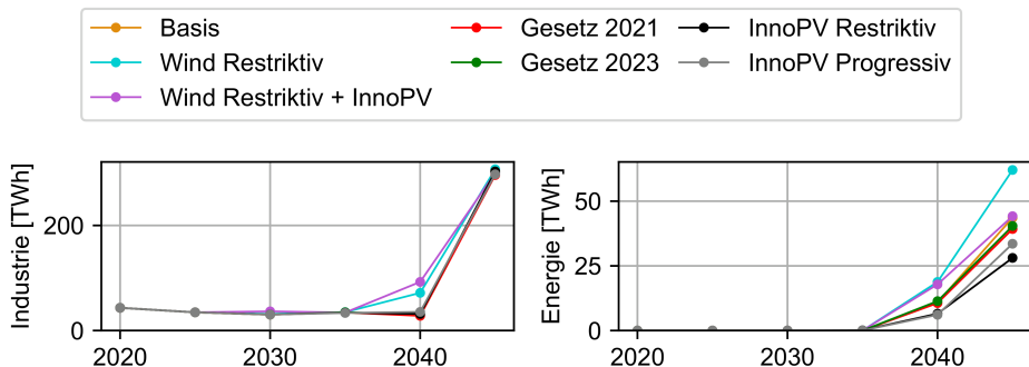
Abbildung 5.7: Einfluss der Potenziale auf die Wasserstoffnachfrage
