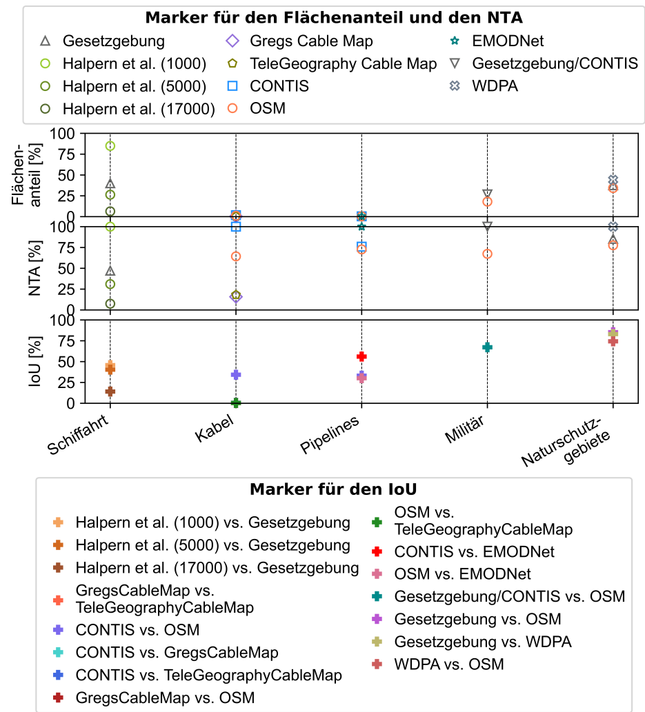
Abbildung 4.1: Analyse des Flächenanteils, der Normalized-Total-Area (NTA) und der Intersection-over-Union (IoU) der Geo-Datensätze für die Potenzialanalyse der Offshore-Windenergieanlagen
