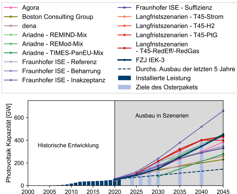
Abbildung 2.12: Historische installierte Kapazität von Photovoltaik-Anlagen in Deutschland, Ausbauziele des Osterpakets und Ausbaupfade der Systemstudien zur Treibhausgasneutralität in 2045
