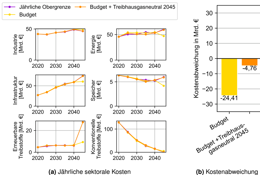
Abbildung 5.34: Einfluss der zeitlichen Emissionsbegrenzung auf die jährlichen sektoralen Kosten und die Gesamtkostenabweichung des Transformationspfades im Vergleich zum Szenario mit jährlichen Emissionsobergrenzen
