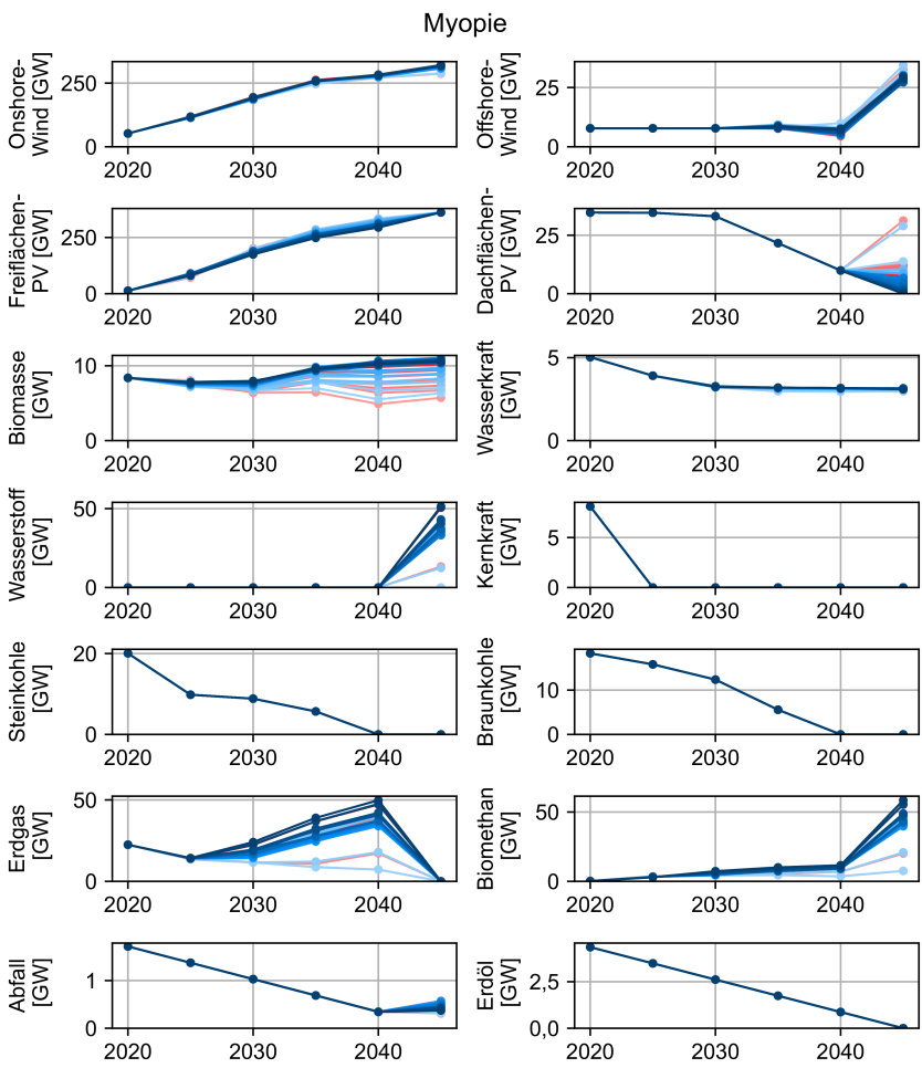
Abbildung C.7: Einfluss der Zeitreihenaggregation auf die Kapazitäten des Stromsystems für die Szenarien mit Myopie
