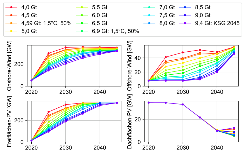
Abbildung 5.38: Einfluss des CO 2 -Budgets auf die Kapazitäten der erneuerbaren Energieträger
