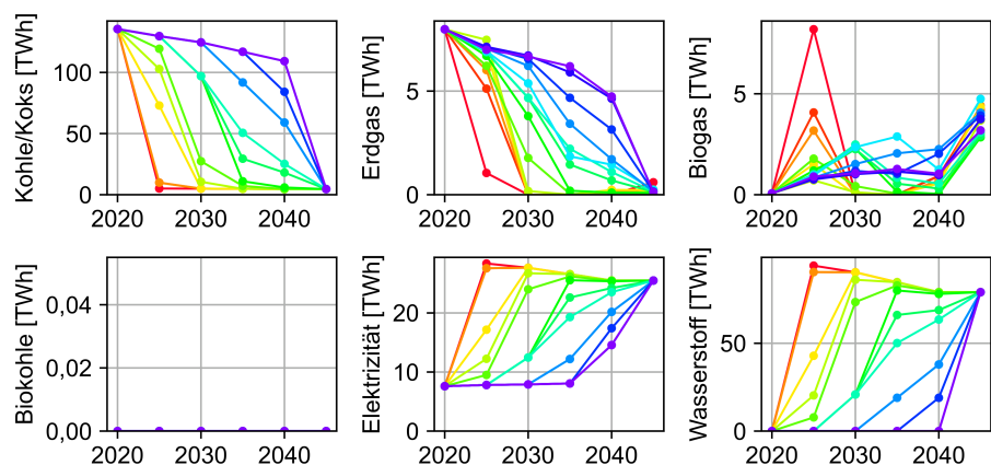
Abbildung C.61: Einfluss des CO 2 -Budgets auf den Energiebedarf der Stahlprozesse des Basis-Szenarios
