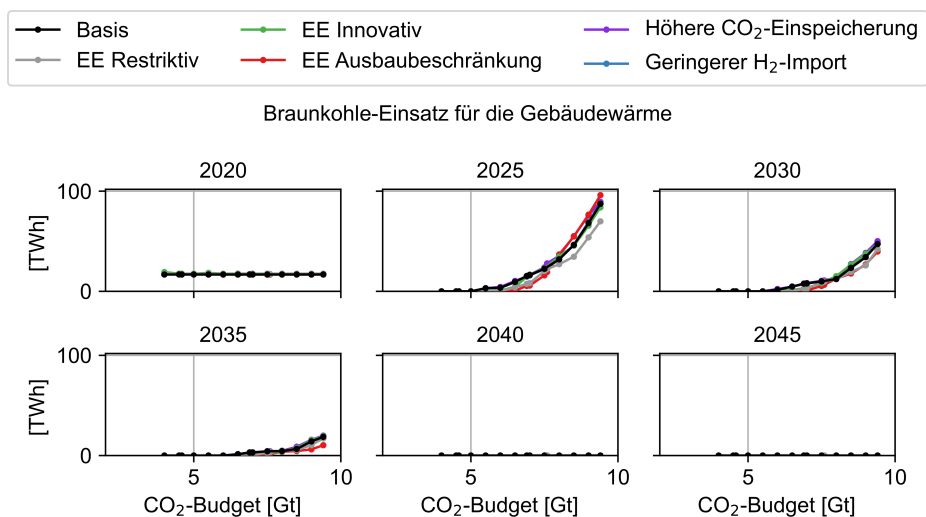
Abbildung C.160: Einsatz von Braunkohle für die Gebäudewärme der Szenarien in Abhängigkeit des CO 2 -Budgets
