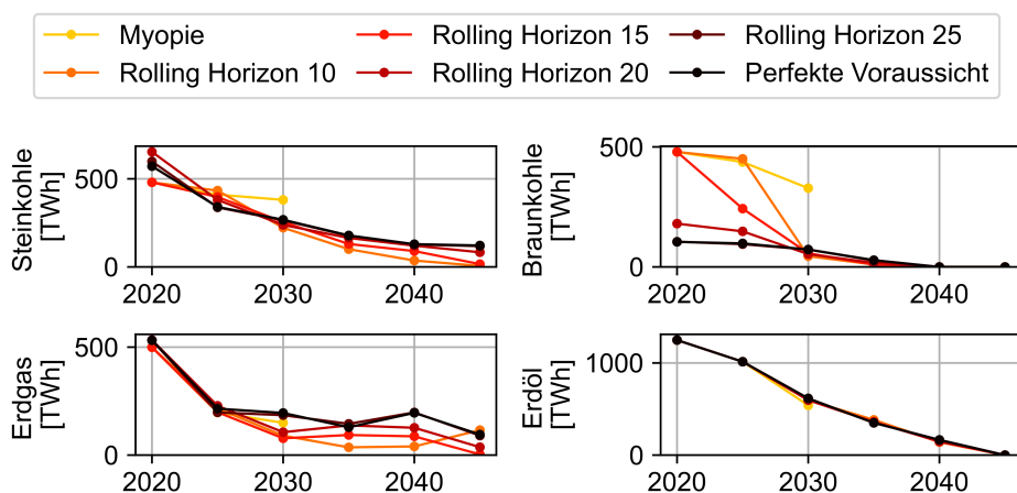
Abbildung 5.27: Einfluss der Voraussicht auf die Primärenergiebereitstellung der zentralen fossilen Energieträger
