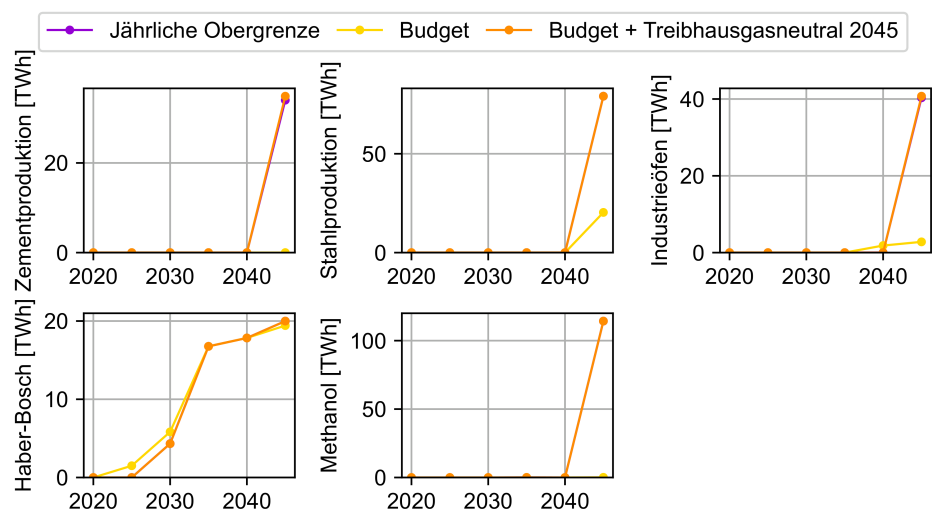
Abbildung C.49: Einfluss der zeitlichen Emissionsbegrenzung auf den Wasserstoffverbrauch
