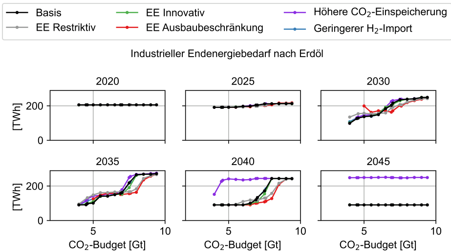
Abbildung C.151: Erdöl-Endenergiebedarf der Industrie der Szenarien in Abhängigkeit des CO 2 -Budgets
