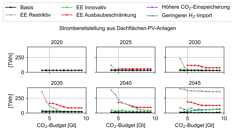
Abbildung C.88: Strombereitstellung durch Dachflächen-PV-Anlagen der Szenarien in Abhängigkeit des CO 2 -Budgets
