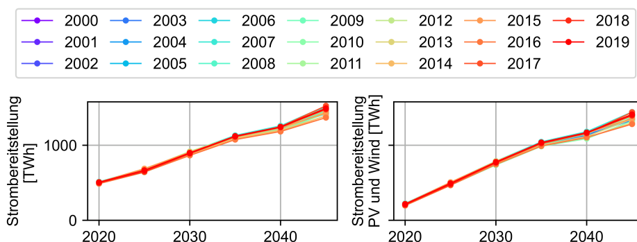
Abbildung 5.12: Einfluss des historischen Wetterjahres zur Simulation der potenziellen Einspeisung der PV- und Windenergieanlagen auf die gesamte Strombereitstellung und die Bereitstellung aus den PV- und Windenergieanlagen
