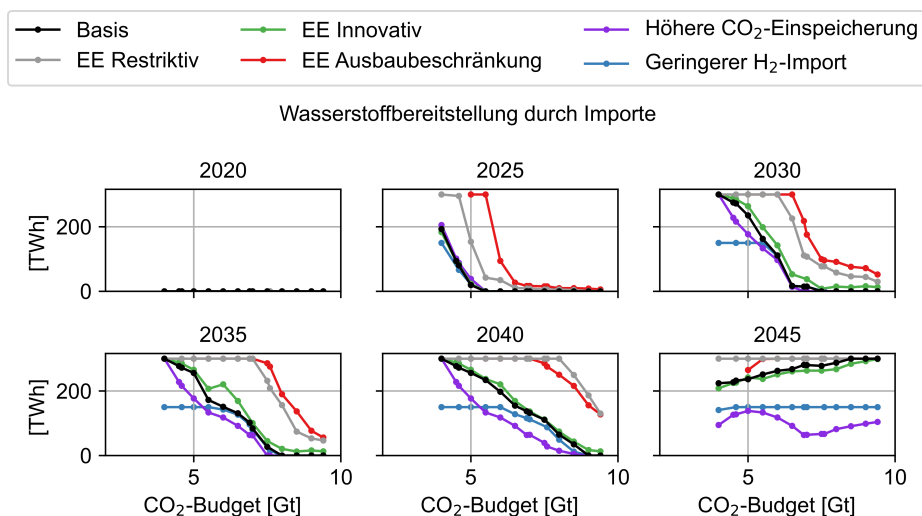
Abbildung 5.45: Wasserstoffimporte der Szenarien in Abhängigkeit des CO 2 -Budgets
