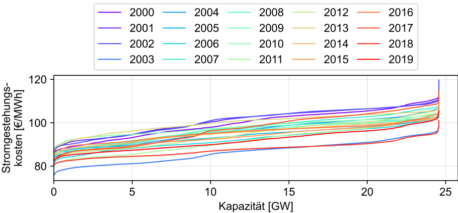
Abbildung 4.11: Stromgestehungskosten der Parkplatz-PV-Anlagen des Szenarios mit mindestens 35 Stellplätzen für Investitionskosten von 1000 €/kW, einem Zinssatz von 6 %, festen Betriebskosten von 1,5 % der Investitionskosten und einer Lebensdauer von 25 Jahren
