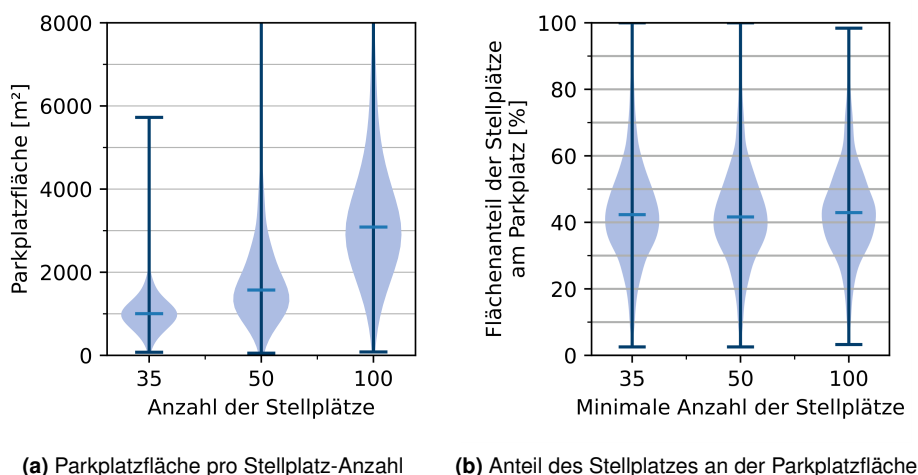
Abbildung 3.1: Verteilung der Parkplatzfläche und der Verteilung des Anteils des Stellplatzes für die Szenarien der Potenzialanalyse von Parkplatz-PV-Anlagen
