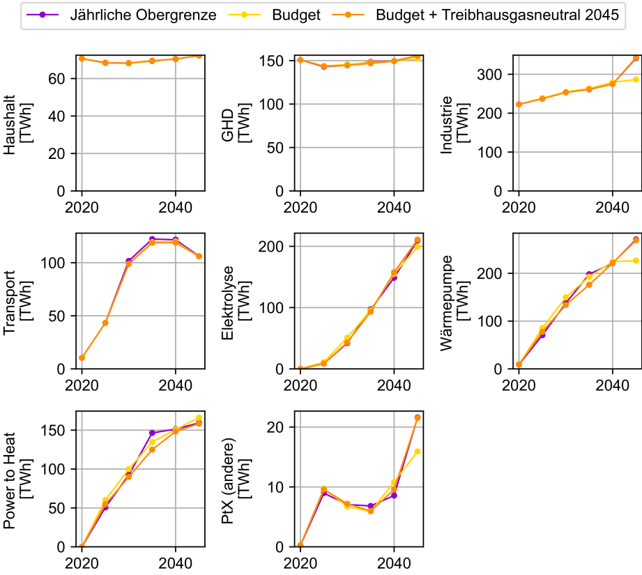
Abbildung C.46: Einfluss der zeitlichen Emissionsbegrenzung auf den Stromverbrauch
