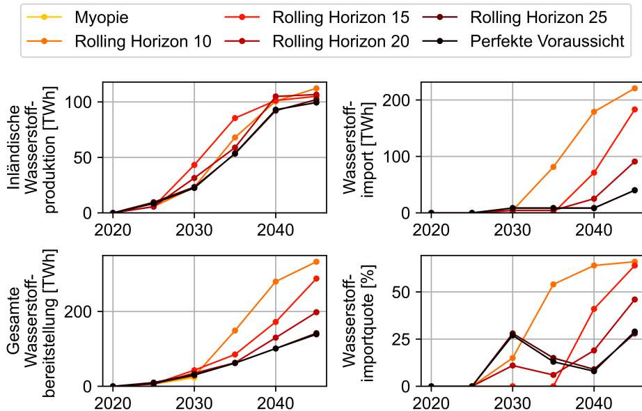
Abbildung 5.26: Einfluss der Voraussicht auf die Wasserstoffbereitstellung
