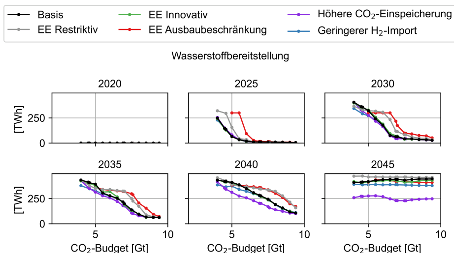
Abbildung 5.51: Wasserstoffbereitstellung der Szenarien in Abhängigkeit des CO 2 -Budgets
