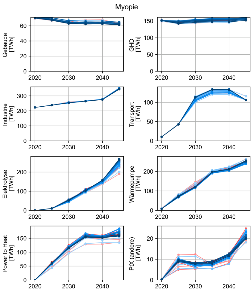
Abbildung C.5: Einfluss der Zeitreihenaggregation auf die Stromnachfrage für die Szenarien mit Myopie
