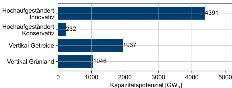
Abbildung 4.6: Kapazitätspotenziale der Agri-PV-Anlagen der vier Potenzialszenarien
