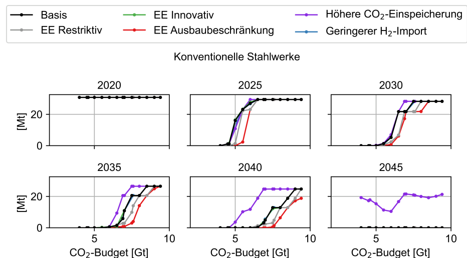
Abbildung C.143: Konventionelle Stahlproduktion der Szenarien in Abhängigkeit des CO 2 -Budgets
