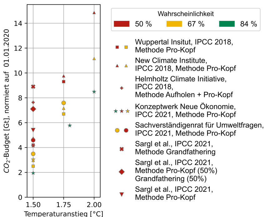
Abbildung 2.7: CO 2 -Budgets für Deutschland, normiert auf das Jahr 2020
