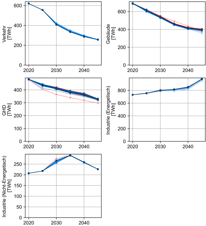
Abbildung C.3: Einfluss der Zeitreihenaggregation auf die Endenergie für die Szenarien mit Myopie
