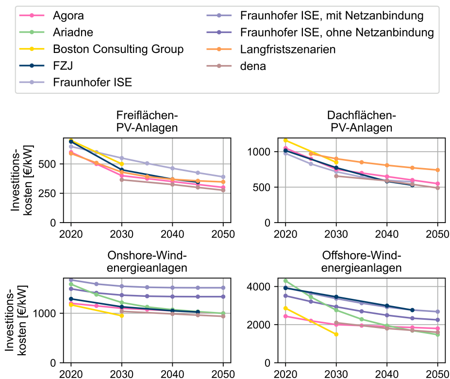
Abbildung 2.9: Spezifische Investitionskosten der erneuerbaren Energien in den Systemstudien zum Klimaschutzgesetz von 2021
