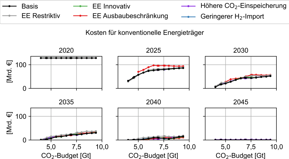
Abbildung C.67: Einfluss des CO 2 -Budgets auf die Kosten der fossilen Energieträger der Szenarien
