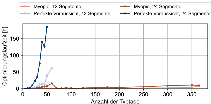
Abbildung 5.2: Einfluss der Zeitreihenaggregation auf die Optimierungslaufzeit der Szenarien mit perfekter Voraussicht und mit Myopie
