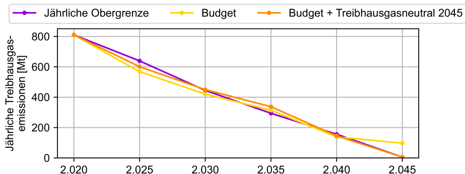
Abbildung 5.30: Einfluss der zeitlichen Emissionsbegrenzung auf die jährlichen Treibhausgasemissionen
