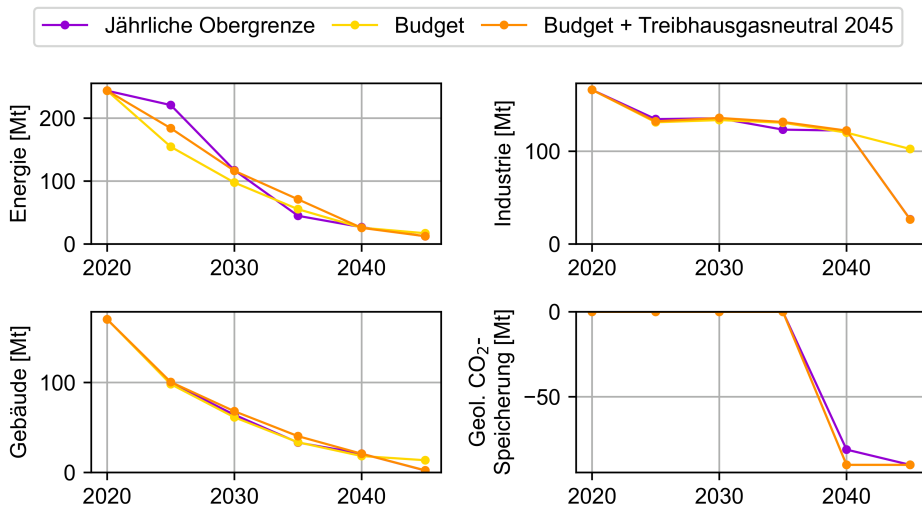
Abbildung 5.31: Einfluss der zeitlichen Emissionsbegrenzung auf die sektoralen Emissionen
