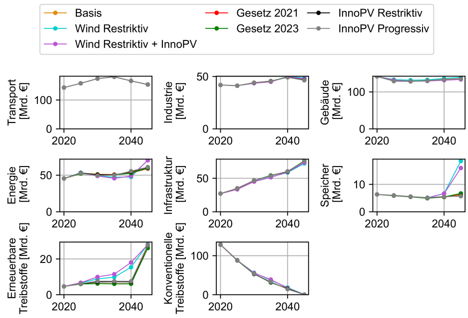
Abbildung C.34: Einfluss der Potenziale auf die Abweichung der Gesamtkosten
