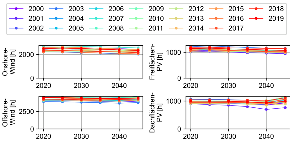
Abbildung C.20: Einfluss des historischen Wetterjahres zur Simulation der potenziellen Einspeisung der PV- und Windenergie-Technologien auf die Volllaststunden
