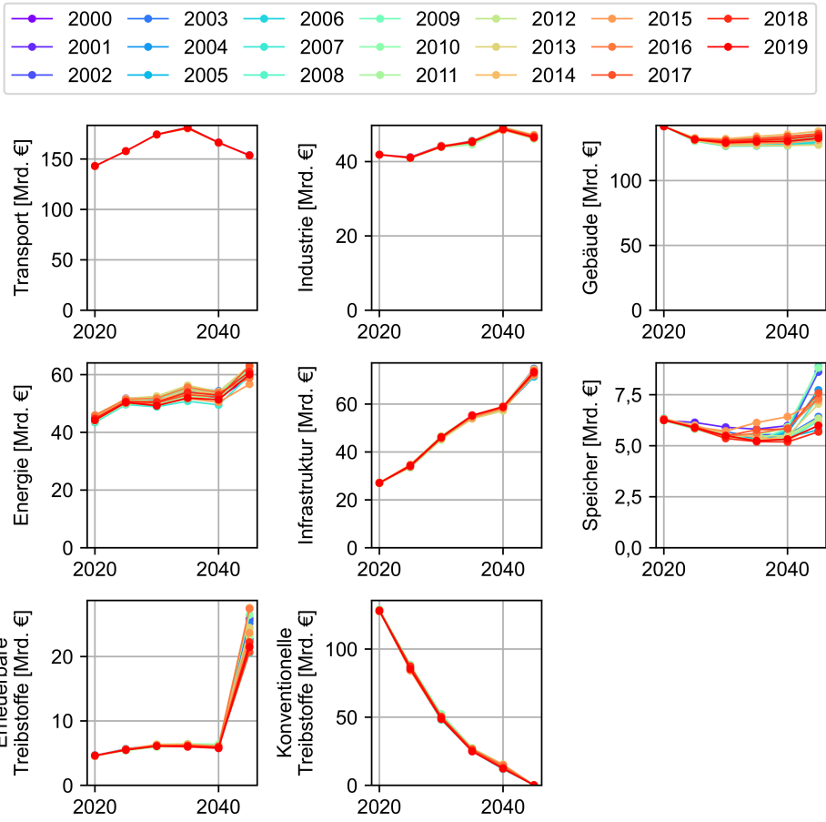
Abbildung C.28: Einfluss des historischen Wetterjahres zur Simulation der potenziellen Einspeisung der PV- und Windenergie-Technologien auf die sektoralen Kosten
