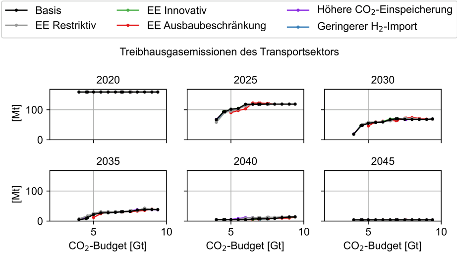
Abbildung C.77: Emissionen des Transportsektors der Szenarien in Abhängigkeit des CO 2 -Budgets
