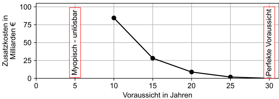
Abbildung 5.29: Mehrkosten der Transformationspfade mit sinkender Voraussicht im Vergleich zum Transformationspfad mit perfekter Voraussicht
