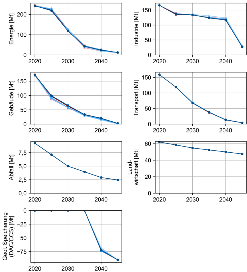
Abbildung C.11: Einfluss der Zeitreihenaggregation auf die Emissionen für die Szenarien mit perfekter Voraussicht
