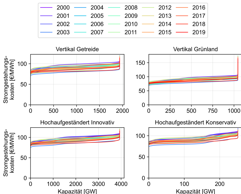
Abbildung 4.8: Stromgestehungskosten der Szenarien für Agri-PV-Anlagen für Investitionskosten von 1100 €/kW für hochaufgeständerte Anlagen und 800 €/kW für vertikale Anlagen, einem Zinssatz von 6 %, festen Betriebskosten von 1,1 % der Investitionskosten und einer Lebensdauer von 25 Jahren. Die vergleichbaren Stromgestehungskosten der vertikalen Agri-PV-Anlagen trotz geringerer Investitionskosten ergeben sich durch die geringeren Volllaststunden der vertikalen Agri-PV-Anlagen aufgrund der vertikalen Ausrichtung.
