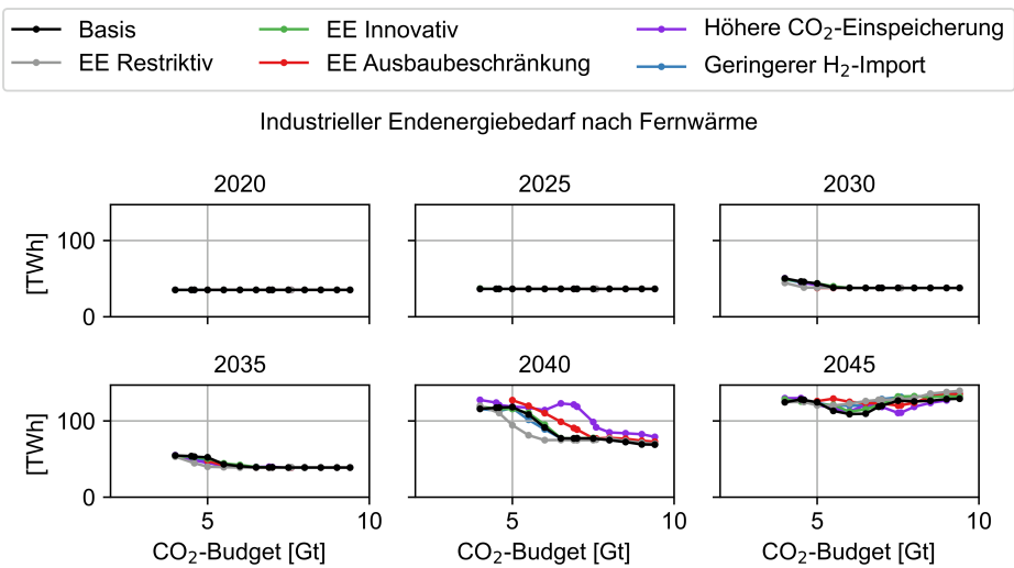
Abbildung C.154: Wärme-Endenergiebedarf der Industrie der Szenarien in Abhängigkeit des CO 2 -Budgets
