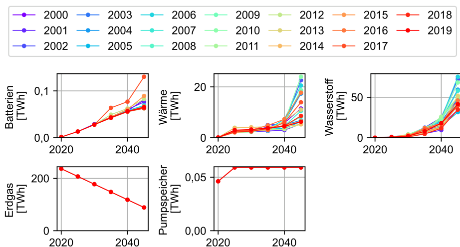
Abbildung 5.15: Einfluss des historischen Wetterjahres zur Simulation der potenziellen Einspeisung der PV- und Windenergieanlagen auf die Speicherkapazitäten
