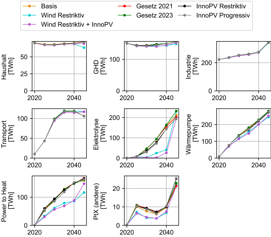
Abbildung C.30: Einfluss der Potenziale auf die Stromnachfrage
