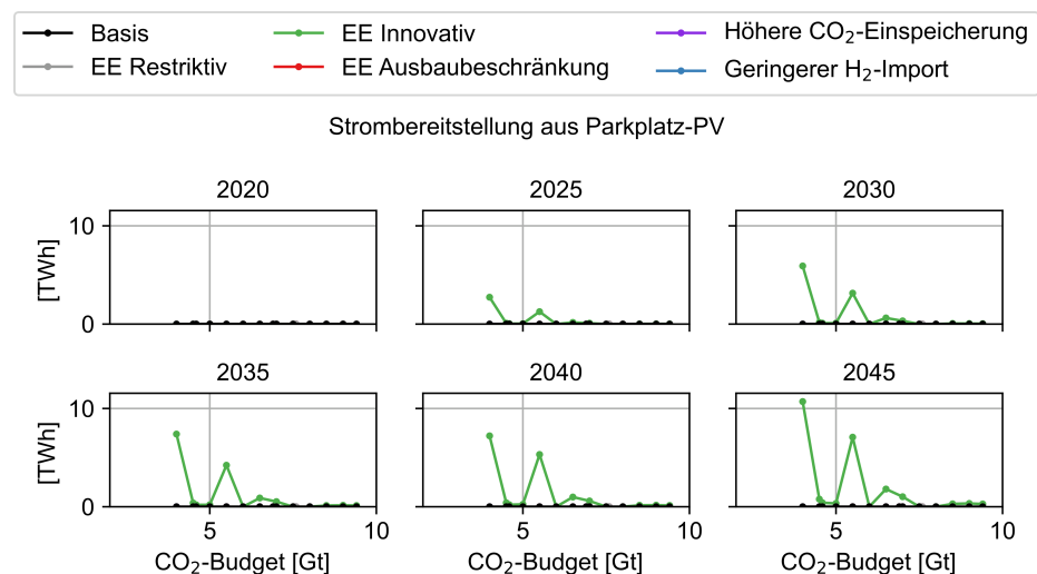
Abbildung C.91: Strombereitstellung durch Parkplatz-PV-Anlagen der Szenarien in Abhängigkeit des CO 2 -Budgets
