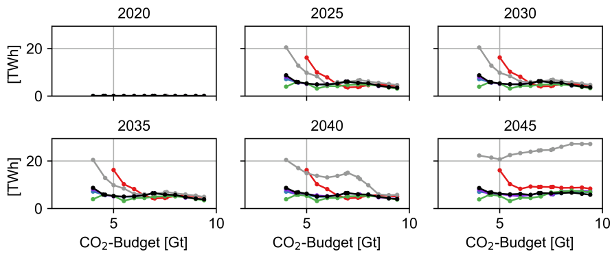
Abbildung C.165: Kapazitäten der Wärmespeicher der Szenarien in Abhängigkeit des CO 2 -Budgets
