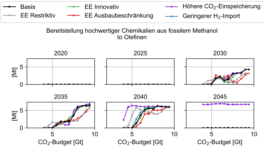
Abbildung C.146: Herstellung hochwertiger Chemikalien aus fossil-basierter Methanolgasifizierung zu Olefinen der Szenarien in Abhängigkeit des CO 2 -Budgets
