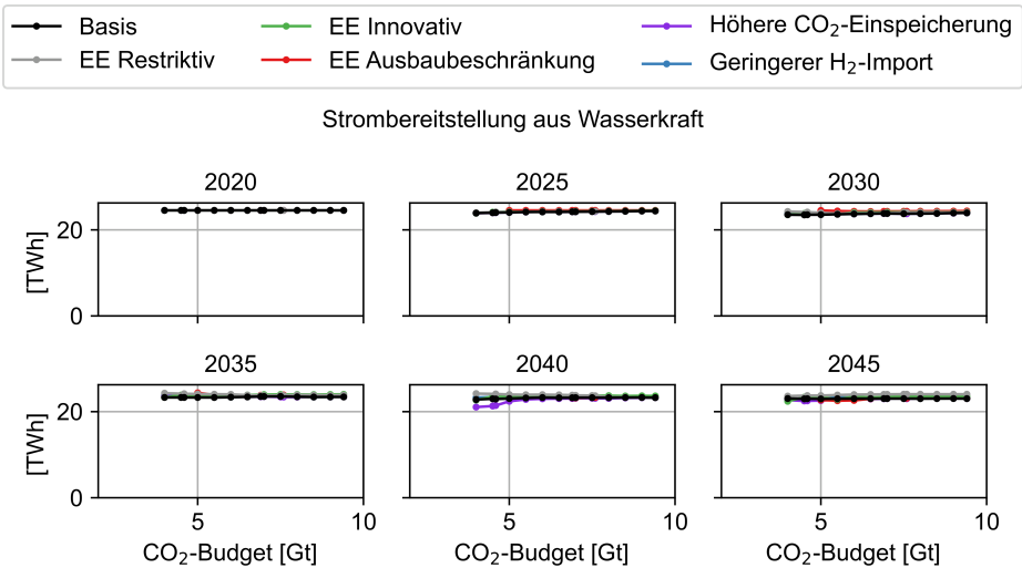
Abbildung C.82: Strombereitstellung durch Wasserkraft der Szenarien in Abhängigkeit des CO 2 -Budgets
