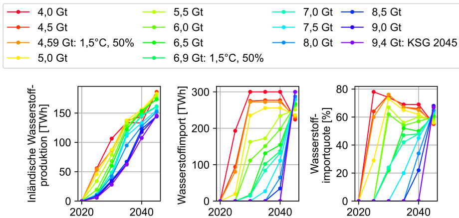
Abbildung 5.43: Einfluss des CO 2 -Budgets auf die Wasserstoff-Bereitstellung
