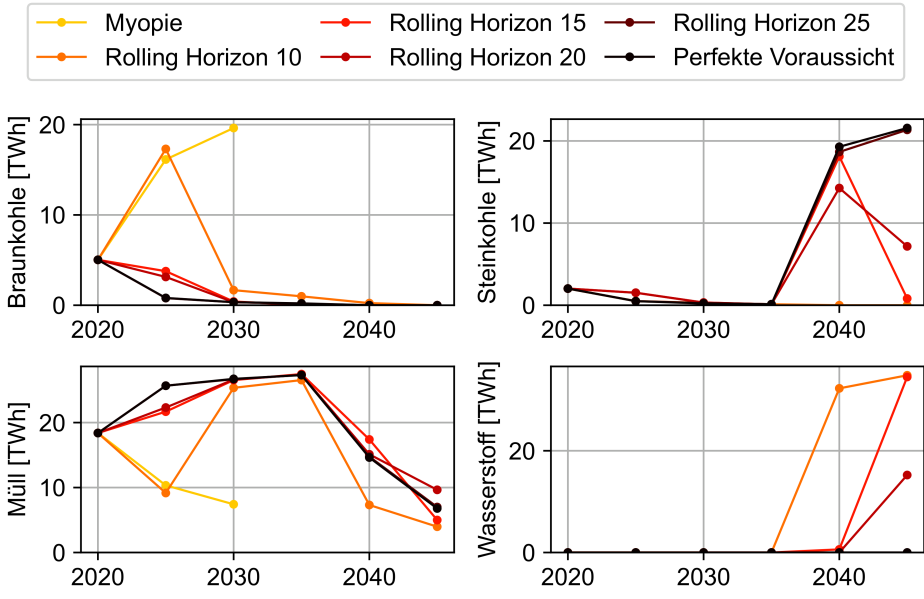
Abbildung C.42: Einfluss der Voraussicht auf den Energieträgereinsatz in der Zementproduktion
