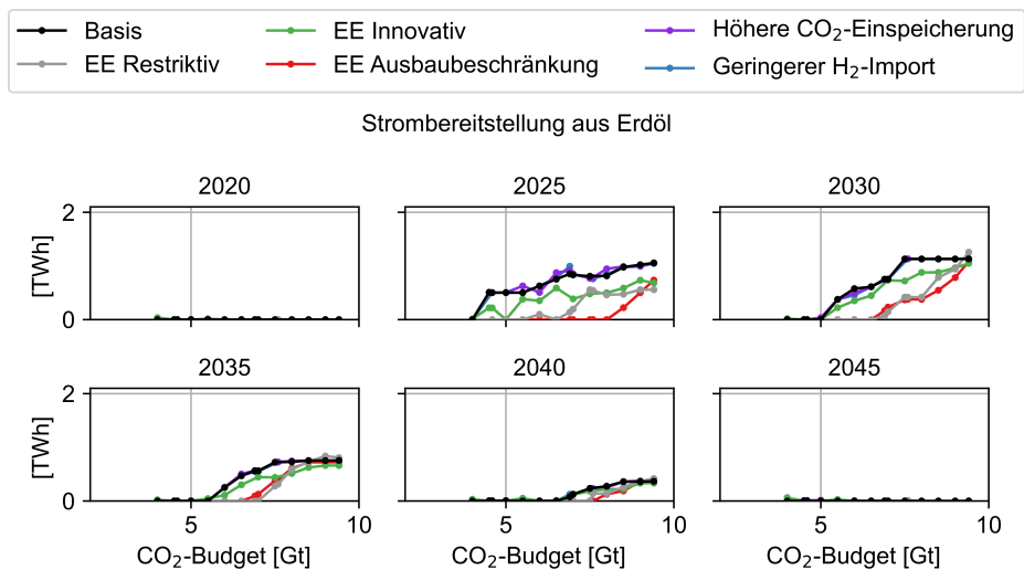
Abbildung C.84: Strombereitstellung durch Erdöl der Szenarien in Abhängigkeit des CO 2 -Budgets
