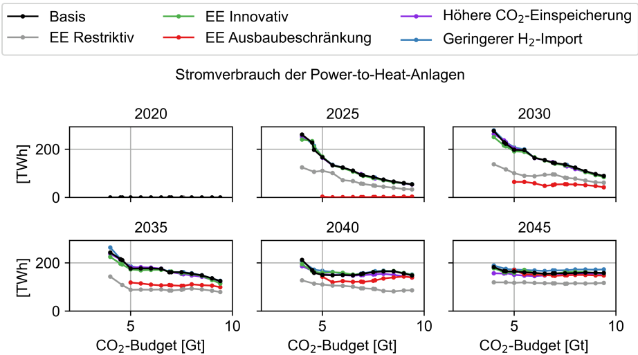
Abbildung C.98: Stromverbrauch der Power-to-Heat-Anlagen der Szenarien in Abhängigkeit des CO 2 -Budgets
