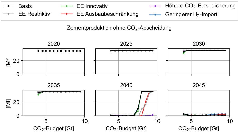
Abbildung C.130: Zementproduktion ohne CO 2 -Abscheidung der Szenarien in Abhängigkeit des CO 2 -Budgets
