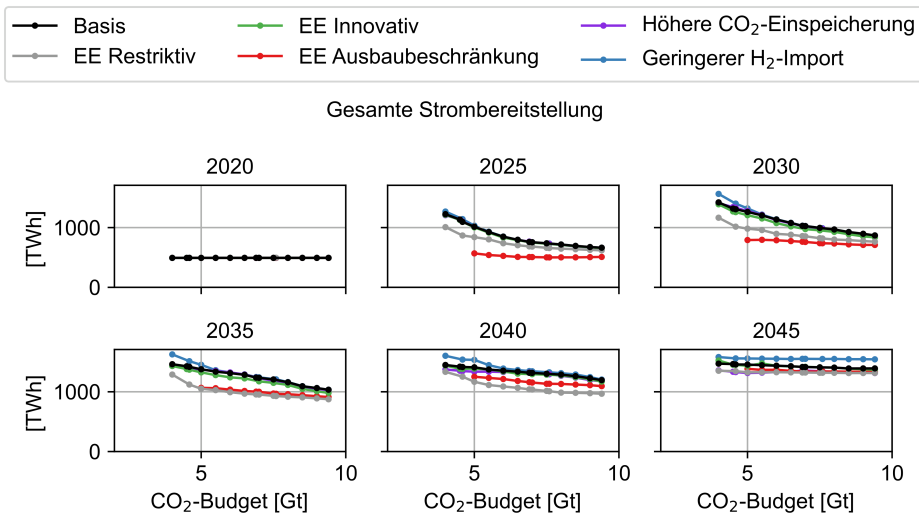
Abbildung 5.48: Strombereitstellung der Szenarien in Abhängigkeit des CO 2 -Budgets
