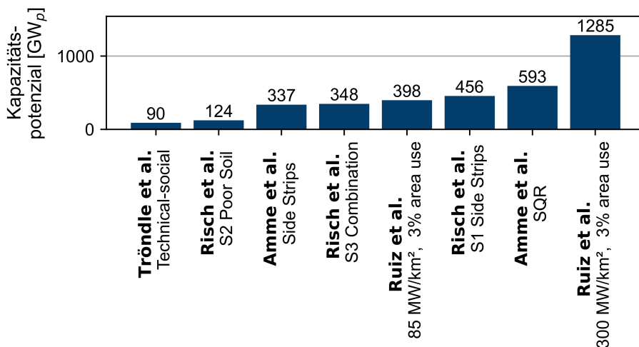
Abbildung 2.5: Kapazitätspotenziale verschiedener Studien für Freiflächen-PV-Anlagen in Deutschland, angelehnt an Risch und Maier et al. [32]
