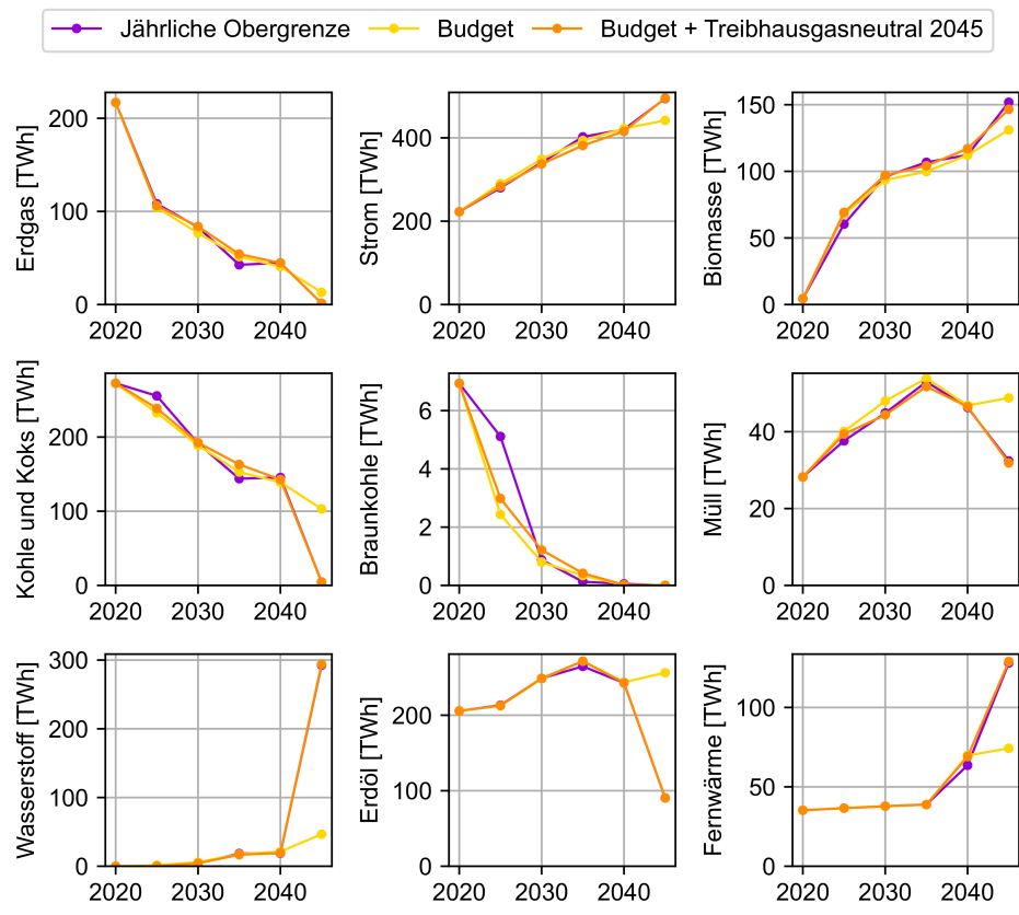
Abbildung C.48: Einfluss der zeitlichen Emissionsbegrenzung auf die Energieträger der Industrie
