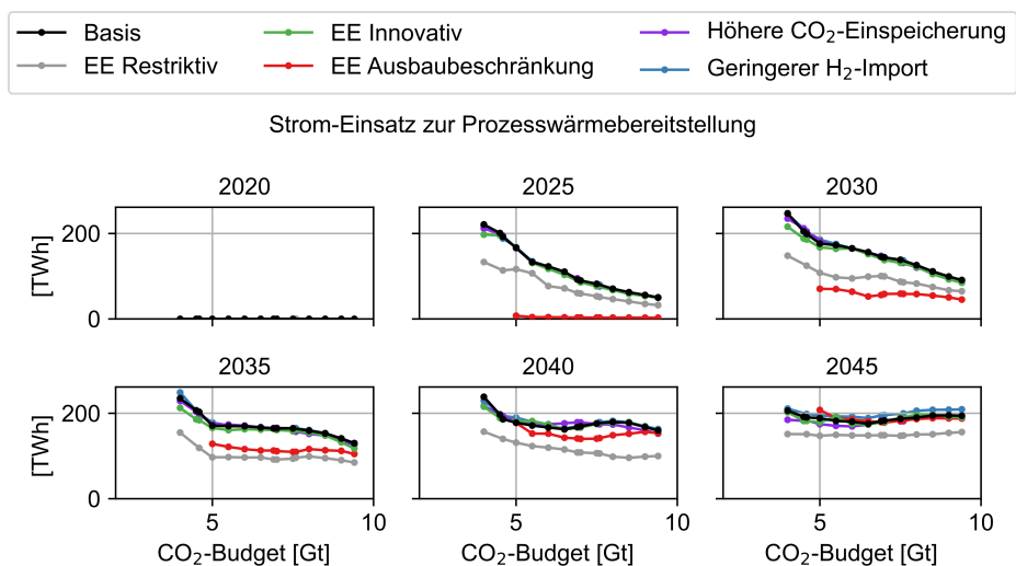
Abbildung C.111: Energieträgereinsatz von Strom für die Prozesswärmebereitstellung der Szenarien in Abhängigkeit des CO 2 -Budgets
