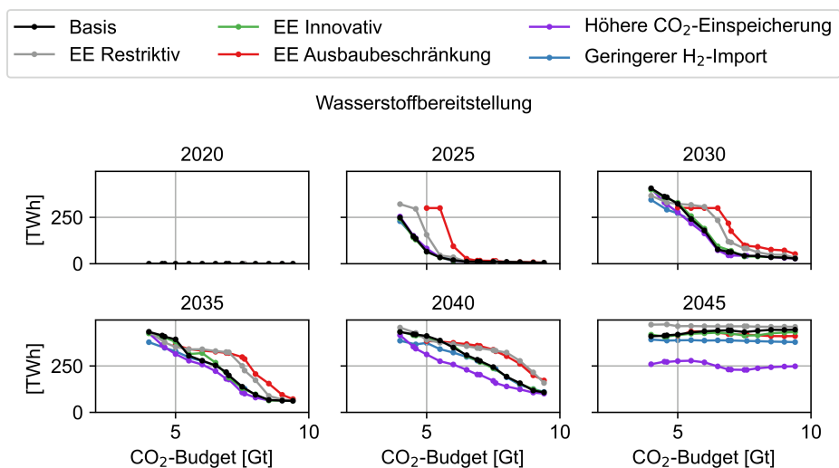
Abbildung C.119: Gesamte Wasserstoffbereitstellung der Szenarien in Abhängigkeit des CO 2 -Budgets
