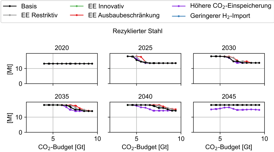
Abbildung C.141: Rezyklierter Stahl der Szenarien in Abhängigkeit des CO 2 -Budgets
