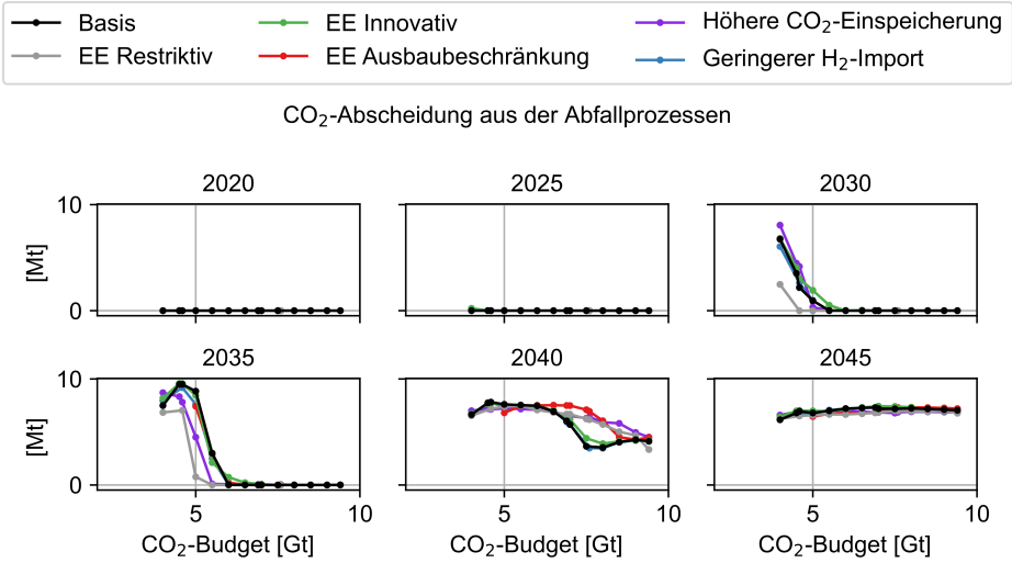
Abbildung C.129: CO 2 -Abscheidung durch Abfallanlagen der Szenarien in Abhängigkeit des CO 2 -Budgets
