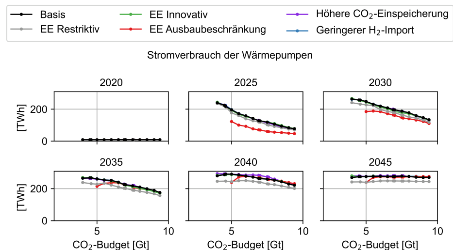
Abbildung C.96: Stromverbrauch der Wärmepumpen der Szenarien in Abhängigkeit des CO 2 -Budgets
