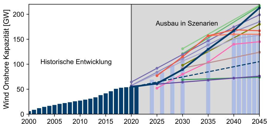
Abbildung 2.10: Historische installierte Kapazität von Onshore-Windenergieanlagen in Deutschland, Ausbauziele des Osterpakets und Ausbaupfade der Systemstudien zur Treibhausgasneutralität in 2045
