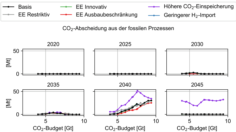
Abbildung C.126: CO 2 -Abscheidung durch fossil betriebene Anlagen der Szenarien in Abhängigkeit des CO 2 -Budgets
