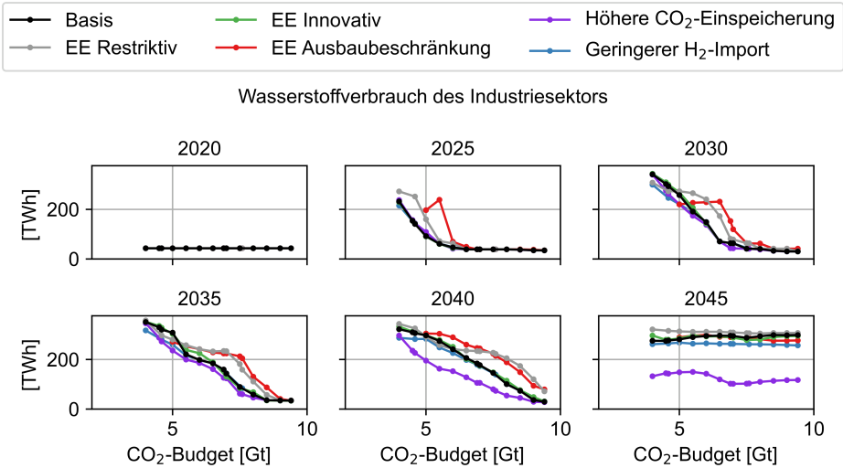
Abbildung C.121: Wasserstoffbedarf der Industrie der Szenarien in Abhängigkeit des CO 2 -Budgets
