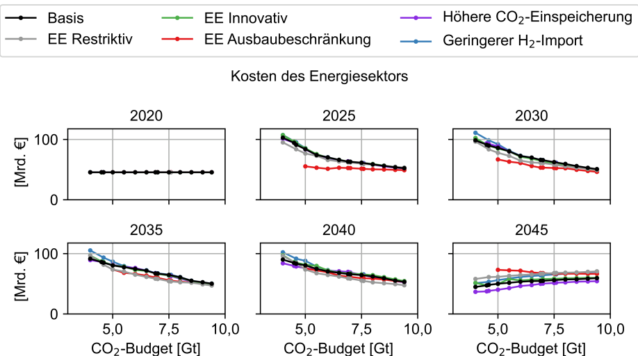
Abbildung C.68: Einfluss des CO 2 -Budgets auf die Kosten des Energiesektors der Szenarien
