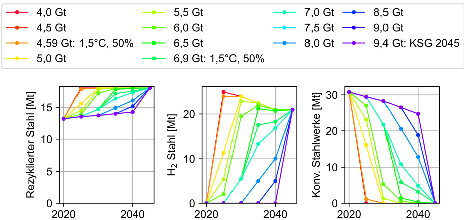
Abbildung C.60: Einfluss des CO 2 -Budgets auf die Stahlproduktion des Basis-Szenarios
