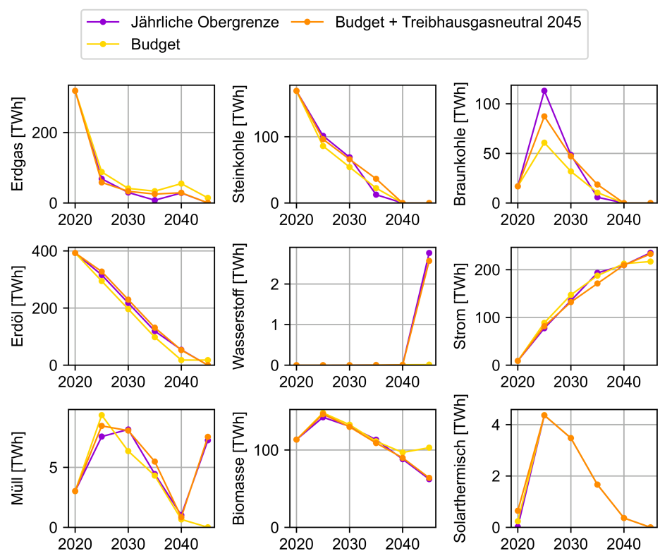
Abbildung C.47: Einfluss der zeitlichen Emissionsbegrenzung auf die Energieträger der Raumwärmeversorgung
