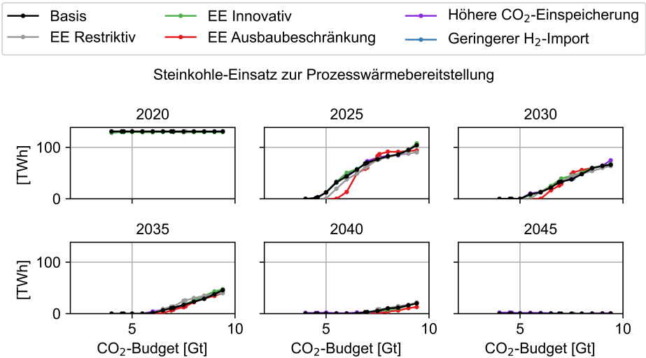
Abbildung C.114: Energieträgereinsatz von Steinkohle für die Prozesswärmebereitstellung der Szenarien in Abhängigkeit des CO 2 -Budgets
