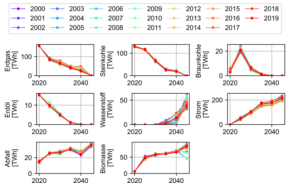
Abbildung C.24: Einfluss des historischen Wetterjahres zur Simulation der potenziellen Einspeisung der PV- und Windenergie-Technologien auf den Energieträgereinsatz für die Prozesswärmebereitstellung
