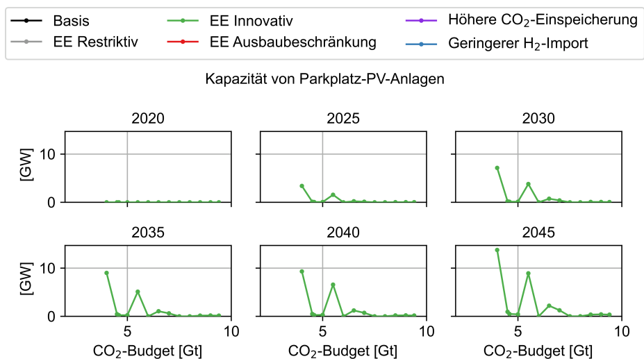
Abbildung C.107: Installierte Leistung der Parkplatz-PV-Anlagen der Szenarien in Abhängigkeit des CO 2 -Budgets
