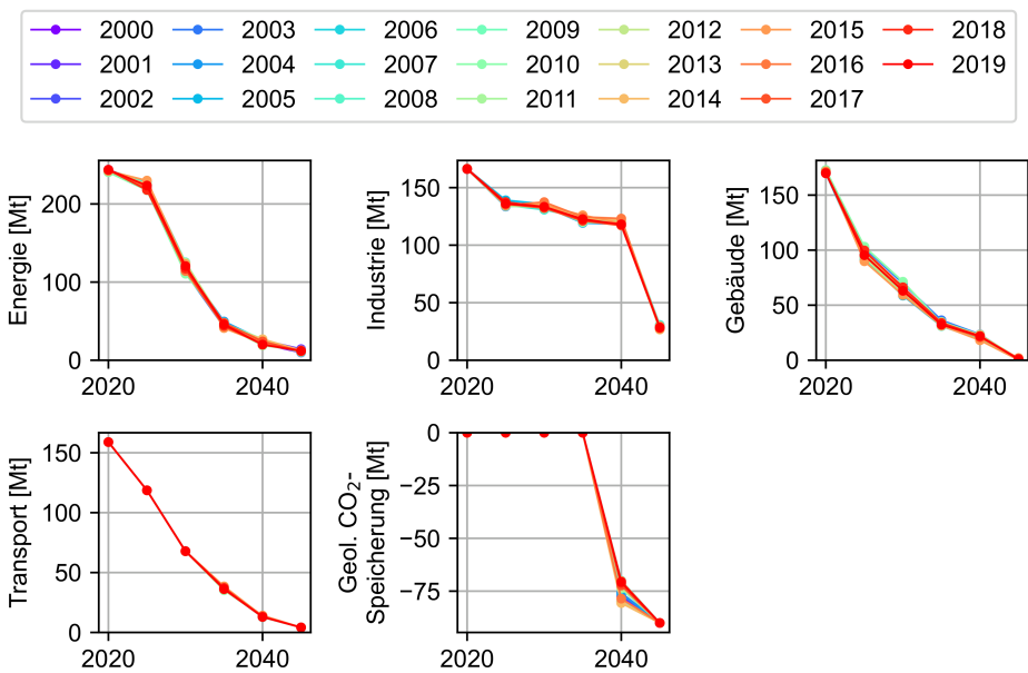
Abbildung C.19: Einfluss des historischen Wetterjahres zur Simulation der potenziellen Einspeisung der PV- und Windenergie-Technologien auf die sektoralen Emissionen
