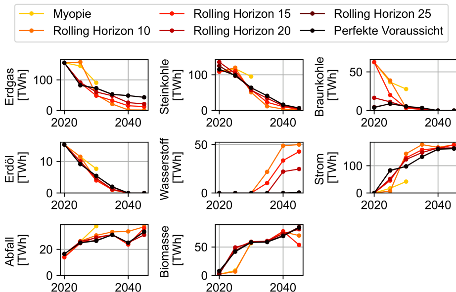
Abbildung 5.24: Einfluss der Voraussicht auf die Prozesswärmebereitstellung
