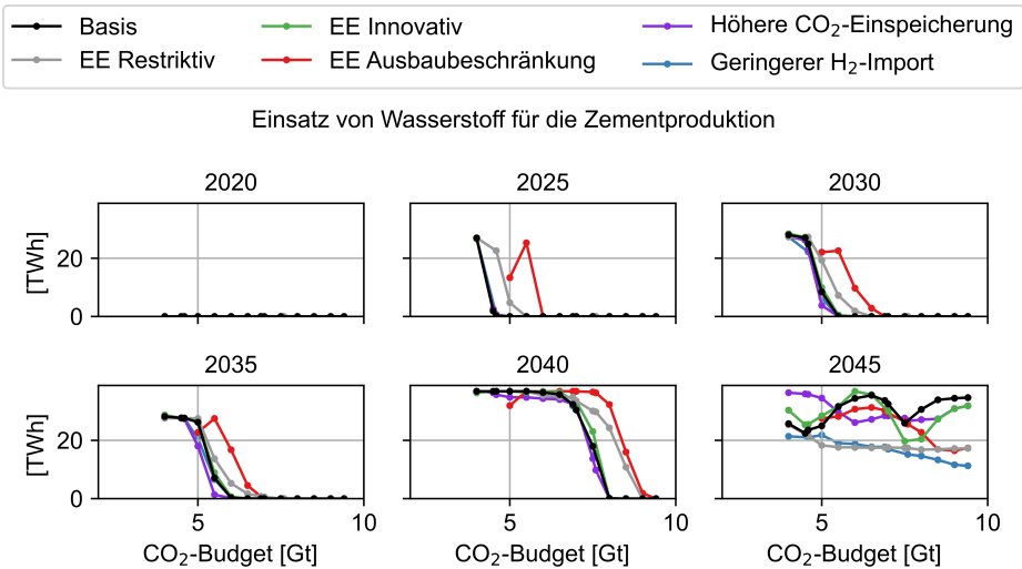
Abbildung C.134: Einsatz von Wasserstoff in der Zementproduktion der Szenarien in Abhängigkeit des CO 2 -Budgets
