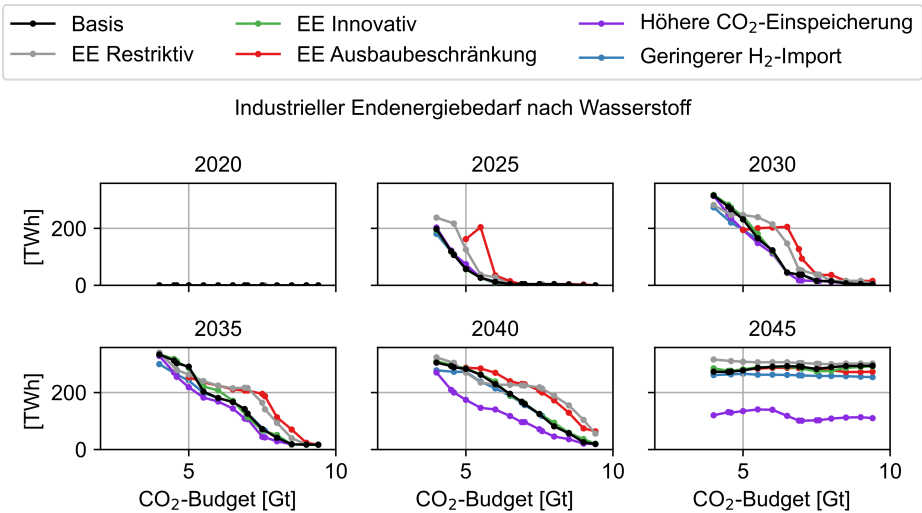
Abbildung C.150: Wasserstoff-Endenergiebedarf der Industrie der Szenarien in Abhängigkeit des CO 2 -Budgets
