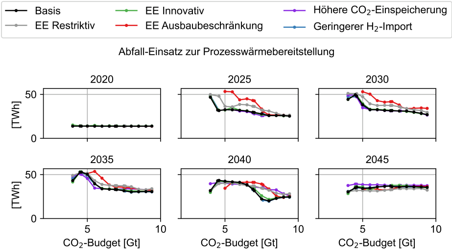
Abbildung C.117: Energieträgereinsatz von Abfall für die Prozesswärmebereitstellung der Szenarien in Abhängigkeit des CO 2 -Budgets
