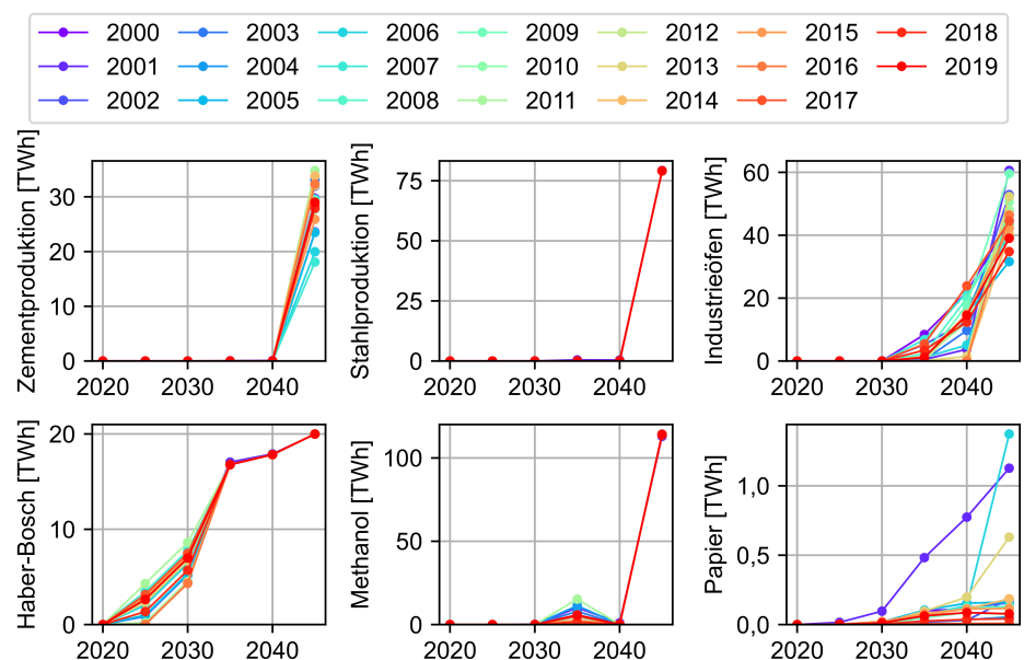
Abbildung C.26: Einfluss des historischen Wetterjahres zur Simulation der potenziellen Einspeisung der PV- und Windenergie-Technologien auf die Wasserstoffnachfrage des Industriesektors
