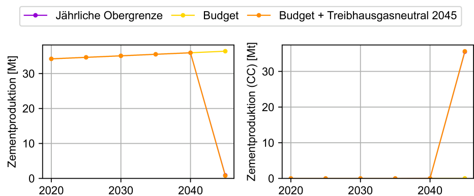
Abbildung C.52: Einfluss der zeitlichen Emissionsbegrenzung auf die Zementproduktion
