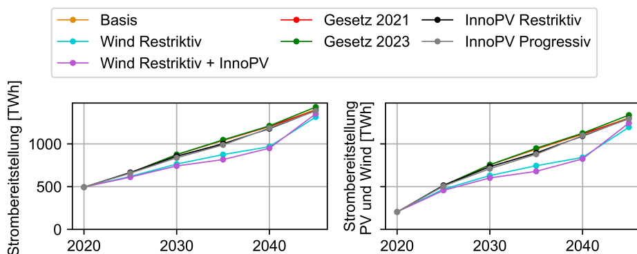
Abbildung 5.4: Einfluss der Potenziale auf die Strombereitstellung aus PV- und Windenergieanlagen und auf die gesamte Strombereitstellung
