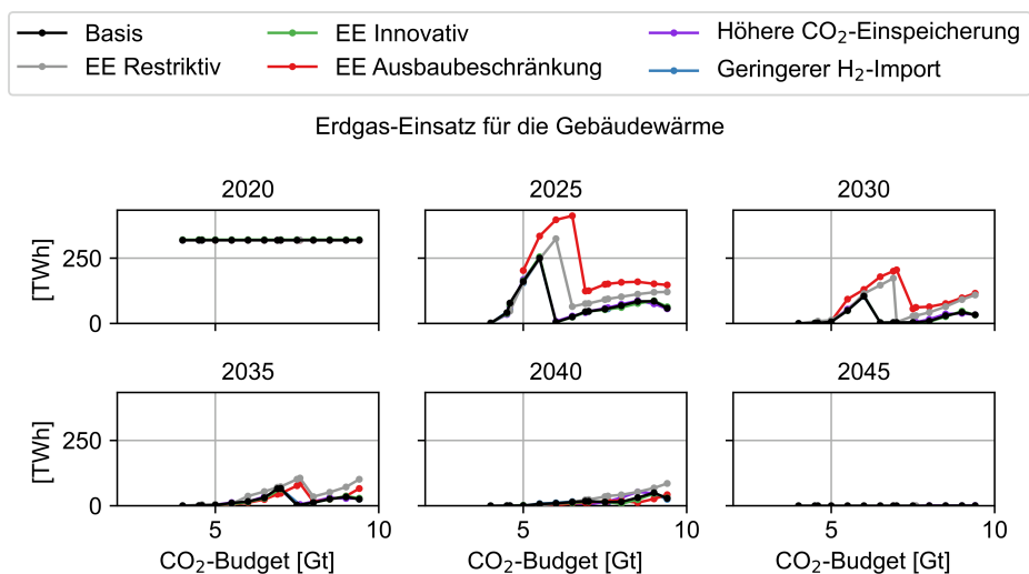
Abbildung C.159: Einsatz von Erdgas für die Gebäudewärme der Szenarien in Abhängigkeit des CO 2 -Budgets
