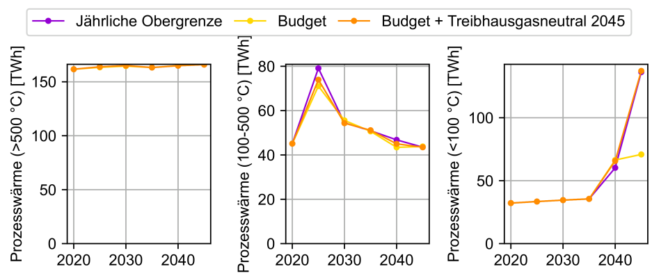
Abbildung C.51: Einfluss der zeitlichen Emissionsbegrenzung auf die Prozesswärmenachfrage
