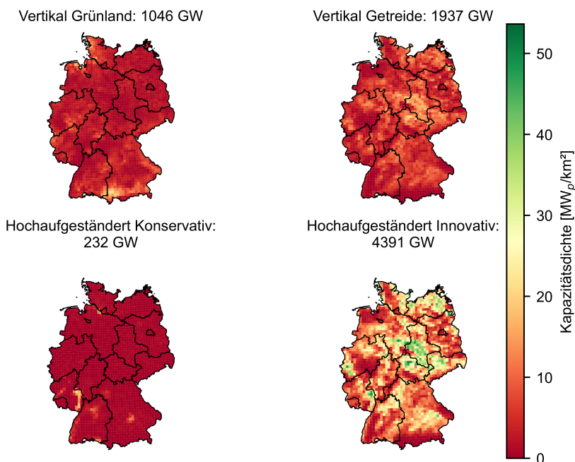
Abbildung 4.7: Kapazitätsdichte der Potenzialszenarien für Agri-PV-Anlagen
