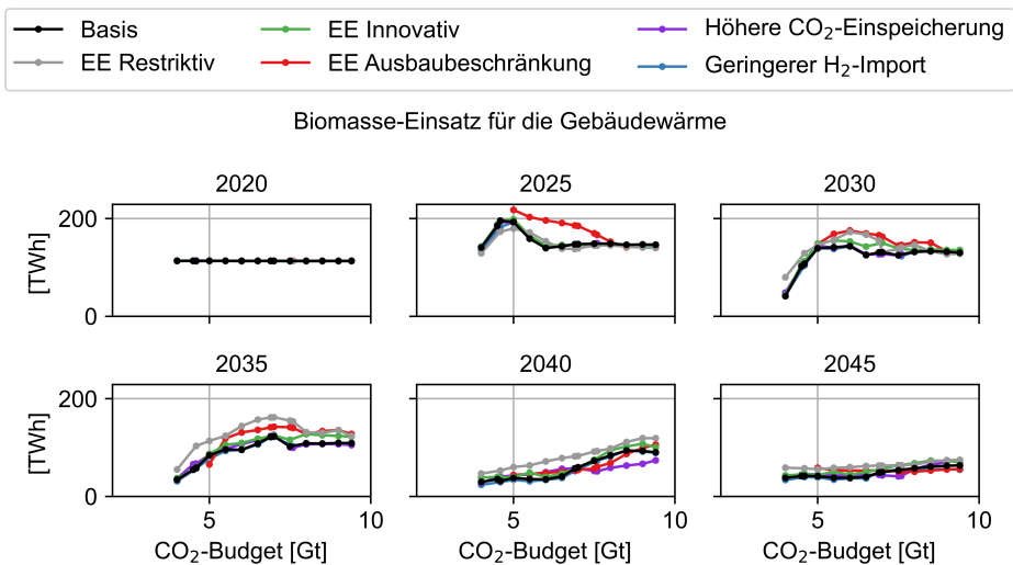
Abbildung C.164: Einsatz von Biomasse für die Gebäudewärme der Szenarien in Abhängigkeit des CO 2 -Budgets
