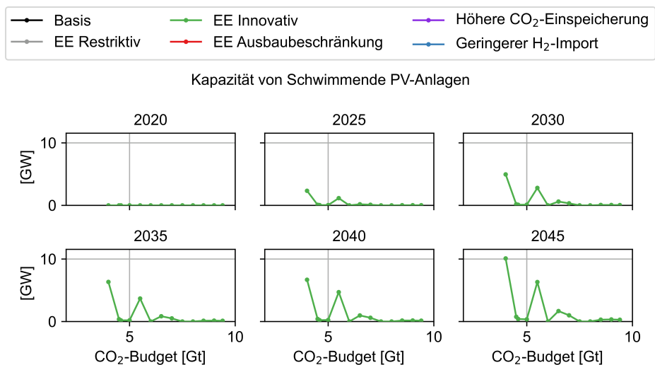
Abbildung C.108: Installierte Leistung der schwimmenden PV-Anlagen der Szenarien in Abhängigkeit des CO 2 -Budgets
