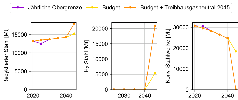
Abbildung C.54: Einfluss der zeitlichen Emissionsbegrenzung auf die Stahlproduktion
