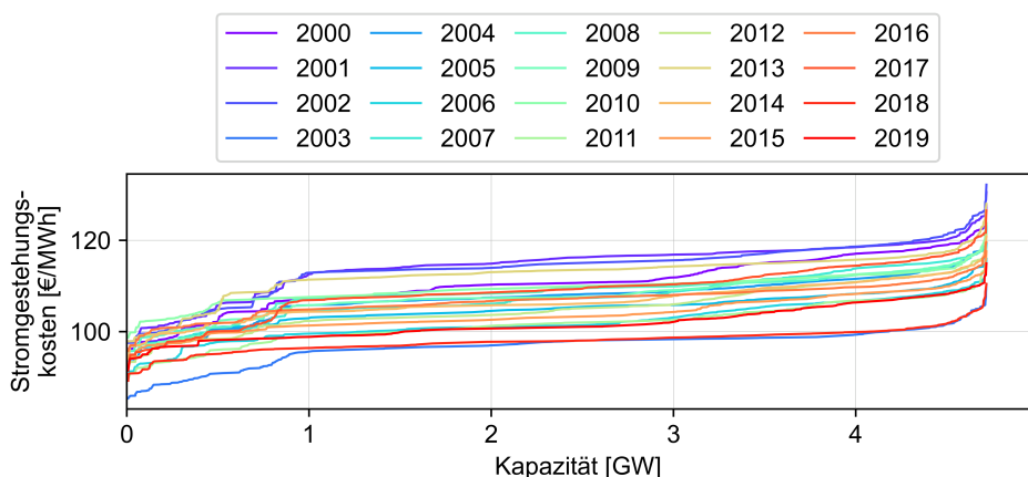
Abbildung 4.14: Stromgestehungskosten des Potenzialszenarios der aktuellen gesetzlichen Vorgaben für schwimmende PV-Anlagen für Investitionskosten von 1000 €/kW, einem Zinssatz von 6 %, festen Betriebskosten von 2,5 % der Investitionskosten und einer Lebensdauer von 25 Jahren
