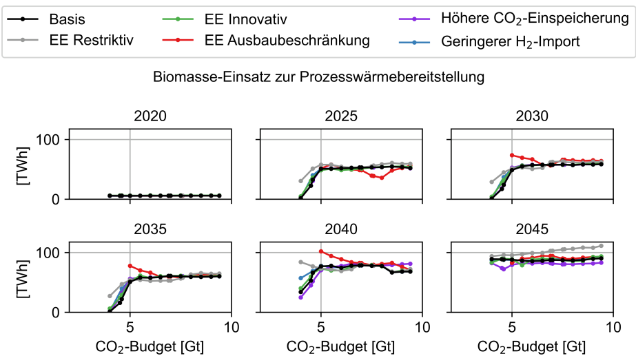
Abbildung C.110: Energieträgereinsatz von Biomasse für die Prozesswärmebereitstellung der Szenarien in Abhängigkeit des CO 2 -Budgets
