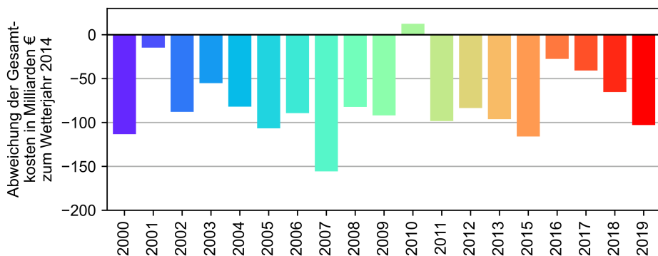
Abbildung 5.16: Abweichung der Gesamtkosten des Transformationspfades durch das historische Wetterjahr zur Simulation der potenziellen Einspeisung der PV- und Windenergieanlagen im Vergleich zum Basis-Szenario mit dem Wetterjahr 2014
