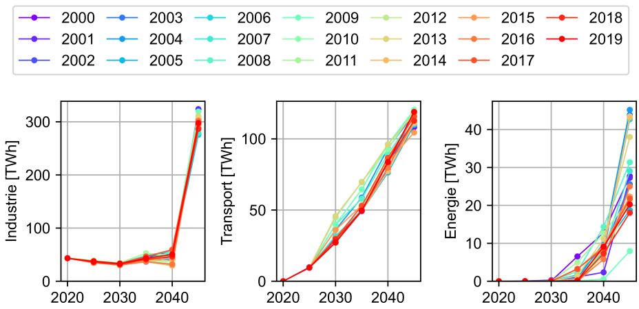
Abbildung C.25: Einfluss des historischen Wetterjahres zur Simulation der potenziellen Einspeisung der PV- und Windenergie-Technologien auf die sektorale Wasserstoffnachfrage
