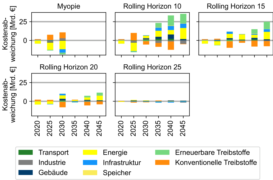
Abbildung 5.28: Abweichung der jährlichen Kosten zum Szenario mit perfekter Voraussicht
