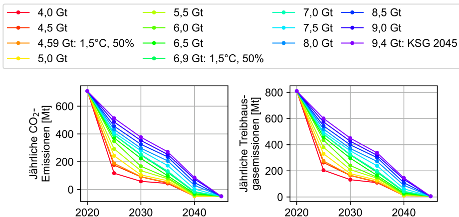
Abbildung 5.35: Einfluss des CO 2 -Budgets auf jährlichen CO 2 - und Treibhausgas-Emissionen
