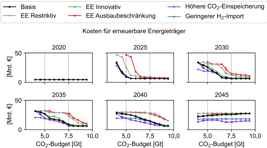
Abbildung C.70: Einfluss des CO 2 -Budgets auf die Kosten der erneuerbaren Treibstoffe der Szenarien
