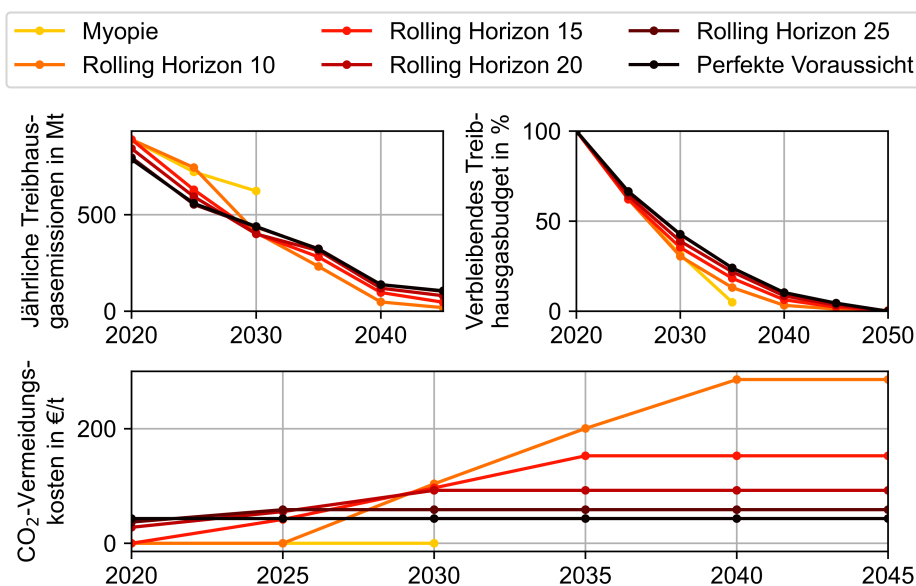
Abbildung 5.17: Einfluss der Voraussicht auf die jährlichen Treibhausgasemissionen und das verbleibende Treibhausgas-Budget sowie die CO 2 -Vermeidungskosten
