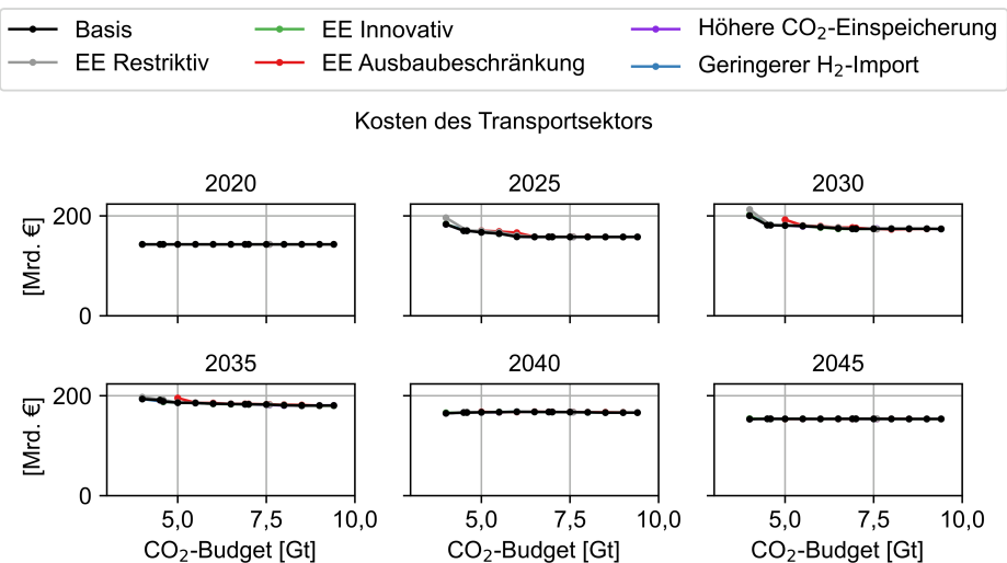
Abbildung C.72: Einfluss des CO 2 -Budgets auf die Kosten des Transportsektors der Szenarien
