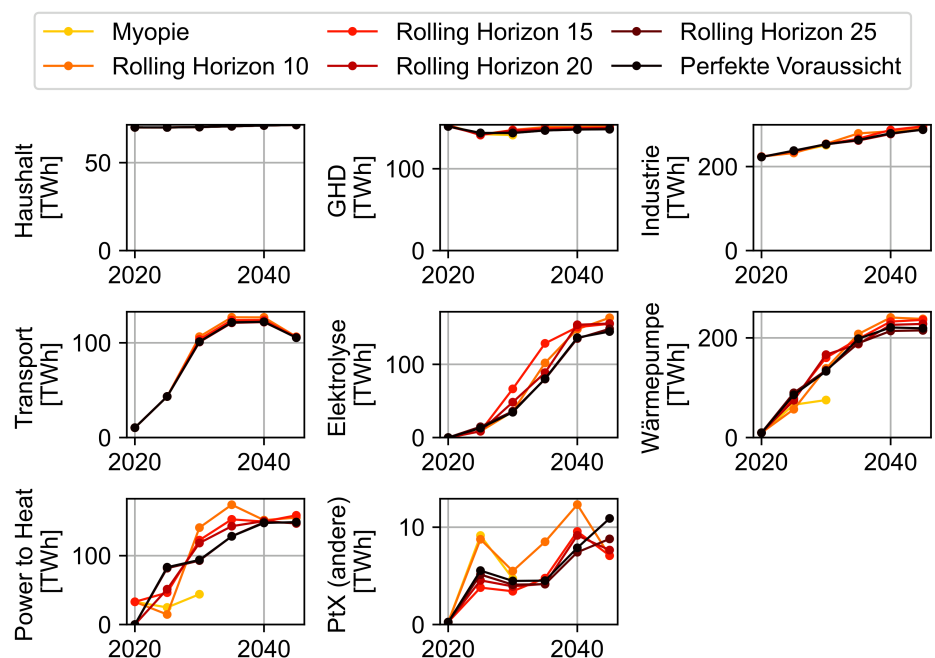
Abbildung C.39: Einfluss der Voraussicht auf die Stromnachfrage
