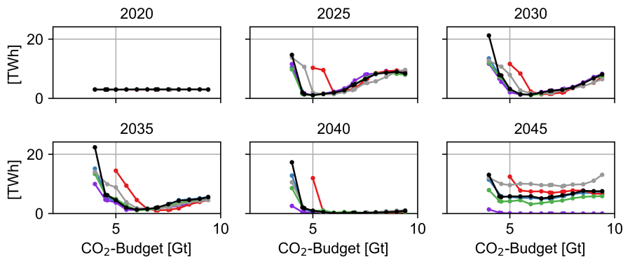
Abbildung C.157: Einsatz von Abfall für die Gebäudewärme der Szenarien in Abhängigkeit des CO 2 -Budgets
