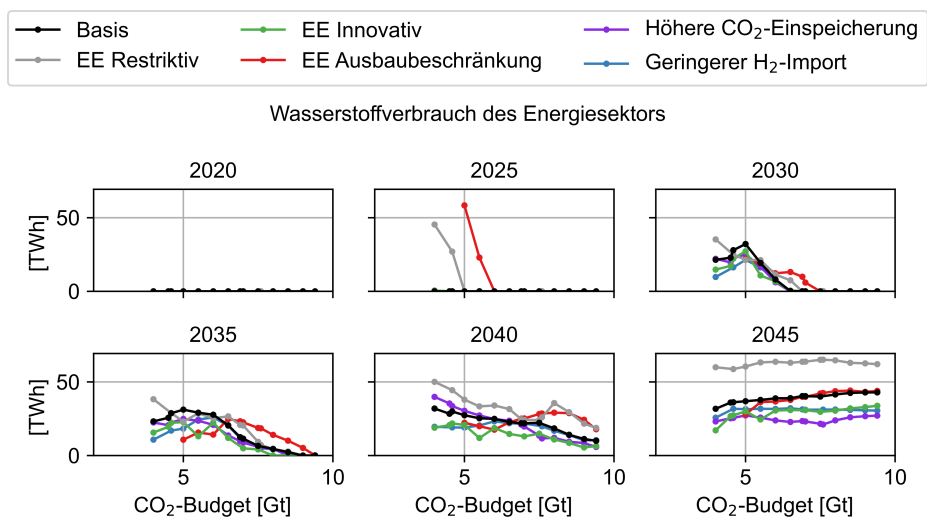
Abbildung C.123: Wasserstoffbedarf des Energiesektors der Szenarien in Abhängigkeit des CO 2 -Budgets
