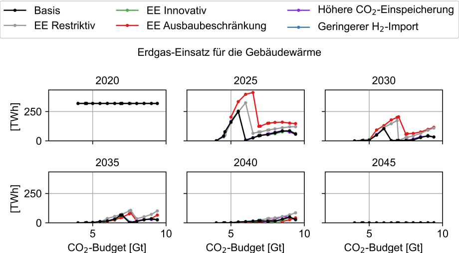
Abbildung 5.50: Einsatz von Erdgas für die Gebäudewärme der Szenarien in Abhängigkeit des CO 2 -Budgets
