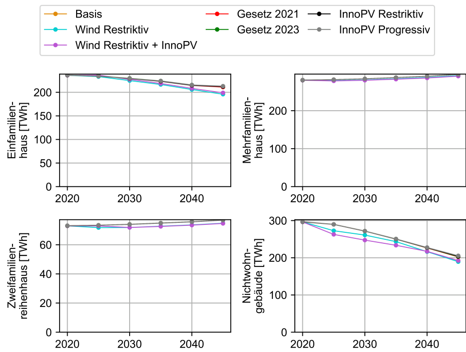
Abbildung C.32: Einfluss der Potenziale auf den Wärmebedarf der Gebäude
