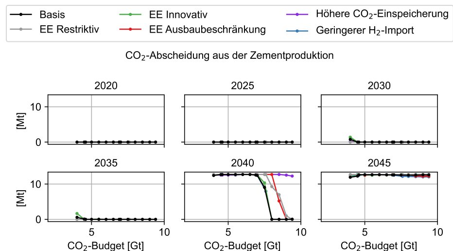
Abbildung C.127: CO 2 -Abscheidung durch Zementprozesse der Szenarien in Abhängigkeit des CO 2 -Budgets
