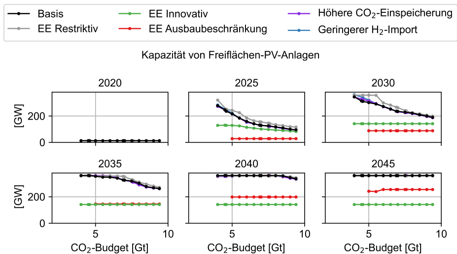
Abbildung C.104: Installierte Leistung der Freiflächen-PV-Anlagen der Szenarien in Abhängigkeit des CO 2 -Budgets
