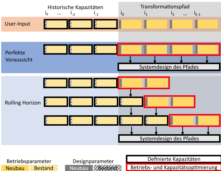
Abbildung 3.3: Modelltechnische Implementierung von Transformationspfaden mit historischen Kapazitäten in ETHOS.FINE beispielhaft für einen Pfad mit perfekter Voraussicht und einen Pfad mit Rolling Horizon mit einer Voraussicht von zwei Investitionsperioden. Der Transformationspfad ergibt sich für die Methodik der perfekten Voraussicht aus einer einzelnen Optimierung, während dieser für Rolling Horizon im vorliegenden Beispiel sich aus drei Optimierungen ergibt.
