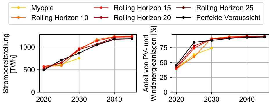
Abbildung 5.20: Einfluss der Voraussicht auf die Gesamtstrombereitstellung und auf den Anteil der Strombereitstellung durch PV- und Windenergieanlagen
