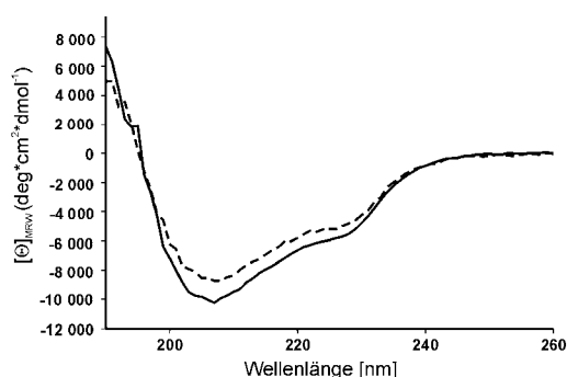
Abbildung 4.18: Untersuchung der CRT-Faltung und -Stabilität über die Zeit mittels Fern-UV-CD. 4 \mu M (0,19 mg/ml) CRT in 50 mM NaPhosphat pH 8,0, wurde in einer Quarzküvette mit 0,5 mm Schichtdicke gemessen. Die durchgezogene Linie zeigt das Spektrum von frisch gereinigtem CRT, während die gestrichelte Linie das Spektrum der identischen Probe nach einer Woche darstellt. Bei beiden Spektren ist das entsprechende Pufferspektrum schon abgezogen.
