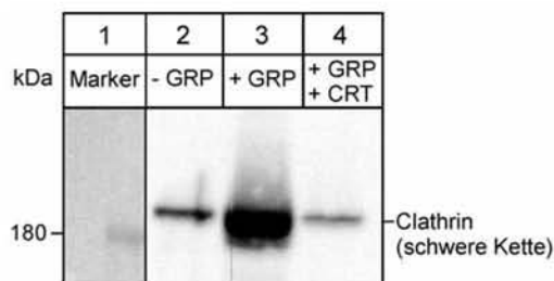
Abbildung 4.33: Endogenes Protein CHC bindet an immobilisiertes, rekombinantes GABARAP. Ungekoppelte Sepharose (Spur 2) und Sepharose-gekoppeltes GABARAP in Abwesenheit (Spur 3) und Anwesenheit (Spur 4) von 70 \mu M CRT wurden mit Rattenhirnextrakten inkubiert. Nach mehreren Waschschritten wurden gebundene Proteine eluiert und per SDS-PAGE aufgetrennt. Die Detektion von ggf. vorhandenem CRT erfolgte durch Western Blot Analyse. Spur 1 zeigt Signale des Prestained Protein Marker, Broad Range, NEB, Beverly, MA, USA).
