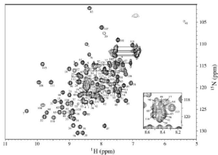
Abbildung aus (Kouno et al. 2004): (^1\text{H}-^{15}\text{N}) -HSQC Spektrum von MAP-LC3. Die Assignments sind dem jeweiligen Resonanzsignal zugeordnet. Manche Signale sind durch horizontale Linien miteinander verbunden und korrespondieren zu den Amidgruppen der Asn und Gln Seitenketten. Die mit einem Stern gekennzeichneten Resonanzsignale sind dem aminoterminalen Tag von MAP-LC3 zuzuordnen.
