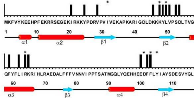
Abbildung 4.35: Lokalisierung der CHC (510-522) Bindestelle von GABARAP. Unter der Darstellung der GABARAP-Sequenztopologie (Aminosäuren sind im Einbuchstaben-Aminosäure-Code angegeben, Anhang S. 156) sind die entsprechenden Sekundärstrukturelemente dargestellt. Von der Bindung von CHC (510-522) am stärksten beeinflusste Aminosäuren sind auf der Y-Achse mit einem Balken gekennzeichnet. Die mit einem Stern (*) markierten Reste kennzeichnen die Aminosäuren, die in dem GABARAP-orthologen Hefeprotein Atg8 als wichtig für die Autophagozytose identifiziert wurden und sind in GABARAP konserviert (Nakatogawa et al. 2007).
