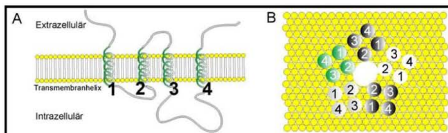
Abbildung 1.1: Schematische Darstellung der Membrantopologie der GABA A -Rezeptor-Untereinheiten und deren Assemblierung im Rezeptor. A: Alle Untereinheiten des GABA A -Rezeptors weisen eine gemeinsame Membrantopologie auf, wobei ein extrazellulärer amino- und carboxyterminaler Teil, vier Transmembranhelices (TM1-4) und zwei zytoplasmatische Loops (TM1/2 Loop und TM3/4 Loop ) vorhanden sind. B: Im Rezeptor lagern sich die Transmembransegmente 2 (TM2) der einzelnen Untereinheiten so zusammen, dass sie die Wand des Ionenkanals bilden.
