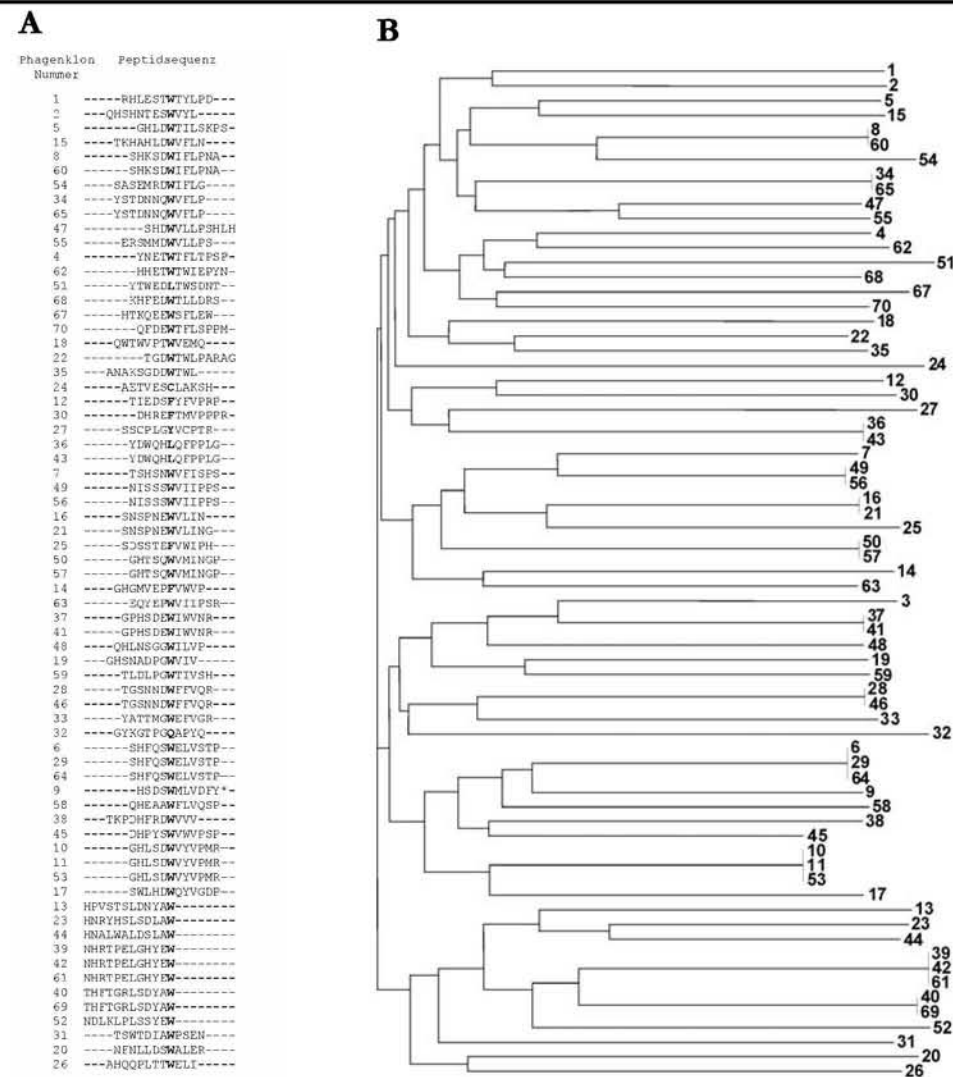
Abbildung 4.5: Analyse der Phagen Display selektierten Peptidsequenzen 1 bis 70 A: Sequenzalignment der Peptidsequenzen, erstellt mit ClustalW. Dick gedruckt ist die Aminosäureposition hervorgehoben, die in den meisten Peptiden ein Tryptophan aufweist. B: Phylogramm der selektierten Peptide, erstellt mit Hilfe von ClustalW. Die Zweiglänge zwischen den Knotenpunkten ist proportional zum Maß der Aminosäure-Unterschiede.
