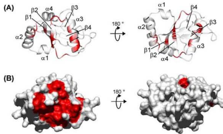
Abbildung 4.10: Visualisierung der N1-Peptid Bindestelle an GABARAP. A: Ribbondarstellung von GABARAP (PDB Code 1kot). Aminosäurereste, deren Resonanzen im HSQC-Experiment von der Bindung des N1-Peptids am stärksten betroffen waren, sind rot eingefärbt. Sekundärstrukturelemente sind mit \alpha ( \alpha -Helix) und \beta ( \beta -Strang) und der entsprechenden Nummerierung gekennzeichnet. B: Oberflächendarstellung von A. Ribbon- und Oberflächendarstellung wurden mit Hilfe der Software „MOlecul analysis and MOlecul display“ (MOLMOI) erstellt.
