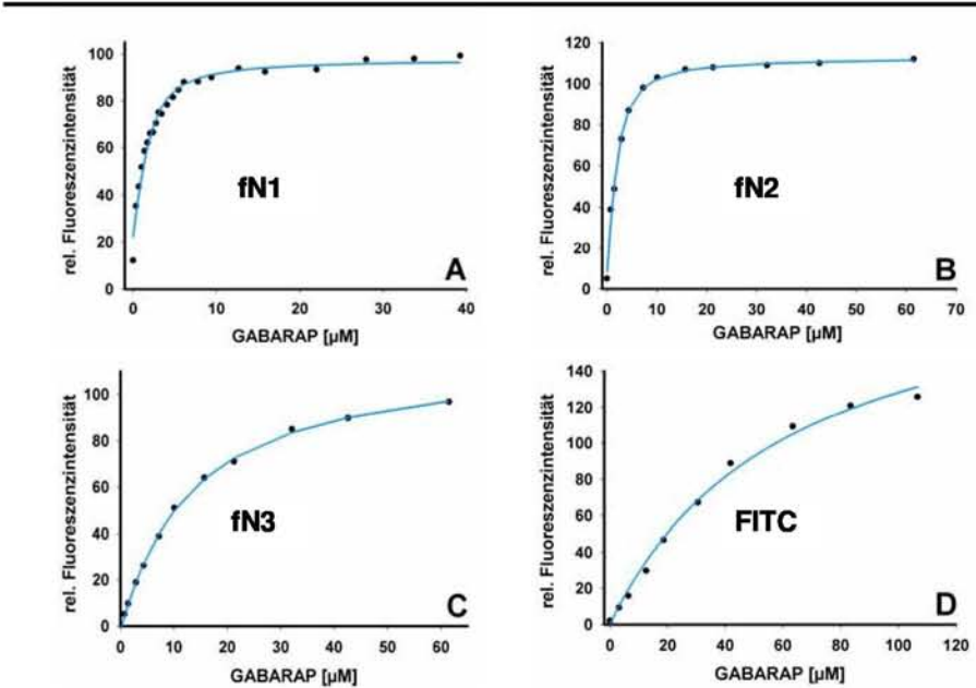
Abbildung 4.6: Fluoreszenztitration von GABARAP zu fN1 (A), fN2 (B), fN3 (C) und FITC (D). Es wurde 2 \mu\text{M} des jeweiligen Peptids bzw. FITC in einem Volumen von 1 ml vorgelegt und GABARAP in aufsteigenden Konzentrationen dazu titriert. Dargestellt sind die gemittelten Fluoreszenzintensitäten nach Abzug des Hintergrundes (schwarze Punkte). Die Excitationswellenlänge war 465 nm und der Detektor wurde auf die Emissionswellenlänge von 520 nm justiert. Der Fit der nichtlinearen Regressionsrechnung der Datenpunkte (blaue Linie) wurde unter Annahme einer einfachen, bimolekularen Reaktion durchgeführt.
