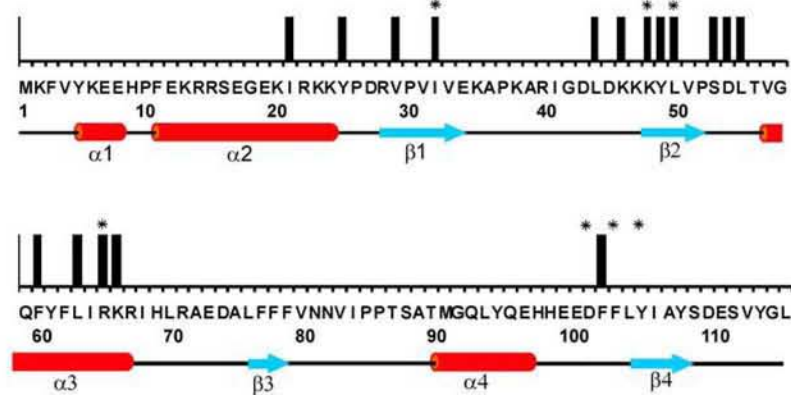
Abbildung 4.9: Lokalisierung der N1-Peptid Bindestelle von GABARAP. Unter der Darstellung der GABARAP-Sequenztopologie (Aminosäuren sind im Einbuchstaben-Aminosäure-Kode angegeben) sind die entsprechenden Sekundärstrukturelemente auf der X-Achse dargestellt. Von der Bindung des N1-Peptids am stärksten beeinträchtigte Aminosäuren sind auf der Y-Achse mit einem Balken gekennzeichnet. Die mit einem Stern (*) markierten Reste kennzeichnen die Aminosäuren, die in dem GABARAP-orthologen Hefeprotein Atg8 als wichtig für die Autophagozytose identifiziert wurden. Diese sind in GABARAP konserviert (Nakatogawa et al. 2007).
