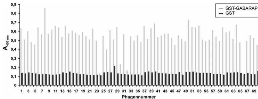
Abbildung 4.4: Einzelphagen-ELISA: Quantifizierung der Absorption bei 450 nm. GABARAP wurde auf einer Plastikoberfläche immobilisiert und mit einer definierten Menge von isolierten Einzelphagen inkubiert. Nach einigen Waschschritten wurde die Menge an gebundenen Phagen mittels Farbreaktion visualisiert und bei 450 nm detektiert. Je größer das detektierte Signal, desto stärker ist die Bindung des entsprechenden Phagen an GST-GABARAP (graue Balken) bzw. GST (schwarze Balken).
