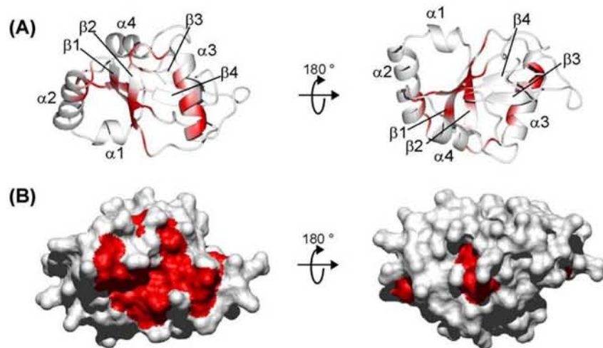
Abbildung 4.26: Visualisierung der CRT (178-188) Bindestelle an GABARAP. A: Aminosäurereste, deren Amidgruppen-Resonanzen im (^1\text{H}-^{15}\text{N}) -HSQC-Experiment von der Bindung des CRT (178-188)-Peptids am stärksten betroffen waren, sind rot eingefärbt. Sekundärstrukturelemente sind mit \alpha ( \alpha -Helix) und \beta ( \beta -Strang) und der entsprechenden Nummerierung gekennzeichnet. B: Oberflächendarstellung von A. Ribbon- und Oberflächendarstellung wurden mit Hilfe der Software „MOLEculum analysis and MOLEculum display“ (MOLEculum) erstellt.
