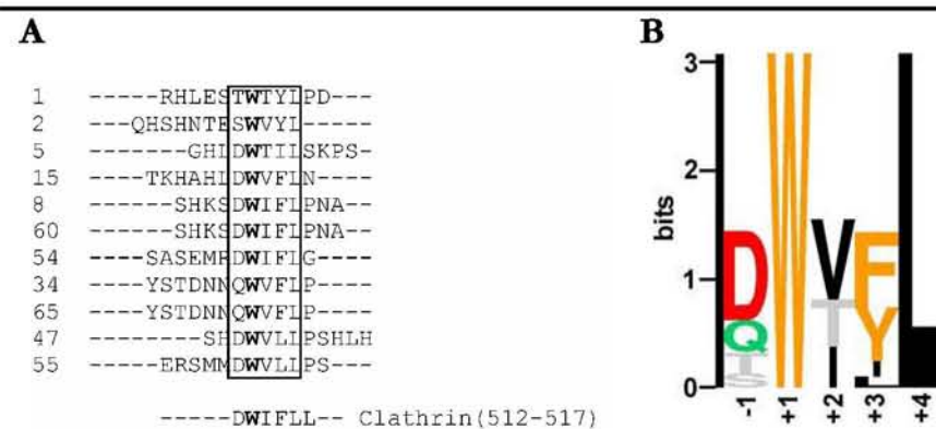
Abbildung 4.11: Erstellung eines „position-specific scoring matrix“ (PSSM) basierten, fünfstelligen Konsensusmotivs (Motiv 1) aus GABARAP-bindenden Peptidsequenzen. A: Multiples Sequenzalignment einer Auswahl von Phagendisplay selektierten GABARAP-bindenden Peptiden und der schweren Kette von Clathrin (CHC) (512 bis 517). Links ist die jeweilige Phagenklon-Nummer zu der entsprechenden Peptidsequenz aufgelistet. Der konservierte Tryptophanrest ist fettgedruckt hervorgehoben. Aminosäurepositionen, die bei der Erstellung der PSSM einbezogen wurden, sind mit einem Kasten umrandet. B: Das aus der PSSM errechnete Sequenzlogo, welches das Konsensusmotiv (Motiv 1) einer GABARAP-bindenden Sequenz grafisch repräsentiert. Die relative Größe der einzelnen Buchstaben ist dabei proportional zur Häufigkeit des mit diesem Buchstaben bezeichneten Restes an dieser Position und die absolute Höhe der jeweiligen Position ist proportional zum Grad der Konservierung.
