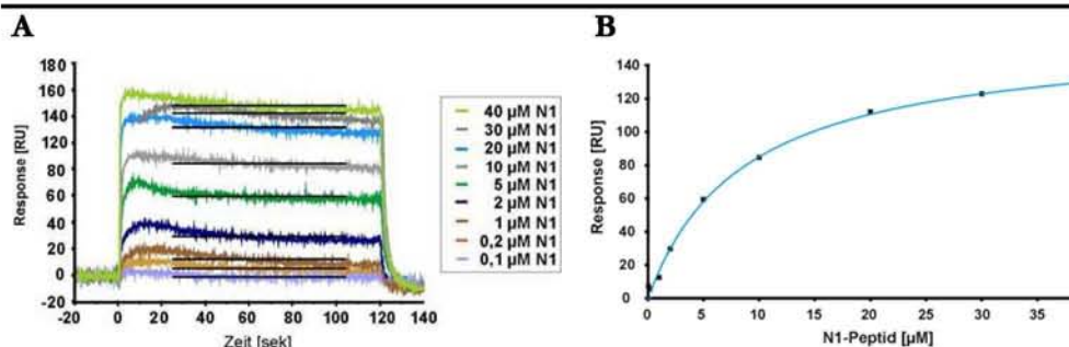
Abbildung 4.7: Bindungsstudie von GABARAP und N1-Peptid mit Oberflächenplasmonenresonanz A: Sensorgramm-Überlagerung der Bindungskurven unterschiedlicher N1-Konzentrationen injiziert auf einen GABARAP-gekoppelten CM5-Chip. Bei einer Flussgeschwindigkeit von 30 \mu\text{l}/\text{min} wurde je 2 min injiziert. Die schwarzen Balken markieren die gemittelte Signalintensität der „ steady state “ Phase der jeweiligen Injektion. B: Bindungskurve der N1-GABARAP Interaktion. Die gemittelte Signalintensität der jeweiligen Injektion ist gegen die entsprechende N1-Konzentration aufgetragen. Der Fit der nichtlinearen Regressionsrechnung ist als blaue Linie dargestellt.
