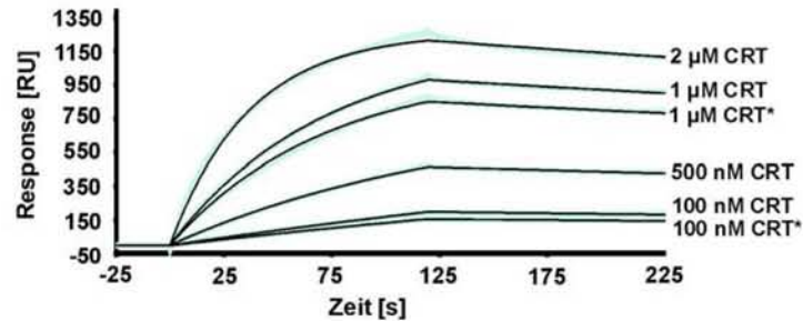
Abbildung 4.15: Kinetische Analyse der CRT-GABARAP Interaktion mittels Oberflächenplasmonenresonanz. Die Sensorgramme (hellblau) wurden sequenziell in der Reihenfolge 100 nM, 1 µM, 2 µM, 500 nM, 100 nM*, 1 µM* aufgenommen. Die Bindungskurven wiederholter Konzentrationen zeigten ein reduziertes Signalmaximum und wurden mit einem Stern (*) gekennzeichnet. Es wurde je Injektion eine 2-minütige Assoziations- und eine 2-minütige Dissoziationsphase aufgenommen und ausgewertet. Der beste Fit eines 1:1 bimolekularen Interaktionsmodells ist in schwarz dargestellt. Assoziations- und Dissoziationsrate, jedoch nicht das Maximalsignal ( R_{max} ), wurden global gefittet. Es ergab sich ein k_{on} = 1,3 \times 10^4 / M \cdot s und ein k_{off} = 8,3 \times 10^{-4} / s und damit eine Dissoziationskonstante K_D = 64 \text{ nM} .
