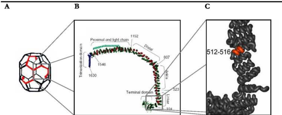
Abbildung 4.13: Lage der putativen GABARAP-Bindestelle (Aminosäurereste 512 bis 516) in der Clathrin heavy chain (CHC) Struktur A: Schema eines hexagonalen Fasses, bestehend aus 36 Clathrin Triskelia (Royle 2006). In rot ist ein einzelnes CHC Triskelion dargestellt. Der grau umrandete Bereich ist in (B) vergrößert zu sehen. B: Darstellung einer einzelnen schweren Kette Clathrin mit Sequenzbereichzuordnung und jeweiliger Beschriftung (Wilbur et al. 2005). Der grau umrandete Bereich ist in (C) vergrößert dargestellt. C: Ausschnitt aus der CHC PDB-Struktur 1X15, dargestellt mit „MOLEcule analysis and MOLEcule display“ (MOLMOL). In rot sind die Aminosäurepositionen 512 bis 516 markiert.
