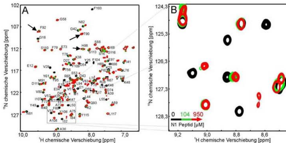
Abbildung 4.8: Überlagerung der (^1\text{H}-^{15}\text{N}) -HSQC-Spektren von GABARAP im freien Zustand und bei Bindung an das N1-Peptid. A: Überlagerung der Gesamt- (^1\text{H}-^{15}\text{N}) -HSQC-Spektren von 213 \mu\text{M} GABARAP ohne Zusatz (schwarz) und in Anwesenheit von 104 \mu\text{M} (grün) und 950 \mu\text{M} (rot) N1-Peptid. Die Zuordnung der Protein-Rückrad Resonanzen nach Stangler et al. ist in schwarz angegeben (Einbuchstaben-Aminosäure-Kode)(Stangler et al. 2002). Die Pfeile kennzeichnen beispielhaft Resonanzen, die nach Peptidzugabe einen doppelten Signalsatz zeigen. B: Vergrößerung des in (A) markierten Bereiches.
