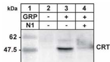
Abbildung 4.21: Endogenes CRT bindet an immobilisiertes GABARAP. Ungekoppelte Sepharose (Spur 2) und Sepharose-gekoppeltes GABARAP in Abwesenheit (Spur 3) und Anwesenheit (Spur 4) von 1150 \mu M N1-Peptid wurden mit Rattenhirnextrakten inkubiert. Nach mehreren Waschschr ten wurden gebundene Proteine eluiert und per SDS-PAGE aufgetrennt. Die Detektion von CRT erfolgte durch Western Blot Analyse. Spur 1 zeigt Signale des Prestained Protein Markers (Prestained Protein Marker, Broad Range, NEB, Beverly, MA, USA).
