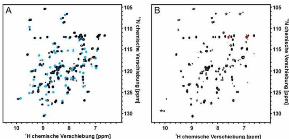
Abbildung 4.19: ( ^1\text{H} - ^{15}\text{N} )-HSQC Spektren von GABARAP in An- und Abwesenheit von Liganden A: GABARAP interagiert mit N1-Peptid. Überlagerung von ( ^1\text{H} - ^{15}\text{N} )-HSQC Spektren von 190 \mu\text{M} GABARAP in Abwesenheit (blaue Signale) und in Anwesenheit (schwarze Signale) von 950 \mu\text{M} N1-Peptid. B: N1-Peptid kompetiert mit CRT um die Bindung zu GABARAP. ( ^1\text{H} - ^{15}\text{N} )-HSQC Spektrum von 20 \mu\text{M} GABARAP in Anwesenheit von 20 \mu\text{M} CRT (rote Signale) überlagert mit einem Spektrum von 16 \mu\text{M} GABARAP, 16 \mu\text{M} CRT und 1180 \mu\text{M} N1-Peptid (schwarze Signale). Die mit einem Stern (*) gekennzeichneten Resonanzsignale entsprechen freiem N1-Peptid und treten aufgrund der natürlichen Häufigkeit von ^{15}\text{N} auf.
