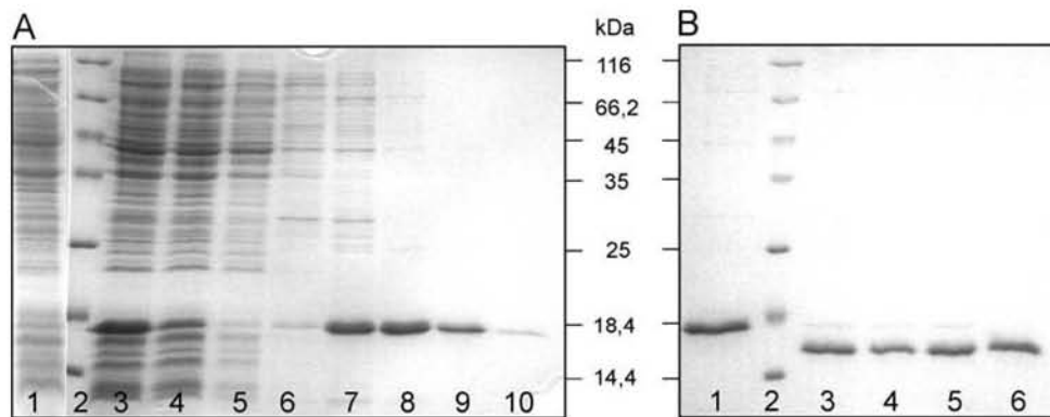
Abbildung 4.28: Reinigung und Proteaseverdau von rekombinantem MAP-LC3b. A: 15% SDS-PAGE zur Analyse der Expression und Ni-NTA-Reinigung von rekombinantem MAP-LC3b. Spur 1: Bakterienrohlysate vor Induktion; Spur 2: Molekulargewichts-Marker (MBI, Fermentas); Spur 3: Überstand des Zellaufschlusses nach Zentrifugation; Spur 4: Durchfluss; Spur 5: Waschschrift mit Bindungspuffer; Spur 6: Elution mit 10 mM Imidazol; Spur 7: Elution mit 50 mM Imidazol; Spur 8: Elution mit 100 mM Imidazol; Spur 9: Elution mit 150 mM Imidazol; Spur 10: Elution mit 500 mM Imidazol B: 15% SDS-PAGE zur Analyse des Proteaseverdaus von MAP-LC3b mit Thrombin bei RT. Spur 1: MAP-LC3b vor Proteaseverdau; Spur 2: Molekulargewichts-Marker (MBI, Fermentas); Spur 3: Thrombinverdau nach 30 min Inkubationszeit; Spur 4: Thrombinverdau nach 60 min Inkubationszeit; Spur 5: Thrombinverdau nach 90 min Inkubationszeit; Spur 6: Thrombinverdau nach 24 h Inkubationszeit
