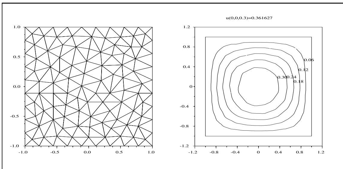
Abbildung 7.2: Ausgangsgitter \mathcal{Q} und die Lösung u(\mathbf{x}, \mathbf{y}, \tau) beim Crank-Nicolson-Verfahrens
