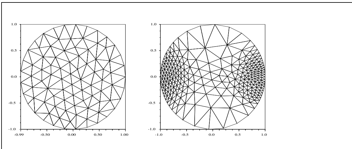
Abbildung 6.1: Ausgangsgitter \mathbf{K} und mit der Gitterfunktion \mathbf{u} adaptiertes Gitter \mathbf{KA}
