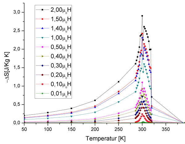
Abbildung A.4.: MCE von MnFe_4Si_3 berechnet aus der temperaturabhängigen Magnetisierung. ( H || [120] )
