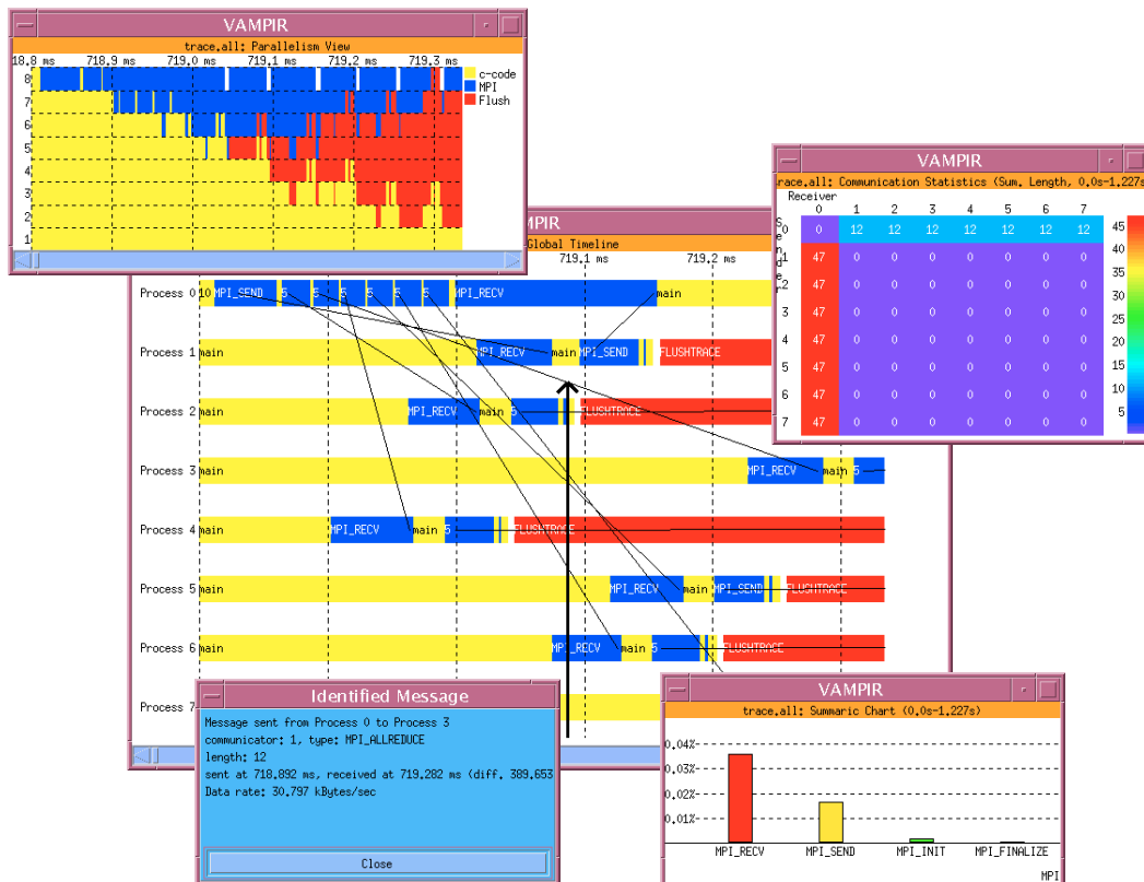
Abbildung 2.8: Analyse mit VAMPIR
