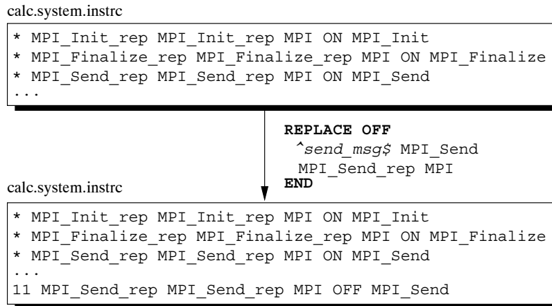
Abbildung 5.14: Abarbeitung einer REPLACE-Anweisung
