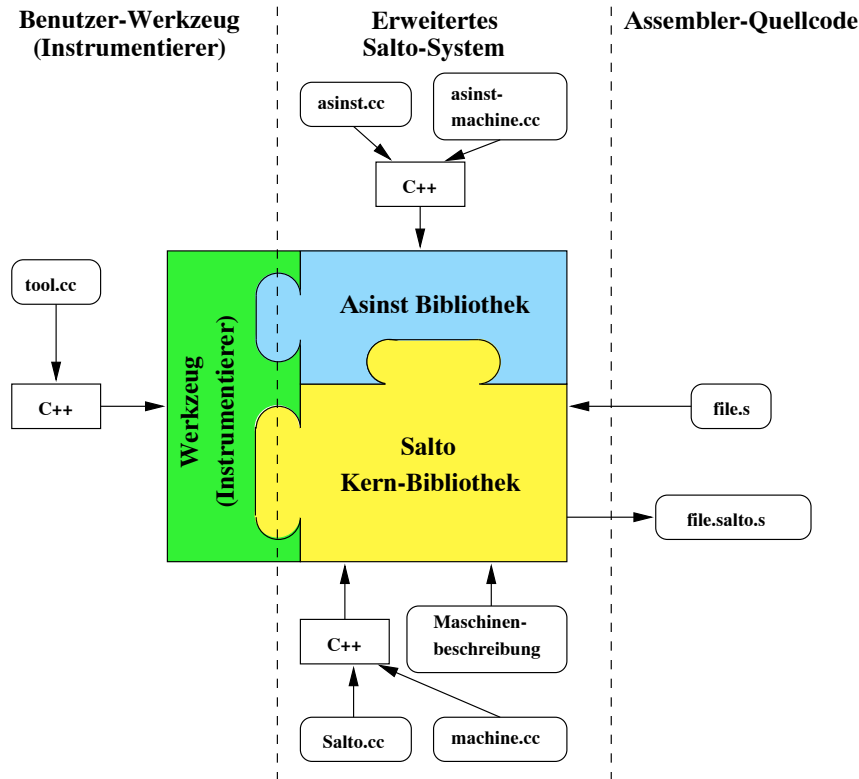
Abbildung 5.2: Implementierung der Bibliothek ASINST
