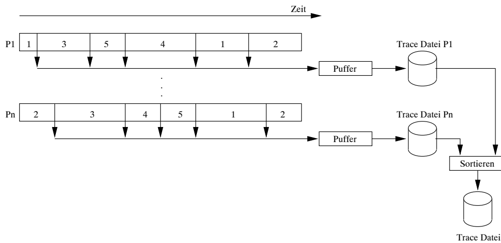
Abbildung 2.1: Tracing von parallelen Programmen
