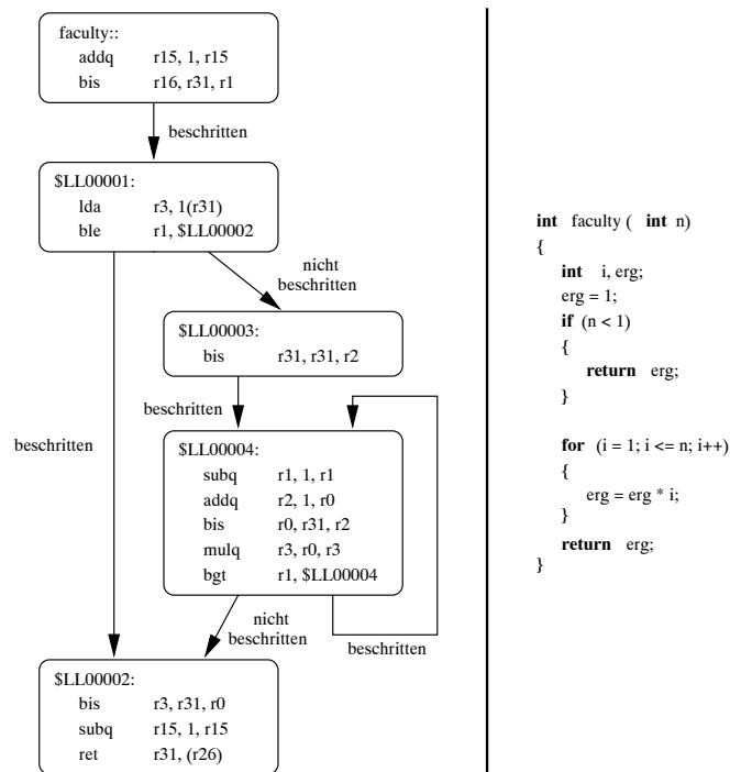
Abbildung 3.2: Kontrollflußgraph einer einfachen Prozedur
