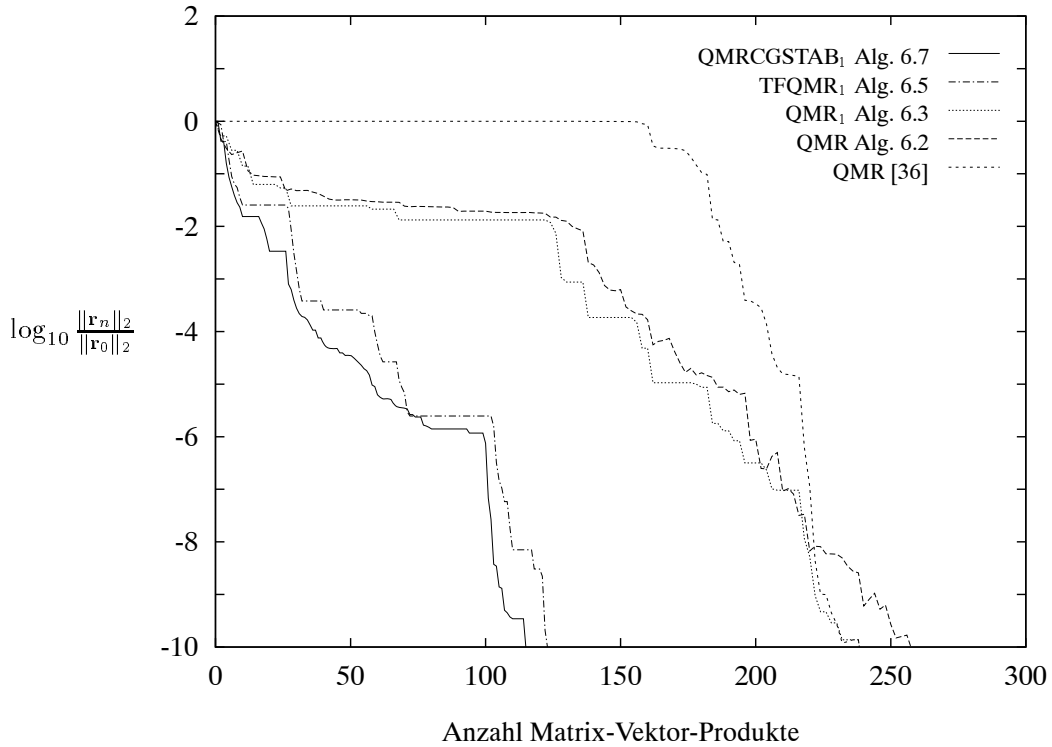
Abbildung 7.5: Konvergenzverläufe aus Exp. 7.3 im Überblick
