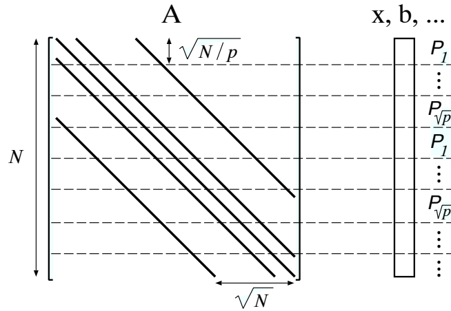
Abbildung 3.3: Blockzyklische Datenverteilung in Matrixrepräsentation
