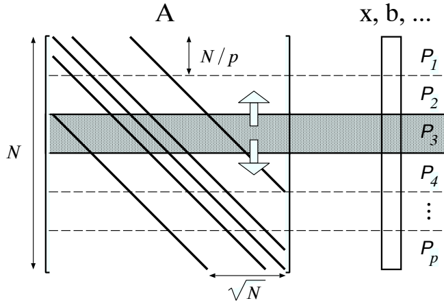
Abbildung 3.2: Blockdatenverteilung
