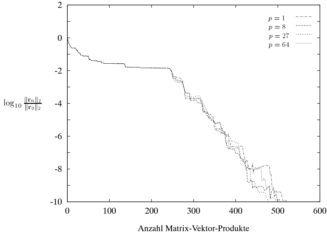
Abbildungung 7.6: Konvergenzverläufe aus Exp. 7.3 in Abhängigkeit der Prozessoranzahl p für die parallele Variante aus Alg. 6.2
