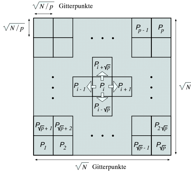
Abbildung 3.4: Blockzyklische Datenverteilung in Gitterpunktrepräsentation
