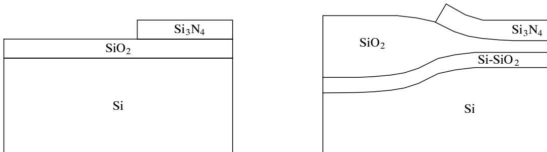
Abbildung 1.1: Zweidimensionaler Schnitt durch eine typische Halbleiterstruktur zum Ausgangszeitpunkt (links) und nach der Verformung durch Oxidation (rechts).
