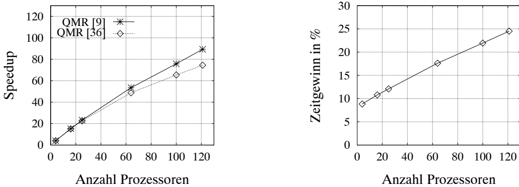
Abbildung 7.8: Speedup und relativer Zeitgewinn der Variante [9] gegenüber der Variante [36] für das zweidimensionale Beispiel aus Exp. 7.3
