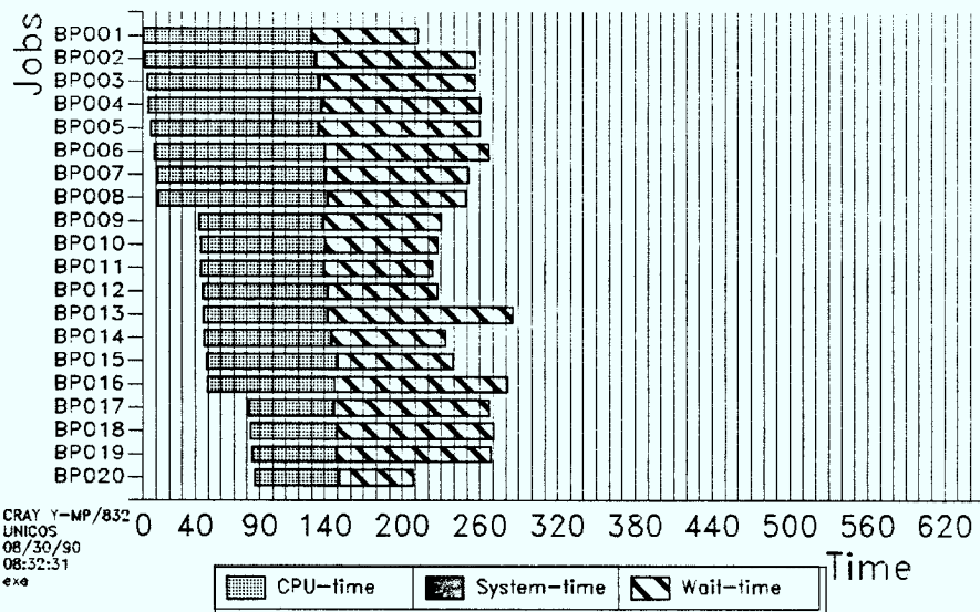
Abb. 31. Der Referenz-Benchmark auf Cray X-MP und Cray Y-MP
