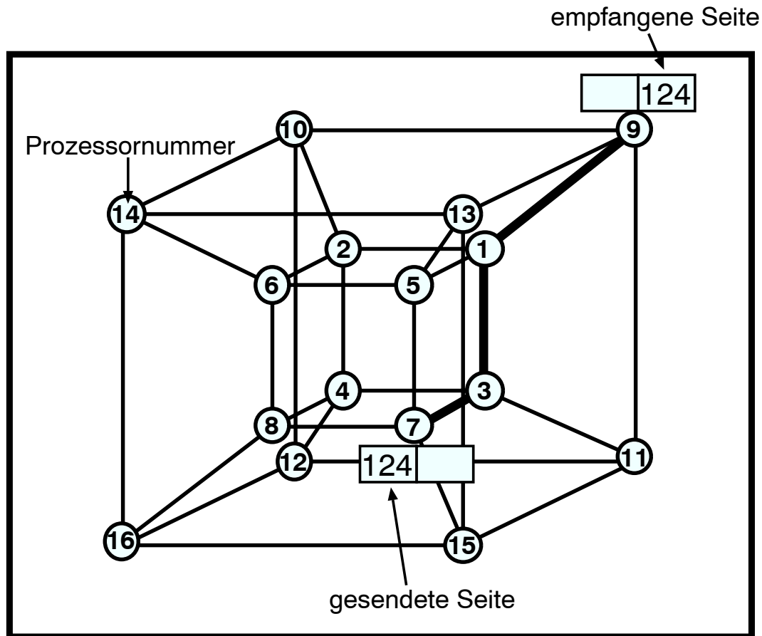
Abbildung 5.9: Visualisierung der Kommunikation im Prozessornetz
