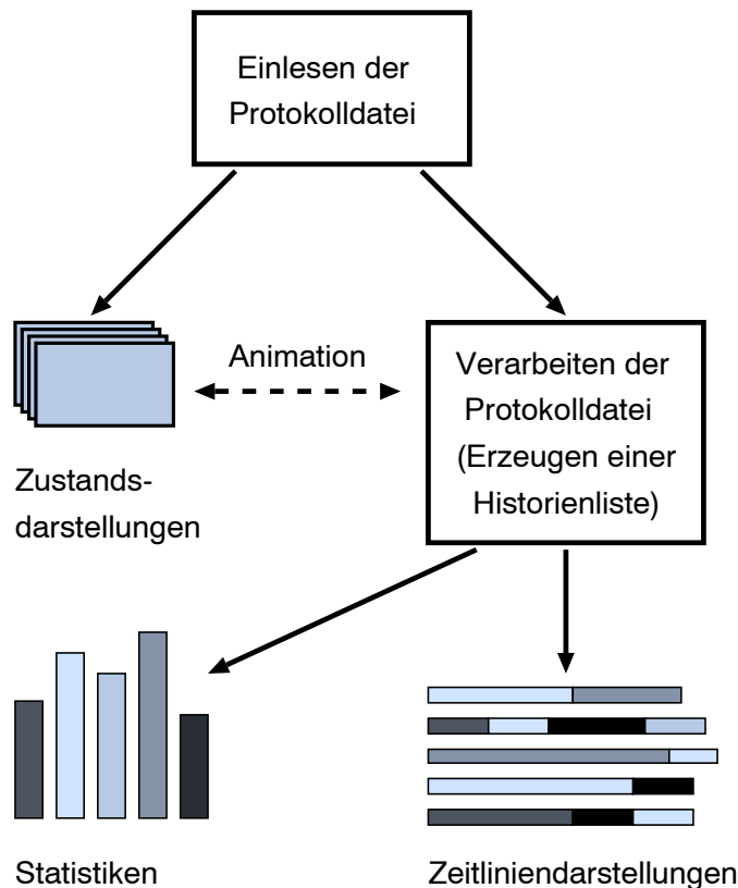
Abbildung 4.3: Die Bedienungsphilosophie der Visualisierungsumgebung PARvis
