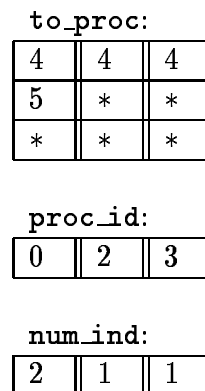
Abbildung 5.9: Speicherung der Indizes der Komponenten, die gesendet werden, Prozessor 1
