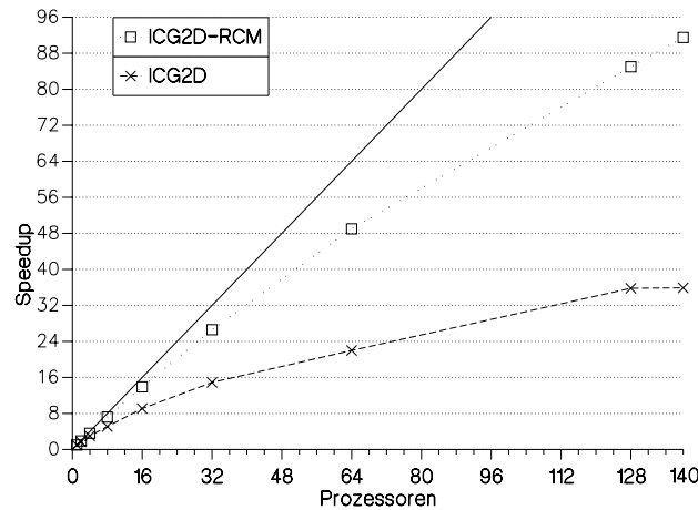
Abbildung 6.7: Speedup-Werte ohne und mit Bandbreitenreduktion, Matrix ICG2D
