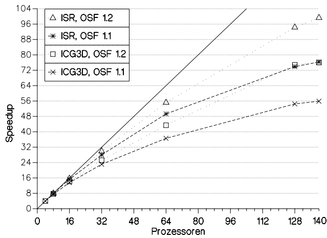
Abbildung 6.17: Speedup-Verhalten ohne und mit Einsatz des Kommunikationsprozessors
