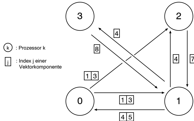
Abbildung 5.12: Datenaustausch der zeilenweisen Matrix-Vektor-Multiplikation, Umordnung in Blöcke
