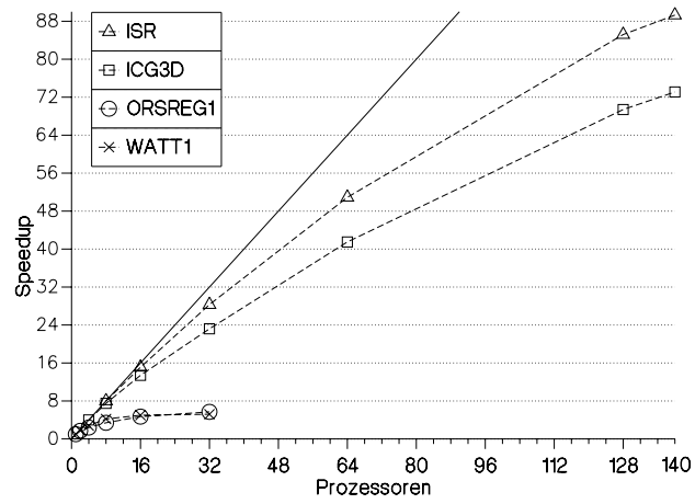
Abbildung 6.27: Speedup-Werte des QMR-Verfahrens
