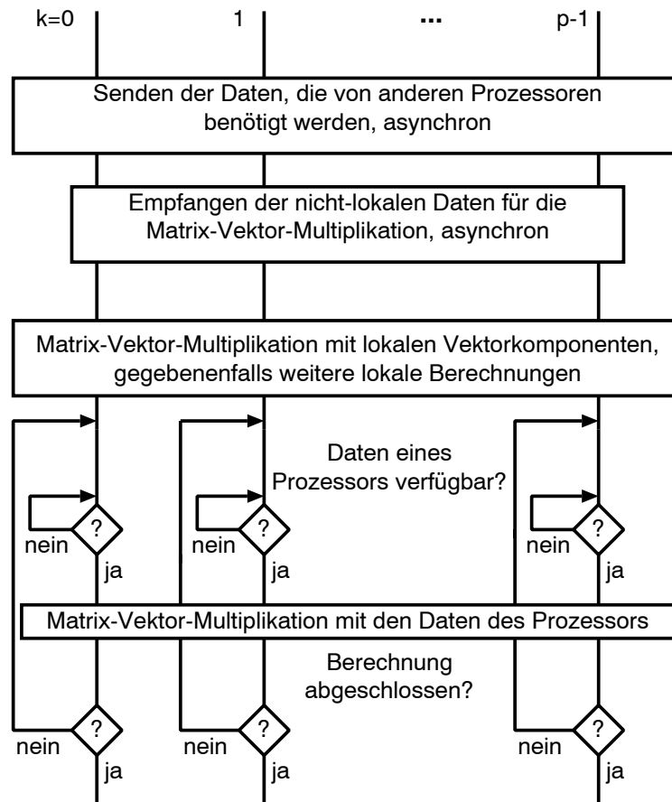
Abbildung 5.14: Ablauf der parallelen zeilenweisen Matrix-Vektor-Multiplikation mit Block-Sortierung
