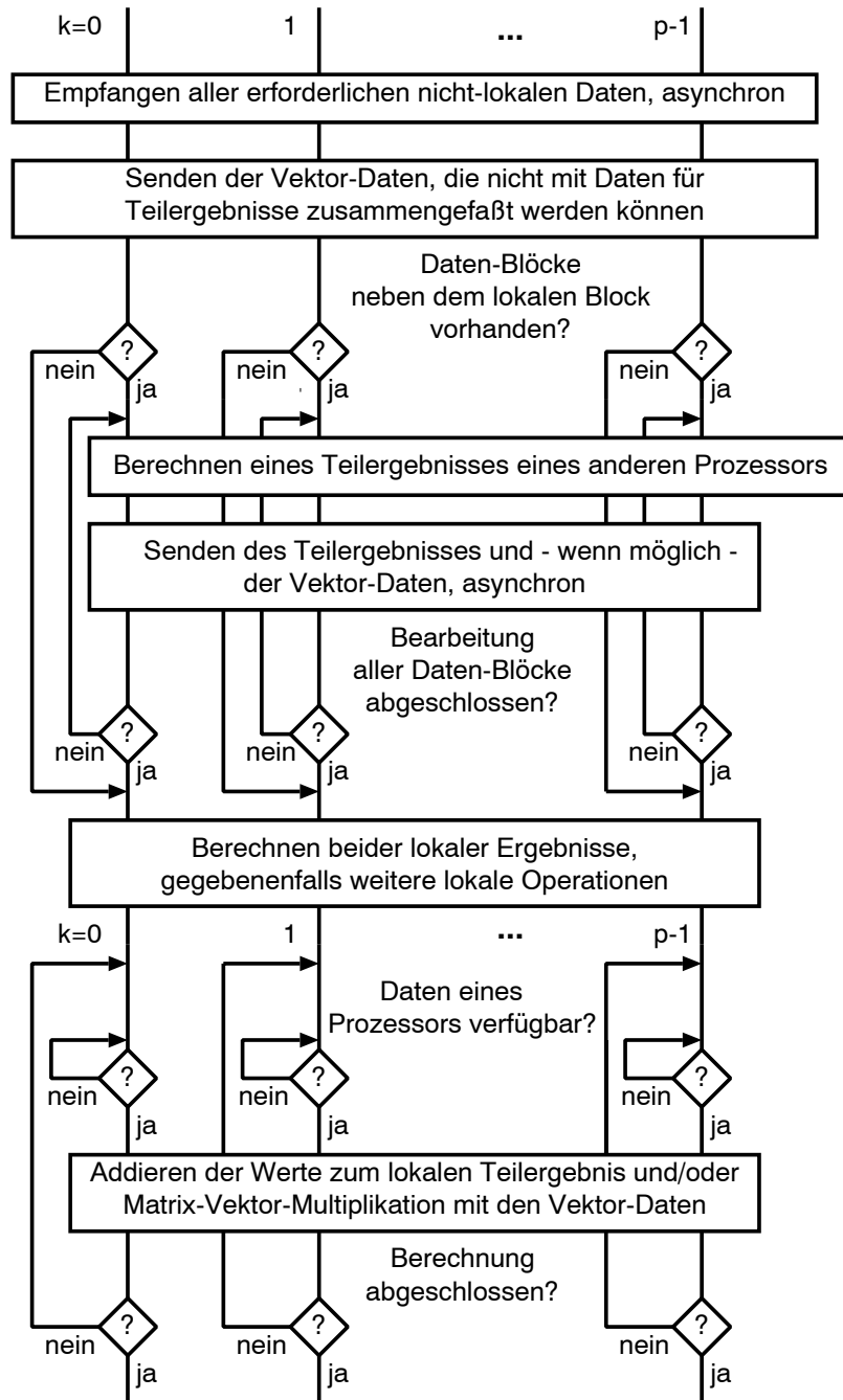
Abbildung 5.20: Kopplung der parallelen zeilen- und spaltenweisen Matrix-Vektor-Multiplikation
