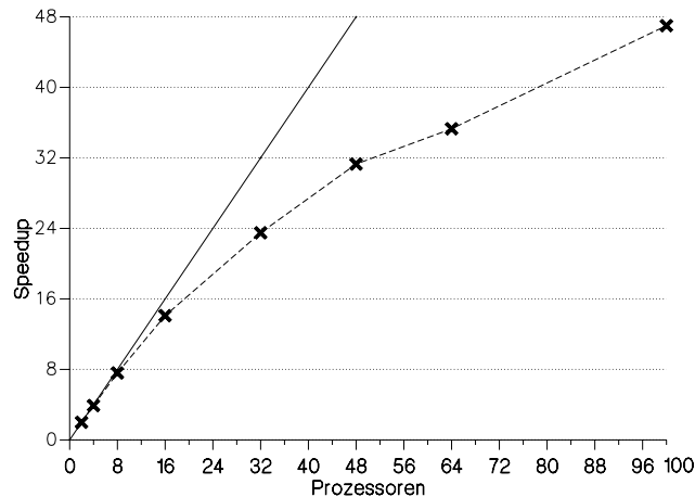
Abbildung 6.36: Speedup-Verhalten der parallelen Matrix-Vektor-Multiplikation, Matrix ICG2D-RCM
