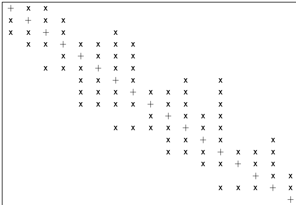
Abbildung 3.17: Struktur einer unsymmetrischen Profil-Matrix
