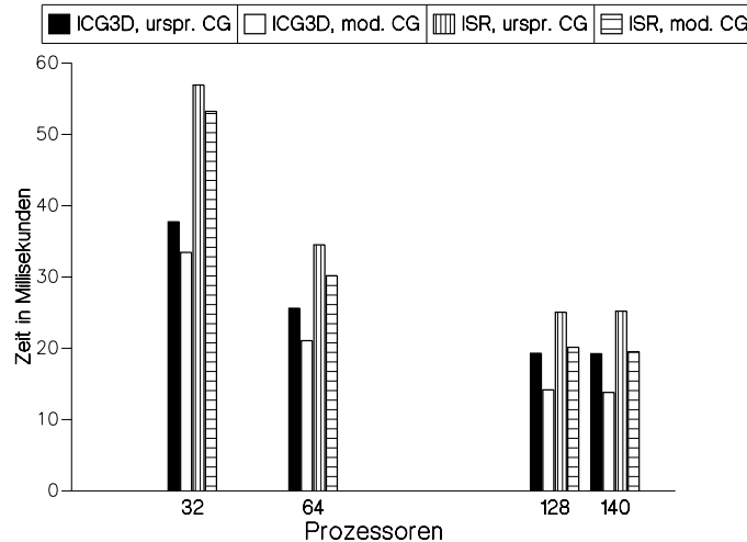
Abbildung 6.11: Ausführungszeiten des ursprünglichen und des modifizierten CG-Verfahrens
