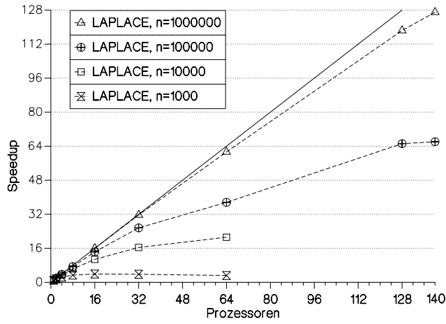
Abbildung 6.16: Speedup-Verhalten des CG-Verfahrens für die Matrizen LAPLACE
