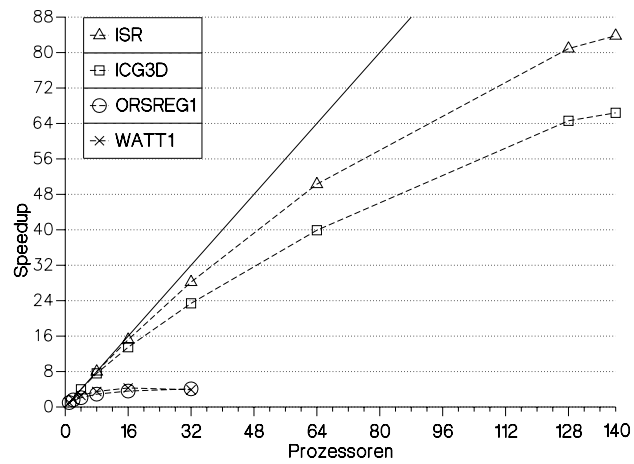
Abbildung 6.28: Speedup-Werte des TFQMR-Verfahrens
