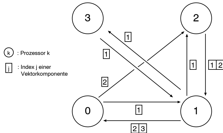
Abbildung 5.17: Datenaustausch der zeilenweisen Matrix-Vektor-Multiplikation, Neuverteilung der Blöcke
