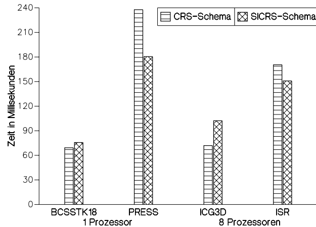
Abbildung 6.4: Vergleich der Algorithmen zur Matrix-Vektor-Multiplikation im CRS- und SICRS-Format
