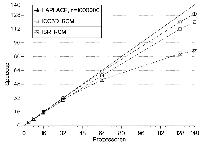
Abbildung 6.34: Speedup-Verhalten der Lanczos-Methode
