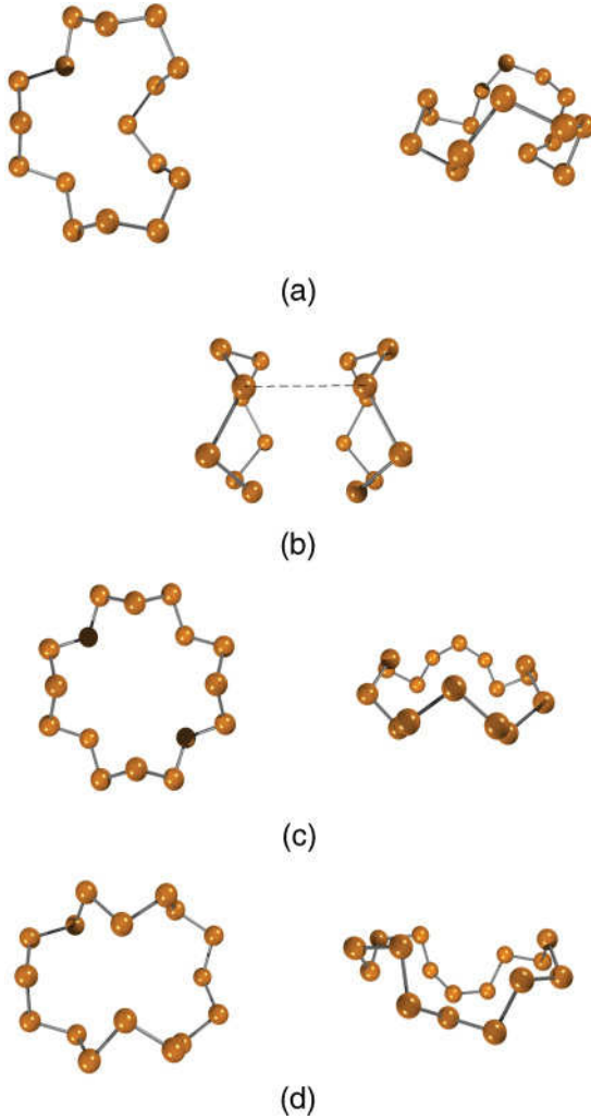
FIG. 3. (Color online) Isomers of \text{Te}_{16} : (a) C_{3s} , (b) \text{Te}_8 dimer, (c) D_{4d} , and (d) C_{5s} .
