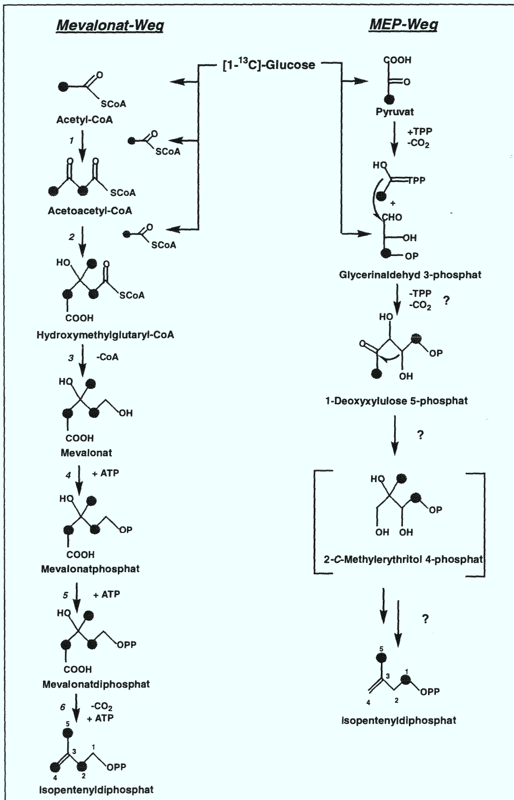
Abb. 2: Inkorporation von [1-^{13}\text{C}] -Glukose über den Mevalonat bzw. über den 2-C-Methylerythritol 4-phosphat-Weg (MEP-Weg); der Glukoseabbau erfolgt über den Embden-Meyerhof-Parnas-Weg; 1: Acetyl-CoA-Acetyltransferase, 2: HMG-CoA-Synthase, 3: HMG-CoA-Reduktase, 4: Mevalonat-Kinase, 5: Phosphomevalonat-Kinase, 6: Diphosphomevalonat-Decarboxylase
