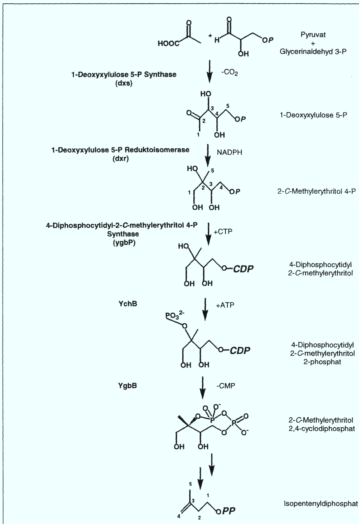
Abb. 35: Biosynthese von Isopentenyl diphosphat über den 2-C-Methylerythritol 4-phosphat Weg
