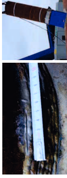
Abbildung 17: Künstlich eingebrachter Fehler, Größe 4,5 mm lang, 5 mm tief ( \frac{1}{3} Rohrstärke), 0,9 mm Öffnungsweite (links) und dessen Detektion mit Ultraschall (rechts)
