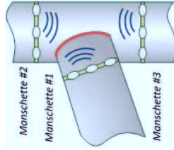
Abbildung 13: Sensormanschetten-technologie zur Überwachung der Schweißnaht (rot gekennzeichnet)
