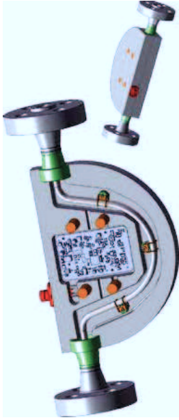
Abbildung 7: Finales Design mit druckfestem Gehäuse, eingebauter Platine, Sensor, Flanschanschlüssen und Subsea-Steckverbinder.
