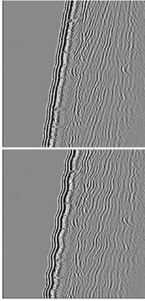
Abbildung 9: Heave Correction zum Herausrechnen der Schiffsbewegung
