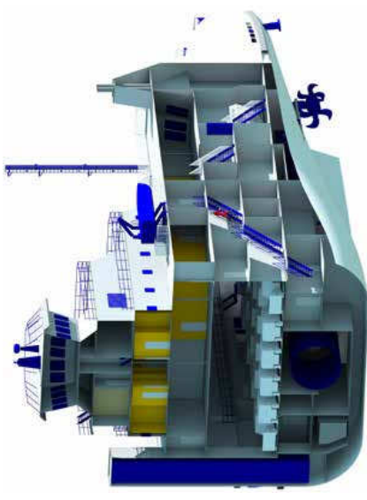
Abbildung 5: Beispiel für ein 3D-Generalplanmodell und die zu modellierenden Geometrien
