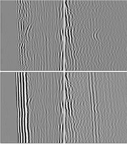
Abbildung 11: Erhöhung der Detektierbarkeit von Hyperbeln durch Eliminierung multipler Bodenreflexionen
