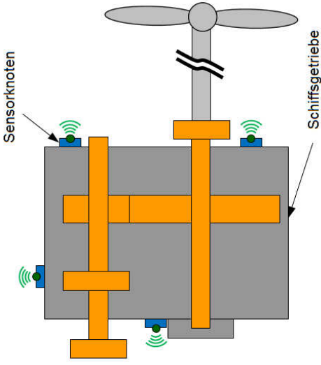
Abbildung 1: Zustandsüberwachung am Schiffsgetriebe mit Hilfe autarker Sensoren
