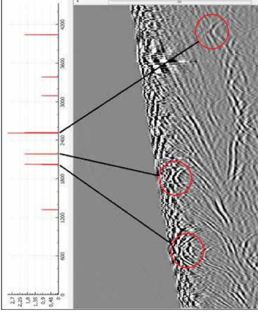
Abbildung 12: MLFF-basierte Objektdetektion
