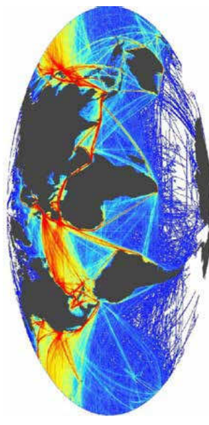
Alle Messungen aller Parameter zu allen Zeiten; große Bereiche der Ozeane – und somit der Erde - werden nicht abgedeckt. Quelle: Dr Boris Kelly-Gerreyn; NOC, EuroGOOS FerryBox Meeting, Göteborg 16-17 March 2010
