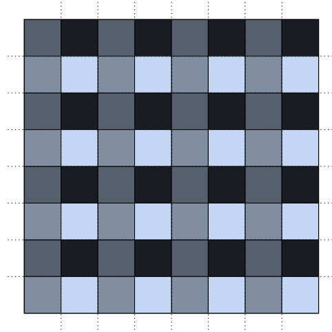
Abbildung 8: Blockzyklische Verteilung einer Matrix auf vier Prozessoren.
