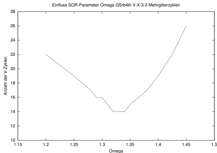
Abbildung 8: HOC Approximation 4. Ordnung mit Gauss-Seidel-Red-Black
