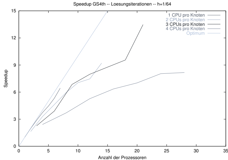
Abbildung 7: HOC Approximation 4. Ordnung mit Gauss-Seidel-Red-Black
