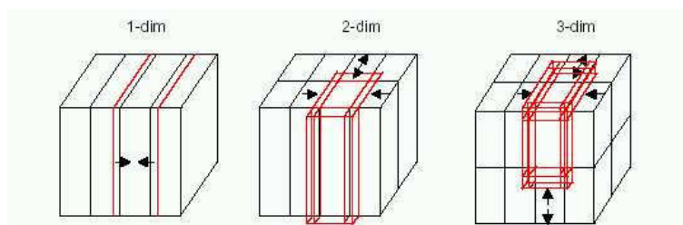
Abbildung 2: Verschiedene Strategien zur Datenverteilung auf die Prozessoren
