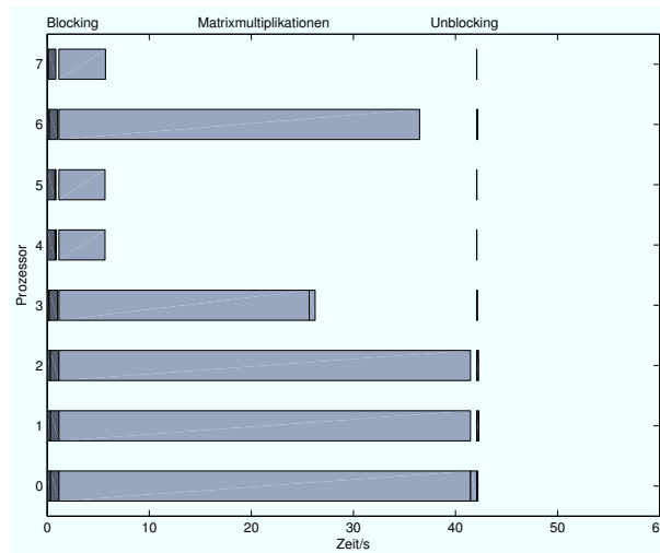
Abbildung 15: Verteilung der Arbeit auf dem ZAMpano Linux-SMP-Cluster bei Ähnlichkeitstransformation einer 4000 \times 4000 Matrix mit 7 Blöcken, Blockgrößen 200, 1200, 700, 200, 500, 800 und 400.
