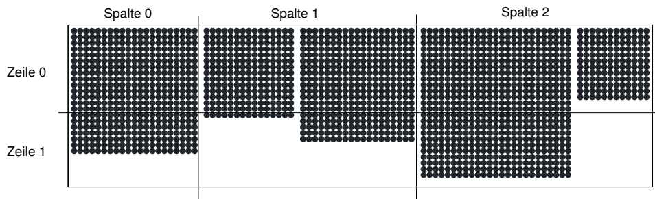
Abbildung 9: Abspeicherung der Blöcke der Beispielmatrix aus Abbildung 1 in einem Feld und Verteilung dieses Feldes auf ein 2 \times 3 -Prozessorgitter.
