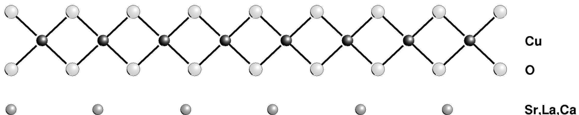
Abbildung 1: Kupferoxidkette in (\text{Sr},\text{La},\text{Ca})_{14}\text{Cu}_{24}\text{O}_{41} . Gezeigt wird die Aufsicht auf einen Ausschnitt einer Kettenebene, ergänzt durch die Positionen der Strontium-, Lanthan- oder Calcium-Atome.
