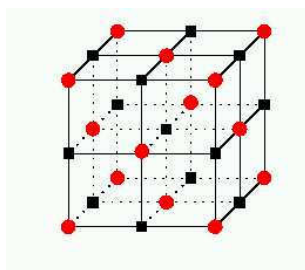
Abbildung 3: Rot-Schwarz-Aufteilung der Gitterpunkte beim Red-Black-Gauss-Seidel
