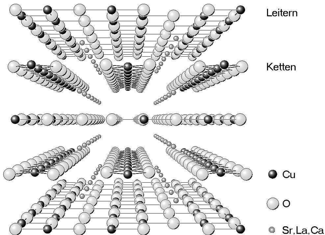
Abbildung 2: Dreidimensionale Darstellung der Ebenenstruktur von (\text{Sr,La,Ca})_{14}\text{Cu}_{24}\text{O}_{41}
