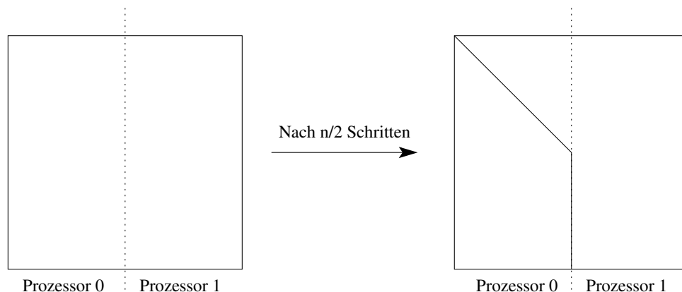
Abbildung 7: Problem der Datenverteilung beim Gauss-Verfahren auf zwei Prozessoren.
