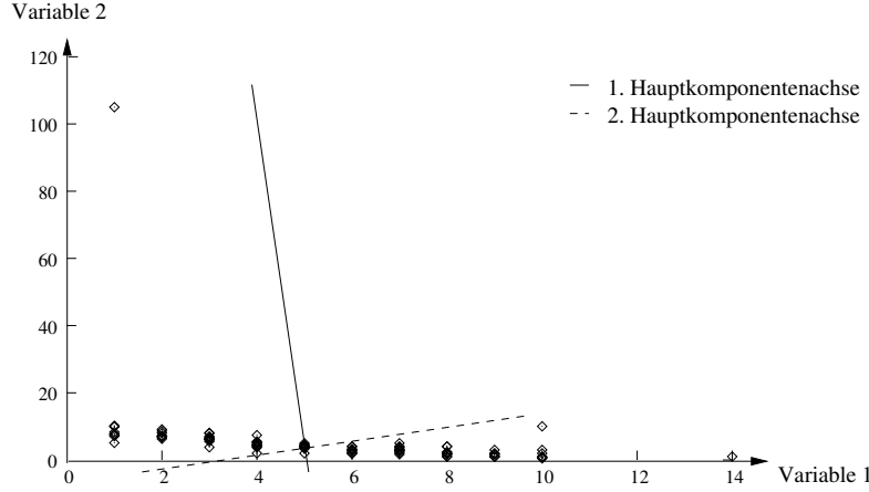
Abbildung 6: Plot der 109 Beobachtungen zweier Variabler mit eingezeichneten Hauptkomponentenachsen (berechnet mittels Kovarianzmatrix)
