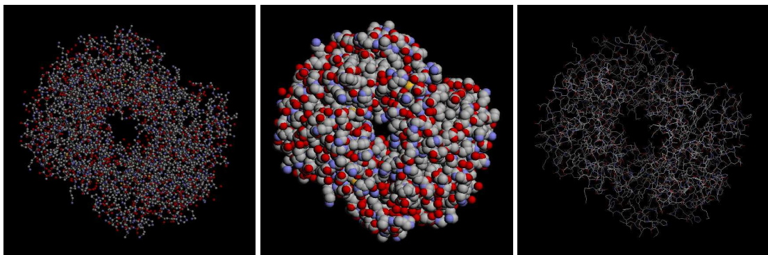
Abbildung 1: Verschiedene Darstellungen eines Moleküls. Von Links nach Rechts: Ball and Stick, Spacefill, Bonds.
