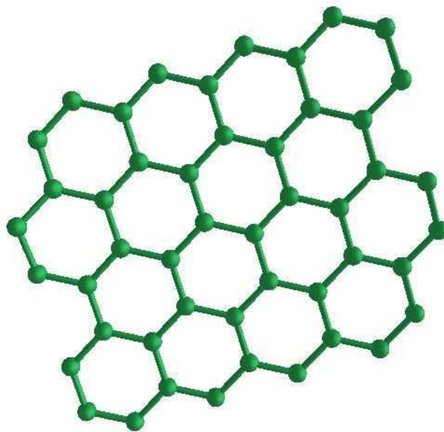
Abbildung 5: Graphitstruktur.
