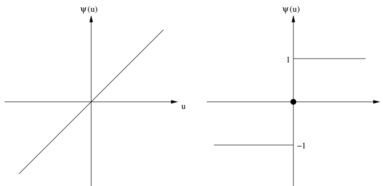
Abbildung 2: Graphen der \psi -Funktionen für die M-Schätzer Stichprobenmittelwert und Median
