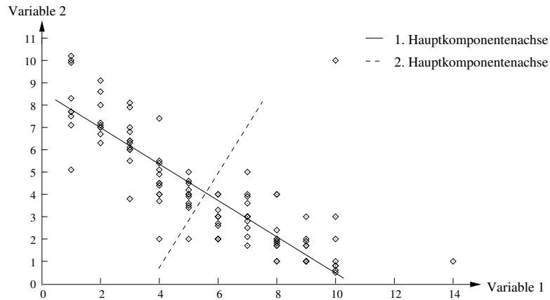
Abbildung 7: Plot der 108 Beobachtungen (außer dem Ausreißer) zweier Variabler mit eingezeichneten Hauptkomponentenachsen (robust berechnet mittels Kovarianzmatrix)
