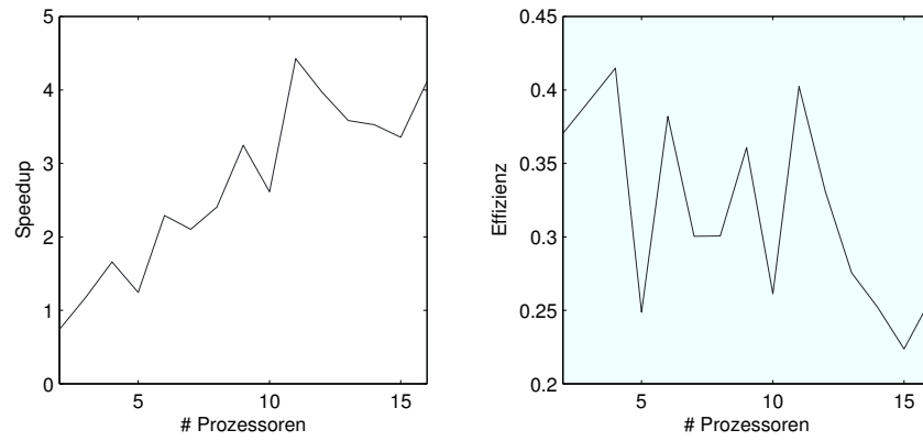
Abbildung 14: Speedup und Effizienz der Lösung des Eigenwertproblems der 12000 \times 12000 -Matrix mit 5 Blöcken (vgl. Tabelle 3).
