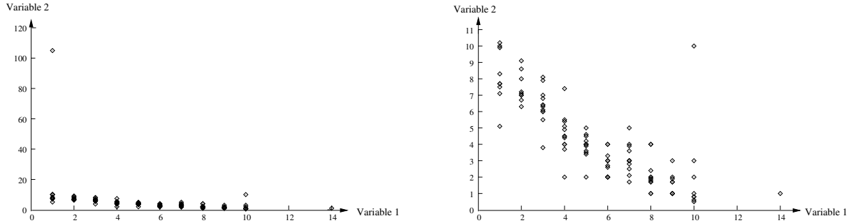
Abbildung 1: Auf der linken Seite Plot von 109 Beobachtungen zweier Variabler, auf der rechten Seite Plot der Daten nach Eliminierung des Ausreißers (1, 105). Man kann erkennen, dass nach der ersten Iteration zur Eliminierung von Ausreißern ein weiterer Ausreißer identifiziert werden kann. In anderen Fällen können noch sehr viel mehr Iterationen nötig sein.
