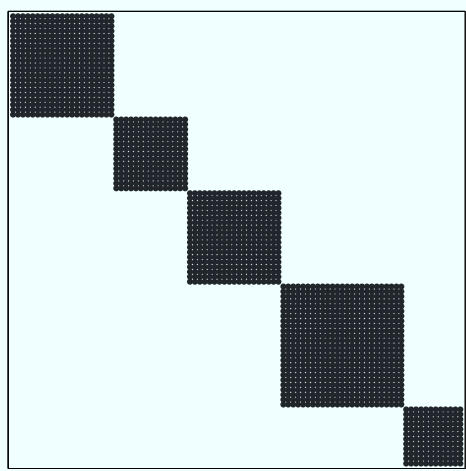
Abbildung 1: Beispiel für eine blockdiagonale Matrix.
