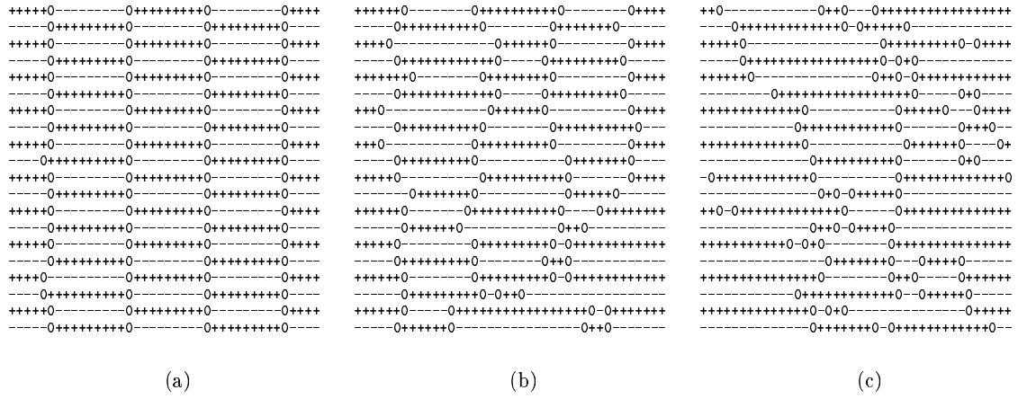
Abbildung 5: Typische Monte Carlo-Konfigurationen im thermodynamischen Gleichgewicht für das Minimalmodell ohne externes Feld, H = 0 , bei einem Pinning-Potential der Stärke E_p = |J_a| . Ausschnitte aus Systemen der Größe M = N = 40 bei den Temperaturen k_B T/|J_a| = 0.8 (a), 2.3 (b) und 2.9 (c).
