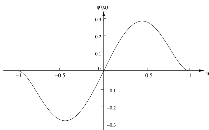
Abbildung 4: Graph der biweight- \psi -Funktion
