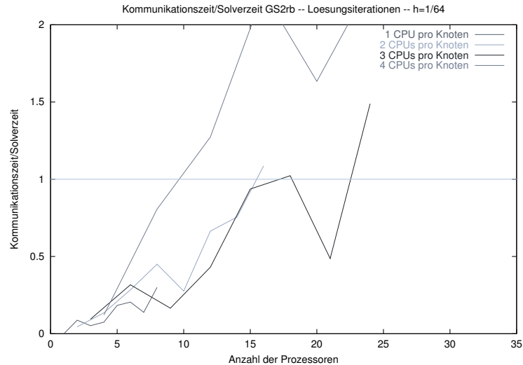
Abbildung 5: Klassische Approximation 2. Ordnung mit Gauss-Seidel-Red-Black
