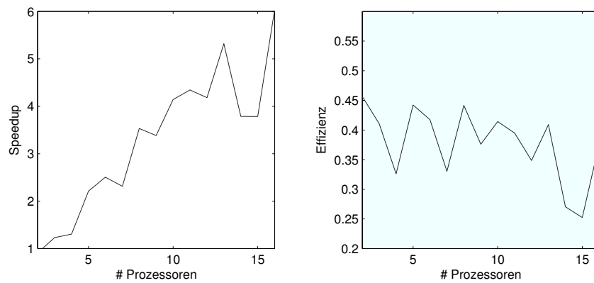
Abbildung 11: Speedup und Effizienz der Ähnlichkeitstransformation der 8000 \times 8000 -Matrix mit 7 Blöcken (vgl. Tabelle 2).
