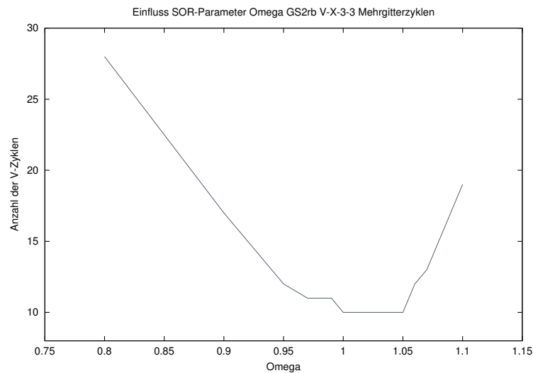
Abbildung 6: Klassische Approximation 2. Ordnung mit Gauss-Seidel-Red-Black
