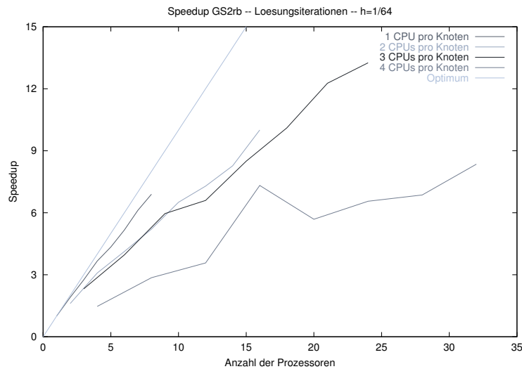
Abbildung 4: Klassische Approximation 2. Ordnung mit Gauss-Seidel-Red-Black
