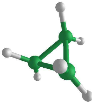
Abbildung 3: Cyclopropan: Molekül aus der Punktgruppe D_{3h} , eine Symmetriegruppe der Ordnung 12.
