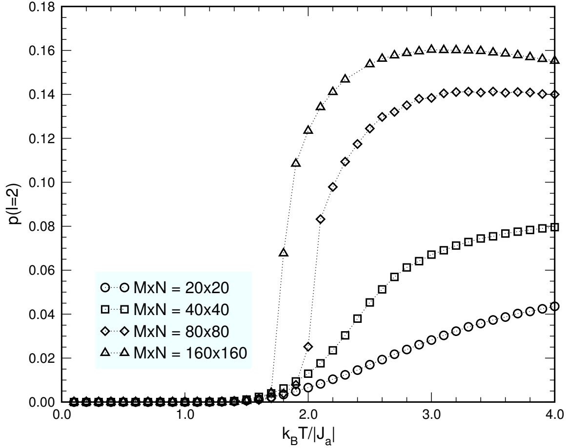
Abbildung 7: Defektpaar-Häufigkeit, p(l = 2) , im Minimalmodell ohne externes Feld, H = 0 , bei einem Pinning-Potential der Stärke E_p = |J_a| .
