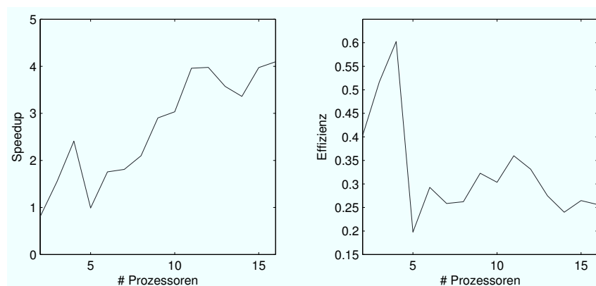
Abbildung 13: Speedup und Effizienz der Ähnlichkeitstransformation der 12000 \times 12000 -Matrix mit 5 Blöcken (vgl. Tabelle 3).
