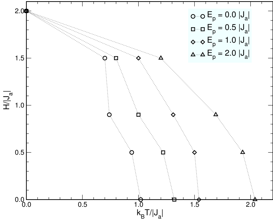
Abbildung 9: Phasengrenzen des Minimalmodell im thermodynamischen Limes, M, N \rightarrow \infty für verschieden starke Pinning-Potentiale in Abhängigkeit von der Temperatur T und der Stärke des externen Feldes H
