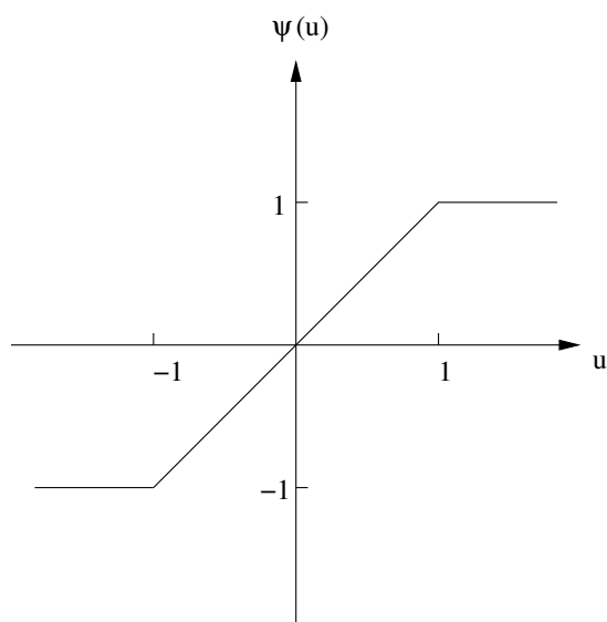
Abbildung 3: Graph der Huber- \psi -Funktion
