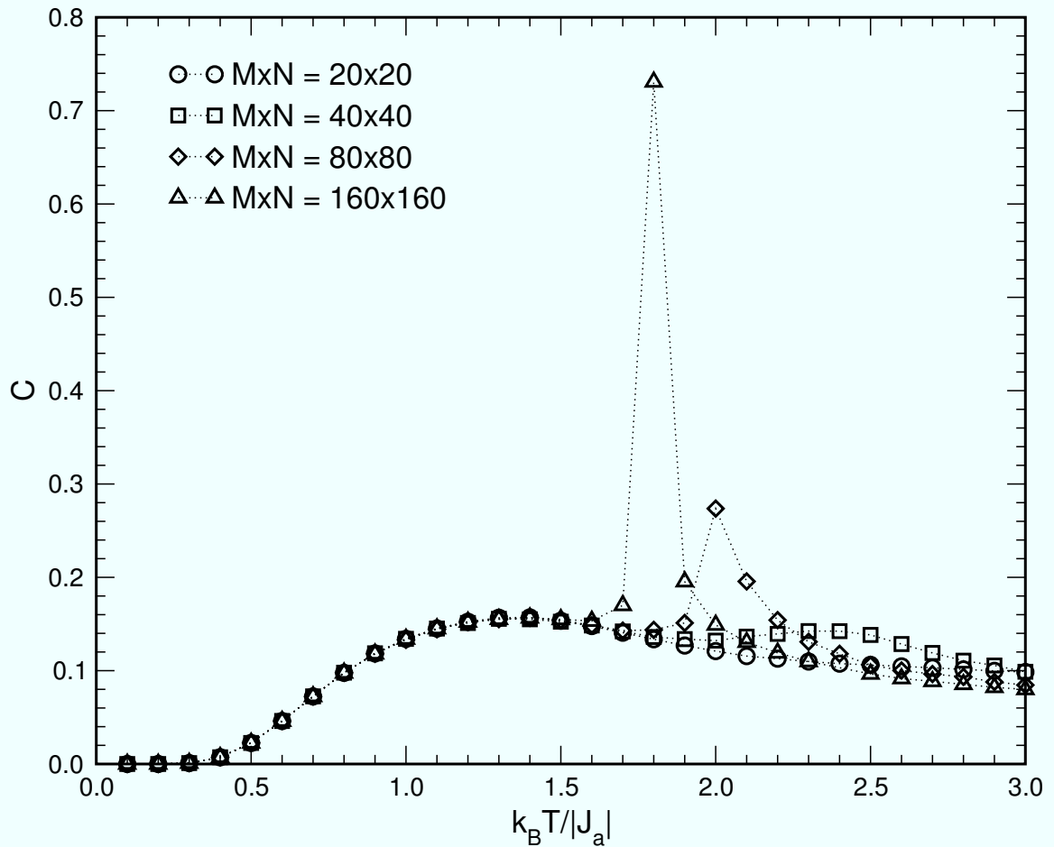
Abbildung 6: Spezifische Wärme C im Minimalmodell ohne externes Feld, H = 0 , bei einem Pinning-Potential der Stärke E_p = |J_a| .
