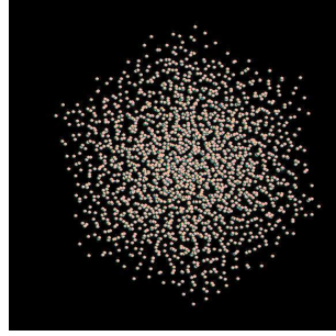
Abbildung 1: Eine Verteilung von geladenen Teilchen im Raum
