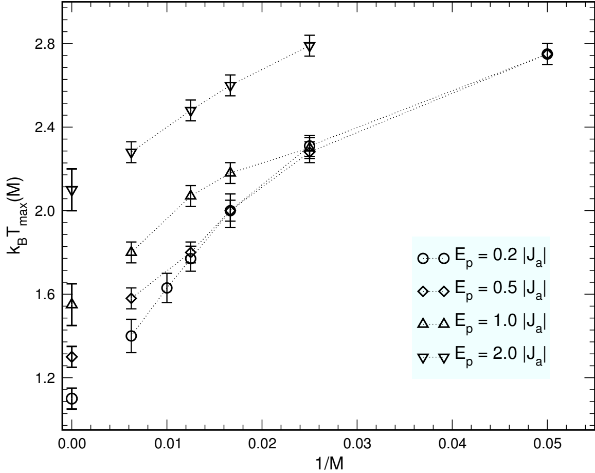
Abbildung 8: Extrapolation der Position des zweiten Maximums der spezifischen Wärme T_{\max} in Abhängigkeit von der inversen Systemlänge 1/M für verschiedene Pinning-Stärken E_p im Minimalmodell ohne externes Feld, H = 0 .
