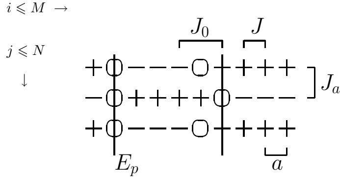
Abbildung 3: Skizze der Wechselwirkungen im Ising-Modell mit periodischem Pinning mobiler Defekte, a bezeichnet die in beiden Gitterachsen gleiche Gitterkonstante. Der 'Spin-Up'-Zustand, S_{ij} = +1 wird hier verkürzend mit '+', der 'Spin-Down'-Zustand, S_{ij} = -1 mit '-' bezeichnet. Defekte, S_{ij} = 0 werden mit dem Symbol '0' dargestellt.
