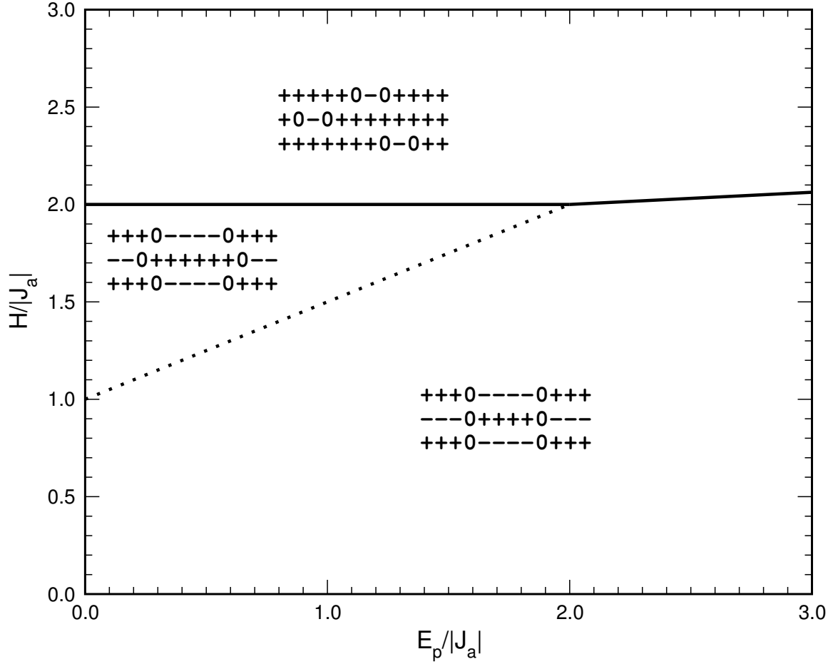
Abbildung 4: Grundzustände des Minimalmodells in Abhängigkeit von der Stärke des externen Feldes H und der des Pinning-Potentials E_p , das externe Feld favorisiert hier den 'Spin-Up'-Zustand.
