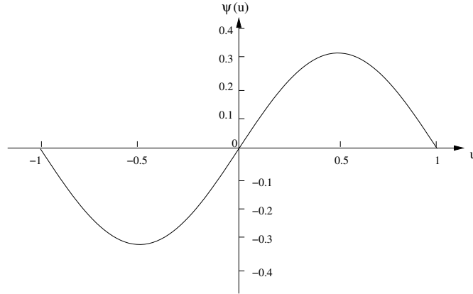
Abbildung 5: Graph der wave- \psi -Funktion
