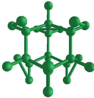
Abbildung 4: Diamantstruktur.
