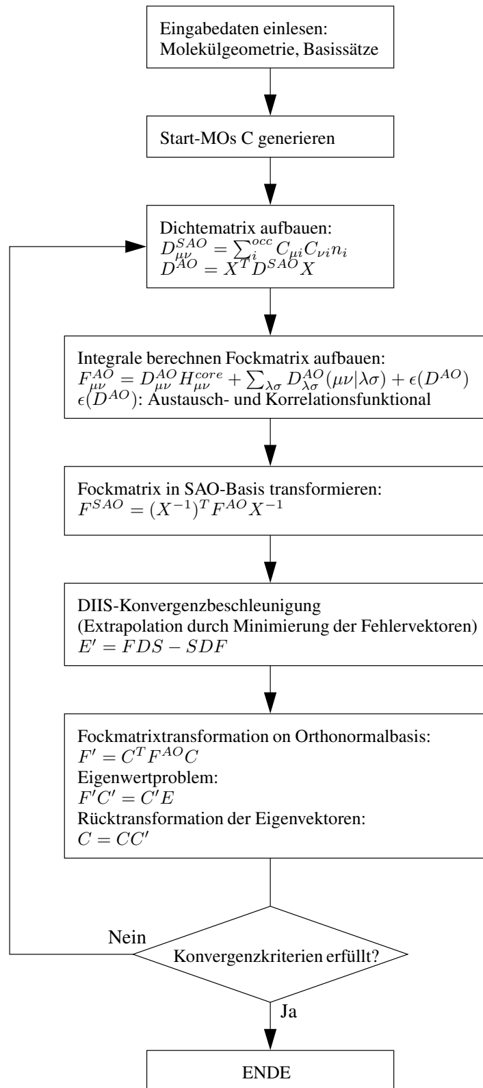
Abbildung 2: Ablauf des Hartree-Fock-Verfahrens.
