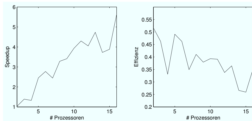
Abbildung 12: Speedup und Effizienz der Lösung des Eigenwertproblems der 8000 \times 8000 -Matrix mit 7 Blöcken (vgl. Tabelle 2).
