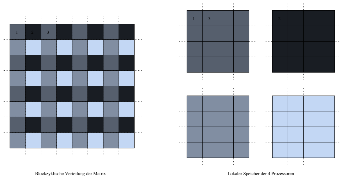
Abbildung 10: Zusammenhang zwischen lokalem Speicher eines Prozessors und blockzyklischer Verteilung.
