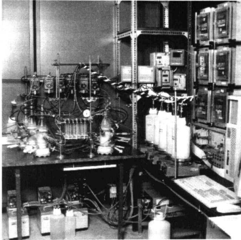
Abb. 4-4 : Photographie der Parallelfertigungsanlage, wie sie z.B. zum Cosubstratscreening in kontinuierlicher Fermentation eingesetzt wurde.
