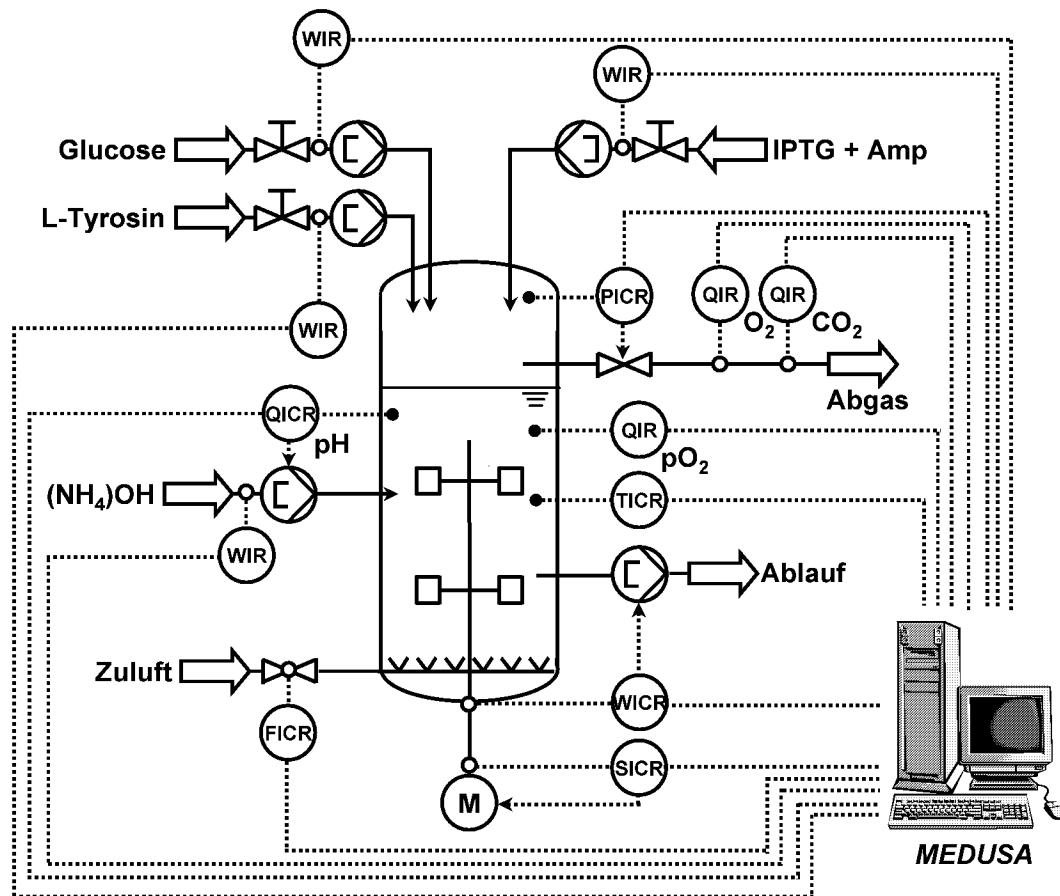
Abbildung 26: Schematischer Aufbau der kontinuierlichen Fermentation im 7,5 l Bioreaktor (Geräteliste in Abschnitt 12.2).
