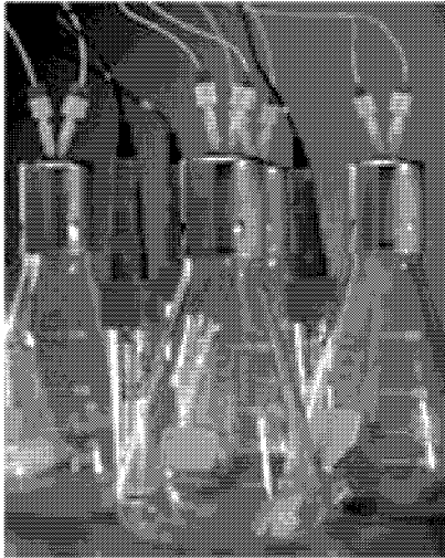
Abbildung 20: Bild eines pH-geregelten Schüttelkolbens im Fed-Batch-Betrieb.
