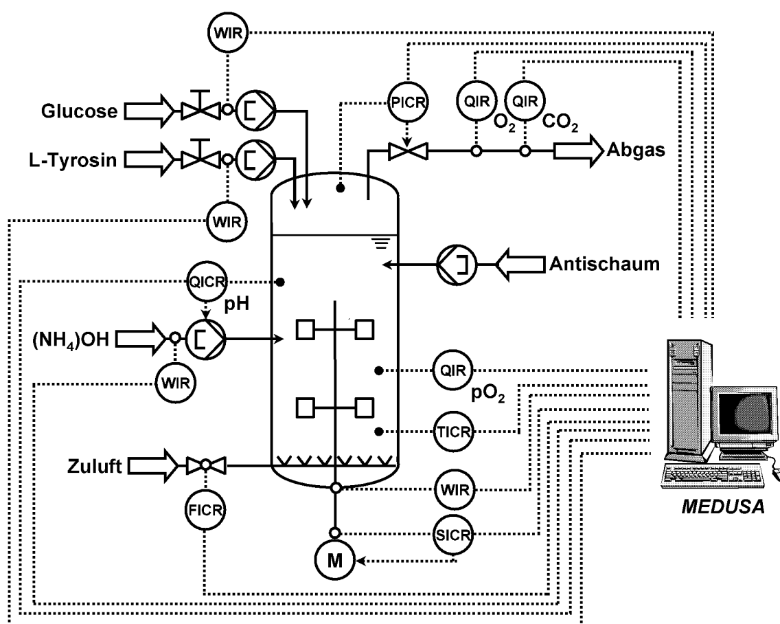
Abbildung 22: Aufbau der 7,5 l Fed-Batch-Fermentation (Geräteliste in Abschnitt 12.2). Der in Abschnitt 5.2.1 detailliert beschriebene Filtrationsumlauf, wurde im Fließbild vernachlässigt. Auf einen vollständigen Prozessaufbau wird in den folgenden Abschnitten zur Apparatechnik von Fermentationen im Zulaufverfahren verzichtet und nur die wesentlichen Elemente dargestellt.
