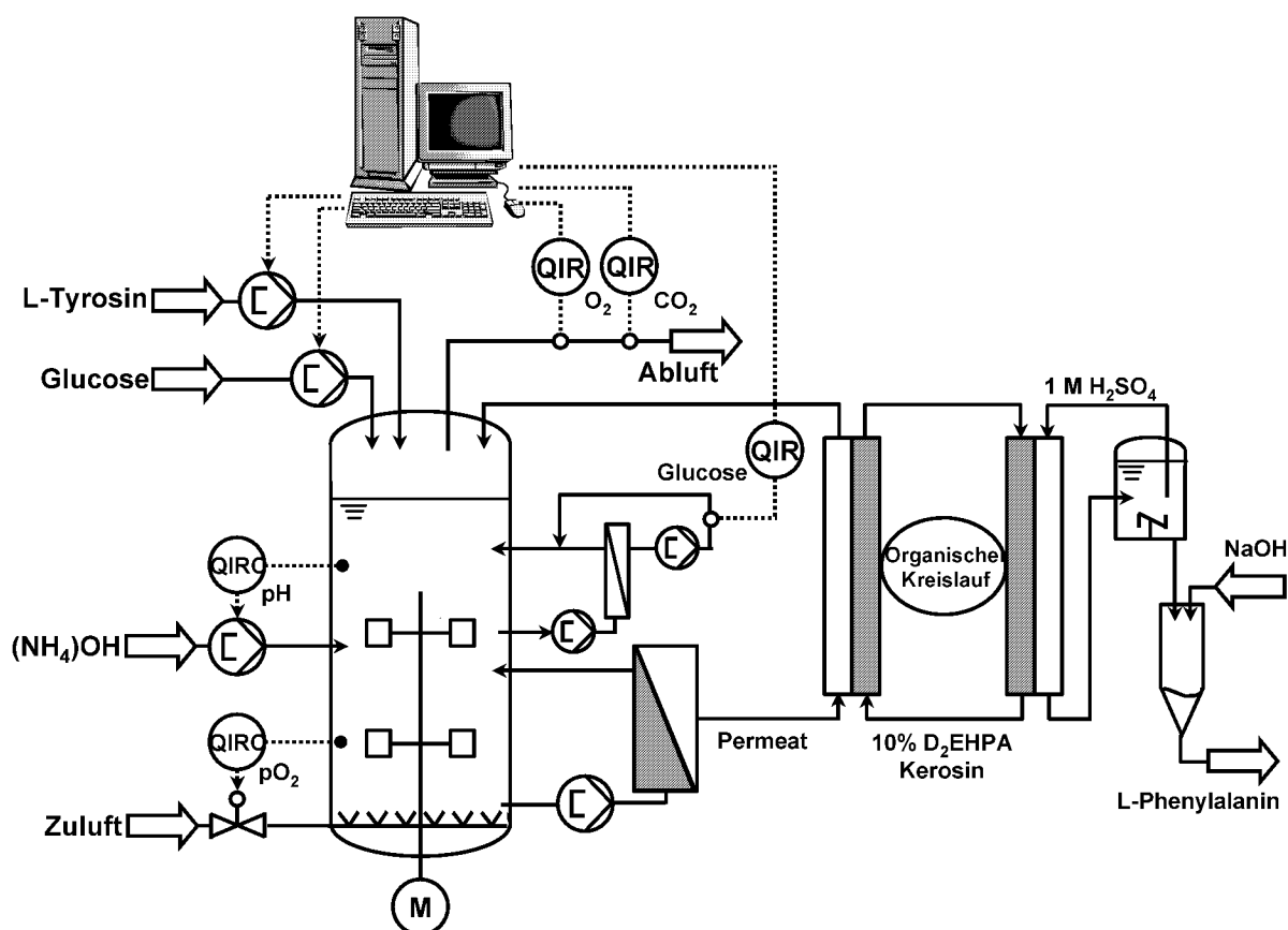
Abbildung 39: Fließbild des Hybridprozesses (Fermentation, Filtration und Reaktiv-Extraktion) (Geräteliste in Abschnitt 12.2).
