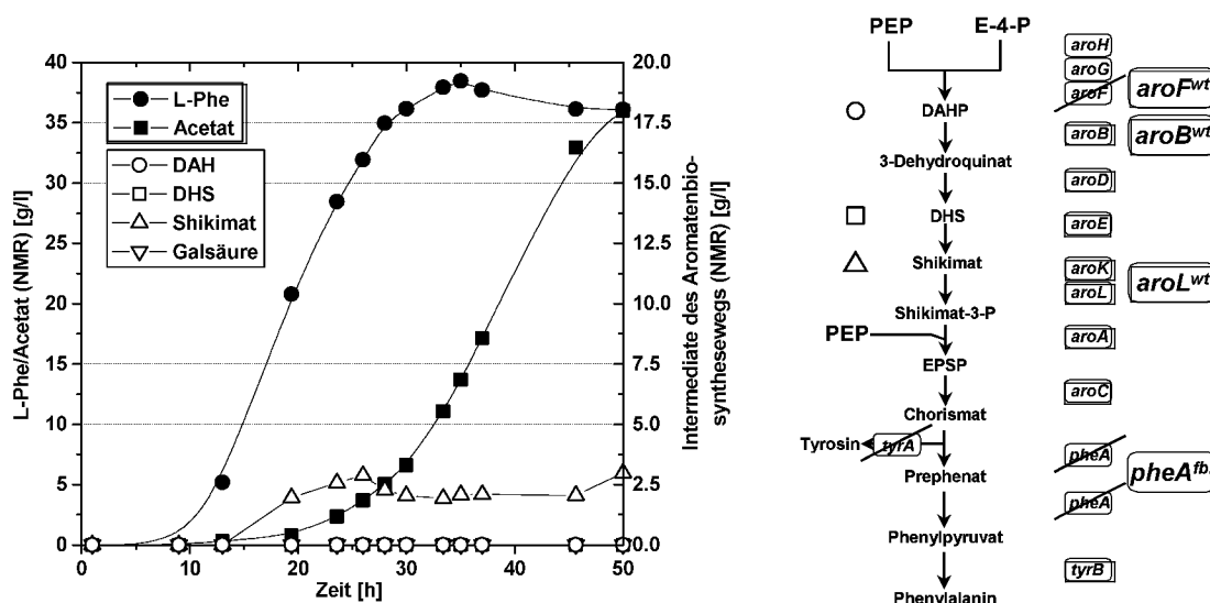
Abbildung 102: Links: Konzentrationsverläufe von L-Phe und Acetat (NMR) sowie der Intermediate der Aromatenbiosynthese (NMR). Rechts: Aromatenbiosynthesebaum mit den kodierenden Genen und Darstellung der gentechnischen Veränderungen ( E. coli 4pF81).
