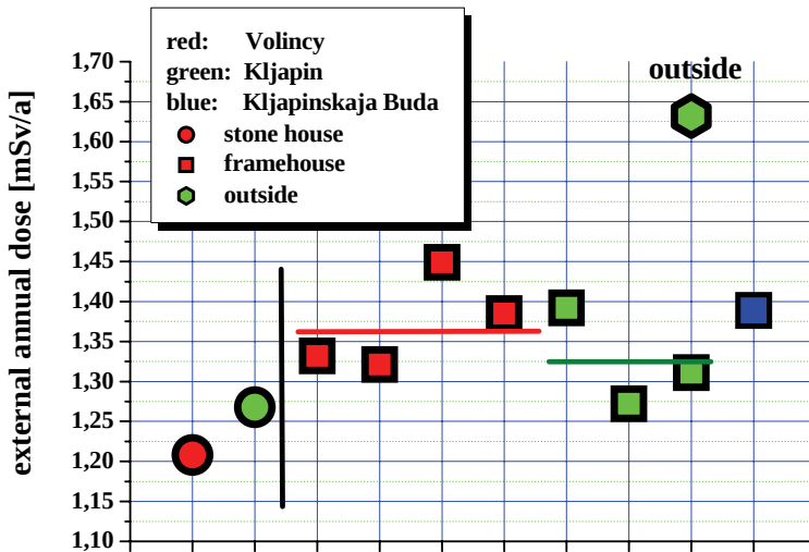
Abbildung 2-6: Externe Jahresdosis 2006-2007 auf Basis von TLD-Messungen
