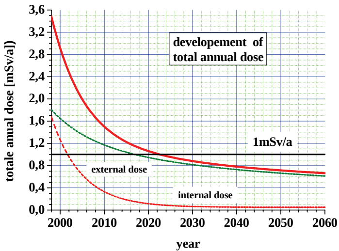
Abbildung 6-6: Abschätzung der Jahresdosis in den fortlaufenden Jahren
