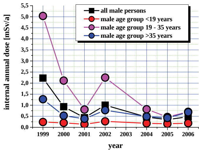
Abbildung 4-7: Entwicklung der internen Jahresdosis der männlichen Bevölkerung in der Gemeinde Volinçy aufgeteilt nach Gesamtzahl und Altersgruppen
