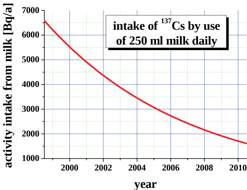
Abbildung 3-2: Jährliche Aktivitätszufuhr ( 137 Cs) bei 0,25l täglichen Milchverzehr
