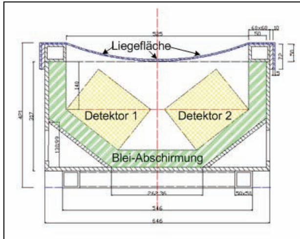
Abbildung 1-6: Schnitt durch den Ganzkörperzähler SM2
