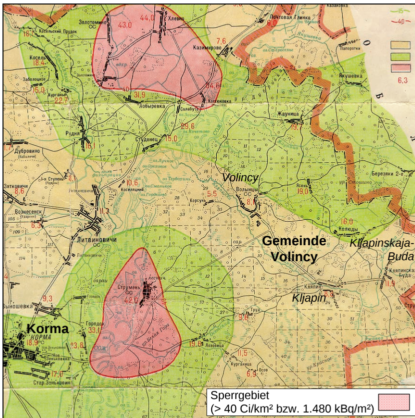
Abbildung 1-4: Die Gemeinde Volincy mit Sperrgebieten (Angaben in \text{Ci/km}^2 ) (Quelle: Комитет геодезии и картографии СССР, Москва, 1991, ergänzt)
