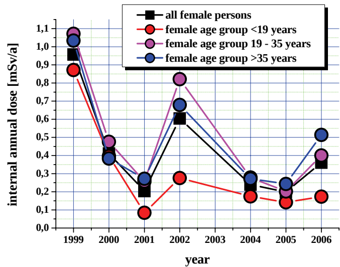
Abbildung 4-8: Entwicklung der internen Jahresdosis der weiblichen Bevölkerung in der Gemeinde Volinçy aufgeteilt nach Gesamtzahl und Altersgruppen
