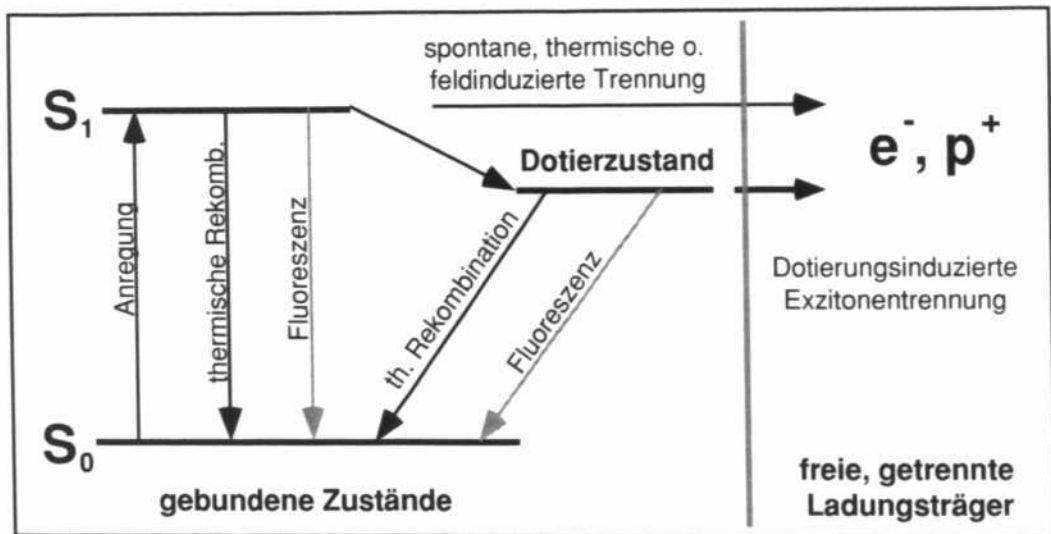
Abbildung 2.6: Exzitonentrennung in H_2 -Pc. Die Generation freier Ladungsträger steht in Konkurrenz zu den Rekombinationsmechanismen. Der Dotierungsunterstützte Prozeß (kleiner, fatter Pfeil) ist wahrscheinlich der bestimmende (s. Text)
