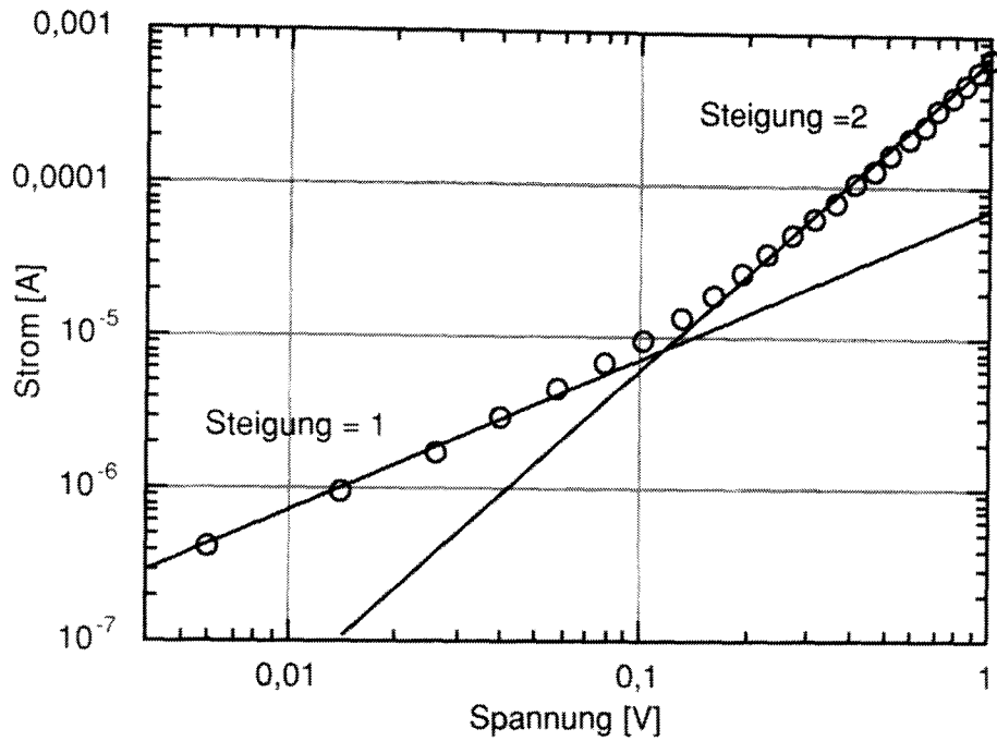
Abbildung 4.7: I/U -Kennlinien einer unbleuchteten undotierten Probe in doppeltlogarithmischer Auftragung. Es ergibt sich Ohm'sches Verhalten für kleine Spannungen und raumladungsbegrenztes Verhalten für höhere Spannungen.
