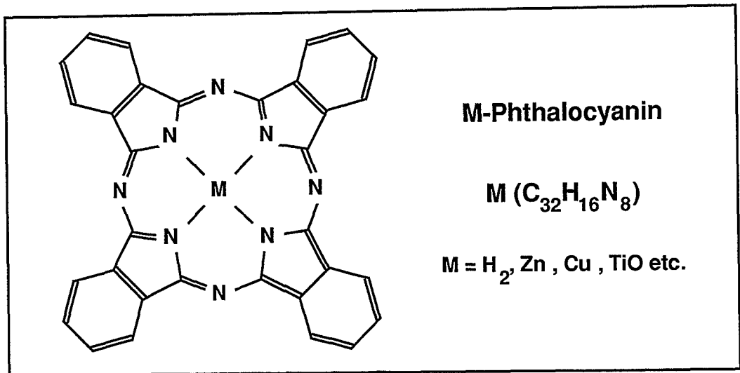
Abbildung 2.1: Struktur von Phthalocyaninen. In der Mitte des Moleküls können diverse Metallatome, Metalloxide oder Wasserstoff sitzen.
