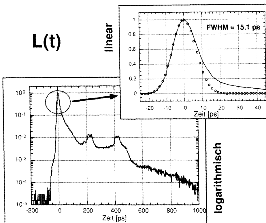
Abbildung 4.11: Zeitauflösung der Fluoreszenzmessung in linearer und logarithmischer Darstellung. Die Kurve zeigt die gemessene Detektionsfunktion L(t) , die Kreise markieren die Anpassung einer Gaußkurve mit der Halbwertsbreite 15 ps. In der unteren halb-logarithmischen Auftragung sieht man Strukturen, die zum großen Teil durch den verwendeten Detektor erzeugt werden.
