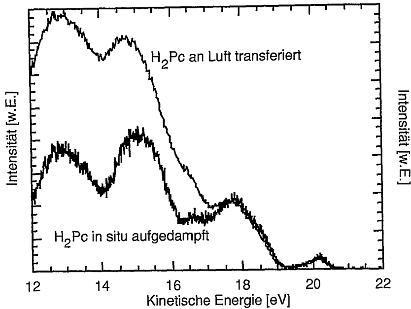
Abbildung 4.20: Die beiden Präparationsmethoden im Vergleich. Die in situ gedampften H 2 -Pc Schichten zeigen einen wesentlich geringeren Untergrund und schärfere Strukturen als die aus der Koverdampfungsanlage transferierten Proben. Zum Vergleich sind die Spektren auf die obersten Valenzbandzustände normiert, der Untergrund macht sich so als ein starker Anstieg zu kleineren kinetischen Energien hin bemerkbar.
