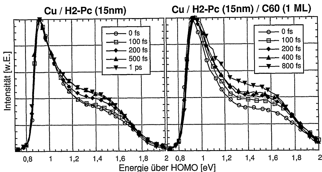
Abbildung 4.17: Zeitentwicklung der niederenergetischen Zustände von H_2\text{-Pc} ohne und mit C_{60} . Die dotierte Schicht zeigt einen zusätzlichen Zustand in der Flanke des Sekundärelektronenhügels, der mit der gleichen Zeitabhängigkeit wie das Singulettexziton bevölkert wird.
