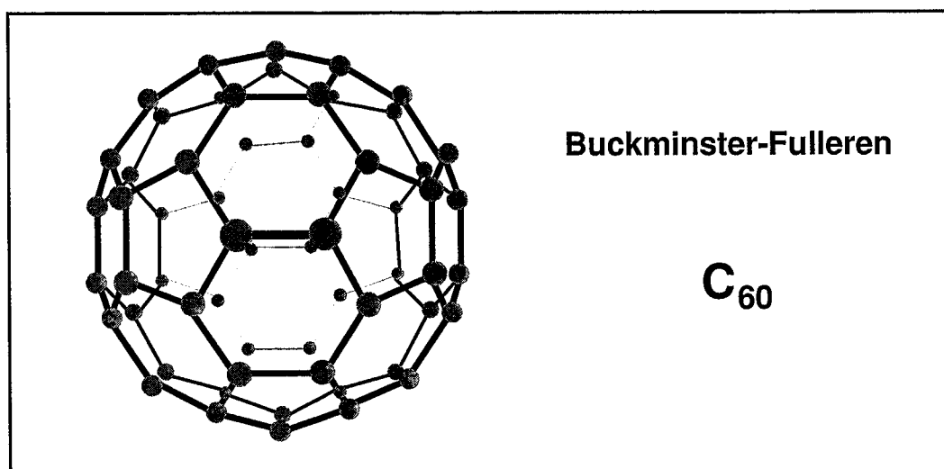
Abbildung 2.4: Das Fulleren C 60
