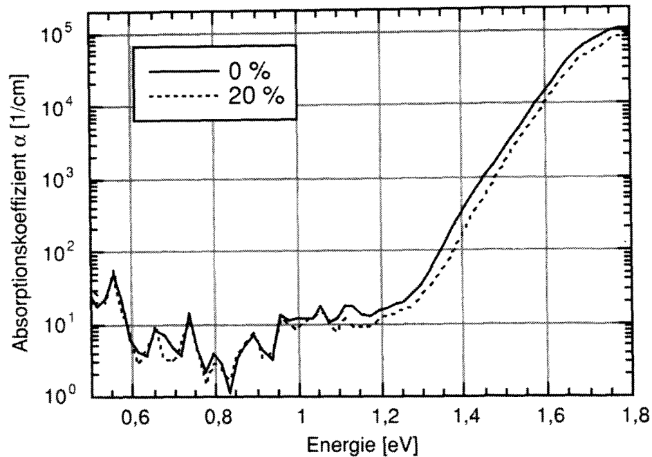
Abbildung 4.3: Absorption einer hochdotierten (20%) H_2 -Pc-Probe. Im infrarot-nahinfraroten Bereich sind keine zusätzlichen Absorptionsbanden zu erkennen. Die Intensität des hochenergetischen Peaks der Q-Bande ist leicht relativ zum niederenergetischen Peak erhöht.
