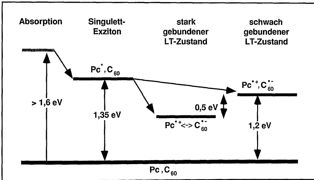
Abbildung 2.12: Energetische Lage der Ladungstransferrniveaus relativ zu Grundzustand und Singulett-Exziton des H_2 -Pc. Der schwach gebundene LT-Zustand liegt etwa 1,2 eV über dem Grundzustand. Der stark gebundene LT-Zustand liegt etwa 0,5 eV unter dem schwach gebundenen LT-Zustand.
