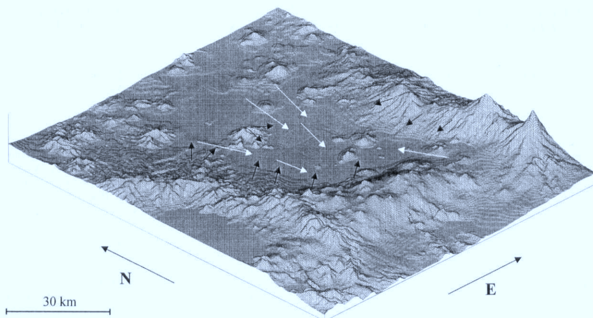
Fig. 1a: 3D-View of the basin of Mexiko. The prevailing winds during the daylight (white) and night hours (black) are shown Dreidimensionale Ansicht des Hochbeckens von Mexiko. Die vorherrschenden Winde während der Tagesstunden (weiß) und der Nachtstunden (schwarz) sind angegeben
