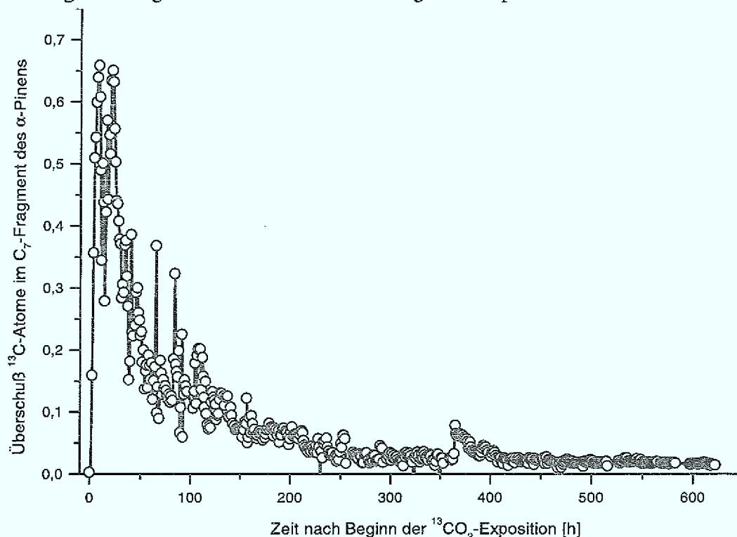
Abbildung 14.7: Markierung des \alpha -Pinens mit ^{13}\text{C} -Atomen über einen Zeitraum von etwa 25 Tagen. Die Exposition mit ^{13}\text{CO}_2 erfolgte im Zeitraum t = 0 - 8 \text{ h} . Die Erhöhung der Markierung zum Zeitpunkt t = 364 \text{ h} ist eine Folge der Verletzung der Pflanze.
