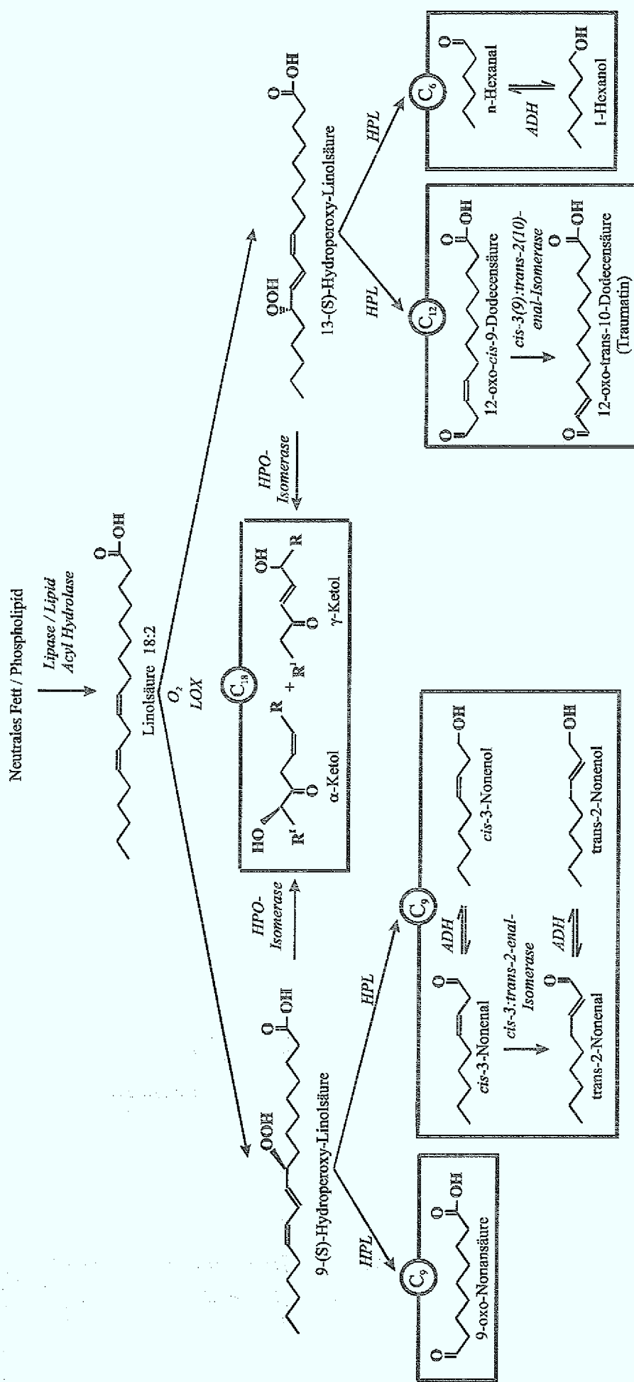
Abbildung 2.9: Schema der Biosynthese einiger oxygenierter Verbindungen aus Linolsäure über den Lipoxygenasezweig (nach HILDEBRAND, 1989; HATANAKA, 1993; GARDNER, 1995).
