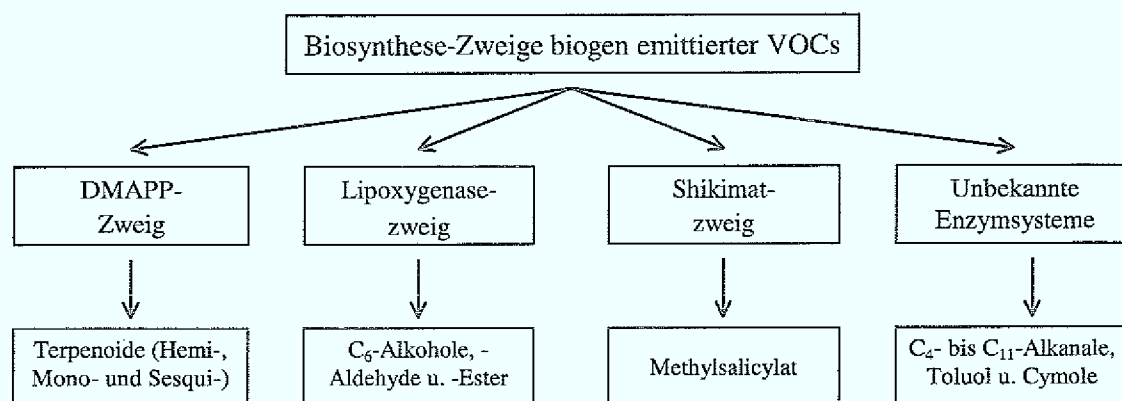
Abbildung 4.1: Übersicht über die in dieser Arbeit untersuchten Substanzklassen biogener Emissionen nach ihren Biosyntheseweigen.
