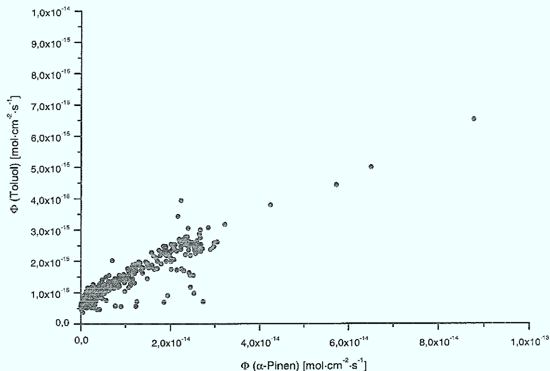
Abbildung 14.3: Auftragung der Emissionsraten des Toluols gegen die des \alpha -Pins.
