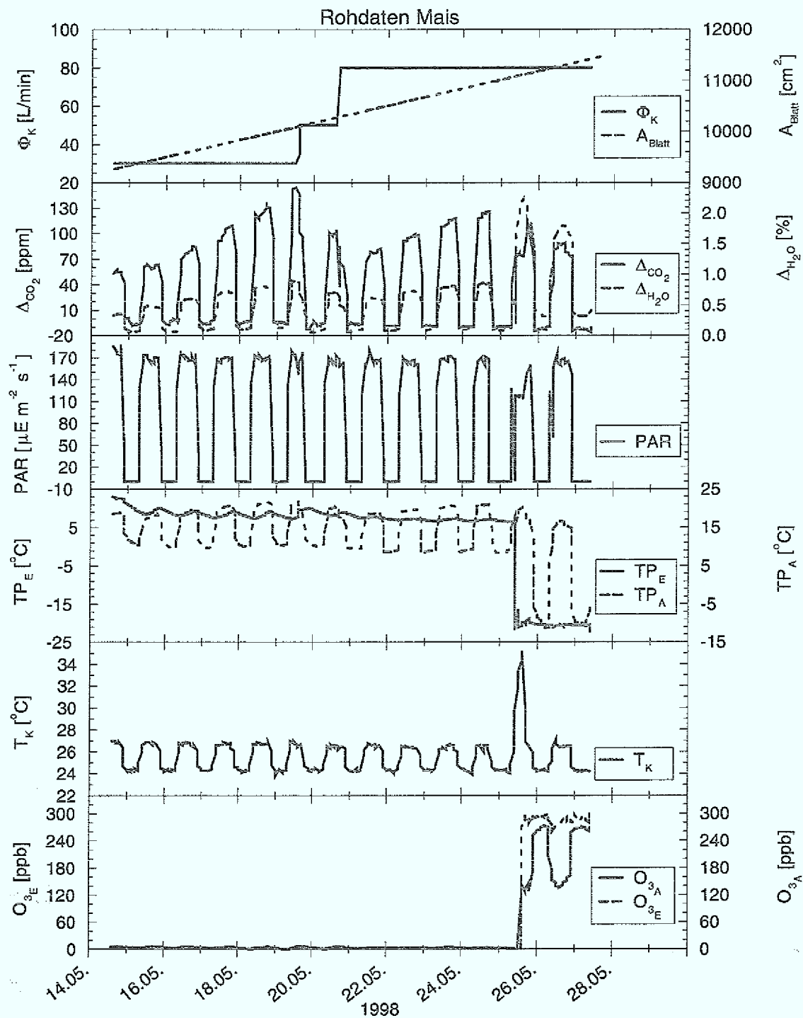
Abbildung 3.9: Beispielhafte Darstellung der Rohdaten für ein Experiment an Mais. Die verwendeten Abkürzungen bezeichnen: \Phi_K = Kammerfluß; A_{\text{Blatt}} = einseitige Blattfläche; \Delta_{\text{CO}_2} und \Delta_{\text{H}_2\text{O}} = CO 2 - bzw. H 2 O-Differenz zw. Eingang (E) und Ausgang (A) der Kammer; PAR = Photosynthetisch aktive Strahlung; TP_E und TP_A = Taupunkt am Eingang und Ausgang der Kammer; T_K = Temperatur der Expositionskammer; O_{3E} und O_{3A} = O 3 -Konzentration am Eingang und Ausgang der Kammer.
