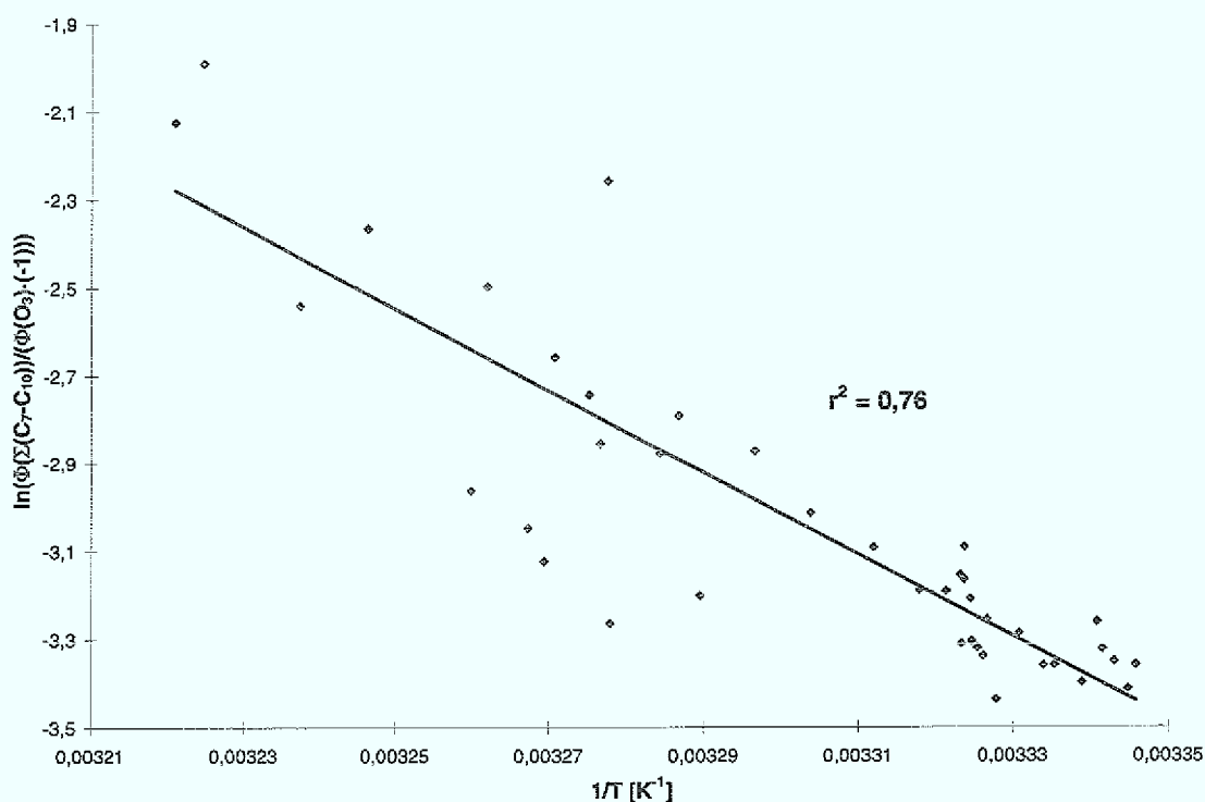
Abbildung 11.10: Logarithmus der Summe der Flußdichten der C_7 - bis C_{10} -Alkanale dividiert durch die Ozonflußdichten als Funktion der inversen Blattemperatur für Experiment R4-OII.
