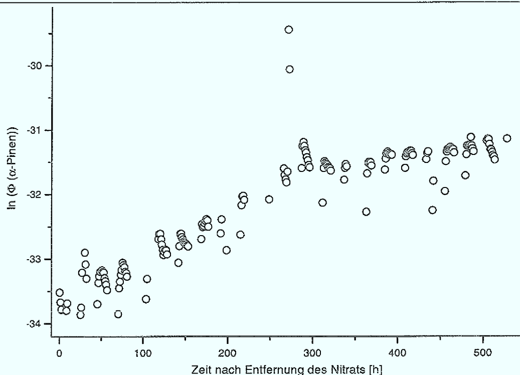
Abbildung 14.4: Auftragung der Logarithmen der Flußdichten des \alpha -Pinen aus einer Sonnenblume unter Stickstoffmangel. Das Nitrat wurde zum Zeitpunkt t = 0 h aus der Nährlösung entfernt und zum Zeitpunkt t = 360 h wieder zugegeben.
