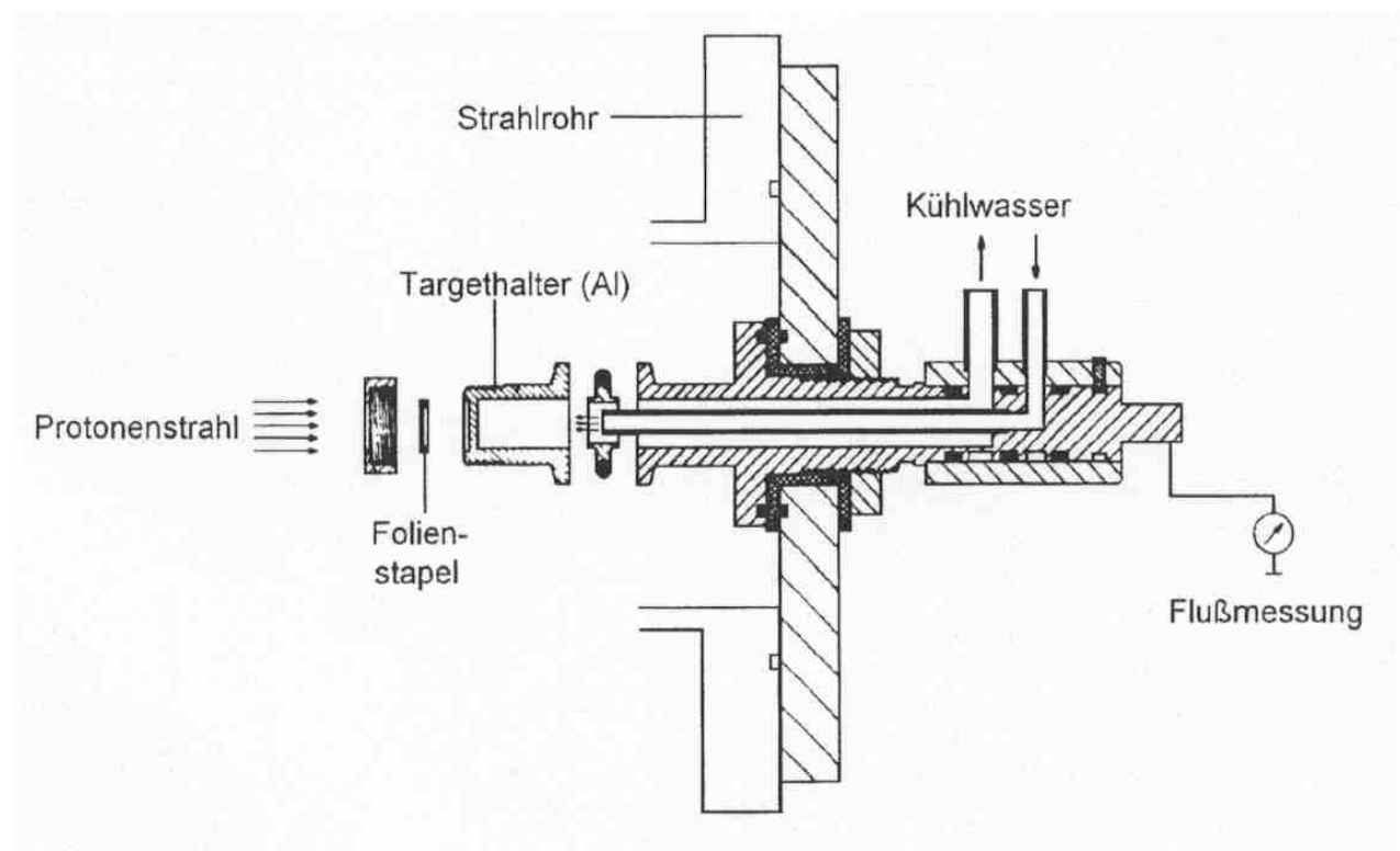
Abbildung 10: Bestrahlungseinrichtung am CV 28 [cf. 42]
