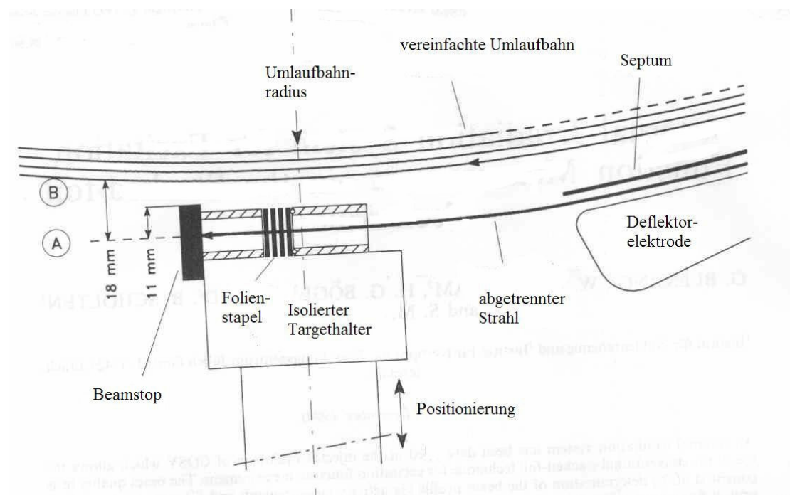
Abbildung 13: Bestrahlungseinrichtung am Injektor des COSY [43]
