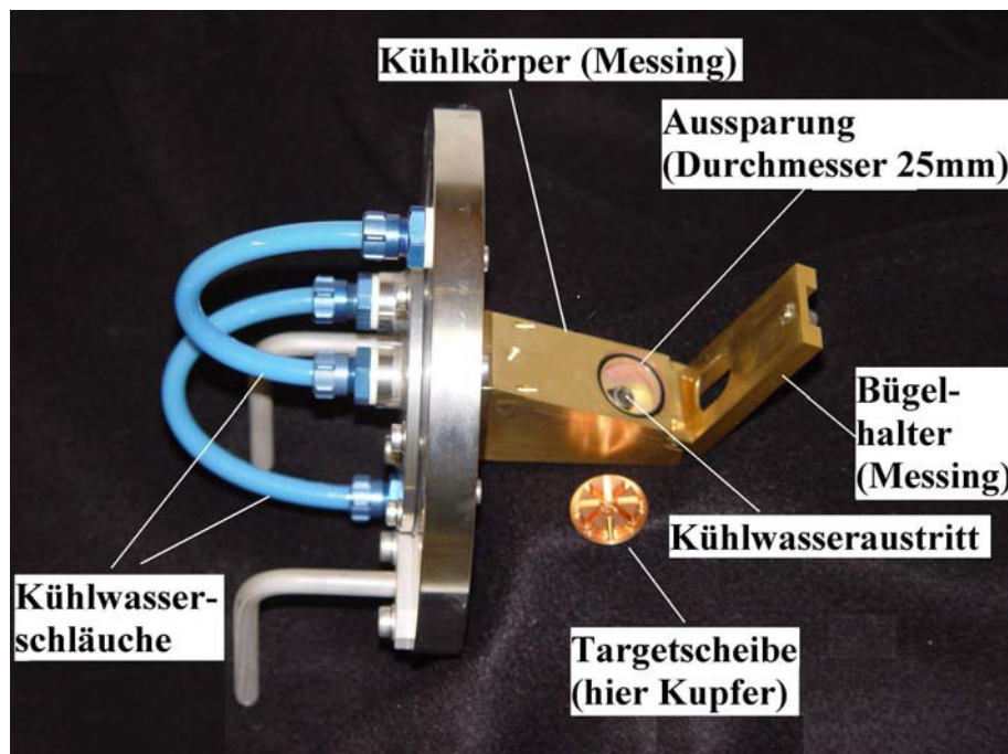
Abbildung 18: Targethalter für die Bestrahlung mit hohen Teilchenströmen
