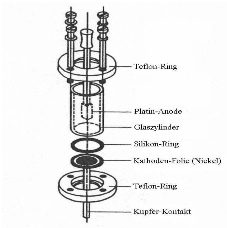
Abbildung 9: Aufbau der Elektrolysezelle nach [41]
