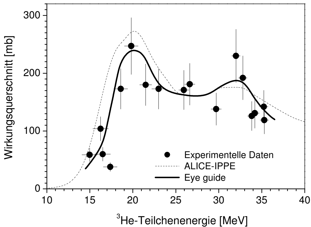
Abbildung 19: Ergebnisse der Experimente und der Rechnungen mit ALICE-IPPE für die ^{\text{nat}}\text{Ce}(^3\text{He},\text{xn})^{141}\text{Nd} Reaktion
