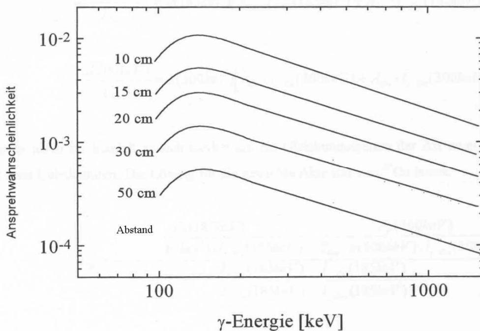
Abbildung 17: Beispiel für den Verlauf der Ansprechwahrscheinlichkeit eines HPGe-Detektors
