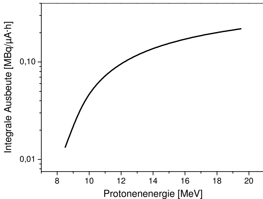
Abbildung 33: Integrale Ausbeute von ^{192}\text{Ir} nach der ^{192}\text{Os}(p,n)^{192}\text{Ir} Reaktion
