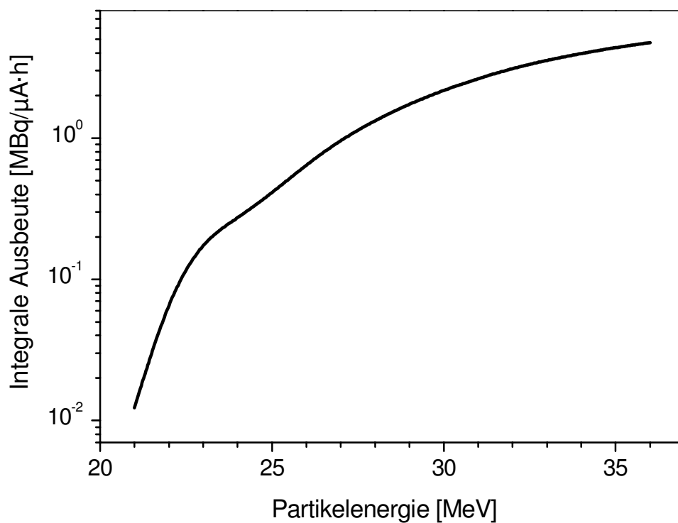
Abbildung 36: Integrale Ausbeute der ^{192}\text{Os}(^3\text{He},4n)^{191}\text{Pt} Reaktion
