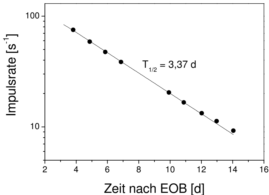
Abbildung 14: Beispiel für eine Zerfallskurve des ^{140}\text{Nd}
