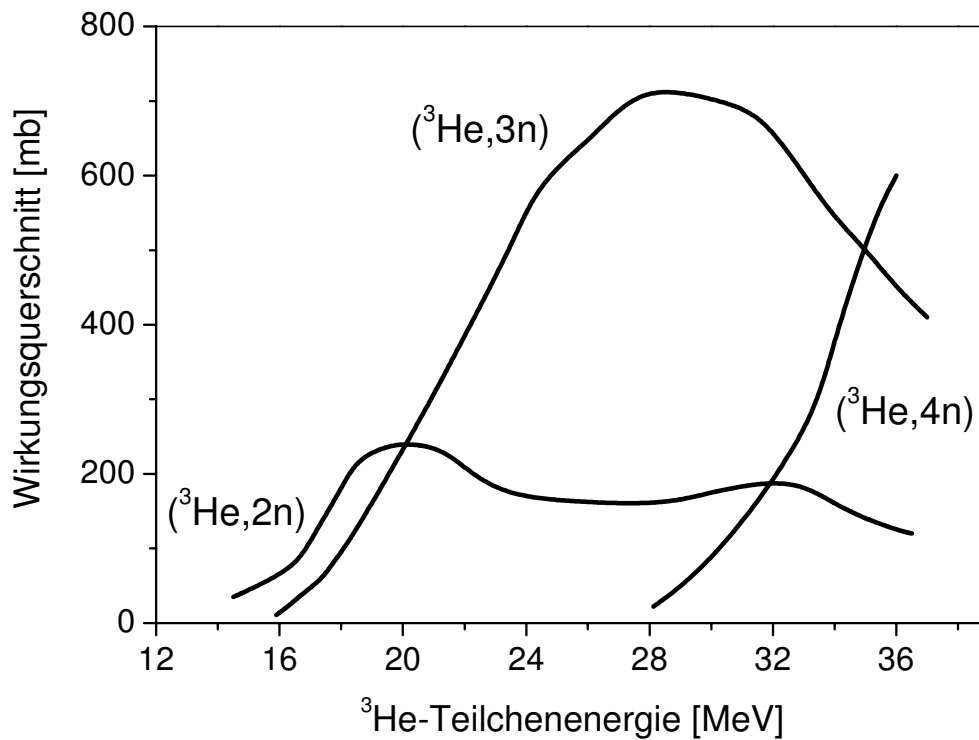
Abbildung 23: Systematik der Anregungsfunktionen der ^{\text{nat}}\text{Ce}(^3\text{He}, xn) -Reaktionen
