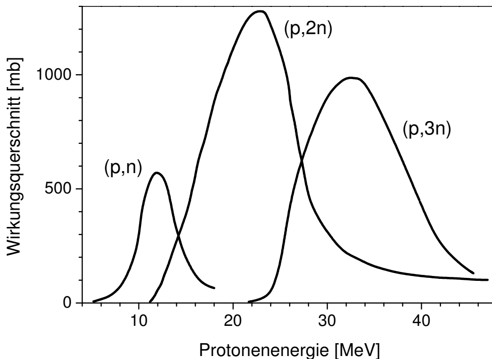
Abbildung 29: Systematik der Anregungsfunktionen der ^{141}\text{Pr}(p,xn) -Reaktionen
