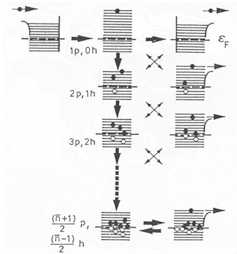
Abbildung 2: Schema des Excitonen-Modells
