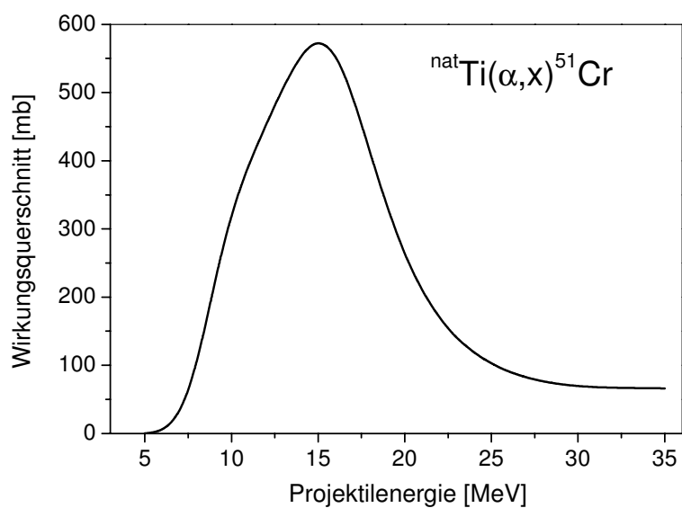
Abbildung 5: Anregungsfunktion der Monitorreaktion {}^{\text{nat}}\text{Ti}(\alpha, x){}^{51}\text{Cr} [cf. 9]
