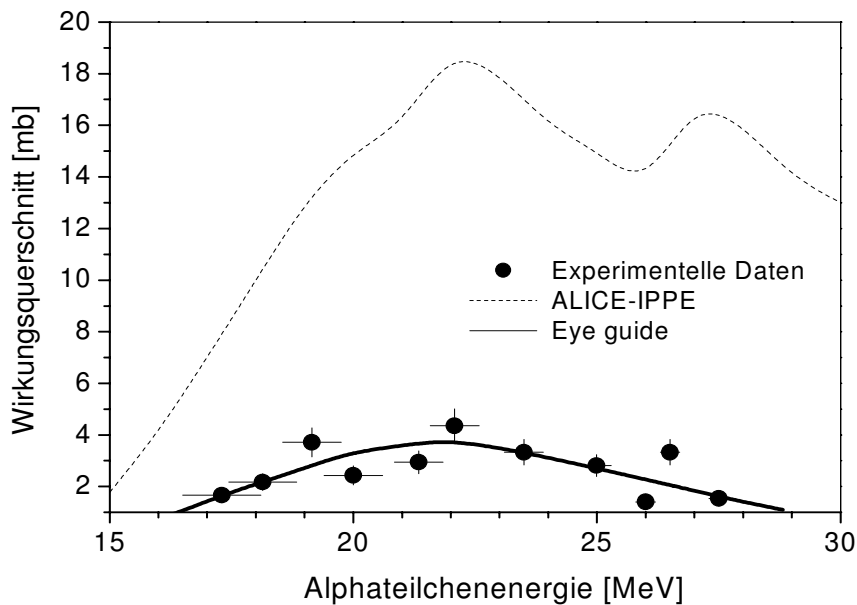
Abbildung 34: Experimentell ermittelte Daten zur ^{192}\text{Os}(\alpha, n)^{195\text{m}}\text{Pt} Reaktion
