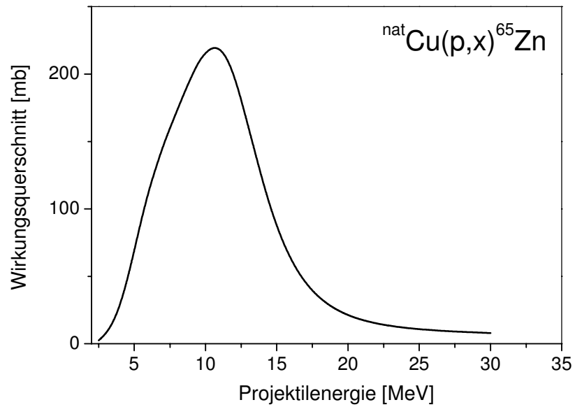
Abbildung 3: Anregungsfunktion der Monitorreaktion {}^{\text{nat}}\text{Cu}(p,x){}^{65}\text{Zn} [cf. 9]
