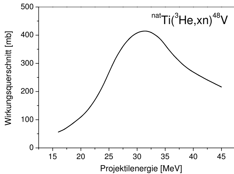
Abbildung 4: Anregungsfunktion der Monitorreaktion {}^{\text{nat}}\text{Ti}({}^3\text{He},x){}^{48}\text{V} [cf. 9]
