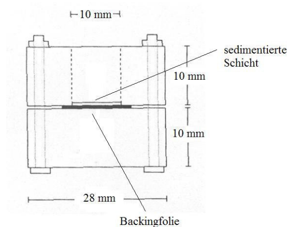
Abbildung 8: Aufbau der Sedimentationszelle nach [37]
