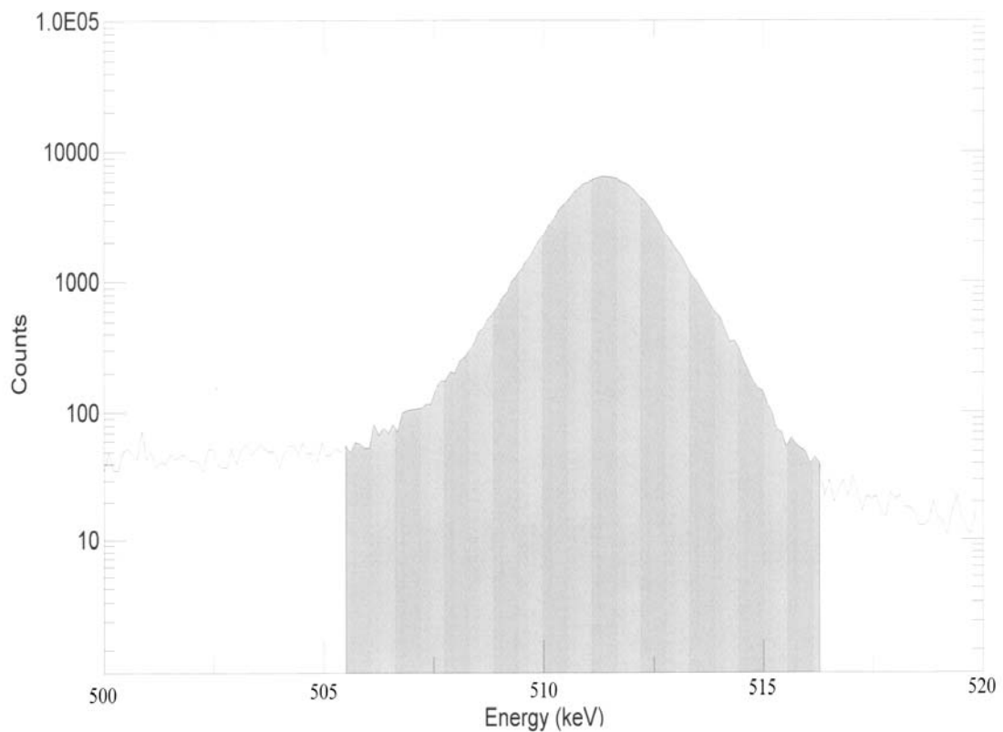
Abbildung 15: Darstellung einer Peakintegration der Vernichtungsstrahlung
