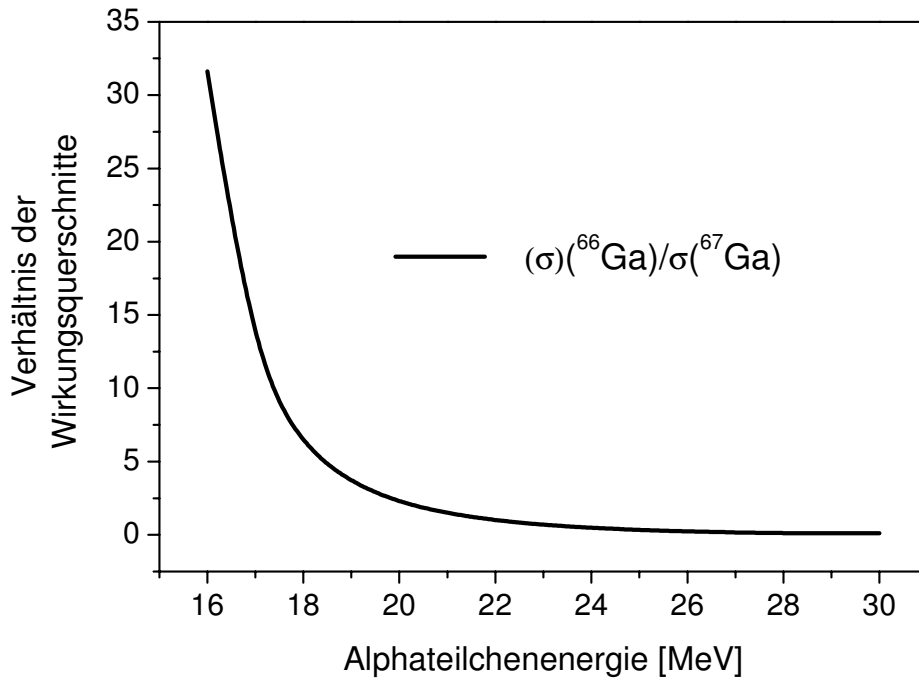
Abbildung 6: Das Verhältnis der Wirkungsquerschnitte der ^{nat}\text{Cu}(\alpha, x)^{66}\text{Ga} und der ^{nat}\text{Cu}(\alpha, x)^{67}\text{Ga} Reaktion
