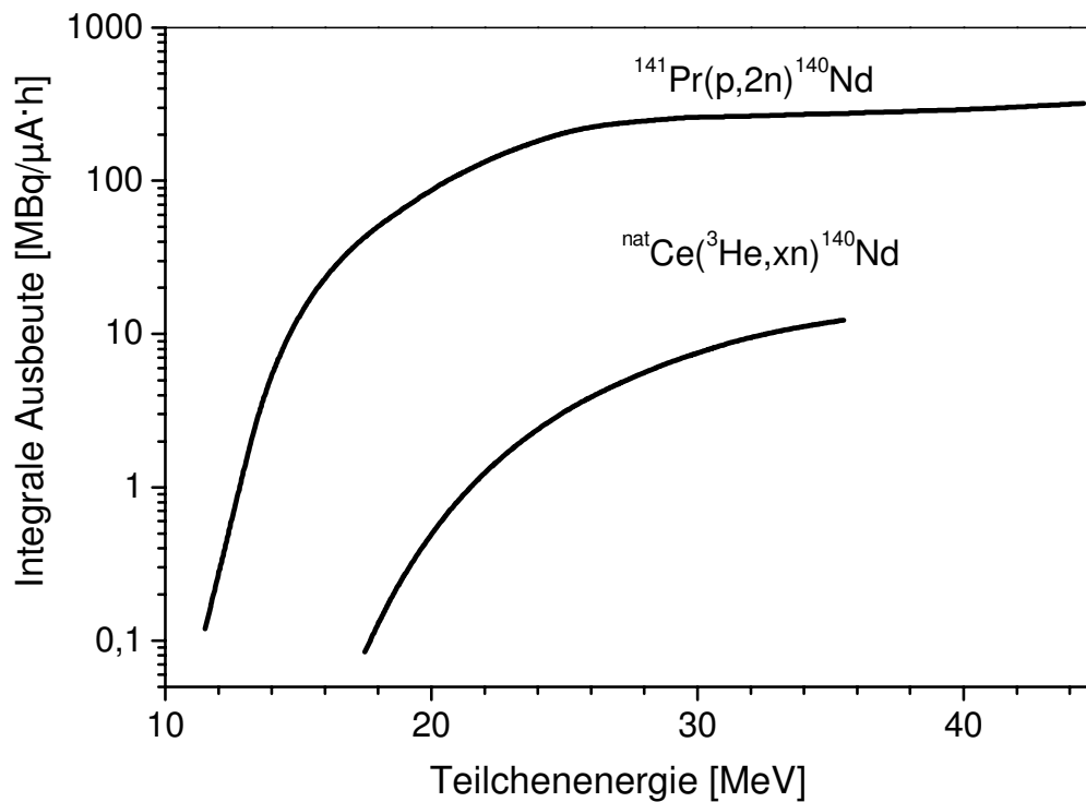
Abbildung 31: Vergleich der integralen Ausbeute von ^{140}\text{Nd} aus den ^{nat}\text{Ce}(^3\text{He},\text{xn})^{140}\text{Nd} - und ^{141}\text{Pr}(\text{p},2\text{n})^{140}\text{Nd} -Reaktionen
