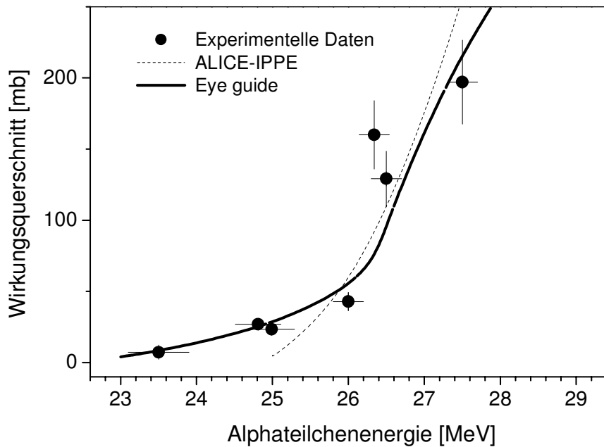
Abbildung 35: Experimentell ermittelte Daten zur ^{192}\text{Os}(\alpha, 3n)^{193\text{m}}\text{Pt} Reaktion.
