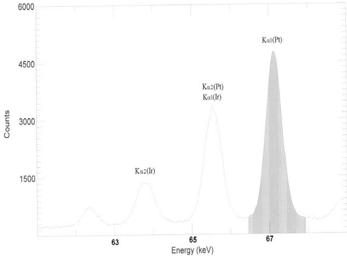
Abbildung 16: Darstellung einer Peakintegration für Röntgenlinien
