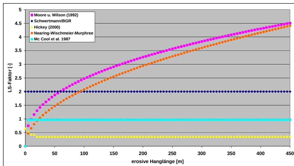
Abb. 20: LS-Faktor bei einer definierten Hangneigung von 5° in Abhängigkeit der erosiven Hanglänge, berechnet nach fünf verschiedenen Algorithmen
