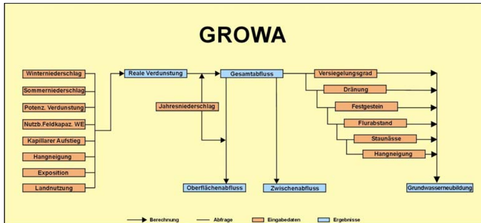
Abb. 6: Schematische Darstellung des Wasserhaushaltsmodells GROWA bei der Berechnung der Wasserhaushaltskomponenten
