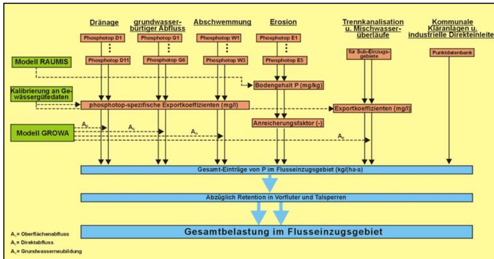
Abb. 5: Schematische Darstellung der Modellierung des mehrjährigen mittleren P-Eintrags mit MEPhos
