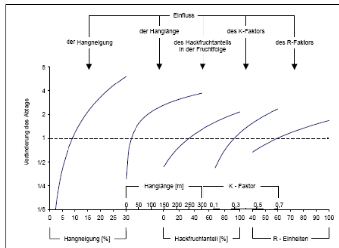
Abb. 15: Sensitivität des Bodenabtrags auf Veränderung der Faktoren relativ zum bayerischen Standardfall (9 % Neigung; 22,1 m Hanglänge; 33 % Hackfruchtanteil; K-Faktor 0,3; R-Faktor 70 (AUERSWALD 1987))
