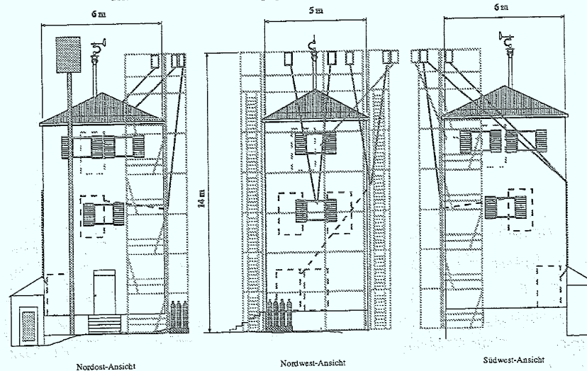
Abbildung 7.3-2: Seitenansichten der TOR Station Schaulinsland während der PRICE Kampagne im August 94. Die kleinen Rechtecke auf dem Gerüst stellen die Einlaßsysteme der verschiedenen chemischen Verstärker dar, die Linien die Gas- und Stromversorgung der Einlaßsysteme. Gestrichelte Linien stehen für Leitungen im oder hinter dem Gebäude. Die Abbildung stammt aus dem Bericht zur PRICE Kampagne (Volz-Thomas et al., 1997)
