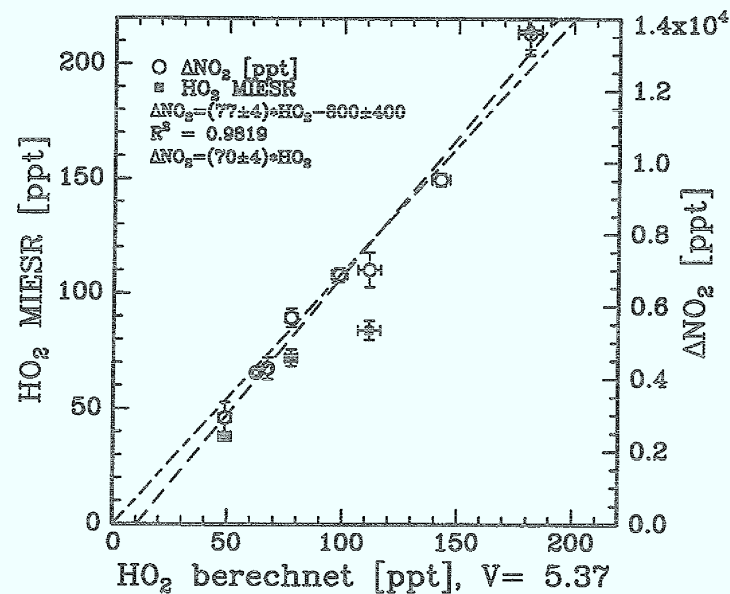
Abbildung 7.2-3: Ergebnis der Messungen des in dieser Arbeit verwendeten chemischen Verstärkers an der HO_2 Quelle. Aus der Steigung der durch den Ursprung gelegten Geraden wurde ein mittlerer Verstärkungsfaktor von 70 \pm 4 bestimmt. Zum Vergleich sind die entsprechenden Meßwerte der MIESR gezeigt.
