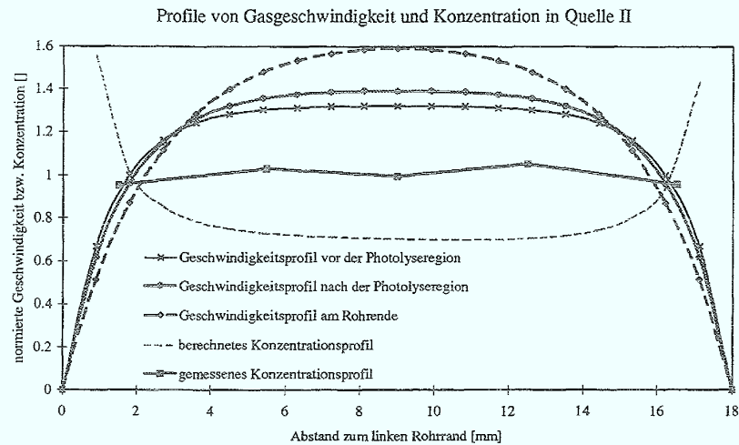
Abbildung 5.2-2: Berechnetes Geschwindigkeitsprofil im Strömungsrohr von Quelle II (nach Langhaar, 1942), sowie das daraus berechnete Konzentrationsprofil von O_3 und HO_2 (normiert auf die mittlere Konzentration). Zur Berechnung des Konzentrationsprofils wurde eine homogene Strahlungsverteilung angenommen. Die Abnahme der Strahlungsintensität mit zunehmendem Abstand zur Lampe aufgrund der optischen Dichte von 0.1 wurde berücksichtigt. Zum Vergleich ist auch das im Abstand von 1 cm zur Photolyseregion quer über den Rohrquerschnitt gemessene (normierte) Konzentrationsprofil von O_3 eingezeichnet.
