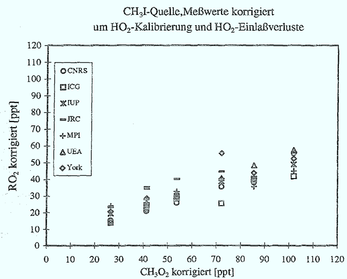
Abbildung 7.2-5: Messungen an der CH 3 I-Quelle, korrigiert auf die Messung an der HO 2 Quelle (oberes Bild) sowie zusätzlich auf die unterschiedlichen Einlaßverluste für HO 2 und CH 3 O 2 (unteres Bild).
