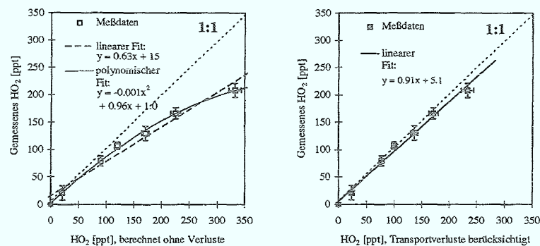
Abbildung 5.1-3: Ergebnis der Vergleichsmessung mit MIESR an Quelle I. Im linken Bild sind die Messungen der MIESR aufgetragen gegen die aus den gemessenen Konzentrationen von \text{H}_2\text{O} und \text{O}_3 berechneten \text{HO}_2 -Konzentrationen. Zur Berechnung wurde ein Verhältnis von \sigma\text{H}_2\text{O} zu \sigma\text{O}_2 von V=5.95 verwendet. Im rechten Bild wurden die theoretischen Werte mit Hilfe eines numerischen Modells berechnet, das die Radikalverluste zwischen der Photolyseregion und der Messung berücksichtigt (s. Text).
