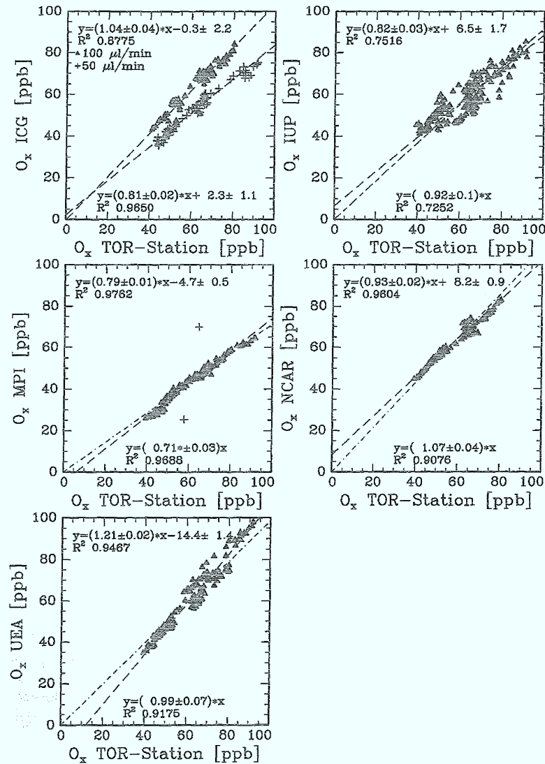
Abbildung 8.1-3: Vergleich der O_2 -Konzentrationen der chemischen Verstärker mit der von der TOR-Station gemessenen O_2 -Konzentration. Dargestellt sind alle 30-Minuten-Mittelwerte der 5 Meßtage. Eingezeichnet sind Regressionsgeraden mit gleicher Gewichtung der Achsen sowie zusätzlich eine Regression durch den Ursprung. Die Daten von ICG wurden getrennt für unterschiedliche Luminolflüsse behandelt. Kreuze kennzeichnen den niedrigen Luminolfluß, Dreiecke den hohen Luminolfluß. Aus Gründen der Übersichtlichkeit sind hier die Regressionen durch den Ursprung nicht gezeigt. Die mit Kreuzen gekennzeichneten Werte bei MPI sind Ausreißer, sie wurden zur Berechnung der Regressionsgeraden nicht berücksichtigt.
