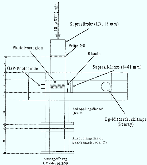
Abbildung 5.2-1: Aufsicht auf das neu entwickelte Strömungsrohr sowie das Lampengehäuse ("Quelle II"). Die Maßangaben sind in mm.
