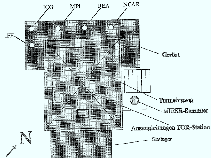
Abbildung 7.3-1: Aufsicht auf die TOR-Station Schaulinsland während der PRICE-Kampagne. Die Einlaßsysteme der verschiedenen chemischen Verstärker befanden sich an den mit Kreisen gekennzeichneten Stellen in etwa 15 Meter über dem Erdboden. Die Abbildung stammt aus dem Bericht zur PRICE Kampagne (Volz-Thomas et al., 1997)
