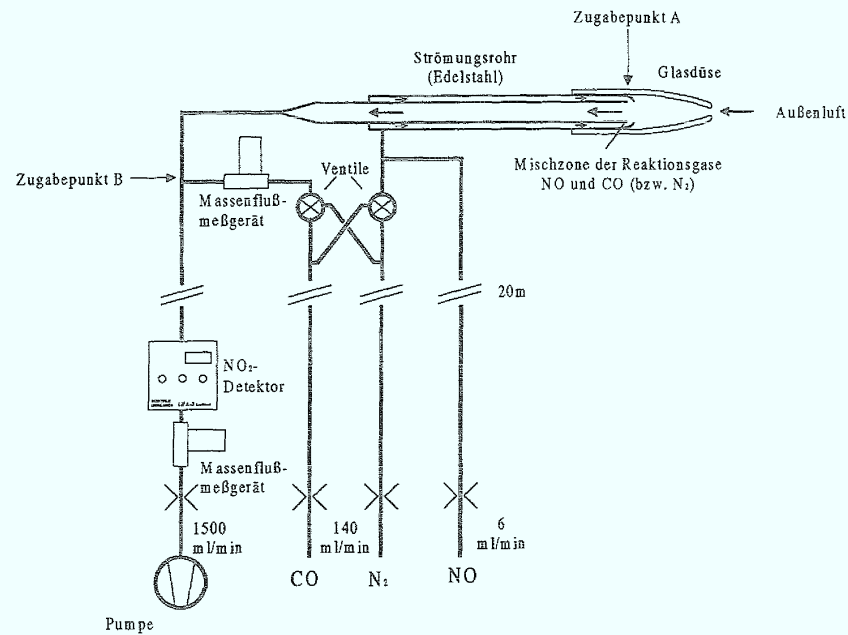
Abbildung 4.2-3: Aufbau des Chemischen Verstärkers
