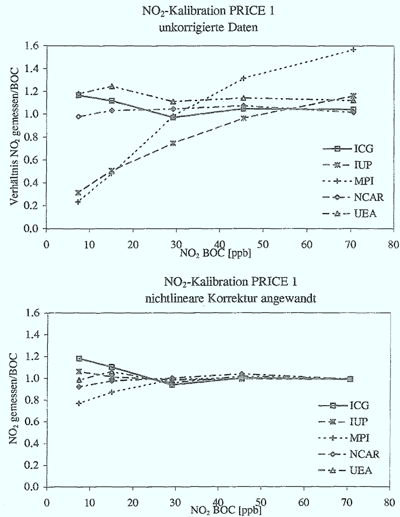
Abbildung 7.1-1: Ergebnisse der während PRICE 1 durchgeführten NO 2 -Kalibration. Dargestellt ist das Verhältnis der gemessenen zur vorgegebenen NO 2 -Konzentration als Funktion der NO 2 -Konzentration. Die vorgegebene Konzentration wurde mittels dynamischer Verdünnung eines NO 2 -Standards (BOC 81667, 8.1 ppm NO 2 in synthetischer Luft) mit synthetischer Luft hergestellt und mit einem Chemolumineszenzdetektor überprüft, der wiederum mittels Gasphasenitration eines NO-Standards kalibriert wurde. Das obere Bild zeigt die Daten mit der Auswertung der einzelnen Gruppen, das untere Bild zeigt die Daten nach Anwendung der in Kapitel 4 beschriebenen nichtlinearen Korrekturfunktion auf die Rohdaten.
