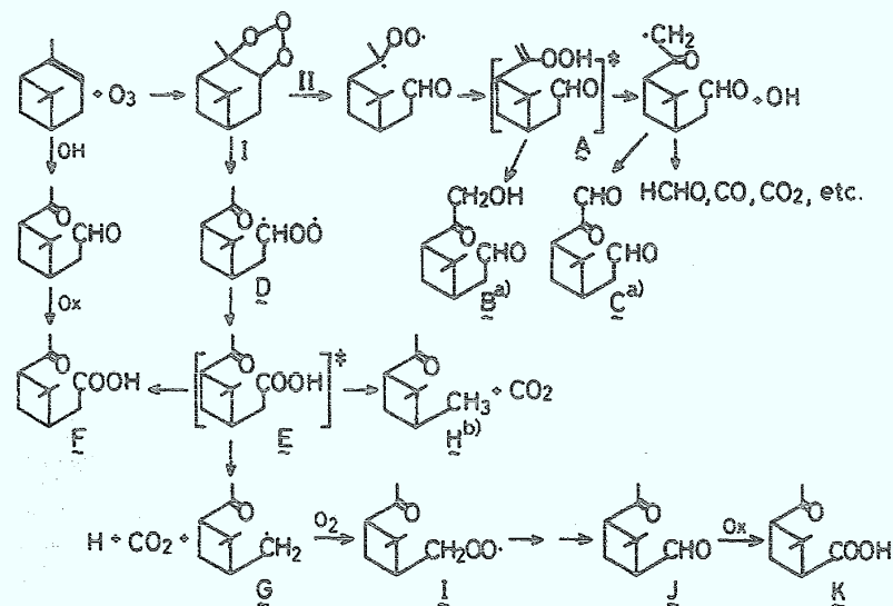
Abbildung 2.2-3: Von Hatakeyama et al. , 1989 vorgeschlagenes Schema der Ozonolyse von \alpha -Pinen. Die Abbildung stammt aus der Originalveröffentlichung. Die mit a) gekennzeichneten Produkte wurden von Hull, 1981 gefunden, die mit b) gekennzeichneten von Yokouchi und Ambe, 1985. Von Hatakeyama et al. , 1989 wurden die Produkte B, C, und H nicht beobachtet.
