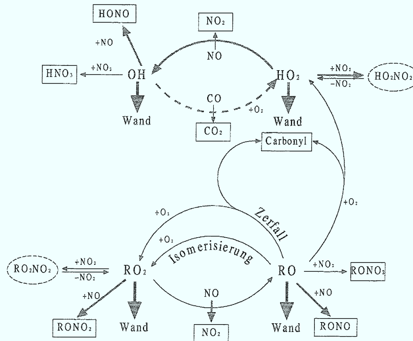
Abbildung 4.1-2: Umwandlungsreaktionen organischer \text{RO}_2 im chemischen Verstärker.
