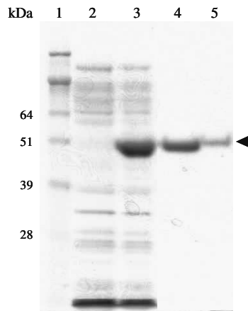
Abb. 20: Aufreinigung von RamB, das durch den Pfeil markiert ist. In Spur 1 befindet sich der Proteinstandard Seebue II prestained Standard (Invitrogen, Karlsruhe). In Spur 2 ist der Zellaufschluss vor der Induktion mit IPTG zu sehen. In Spur 3 ist überexprimiertes RamB 4 h nach Induktion mit IPTG zu sehen. In Spur 4 sieht man aufgereinigtes RamB nach Elution mit Imidazol von einer Nickelchelataffinitätssäule und in Spur 5 aufgereinigtes RamB nach Umpuffern in den BS-Puffer. Die Proteine wurden auf einem 10% SDS-Polyacrylamidgel aufgetrennt und mit Coomassieblau gefärbt.
