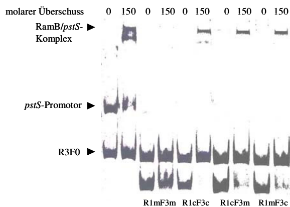
Abb. 24: Gelretardierungstests mit RamB und dem pstS -Promotor. Das Gel zeigt die Bindung von aufgereinigtem RamB (150-facher molarer Überschuss) an den pstS -Promotor (15 nM, 507 bp Fragment) und an die Fragmente R1mF3m (61 nM, 124 bp Fragment), R1cF3m, R1mF3c und R1cF3c.
