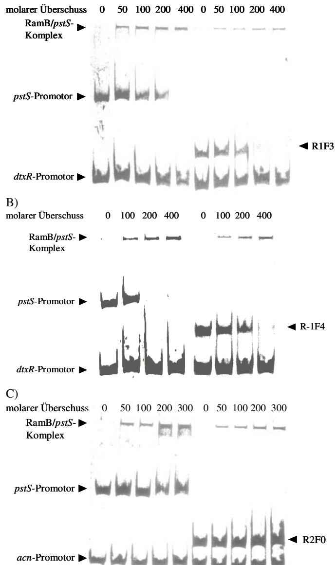
Abb. 23: Gelretardierungstests mit RamB und dem pstS -Promotor. A) Das Gel zeigt die Bindung von aufgereinigtem RamB (50 – 400-facher molarer Überschuss) an den pstS -Promotor (15 nM, 507 bp Fragment) und an das Fragment R1F3 (35 nM, 213 bp Fragment). B) Das Gel zeigt die Bindung von aufgereinigtem RamB (100 – 400-facher molarer Überschuss) an den pstS -Promotor (15 nM, 507 bp Fragment) und an das Fragment R-1F4 (33 nM, 230 bp Fragment). C) Das Gel zeigt die Bindung von aufgereinigtem RamB (50 – 300-facher molarer Überschuss) an den pstS -Promotor (15 nM, 507 bp Fragment) und an das Fragment R2F0 (21 nM, 324 bp Fragment). Das 122 bp lange dtxR -Promotorfragment (62 nM) und das 101 bp lange acn -Promotorfragment (50 nM) diente als Negativkontrolle.
