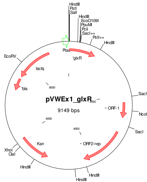
Abb. 48: Plasmidkarte pVWEx1_glxR zur homologen Überexpression des Transkriptionsregulators GlxR.
