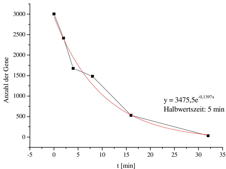
Abb. 29: Bestimmung der durchschnittlichen mRNA-Stabilität der Gene des C. glutamicum Genoms. Aufgetragen wurde die Anzahl in den Hybridisierungsexperimenten nachweisbaren Transkripte gegen die Zeit nach Zugabe von 0,25 g/l Rifampicin. Die mRNA aller Gene zeigt eine durchschnittlichen Halbwertszeit von 5 min.
