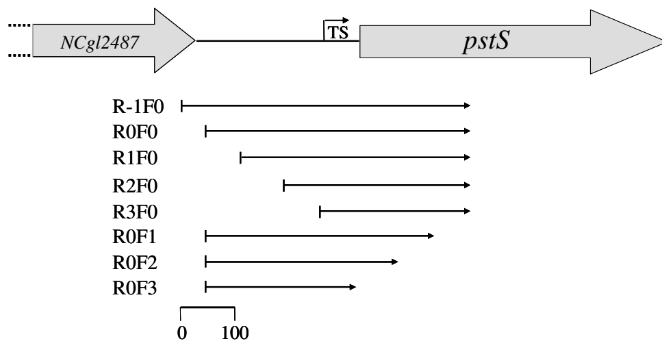
Abb. 6: Übersicht über die pstS -Promotorregion im Genom von C. glutamicum und die für die Deletionsanalyse des pstS -Promotors benutzten Teilfragmente. Der Transkriptionsstart ist als TS angezeigt.
