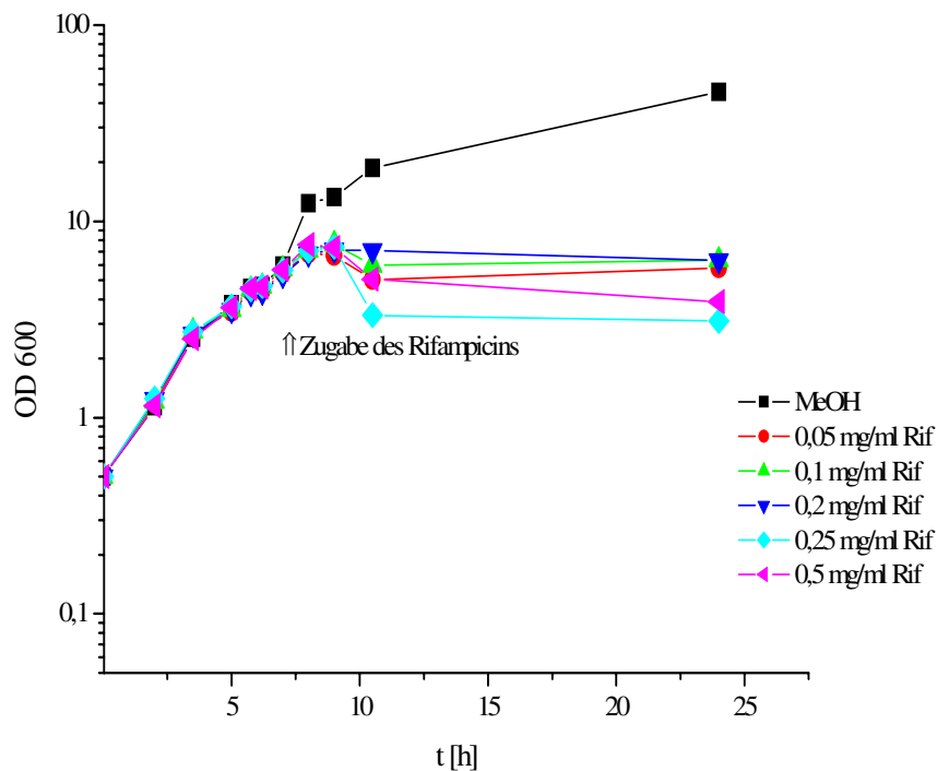
Abb. 28: Anzucht von C. glutamicum WT in CGXII-Minimalmedium mit 40 g/l Glucose, ausreichender Phosphatkonzentration und verschiedenen Rifampicinkonzentrationen, um die geeignete Rifampicinkonzentration zu ermitteln, die die Transkription in C. glutamicum inhibiert. Die Zugabe des Rifampicins (Rif) erfolgte bei einer OD 600 von 4 nach 5 h und 45 min. Rifampicin ist in Methanol (MeOH) löslich. Aus diesem Grund wurde eine Kultur mit dem entsprechenden Lösungsvolumen Methanol kultiviert. Diese zeigte ein normales Wachstum. Anhand dieses Wachstumsexperimentes wurden 0,25 g/l Rifampicin für die mRNA-Abbauxperimente gewählt.
