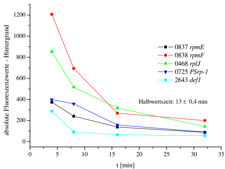
Abb. 30: Stabilität der mRNA ribosomaler Proteine. Die mRNA dieser Gene ist mit einer durchschnittlichen Halbwertszeit von 13 \pm 0,4 min sehr stabil. In der Legende sind die NCgl-Nummern der entsprechenden Gene und die Gennamen angegeben.
