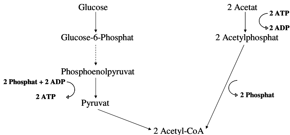
Abb. 36: Umsetzung von Phosphat in der Glycolyse, der oxidativen Decarboxylierung und der Acetataktivierung bei Wachstum von C. glutamicum auf Glucose bzw. Acetat.
