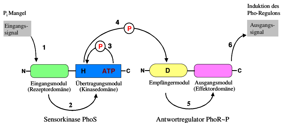
Abb. 3: Modell der Signalübertragung im Zweikomponentensystem PhoRS in C. glutamicum . Phosphatmangel ist das direkte oder indirekte Eingangssignal, das von der Rezeptordomäne der Sensorkinase PhoS dedektiert wird (1). Dadurch verändert sich die Konformation der Rezeptordomäne und das Signal wird auf die Kinasedomäne übertragen (2). Diese autophosphoryliert einen konservierten His-Rest (H) (3) und transferriert die energiereiche Phosphatgruppe an den konservierten Asp-Rest (D) des Empfängermoduls des Antwortregulators PhoR (4). Durch Konformationsänderung im Empfängermodul von PhoR gelangt das Signal ins Ausgangsmodul (5). PhoR~P ist auf diese Weise aktiviert und induziert die Gene des Pho-Regulons (6).
