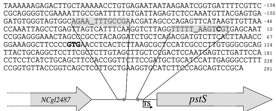
Abb. 19: Identifizierung von zwei RamB-Bindemotiven im pstS -Promotor. Das Bindemotiv A befindet sich von -74 bis -88, während das Bindemotiv B von -9 bis +4 relativ zum Transkriptionsstart (Kocan et al. 2006) zu finden ist (TS). Das Bindemotiv A zeigt eine direkte Übereinstimmung in 10 von 13 bp (grau markiert) ausgehend vom hochkonservierten 13 bp Motiv (Gerstmeir et al. 2004). Das Bindemotiv B zeigt die Übereinstimmung in entgegengesetzter Richtung in 8 (grau markiert) von 13 bp (Gerstmeir et al. 2004). Die Pfeile zeigen die Lokalisation der zwei RamB-Bindemotive im pstS -Promotor an. Der Transkriptionsstart ist durch C (fett) und der Translationsstart durch GTG (fett) dargestellt.
