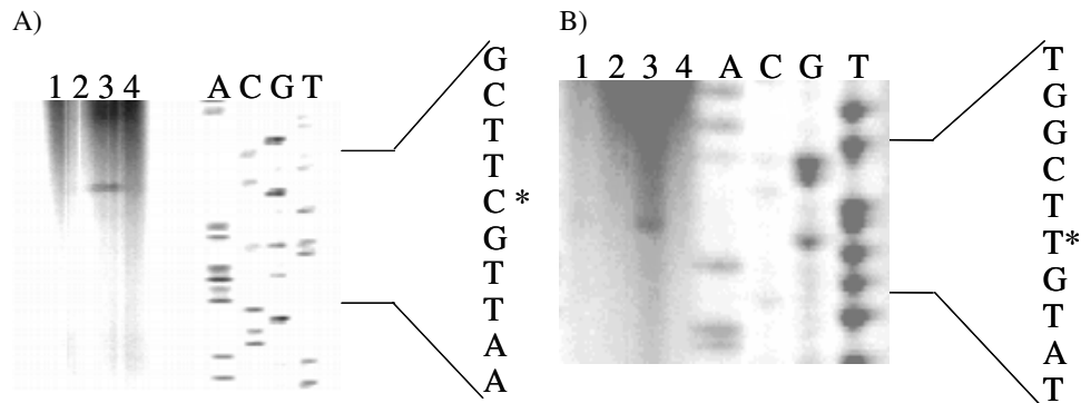
Abb. 5: Expressionsanalyse und Bestimmung des Transkriptionsstarts A) des ushA -Gens von C. glutamicum und B) des nucH -Gens von C. glutamicum . Für die Primerextensionsanalyse wurden 20 µg Gesamt-RNA von C. glutamicum \Delta phoRS für 0 min (Spur 1) und 90 min (Spur 2) in phosphatfreiem CGXII-Minimalmedium isoliert. Für C. glutamicum WT wurden ebenfalls 20 µg Gesamt-RNA für 0 min (Spur 3) und 90 min (Spur 4) nach Auslösen des Phosphatmangels benutzt. Der Transkriptionsstart ist durch einen Stern gekennzeichnet. Die korrespondierende Sequenzierreaktion (Spuren A, C, G und T) wurde durch dieselben IRD-800 markierten Oligonukleotide generiert, die auch für die Primerextensionsanalyse eingesetzt wurden. Als Template-DNA für die Sequenzierreaktion wurden die PCR-Produkte eingesetzt, in der sich der mutmaßliche Transkriptionsstart befindet.
