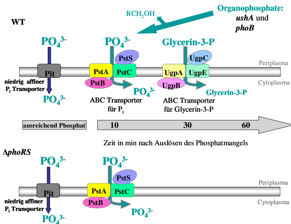
Abb. 2: Phosphatmangelantwort von C. glutamicum . Bei ausreichender Phosphatkonzentration wird Phosphat sowohl in C. glutamicum WT als auch in der Deletionsmutante \Delta phoRS über den niedrig affinen Transporter PitA aufgenommen. Bei Phosphatmangel wird nach Aktivierung des Zweikomponentensystems PhoRS zuerst das pstSCAB -Operon induziert. Dieses kodiert für die hochaffine, ATP-getriebene Aufnahme von Phosphat. Im Anschluss daran kommt es in C. glutamicum WT zur Expression des ugpABCE -Operons, das für die Aufnahme von Glycerin-3-Phosphat notwendig ist. Nach 60 min unter Phosphatmangelbedingungen werden Gene zur Nutzung von Phosphat aus nicht transportierbaren Phosphorquellen wie ushA und phoB induziert. In der Deletionsmutante \Delta phoRS wird im selben Zeitraum nur das pstSCAB -Operon aktiviert.
