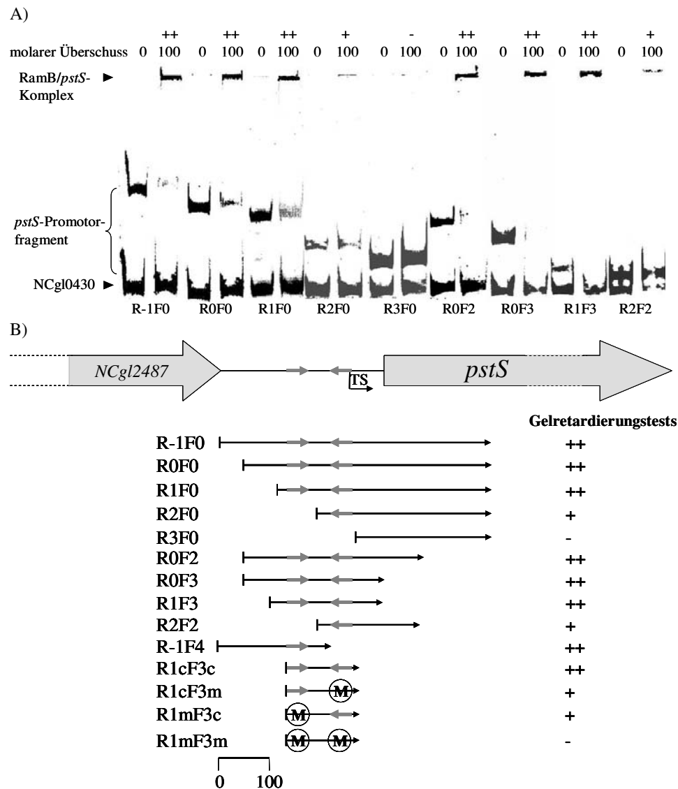
Abb. 22: A) Das Gel zeigt die Bindung von aufgereinigtem RamB (100-facher molarer Überschuss) an verschiedene Fragmente des pstS -Promotors (124 bp - 507 bp, Endkonzentrationen 61 nM - 15 nM). Über dem Gel ist angegeben, ob RamB an das Fragment genauso gut gebunden hat wie an den vollständigen Promotor R-1F0 (++), schlechter als an R-1F0 (+) oder überhaupt nicht (-). Die DNA-Protein-Mischung wurde für 30 min bei Raumtemperatur inkubiert, bevor sie auf einem 10%igen nativen Polyacrylamidgel aufgetrennt und mit Sybr Green I gefärbt wurde. B) Darstellung der DNA-Fragmente, die benutzt wurden, um die Bindung von RamB an den pstS -Promotor durch Gelretardierungstests nachzuweisen. Die Pfeile markieren zwei mögliche RamB-Bindemotive. Auf der rechten Seite ist gezeigt, ob RamB an das Fragment genauso gut gebunden hat wie an den vollständigen Promotor R-1F0 (++), schlechter als an R-1F0 (+) oder überhaupt nicht (-). Der Transkriptionsstart ist mit TS angegeben. M zeigt ein mutiertes RamB-Bindemotiv an.
