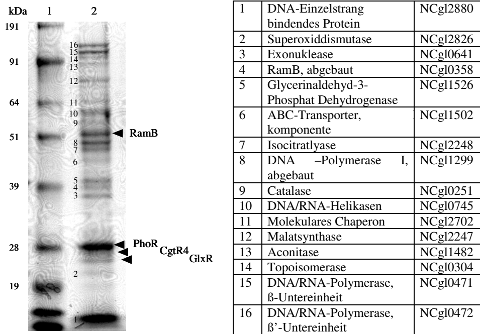
Abb. 13: Coomassie gefärbtes SDS-Gel von Proteinen, die über DNA-Affinitätschromatographie mit dem pstS -Promotor R-1F0 angereichert wurden. Es wurden Rohextrakte von C. glutamicum WT nach Kultivierung in CGXII-Minimalmedium unter Phosphatmangelbedingungen und 20 g/l Acetat verwendet. Spur 1: Proteinstandard Seebblue II prestained Standard (Invitrogen, Karlsruhe). Spur 2: Eluat der DNA-Affinitätschromatographie. Die Proteinbanden in Spur 2, in denen GlxR, CgtR4, PhoR und RamB durch MALDI-TOF MS identifiziert werden konnten, sind durch einen Pfeil markiert. Die übrigen durch MALDI-TOF MS identifizierten Proteine sind nummeriert und in der abgebildeten Tabelle dargestellt.
