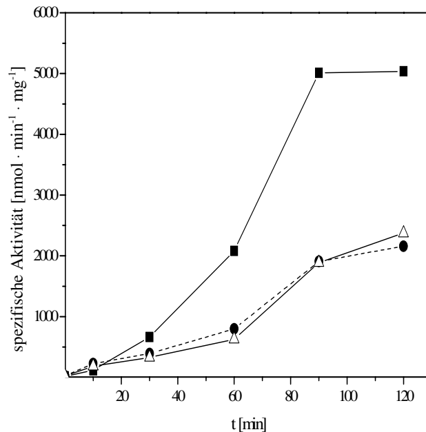
Abb. 9: Expression der Transkriptionsfusionen der pstS -Promotorfragmente in C. glutamicum WT und \Delta phoRS nach Phosphatlimitierung. Der vollständige pstS -Promotor R-1F0 in C. glutamicum WT ist durch das Quadrat, das Promotorfragment R0F0 in C. glutamicum WT durch einen Kreis und der pstS -Promotor R-1F0 in der Deletionsmutante \Delta phoRS durch ein offenes Dreieck dargestellt. Abkürzungen für die getesteten Promotorfragmente sind in Abb. 6 beschrieben.
