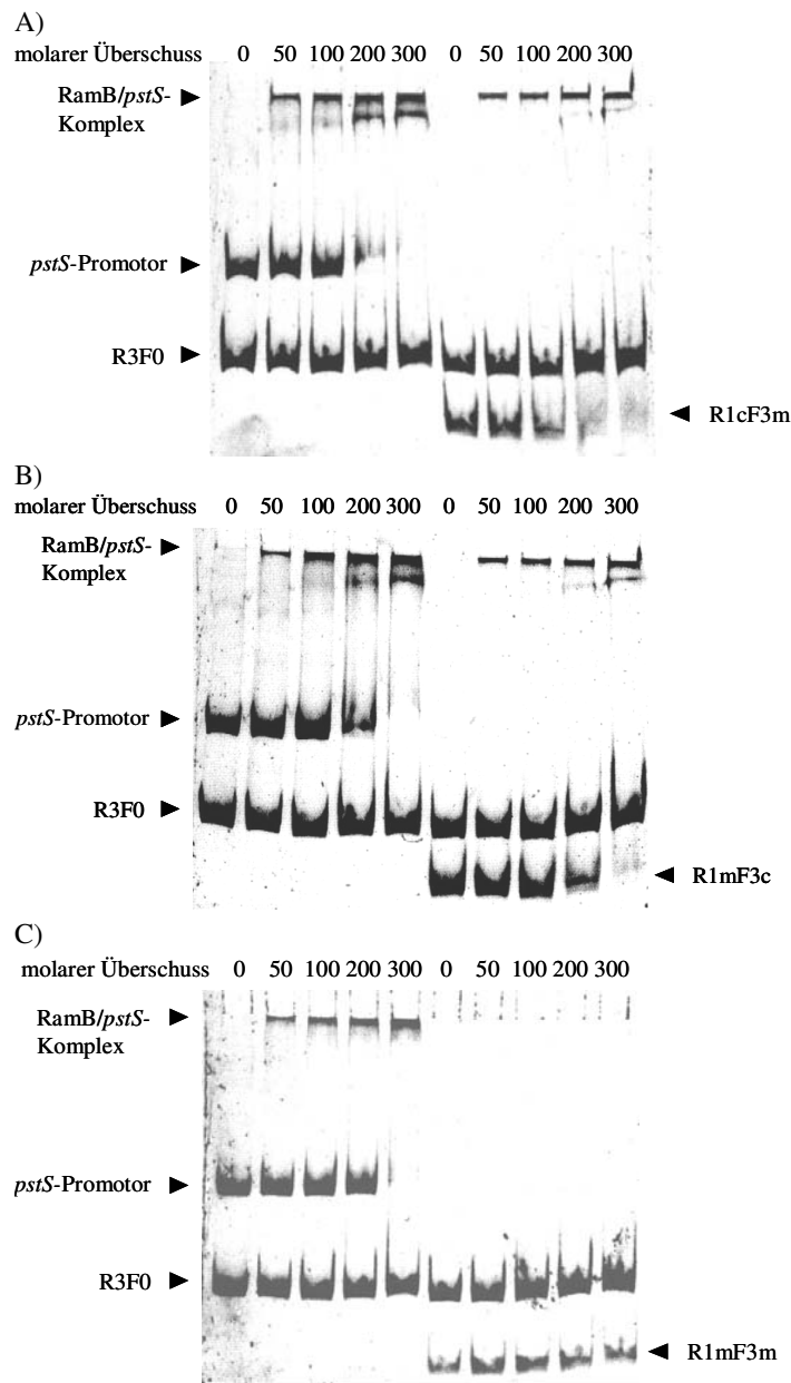
Abb. 25: Gelretardierungstests mit RamB und dem pstS -Promotor. A) Das Gel zeigt die Bindung von aufgereinigtem RamB (50 - 300-facher molarer Überschuss) an den pstS -Promotor (15 nM, 507 bp Fragment) und an das Fragment R1cF3m (61 nM, 124 bp Fragment). B) Das Gel zeigt die Bindung von aufgereinigtem RamB (50 - 300-facher molarer Überschuss) an den pstS -Promotor (15 nM 507 bp Fragment) und an das Fragment R1mF3c (61 nM, 124 bp Fragment). C) Das Gel zeigt die Bindung von aufgereinigtem RamB (50 - 300-facher molarer Überschuss) an den pstS -Promotor (15 nM, 507 bp Fragment) und an das Fragment R1mF3m (61 nM, 124 bp Fragment). Ein 267 bp langes Fragment R3F0 (30 nM) aus der pstS -Promotorregion wurde als Negativkontrolle eingesetzt.
