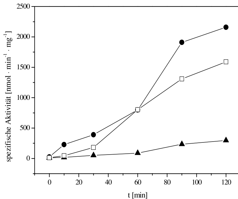
Abb. 26: Expression der R0F0-Transkriptionsfusion in C. glutamicum WT und \Delta ramB nach Phosphatlimitierung in CGXII-Minimalmedium sowohl auf 40 g/l Glucose als auch auf 20 g/l Acetat. Das Promotorfragment R0F0 in C. glutamicum WT, angezogen auf CGXII-Minimalmedium mit 40 g/l Glucose und unter Phosphatmangelbedingungen, ist durch einen Kreis dargestellt. Das Promotorfragment R0F0 in C. glutamicum WT angezogen auf CGXII-Minimalmedium mit 20 g/l Acetat und unter Phosphatmangelbedingungen, ist durch ein Dreieck dargestellt. Das Promotorfragment R0F0 in der Mutante \Delta ramB , angezogen auf CGXII-Minimalmedium mit 40 g/l Glucose und unter Phosphatmangelbedingungen, ist durch ein offenes Quadrat dargestellt.
