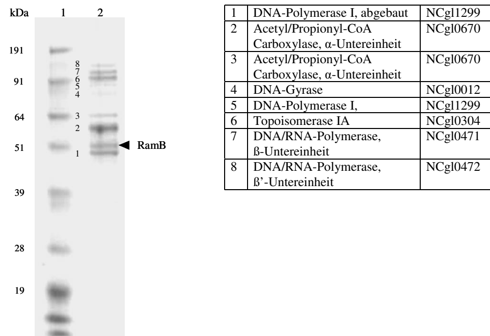
Abb. 11: Coomassie gefärbtes SDS-Gel von Proteinen, die über DNA-Affinitätschromatographie mit dem pstS -Promotorfragment R0F2 angereichert wurden. Es wurden Rohextrakte von C. glutamicum \Delta phoRS nach Kultivierung in CGXII-Minimalmedium mit 40 g/l Glucose und unter ausreichender Phosphatkonzentration verwendet. Spur 1: Proteinstandard Seebue II prestained Standard (Invitrogen, Karlsruhe). Spur 2: Eluat der DNA-Affinitätschromatographie. Die Proteinbande in Spur 2, in der RamB durch MALDI-TOF MS identifiziert werden konnte, ist durch einen Pfeil markiert. Die übrigen durch MALDI-TOF MS identifizierten Proteine sind nummeriert und in der abgebildeten Tabelle dargestellt.
