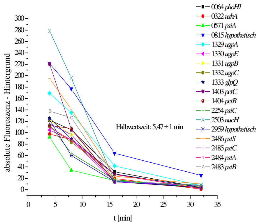
Abb. 32: Stabilität der mRNA des Pho-Regulons. Die mRNA dieser Gene zeigte eine Halbwertszeit von 5,47 \pm 1 \text{ min} und entspricht damit fast der durchschnittlichen Halbwertszeit aller Gene. In der Legende sind die NCgl-Nummern der entsprechenden Gene und die Gennamen angegeben.
