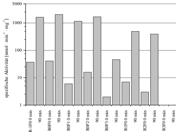
Abb. 8: Expression der verschiedenen pstS' - cat -Promotorfusionen in C. glutamicum \Delta phoRS : Die Expressionsniveaus wurden 0 und 90 min nach Auslösen des Phosphatmangels als spezifische Aktivität der Chloramphenicolacetyltransferase gemessen. Abkürzungen für die getesteten Promotorfragmente sind in Abb. 6 beschrieben.
