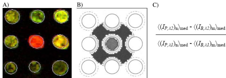
Abb. 4: Quantifizierung der Fluoreszenz von Hybridisierungssignalen auf einem DNA-Chip mit der Software GenePix Pro 4.1. A) Ausschnitt aus einem Fluorogramm mit identifizierten Hybridisierungssignalen (Polen 2002) B) Schematische Quantifizierung der Hybridisierungssignal-Fluoreszenz (Handbuch zur GenePix 4.1 Software) C) Berechnung des Quotienten der Mediane eines Hybridisierungssignals (Handbuch zur GenePix 4.1 Software)
