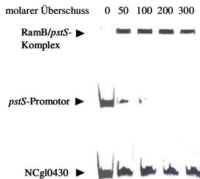
Abb. 21: Gelretardierungstests mit RamB und der pstS -Promotorregion. A) Das aufgereinigte RamB-Protein wurde in verschiedenen Konzentrationen (50 – 300-facher molarer Überschuss) mit 15 nM des vollständigen pstS -Promotors (R-1F0) inkubiert. Dieses Promotorfragment ist 507 bp lang und erstreckt sich von -216 bis +290, bezogen auf den Transkriptionsstart. In dieser Region sind zwei mögliche RamB-Bindemotive (AA/GAACTTTGCAAA) enthalten. Als Negativkontrolle wurde ein 185 bp langes Fragment des Promotors von NCgl0430 (41 nM) benutzt.
