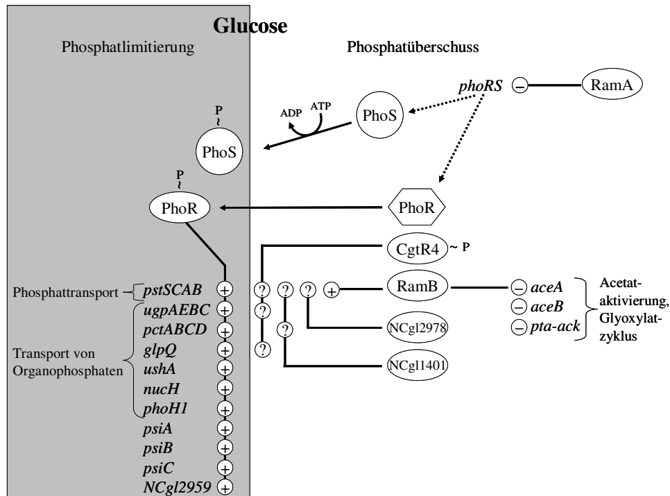
Abb. 33: Modell der Phosphatregulation in C. glutamicum bei Kultivierung auf Glucose.
