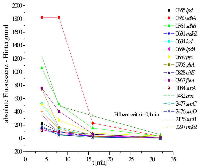
Abb. 31: Stabilität der mRNA der Enzyme des Tricarbonsäure-Zyklus. Die mRNA dieser Gene entspricht mit einer durchschnittlichen Halbwertszeit von 6 min dem Durchschnitt aller Gene. In der Legende sind die NCgl-Nummern der entsprechenden Gene und die Gennamen angegeben.
