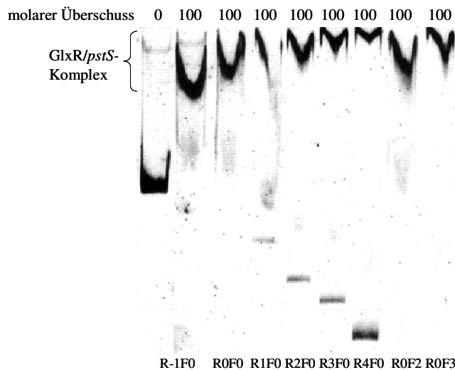
Abb. 18: Gelretardierungstests mit GlxR und dem pstS -Promotor. Das Gel zeigt die Bindung von aufgereinigtem GlxR (100-facher molarer Überschuss) an den pstS -Promotor (15 nM, 507-bp Fragment) oder die Fragmente R0F0, R1F0, R2F0, R3F0, R4F0, R0F2 und R0F3. (15 nM, 507-bp Fragment) in Abhängigkeit von 0,2 mM cAMP. Mit zunehmender Verkürzung der 5'-Region (R1 bis R4) nimmt die Interaktion zwischen GlxR und den Teilfragmenten des pstS -Promotors ab. Es wurde keine Negativkontrolle eingesetzt.
