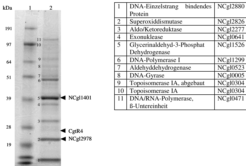
Abb. 14: Coomassie gefärbtes SDS-Gel von Proteinen, die über DNA-Affinitätschromatographie mit dem pstS -Promotor R-1F0 angereichert wurden. Es wurden Rohextrakte aus C. glutamicum WT nach Kultivierung in CGXII-Minimalmedium unter ausreichender Phosphatkonzentration und 40 g/l Glucose verwendet. Spur 1: Proteinstandard Seebblue II prestained Standard (Invitrogen, Karlsruhe). Spur 2: Eluat der DNA-Affinitätschromatographie. Die Proteinbanden in Spur 2, in der CgtR4 und NCgl1401 durch MALDI-TOF MS identifiziert werden konnten, sind durch einen Pfeil markiert. Die übrigen durch MALDI-TOF MS identifizierten Proteine sind nummeriert und in der abgebildeten Tabelle dargestellt.
