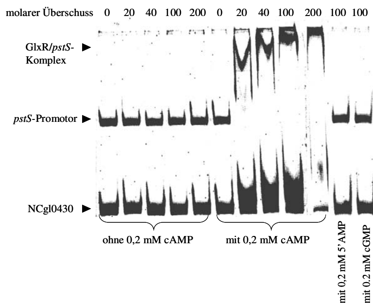
Abb. 17: Gelretardierungstests mit GlxR und dem pstS -Promotor. Das Gel zeigt die Bindung von aufgereinigtem GlxR (20 – 200-facher molarer Überschuss) an den pstS -Promotor (15 nM, 507-bp Fragment) in Abhängigkeit von 0,2 mM cAMP. Die Gelretardierung erfolgt nicht mit 0,2 mM 5'AMP oder 0,2 mM cGMP. Als Negativkontrolle wurde ein 185 bp langes Fragment des Promotors NCgl0430 (41 nM) eingesetzt. Dieses zeigte aber auch eine Bindung an GlxR.
