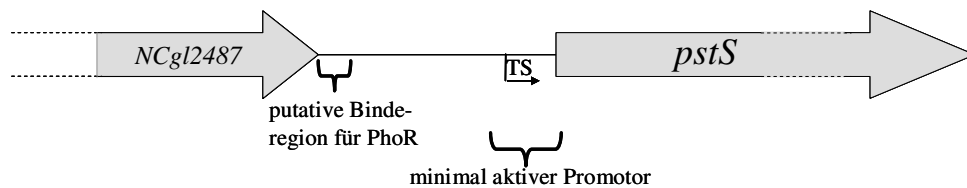
Abb. 10: Beschreibung der putativen Binderegion für PhoR und des minimal aktiven Promotors.
