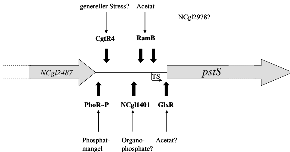
Abb. 15: Modell der Regulation des pstS -Promotors durch sechs verschiedene Transkriptionsregulatoren und deren möglichen Stimuli.
