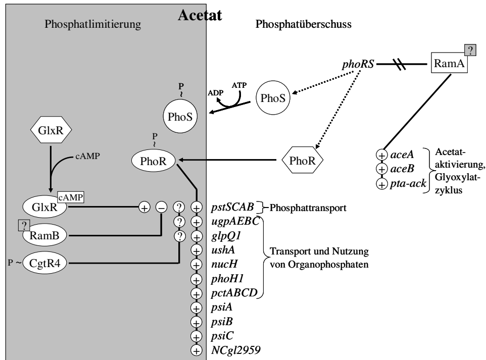
Abb. 34: Modell der Phosphatregulation in C. glutamicum bei Kultivierung auf Acetat.
