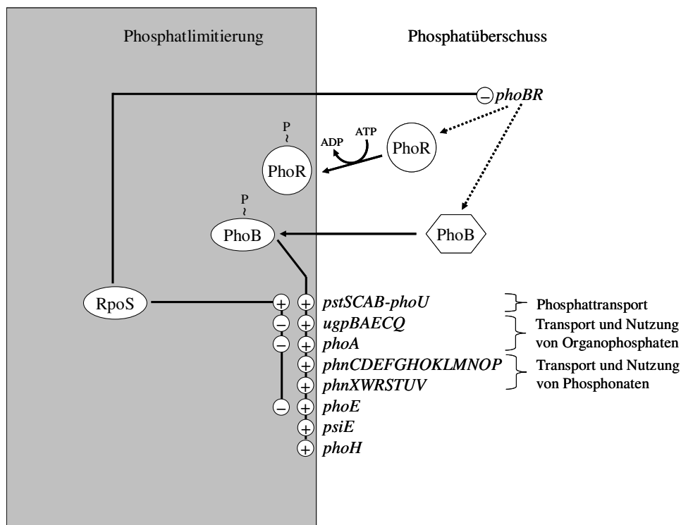
Abb. 1: Regulationsnetzwerk in E. coli . Bei Phosphatmangel phosphoryliert die Sensorkinase PhoR den Antwortregulator PhoB und phosphoryliertes PhoB aktiviert die Expression seiner Zielgene. Unter Stressbedingungen vermittelt der Sigma-Faktor RpoS der RNA-Polymerase verringerte Transkription von phoA , phoE , des phoBR -Operons und des ugpBAECQ -Operons, während das pstSCAB-phoU -Operon verstärkt transkribiert wird.
