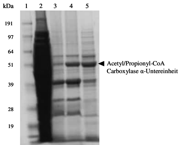
Abb. 12: Coomassie gefärbtes SDS-Gel der Waschfraktionen, die über DNA-Affinitätschromatographie mit dem pstS -Promotor R0F2 angereichert wurden. Es wurden Rohextrakte von C. glutamicum \Delta phoRS nach Kultivierung in CGXII-Minimalmedium mit 40 g/l Glucose und unter ausreichender Phosphatkonzentration verwendet. Spur 1: Proteinstandard Seeblue II prestained Standard (Invitrogen, Karlsruhe). Spur 2 - 5: Waschschriffe. Die Analyse der Waschschriffe der Spuren 3 – 5 diente dem Nachweis, ob RamB spezifisch an den pstS -Promotor bindet und sich nicht in den Waschschriffen findet. In der entsprechenden Bande, markiert durch einen Pfeil, konnte nur das Enzym Acetyl/Propionyl-CoA Carboxylase durch MALDI-TOF MS identifiziert werden.
