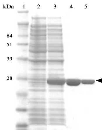
Abb. 16: Aufreinigung von GlxR, das durch den Pfeil markiert ist. In Spur 1 befindet sich der Proteinstandard Seebblue II prestained Standard (Invitrogen, Karlsruhe). In Spur 2 ist der Zellaufschluss vor der Induktion mit IPTG zu sehen. In Spur 3 ist überexprimiertes GlxR 4 h nach Induktion mit IPTG zu sehen. In Spur 4 sieht man aufgereinigtes GlxR nach Elution mit Imidazol von einer Nickelchelataffinitätssäule und in Spur 5 aufgereinigtes GlxR nach Umpuffern in den BS-Puffer und Verdau mit Faktor Xa. Die Proteine wurden auf einem 10% SDS-Polyacrylamidgel aufgetrennt und mit Coomassieblau gefärbt.
