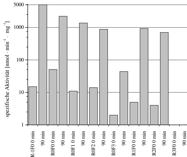
Abb. 7: Expression der verschiedenen pstS' - cat -Promotorfusionen in C. glutamicum WT: Die Expressionsniveaus wurden 0 und 90 min nach Auslösen des Phosphatmangels als spezifische Aktivität der Chloramphenicolacetyltransferase gemessen. Abkürzungen für die getesteten Promotorfragmente sind in Abb. 6 beschrieben.
