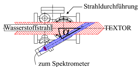
Abbildung 5.3.: Beobachtung der Strahlemission zur Bestimmung der Speziesverteilung.
