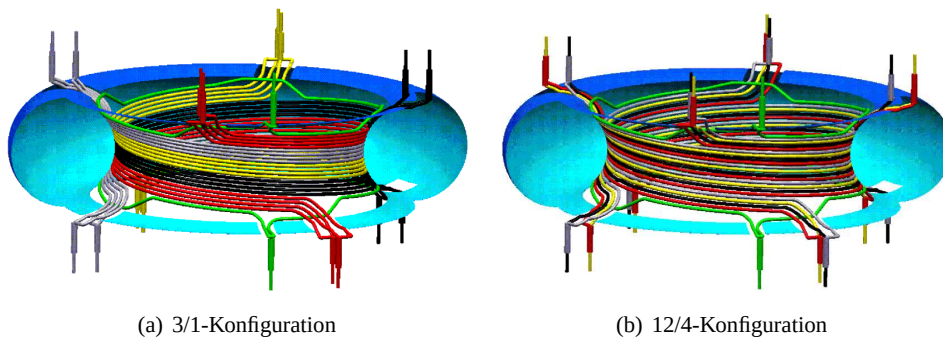
Abbildung 4.2.: Aufbau des Dynamischen Ergodischen Divertors auf der Hochfeldseite von TEXTOR. Gezeigt sind die in dieser Arbeit verwendeten Spulen-Konfigurationen
