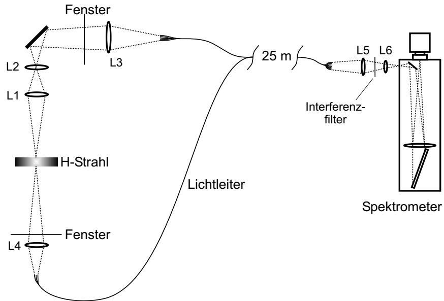
Abbildung 5.6.: Schema des optischen Weges: Abbildung des Beobachtungsvolumens im TEXTOR-Plasma auf die Lichtleiter, Übertragung zum Spektrometer und Durchgang zur CCD-Kamera.
