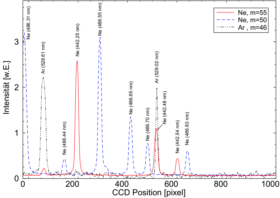
Abbildung 5.10.: Neon- und Argon-Lampenlinien verschiedener Ordnungen zur Bestimmung der Dispersion des CCD-Detektors. Das Spektrometer ist auf \lambda = 529.0525 \text{ nm} , m = 46 eingestellt.
