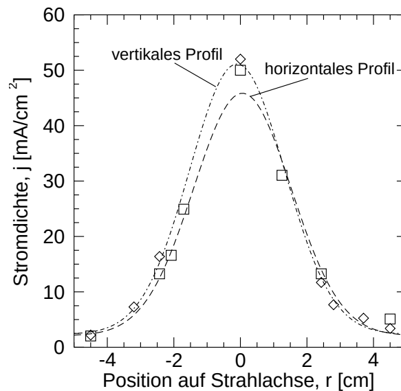
Abbildung 5.2.: Profil des Wasserstoffstrahls entlang der vertikalen und horizontalen Achse, gemessen mit dem Kalorimeter in 2 m Entfernung von der Ionenquelle. Die 1/e-Breite beträgt hier 4 cm, zwei Meter weiter im Plasma 8 cm.
