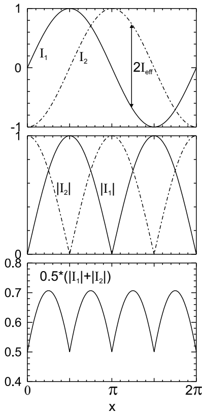
Abbildung 4.3.: Zur Berechnung des effektiven Spulenstroms im dynamischen Betrieb zum Vergleich mit dem statischen Betrieb.
