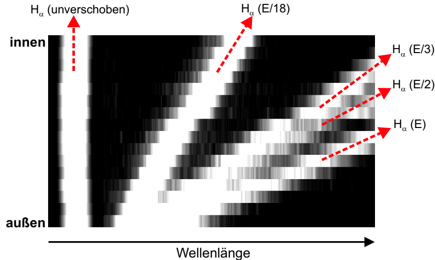
Abbildung 5.8.: Zweidimensionale Aufnahme eines Strahlemissionsspektrums zur Radiuskalibrierung. Zu sehen sind die H_\alpha -Spektrallinien der unverschobenen Komponente des Hintergrundes sowie der dopplerverschobenen Strahlkomponenten bei 1/18, 1/3, 1/2 und voller Energie (bei dieser Aufnahme ist die 1/18-Komponente ungewöhnlich stark). Die Raumkanäle sind entlang der vertikalen Achse angeordnet, sodaß sich das Spektrum einer jeden Zeile einer radialen Position in TEXTOR zuordnen läßt.
