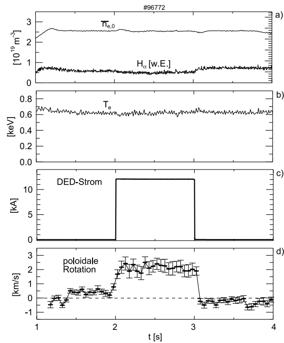
(b) DED 12/4 Konfiguration
