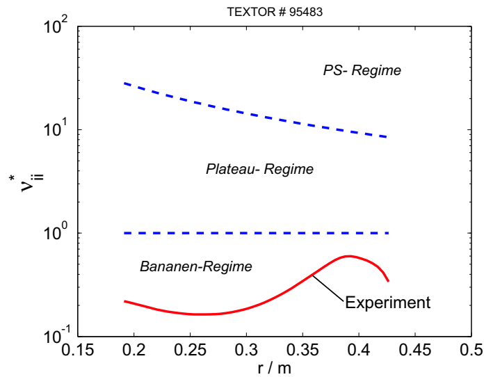
Abbildung 6.3.: Profil der Ionen-Ionen-Stößeigkeit der Entladung #95483. Auf den inneren Radien befindet sich die Stößeigkeit im Bananen-Regime, nach außen nähert sie sich dem Plateau-Regime.
