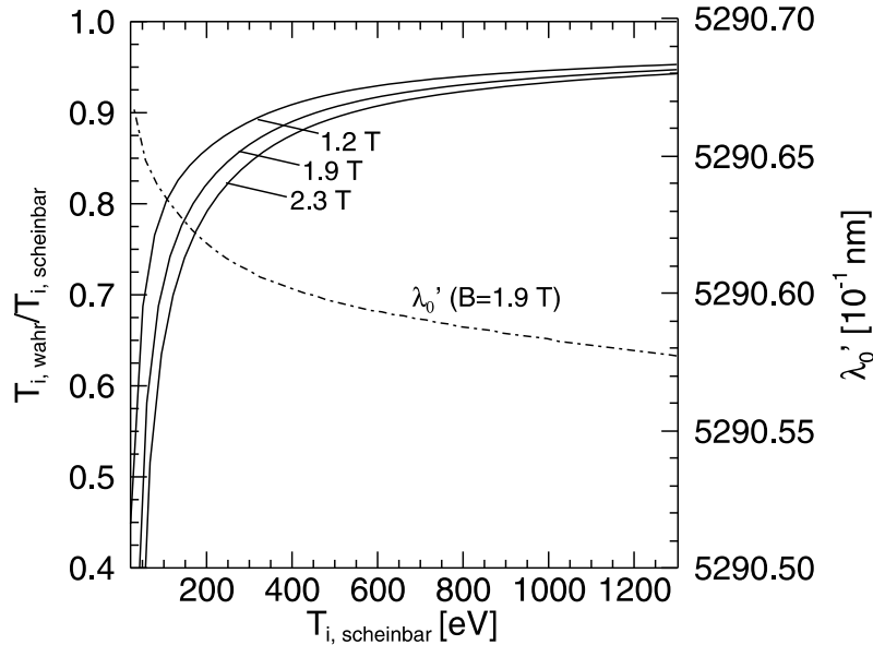
Abbildung 3.3.: Korrekturen für die Ionentemperatur (—) bei drei verschiedenen Magnetfeldstärken und zentrale Wellenlänge (---) für ein Magnetfeld aufgrund von Feinstruktur und Zeeman-Effekt. Der Winkel zwischen Beobachtungsrichtung und Magnetfeld beträgt ungefähr 85^\circ .
