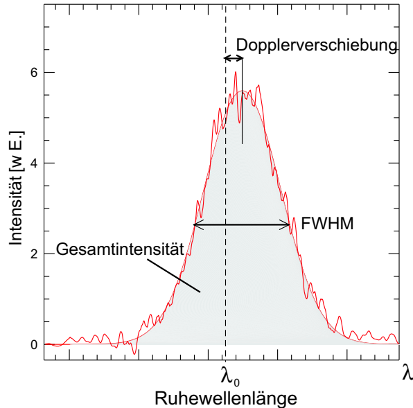
Abbildung 3.2.: Bestimmungsgrößen der aktiven Ladungsaustauschspektroskopie: Die Kohlenstoffdichte ergibt sich aus der Gesamtintensität der Linie, die Temperatur aus der Linienbreite (volle Breite auf halber Höhe, FWHM) und die Rotation aus der Dopplerverschiebung des Linienzentrums gegenüber der Ruhewellenlänge.
