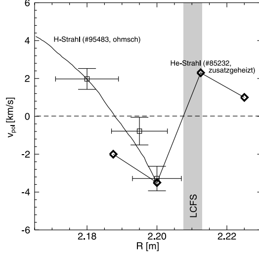
Abbildung 6.4.: Vergrößerung des Randbereiches von Abbildung 6.1 c). Zusätzlich gezeigt ist ein ebenfalls aktiv gemessenes Profil aus [49], welches allerdings einer zusatzgeheizten Entladung entstammt.
