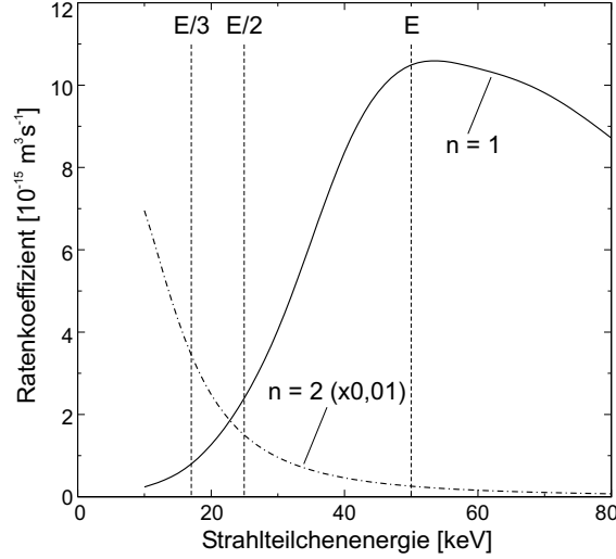
Abbildung 3.1.: Ratenkoeffizient des CVI(529)-Übergangs durch Ladungsaustausch mit einem 50 keV Wasserstoffstrahl. Dargestellt sind sowohl Ladungsaustausch mit Wasserstoff im Grundzustand (—) als auch aus dem ersten angeregten Zustand (---, zur besseren Darstellung um einen Faktor 100 verkleinert).
