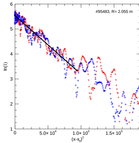
Abbildung 5.14.: Halblogarithmische Darstellung der Intensität des aktiven Spektrums für beide Flanken gegen den quadrierten Abstand vom Zentrum. Der lineare Abfall über \Delta \ln(I) \geq 2.3 bedeutet, daß das Spektrum über mindestens eine Größenordnung durch eine Gaußfunktion beschrieben werden kann.
