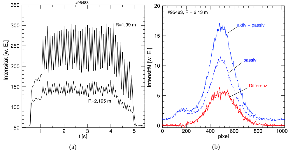
Abbildung 5.12.: a) Zeitspur des CVI-Signals während einer ohmschen Entladung auf dem innersten und dem äußersten Kanal ( \bar{n}_{e,0} = 2 \cdot 10^{19} \text{ m}^{-3} ). Der Wasserstoffstrahl läuft moduliert mit 10 Hz von t = (1-5) \text{ s} . b) Gemittelte Spektren aus der Strahl-An Phase (aktiv+passiv) und der Strahl-Aus Phase (passiv) sowie deren Differenz (aktiv) bei R = 2.13 \text{ m} . Gezeigt ist zusätzlich die Gaußkurve, durch die sich das aktive Spektrum beschreiben läßt.
