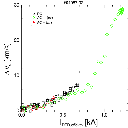
Abbildung 6.14.: Änderung der toroidalen Rotation als Funktion des DED-Stromes
