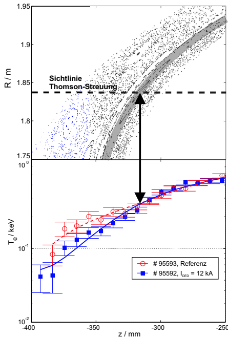
Abbildung 6.11.: Mit Thomson-Streuung gemessene T_e -Profile der Entladung #95592 mit (■) und ohne Ergodisierung (○). Die obere Hälfte der Abbildung zeigt die gerechnete Poincaré-Struktur. Die letzte ungestörte Flußfläche korreliert mit der Position, ab der die Temperatur im ergodischen Profil niedriger ist als im Referenzprofil.
