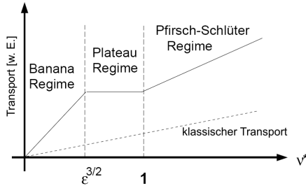
Abbildung 2.2.: Abhängigkeit des Transports von der Plasmastößigkeit. In dieser Arbeit liegt am Plasmarand das Plateauregime vor.
