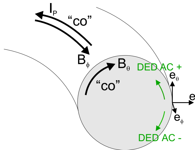
Abbildung 4.4.: Standardkonfiguration von Plasmastrom und Magnetfeld an TEXTOR, das Tokamak-Koordinatensystem ( e_r, e_\theta, e_\phi ) und die Drehrichtung des DED-Feldes im dynamischen Betrieb. Zusätzlich ist die Richtung der diamagnetischen Drift von Ionen und Elektronen angezeigt.
