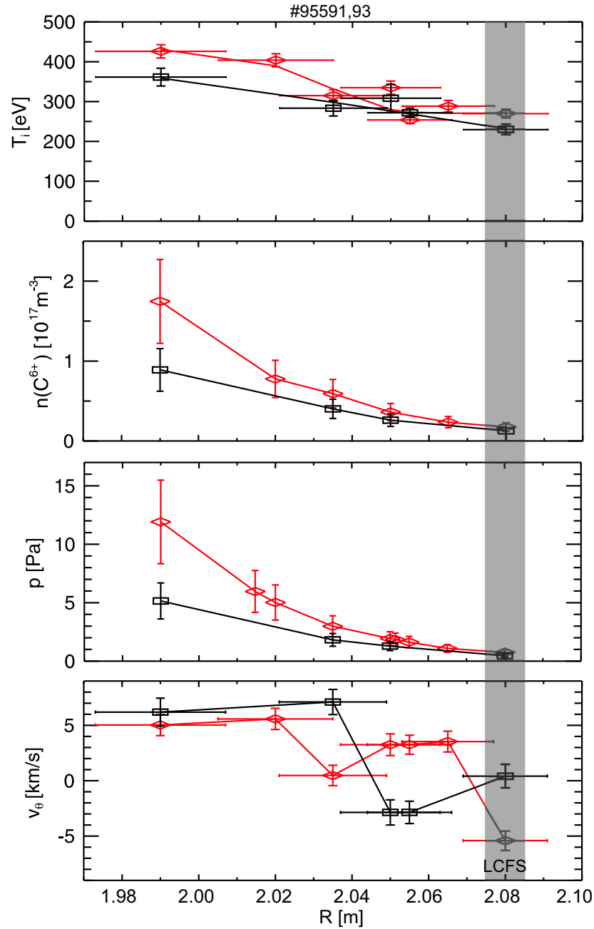
Abbildung 6.8.: C^{6+} Profile von Ionentemperatur, Kohlenstoffdichte, -druck und poloidaler Rotation für eine Referenzentladung ohne ( \square ) und mit DED ( \diamond ). Die Profile sind über 0.6 s integriert. Die letzte geschlossene Flußfläche des Referenzschusses ist um R_{LCFS} = 2.08 m schraffiert angegeben.
