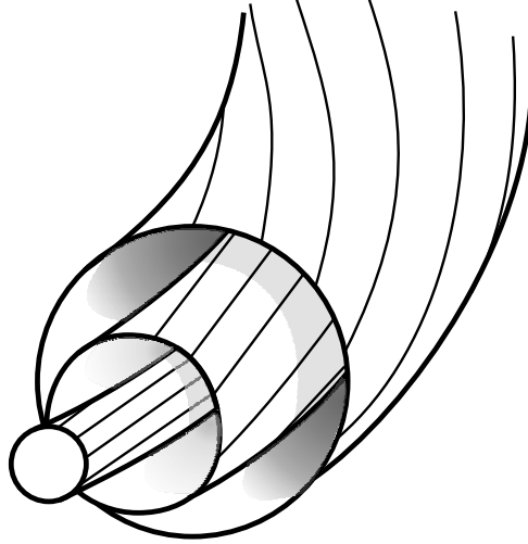
Abbildung 2.1.: Aufbau der magnetischen Flußflächen durch poloidales und toroidales Magnetfeld
