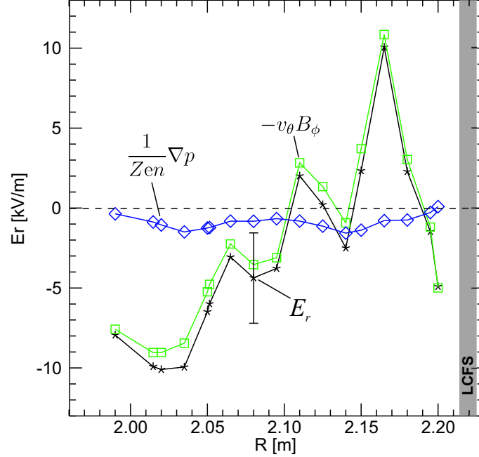
Abbildung 6.5.: Profil des radialen elektrischen Feldes für die ohmsche Entladung #95483, berechnet nach der radialen Kraftgleichung 2.5 aus den gemessenen Profilen von Abbildung 6.1. Die Punkte sind lediglich zur besseren Zuordnung mit Linien verbunden.
