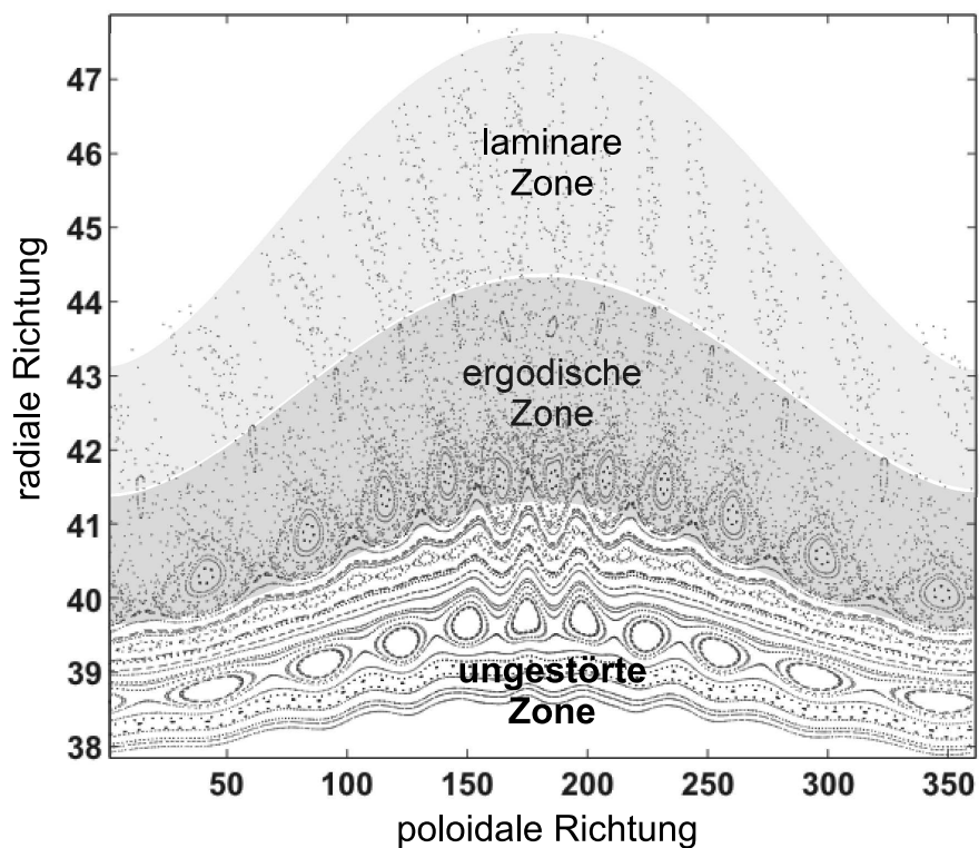
Abbildung 2.3.: Poincaré-Bild der gestörten magnetischen Topologie. Die ergodische Zone wird durch überlappende magnetische Inseln gebildet, sodaß die intakten Flußflächen aufgelöst werden. Inselreste sind noch vorhanden. Die laminare Zone zeichnet sich durch Feldlinien aus, die in fingerähnlichen Strukturen das Plasma verlassen, und durch Feldlinien kurzer Verbindungsänge zur Wand.
