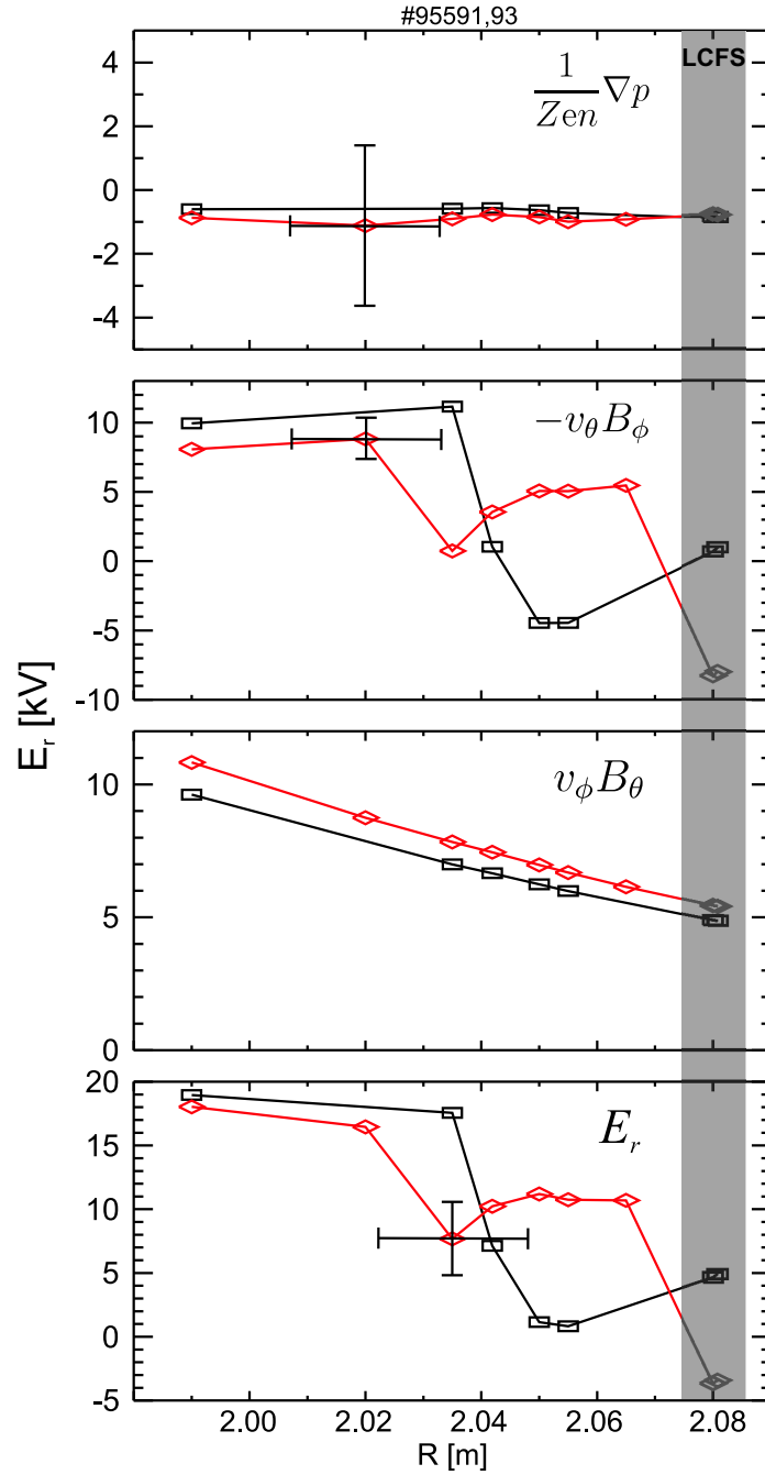
Abbildung 6.9.: Beiträge zum radialen elektrischen Feld für die Entladung ohne (schwarz) und mit Dynamisch Ergodischem Divertor (rot). Die Absolutwerte des v_\phi B_\theta -Terms sind mit einer großen Unsicherheit behaftet, weswegen nur die Änderungen zwischen den beiden Entladungen betrachtet werden.
