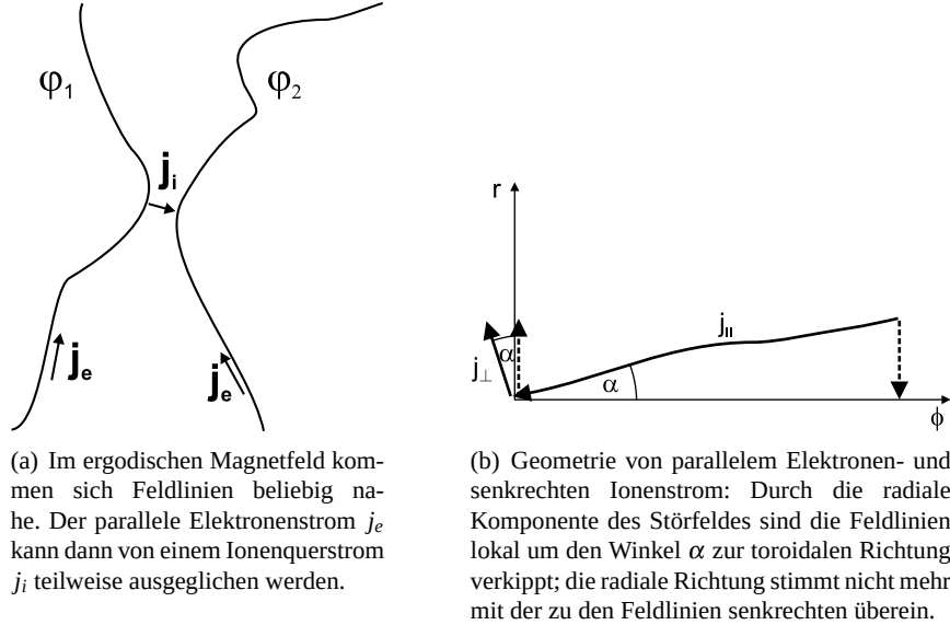
Abbildung 2.4.: Elektronen- und Ionenausgleichstrom im ergodisierten Magnetfeld
