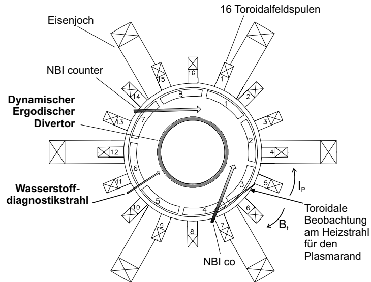
Abbildung 4.1.: Aufsicht des Tokamak-Experiments TEXTOR
