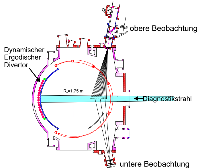
Abbildung 5.5.: Aufbau des Beobachtungssystems am Plasmarand zur Ladungsaustauschspektroskopie am Diagnostikstrahl. Es beobachtet einen radialen Bereich von R = (2.00-2.23) m. Die zusätzlichen Sichtlinien von unten ermöglichen die Kalibrierung und präzise Vermessung der Plasmarotation.
