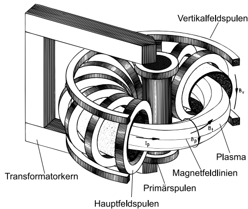
Abbildung 1.1.: Prinzip des magnetischen Einschlusses am Tokamak
