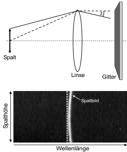
Abbildung 5.11.: Linienkrümmung durch die endliche Höhe von Spalt und Gitter.
