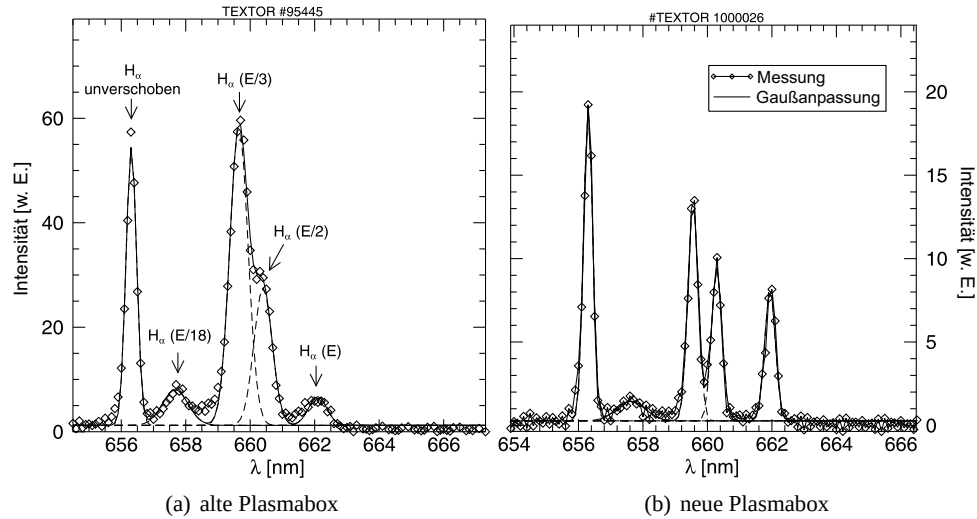
Abbildung 5.4.: H_\alpha -Strahlemissionsspektren des Diagnostikstrahls für die alte (a) und die neue (b) Plasmabox. Mit der neuen Plasmabox ist das Verhältnis der vollen Energiekomponente zu den anderen Komponenten deutlich gestiegen.
