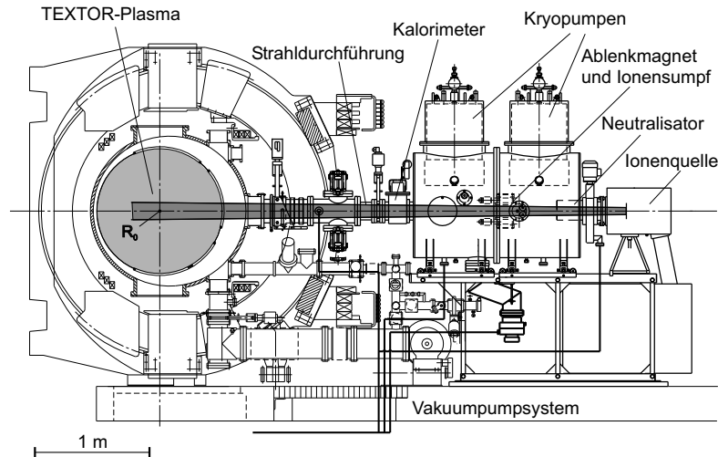
Abbildung 5.1.: Aufbau des Wasserstoffdiagnostikstrahl-Injektors an TEXTOR. Wesentliche Komponenten sind die Hochfrequenz-Ionenquelle zusammen mit der 4-Gitter-Ionenoptik, die Neutralisator-Kammer und das Kalorimeter zur Messung des Strahlprofils. Der Ablenkmagnet entfernt nicht-neutralisierte Strahlteilchen. Der Strahl wird radial injiziert.
