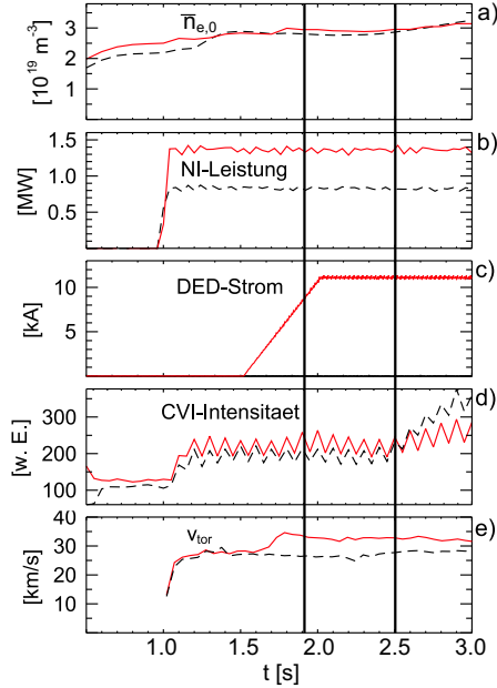
Abbildung 6.6.: Plasmaparameter zu den Profilmessungen zusammen mit dem Dynamischen Ergodischen Divertor (— #95591) und eine Referenzentladung ohne (--- #95593). Das Intervall der Auswertung geht von t = (1.9-2.5) s.
