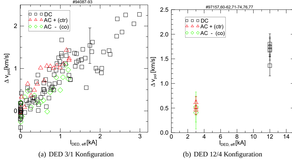
Abbildung 6.13.: Änderung der poloidalen C^{2+} Rotation mit dem effektiven DED-Strom
