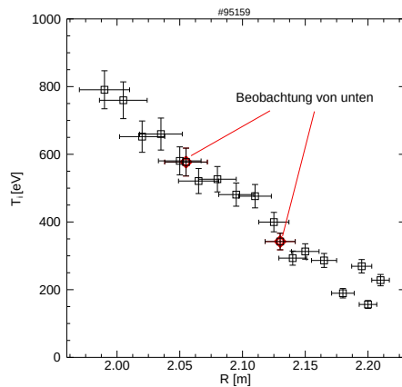
Abbildung 5.9.: Temperaturprofil mit anhand der Strahlemission justierten Beobachtungskanälen. Die Kanäle von unten ( \diamond ) reihen sich korrekt in den Verlauf der Kanäle von oben ein.
