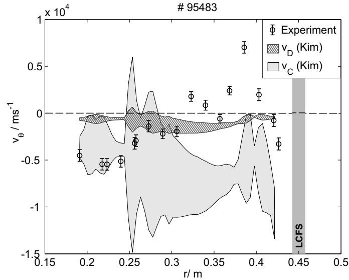
Abbildung 6.2.: Berechnete neoklassische Kohlenstoff- und Deuterium-Rotation für die Entladung #95483, basierend auf dem Formalismus nach Kim [11], im Vergleich mit den Meßwerten. Die gemusterten Bereiche repräsentieren jeweils das Werteband, das sich aus den Meßfehlern der Eingangsgrößen ergibt. Der Radius ist in Flußflächenkoordinaten angegeben (siehe auch Anhang A).
