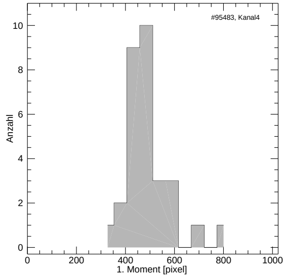
Abbildung 5.13.: Histogramm des 1. Momentes aller zu mittelnden Spektren. Ausreißer von der Normalverteilung wie die beiden Werte bei 700 und 800 werden bei der weiteren Auswertung nicht berücksichtigt
