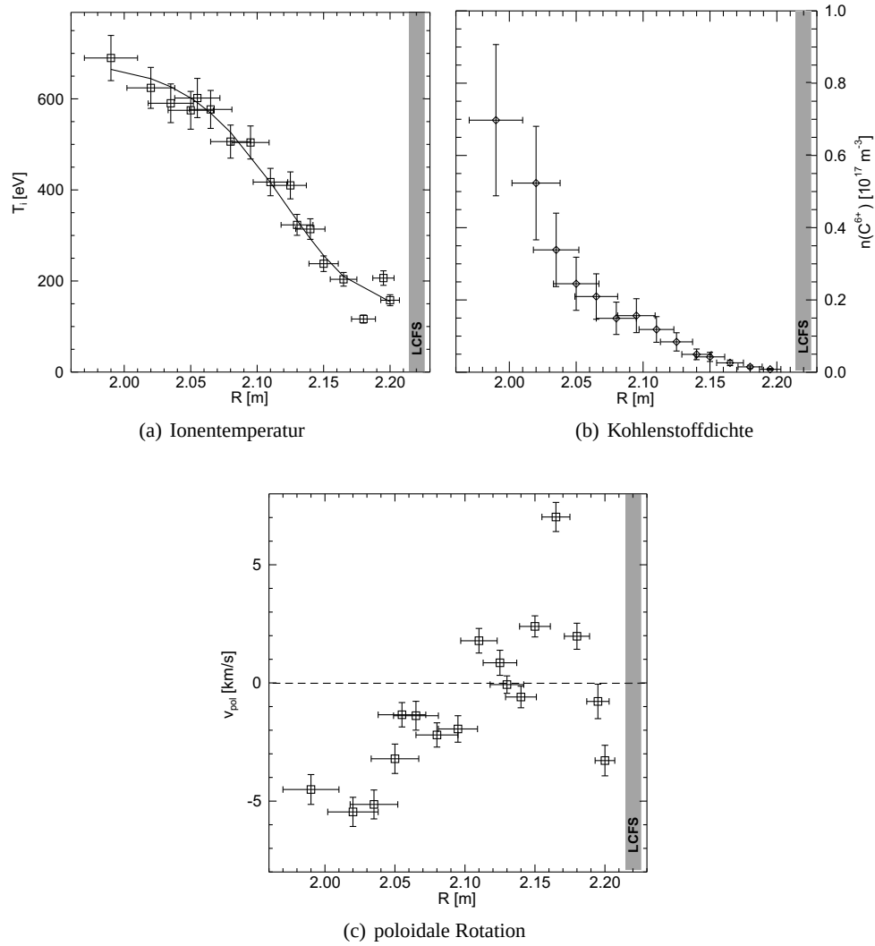
Abbildung 6.1.: Gemessene Profile der ohmschen Entladung #95483 ( \bar{n}_{e,0} = 2 \cdot 10^{19} \text{ m}^{-3} , I_p = 400 \text{ kA} , B_t = 1.9 \text{ T} , R_0 = 1.77 \text{ m} ) sowie daraus abgeleitet die Beiträge zum radialen elektrischen Feld. Die Profile stammen aus der gesamten stationären Phase der Entladung, t = (1-4) \text{ s} . Die letzte geschlossene Flußfläche liegt bei R = 2.21 \text{ m} . An das Temperaturprofil wurde eine Funktion der Form T(r) = a + b \exp(-cr^d) angepaßt mit den freien Parametern a , b , c und d [22].
