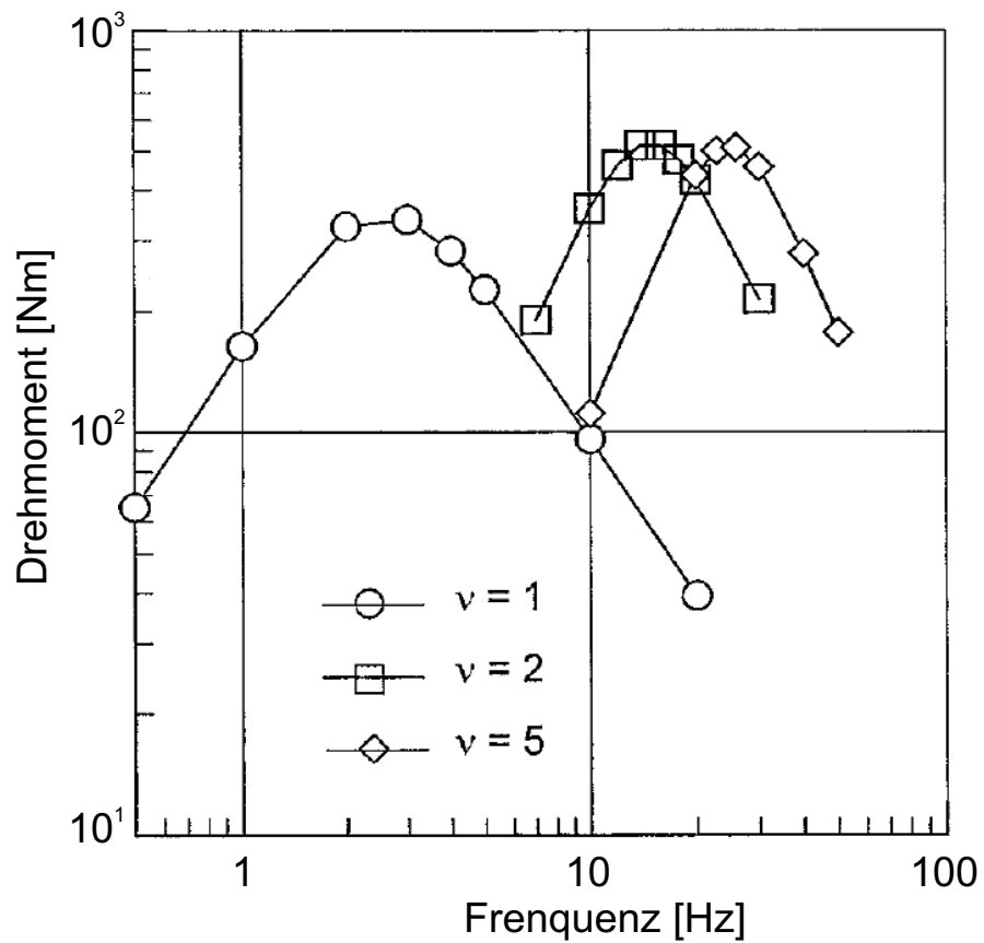
Abbildung 2.5.: Kraftübertrag eines rotierenden Störfeldes auf das Plasma bei verschiedenen Frequenzen durch die Wechselwirkung mit induzierten Abschirmströmen. Gezeigt sind Rechnungen für verschieden Ausdehnungen der Schicht, in der die Ströme fließen (aus [26]).
