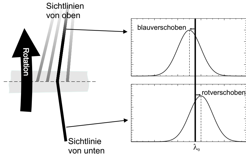
Abbildung 5.7.: Prinzip der differentiellen Dopplerspektroskopie mittels von oben und unten auf den Diagnostikstrahl blickender Sichtlinien. Die beiden schwarz markierten beobachten das selbe Plasmavolumen und sehen eine Plasmarotation sowohl rot- als auch blauverschoben. Die Mitte zwischen beiden Spektren definiert die Position der unverschobenen Wellenlänge \lambda_0 . In diesem Beispiel rotiert das Plasma nach oben.
