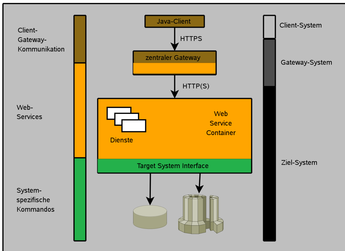
Abbildung 4.1: UNICORE Übersicht
