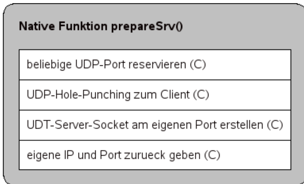
Abbildung 4.11: Funktion prepareSrv()
