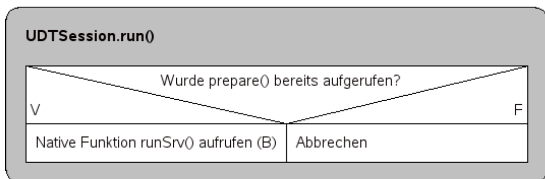
Abbildung 4.10: Methode UDTSession.run()
