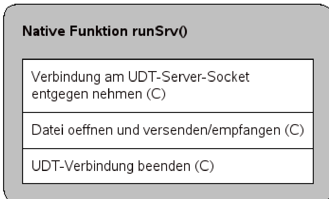
Abbildung 4.12: Funktion runSrv()
