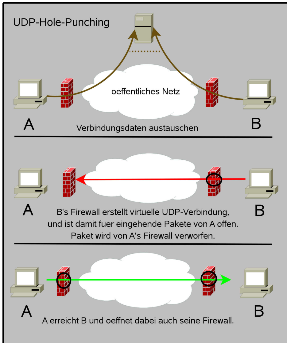
Abbildung 2.2: Prinzip des UDP-Hole-Punching
