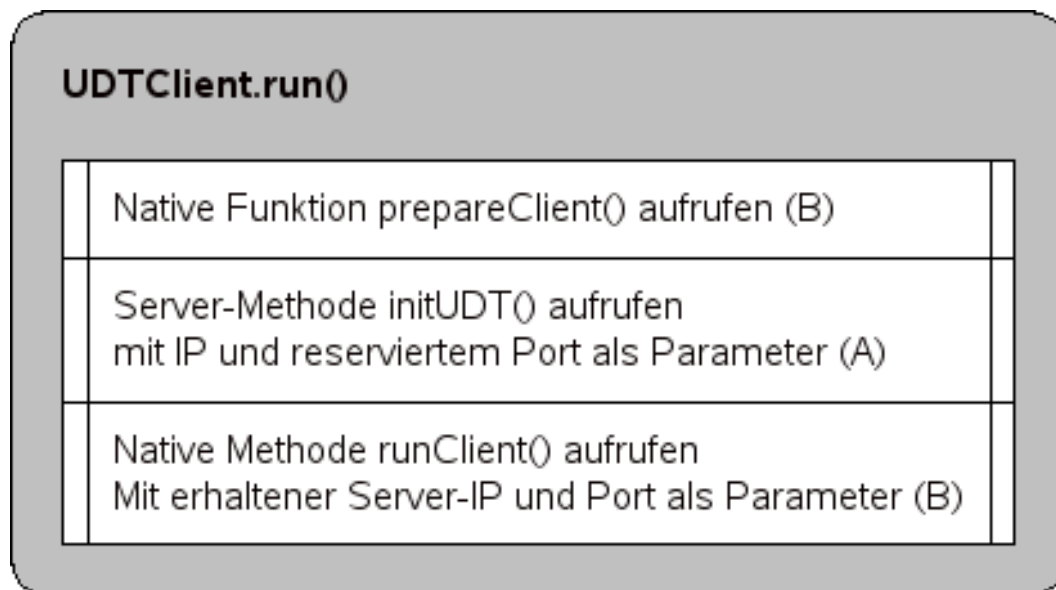
Abbildung 4.5: Methode UDTClient.run()
