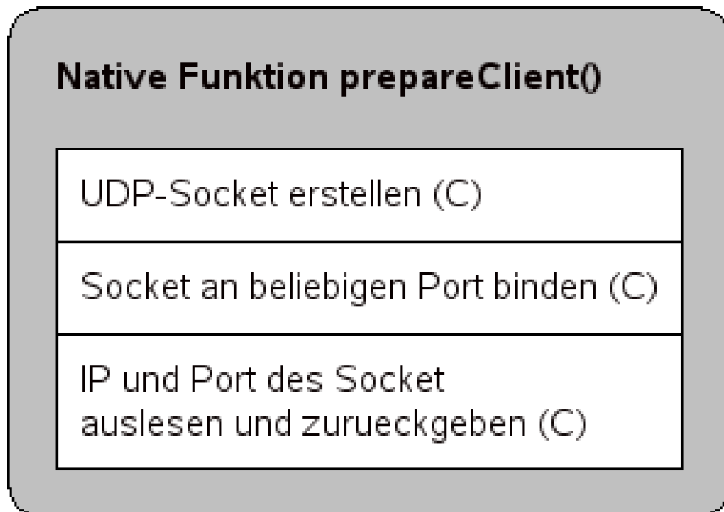
Abbildung 4.6: Funktion prepareClient()
