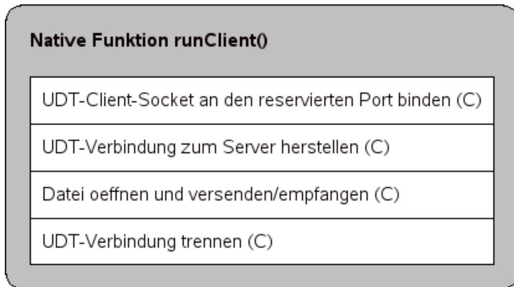
Abbildung 4.7: Funktion runClient()
