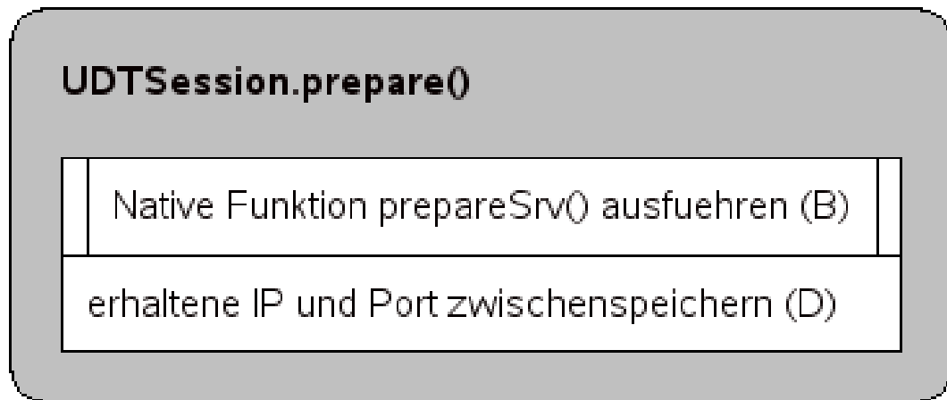
Abbildung 4.9: Methode UDTSession.prepare()
