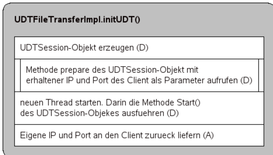
Abbildung 4.8: Methode UDTFileTransferImpl.initUDT()
