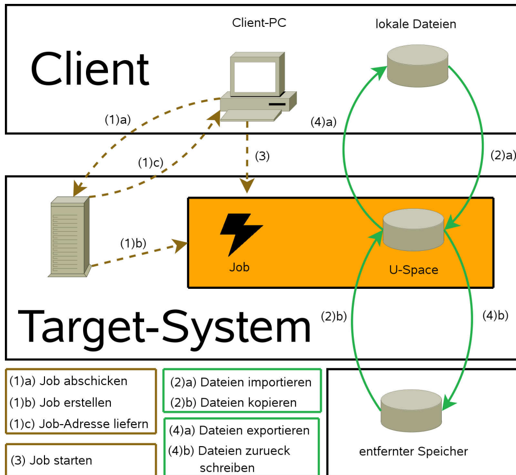
Abbildung 4.2: UNICORE Abläufe
