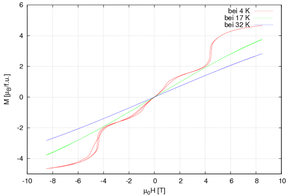
Abbildungung 32: Hysteresemessungen eines \text{TbMnO}_3 -Einkristalls im Bereich von -8.5 T bis 8.5 T. Das angelegte Magnetfeld lag parallel zur b -Orientierung. Es wurde bei den Temperaturen 4 K, 17 K und 32 K gemessen.
