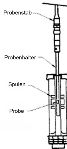
Abbildung 16: Skizze zum Aufbau des VSM, aus [26]
