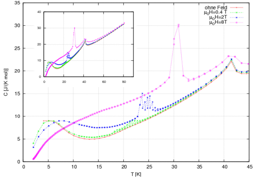
Abbildungung 24: Spezifische Wärmekapazität eines \text{GdMnO}_3 -Einkristalls bei verschiedenen Feldern parallel zur c -Orientierung. Das Fenster zeigt den Verlauf über den gesamten gemessenen Temperaturbereich von 2 bis 82 K.
