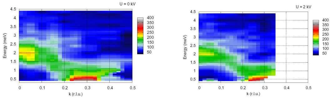
Abbildung 40: Farbplots der Energieüberträge bei unterschiedlichen Streuvektoren ( 0 \leq k \leq 1 ) bei 17 K. Die Farbskala deutet die Intensitäten an. Links ist die Messung ohne Feld zu sehen. Rechts ist die Messung bei einer angelegten Spannung von 2 kV dargestellt. Es wurde bei einem festen |\vec{k}_f| von 1.5 \text{ \AA}^{-1} gemessen.
