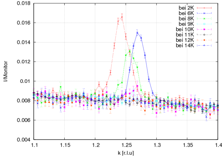
Abbildung 64: Temperaturabhängigkeit eines magnetischen Reflexes von \text{GdMnO}_3 . Der Streuvektor lautet (1 \ 1+q \ 0) , wobei q variiert wird. Es wurde bei einer Wellenlänge von 0.55 \text{ \AA} gemessen. Die Messungen oberhalb von 16 \text{ K} sind zur besseren Übersicht nicht mit eingezeichnet. Hier lag kein Reflex mehr vor.
