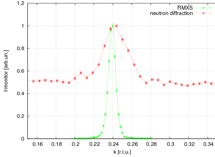
Abbildung 63: Vergleich der Intensität des (0 2+q 0)-Reflexes der resonanten Austauschstrahlung (RMXS) bei 4 K und der Intensität des (1 1+q 0)-Reflexes, der durch Neutronenbeugung bei 2 K gemessen wurde (neutron diffraction)
