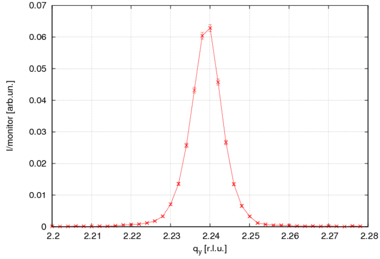
Abbildung 54: Messung eines magnetischen Reflexes bei dem Streuvektor (0\ 2+q\ 0) . Es wurde mit einer Energie von E = 7.934\text{ keV} bei 4\text{ K} gemessen.
