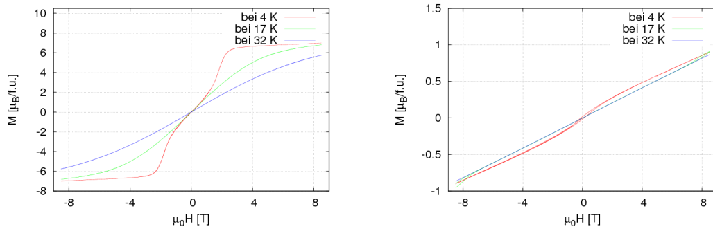
Abbildungung 32: Hysteresemessungen eines \text{TbMnO}_3 -Einkristalls im Bereich von -8.5 T bis 8.5 T. Das angelegte Magnetfeld lag parallel zur b -Orientierung. Es wurde bei den Temperaturen 4 K, 17 K und 32 K gemessen.
