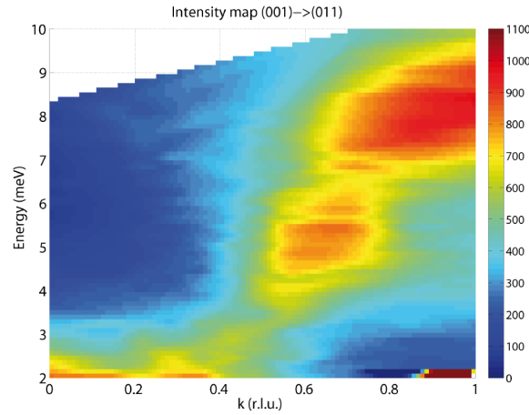
Abbildung 37: Farbplot der Abhängigkeit des Energieübertrages von dem Streuvektor (0\ k\ 1) . Die Farbskala zeigt die Intensitäten des Reflexes an. Diese Messungen wurden ohne elektrisches Feld und bei einer Temperatur von 17 K durchgeführt. Es wurde bei einem festen |\vec{k}_f| von 2.662\ \text{\AA}^{-1} gemessen.
