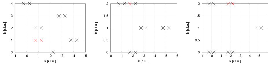
Abbildung 61: Messungen der Streuvektoren (h k 0) (links) und (h k 1) (Mitte) und (h k 2) (rechts). Die roten Kreuze bedeuten, dass hier ein Reflex gemessen wurde, ein schwarzes Kreuz bedeutet, dass kein Reflex bei diesem Streuvektor gefunden wurde. Es wurde bei einer Wellenlänge von 0.55 Å bei 2 K gemessen.
