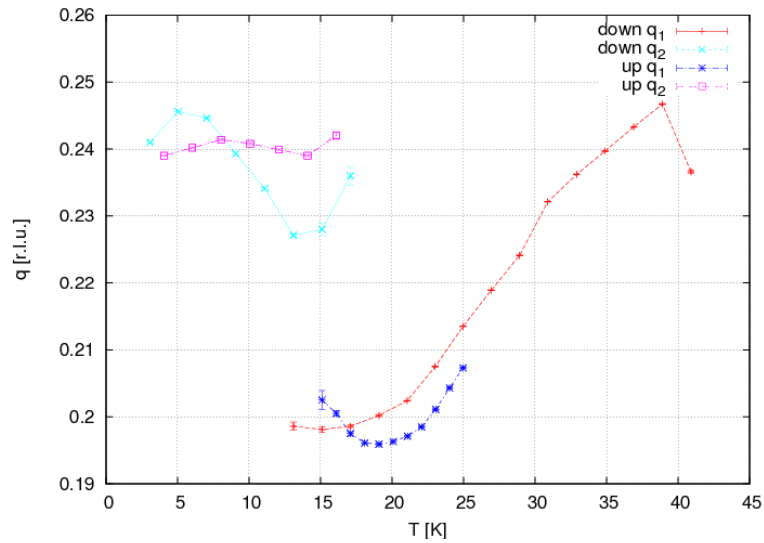
Abbildung 55: Positionen der Propagationsvektoren vom (0\ 2+q\ 0) -Reflex von \text{GdMnO}_3 . Es wurde bei der Energie E = 7.934\text{ keV} gemessen. Der Temperaturbereich ging von 3\text{ K} bis 42\text{ K} . Es wurde beim Aufheizen der Probe (up) und beim Abkühlen der Probe (down) gemessen. Ab 41\text{ K} konnten keine Reflexe mehr identifiziert werden.
