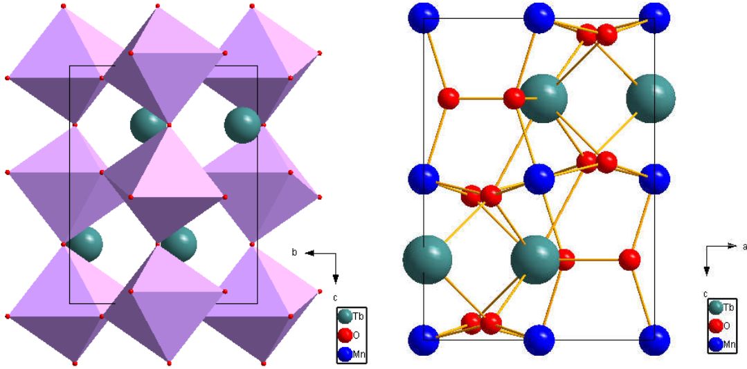
Abbildung 8: Einheitszelle von \text{TbMnO}_3
