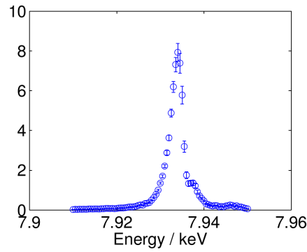
Abbildung 52: Absorptionskorrigierte Energieabhängigkeit des (0\ 2\text{+}q\ 0) -Reflexes bei T = 22\ \text{K} . Auf der y-Achse sind die Intensitäten in beliebigen Einheiten aufgetragen. Die Spitzen der Resonanz befinden sich bei E = 7.934\ \text{keV} und E = 7.937\ \text{keV} .
