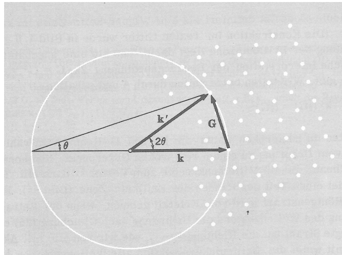
Abbildung 18: Ewald-Konstruktion, aus [27]
