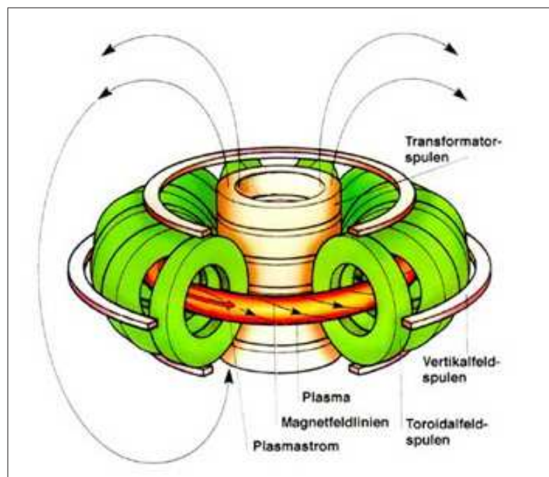
Abbildung 2.3: Das TOKAMAK-Prinzip (Quelle: www.euronuclear.org )
