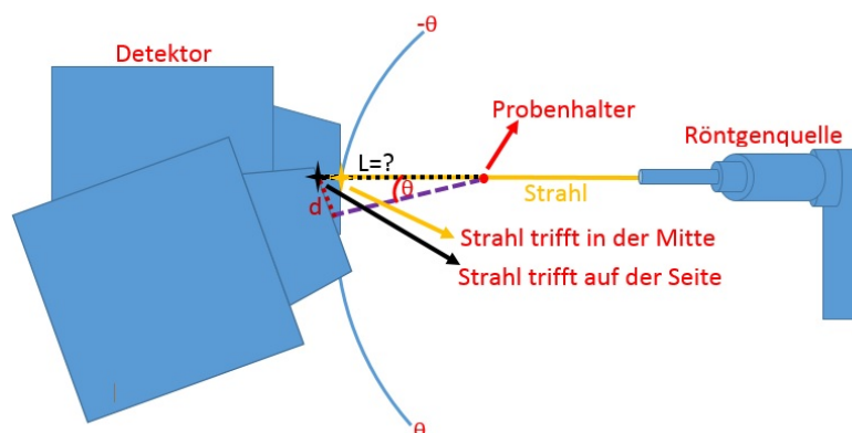
Abbildung 37: Messung des Abstands zwischen Probe und Detektor. Selbst gezeichnete Abbildung
