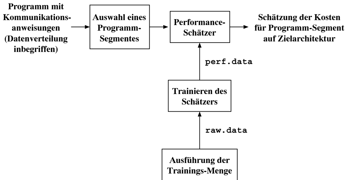
Abbildung 2.3: Performance-Schätzung in Fortran D
