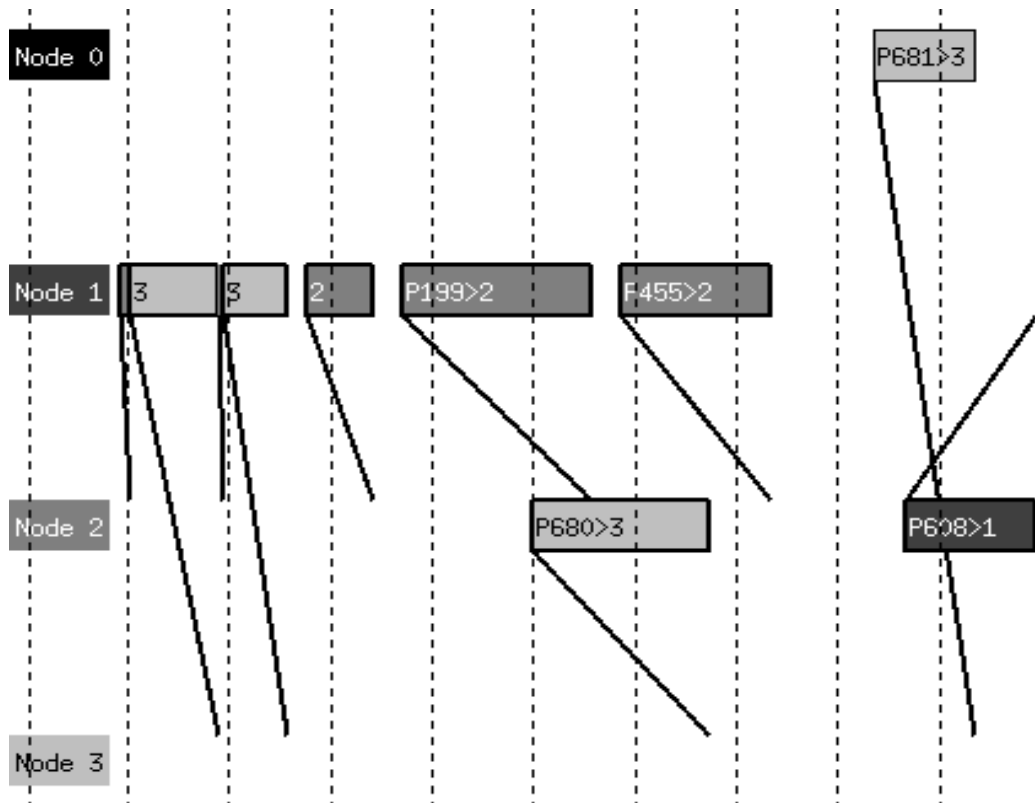
Abbildung 4.2: Kommunikationszeitlinien-Darstellung am Beispiel eines SVM-Fortran -Programms
