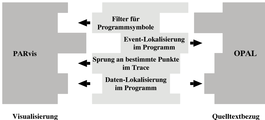
Abbildung 5.3: Konzept einer Schnittstelle zwischen PARvis und OPAL
