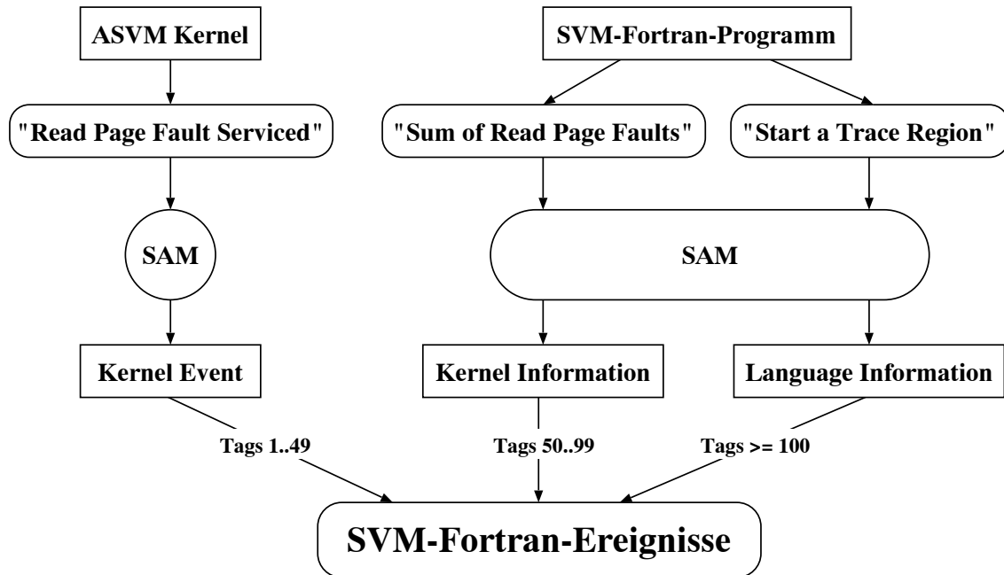
Abbildung 3.12: Übersicht über die Ereignis-Gruppen für SVM-Fortran
