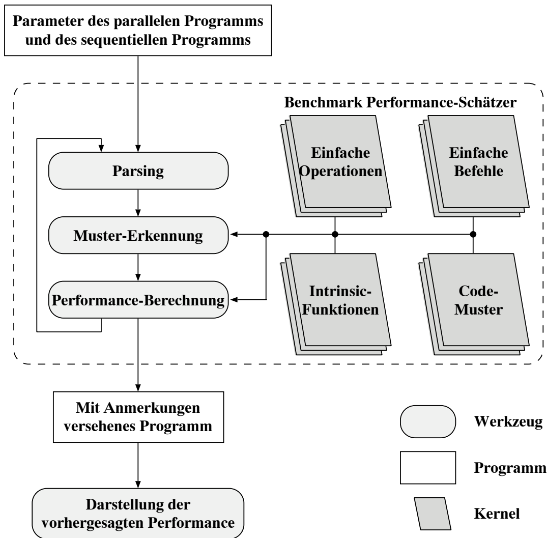
Abbildung 2.1: Performance-Vorhersage mit Benchmark-Kernel-Library
