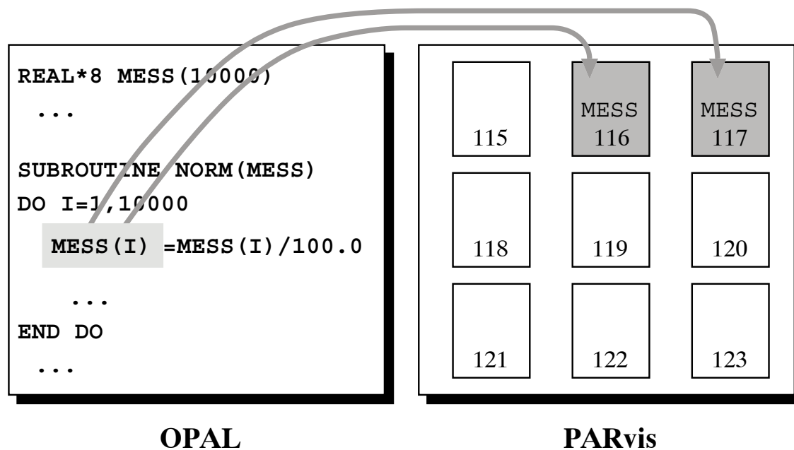
Abbildung 5.5: Lokalisierung von Variablen auf Speicherseiten
