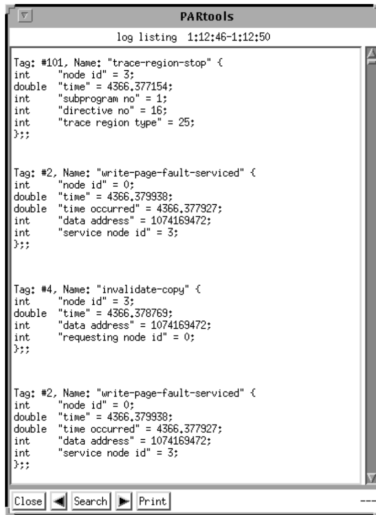
Abbildung 4.3: Anzeige von Ereignissen in ASCII-Form
