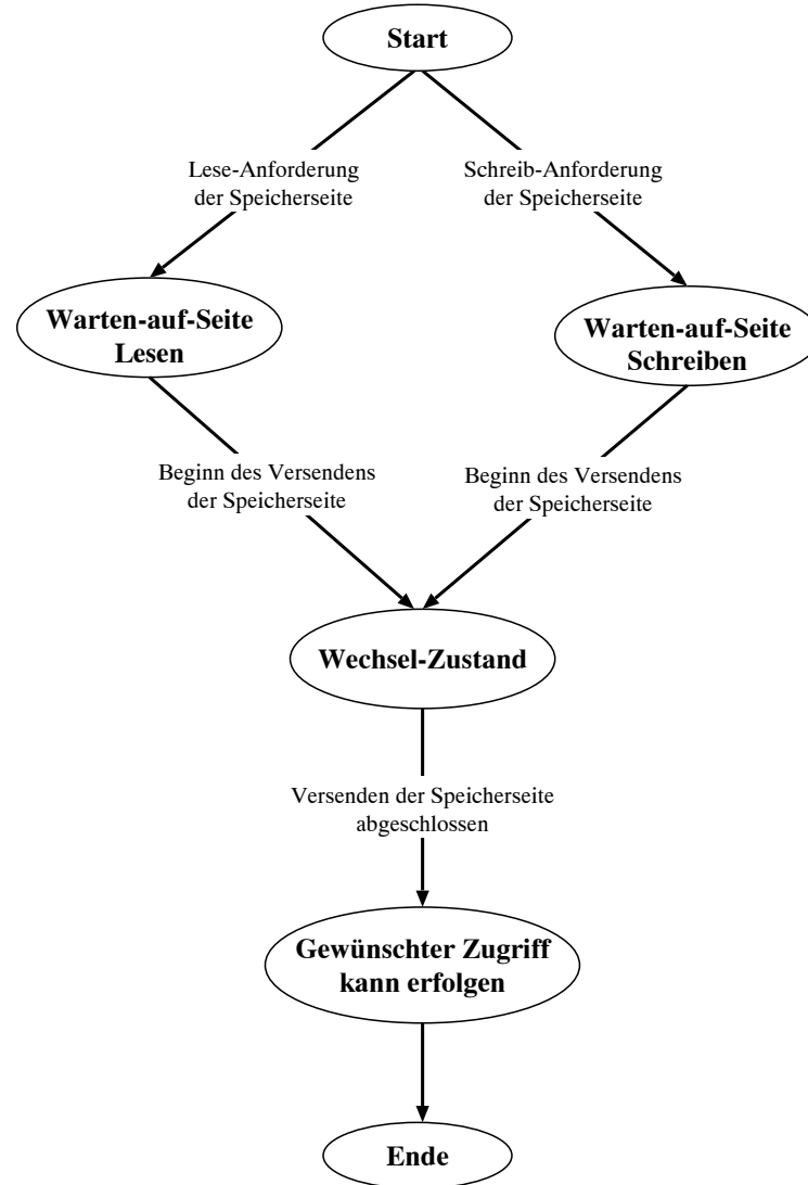
Abbildung 4.1: Zustandsübergänge beim Versenden einer Speicherseite
