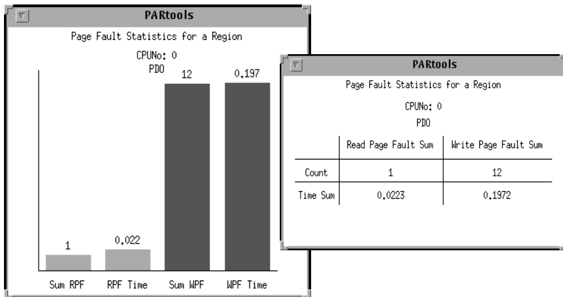
Abbildung 4.5: Darstellung von Summen-Ereignissen in PARvis
