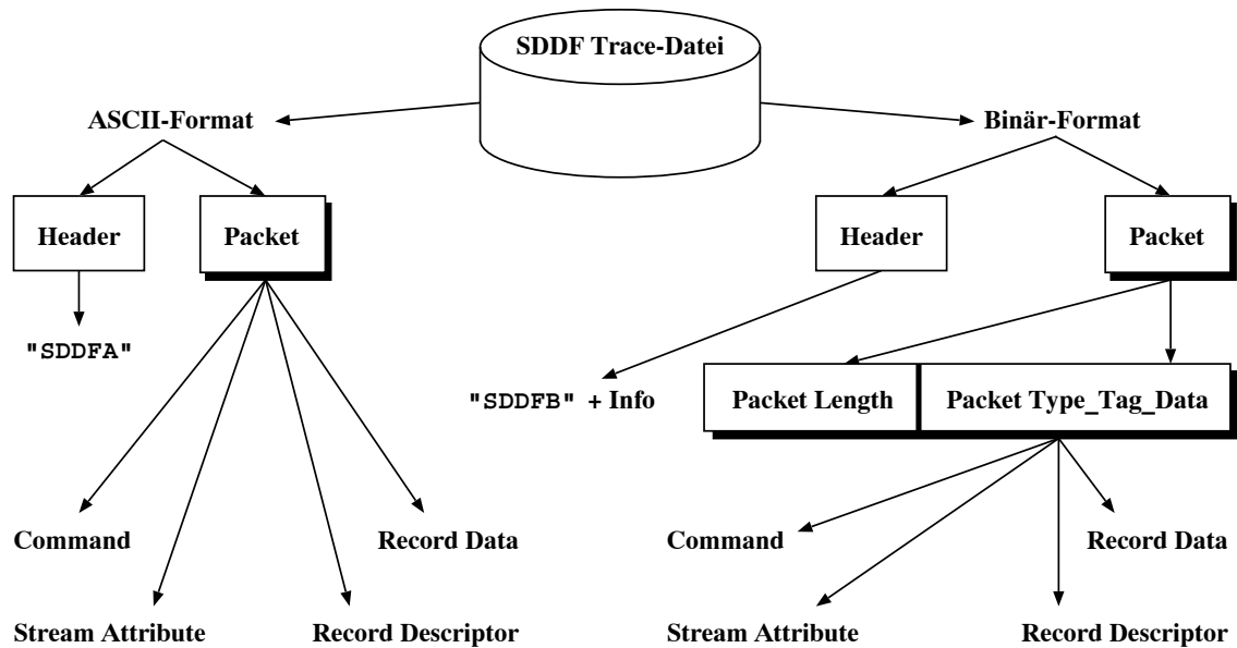
Abbildung 3.10: Übersicht über die SDDF-Grammatik
