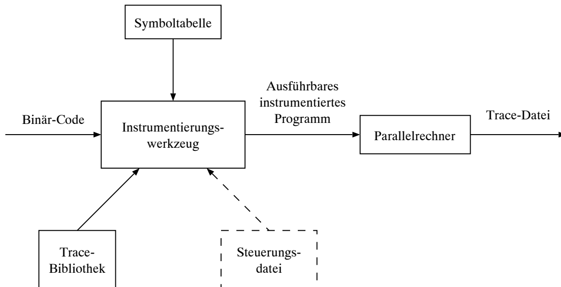
Abbildung 3.5: Instrumentierung auf Binär-Code Ebene
