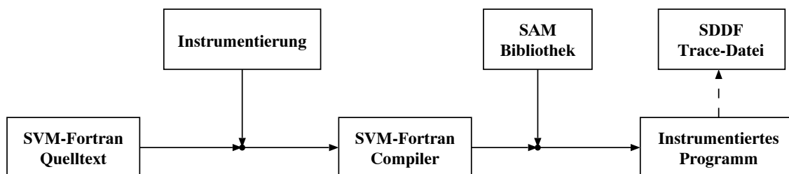
Abbildung 3.8: Erzeugung von Ereignissen mit dem SAM
