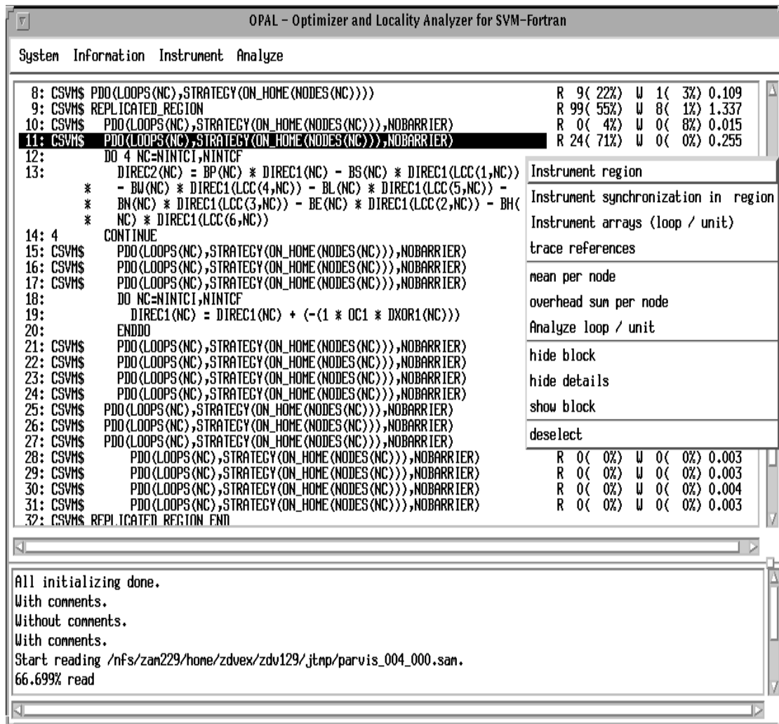
Abbildung 3.7: OPAL – Optimizer and Locality Analyzer für SVM-Fortran
