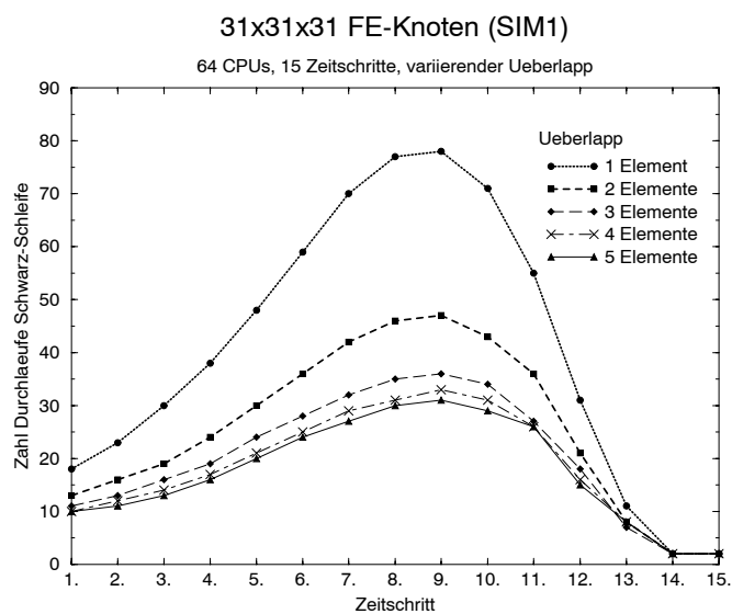
Abbildung 7.5: Zahl der Durchläufe der Schwarz-Schleife in Abhängigkeit des Überlapps und des Zeitschritts beim Einsatz von 64 Prozessoren
