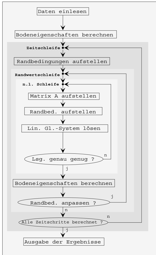
Abbildung 3.2: Sequentielle Struktur des Programms TRACE
