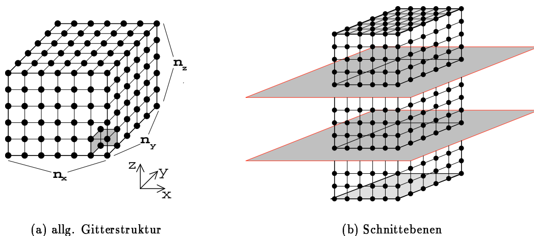
Abbildung 4.1: Das Finite-Elemente-Gitter
