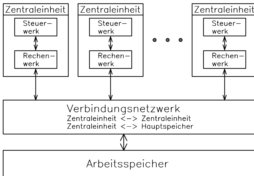
Abbildung 1.2: Prinzipieller Aufbau eines Parallelrechners
