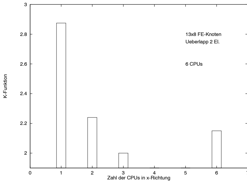
Abbildung 4.8: 2D-Beispiel: K-Funktion
