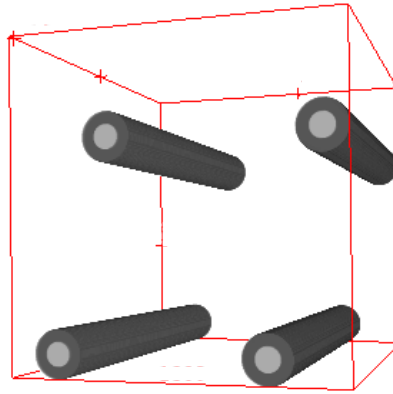
Abbildung 5.11.: 4 gerade horizontale Fasern für die die gekippte und ungekippte Simulation verglichen wurde.
