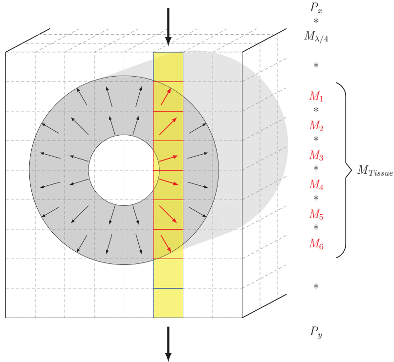
Abbildung 3.5.: Beispiel für den Jones Matrix Calculus anhand einer horizontalen Faser mit radialen optischen Achsen. Für jede der eingefärbten Würfel wird eine Matrix vom Typ 3.7 erstellt und in der abgebildeten Reihenfolge multipliziert. [2]
