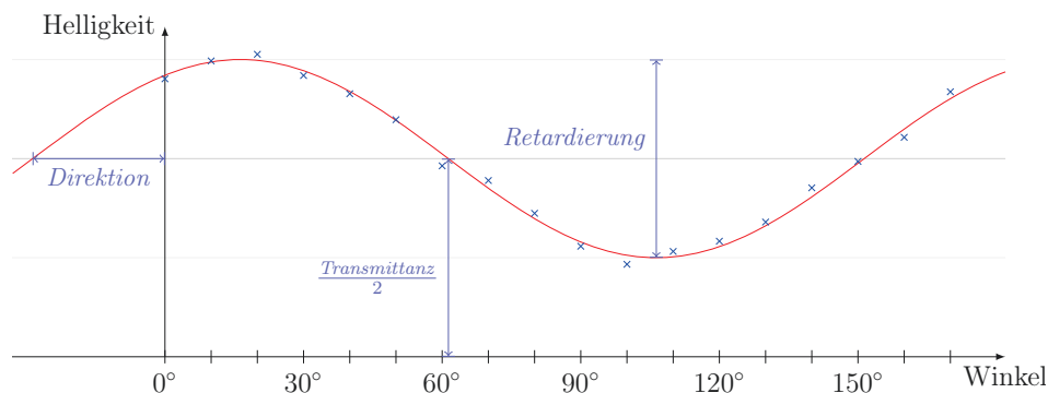
Abbildung 2.3.: Direktion, Transmittanz, Retardierung
