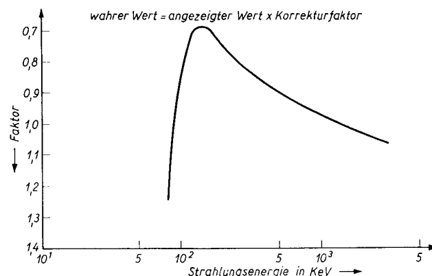
Bild 3: Energieabhängigkeit des Zählrohr-Gammadosisleistungsmessgerätes Graetz X 50
