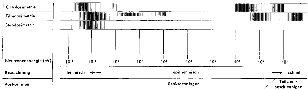
Bild 5: Derzeitiger Stand der Neutronendosimetrie (schematisch)
