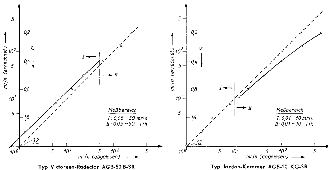
Bild 2: Kalibrierung von Ionisationskammer-Dosisleistungsmessern
