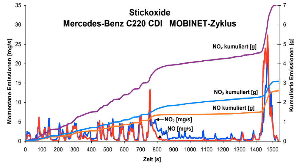
Abbildung 28: Stickoxid-Emissionen des Mercedes-Benz C220 CDI in einem Prüfstands-Zyklus („MOBINET-Zyklus“, aus: [Klemp et al., 2012]).
