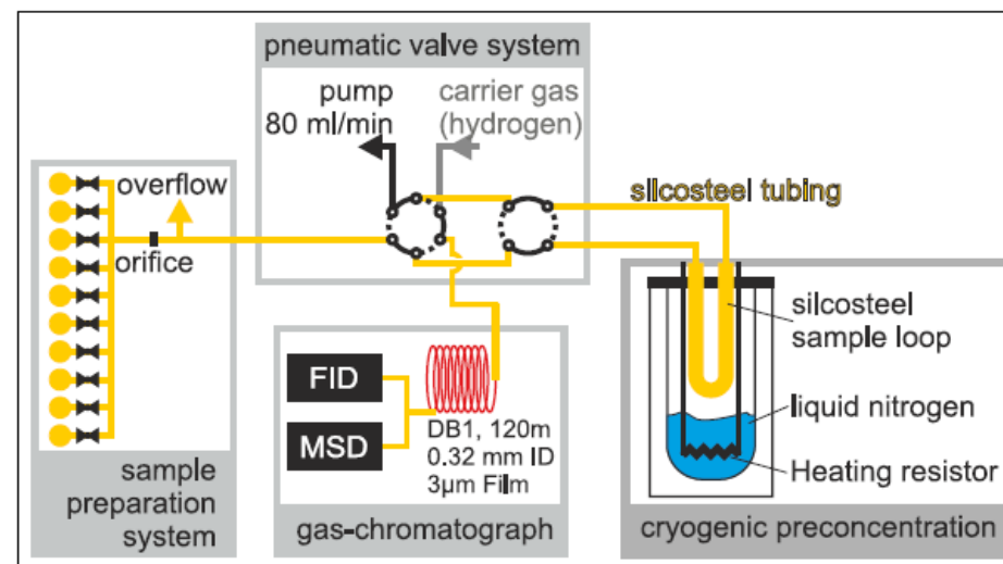
Abbildung 24: Schematischer Überblick des Jülicher GC/MS-Systems (aus: [Ehlers et al., 2015], welches sowohl zur Analyse von Außenluft-Proben als auch zur Abgasanalyse eingesetzt wird. Die Apparatur besteht aus einem Probenaufgabesystem (sample preparation system), einer kryogenen Anreicherung (cryogenic preconcentration), einem pneumatisch betriebenen Ventilsystem und dem eigentlichen Gaschromatografen, bestückt mit einer 120 m DB1-Säule mit 0.31 mm Durchmesser und einer Filmdicke von 3 µm.
