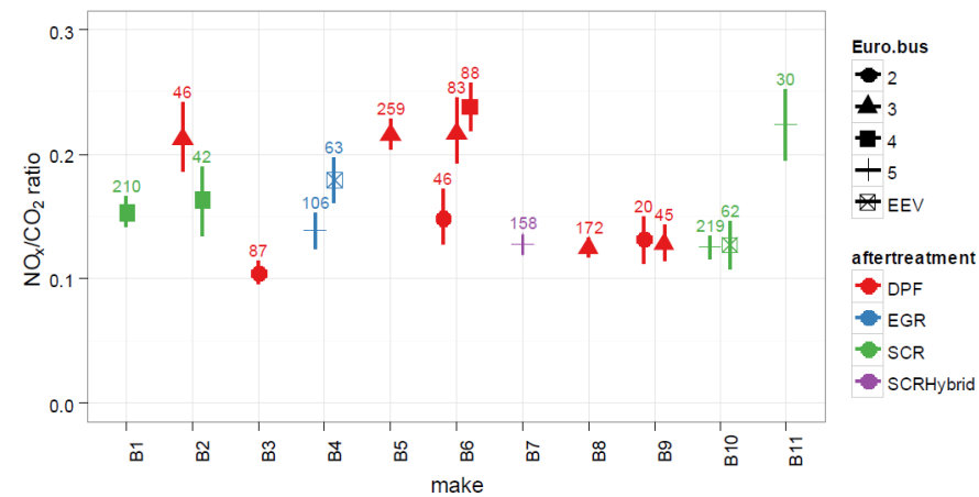
Abbildung 31: Auf den CO 2 -Ausstoß normierter NO x -Ausstoß von Stadtbussen unterschiedlicher EURO-Normen mit verschiedenen Abgas-Reinigungstechniken. Abkürzungen: B1,, B11: Untersuchte Busse; Euro.bus 2 – 5: EURO-Norm 2 bis EURO-Norm 5, EEV: Nachfolgestufe EURO-Norm-5, Spezifikationen siehe Tabelle 2; DPF: Diesel-Partikelfilter, EGR: Abgas-Rückführung zur Reduzierung des NO x -Ausstoßes im Abgas, SCR: Stickoxid-Reduktion mittels Harnstoff-Beimengung, SCRHybrid: SCR-Technik bei Verwendung eines Diesel-Hybrid-Fahrzeuges, aus: [Carslaw et al., 2013].
