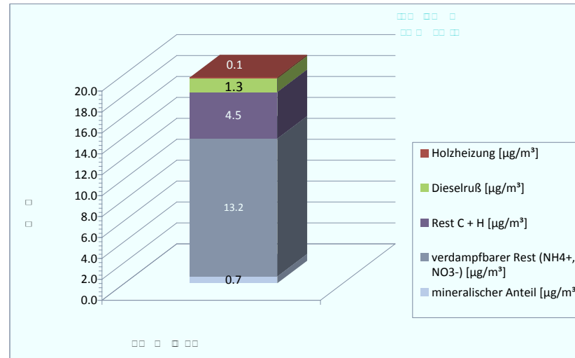
Abbildung 19: Speziation der PM-10-Filtersammlung am Kurpark im November 2014. Nicht detektierbar war die Feinstaubquelle Ölheizung, der Beitrag der Reifenabrieb lag bei weniger als 0.02 µg/m³.
