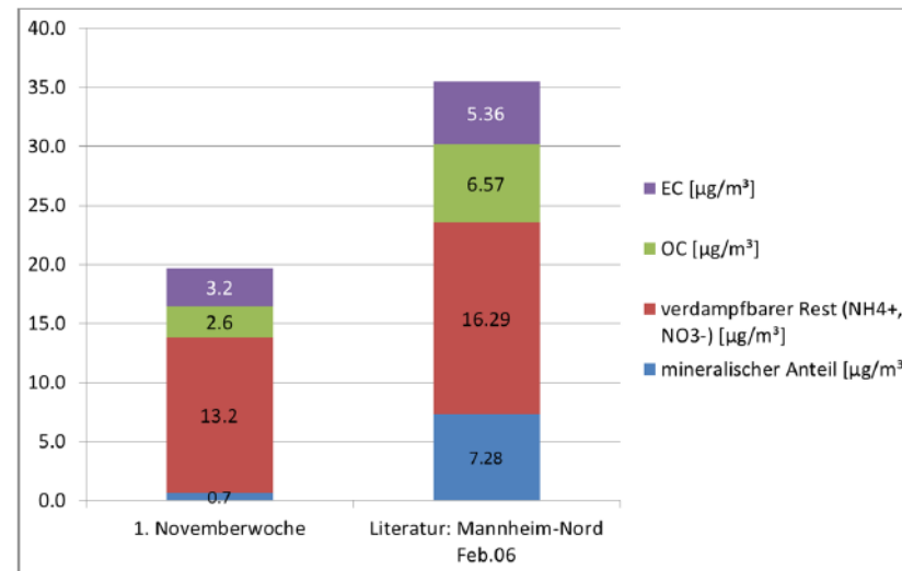
Abbildung 20: Speziation der PM-10-Filtersammlung am Kurpark im November 2014. Vergleich mit Resultaten aus städtischer Umgebung in Mannheim-Nord im Winter 2006 [Einflussgrößen auf die zeitliche und räumliche Struktur der Feinstaubkonzentrationen" (LUBW 2007)]. Für die bessere Vergleichbarkeit wurden die in Abb. 19 dargestellten Resultate auf die in der Literatur gewählten Kategorien umgerechnet.
