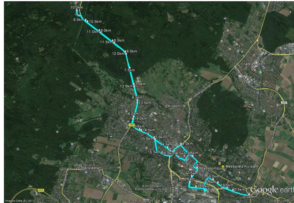
Abbildung 10: Teststrecke für die NO x -Chasing-Experimente unter realen Betriebsbedingungen. Länge der Strecke: 19.5 km, tiefster Punkt der Strecke: U-Bahn Haltepunkt Bad Homburg (151 m), höchster Punkt: Saalburg (416 m).
