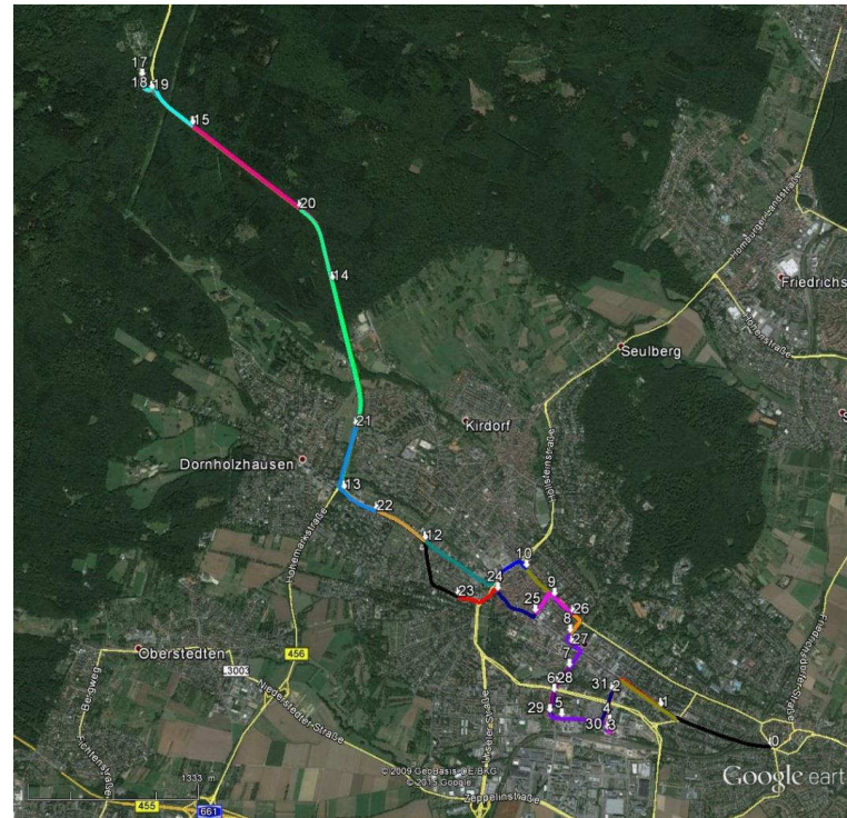
Abbildung 46: Eingefärbte Streckenabschnitte der Teststrecke für den EURO-5-Gelenk-Bus „Vollgas“. Die Einfärbungen der 100-s-Streckenabschnitte entsprechen denen der Farbskala der „Box-and-Whisker“-Plots. Zusätzlich wurde die Abfolge der 100-s-Streckenabschnitte in aufsteigender Reihenfolge nummeriert; die dargestellten „Box-and-Whisker“-Plots sind in gleicher Reihenfolge dargestellt.
