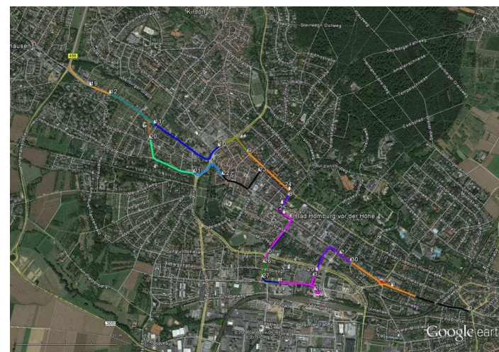
Abbildung 33: Eingefärbte Streckenabschnitte der Teststrecke für den EURO-6-Bus „Normalbetrieb“. Die Einfärbungen der 100-s-Streckenabschnitte entsprechen denen der Farbskala der „Box-and-Whisker“-Plots. Zusätzlich wurde die Abfolge der 100-s-Streckenabschnitte in aufsteigender Reihenfolge nummeriert; die dargestellten „Box-and-Whisker“-Plots sind in gleicher Reihenfolge dargestellt.
