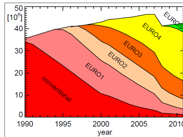
Abbildung 52: EURO-Normen-Anteile für Pkw in Deutschland in den Jahren zwischen 1990 und 2010 (aus: Ehlers et al. 2015).
