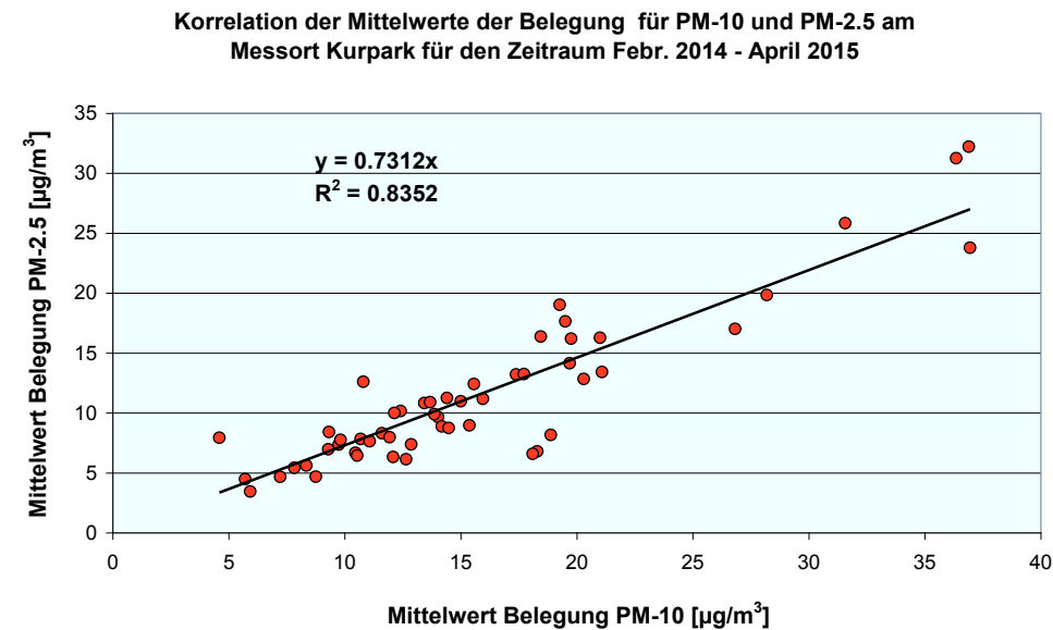
Abbildung 14: Korrelation der Mittelwerte der Belegung für die parallel durchgeführten PM-10- und PM-2.5 Feinstaubsammlungen. Im Mittel ist das Tagesmittel für PM-10 um 27 % größer als das für PM-2.5. Die Korrelation zwischen beiden Messserien hat ein hohes R^2 von 0.835.
