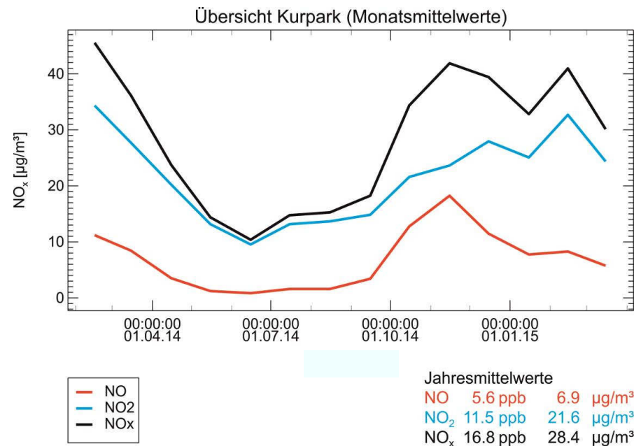
Abbildung 11: Jahresgang der Stickoxide (Monatsmittel) am Messplatz Kurpark. Zusätzlich angegeben sind die Jahresmittel für NO, NO 2 und NO x in ppb und µg/m 3 für den Zeitraum Febr. 2014 – Febr. 2015.
