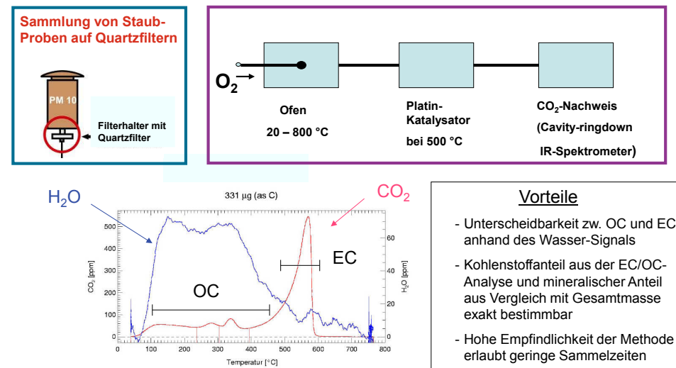
Abbildung 2: Prinzipskizze der EC/OC-Apparatur zur Analyse der organischen Fraktion von Feinstaubproben in sauerstoffhaltigem Betriebsgas. Ofen mit innenliegendem Quarzrohr; Pt-Katalysator zur Umwandlung der gasförmigen organischen Phase zu CO 2 ; Flusssteuerung der Betriebsgase; Cavity-ringdown-Spektrometer zum Nachweis des im Katalysator gebildeten CO 2 .
