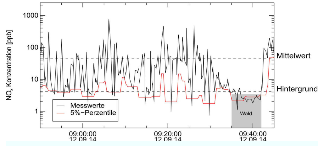
Abbildung 8: Konzentrationsprofil für die zeitlich hochauflösende Messung von \text{NO}_x während der Messfahrt in Bad Homburg vom 12. 09. 2014. Die gemessenen Stickoxidkonzentrationen variieren um nahezu zwei Größenordnungen, abhängig davon, ob sich das Messfahrzeug im Nahbereich voranfahrender Kfz befindet oder ob es bei der Befahrung eines stadtnahen Waldweges allein durch das vorgelagerte Waldgebiet bewegt. Es ist bemerkenswert, dass die \text{NO}_x -Konzentrationen im nah benachbarten Waldgebiet auf atmosphärische Hintergrundwerte von 2 - 3 ppb absinken (Wind aus 340 – 360 °). Diese Beobachtung macht deutlich, dass der regionale Beitrag von \text{NO}_x bei nördlichen Windrichtungen sehr gering ist. Zusätzlich dargestellt ist der Mittelwert der gemessenen \text{NO}_x -Konzentrationen (Mittelwert) sowie der Mittelwert der niedrigsten 5%-Perzentile (Hintergrund). Die Differenz beider Mittelwerte ist ein Maß für die maximal erreichbare Reduktion bei Sperrung des jeweiligen Straßenbereiches.
