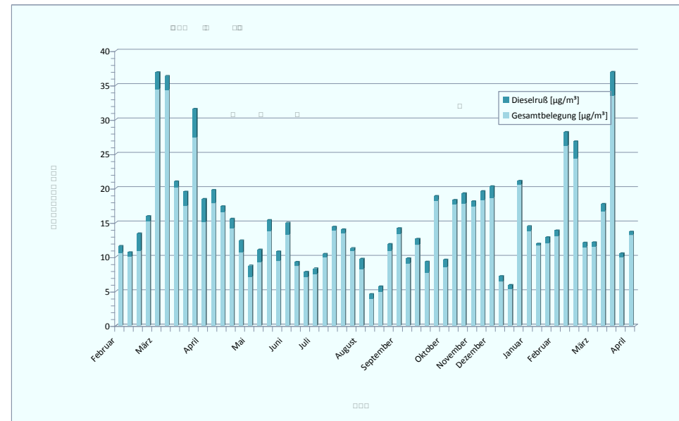
Abbildung 15: Wochenmittel der PM-10-Filtermessungen an der Dauermessstelle Kurpark. Der Jahresmittelwert der PM-10-Filterproben liegt bei 15.4 \mu\text{g}/\text{m}^3 . Der Jahresmittel des Dieselrußbeitrags wurde zu 1.2 \mu\text{g}/\text{m}^3 bestimmt (Methodik vgl. Abschnitt 4 a).
