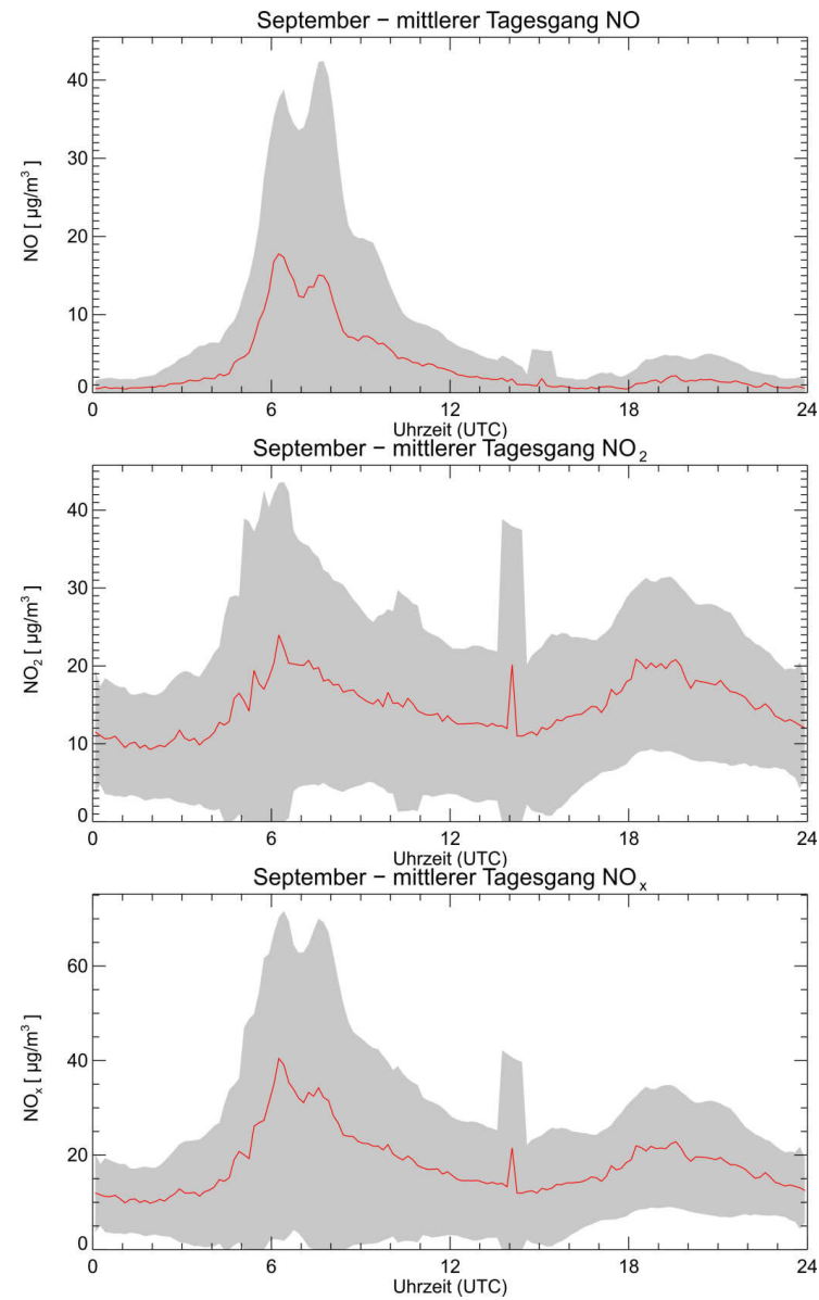
Abbildung 12: Mittlerer Tagesgang der Stickoxide (NO, NO 2 und NO x ) im Monat September am Messort „Kurpark“. Die grauen Flächen geben die Standardabweichungen für die gemittelten Tagesgänge wieder. Die Uhrzeit ist in Coordinated Universal Time (UTC) angegeben. Bei der Umrechnung auf MESZ sind 2 Stunden zu UTC zu addieren.
