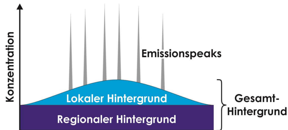
Abbildung 6: Zusammensetzung der Schadstoffkonzentration in städtischer Umgebung: Regionaler Hintergrund: Beitrag der umgebenden Emissionsquellen (Städte, benachbarte Autobahnen und Fernstraßen, usw.) auf regionaler Ebene; Lokaler Hintergrund: Mittelwert in städtischer Umgebung nach erfolgter Durchmischung; Emissionspeaks: Emissionspeaks einzelner vorausfahrender Emittenten, welche auf dem Gesamthintergrund aufsetzen. [nach: Lenschow et al., 2001]
