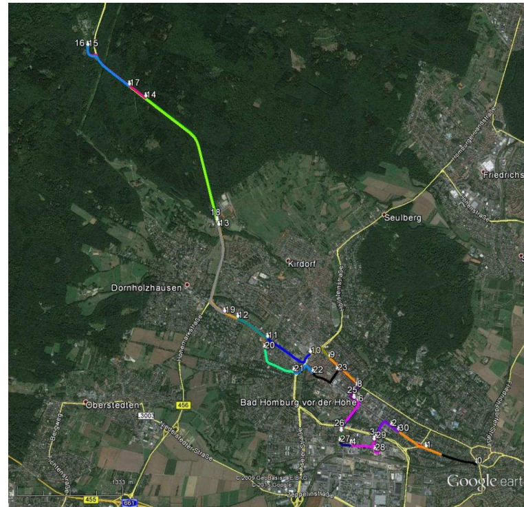
Abbildung 33: Eingefärbte Streckenabschnitte der Teststrecke für den EURO-6-Bus „Normalbetrieb“. Die Einfärbungen der 100-s-Streckenabschnitte entsprechen denen der Farbskala der „Box-and-Whisker“-Plots. Zusätzlich wurde die Abfolge der 100-s-Streckenabschnitte in aufsteigender Reihenfolge nummeriert; die dargestellten „Box-and-Whisker“-Plots sind in gleicher Reihenfolge dargestellt.
