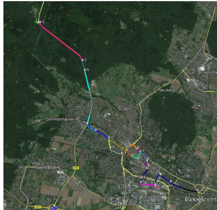
Abbildung 37: Eingefärbte Streckenabschnitte der Teststrecke für den EURO-6-Bus „Vollgasfahrt“. Die Einfärbungen der 100-s-Streckenabschnitte entsprechen denen der Farbskala der „Box-and-Whisker“-Plots. Zusätzlich wurde die Abfolge der 100-s-Streckenabschnitte in aufsteigender Reihenfolge nummeriert; die dargestellten „Box-and-Whisker“-Plots sind in gleicher Reihenfolge dargestellt.
