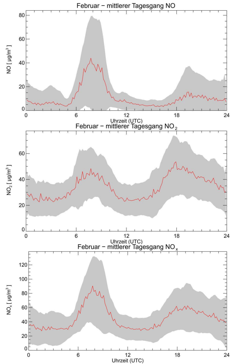
Abbildung 13: Mittlerer Tagesgang der Stickoxide (NO, NO 2 und NO x ) im Monat Februar am Messort „Kurpark“. Die grauen Flächen geben die Standardabweichungen für die gemittelten Tagesgänge wieder. Die Uhrzeit ist in Coordinated Universal Time (UTC) angegeben. Bei der Umrechnung auf MEZ ist 1 Stunde zu UTC zu addieren.
