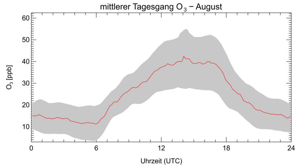
Abbildung 29: Mittlerer Tagesgang von Ozon sowie die zugehörige Standardabweichungen für den Monat August am Messort „Kurpark“. Weiterhin ist erkennbar, dass das unterhalb der nächtlichen Inversionsschicht vorhandene Ozon durch nächtliche NO-Emissionen nicht vollständig heraus“titriert“ wird (und somit für die unterhalb der nächtlichen Inversion vorhandenen NO-Mischungsverhältnisse gleiche NO 2 -Mischungsverhältnisse gebildet werden).
