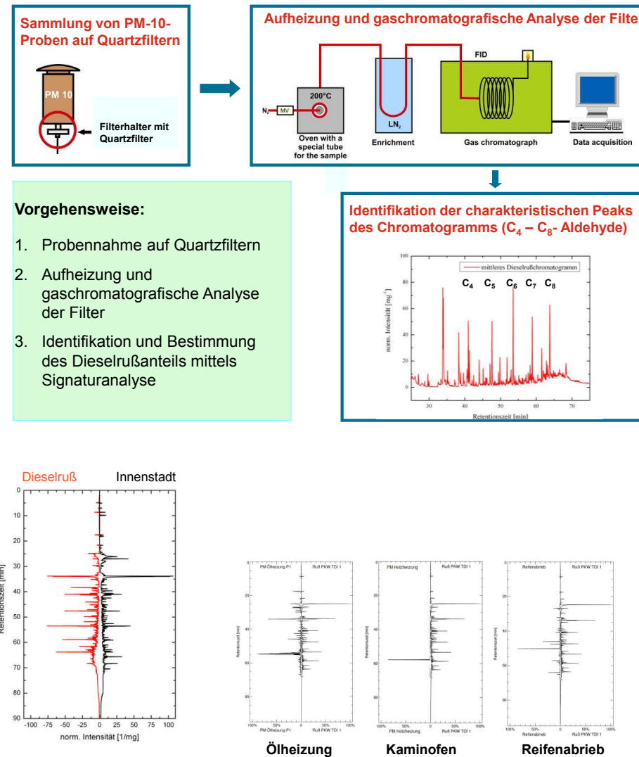
Abbildung 3: Beschreibung der Vorgehensweise zur Verursacheridentifikation in Feinstaubproben:
