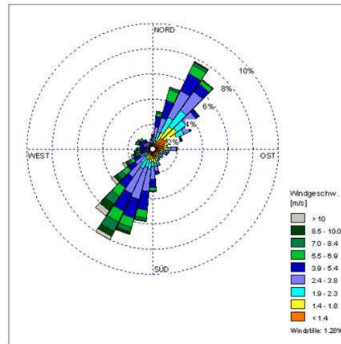
Abbildung 21: Windrichtungs- und Windgeschwindigkeitsverteilung für den nur wenige km von der Stadt Bad Homburg entfernten Flughafen Frankfurt. [Quelle: TÜV: Ausbau Flughafen Frankfurt Main, Gutachten G15.2, 2006].
