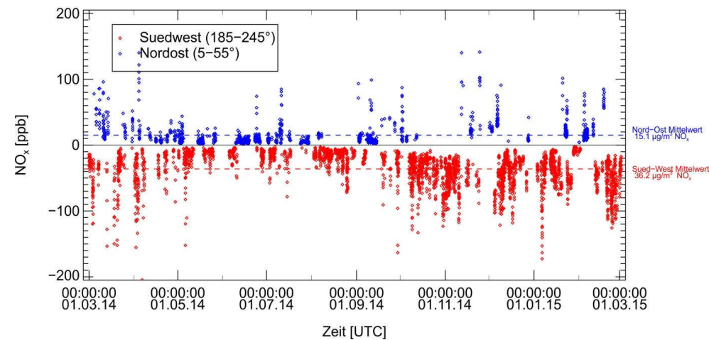
Abbildung 22: Halbstundenmittel der \text{NO}_x -Konzentrationen für die beiden Haupt-Windrichtungen Südwest (185 - 245°) und Nordost (5 - 55°) für den Messzeitraum 01.03.2014 – 01.03.2015. Im Jahresmittel ist der \text{NO}_x -Mittelwert für den Nordost-Sektor (Mittelwert: 15.1 \mu\text{g}/\text{m}^3 ) um den Faktor 2.4 niedriger als der des Südwest-Sektors (36.2 \mu\text{g}/\text{m}^3 ).
