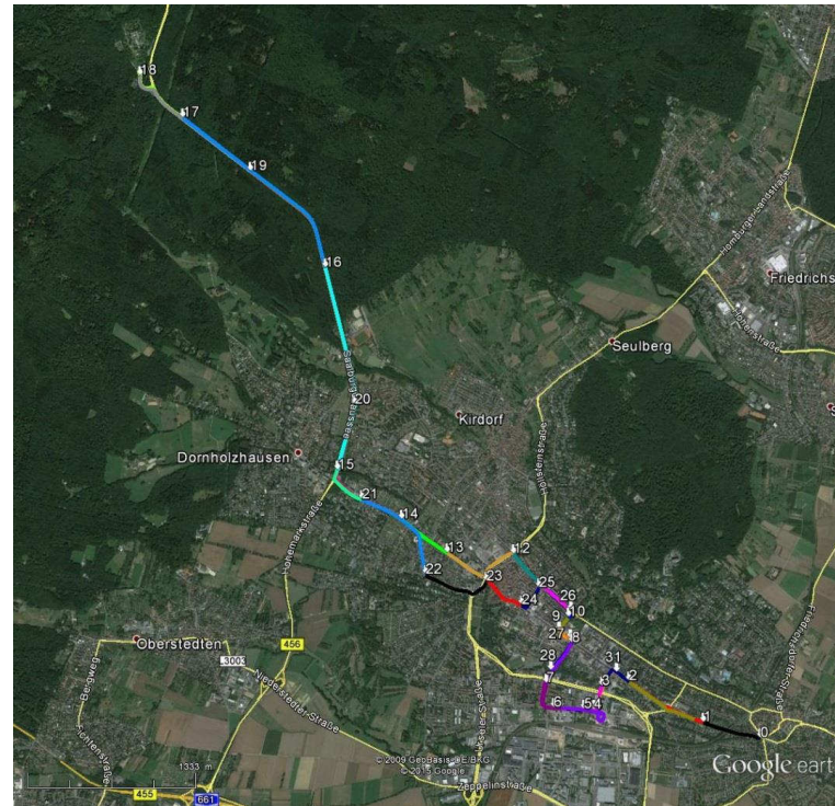
Abbildung 42: Eingefärbte Streckenabschnitte der Teststrecke für den EURO-5-Gelenk-Bus „Normalbetrieb“. Die Einfärbungen der 100-s-Streckenabschnitte entsprechen denen der Farbskala der „Box-and-Whisker“-Plots. Zusätzlich wurde die Abfolge der 100-s-Streckenabschnitte in aufsteigender Reihenfolge nummeriert; die dargestellten „Box-and-Whisker“-Plots sind in gleicher Reihenfolge dargestellt.
