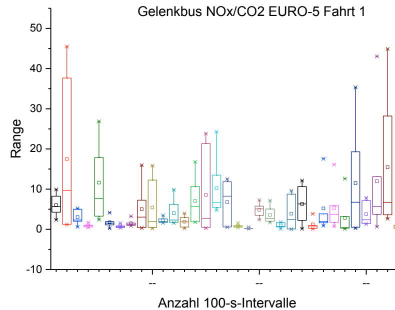
Abbildung 45: Box-and-Whisker-Plot für \text{NO}_x/\text{CO}_2 -Verhältnisse in [ppb/ppm] für einzelne 100-s-Intervalle der Messfahrt des EURO-5-Gelenk-Busses „Normalbetrieb“)
