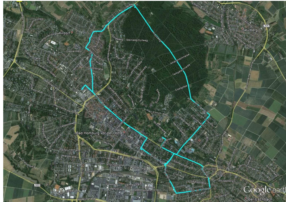
Abbildung 7: Fahrtroute von MOBILAB (12. 09. 2014) zur Untersuchung der innerstädtischen Verkehrsbelastung durch Stickoxide und Feinstaub. Derartige episodische Befahrungen des Stadtgebietes mittels MOBILAB wurden über den gesamten Untersuchungszeitraum zu unterschiedlichen Tageszeiten und Anströmbedingungen vorgenommen. Wesentliche Untersuchungsziele waren: Charakterisierung des typischen Emissionsverhaltens verschiedener Fahrzeugtypen (Pkw (Benziner), Pkw (Diesel), Lkw, Busse, ...), Beschreibung der vorgefundenen Hintergrundbelastung durch \text{NO}_x und Feinstaub bei systematischer Umfahrung des Stadtgebietes auf verkehrsarmen Umgehungsstraßen (vgl. z. B. Befahrung eines Waldweges ohne Straßenverkehr im nordöstlichen Vorfeld der Stadt).
