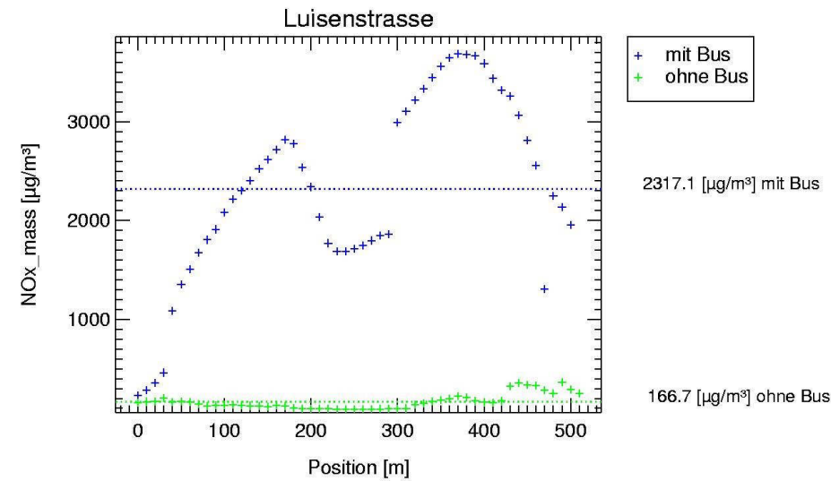
Abbildung 9: Gemittelte NO x -Konzentrationsprofile beim mehrfachen Durchfahren der Luisenstraße mit dem Startpunkt Europakreisel bis zur Kreuzung Ferdinandstraße/Luisenstraße. „Blau“: gemitteltes NO x -Konzentrationsprofil aufgenommen bei der „Verfolgung“ von Stadtbussen mit dem mobilen Messlabor. „Grün“: gemitteltes NO x -Konzentrationsprofil aufgenommen bei der „Verfolgung“ von Pkw's.
