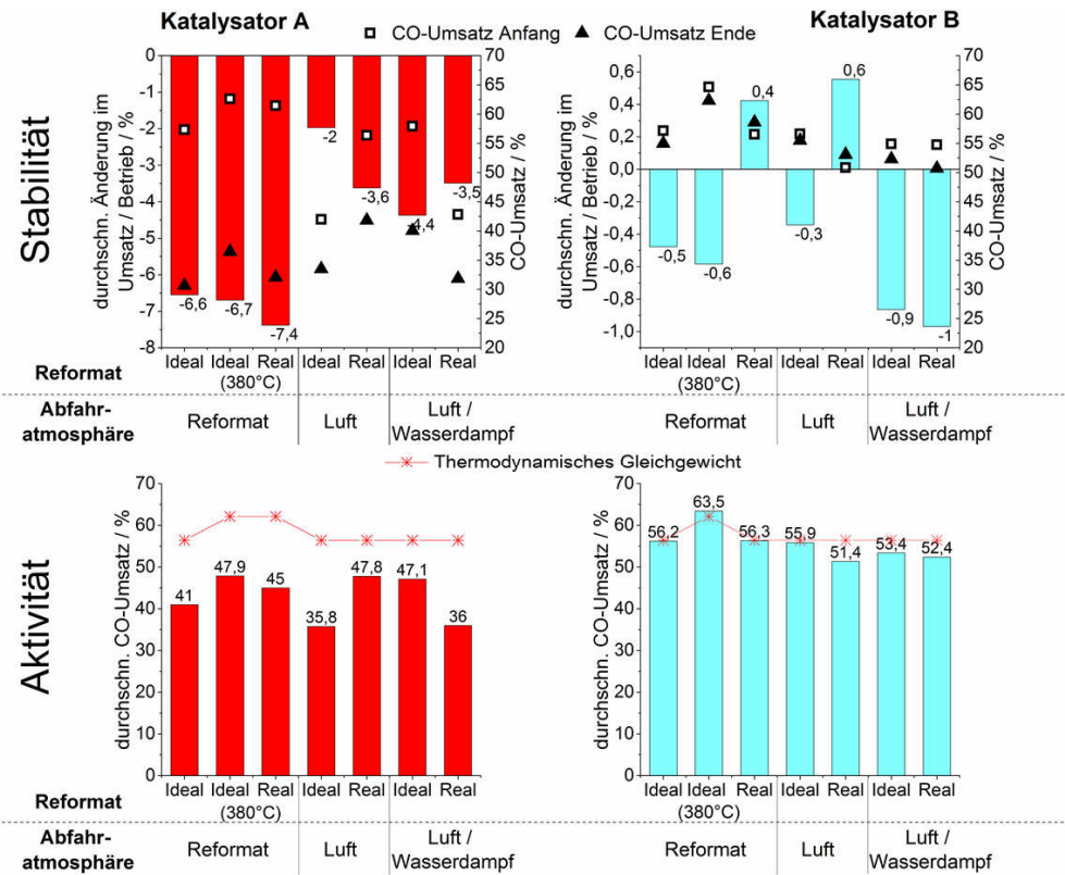
Abbildung 6.6: Stabilität und Aktivität der Katalysatoren A und B unter HTS-Bedingungen in Abhängigkeit der Reformatqualität und Abfahratmosphäre. Messwerte nach „Multigas™ 2030D“ und „Cirrus™ 2“. Nachgebildet aus [162] mit Genehmigung von Elsevier.
