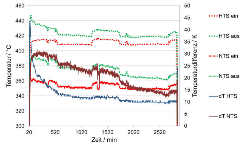
Abbildung 5.4: Typischer Verlauf der Katalysatoraktivität innerhalb des zweiten Teils der Testreihe mit Package 2. Als Beispiel wurde der Versuch 3 mit dem Kraftstoff Ultimate-Diesel gewählt.
