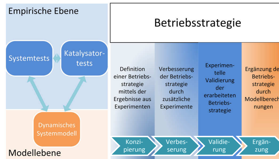
Abbildung 1.3: Methodische Vorgehensweise zur Konzipierung einer Betriebsstrategie für das Brenngaserzeugungssystem.
