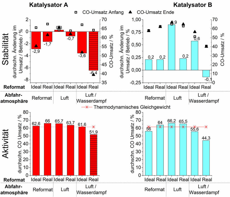
Abbildung 6.7: Stabilität und Aktivität der Katalysatoren A und B unter NTS-Bedingungen in Abhängigkeit der Reformatqualität und Abfahratmosphäre. Messwerte nach „Prima 600 S“ und „MultigasTM 2030D“ und „CirrusTM 2“. Nachgebildet aus [160] mit Genehmigung von ECS – The Electrochemical Society.
