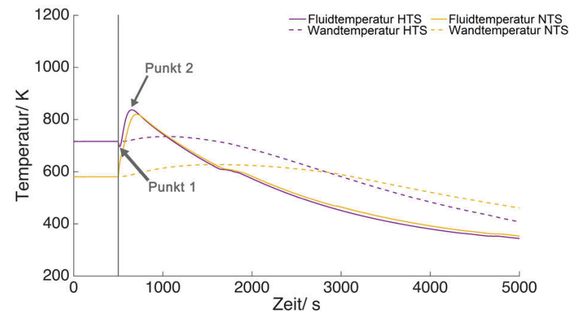
Abbildung 9.3: Fluid- und Wandtemperaturen im Wassergas-Shift-Reaktor während des Abfahrvorgangs. Als Spülmedium wurde Luft mit 20000\text{ l}_N/\text{h} gewählt.
