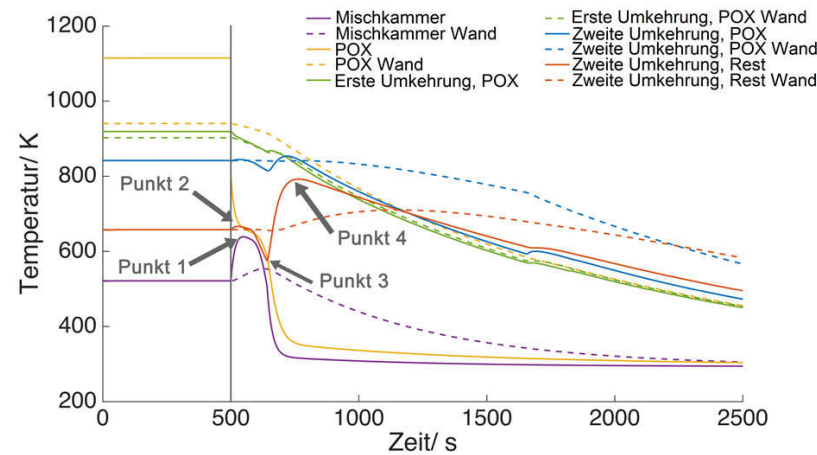
Abbildung 15.16: Fluid- und Wandtemperaturen im autothermen Reformer während des Abfahrvorgangs. Als Spülmedium wurde Wasserdampf mit 10000 g/h gewählt. Nach T_{krit} wurden 20000 l N /h Luft dem Reformer zugegeben.
