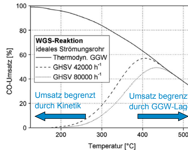
Abbildung 2.7: Gleichgewichtslage (GGW) und angepasste S-Kurven für ein ideales Strömungsrohr bei unterschiedlichen Raumgeschwindigkeiten in Abhängigkeit von der Temperatur [11]. Nachgebildet aus [63] mit Genehmigung von Elsevier.
