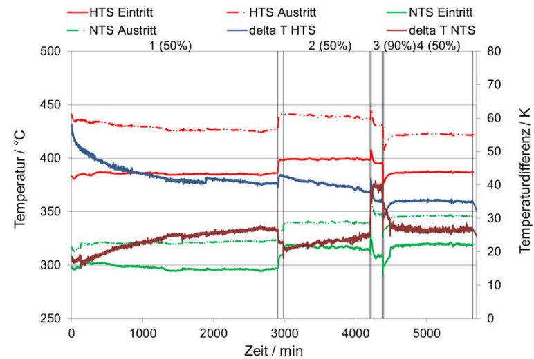
Abbildung 8.1: WGS-Temperaturen während des 100 h-Versuchs mit Katalysator B und NExBTL-Diesel. Die Degradation des WGS-Katalysators B konnte an einer sinkenden Temperaturdifferenz von anfänglich 58,2 K bis auf 40,4 K zum Ende der ersten Versuchsperiode identifiziert werden. Der linear angenäherte exponentielle Abfall der Temperaturdifferenz betrug 0,37 K/h. Gleichzeitig stieg die Kohlenmonoxidkonzentration hinter dem HTS-Reaktor von 3,5 Vol.-% auf 5,2 Vol.-% an. Die Reformeraustrittskonzentration hingegen variierte nur marginal zwischen 9,7 Vol.-% und 9,9 Vol.-%.
