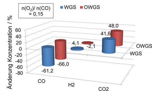
Abbildung 7.7: Durchschnittliche Änderung der Konzentrationen an CO, H 2 und CO 2 während des WGS- und OWGS-Betriebs mit Katalysator B. Es wurden HTS-Bedingungen und ein molares O 2 /CO-Verhältnis von 0,15 gewählt. Messwerte nach „Multigas™ 2030D“ und „Cirrus™ 2“.
