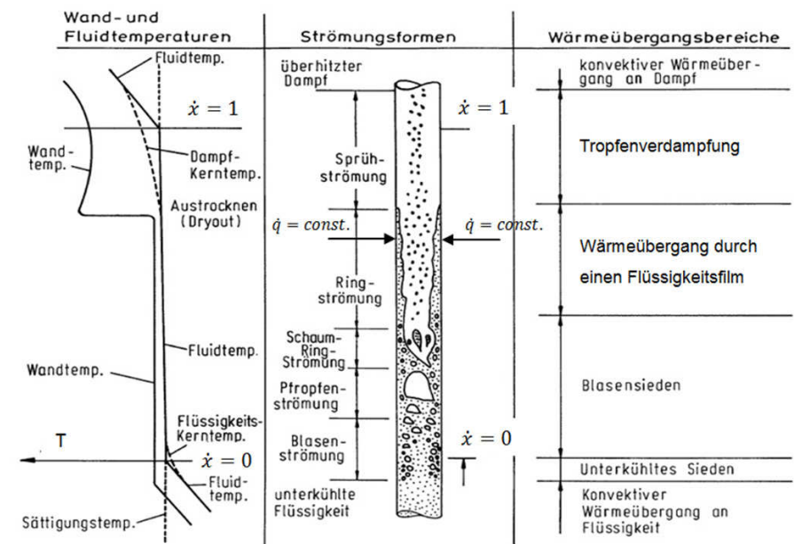
Abbildung 15.8: Wand- und Fluidtemperaturen, Strömungsformen und entsprechende Wärmeübergangsbereiche bei einem vertikal aufwärts durchströmten Rohr, nach [151].
