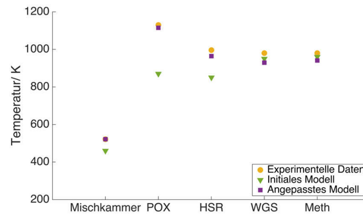
Abbildung 4.8: Vergleich der experimentell ermittelten und simulierten Temperaturen im autothermen Reformer bei stationärem Betrieb.
