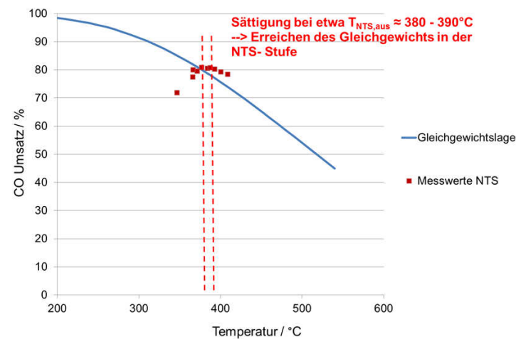
Abbildung 5.2: Bestimmung des optimalen Betriebspunkts für die NTS-Stufe bei bereits zum Teil deaktivierter HTS-Stufe.
