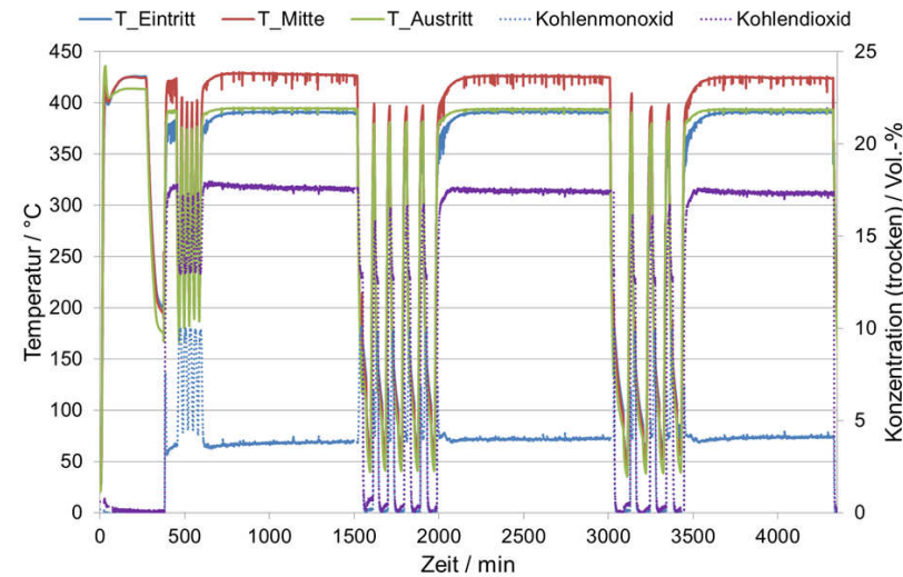
Abbildung 15.11: Stabilität von Katalysator B bei drei unterschiedlichen Temperaturzyklusintervallen. Betrieb unter HTS-Bedingungen und idealem Reformat. Messwerte nach „Multigas™ 2030D“ und „Cirrus™ 2“.
