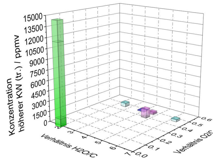
Abbildung 7.2: Maximalkonzentrationen höherer Kohlenwasserstoffe hinter dem ATR während des Abfahrens des Systems mit NExBTL. Farben: grün: klassische Strategie; blau: neue Strategie 1, magenta: neue Strategie 2; cyan: neue Strategie 3. Messwerte nach „Multigas™ 2030D“ und „Cirrus™ 2“. Nachgebildet aus [162] mit Genehmigung von Elsevier.
