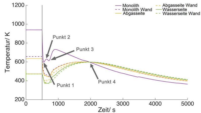
Abbildung 15.18: Fluid- und Wandtemperaturen im Katalytbrenner während des Abfahrvorgangs. Als Spülmedium wurde Wasserdampf mit 10000 g/h gewählt. Nach T_{krit} wurden 20000 l/h Luft dem Reformer zugegeben.
