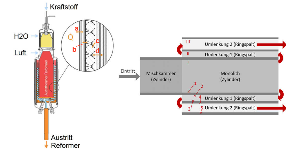
Abbildung 4.9: Abstraktion der Geometrie des autothermen Reformers ATR 9.2 und berechnete Wärmeübergänge im Modell.
