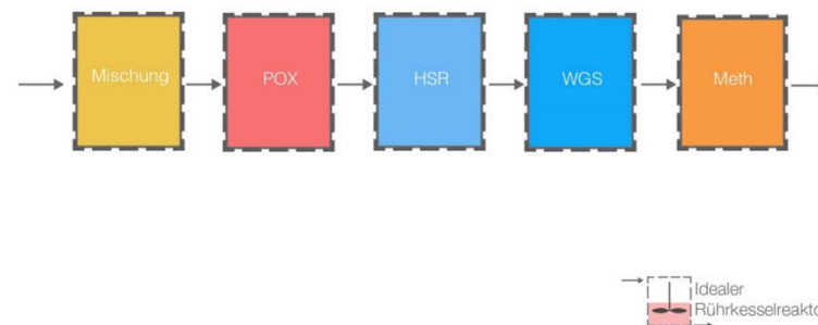
Abbildung 4.7: Initiales Reaktionsschema im autothermen Reformer.
