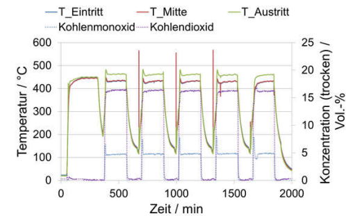
Abbildung 6.21: Stabiler Betrieb von Katalysator B trotz mehrfach hintereinander auftretenden Temperaturspitzen bis 560 °C. Messwerte nach „Multigas™ 2030D“ und „Cirrus™ 2“.
