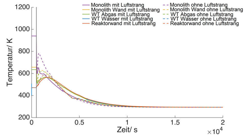
Abbildung 15.23: Verbesserung (a): kurze Abfahrdauer. Temperaturverläufe im Katalytbrenner. Im Fall mit zusätzlichem Luftstrang wurde zunächst mit 10000 l N /h Luft und 500 g/h Wasserdampf gespült. Nach T_{krit} wurden zusätzlich 10000 l N /h Luft hinzugegeben. Im Fall ohne zusätzlichen Luftstrang wurde von Anfang an mit 20000 l N /h Luft und 500 g/h Wasserdampf gespült. Nach T_{krit} wurde die Wasserzufuhr gestoppt.
