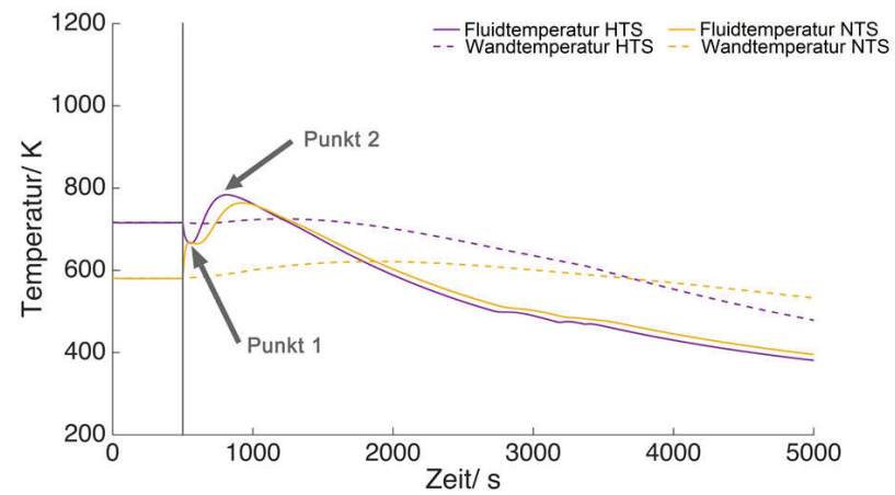
Abbildung 15.20: Fluid- und Wandtemperaturen im Wassergas-Shift-Reaktor während des Abfahrvorgangs. Als Spülmedium wurde Luft/ Wasserdampf mit 10000 l N /h Luft und 10000 g/h Wasserdampf gewählt. Nach T_{krit} wurde die Wasserdampfzufuhr unterbunden.
