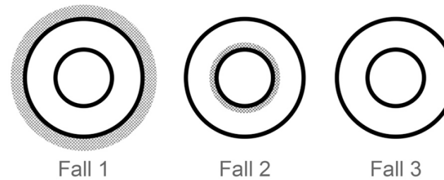
Abbildung 15.7: Fallunterscheidung bei der Wärmeübertragung am konzentrischen Ringspalt. Fall 1: Wärmeübertragung am Innenrohr, Außenrohr wärme-gedämmt; Fall 2: Wärmeübertragung am Außenrohr, Innenrohr wärme-gedämmt; Fall 3: Wärmeübertragung an beiden Rohren, nach [150].
