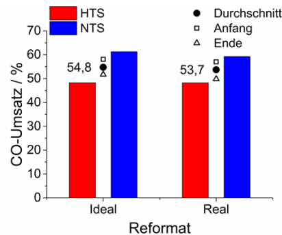
Abbildung 6.8: Einfluss der Reformatqualität auf die Katalysatoraktivität. Messwerte nach „Prima 600 S“ und „Multigas™ 2030D“ und „Cirrus™ 2“.
