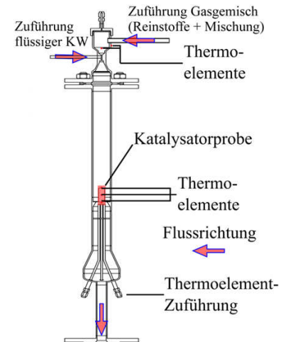
Abbildung 4.2: Schnittzeichnung des Katalysator-Testreaktors.
