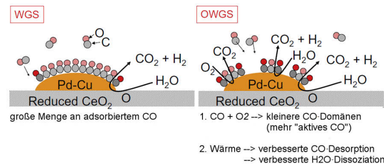
Abbildung 3.5: Mechanismus für die Verbesserung der WGS-Reaktion durch zusätzliche Zugabe von Sauerstoff. Nachgebildet aus [128] mit Genehmigung von Elsevier.
