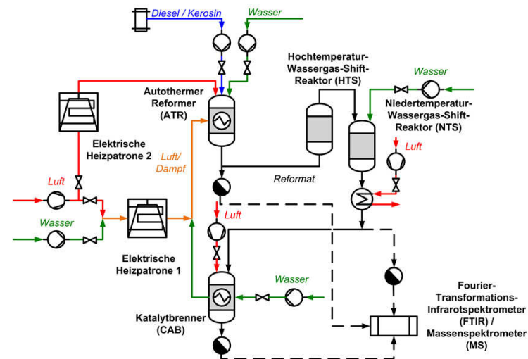
Abbildung 4.5: Fließbild des Systemteststands für Package 4.
