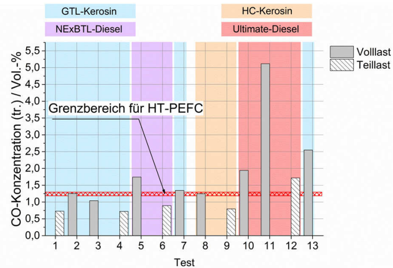
Abbildung 5.1: Kohlenmonoxidkonzentration (trocken) am Austritt des Wassergas-Shift-Reaktors über Versuchsreihe Package 2, Teil 1. Messwerte nach „Prima 600 S“. Nachgebildet aus [160] mit Genehmigung von ECS – The Electrochemical Society.
