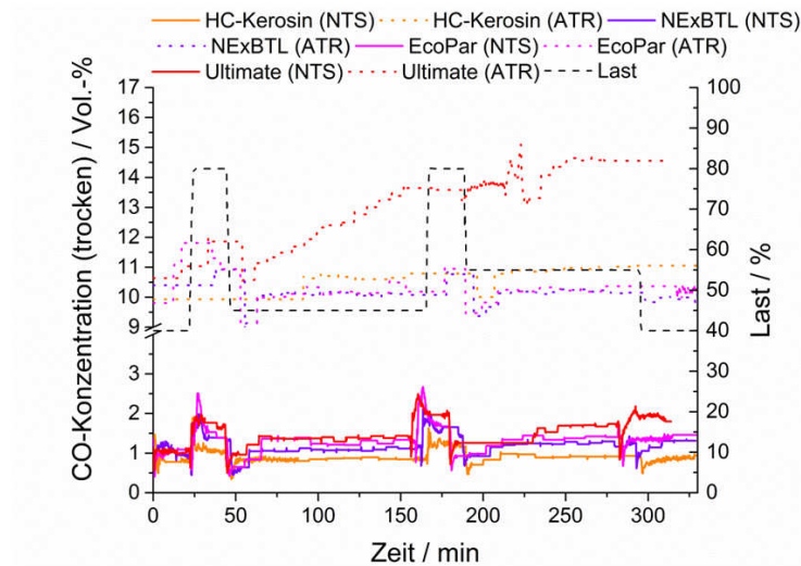
Abbildung 8.10: CO-Konzentrationen hinter dem NTS-Reaktor und dem ATR für alle vier Kraftstoffe bei dem Profil „Lutsey Modi Mittel“. Messwerte nach „Multigas™ 2030D“ und „Cirrus™ 2“.
