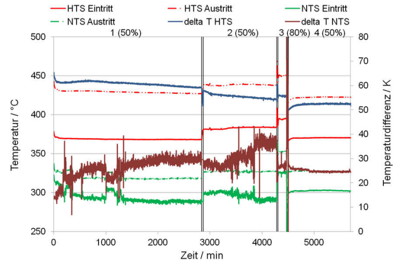
Abbildung 8.4: WGS-Temperaturen während des ersten 100 h-Versuchs mit Katalysator B und HC-Kerosin.
