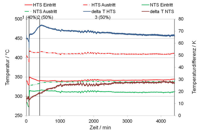
Abbildung 8.8: WGS-Temperaturen während des dritten Langzeitversuchs mit Katalysator B und HC-Kerosin. Es wurden Teillastbetrieb und ein niedriges HTS-Temperaturniveau gewählt.
