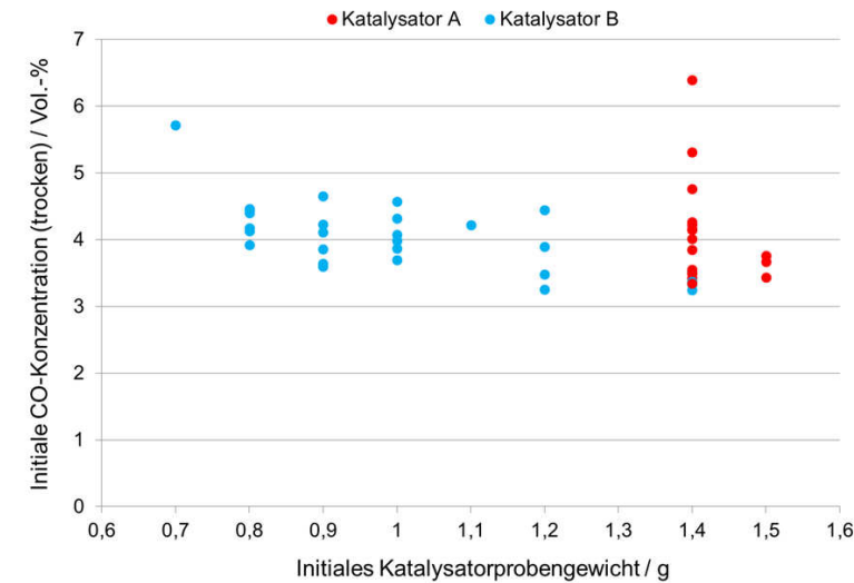
Abbildung 15.9: Probenvariabilität der Katalysatoren A und B. Aufgetragen ist die initial gemessene CO-Konzentration in Abhängigkeit des gemessenen Probengewichts.
