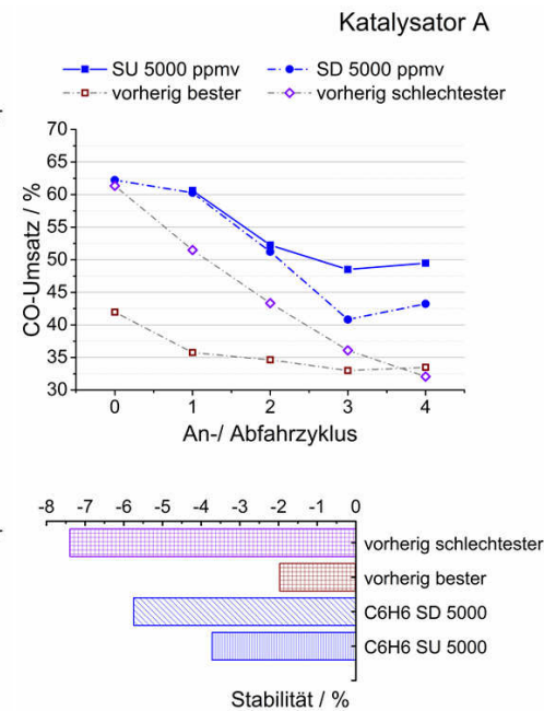
Abbildung 6.15: Einfluss von C_6H_6 auf die Stabilität von Katalysator A während des An- und Abfahrens (SU=startup, SD=shutdown). Messwerte nach „Multigas™ 2030D“ und „Cirrus™ 2“.
