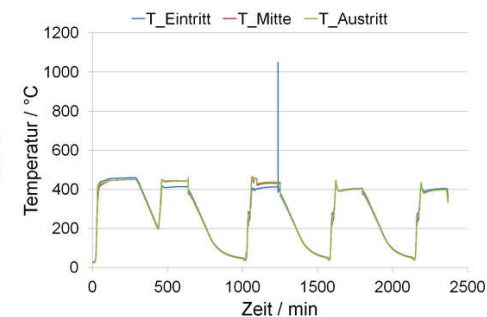
Abbildung 6.20: Vollständige Deaktivierung von Katalysator A durch eine kurzzeitige Temperaturspitze bis 1048 °C.
