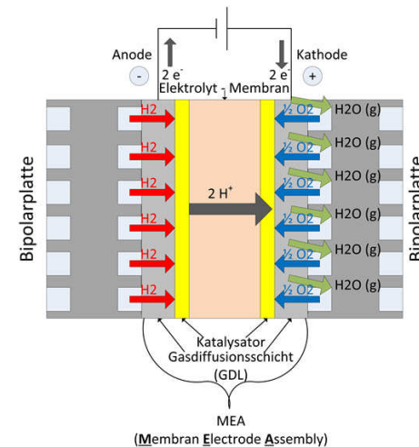
Abbildung 2.2: Funktionsweise einer Brennstoffzelle am Beispiel einer HT-PEFC, nach [50].
