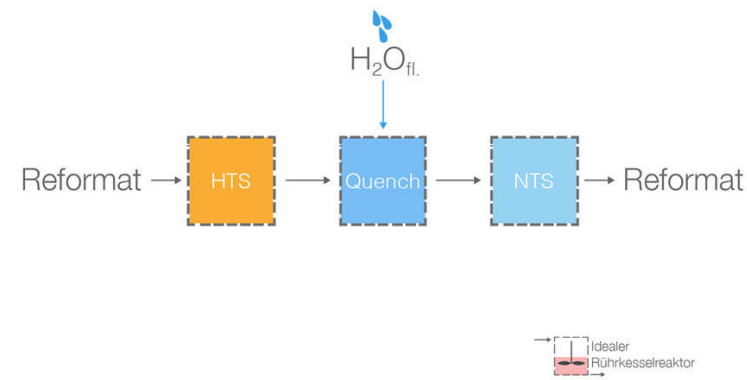
Abbildung 4.12: Gesamtmodell des Wassergas-Shift-Reaktors WGS 4.
