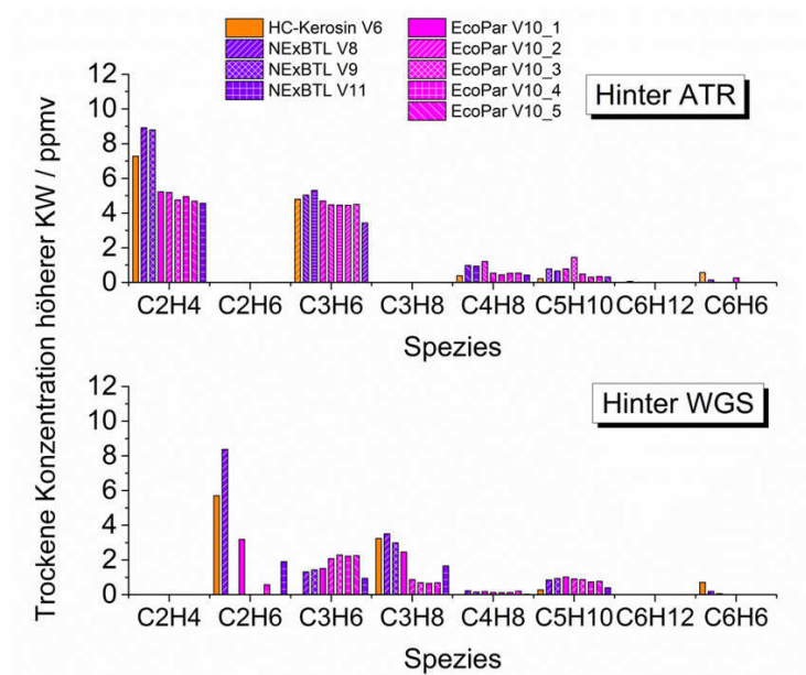
Abbildung 5.5: Unterschiedliche Konzentrationen höherer Kohlenwasserstoffe hinter dem Reformer und dem Wassergas-Shift-Reaktor bei stationärem Betrieb. Messwerte nach „HP 6890 Series“ und „HP G1099A“. Nachgebildet aus [160] mit Genehmigung von ECS – The Electrochemical Society.
