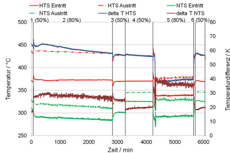
Abbildung 8.6: WGS-Temperaturen während des zweiten 100 h-Versuchs mit Katalysator B und HC-Kerosin.
