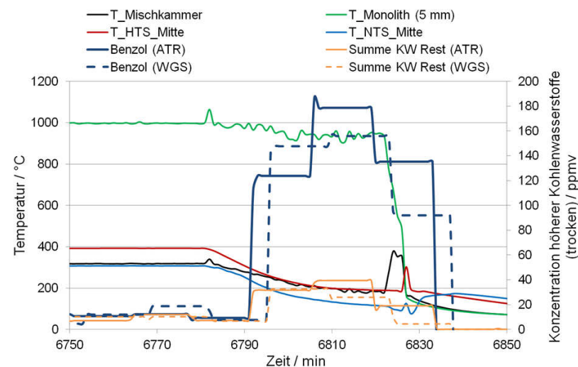
Abbildung 5.7: Konzentrationsverlauf höherer Kohlenwasserstoffe hinter dem ATR und dem WGS während des unplanmäßigen Abschaltens von Package 1. Messwerte nach „Multigas™ 2030D“ und „Cirrus™ 2“.
