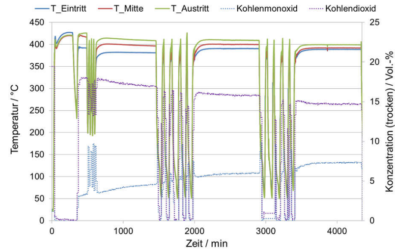
Abbildung 15.10: Stabilität von Katalysator A bei drei unterschiedlichen Temperaturzyklusintervallen. Betrieb unter HTS-Bedingungen und idealem Reformat. Messwerte nach „Multigas™ 2030D“ und „Cirrus™ 2“.
