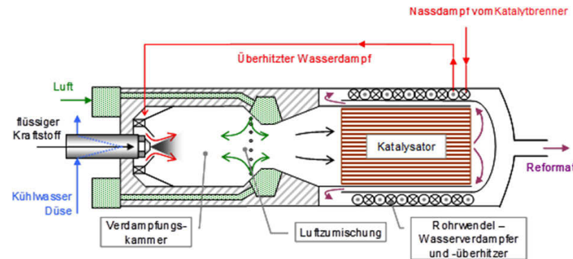
Abbildung 2.5: Schematische Zeichnung des ATR 9.2 des IEK-3 in der 10 kW el -Leistungsklasse.
