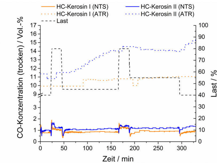
Abbildung 8.13: CO-Konzentrationen hinter dem NTS-Reaktor und dem ATR für die Versuche „HC-Kerosin I“ und „HC-Kerosin II“ bei dem Profil „Lutsey Modi Mittel“. Messwerte nach „Multigas™ 2030D“ und „Cirrus™ 2“.
