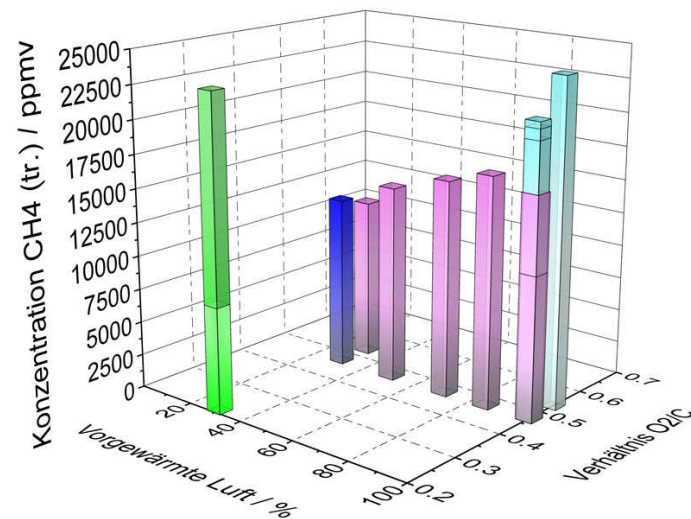
Abbildung 15.13: Maximalkonzentrationen von CH 4 während des Systemstarts mit NExBTL. Farben: grün: klassische Strategie; blau: neue Strategie 1, magenta: neue Strategie 2; cyan: neue Strategie 3.
