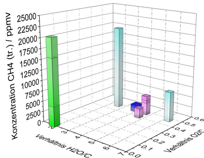
Abbildung 15.14: Maximalkonzentrationen von CH 4 während des Abfahrens des Systems mit NExBTL. Farben: grün: klassische Strategie; blau: neue Strategie 1, magenta: neue Strategie 2; cyan: neue Strategie 3.
