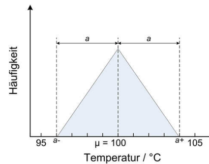
Abbildung 4.6: Beispiel für eine Dreiecksverteilung, nach [141].
