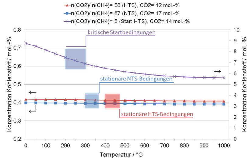
Abbildung 5.10: Potential der Kohlenstoffbildung durch Methan für stationäre HTS- und NTS-Bedingungen sowie Systemstartbedingungen.
