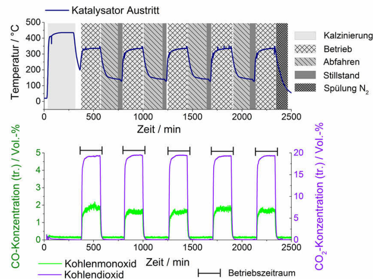
Abbildung 6.5: Testprozedur und Beispieltest der Abfahrvorgänge am Katalysator-Testreaktor. Nachgebildet aus [160] mit Genehmigung von ECS – The Electrochemical Society.
