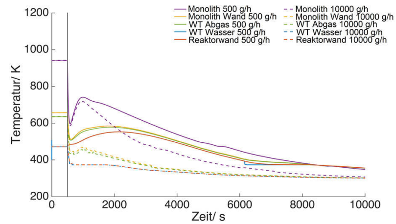
Abbildung 15.24: Temperaturverläufe im Katalytbrenner während der Warmwasserproduktion mit 500 g/h oder 10000 g/h Wasser. Als Spülmedium wurden 10000 l/h Luft gewählt.
