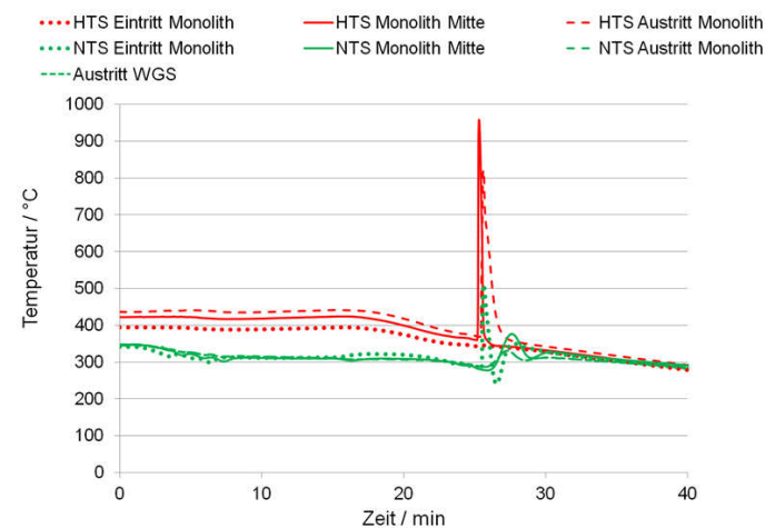
Abbildung 5.8: Kritische Temperaturpeaks durch Oxidationsreaktionen auf dem Wassergas-Shift-Katalysator.
