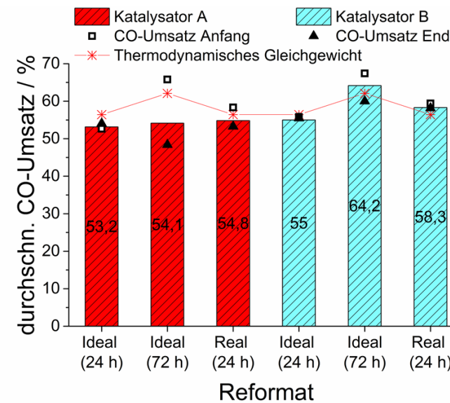
Abbildung 6.3: CO-Umsatz bei stationärem Betrieb unter HTS-Bedingungen mit idealem und realem Reformat. Vergleich zwischen Katalysator A und B. Messwerte nach „Multigas™ 2030D“ und „Cirrus™ 2“.
