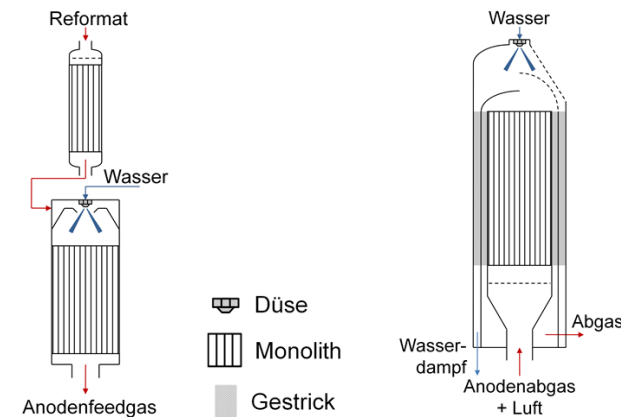
Abbildung 2.6: Schematische Darstellung des Wassergas-Shift-Reaktors (links) und des Katalytbrenners mit internem Wärmetauscher (rechts), nach [11].
