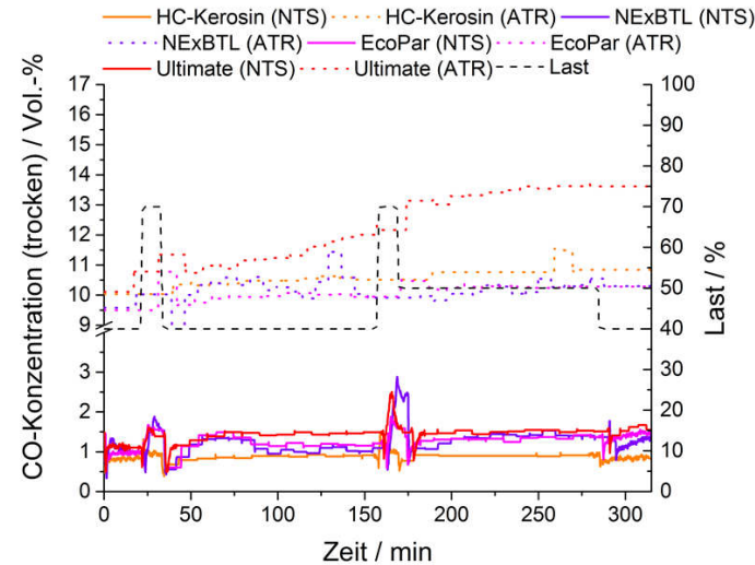
Abbildung 8.11: CO-Konzentrationen hinter dem NTS-Reaktor und dem ATR für alle vier Kraftstoffe bei dem Profil „Lutsey Modi Einfach“. Messwerte nach „Multigas™ 2030D“ und „Cirrus™ 2“.
