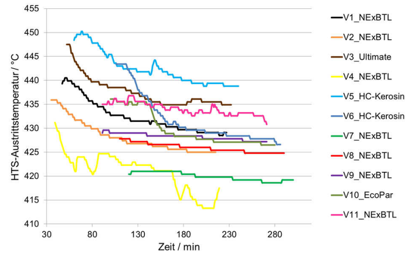
Abbildung 5.6: Profil der HTS-Austrittstemperatur innerhalb der ersten drei Betriebsstunden.
