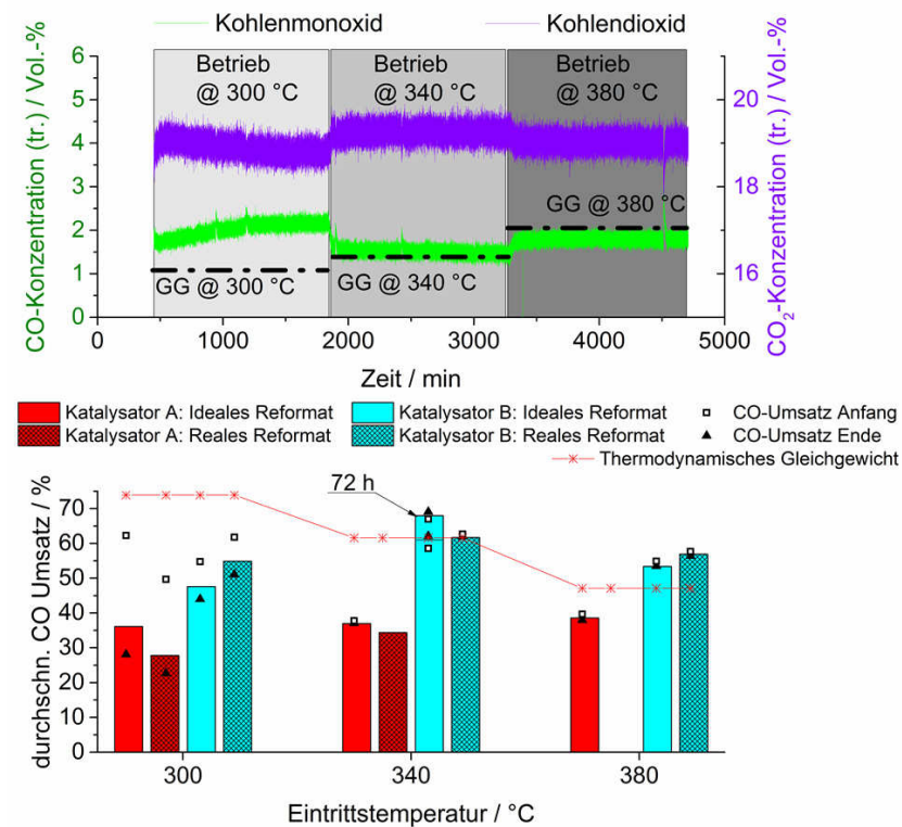
Abbildung 6.4: CO- und CO 2 -Konzentrationen in Abhängigkeit des Betriebstemperaturniveaus bei idealem Reformat und Katalysator B (oben, GG= Thermodynamisches Gleichgewicht). CO-Umsatz bei stationärem Betrieb unter NTS-Bedingungen mit idealem und realem Reformat. Vergleich zwischen Katalysator A und B (unten). Messwerte nach „Multigas™ 2030D“ und „Cirrus™ 2“. Nachgebildet aus [160] mit Genehmigung von ECS – The Electrochemical Society.
