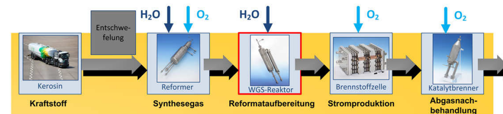
Abbildung 1.1: Beispiel eines Brennstoffzellensystems als APU.
