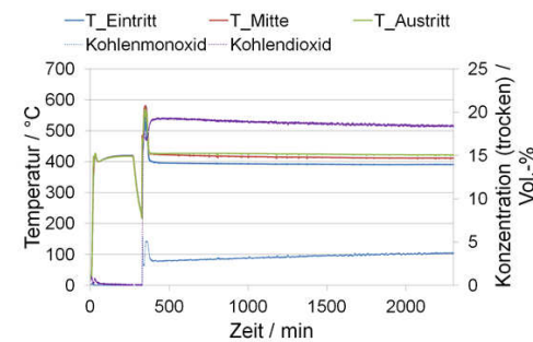
Abbildung 6.19: Kein Einfluss eines langen Temperaturpeaks bis 580 °C auf die Aktivität von Katalysator A. Messwerte nach „Multigas™ 2030D“ und „Cirrus™ 2“.
