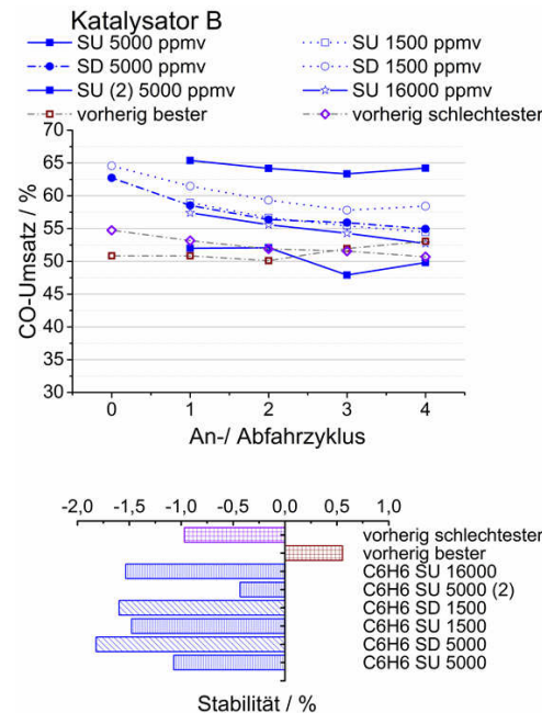
Abbildung 6.14: Einfluss von C_6H_6 auf die Stabilität von Katalysator B während des An- und Abfahrens (SU=startup, SD=shutdown). Messwerte nach „Multigas™ 2030D“ und „Cirrus™ 2“.
