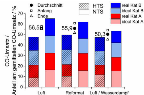
Abbildung 6.9: Einfluss des Spülmediums auf die Katalysatoraktivität. Messwerte nach „Prima 600 S“ und „Multigas™ 2030D“ und „Cirrus™ 2“.
