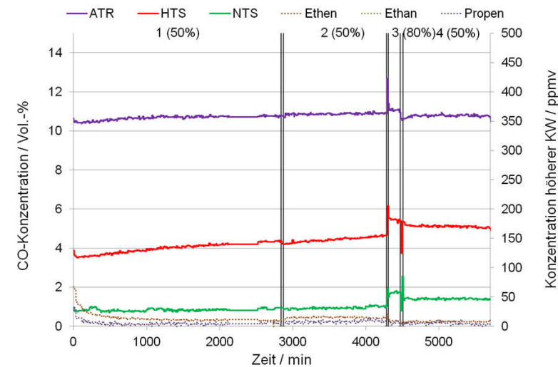
Abbildung 8.5: Konzentrationen von CO und höherer Kohlenwasserstoffe (ATR) während des ersten 100 h-Versuchs mit Katalysator B und HC-Kerosin. Messwerte nach „Multigas™ 2030D“ und „Cirrus™ 2“.
