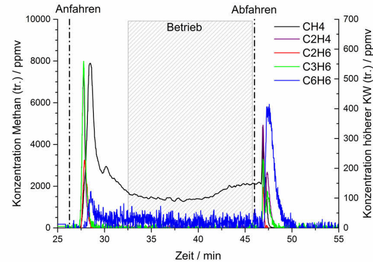
Abbildung 5.9: Beispiel für die unterschiedlichen Konzentrationen an Methan und höheren Kohlenwasserstoffen während des Anfahrens, des stationären Betriebs und des Abfahrens. Messwerte nach „Mültigas™ 2030D“ und „Cirrus™ 2“. Nachgebildet aus [162] mit Genehmigung von Elsevier.
