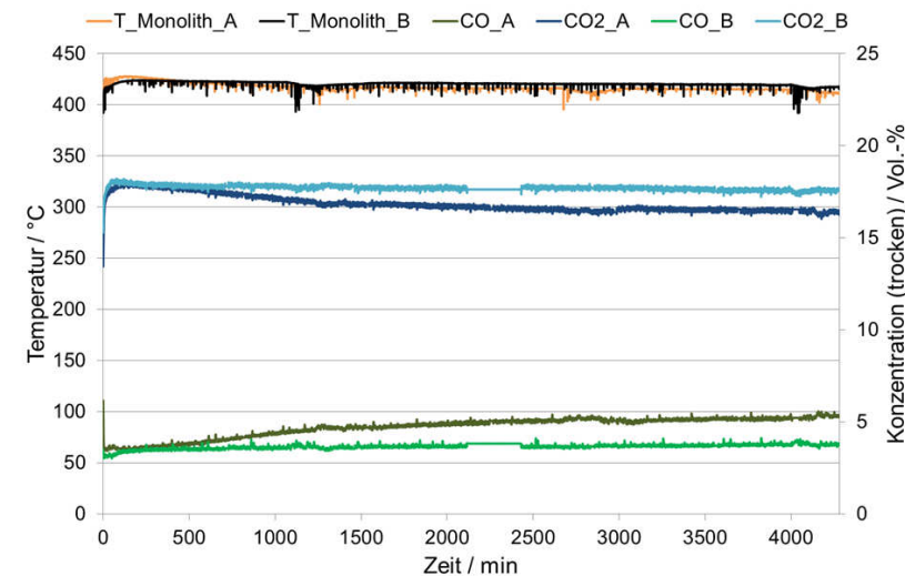
Abbildung 6.2: Verlauf der CO- und \text{CO}_2 -Konzentrationen bei 72 h stationärem Betrieb unter HTS-Bedingungen mit idealem Reformat. Vergleich zwischen Katalysator A und B. Messwerte nach „Multigas TM 2030D“ und „Cirrus TM 2“.
