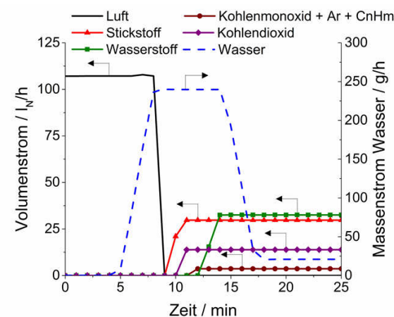
Abbildung 6.1: Sequentielle Zugabe der Reformatkomponenten zur Vermeidung von Temperaturpeaks zu Beginn jedes Versuchs. Nachgebildet aus [160] mit Genehmigung von ECS – The Electrochemical Society.
