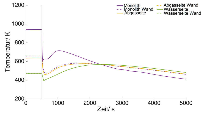
Abbildung 15.21: Fluid- und Wandtemperaturen im Katalytbrenner während des Abfahrvorgangs. Als Spülmedium wurde Luft/ Wasserdampf mit 10000 l N /h Luft und 10000 g/h Wasserdampf gewählt. Nach T_{krit} wurde die Wasserdampfzufuhr unterbunden.
