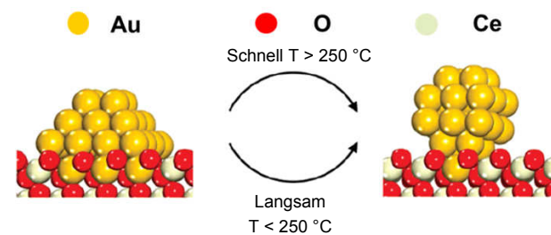
Abbildung 3.4: Änderung der Struktur eines Au/ CeZrO 4 -Katalysators während der WGS-Reaktion. Nachgebildet mit Genehmigung von [98]. Copyright (2007) American Chemical Society.
