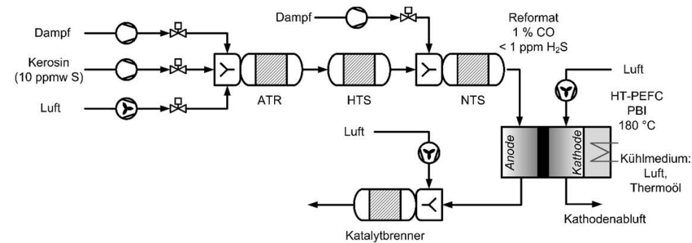
Abbildung 2.4: Basisfließschema eines integrierten Brennstoffzellensystems mit Kerosinreformierung und HT-PEFC, nach [31].
