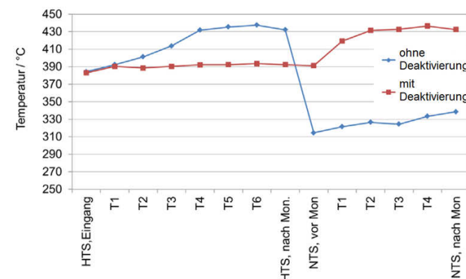
Abbildung 1.2: Temperaturverlauf im Wassergas-Shift-Reaktor mit und ohne Deaktivierung des Katalysators in der HTS-Stufe [13].
