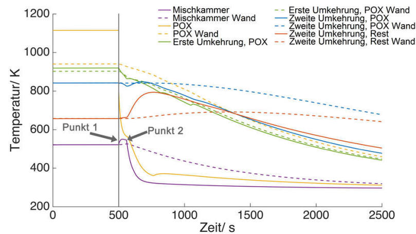
Abbildung 15.19: Fluid- und Wandtemperaturen im autothermen Reformer während des Abfahrvorgangs. Als Spülmedium wurde Luft/ Wasserdampf mit 10000 l/h Luft und 10000 g/h Wasserdampf gewählt. Nach T_{krit} wurde die Wasserdampfzufuhr unterbunden.
