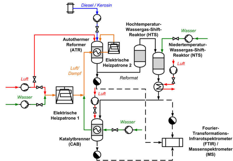
Abbildung 4.4: Fließbild des Systemteststands für Package 1 und 2.
