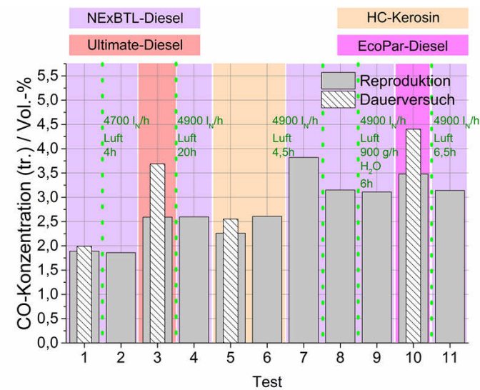
Abbildung 5.3: Kohlenmonoxidkonzentration (trocken) am Austritt des Wassergas-Shift-Reaktors über Versuchsreihe Package 2, Teil 2. Messwerte nach „Prima 600 S“.
