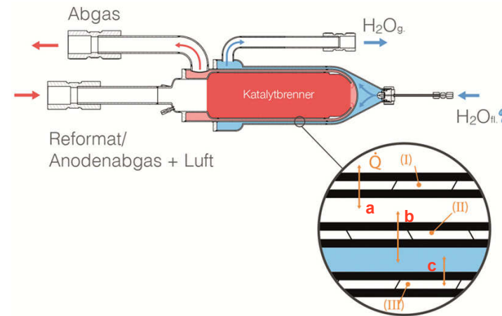
Abbildung 4.13: Abstraktion der Geometrie des Katalytbrenners CAB 3 und berechnete Wärmeübergänge im Modell.
