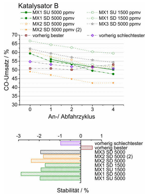
Abbildung 6.16: Einfluss von C n H m -Mischungen auf die Stabilität von Katalysator B während des An- und Abfahrens (MX=mixture, SU=startup, SD=shutdown). Messwerte nach „Multigas™ 2030D“ und „Cirrus™ 2“.
