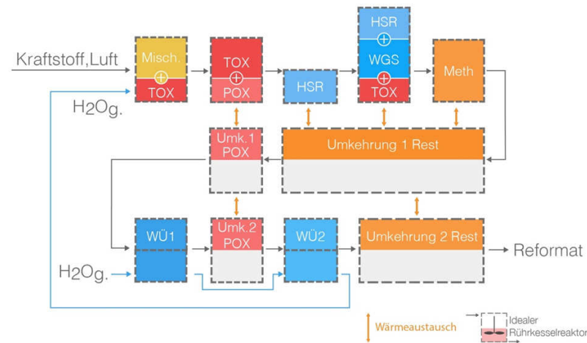
Abbildung 4.10: Gesamtmodell des autothermen Reformers ATR 9.2.
