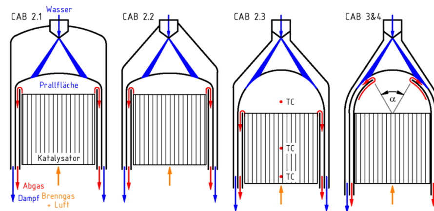
Abbildung 15.3: Geometrien der Katalytbrenner-Generationen 2 bis 4 (TC=thermocouple). Nachgebildet aus [68] mit Genehmigung von Elsevier.
