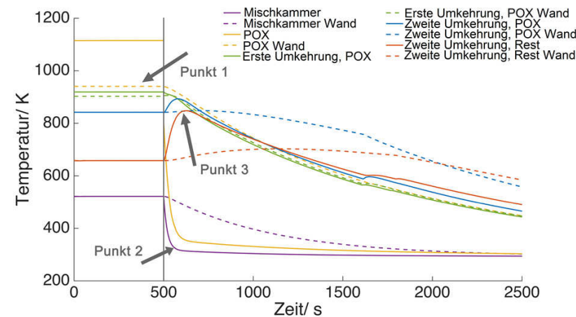
Abbildung 9.2: Fluid- und Wandtemperaturen im autothermen Reformer während des Abfahrvorgangs. Als Spülmedium wurde Luft mit 20000 l N /h gewählt.
