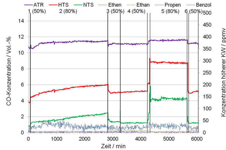
Abbildung 8.7: Konzentrationen von CO und höherer Kohlenwasserstoffe (ATR) während des zweiten 100 h-Versuchs mit Katalysator B und HC-Kerosin. Messwerte nach „Multigas™ 2030D“ und „Cirrus™ 2“.
