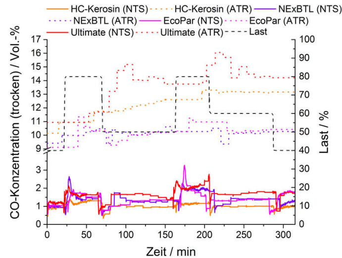
Abbildung 8.12: CO-Konzentrationen hinter dem NTS-Reaktor und dem ATR für alle vier Kraftstoffe bei dem Profil „Lutsey Modi Schwer“. Messwerte nach „Multigas™ 2030D“ und „Cirrus™ 2“.
