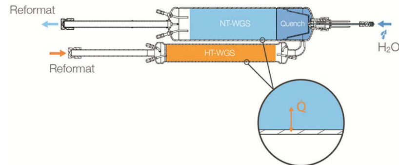
Abbildung 4.11: Abstraktion der Geometrie des Wassergas-Shift-Reaktors WGS 4 und berechnete Wärmeübergänge im Modell.
