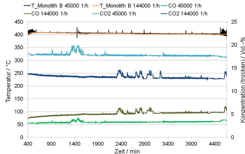
Abbildung 6.18: Stabilität von Katalysator B bei Raumgeschwindigkeiten von 45000 1/h und 144000 1/h. Betrieb unter HTS-Bedingungen und idealem Reformat. Messwerte nach „Multigas™ 2030D“ und „Circus™ 2“.
