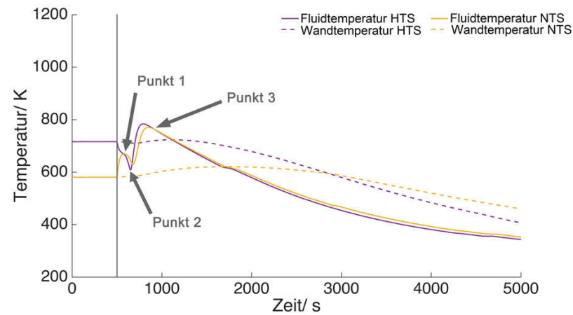
Abbildung 15.17: Fluid- und Wandtemperaturen im Wassergas-Shift-Reaktor während des Abfahrvorgangs. Als Spülmedium wurde Wasserdampf mit 10000 g/h gewählt. Nach T_{krit} wurden 20000 l N /h Luft dem Reformer zugegeben.
