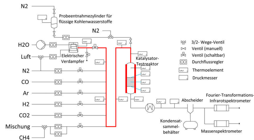
Abbildung 4.1: Fließbild des Katalysator-Testreaktor-Teststands.
