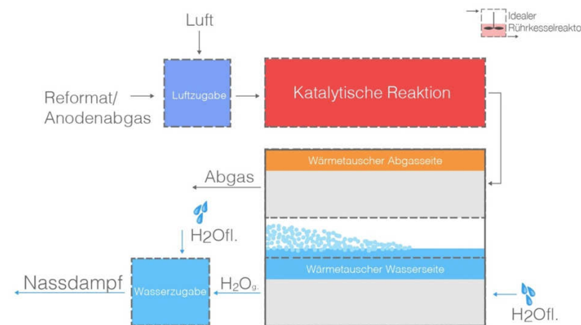
Abbildung 4.14: Gesamtmodell des Katalytbrenners CAB 3.
