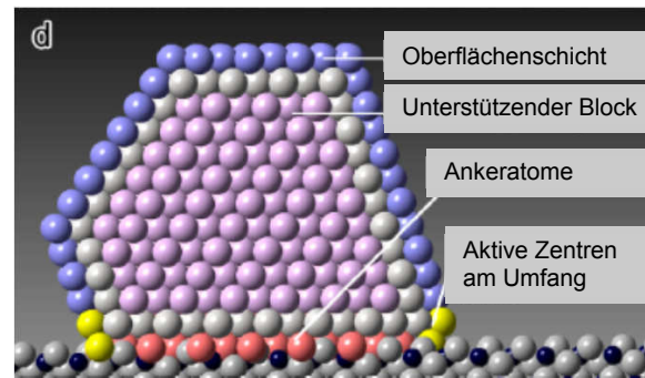
Abbildung 3.3: Schema eines Gold-Nanopartikels, welches auf dem Washcoat \text{CeO}_2 verankert ist. Nachgebildet mit Genehmigung von [93]. Copyright (2012) American Chemical Society.
