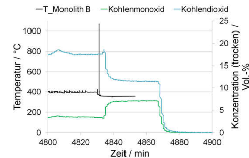
Abbildung 6.22: Starke Deaktivierung von Katalysator B durch einen kurzzeitigen Temperaturpeak von 1070 °C. Messwerte nach „Multigas™ 2030D“ und „Cirrus™ 2“.
