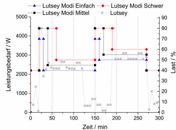
Abbildung 8.9: Charakteristisches Tageslastprofil eines Lkw, nach Lutsey [165] und abgeleitete Profile für diese Arbeit.
