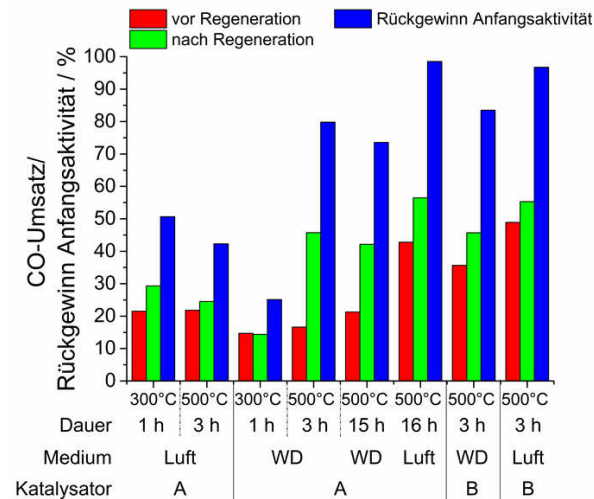
Abbildung 7.4: Regeneration deaktivierter Proben von Katalysator A und B in Luft oder Wasserdampf unter verschiedenen Temperaturniveaus und Regenerationszeiträumen. Messwerte nach „Multigas™ 2030D“ und „Cirrus™ 2“.
