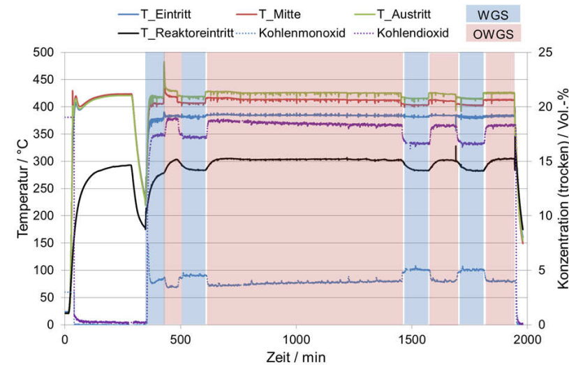
Abbildung 7.5: Temperaturen und Konzentrationen während der Untersuchung von wechselndem WGS und OWGS-Betrieb bei Katalysator B. Es wurden HTS-Bedingungen und ein molares O_2/CO -Verhältnis von 0,25 gewählt. Messwerte nach „Multigas™ 2030D“ und „Cirrus™ 2“.
