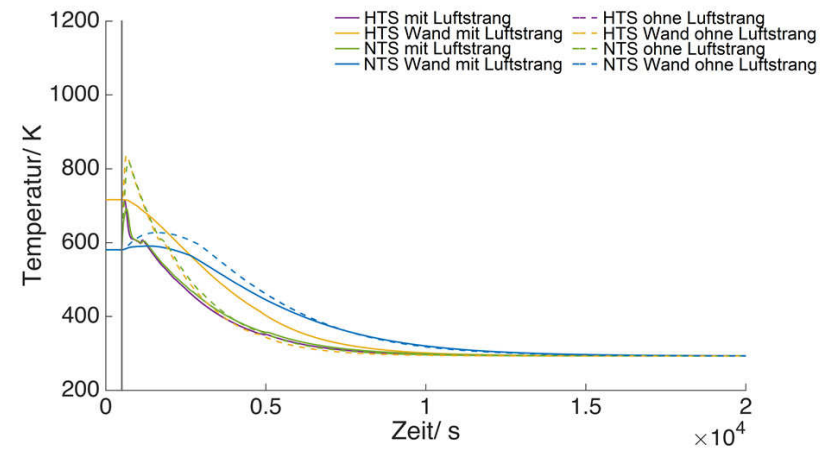
Abbildung 15.22: Verbesserung (a): kurze Abfahrdauer. Temperaturverläufe im Wassergas-Shift-Reaktor. Im Fall mit zusätzlichem Luftstrang wurde zunächst mit 10000 l N /h Luft und 500 g/h Wasserdampf gespült. Nach T_{krit} wurden zusätzlich 10000 l N /h Luft hinzugegeben. Im Fall ohne zusätzlichen Luftstrang wurde von Anfang an mit 20000 l N /h Luft und 500 g/h Wasserdampf gespült. Nach T_{krit} wurde die Wasserzufuhr gestoppt.
