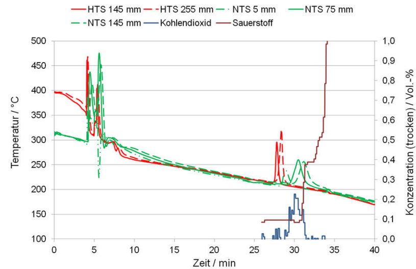
Abbildung 8.3: Temperaturspitzen im Wassergas-Shift-Reaktor während des Abfahrens des Systems und der anschließenden Regeneration mit 80 l N /h Luft. Messwerte nach „Multigas™ 2030D“ und „Cirrus™ 2“.
