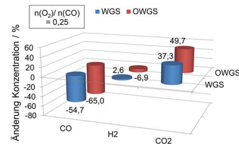
Abbildung 7.6: Durchschnittliche Änderung der Konzentrationen an CO, H 2 und CO 2 während des WGS- und OWGS-Betriebs mit Katalysator B. Es wurden HTS-Bedingungen und ein molares O 2 /CO-Verhältnis von 0,25 gewählt. Messwerte nach „Multigas™ 2030D“ und „Cirrus™ 2“.
