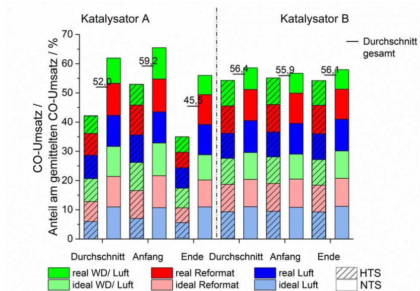
Abbildung 6.10: Unterschiedliche Aktivität/ Stabilität der Katalysatoren A und B. Messwerte nach „Prima 600 S“ und „Multigas™ 2030D“ und „Cirrus™ 2“.
