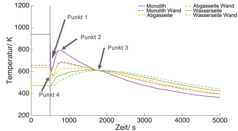
Abbildung 9.4: Fluid- und Wandtemperaturen im Katalytbrenner während des Abfahrvorgangs. Als Spülmedium wurde Luft mit 20000 l N /h gewählt.
