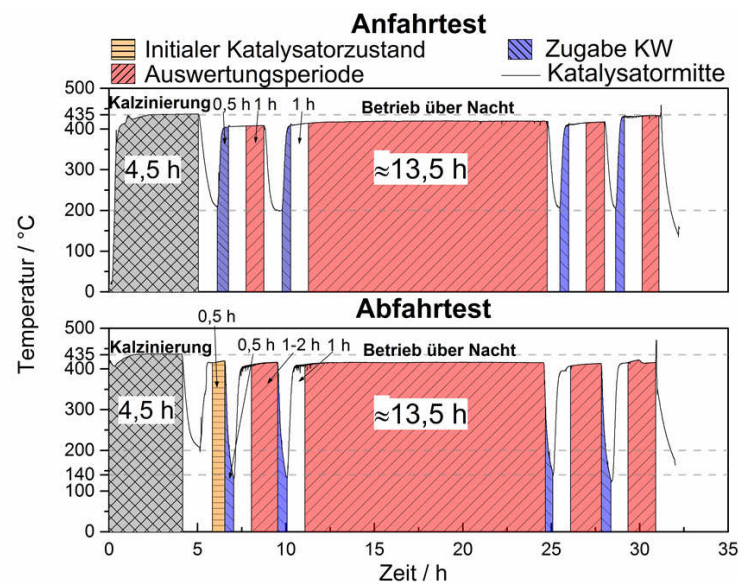
Abbildung 6.11: Testprozedur zur Identifikation kritischer Reformatkomponenten am Katalysator-Testreaktor.
