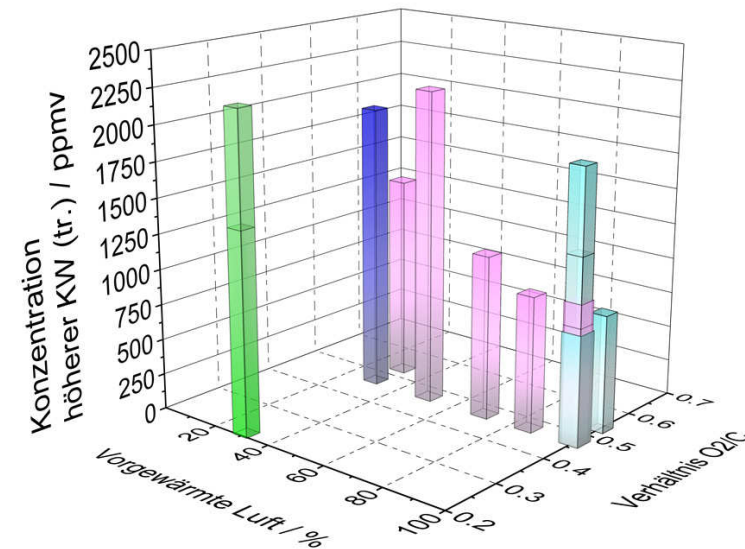
Abbildung 7.1: Maximalkonzentrationen höherer Kohlenwasserstoffe hinter dem ATR während des Systemstarts mit NExBTL. Farben: grün: klassische Strategie; blau: neue Strategie 1, magenta: neue Strategie 2; cyan: neue Strategie 3. Messwerte nach „Multigas™ 2030D“ und „Cirrus™ 2“. Nachgebildet aus [162] mit Genehmigung von Elsevier.
