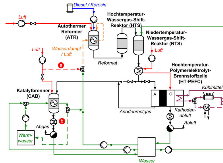
Abbildung 9.5: Fließbild des Brennstoffzellensystems des IEK-3 mit den Verbesserungen (a) kurze Abfahrdauer und (b) Energierückgewinnung.
