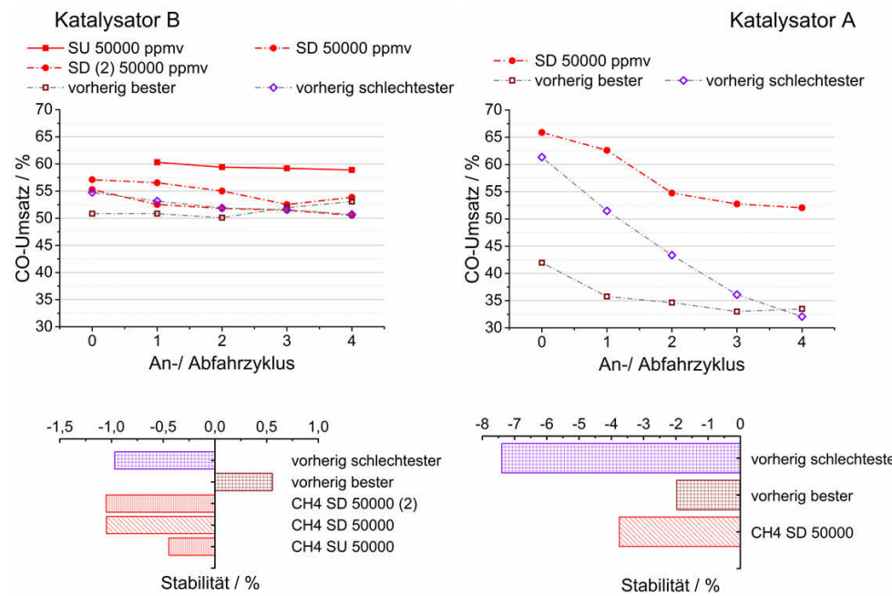
Abbildung 6.12: Einfluss von CH 4 auf die Stabilität von Katalysator B während des An- und Abfahrens (SU=startup, SD=shutdown). Messwerte nach „Multigas™ 2030D“ und „Cirrus™ 2“.
