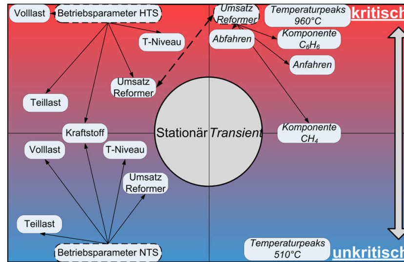
Abbildung 5.11: Übersicht der identifizierten, potentiell kritischen Parameter für den Betrieb des WGS-Reaktors unter stationären und transienten Bedingungen.
