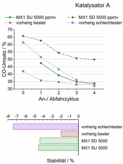
Abbildung 6.17: Einfluss von C n H m -Mischungen auf die Stabilität von Katalysator A während des An- und Abfahrens (MX=mixture, SU=startup, SD=shutdown). Messwerte nach „Multigas™ 2030D“ und „Cirrus™ 2“.
