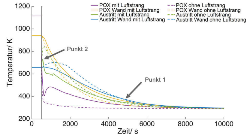
Abbildung 9.6: Verbesserung (a): kurze Abfahrdauer. Temperaturverläufe im autothermen Reformer. Im Fall mit zusätzlichem Luftstrang wurde zunächst mit 10000 l N /h Luft und 500 g/h Wasserdampf gespült. Nach T_{krit} wurden zusätzlich 10000 l N /h Luft hinzugegeben. Im Fall ohne zusätzlichen Luftstrang wurde von Anfang an mit 20000 l N /h Luft und 500 g/h Wasserdampf gespült. Nach T_{krit} wurde die Wasserzufuhr gestoppt.
