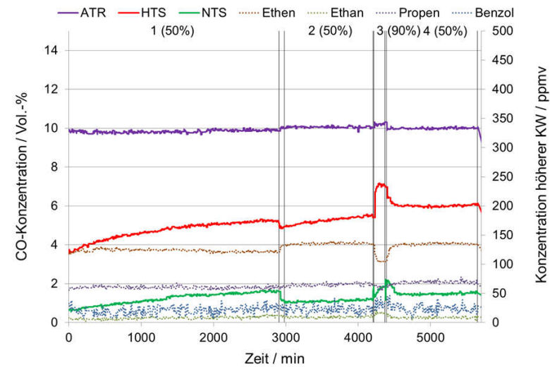
Abbildung 8.2: Konzentrationen von CO und höherer Kohlenwasserstoffe (ATR) während des 100 h-Versuchs mit Katalysator B und NExBTL-Diesel. Messwerte nach „Multigas™ 2030D“ und „Cirrus™ 2“. In den ersten 15 h des Versuchs nahm die CO-Konzentration hinter der HTS-Stufe um ungefähr einen Prozentpunkt zu. Die Versuche auf Katalysatorebene zeigten innerhalb des gleichen Zeit-
