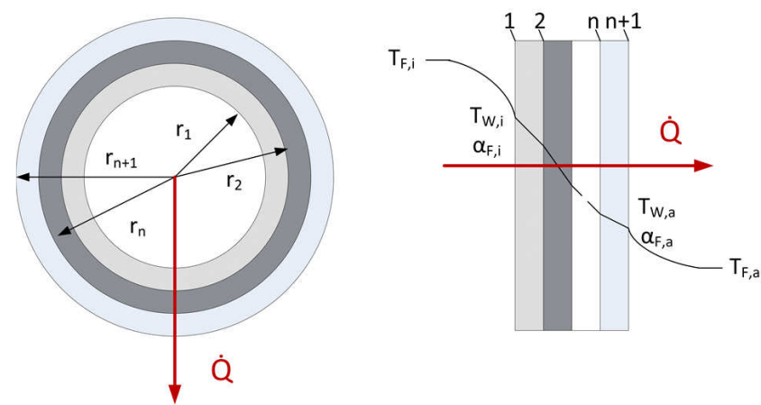
Abbildung 15.6: Wärmeübertragung in einem Hohlzylinder, bestehend aus mehreren unterschiedlichen Materialschichten, nach [153].
