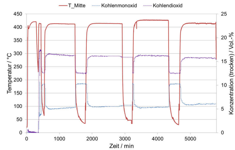
Abbildung 15.12: Einfluss der Wasserkondensation auf die Stabilität von Katalysator B. Betrieb unter HTS-Bedingungen und idealem Reformat. Messwerte nach „Multigas™ 2030D“ und „Cirrus™ 2“.
