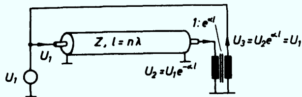
Abb. 1 Rückgespeicher Kettenleiter.
