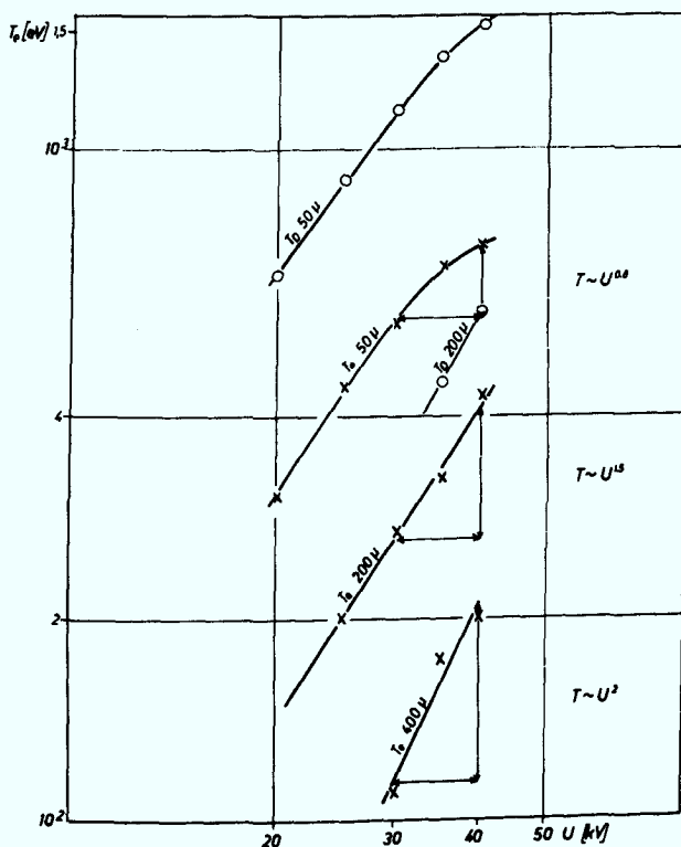
Elektronentemperatur T_e und Deuterontemperatur T_D als Funktion der Ladespannung bei verschiedenen Anfangsdrücken.
