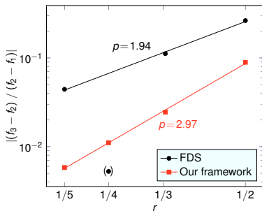
Abbildung: Ortskonvergenz.
