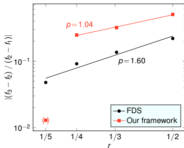
Abbildung: Zeitkonvergenz.
