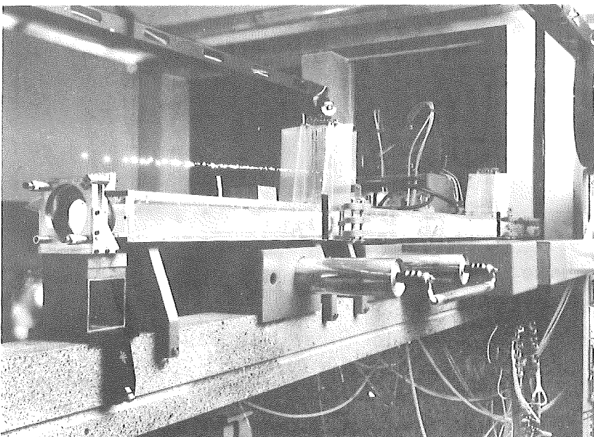
Abb. 16: 300 MW TEA- \text{CO}_2 -Laser im Betrieb.
