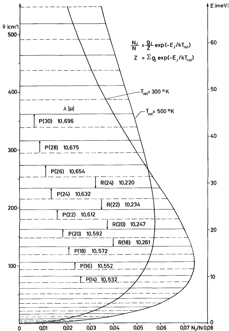
Abb. 5: Rotationsniveaus von \text{CO}_2 , deren Besetzungsdichte N_J für zwei verschiedene Verteilungstemperaturen T_{\text{rot}} sowie die Wellenlängen der stärksten Laserübergänge.
