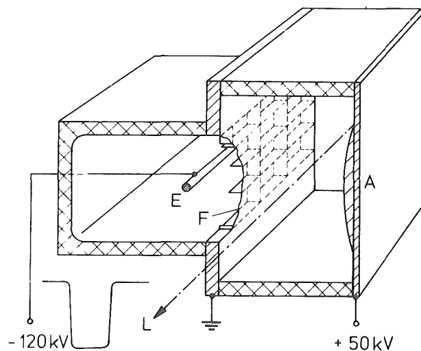
Abb. 19: Prinzipskizze eines \text{CO}_2 -Lasers mit Elektronenstrahlionisierung. E: Elektronenemitter, F: Abgestützte Folie, dient als Anode für den Elektronenstrahlerzeuger und als Kathode für die Gasentladung, A: Anode für Entladung, L: Resonatorachse.
