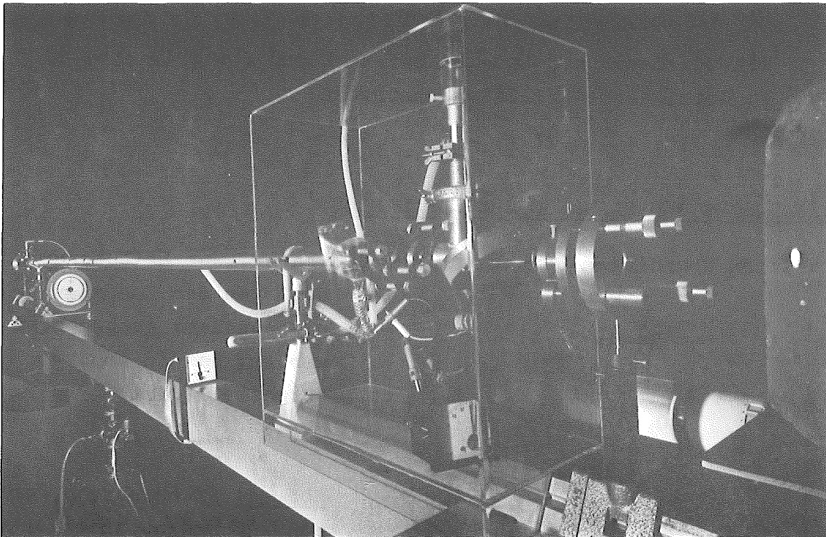
Abb. 2: CO 2 -Dauerstrichlaser im Betrieb. Daten wie in Abb. 1.
