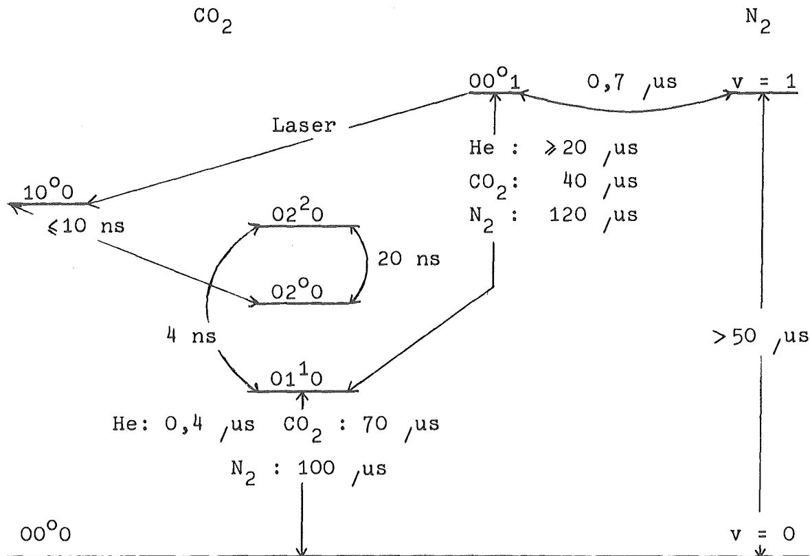
Abb. 8: Stoßprozesse und deren Zeitkonstanten in einem Gemisch aus 0,8 bar He, 0,1 bar CO 2 und 0,1 bar N 2 . Bei zwei Prozessen ist der Beitrag der einzelnen Gase angegeben.
