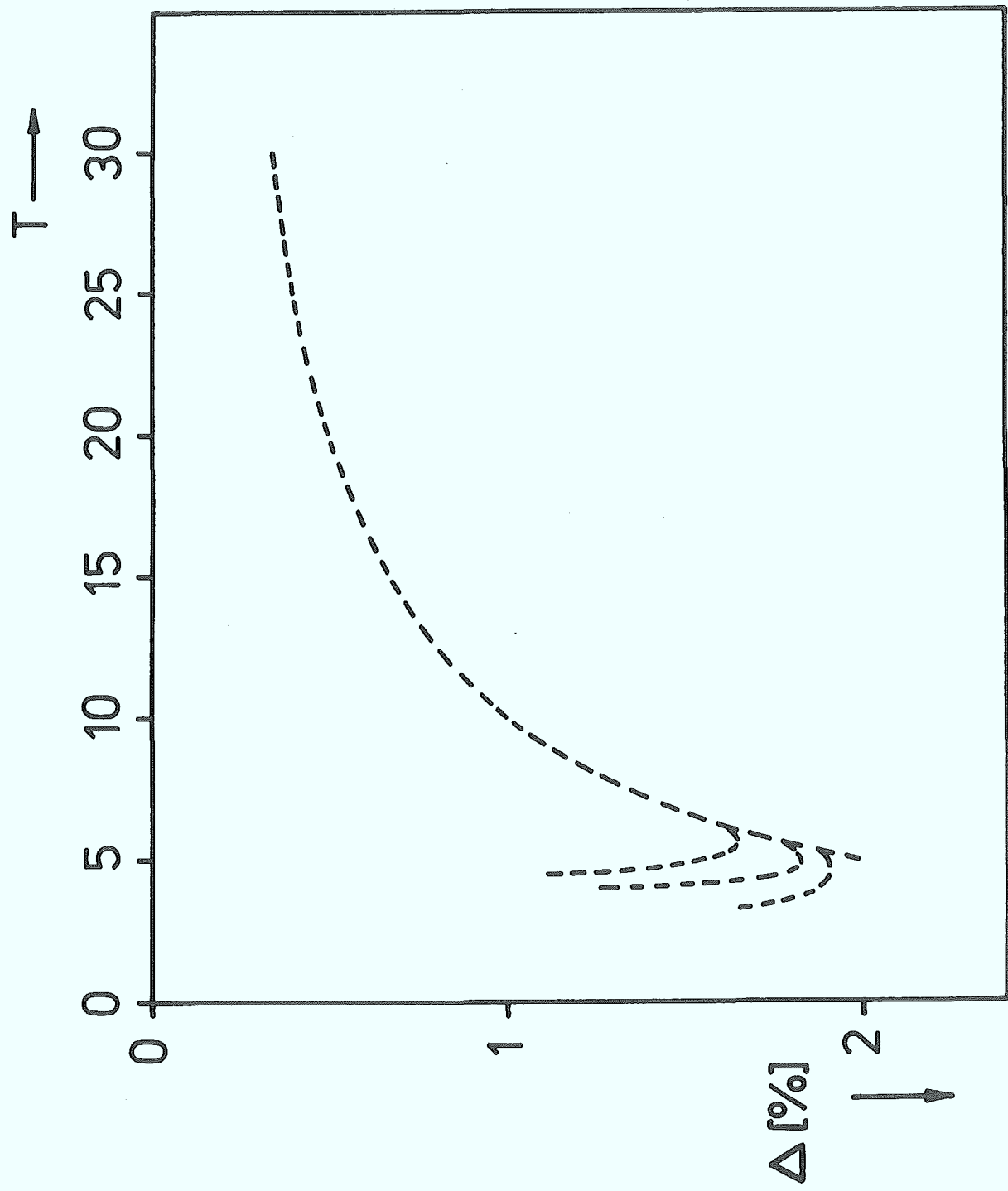
Abb.19: Temperaturabhängigkeit der Relaxationsstärke bei Orientierungsrelaxation nach Gl. 4.3. (19)
