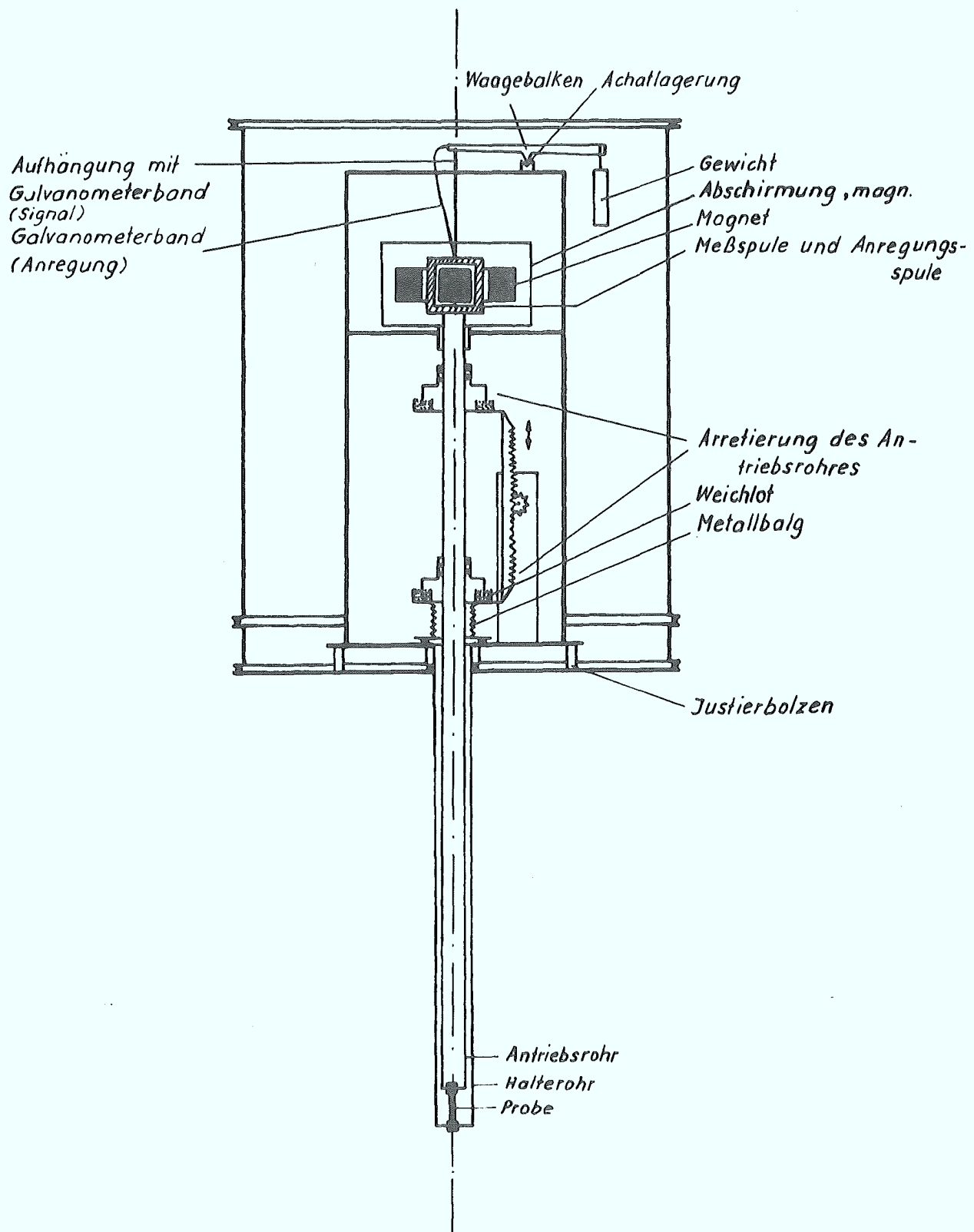
Abb.4: Aufbau des Torsionspendels
