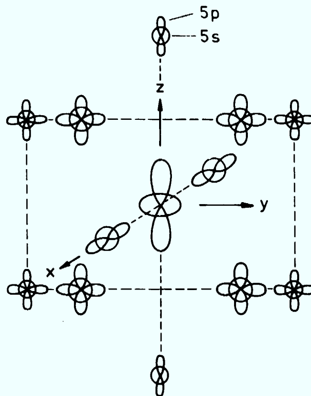
Abb. 39 Ausdehnung des d_{z^2} -Orbitals des \text{Re(IV)} bzw. \text{Tc(IV)} und der benachbarten Sauerstoff- und Zinnorbitale
