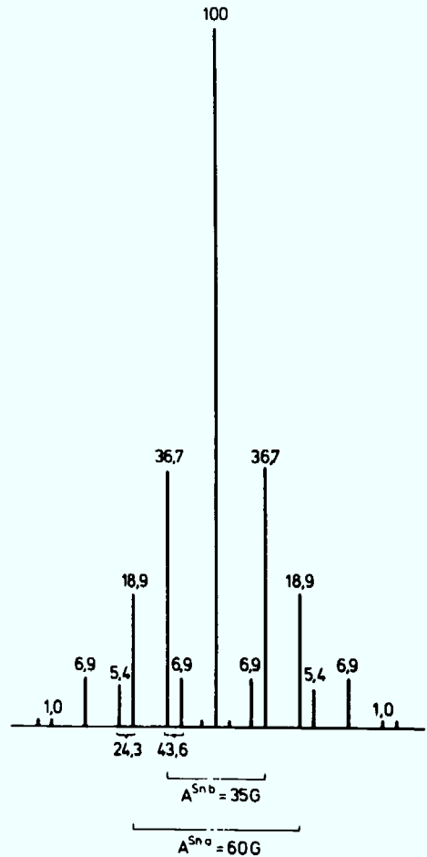
Abb. 37 Aufspaltungsmodell der SHFS in \text{SnO}_2:\text{Re(IV)} für \text{H [001]}_2 bei Annahme gemeinsamer Überlagerung durch zwei und vier Sn-Kerne
