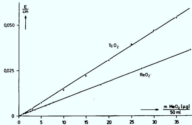
Abb. 5 Eichkurven zur spektralphotometrischen Bestimmung von Re und Tc in \text{SnO}_2
