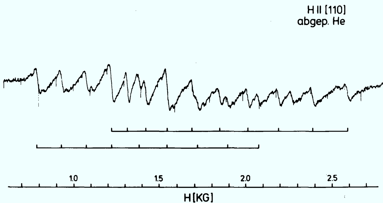
Abb. 22 ESR-Spektren von \text{SnO}_2:\text{Tc(IV)} im X-Band ( \nu = 9,3440 \text{ GHz} )
