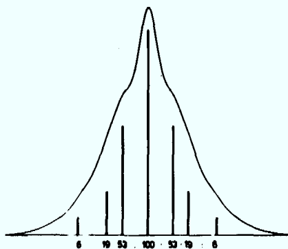
Abb. 36 SnO_2:Re(IV) , integriertes Signal (Übergang m_S = \pm\frac{1}{2} , m_I = -\frac{5}{2} ) mit überlagelter SHFS und Intensitätsverhältnissen der Nebenlinien
