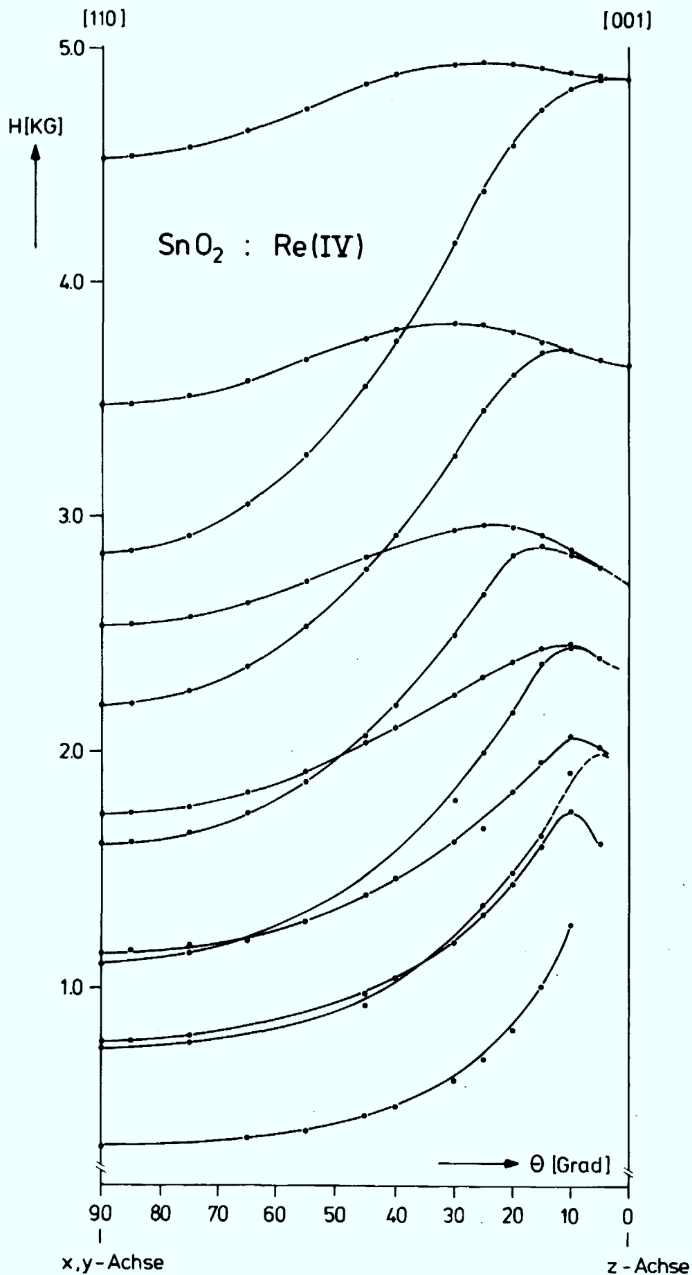
Abb. 11 Winkelabhängigkeit des X-Band-Spektrums von \text{SnO}_2:\text{Re(IV)} in der (110)-Ebene. Aufgetragen sind die Mittelwerte der Feldstärken von ^{185}\text{Re} und ^{187}\text{Re} .
