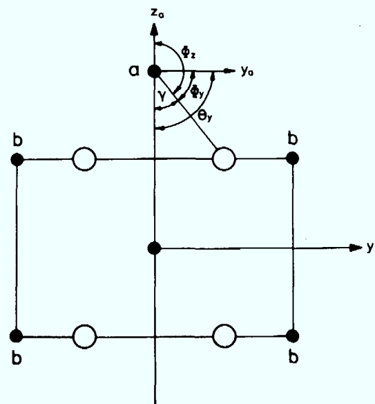
Abb. 41 Zur Kennzeichnung der Winkel \theta und \phi . Schnitt durch die Einheitszelle des \text{SnO}_2 in der (110)-Ebene. ● = Zinn ○ = Sauerstoff
