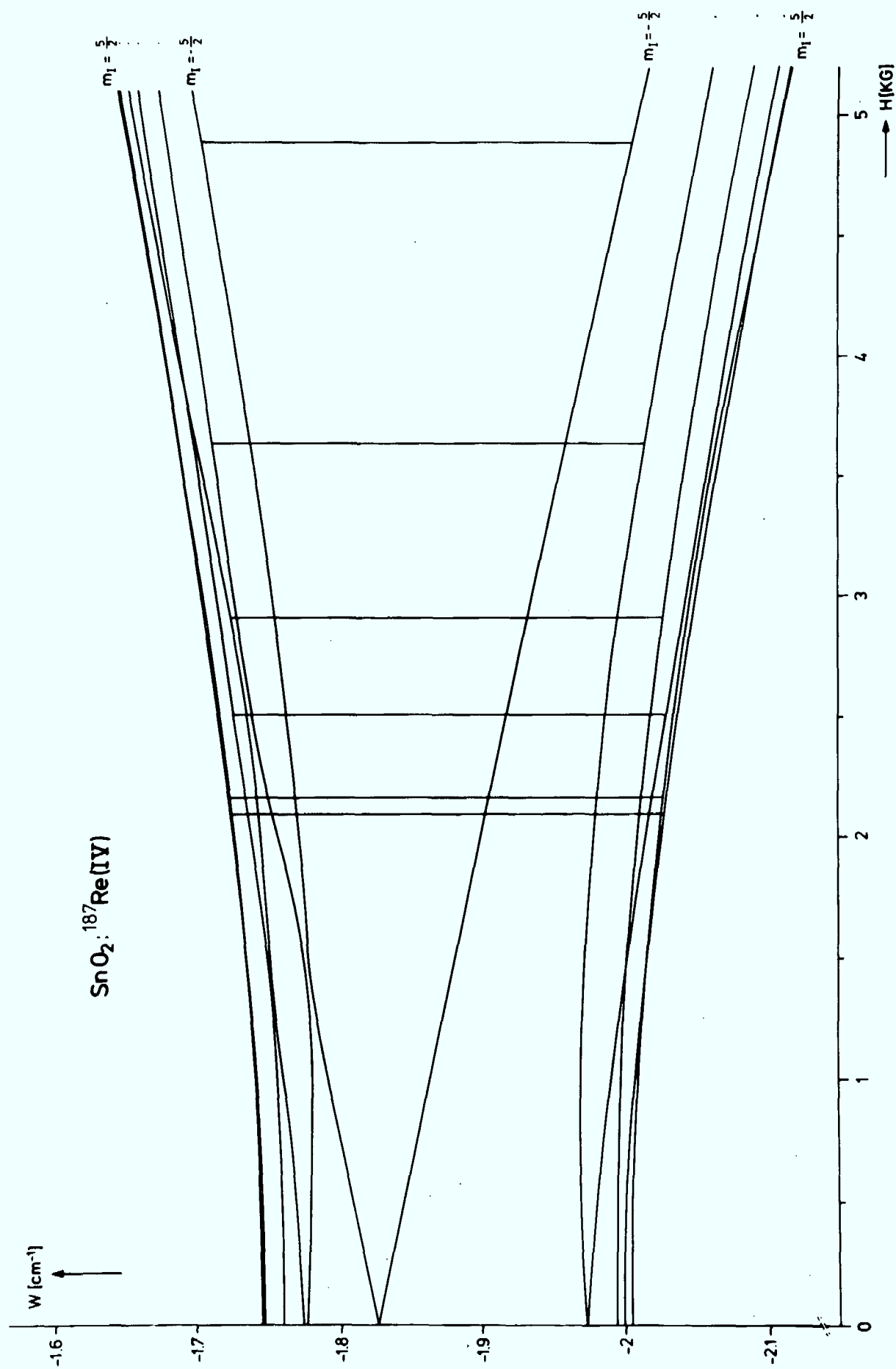
Abb. 20 Verlauf der Hyperfein-Energieniveaus für \text{SnO}_2: {}^{187}\text{Re}(\text{IV}) im Bereich der X-Band-Übergänge. Elektronenübergang \frac{1}{2} \longleftrightarrow -\frac{1}{2}
