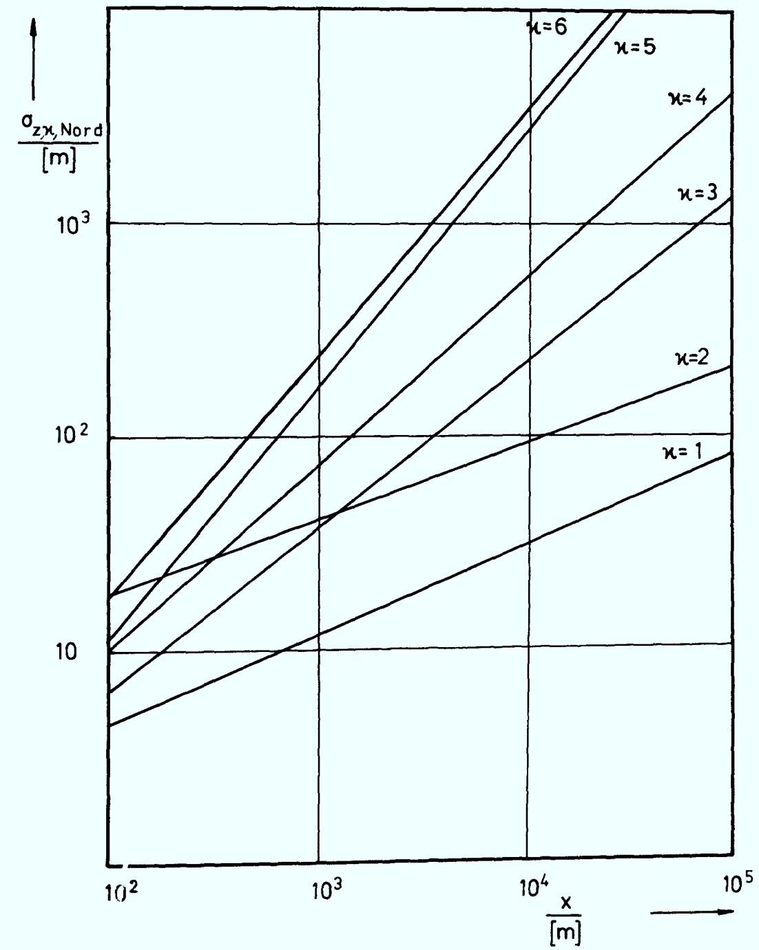
Abb. 3.2.3.1 : Vertikalparameter für die Basisstandort- klasse SÜD.
