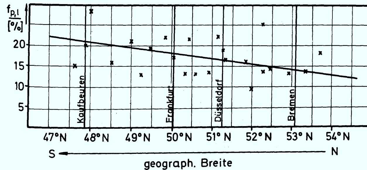
Abb. 3.2.2.k: Fehler der bei der Berechnung der Langzeitausbreitungsfunktion gemacht wird, wenn man annimmt p_{ijk} = p_i \cdot p_{jk} , dargestellt in Abhängigkeit von der geographischen Lage der jeweiligen meteorologischen Stationen. (vergl. Tab. A I im Anhang).
