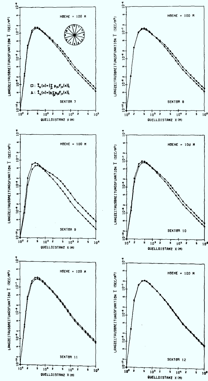
Abb. 3.2.2.f: Darstellung der Langzeitausbreitungsfunktion in Abhängigkeit von der Windrichtung und der Quelldistanz für den Standort Düsseldorf, f_{pl} = 18 \% .
