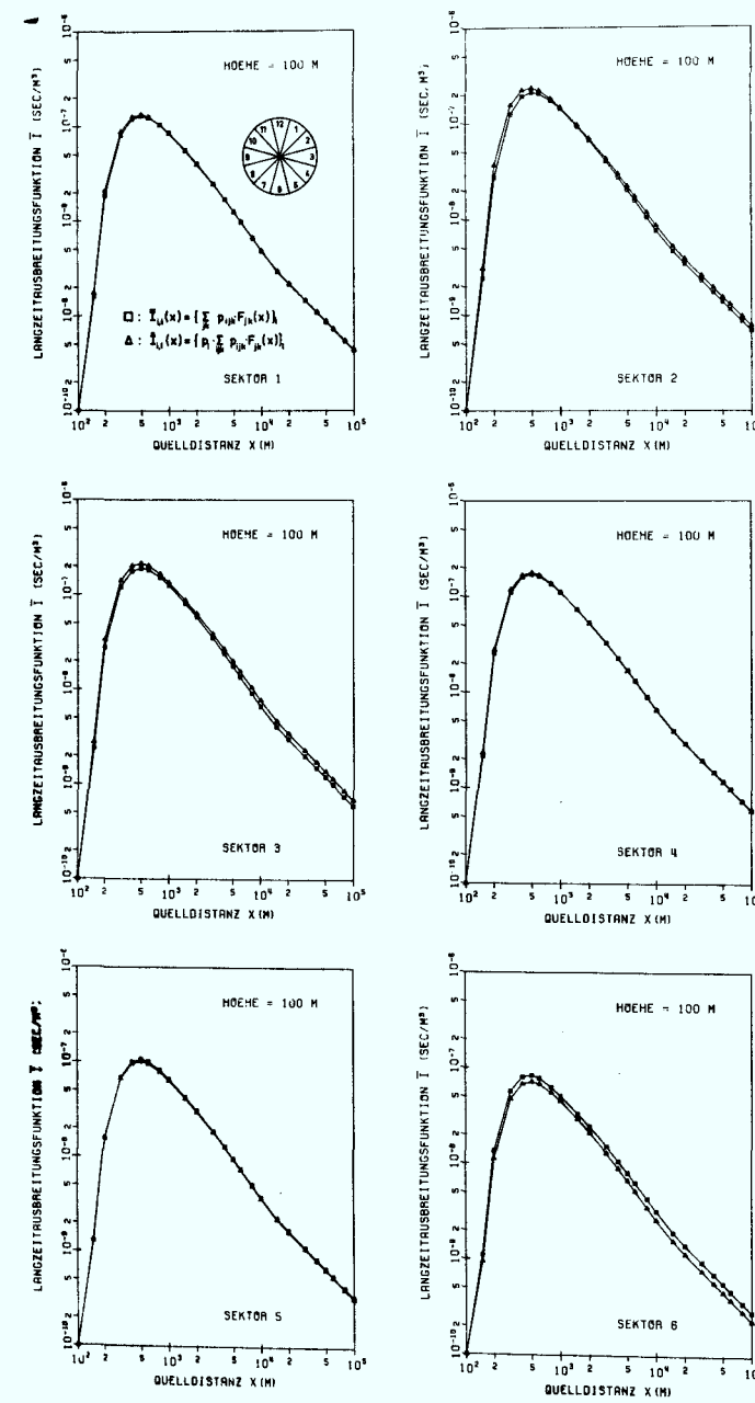
Abb. 3.2.2.d: Darstellung der Langzeitausbreitungsfunktion in Abhängigkeit von der Windrichtung und der Quelledistanz für den Standort Bremen, f_{p1} = 10 \% .
