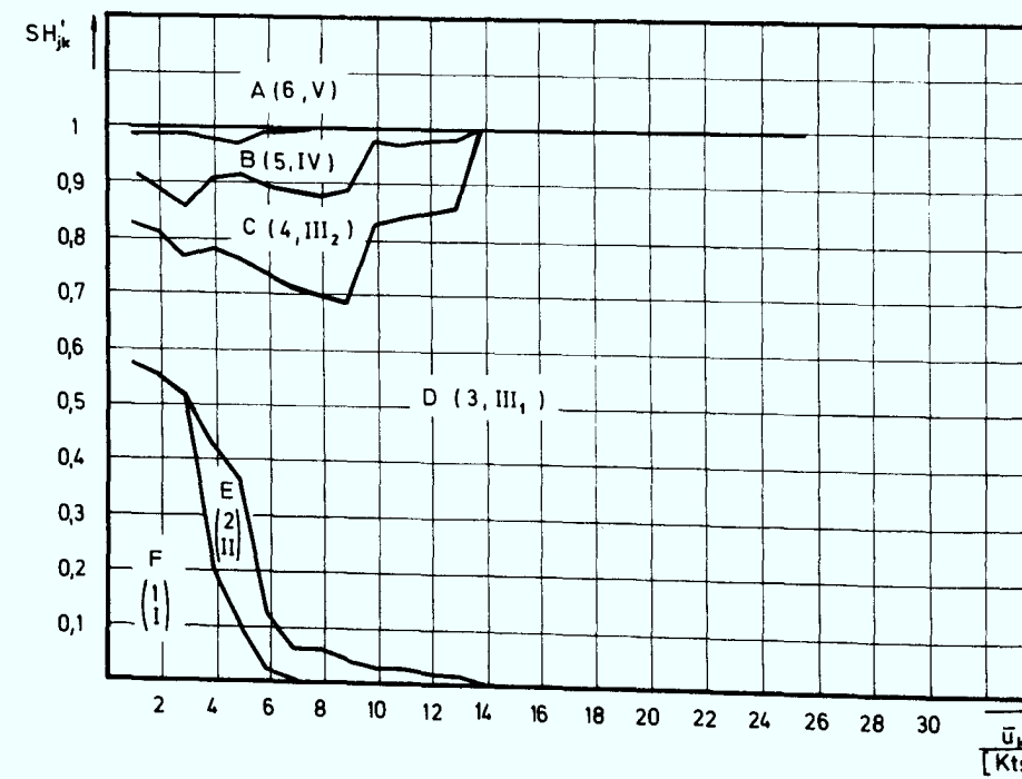
Abb. 2.2.d: Normierte Summenhäufigkeit SH'_{jk} der Diffusionskategorien als Funktion der mittleren Windgeschwindigkeiten in 10 m Höhe über ungestörtem Gelände in Jülich.
