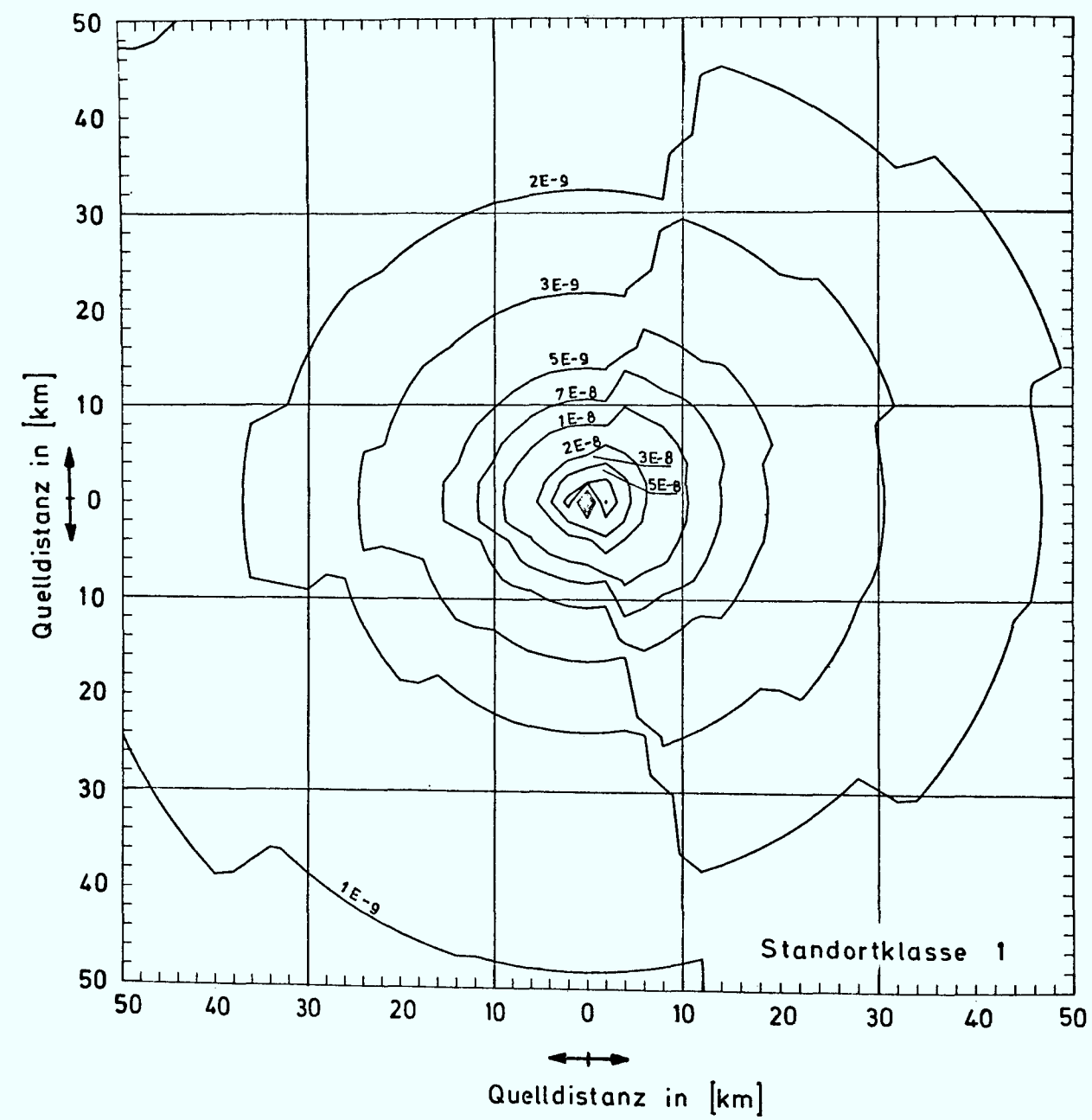
Abb. 3.2.3.a: Darstellung der sektor- und quelldistanz-abhängigen Langzeitausbreitungsfunktionen I_{iv}(x) für die Standortklasse 1
