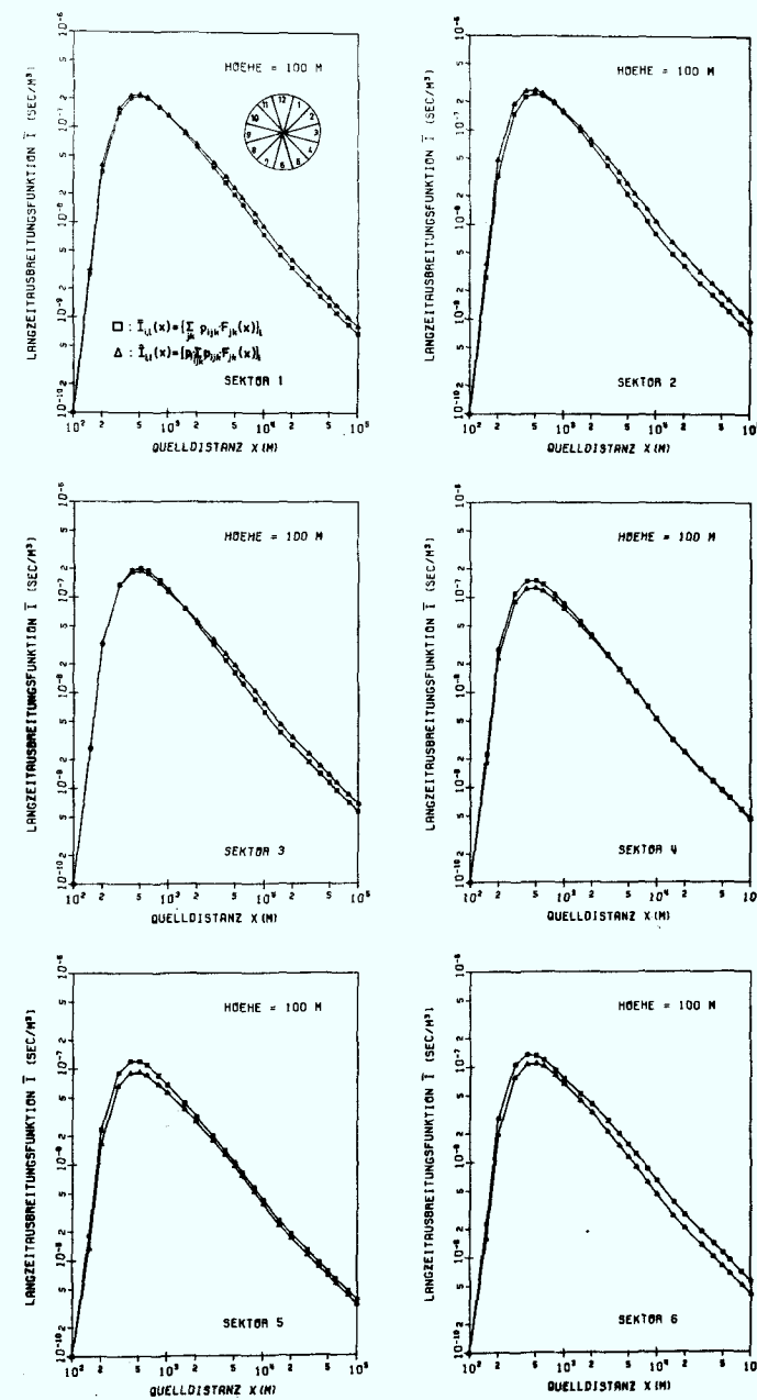
Abb. 3.2.2.e: Darstellung der Langzeitausbreitungsfunktion in Abhängigkeit von der Windrichtung und der Quelledistanz für den Standort Düsseldorf, f_{p1} = 18 \% .
