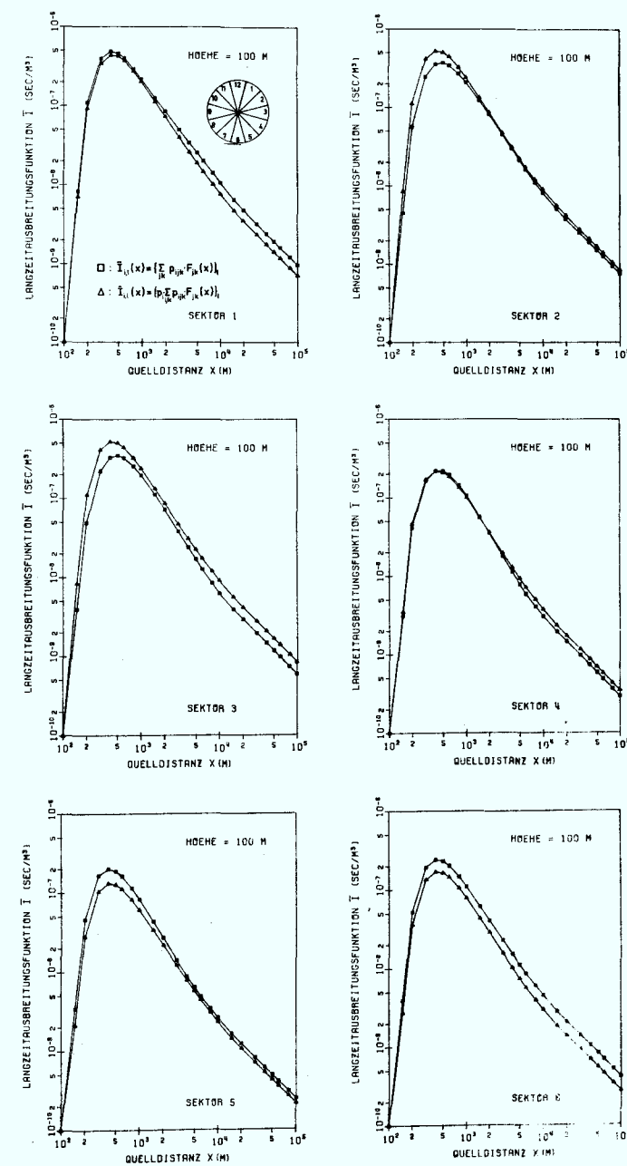
Abb. 3.2.2.i: Darstellung der Langzeitausbreitungsfunktion in Abhängigkeit von der Windrichtung und der Quelldistanz für den Standort Kaufbeuren, f_{p1} = 20,5 \% .
