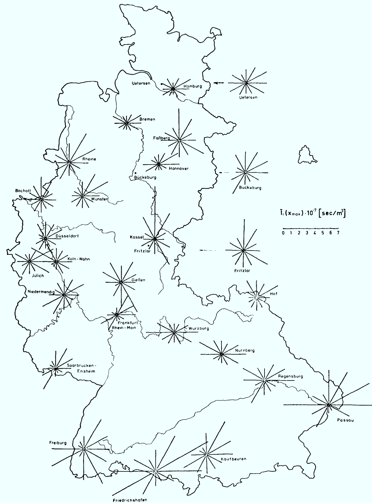
Abb. 3.2.2.a: \bar{I}_i(x_{\text{MAX}}) -Verteilungen für 25 meteorologische Stationen in der Bundesrepublik Deutschland
