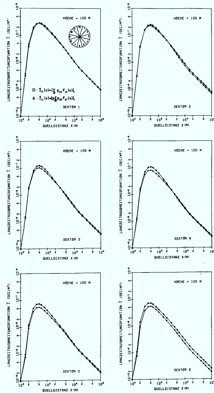
Abb. 3.2.2.g: Darstellung der Langzeitausbreitungsfunktion in Abhängigkeit von der Windrichtung und der Quelldistanz für den Standort Frankfurt, f_{p1} = 15,5 \% .
