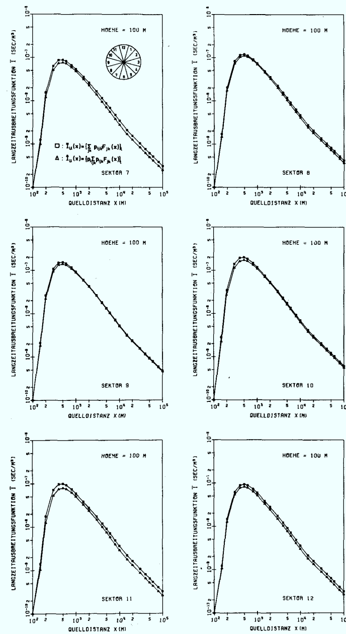
Abb. 3.2.2.c: Darstellung der Langzeitausbreitungsfunktion in Abhängigkeit von der Windrichtung und der Quelledistanz für den Standort Bremen, f_{p1} = 10 \% .
