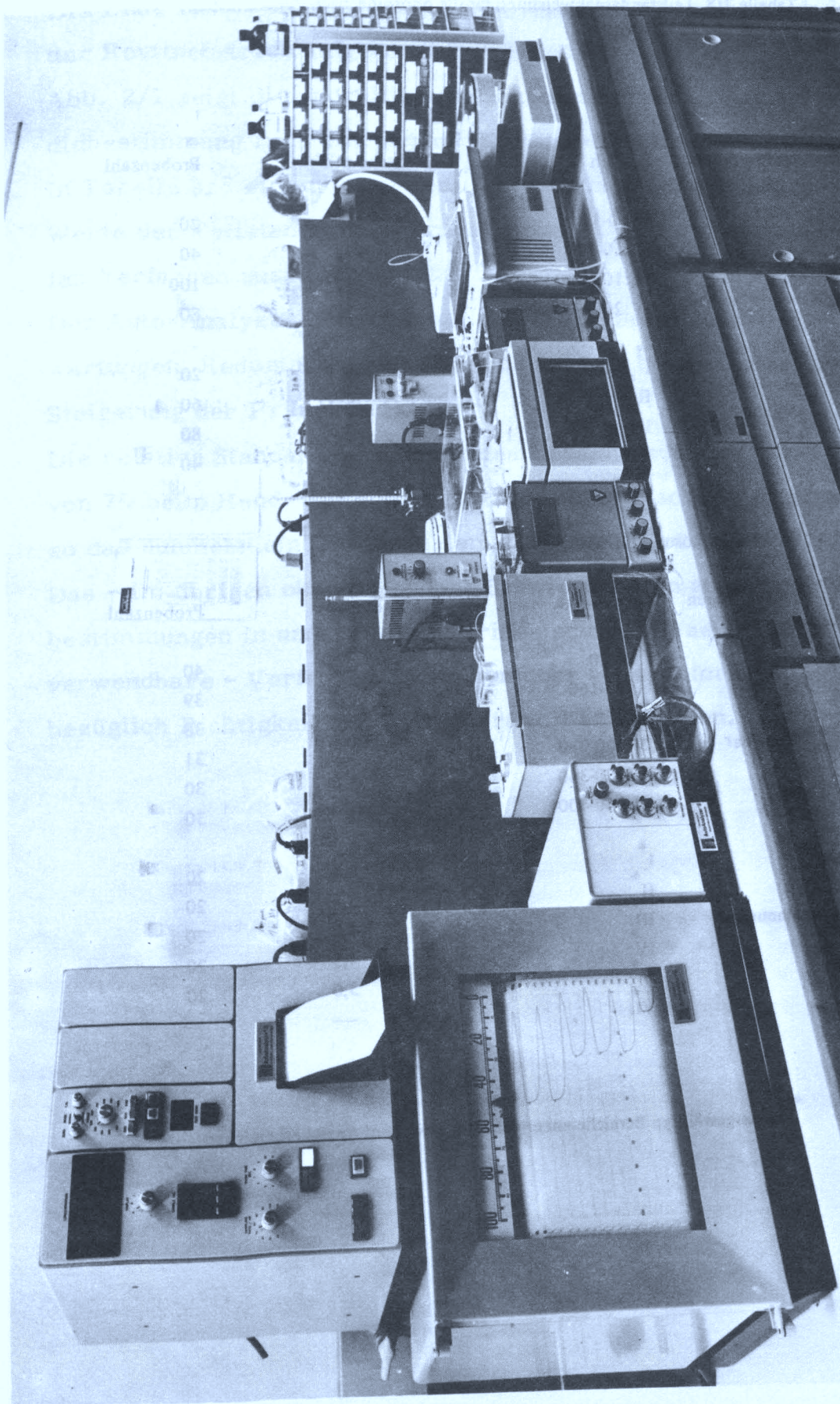
Abb. 1 Automatisierter Meßplatz zur Jod-Analyse der Gras- und Filterproben
